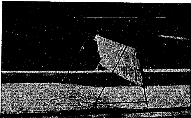
写真—3.5 75 型吹き払い柵の防雪効果，風洞模型実験，向つて右が風下側
