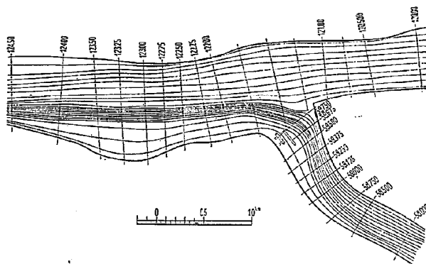
図-29 C-2-II 10,000 m³/s 流線
