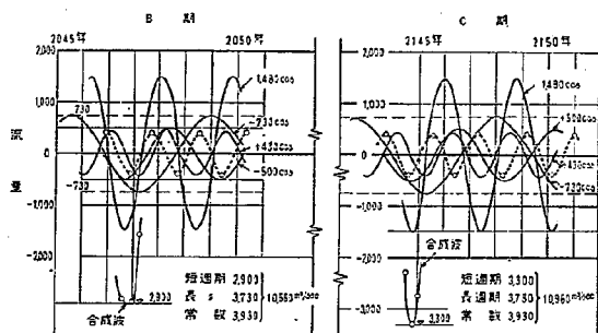
図—19 栗橋洪水流量の短週期の波の合成
