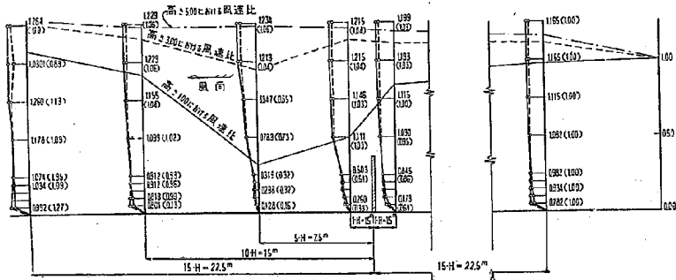
図-2.13 HS-150 型透過柵の防风効果, 現地実験, 10 分間平均風速比分布
