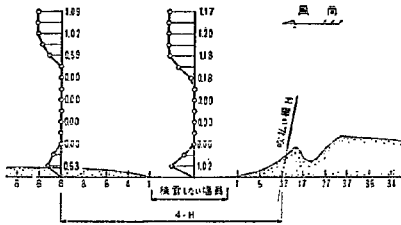
図-3.11 傾斜角度 80° の効果, 基準平均風速 6 m/sec
