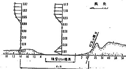
図—3.10 傾斜角度 70^\circ の効果，基準平均風速 6\text{ m/sec}
