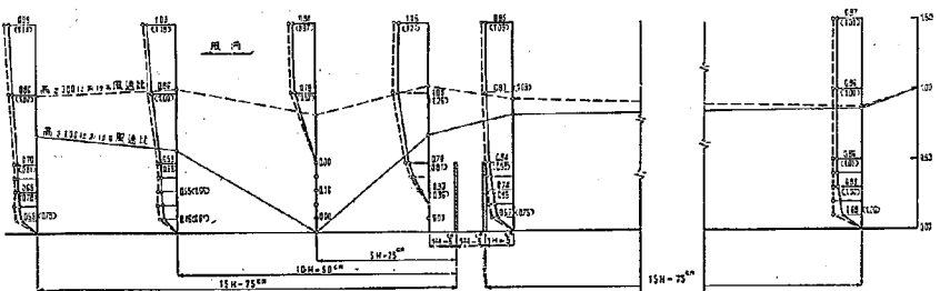
図—2.11 HS—100 2列1段型 (千鳥型) 防風柵の防風効果, 風洞模型実験, 基準平均風速 8 m/sec
