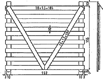
図-2.2 VH-150 型防雪柵透過率 38.0 %
