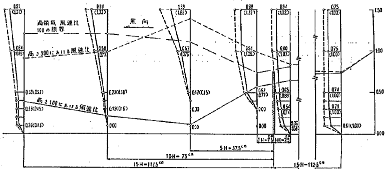
図-2.8 VHS-150型透過柵の防風効果, 風洞模型実験, 基準平均風速 8 m/sec
