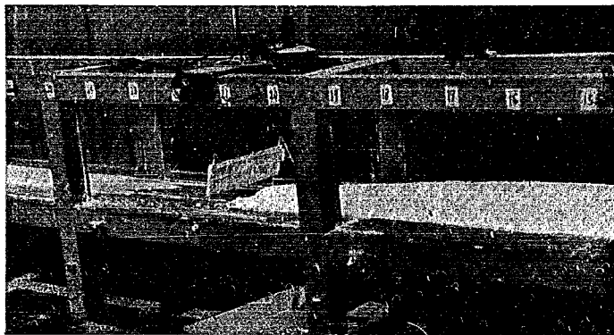
写真—3.4 75 型吹き払い柵の防雪効果，風洞模型実験，向つて左が風下側，柵の真下から風下側附近にかけてきれいに吹払われているのが認められる。
