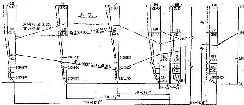
図-2.7 RHS-150型透過柵の防風効果, 風洞模型実験, 基準平均風速 8 m/sec
