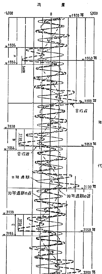
図—18 栗橋洪水流量の99年、33年、11年週期の波の合成
