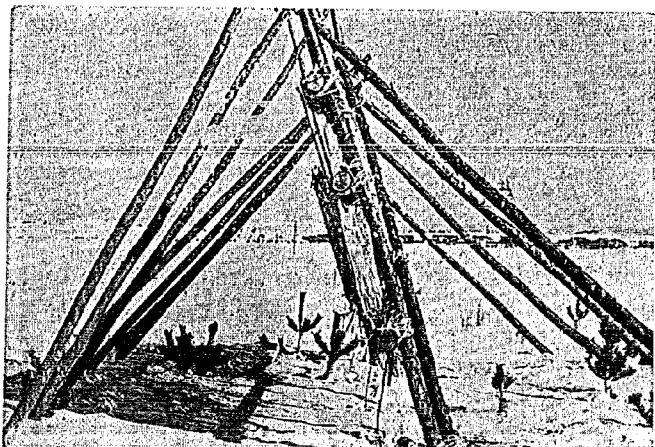
写真—3.9 75 型火払い網の防雪効果，現地実験，向つて右が風下側
