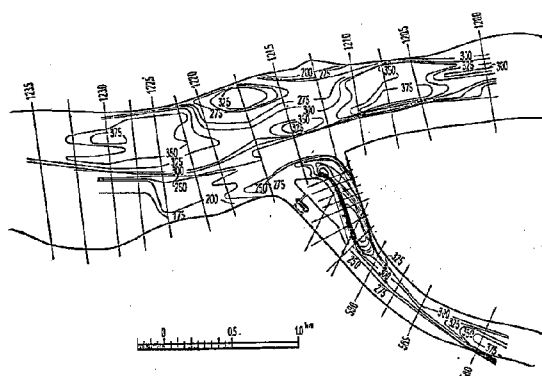
図-9・1 改修中間段階 14,000 m 3 /s 流速分布
