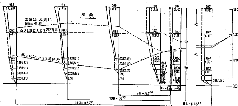
図-2.4 HS-150型透過柵の防風効果, 風洞模型実験, 基準平均風速 4 m/sec
