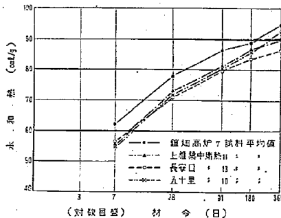
図-2 水和熱比較図
