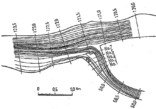
図-10-1 改修中間段階 14,000 m^3/s 流線
