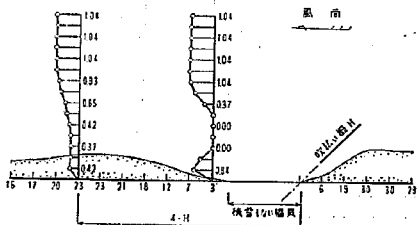
図—3.8 傾斜角度 60^\circ の効果，基準平均風速 6\text{ m/sec}
