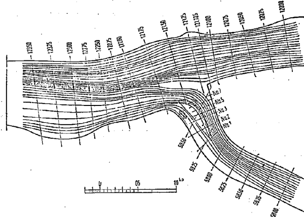
図-20 決定案 14,000 流域
