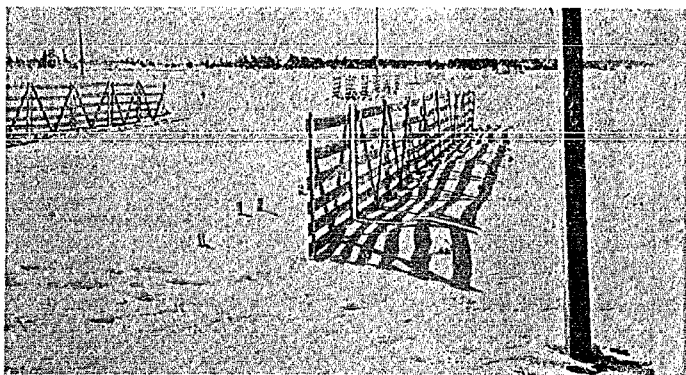
写真—2.11 HS-100 2 段型透過柵の防雪効果，現地実験，向つて右が風上側
