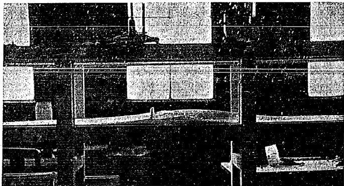
写真—2.5 UHS-150 型透過柵の防雪効果，風洞模型実験，向って右が風下側，柵の風下側の吹溜りのすそは 15 \cdot H 附近の距離までのびている。
