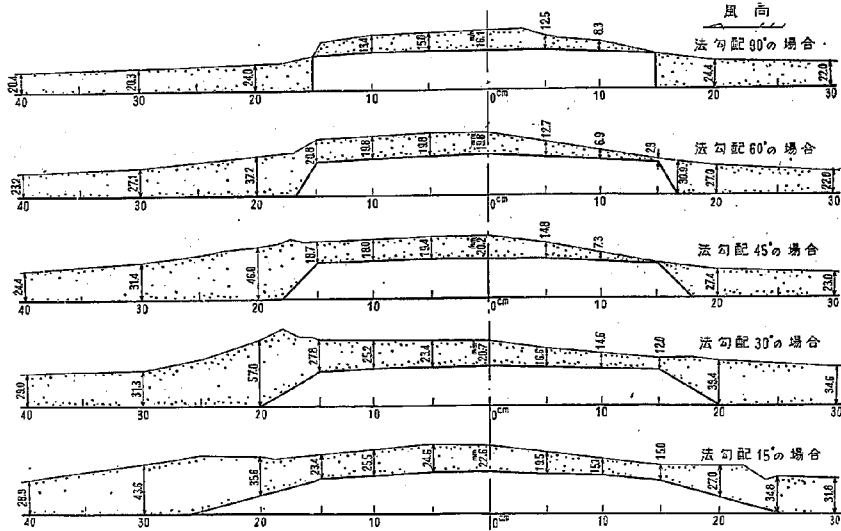
図-5.1 盛土路面形状の防除雪効果
