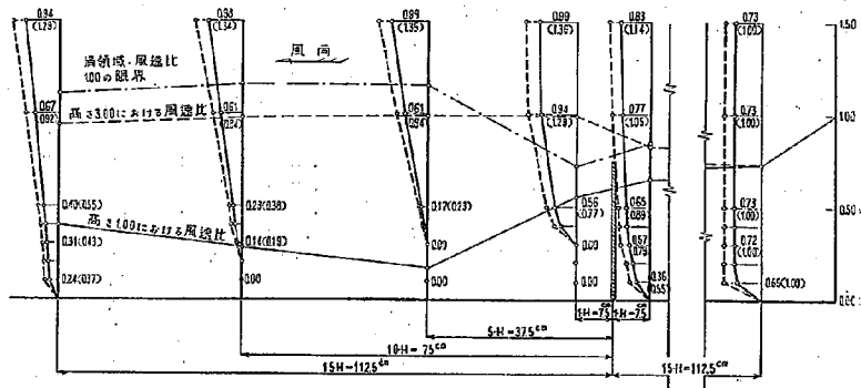
図-2.5 HS-150型透過柵の防風効果, 風洞模型実験, 基準平均風速 8 m/sec
