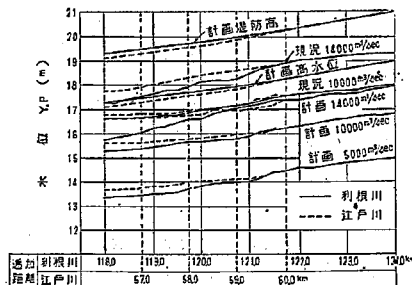
図-22 決定案における水位曲線
