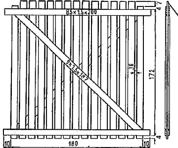
図-2.3 VS-180 型防雪柵透過率 28.5 %
