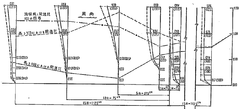
図-2.6 HS-150型透過柵の防風効果, 風洞模型実験基準平均風速 12 m/sec
