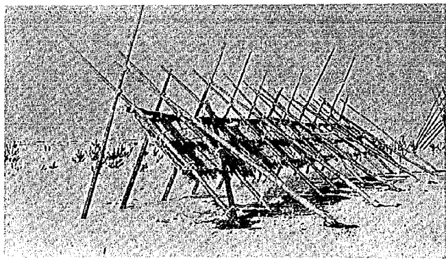
写真—3.8 45 型吹払い柵の防雪効果，現地実験，向つて右が風下側
