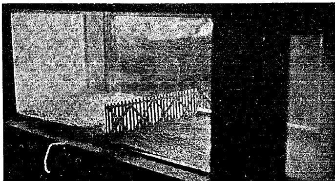
写真—2.6 VS-180 型透過柵の防雪効果，風洞模型実験，向って右が風下側
