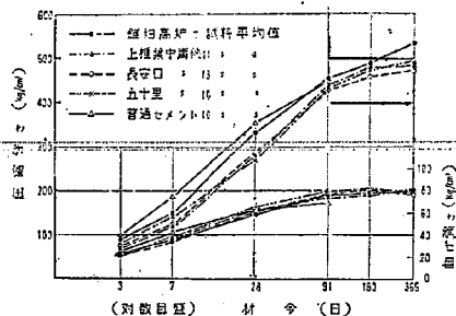
図-1 曲げおよび圧縮強さ比較
