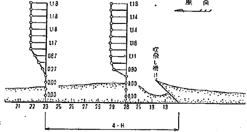
図-3.16 傾斜角度 135° の効果, 基準平均風速 6 m/sec
