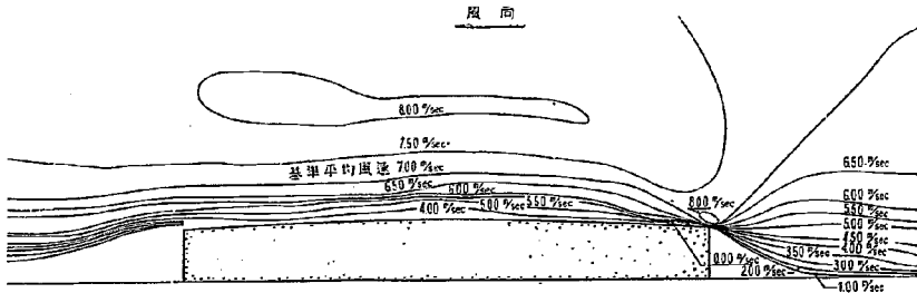
図-5.2 法勾配 90° の場合の風速分布
