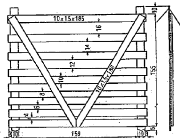
図-2.1 HS-150 型防雪柵透過率 38.0 %
