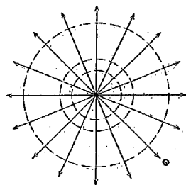
図4(a) 3次元のすいこみとわき出し
