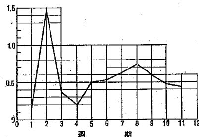
図-4 各週期のフーリエ係数その1
