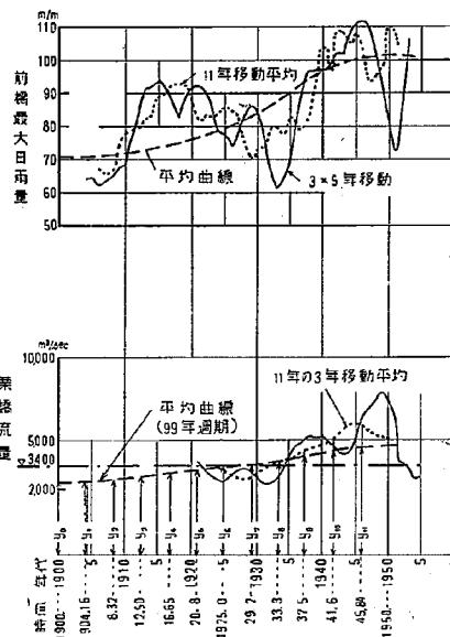
図一16 前橋最大日雨量と栗橋流量
