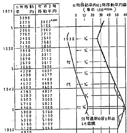
図一14 要橋流量の11年移動平均の3年移動平均
