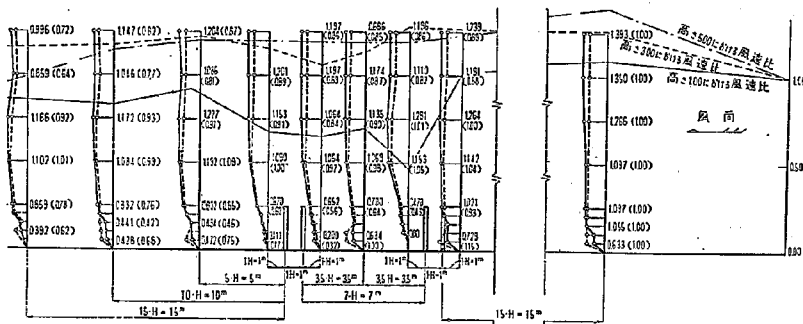
圖—2.18 HS—100 2列2段型透過網の防風効果，現地実験，5分間平均風速比分布
