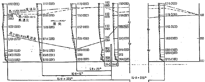
図-2.14 RHS-150 型透過柵の防雪効果, 現地実験, 10 分間平均風速比分布
