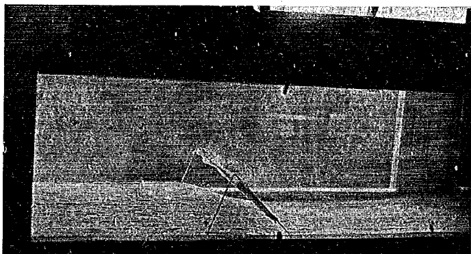
写真—3.1 45型吹払い柵の防雪効果, 風洞模型実験, 向つて右が風下側
