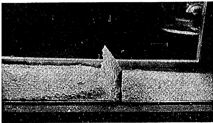
写真—2.7 VS-180 型透過柵の防雪効果，風洞模型実験，向って左が風上側
