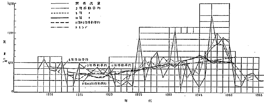
図—11 栗橋流量
