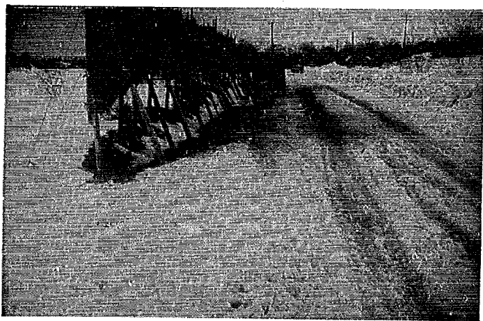
写真—3.10 1 級国道 7 号線（秋田県山本郡浅内村寒川）において火払い網が設立されている状況
