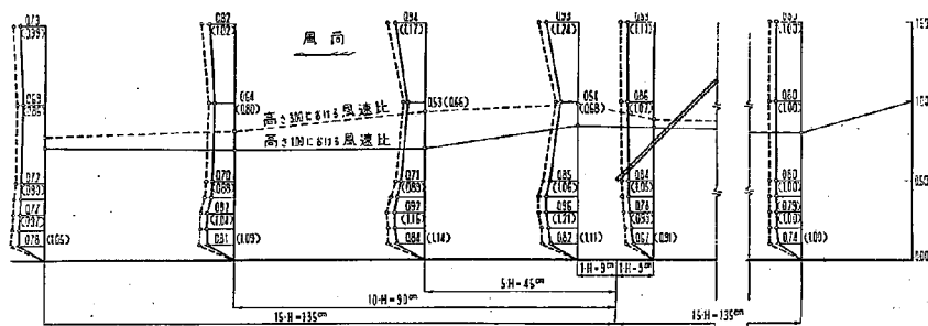
図—3.1 45 型吹き払い柵の防風効果, 風洞模型実験, 基準平均風速 8 m/sec
