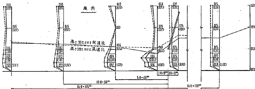
図—3.2 75 型吹き払い柵の防風効果, 風洞模型実験, 基準平均風速 4 m/sec
