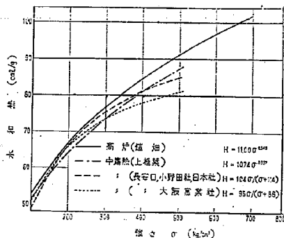
図-3 圧縮強さと水和熱関係
