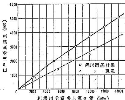
図-23 決定案に於ける流量配分曲線
