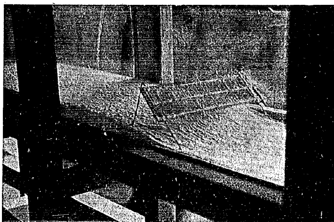
写真—3.2 45型吹払い柵の防雪効果, 風洞模型実験, 向つて右が風下側
