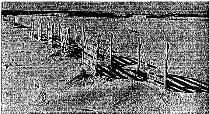
写真—2.13 HS-100 2 列型 (HS-100 千鳥型) 透過柵の防雪効果，現地実験，向つて左が風下側，吹雪の初期における吹溜りの状態その 2
