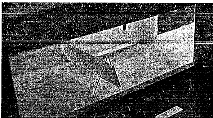
写真—3.6 75 型吹払い柵の防雪効果，風洞模型実験，向つて右が風下側，ここでも柵の真下から風下側附近にかけてきれいに吹払われているのが認められる。
