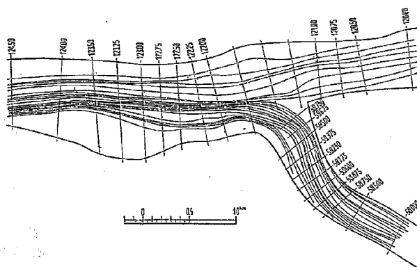
図-30 C-2-II 5,000 m³/s 流線
