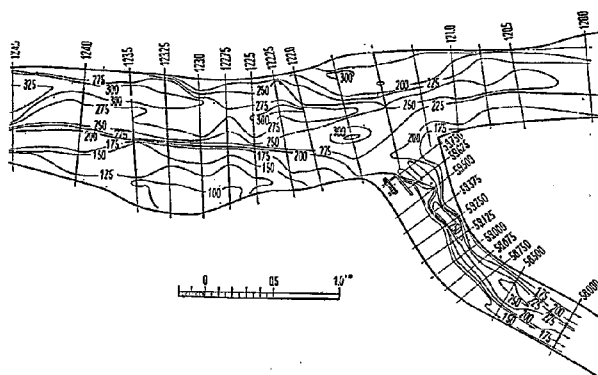
図-26 C-2-II 流速分布 10,000 m³/s
