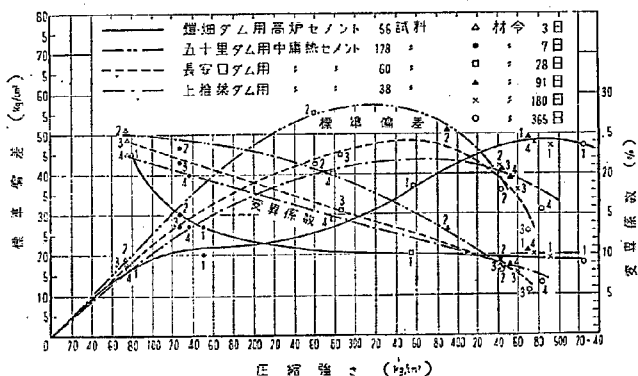
図-4 圧縮強さと標準偏差変異係数の関係
