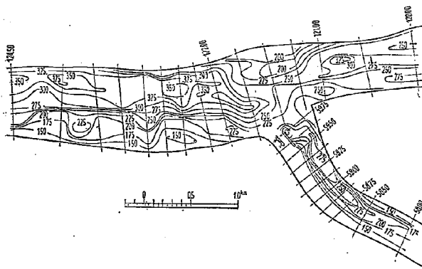
図-31 C-3-II 流速分布
