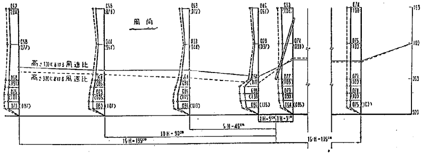
図—3.4 76型段払い柵の防風効果, 風洞模型実験, 基準平均風速 12 m/sec
