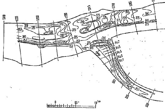
図—7・1 現況—14,000 \text{m}^3/\text{s} 流速分布
