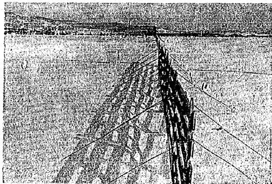
写真—2.10 RHS-150 型透過柵の防雪効果，現地実験，向つて左が風上側，吹雪の初期においてはまず風上側の柵近くに吹溜りが発生することが，柵の影の歪みで認められる。
