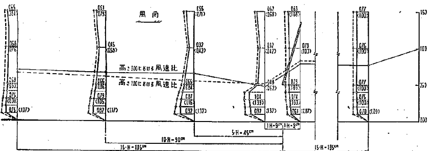
図—3.3 75 型吹き払い柵の防風効果, 風洞模型実験, 基準平均風速 8 m/sec
