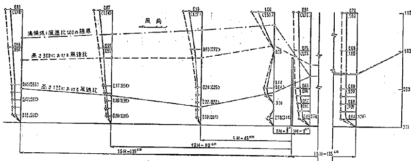
図—2.9 VS—180型透過柵の防風効果, 風洞模型実験, 基準平均風速 8 m/sec
