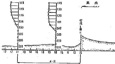
図-3.13 傾斜角度 90° の効果, 基準平均風速 6 m/sec
