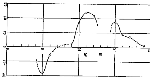
図-10 前橋最高日雨量の週期性向；フーリエ係数
