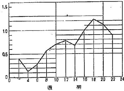
図—5 各週期のフーリエ係数その2
