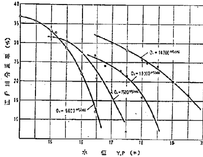
図—5 水位分流率相関図
