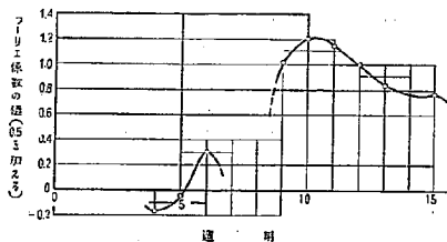
図—13 栗橋流量の週期検定
