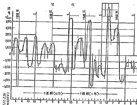
図-17 栗橋流量より 99 年、33 年週期の波を取除いたもの
