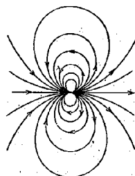
図4(b) 3次元の2重わき出し
