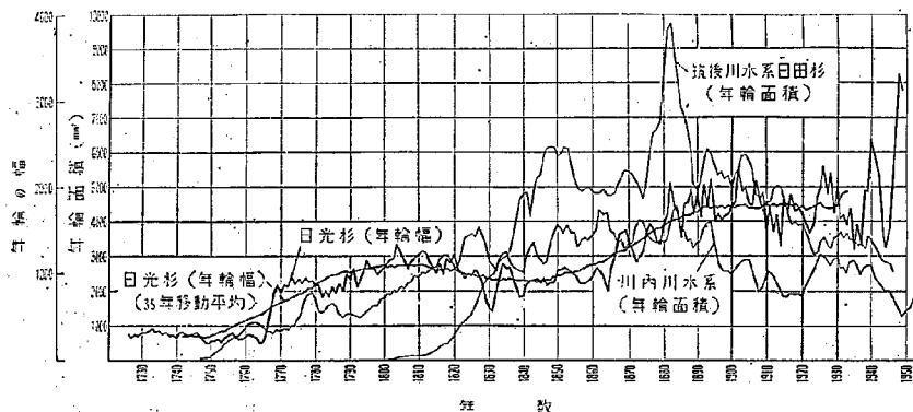
図-1 杉の年輪成長率図 (3年移動平均)
