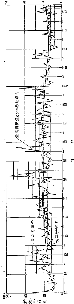
図—7 京城最大月雨量、同3年移動平均および35年移動平均
