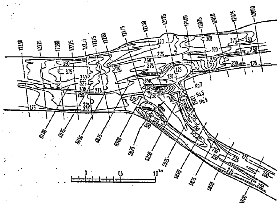
図-17 B-Ⅲ 14,000 m³/s 流速分布
