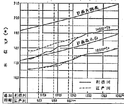
図—6 現況水位図
