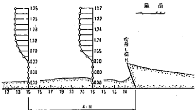
図-3.14 傾斜角度 110° の効果, 基準平均風速 6 m/sec
