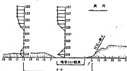
図—3.9 傾斜角度 45^\circ の効果，基準平均風速 6\text{ m/sec}
