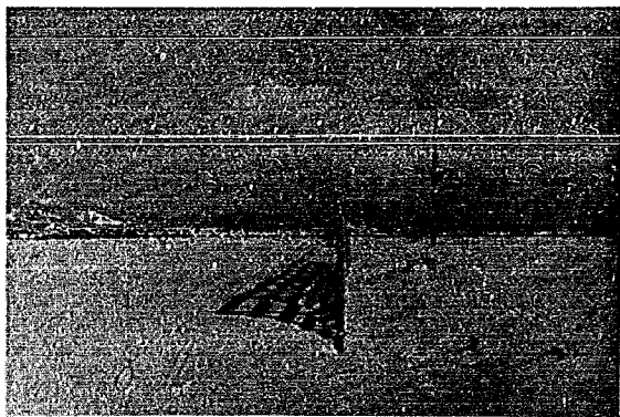
写真—2.8 HS-150 型透過柵の防雪効果，現地実験，向つて左が風上側，吹雪の初期においてはまず風上側の附近に吹溜りが発生することが，柵の影の歪みで認められる。
