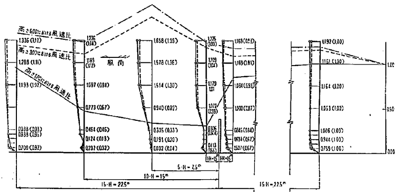
図—2.15 VHS—150 型透過柵の防風効果，現地実験，10 分間平均風速比分布
