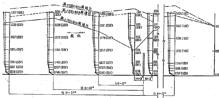
図—2.16 VS—180 型透過柵の防風効果，現地実験，10 分間平均風速比分布
