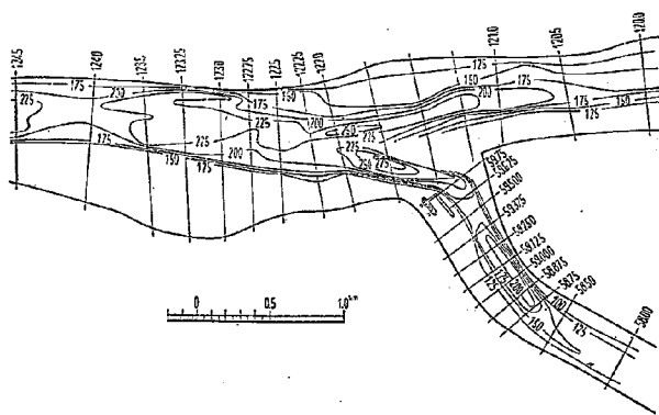
図-27 C-2-II 流速分布 5,000 m³/s
