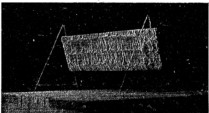
写真—3.7 75 型吹払い柵，風洞模型実験，実験中吹雪流のなかの模型雪（炭酸マグネシウム）が柵に附着して実感を与える。
