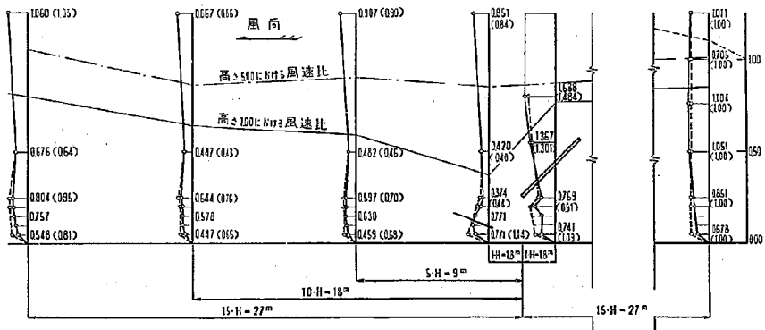
図—3.5 45型吹払い柵の防風効果, 現地実験, 5分間平均風速比
