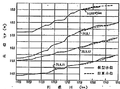
図-4 利根川水位図
