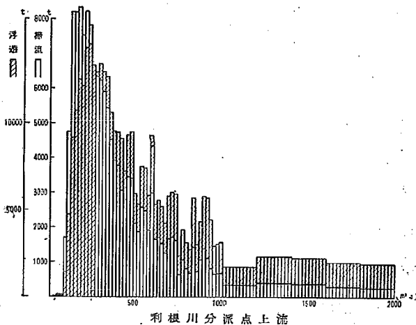
図—38 改修案に於ける年間流砂量、流量相関図
