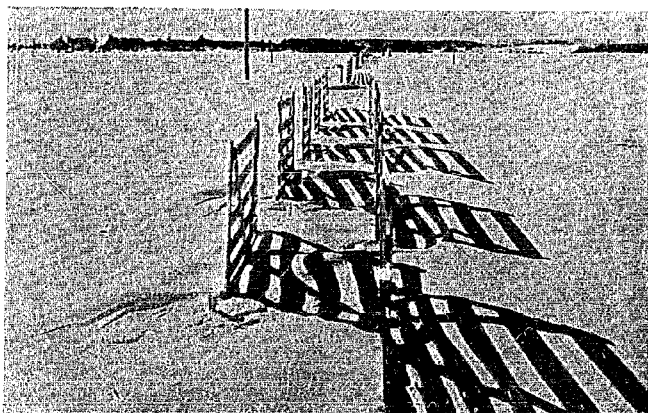
写真—2.12 HS-100 2 列型 (HS-100 千鳥型) 透過柵の防雪効果，現地実験，向つて右が風上側，吹溜りの初期における吹溜りの状態その 1
