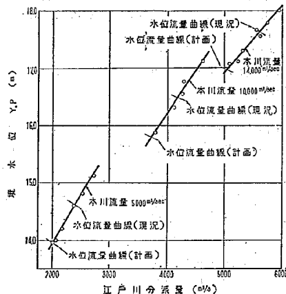
図-24 決定案に於ける境界水位及分派量相関図
