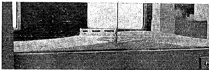
写真—2.2 HS-150 型透過柵の防雪効果, 風洞模型実験, 向つて右が風下側, 柵の風下側の吹溜りのすそは 15 \cdot H 附近の距離までのびている。
