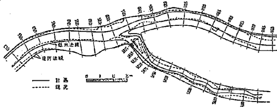
図-21 決定案 平面図
