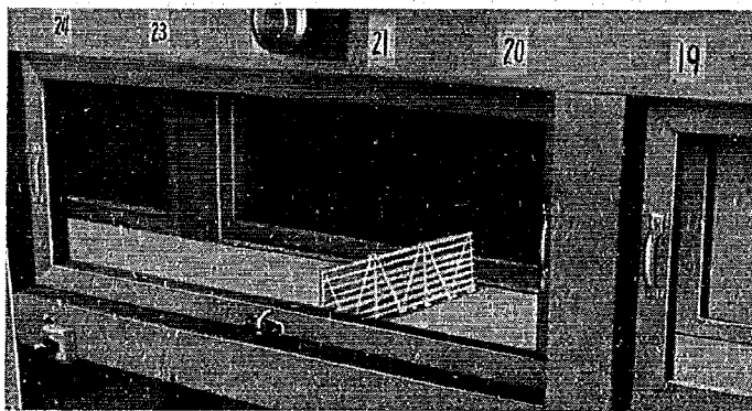
写真—2.4 UHS-150 型透過柵の防雪効果, 風洞模型実験, 向つて左が風下側, 吹雪の初期においては柵の風下側近くには吹溜らないのが認められる。
