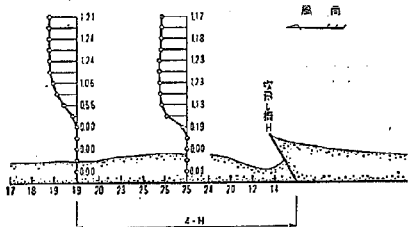
図-3.15 傾斜角度 120° の効果, 基準平均風速 6 m/sec
