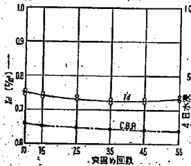
図—20 Over-Compaction と Remoulding 附影響
