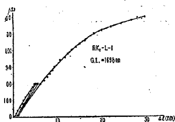
図-24. 鋼索Lの維持荷重試験(II)の P \sim \Delta l 線図
