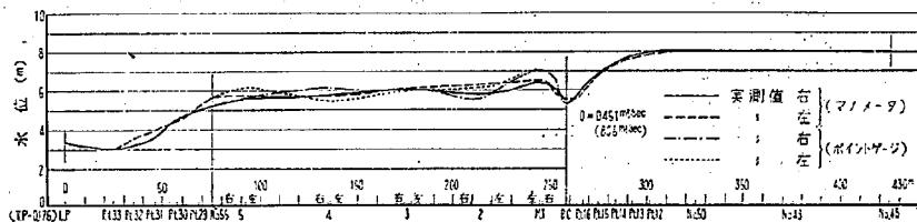
図-22 トンネル内水位 (入口原案)
