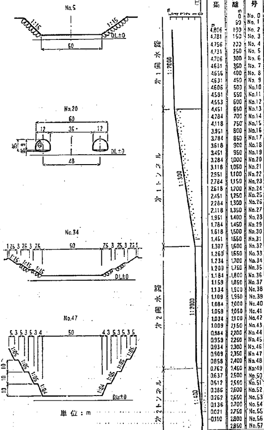
図-1 放水路縦断面形、開水路、トンネル部横断面形(当初計画案)
