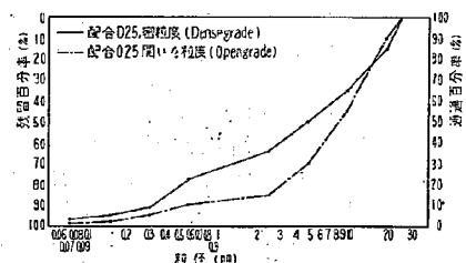
図-1 最大粒径 25mm, アスファルトコンクリート骨材粒度
