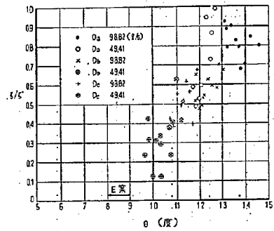
図-31 形状損失係数と \theta との関係
