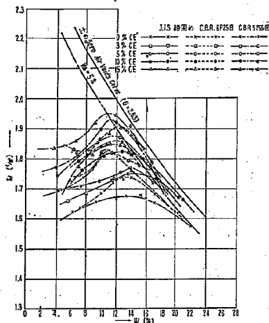
図—5 締固めエネルギーとその結果試料「名一神」千里山 (試料 No. 7)
