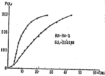
図—14. 鋼索RAの繰返引張試験 P \sim \Delta L 線図
