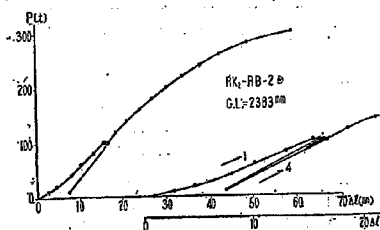
図-20. 鋼索RBの維持荷重試験(II)の P \sim \Delta l 線図
