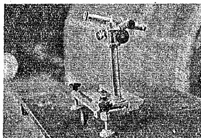
(a) 固定側
