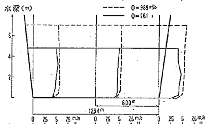
図-23 トンネル内水位(入口改良)
