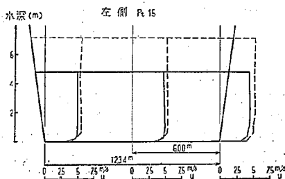
図-24 トンネル入口の流速分布
