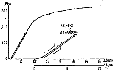
図-4. 鋼索Pの維持荷重試験(I)の P \sim \Delta L 線図
