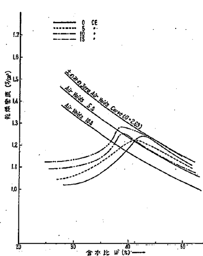
附圖-1 (1) セメント安定材が締固め結果に及ぼす効果
