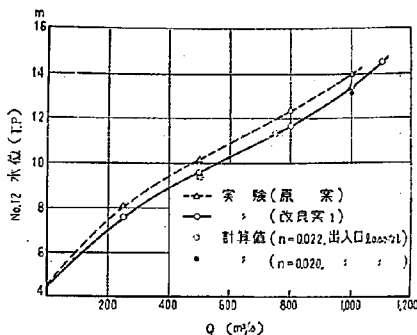
図-8 No. 12 における水位流量曲線
