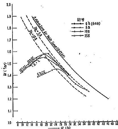
図—4 (2) セメント系材料の締固め結果に及ぼす影響
