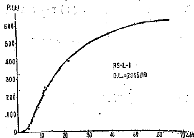
図-21. 鋼索Lの単引張試験の P \sim \Delta l 線図
