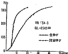
図-7. 鋼索SAの繰返引張試験の P \sim \Delta L 線図
