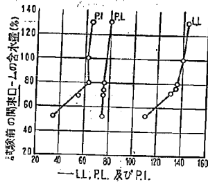
図—19 関東ローム (試料 No.17) の試験前含水量による L, L.P.I. の變化
