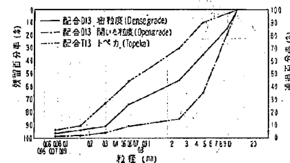
図-2 最大粒径 12.7mm, アスファルトコンクリート骨材粒度
