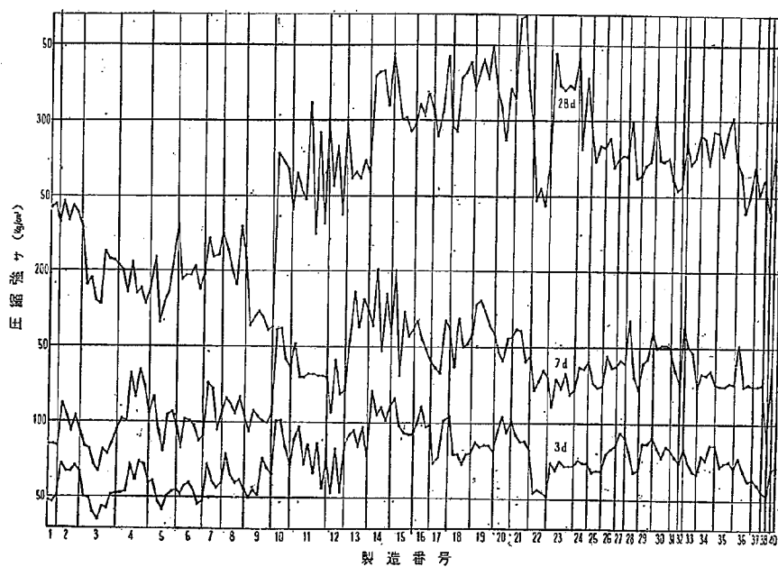
図-5 圧縮強サの推移
