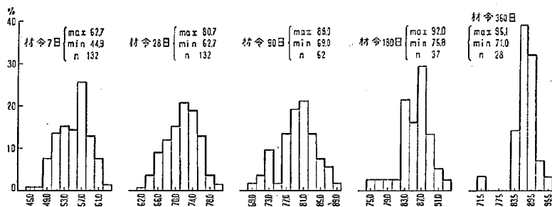
図-3 水和熱測定値の分布図
