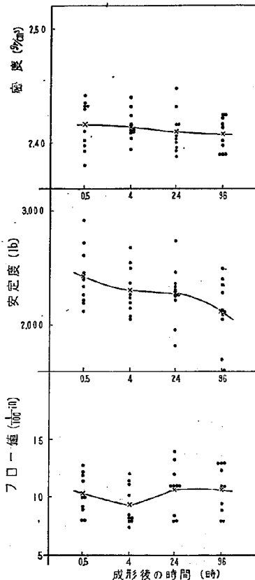
図-7 成型後の時間と安定度の関係(配合 D25, ストレートアスファルト I)
