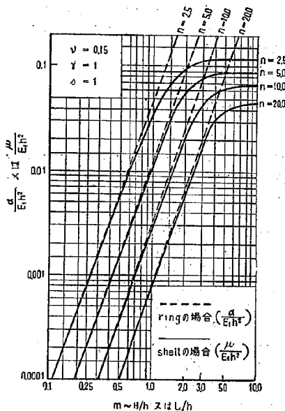
図-5 \frac{\alpha}{E_1 h^2} または \frac{\mu}{E_1 h^2} と m との関係の 1 例
