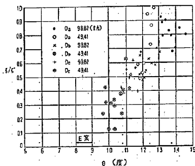
図-31 形状損失係数と \theta との関係
