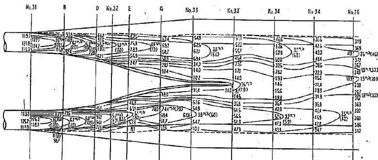
図-13 流速分布 ( E_a 案)
