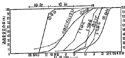
図-3 砂、砂利、碎石などの分け結果
