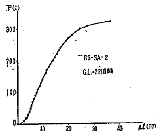
図-6. 鋼索SAの単純引張試験の P \sim \Delta L 線図
