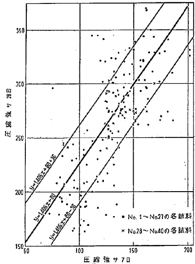
図-7 \sigma_7 と \sigma_{28} との関係
