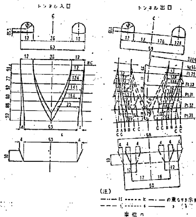
図-5c 第2トンネル入口出口
