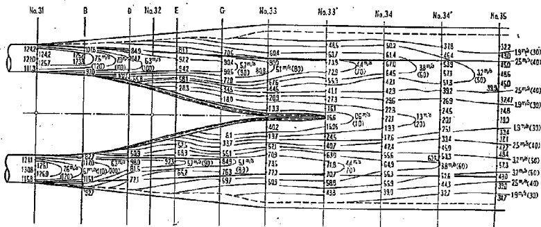
図-12 流況図 ( E_a 案)
