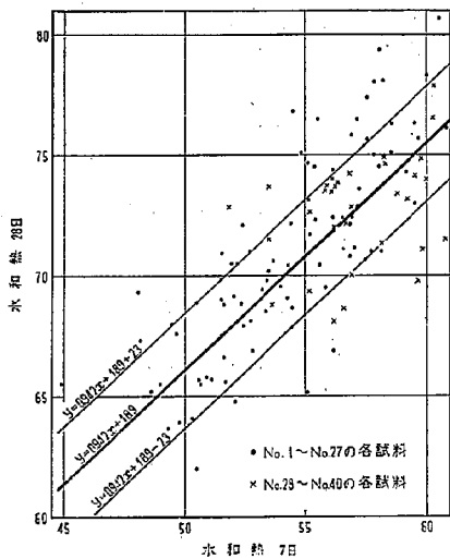
図-8 H_7 と H_{28} との関係
