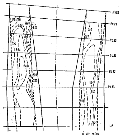
図—21 平面流速分布 (C案)
