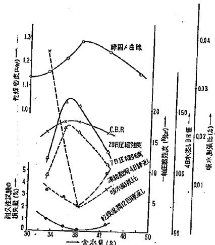
図—25 安定度と耐久性との関係、炭手大灰質、粘土質ローム A-7-6 (20) LL=64 PI=31 o.m.c.=38.4\% セメント 15%
