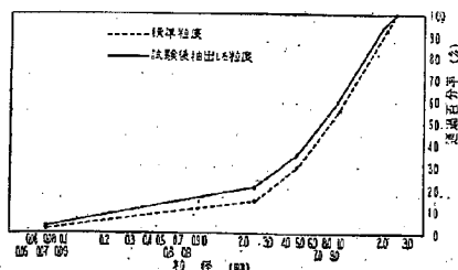
図-11 開いた粒度配合 O25 を用いた混合物の骨材破砕状態
