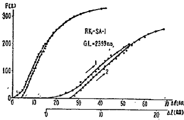
図—8. 鋼索SAの維持荷重試験(I)の P \sim \Delta L 線図
