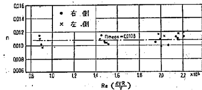
図-7a 粗度係数 \sim R_e (第1トンネル)
