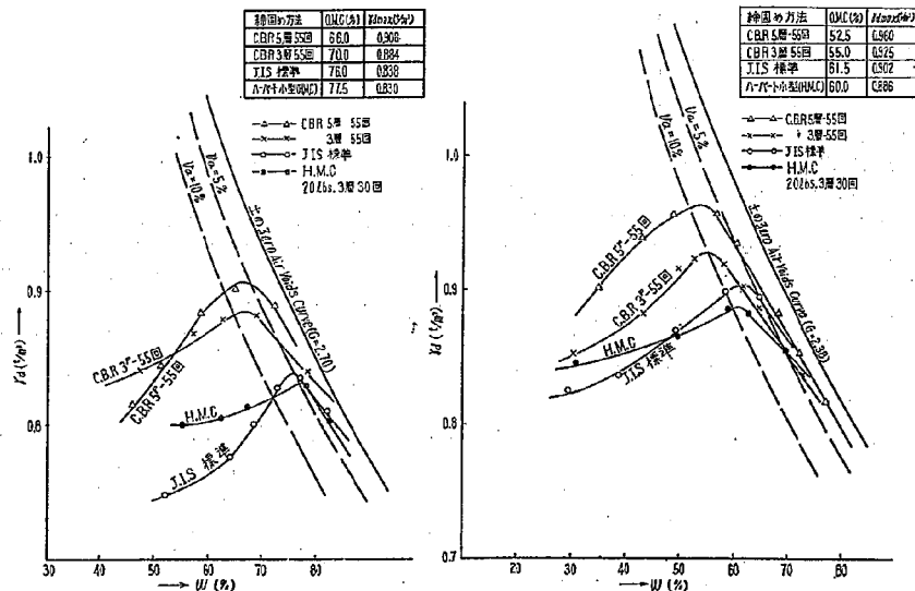
図-1 (1) 締固め結果の比較、試料南部国道黒ボク (試料 No. 18)
