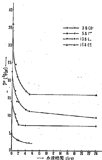
図-14 水浸時間とソイル・セメントの単軸圧縮強度との関係
