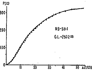
図—9. 鋼索SBの単純引張試験 P \sim \Delta L 線図
