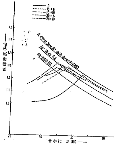
(試料=南国道典中山ローム (試料 No. 12) (締固め=ハーバード小型, 20 lbs, 3 尺, 30 回) 附図—1 (5) 「四磷酸ナトリウム」が締固め結果に及ぼす影響
