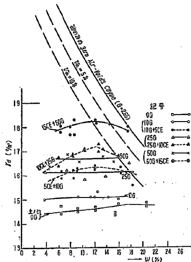
図-6 粒度の悪い砂または「砂-砂利」混合物の締固め結果
