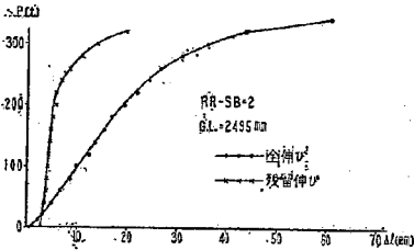
図—10. 鋼索SBの繰返引張試験 P \sim \Delta L 線図
