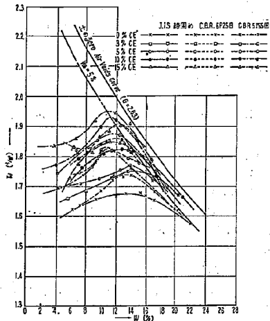
図—5 締固めエネルギーとその結果試料「名一神」千里山 (試料 No. 7)
