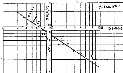
図-2(a) 狩野川大仁地点の貯留関数 (昭. 27. 6. 24. 洪水, I=Q_i と考えた場合)
