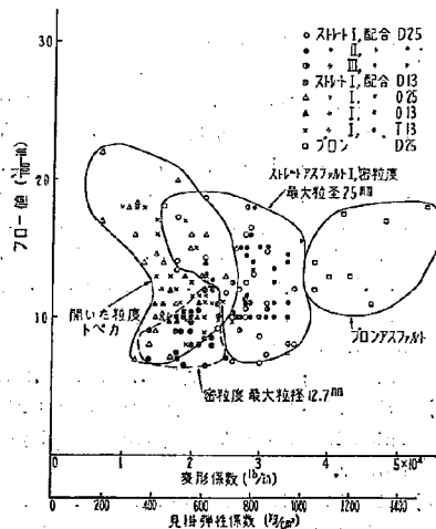
図-17 見掛弾性係数 (変形係数) とフロー値の関係
