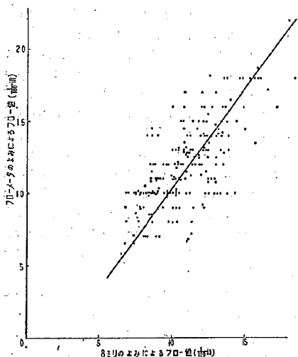
図-15 フロー値の比較
