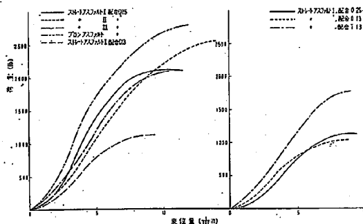
図-14 アスファルト混合物の種類と荷重-変位曲線
