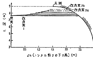
図-3 天端余裕高比較図
