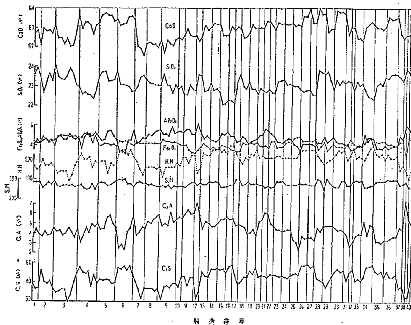
図-4 化学組成の推移
