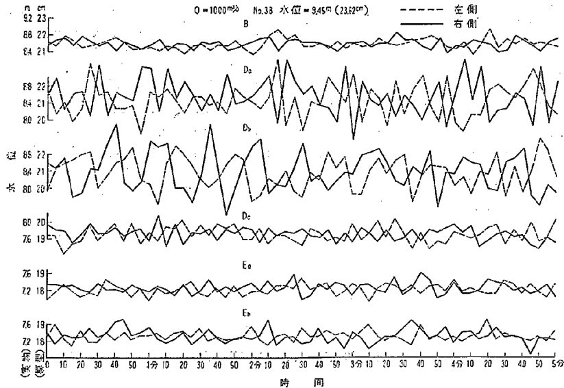
図-10 第1トンネル出口水位振動図
