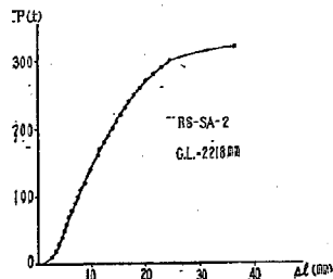
図-6. 鋼索SAの単純引張試験の P \sim \Delta L 線図
