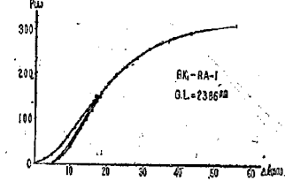
図—15. 鋼索RAの維持荷重試験(I) P \sim \Delta L 線図
