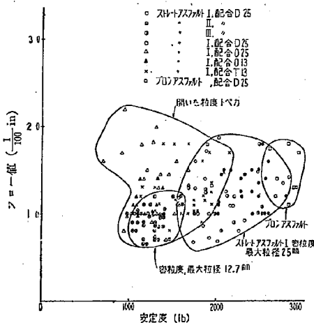
図-18 安定度とフロー値の関係
