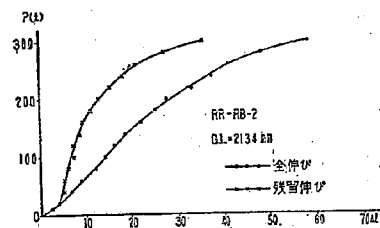
図-18. 鋼索RBの繰返引張試験の P \sim \Delta l 線図
