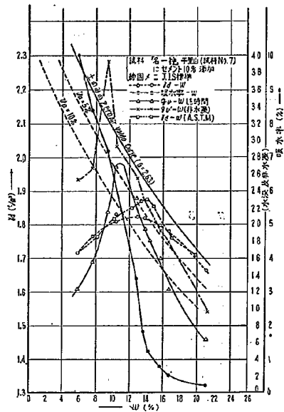
図-9 試料「名神」千里山 (試料 No. 7)
