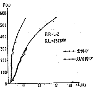
図-22. 鋼索L繰返引張試験 P \sim \Delta l の線図
