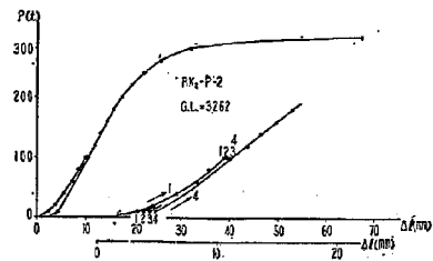
図-5. 鋼索Pの維持荷重試験(II)の P \sim \Delta L 線図
