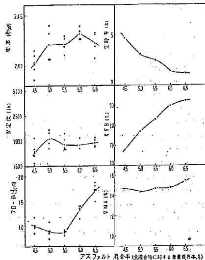
図—5 標準混合物 (配合 D25, ストレートアスファルト I) に対するマーシャル安定度試験結果
