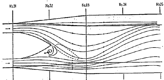
図-9 流況図 (原案)
