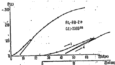
図-20. 鋼索RBの維持荷重試験(II)の P \sim \Delta l 線図
