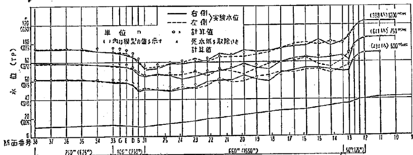
図-15 計算値と実験値の比較
