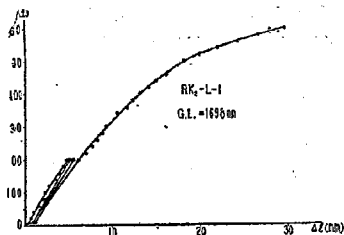
図-24. 鋼索Lの維持荷重試験(II)の P \sim \Delta l 線図
