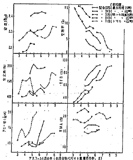
図-12 骨材の粒度と安定度試験値
