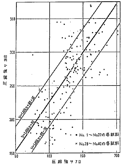
図-7 \sigma_7 と \sigma_{28} との関係
