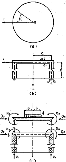
図-3 周辺が有限長の円筒殻に弾性固定されている円版
