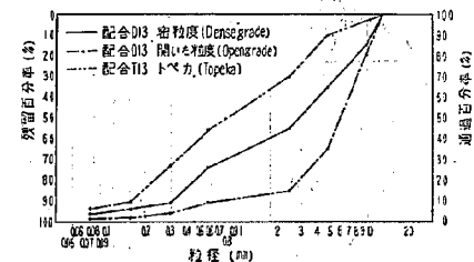
図-2 最大粒径 12.7mm, アスファルトコンクリート骨材粒度
