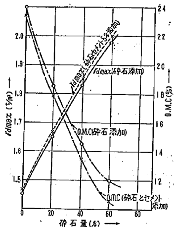
図-7 砕石混合率と r_{dmax} o.m.c の関係 2) 砂、砂利、砕石などの影響
