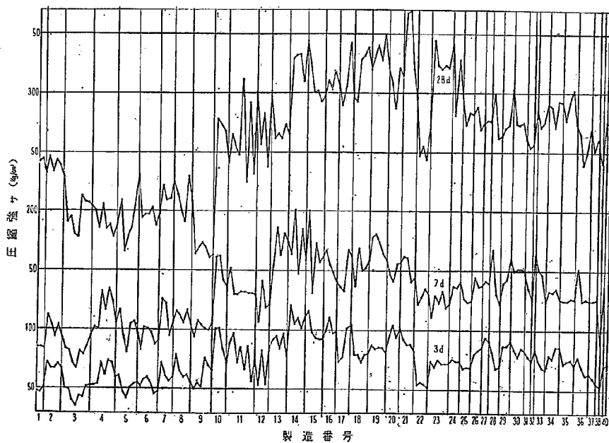
図-5 圧縮強サの推移
