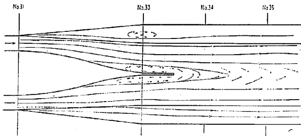
図-12 流況図 ( E_a 案)
