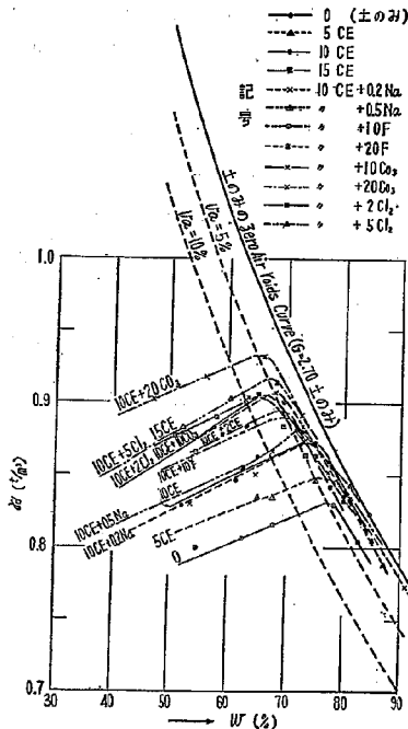
図—4 (1) セメント系材料の締固め結果に及ぼす影響
