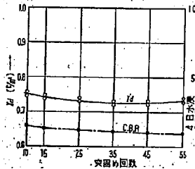
図—20 Over-Compaction と Remoulding の影響
