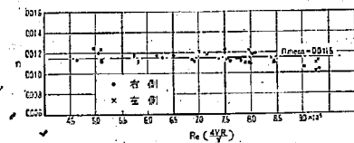
図-7b 粗度係数 \sim R_e (第2トンネル)
