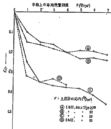
図—17 各試験路盤の荷重分散効果
