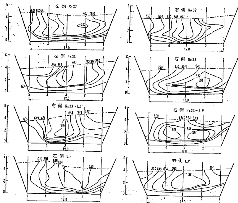
図—20 横断面内の流速分布 (C案)
