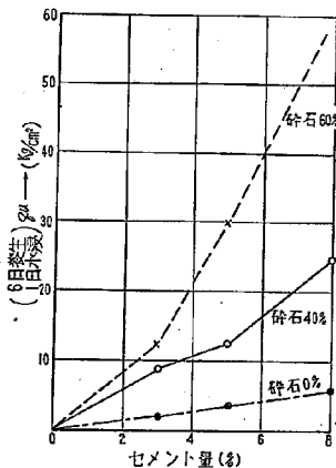
図—11 ソイル・セメントの安定度にはらず砕石の影響 試料 関東四号国道、砂(試料No.3) J.I.S 標準締固めの最適条件
