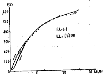
図-23. 鋼索Lの維持荷重試験(I)の P \sim \Delta l 線図
