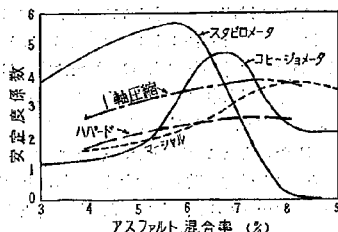
図-8 各安定度試験の鋭敏度
