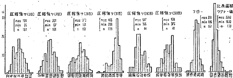
図-2 圧縮強サ, フロー値および比表面積値の度数分布図
