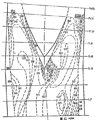
図—17 平面流速分布 (A案)
