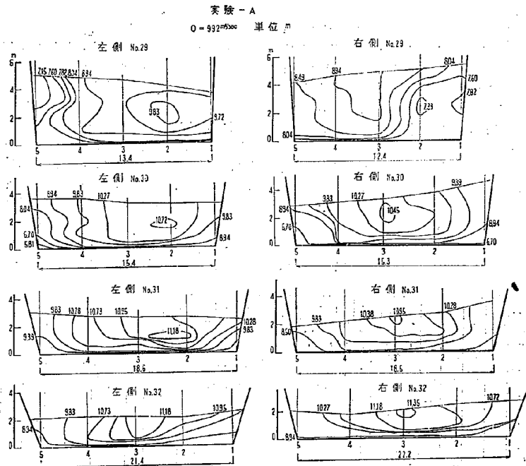
図-16 横断内の流速分布 (A案)
