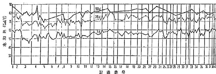
図—6 水和熱の推移
