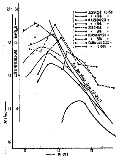
試料「関東四号」砂 (試料 No. 2)
