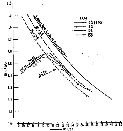
図—4 (2) セメント系材料の締固め結果に及ぼす影響
