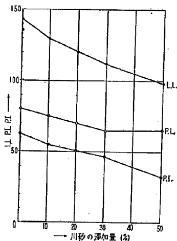
図—24 砂の添加量による L.L.P.I. の変化。試料に關東ローム (試料 No.17)
