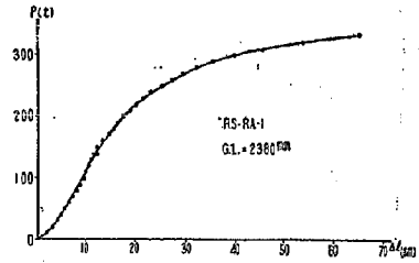
図—13. 鋼索RAの単純引張試験 P \sim \Delta L 線図
