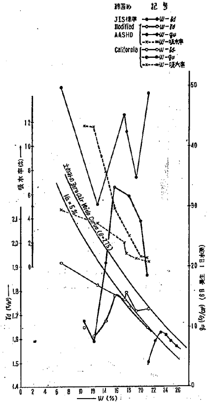
試料=即山国道 (試料 No. 9) にセメント 5% 添加 附図—2 締固め含水量, 強度, 吸水率の関係
