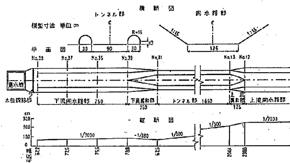
図-4a 第1トンネル模型平面図
