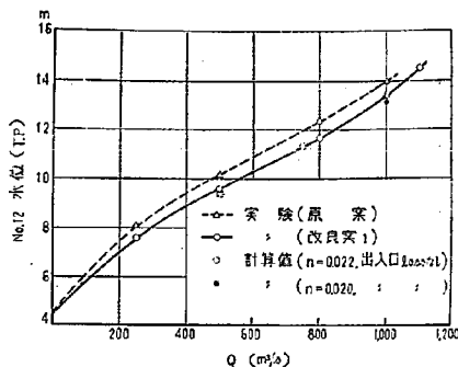
図-8 No.12 における水位流量曲線
