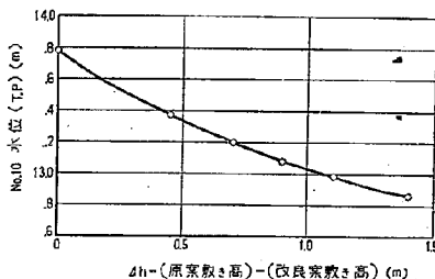
図-2 改良案Ⅰにおける河床の下り高とトンネル入口部水位の関係
