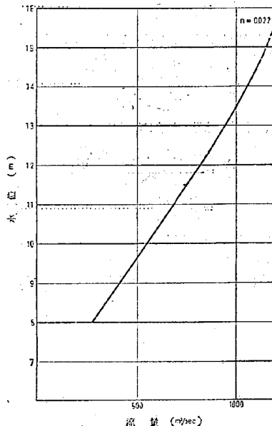
図-28 No. 2断面水位～流量曲線
