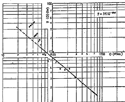
図-1(a) 狩野川大仁地点の貯留関数 (昭. 27. 6. 24. 洪水, I=0 と考えた場合)
