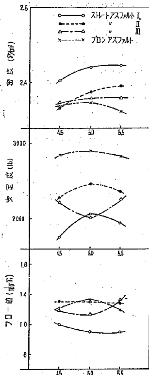
図-10 アスファルトの種類と安定度試験値 (配合 D25)
