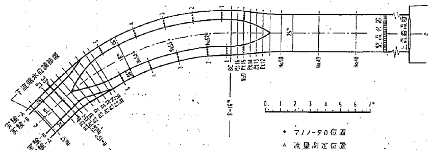
図-4b 第2トンネル模型平面図
