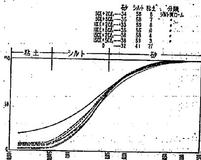
図—18 セメント系材料添加後の粒径加積曲線の1例 (1週間養生後)
