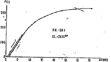
図—11. 鋼索SBの維持荷重試験(I) P \sim \Delta L 線図
