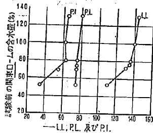
図—19 関東ローム (試料 No. 17) の試験前含水量による L, P, I の変化
