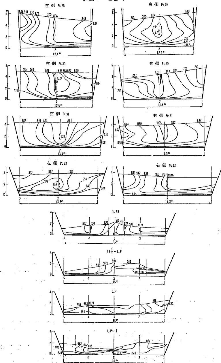
図-18 横断内の流速分布 (B案)
