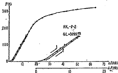
図-4. 鋼索Pの維持荷重試験(I)の P \sim \Delta L 線図
