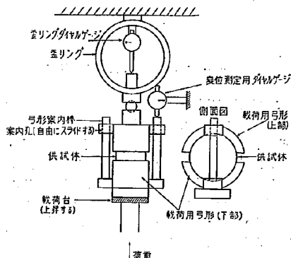
図-13 8 ミリ撮影時の載荷状態
