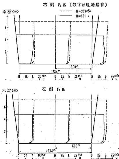
図-24 トンネル入口の流速分布
