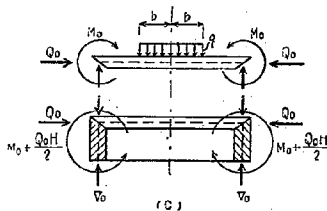
図-4 周辺が円環に弾性固定されている円版
