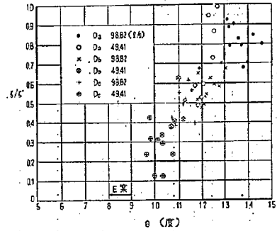
図-31 形状損失係数と \theta との関係
