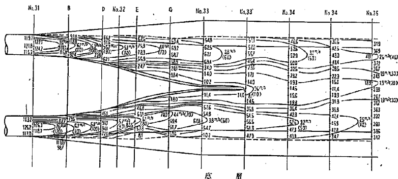
図-13 流速分布 ( E_a 案)
