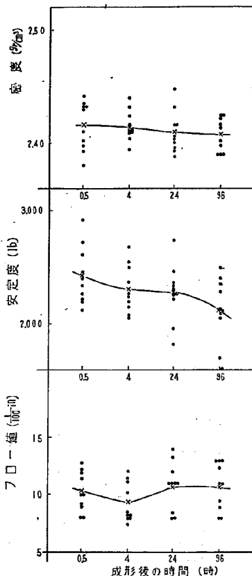
図-7 成型後の時間と安定度の関係(配合 D25, ストレートアスファルト I)
