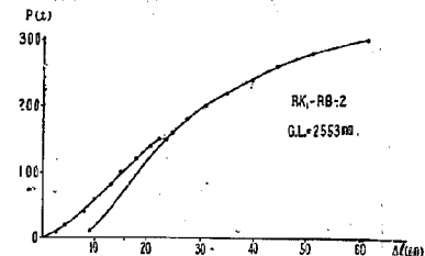
図-19. 鋼索RBの維持荷重試験(I)の P \sim \Delta l 線図
