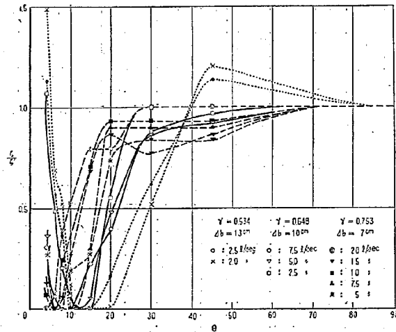
図-32 形状損失係数と \theta との関係 (長方形水路)
