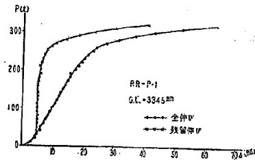
図-3. 鋼索のP繰返引張 P \sim \Delta L 線図
