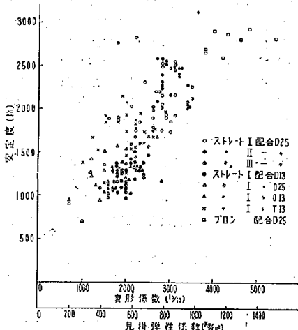
図-16 見掛弾性係数 (変形係数) と安定度の関係
