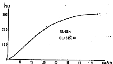
図—17. 鋼索RBの単純引張試験の P \sim \Delta L 線図
