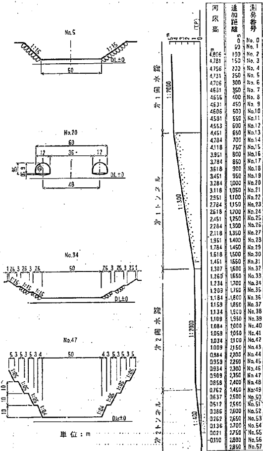
図-1 放水路縦断面形、開水路、トンネル部横断面形(当初計画案)
