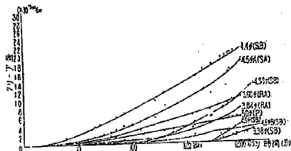
図-1. クリーブ状況
