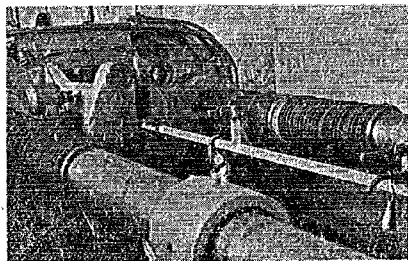
写真-11. 鋼索試験機 (1,000 ton)
