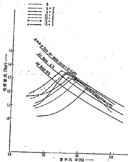
附圖一（1）セメント安定材が締固め結果に及ぼす効果
