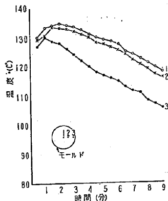
図—4 モールド内の混合物温度
