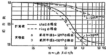
図-6 円版中央部下面に於ける応力比の計算値と実験値
