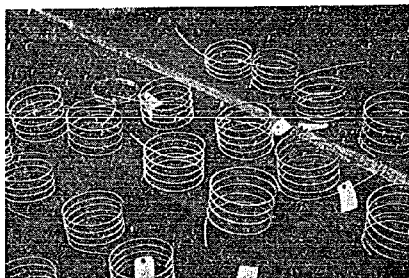
写真-16. 巻付試験片
