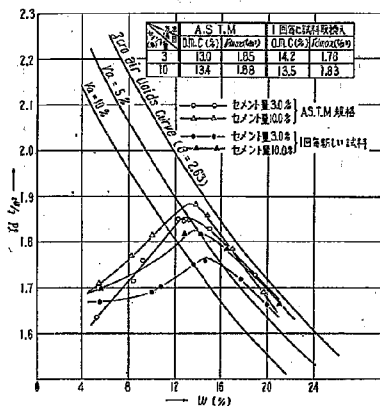
図-8 A.S.T.M. 規格 D558-44 による場合と 1 回毎に新しいソイルセメント試料を使用した場合の締固め結果の相異
