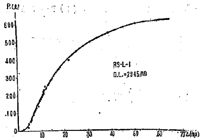
図-21. 鋼索Lの単純引張試験の P \sim \Delta l 線図
