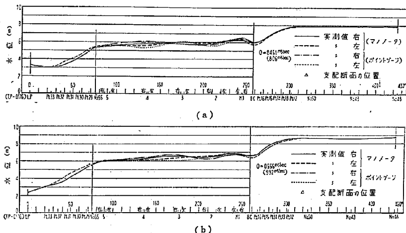
図-23 トンネル内水位 (入口改良)
