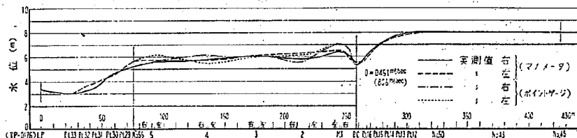
図-22 トンネル内水位 (入口原案)
