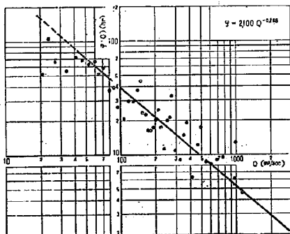
図-2(b) 神流川渡瀬地点の貯留関数 (昭. 24. 8. 31. 洪水, I=Q_i と考えた場合)
