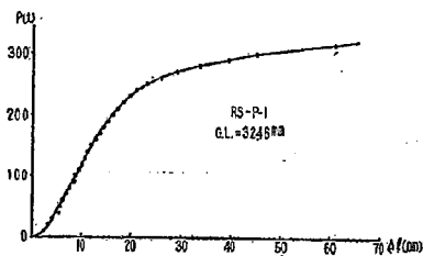
図-2. 鋼索Pの引張 P \sim \Delta L 線図
