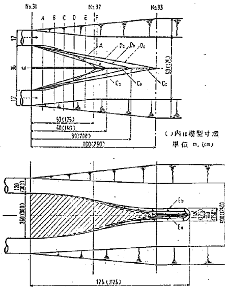
図-5b 第1トンネル入口
