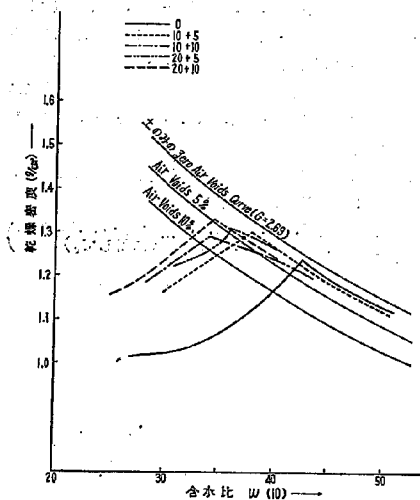
附圖一（4）「フライアッシュと炭酸石灰」が締固め結果に及ぼす影響
