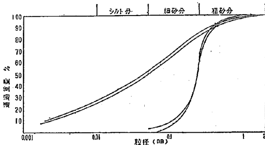
図-4 粒度曲線
