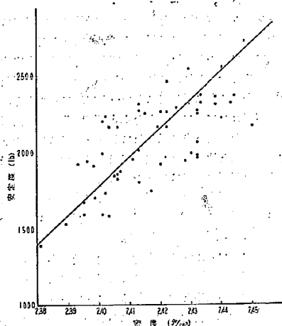
図-9 安定度と密度の関係 (配合D25, ストレートアスファルトI)
