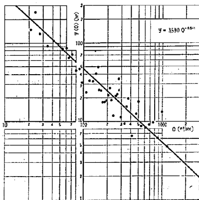
図-1(b) 神流川渡瀬地点の貯留関数 (昭. 24. 8. 31. 洪水, I=0 と考えた場合)
