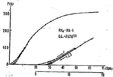
図—16. 鋼索RAの維持荷重試験(II) P \sim \Delta L 線図
