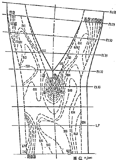
図-19 平面流速分布 (B案)
