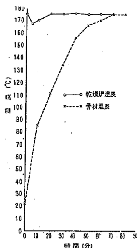
図-3 乾燥炉内の骨材温度
