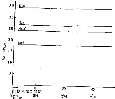
図一2. 第3回実験塩素イオン濃度変化図(1957年9月) れている P-32 の時間基点としては、P-32 の投入時刻、すなわち 26 日 13:00 が取ってある。
