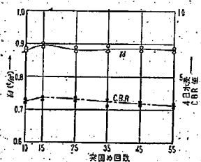
図—20 Over-Compaction と Remoulding の影響
