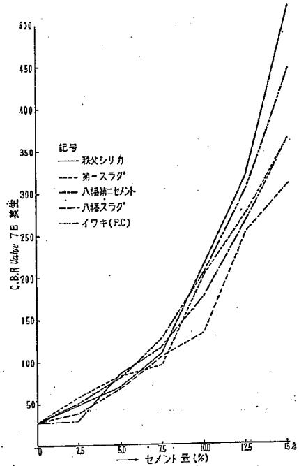
図-15 各種セメントとソイルセメント C.B.R
