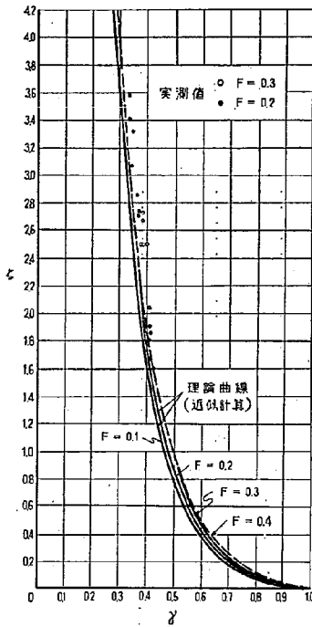
図-30 \theta=90^\circ の形状損失係数と r との関係
