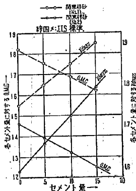
附図—1 (6) セメント添加による締固め効果
