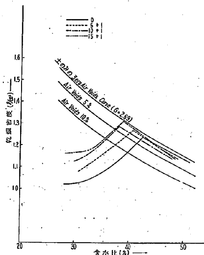
附圖一（2）「セメントと塩化カルシウム」が締固め結果に及ぼす影響
