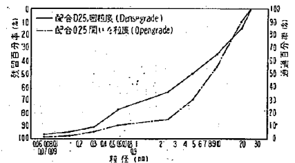
図-1 最大粒径 25mm, アスファルトコンクリート骨材粒度
