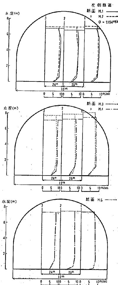
図-25 トンネル内流速分布
