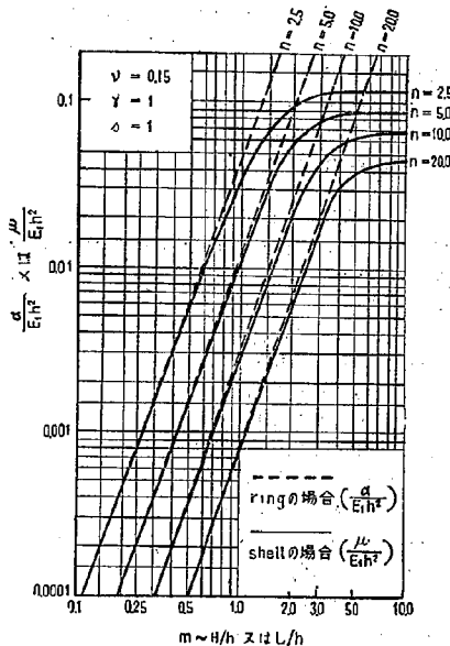
図-5 \frac{\alpha}{E_1 h^2} 又は \frac{\mu}{E_1 h^2} と m との関係の 1 例
