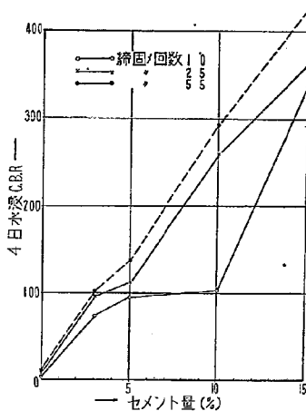
図—10 締固めエネルギーと安定度との関係 試料「名一神」千里山(試料No.7) J.I.S 標準締固めの最適条件
