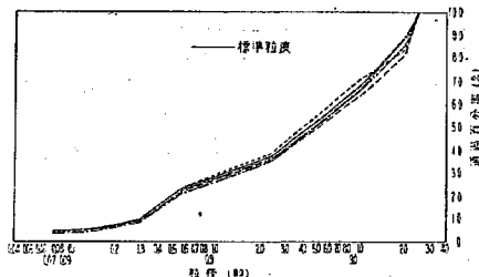
図-6(a) 3kg 混合の場合の骨材の分離(配合 D25, ストレートアスファルト I)
