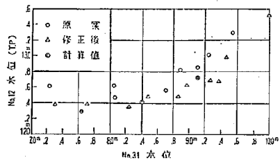
図-14 No. 31 水位と No. 12 水位との関係 ( Q=1,000 \text{ m}^3/\text{sec} )
