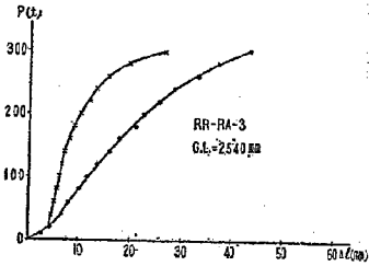
図—14. 鋼索RAの繰返引張試験 P \sim \Delta L 線図
