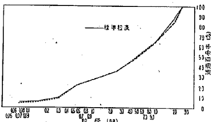
(b) 1.2kg 混合の場合の骨材の分離(配合 D25, ストレートアスファルト I)
