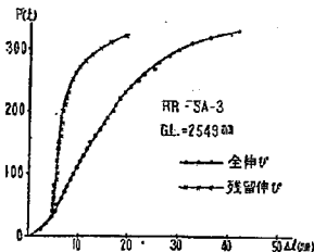
図-7. 鋼索SAの繰返引張試験の P \sim \Delta L 線図
