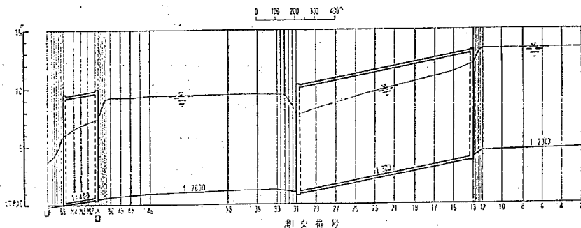
図-27 不等流計算水位
