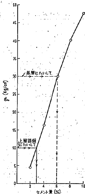
図-11 必要なセメント量のきめ方
