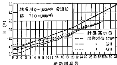
図-4 篠川背水曲線図
