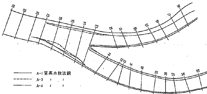
図-23 A 案平面図
