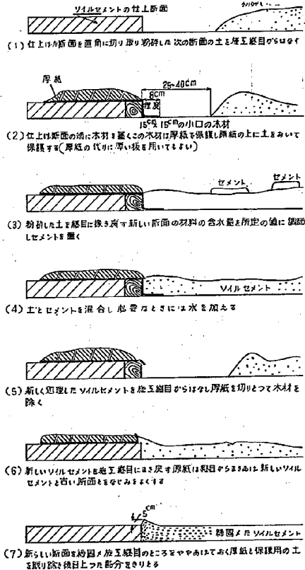
図-12 施工継ぎ目の施工要領
