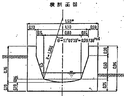
図-3 猫沢発電所余水吐横断面図
