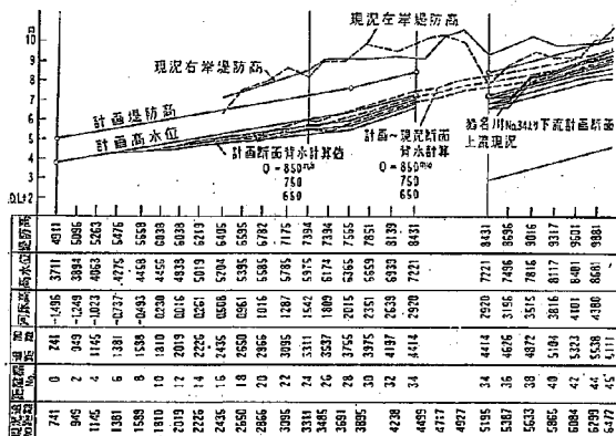
図-6 猪名川縦断面図 (3)
