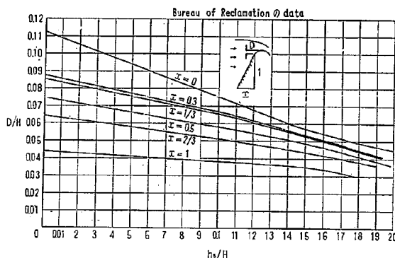
図-4 h_1/H と D/H の関係
