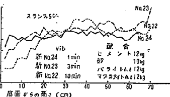
図—8 振動が材料分離に及ぼす影響
