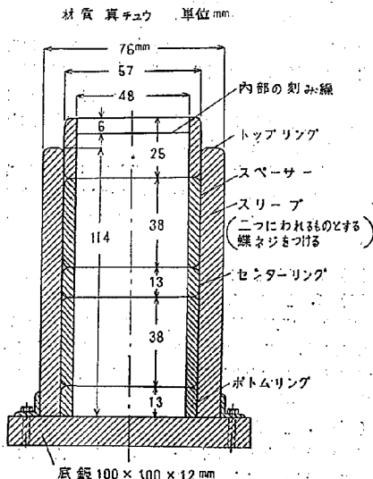
図-10 B.S. 式鉾物粉沈降試験装置(材質真チウ)
