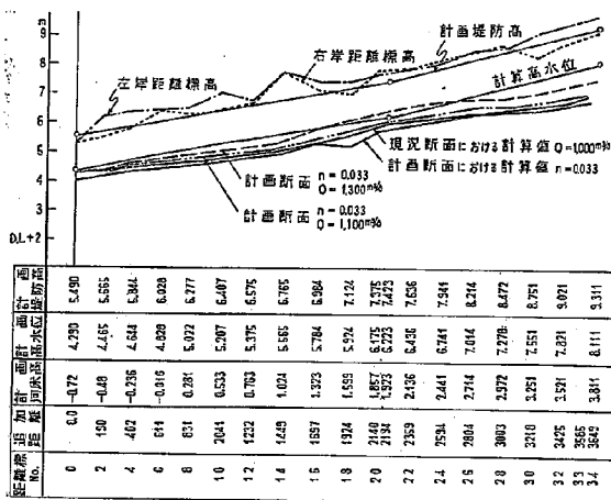
図-5 篠川縦断面図
