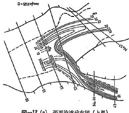
図-12 (a) 平面流速分布図 (上層)
