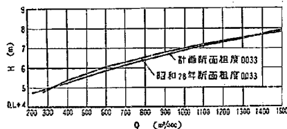
図-3 篠川 No. 39' 水位-流量曲線
