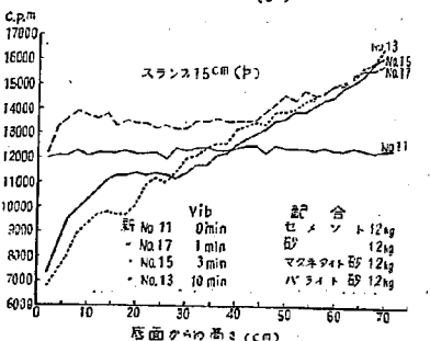
図—10 A.E 剤の混入が材料分離に及ぼす影響 (ボジリス (P): 0.3% 添加 ダレックス (D): 0.001% 添加)
