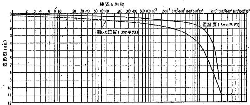
図-15 温度 25°C, 圧力 4 kg/cm², 荷重 290 kg, アスファルト量=5%
