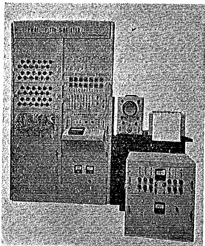
写真-1 洪水流出計算機の外観
