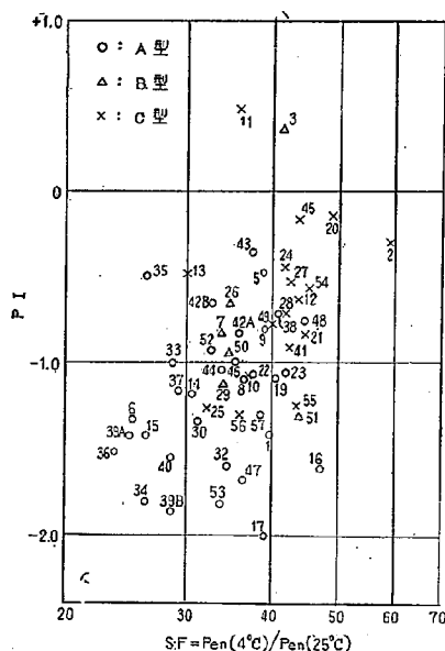
図—4 針入度比 (S.F.) と P.I. との関係
