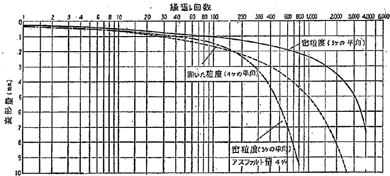
図-16 温度 25°C, 圧力 8 kg/cm², 荷重 630 kg, アスファルト量=5%
