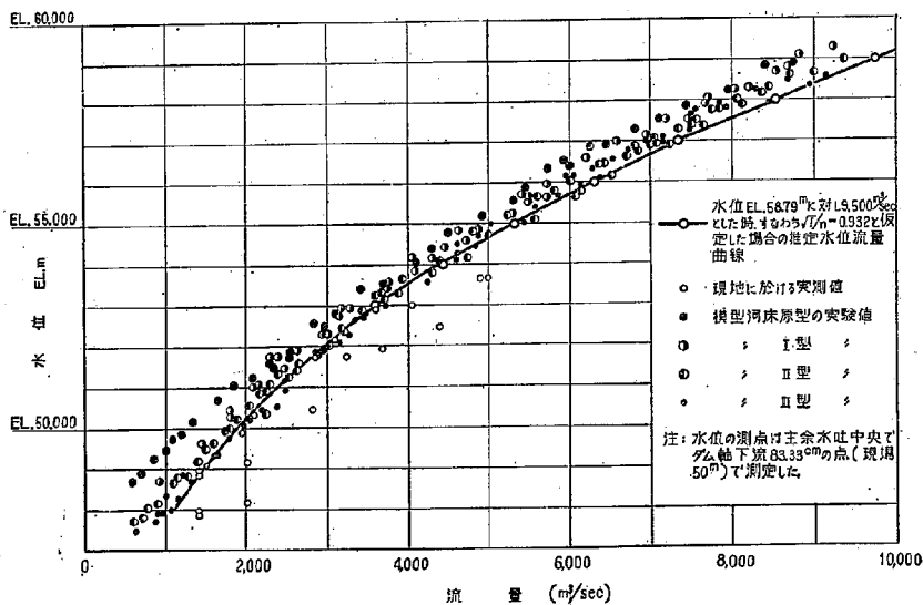
図 — 5 ダム下流水位推定値と実測値・実験値の関係
