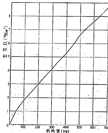
図-7 空気圧と載荷重の関係 (0.5秒載荷, 1.5秒休止の場合)
