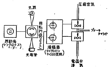
図-4 パルス発生機構
