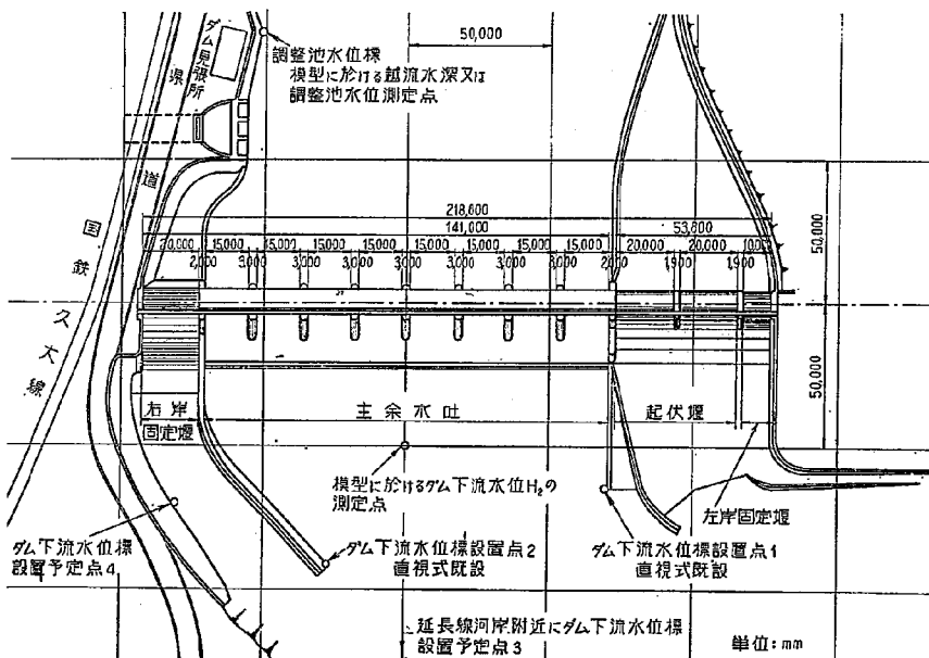
図一2 夜明ダム平面図
