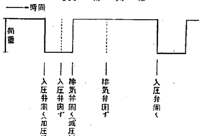
図-9 入圧弁、排気弁の作動
