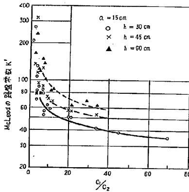
図—10 路盤材料の性質と McLeod 路盤係数との関係 (30cm 載荷板の場合)
