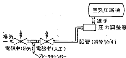
図-3 加圧機構
