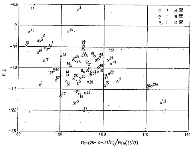
図—6 針入度(25-4-25°C) / 針入度(25°C) と P.I. との関係
