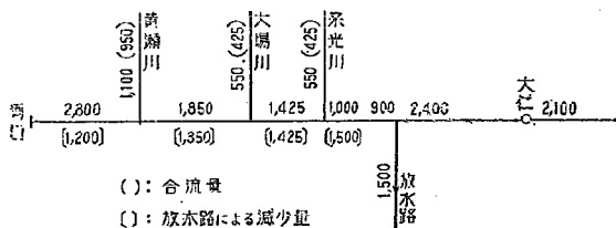
図-5 狩野川計画高水流量配分図 (沼津工事業務所案)
