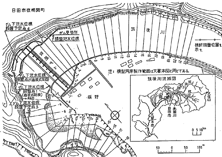
図一1 夜明ダム附近平面図
