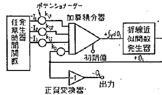
図-4 追跡計算の単位区間のブロック線図
