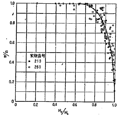
図—9 自由越流時の H_2/H_1 と m'/m の関係
