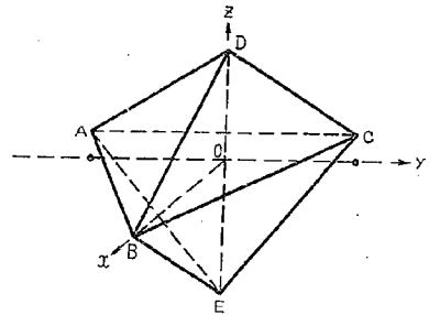
図一 非対称六面体型三次元土圧計
