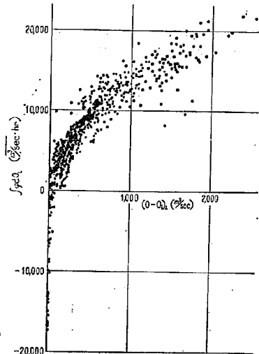
図-10 筑後川夜明上流流域の貯留関数 (総合)
