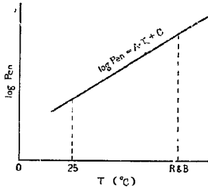
図-2 温度と針入度との関係
