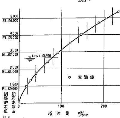
図-13 左岸固定堰の水位流量曲線
