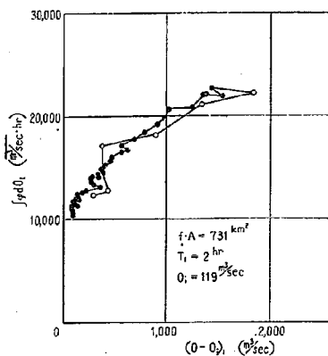
図-9 筑後川夜明上流流域の貯留関数（洪水ごと） (a) 昭. 29. 5. 26. ~28. (洪水番号 2-1)
