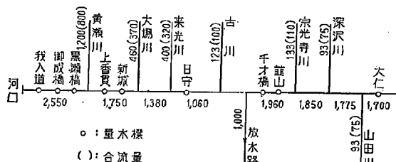
図-3 狩野川計画洪水流量配分図 (昭33.現在)
