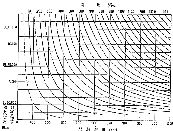
図—19 門扉1門当りの門扉開度と水位流量図
