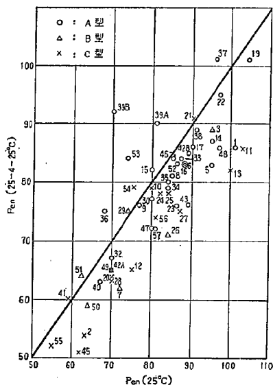
図—5 針入度に対する温度感度の影響
