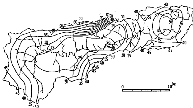
図-13 (5) 一雨雨量と真値との相対誤差の標準偏差, 地域 V
