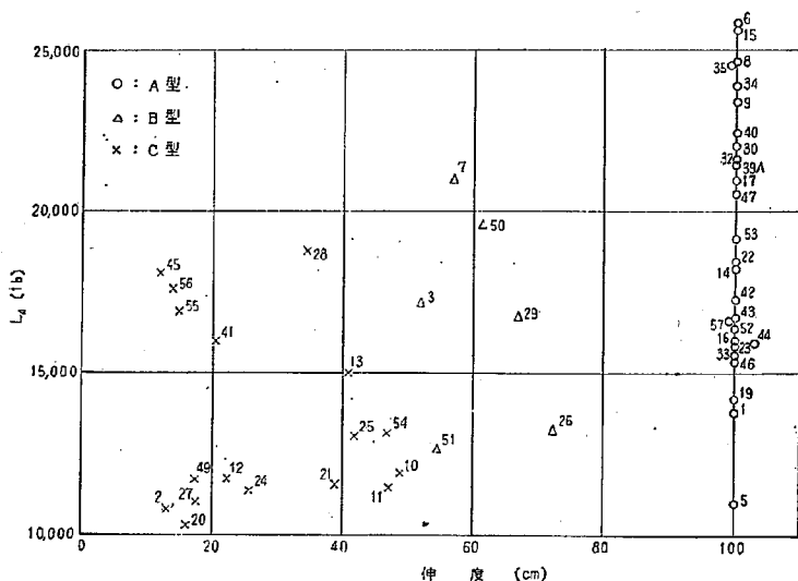
図—8 伸度(10°C)と低温安定度(4°C)との関係
