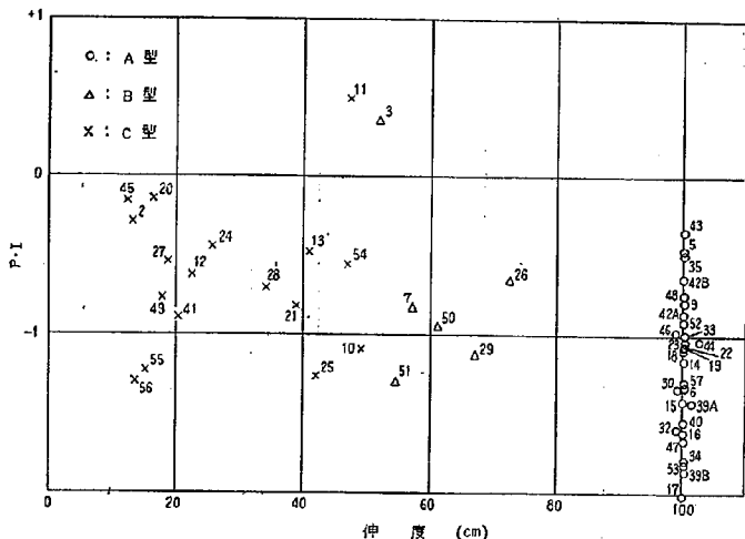
図-7 伸度 (10°C) と P.I. との関係
