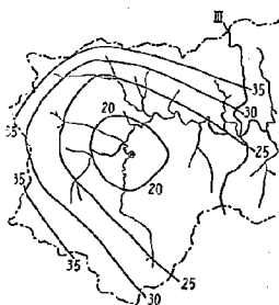
図-13 (3) 一雨雨量と真値との相対誤差の標準偏差, 地域 III
