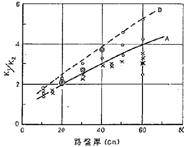
(a) 砂利、砂、粘土混合物の路盤
