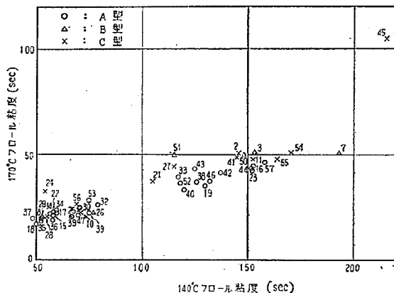
図—9 温度によるフロー粘度の相違
