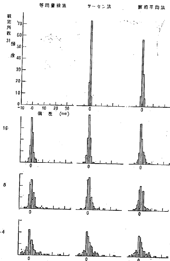
図-7 一雨雨量と真値との絶対誤差(mm)の頻度
