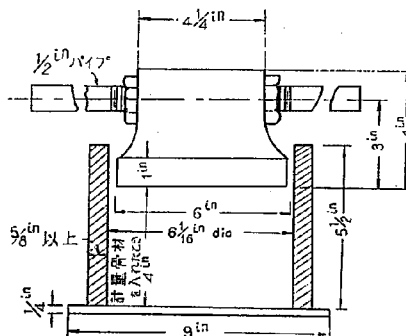
附図—1 破砕試験用モールド
