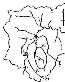
図-13 (1) 一雨雨量と真値との相対誤差の標準偏差, 地域 I
