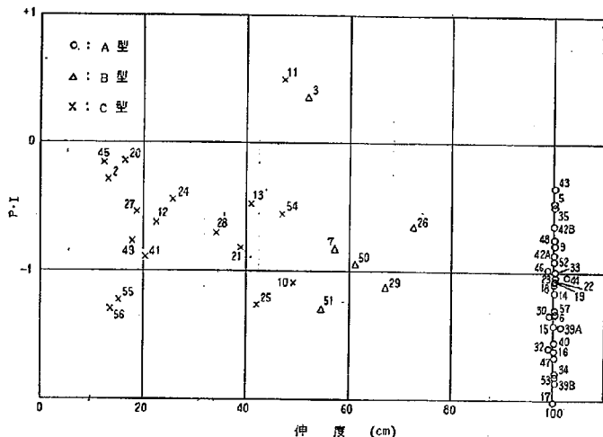
図一七 伸度(10°C)と P.I. との関係
