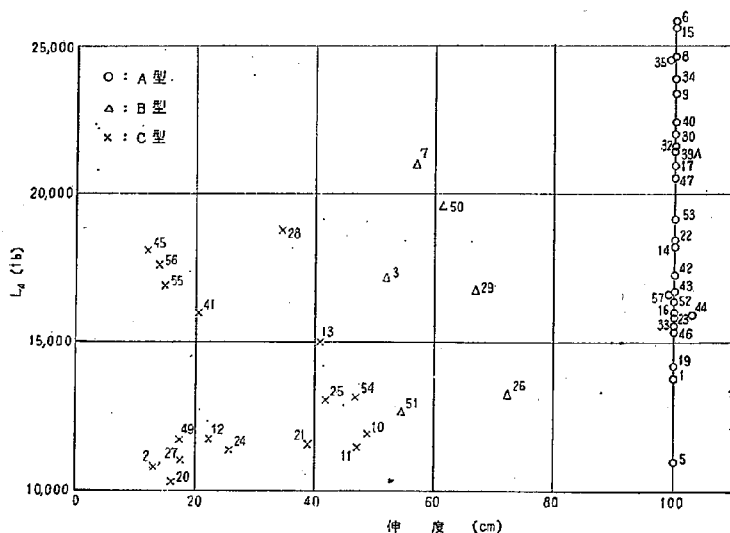
図一八 伸度(10°C)と低温安定度(4°C)との関係
