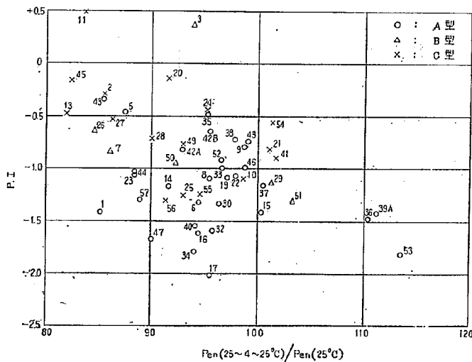
図—6 \frac{\text{針入度}(25-4^\circ\text{C})}{\text{針入度}(25^\circ\text{C})} と P.I. の関係
