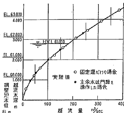
図-14 右岸固定堰の水位流量曲線
