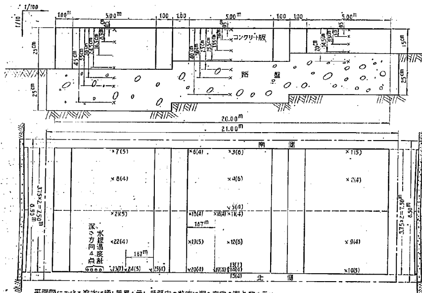
平面図における数字は通し番号を示し、括弧内の数字は深さ方向の測点数を示す。 No.13は緑から5 \text{cm} , No.14は緑から10 \text{cm} , No.15は緑から5 \text{cm} の位置である。その他はすべて緑から15 \text{cm} に位置している。
