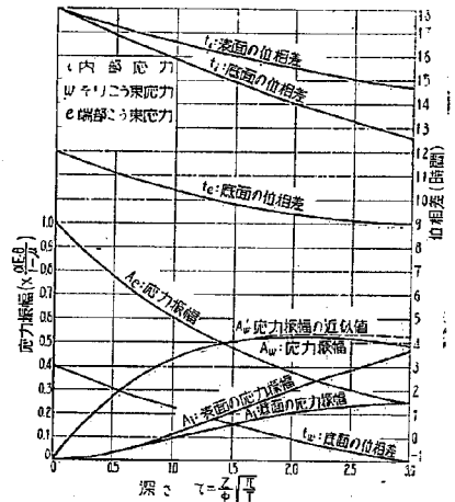
図-4 Thomlinson の温度応力の振幅と位相差
