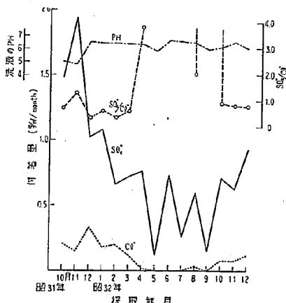
図-3 Cl - , SO 4 - 付着量
