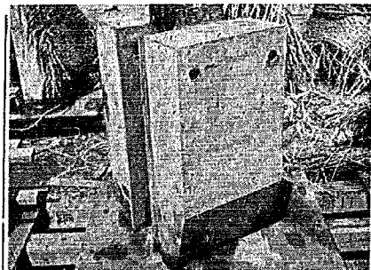
写真-2 コンクリート打ち後1週間を経た型枠をははずされた供試体
