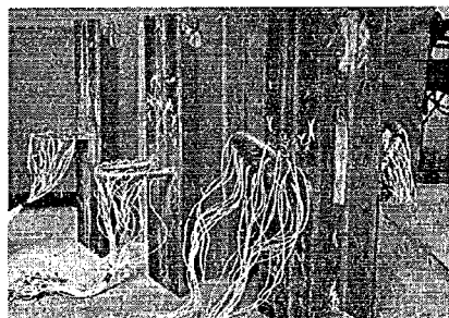
Channel および hoop shear connector に貼付されたストレインゲージ、既にコーテ ングは完了している。
