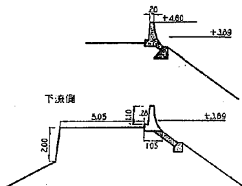
図-3.9 鍋田川左岸芝井 4.2km 地点
