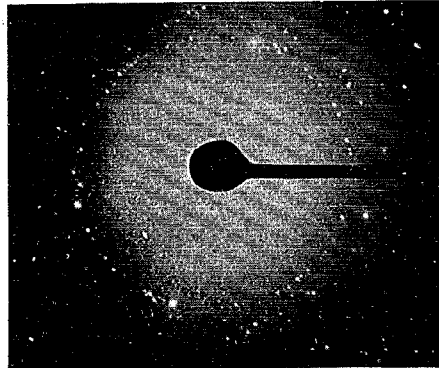
写真-3 アロファンと \text{Ca}(\text{OH})_2 との反応生成物の電子顕微鏡写真
