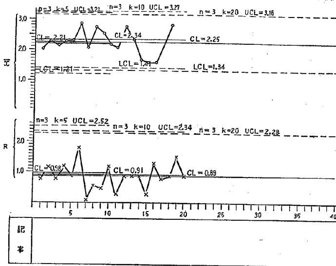
図-1 \bar{x} -R 管理図
