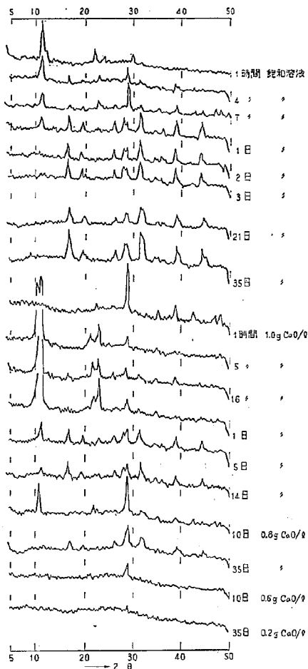
図-13 80°C における反応生成物のX線回折図
