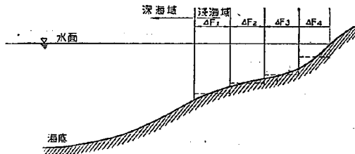
図-2.7 水深が変化する浅海における波の推算
