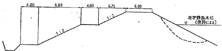
図-3.11 長良川右岸野寺地先堤防断面図
