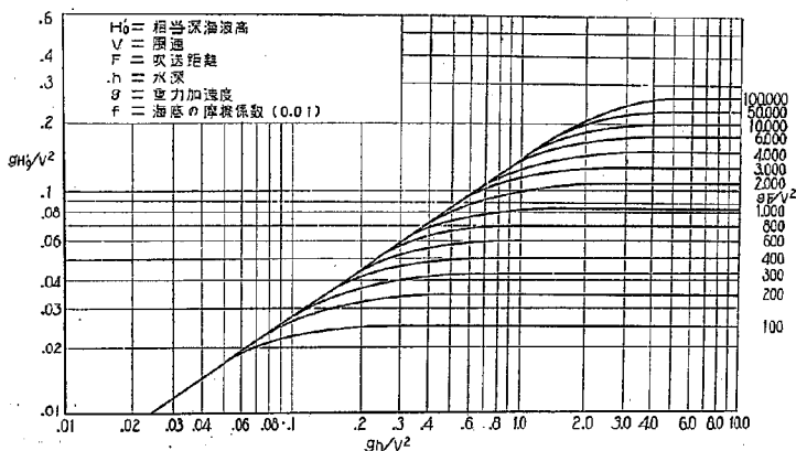
図-2.6 一般水深の浅海における波の推算図
