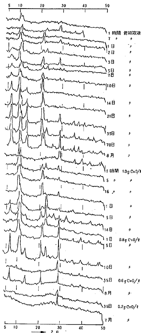
図-1 220°C における反応生成物のX線回折図 が、この間でもYとZによる粉末線強度の比は一定の傾向で増減しない。
