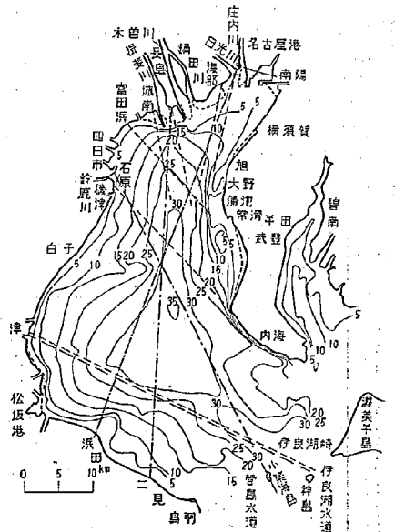
図-2.10 波を計算した場所と Fetch
