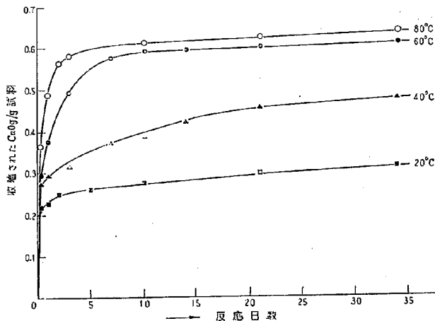
図-20 反応温度が異なる場合飽和 \text{Ca}(\text{OH})_2 溶液からの \text{CaO} 取着量と反応日数
