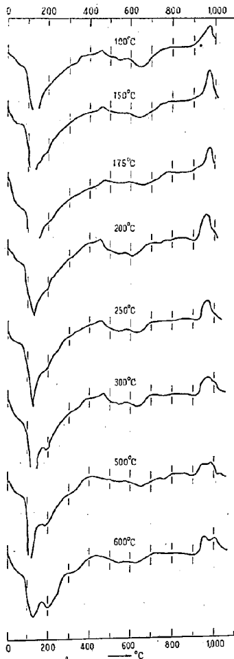
図-5 加熱処理したアロファン粘土と \text{Ca}(\text{OH})_2 の反応生成物の DTA 曲線
