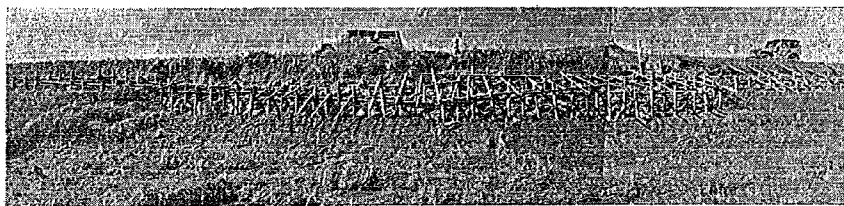
写真-3.15 長良川右岸堤防表の崩壊状況
