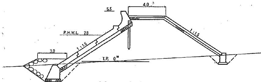
図-3.6 磯津海岸堤防標準断面図
