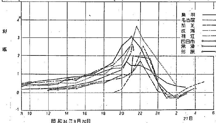
図-4.66 伊勢湾各地の偏差
