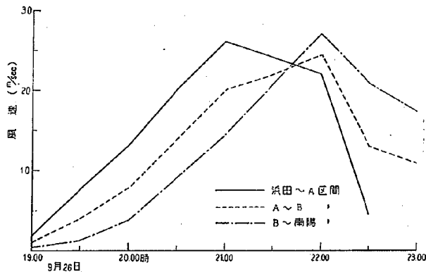
図-2.13(a) 南陽～浜田間の各区間における風速の変化
