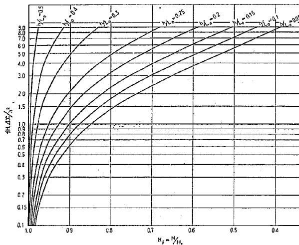
図-2.3 海底摩擦による波高減衰率
