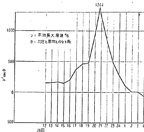
図-1.5 伊良湖岬における風力
