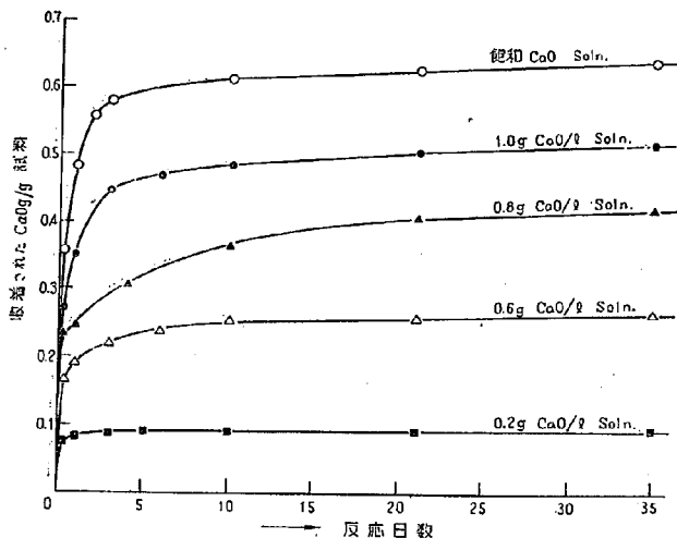
図-21 各種濃度の CaO 溶液からの CaO の吸着量と反応日数 (80°C)
