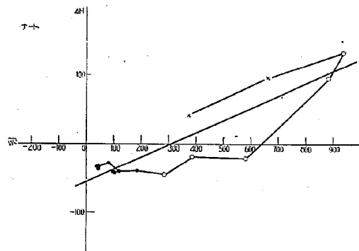
図-1.7 (a) 風力と潮位落差との関係 (名古屋一鳥羽) 単位は \Delta H : cm W^2 : m^2/sec^2 他も同様
