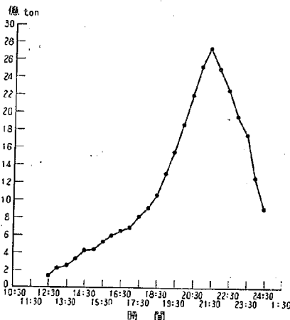
図-1.3 湾の入口からの流入総量
