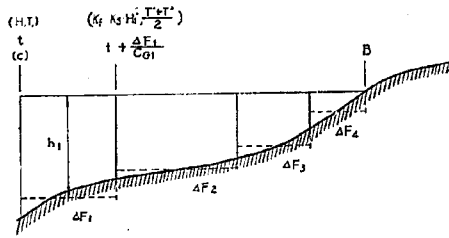
図-2.9 風向・風速の変化および海底摩擦を考慮した SMB 法による波の推算（浅海域）
