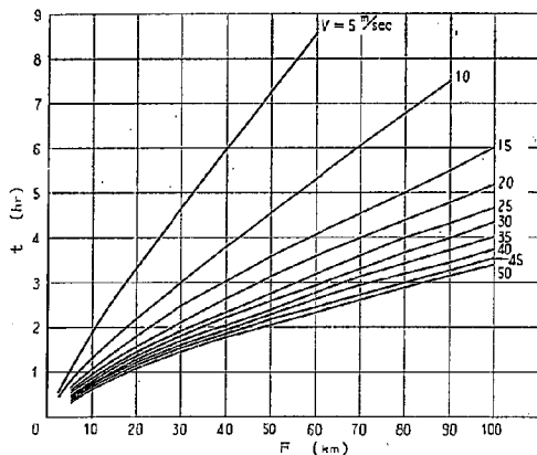
図-2.2(c) Fetch・風速・最小吹送時間の関係
