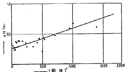
図-1.8 横溝蔵と船頭平の両量水標での水位差と桑名(一部名古屋)の風力との関係
