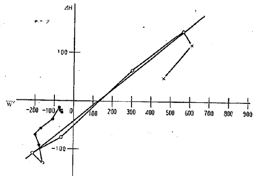
図-1.7 (b) 風力と潮位落差との関係 (名古屋一津)
