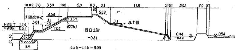
図-3.7 碧南干拓河川第1号堤（上流）矢作川右岸
