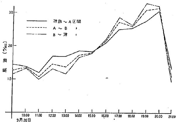
図-2.13(d) 津～福島間の各区間における風速の変化
