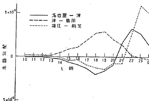
図-1.9 各地点間の水面こう配変動状況
