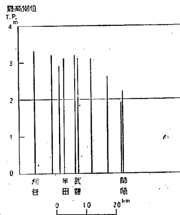
図-1.2 (c) 最高潮位 (知多湾)
