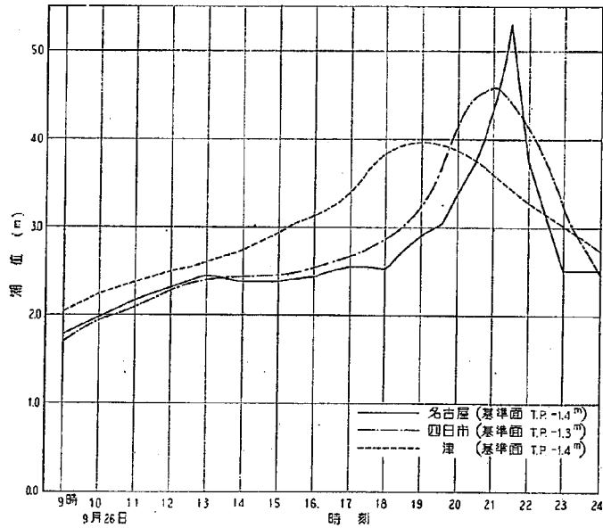
図-2.12 名古屋、四日市、津における実測潮位
