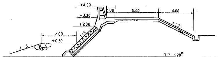
図-3.5 石原海岸堤防標準断面図
