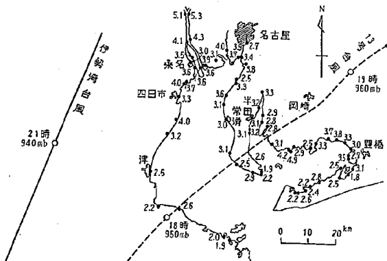
図-1.1 最高潮位分布
