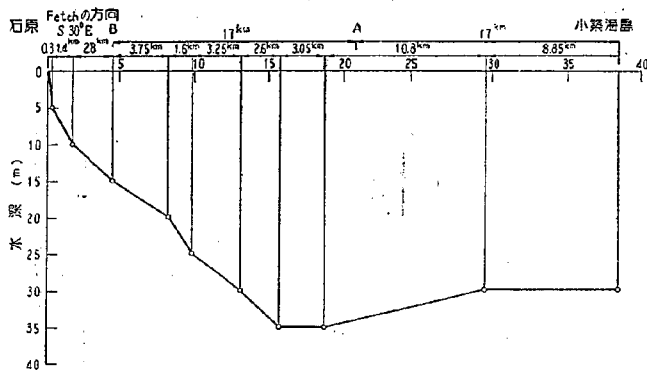
図-2.11(c) 石原～小築海島間の海底断面
