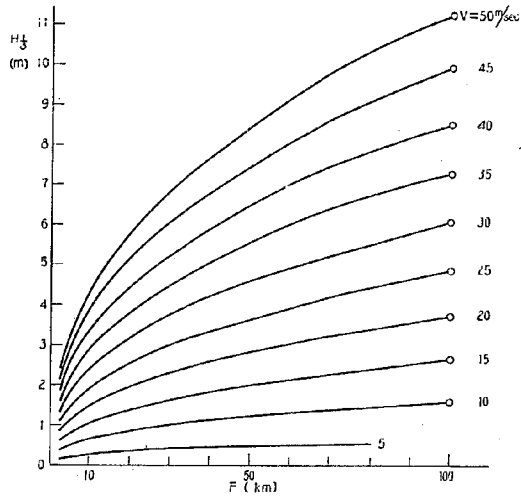
図-2.2(a) Fetch・風速・波高の関係
