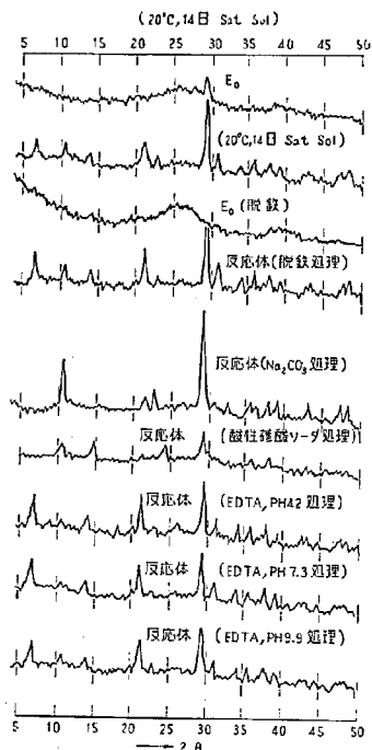
図-6 種々の処理を加えた鹿沼土 ( \text{E}_0 ) と \text{Ca}(\text{OH})_2 溶液の反応生成物
