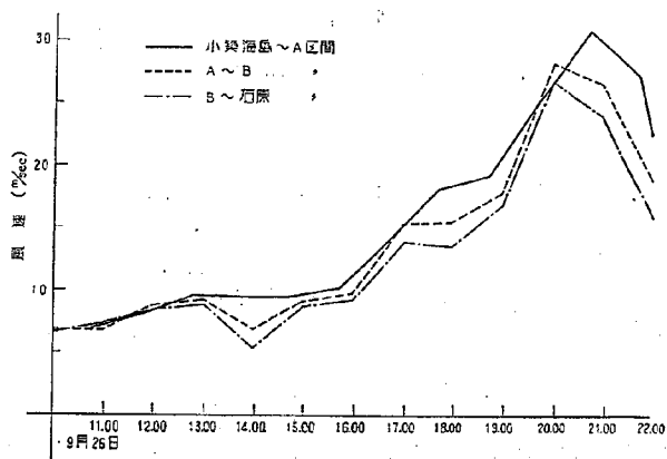
図-2.13(c) 石原～小築海島間の各区間における風速の変化
