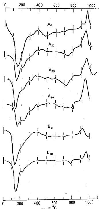
図-2 鹿沼土よりの土壌コロイドと \text{Ca}(\text{OH})_2 との反応生成物のDTA線
