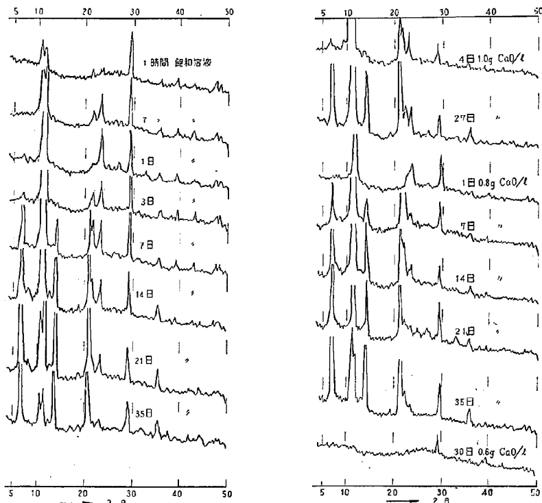
図-14 40°Cにおける反応生成物のX線回折図
