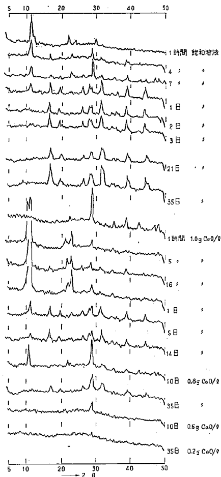
図-13 80°C における反応生成物のX線回折図
