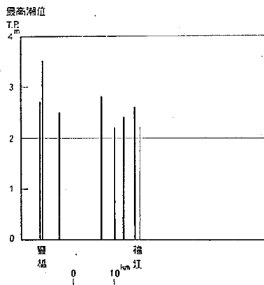
図-1.2 (d) 最高潮位 (渥美湾南岸)
