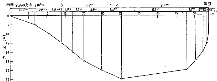
図-2.11(a) 南陽～浜田間の海底断面
