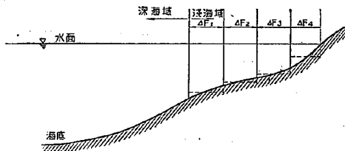
図-2.7 水深が変化する浅海における波の推算
