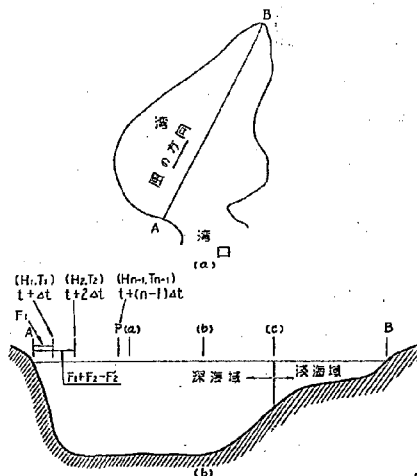
図-2.8 風向・風速の変化および海底摩擦を考慮した SMB 法による波の推算 (深海域)
