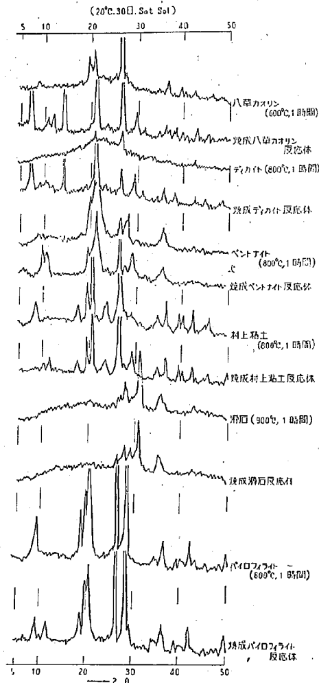
図-11 各種粘土鉱物焼成物と \text{Ca}(\text{OH})_2 との反応生成物
