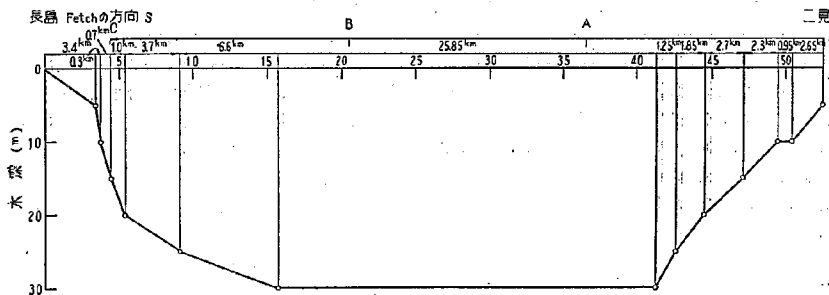
図-2.11(b) 長島～二見間の海底断面
