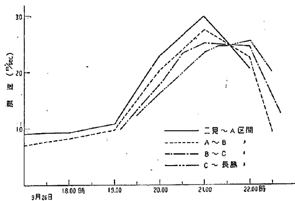
図-2.13(b) 長島～二見間の各区間における風速の変化
