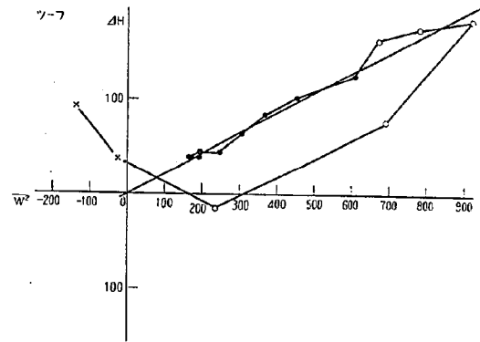
図-1.7 (d) 風力と潮位落差との関係 (津一福江)
