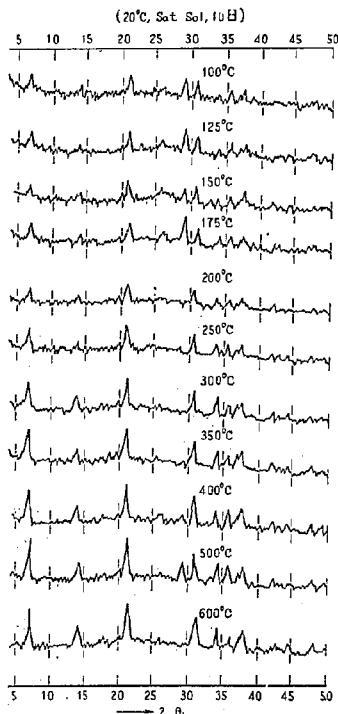
図-4 加熱処理したアロファン粘土と \text{Ca}(\text{OH})_2 の反応生成物
