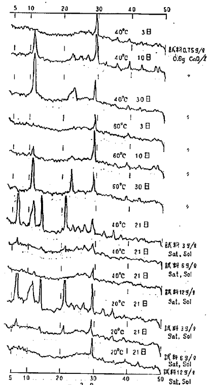
図-17 試料量を変えた場合の反応生成物のX線回折図
