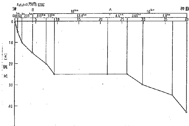
図-2.11(d) 津～小築島間の海底断面
