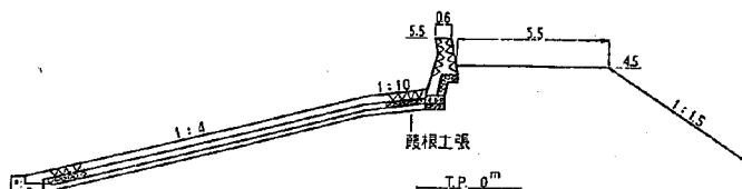
図-3.4(b) 城南海岸堤防標準断面図
