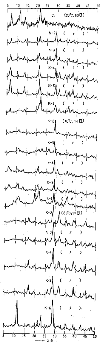
図-10 各種アロファン粘土と \text{Ca}(\text{OH})_2 溶液との反応生成物のX線回折図
