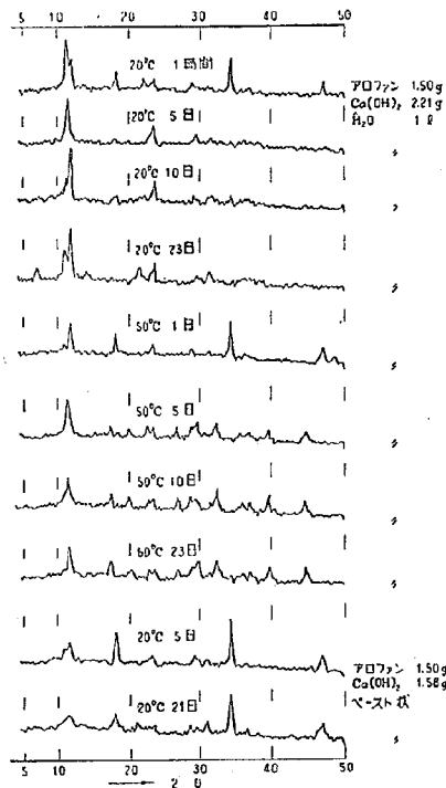
図-19 \text{Ca}(\text{OH})_2 の過量ペースト状の場合の反応生成物
