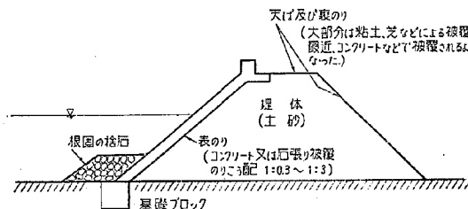
図-3.1 伊勢湾、知多湾および温帯湾沿岸における海岸堤防の一般的形式
