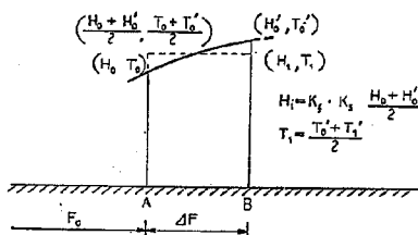
図-2.4 一般水深の浅海における波の推算
