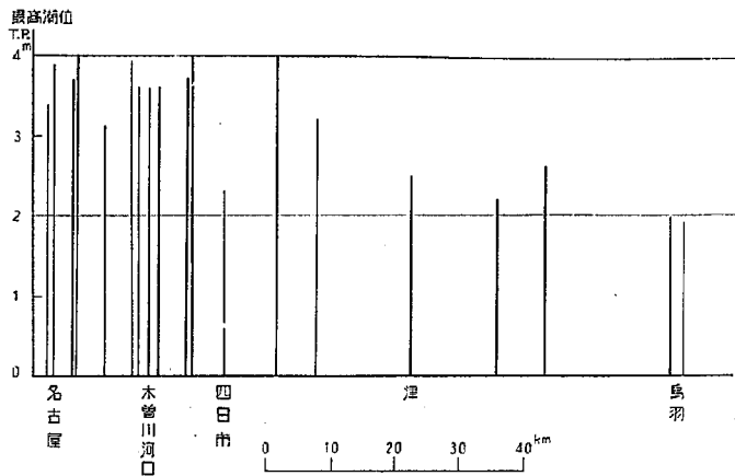
図-1.2 (a) 最高潮位 (伊勢湾 三重県沿い)
