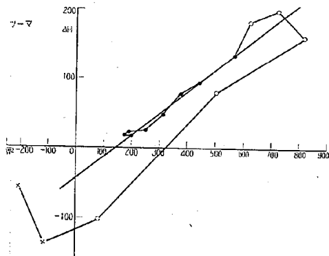
図-1.7 (e) 風力と潮位落差との関係 (津—前芝)
