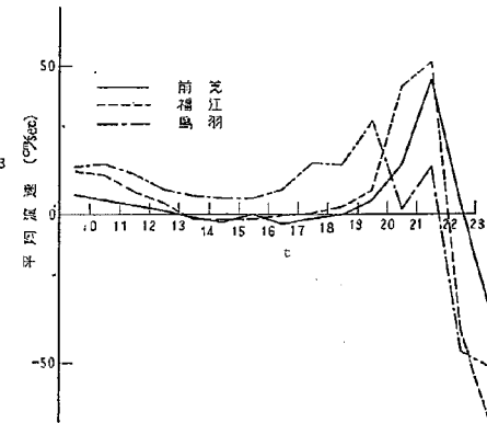
図-1.11(b) 各地点における平均流速の変動状況
