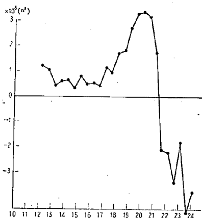
図-1.4 湾の入口からの流入量 (30分間の量)
