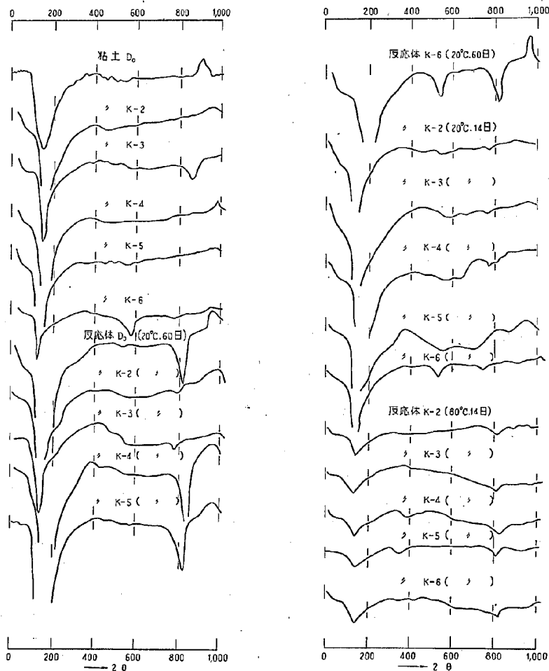
図-8 各種アロファン粘土と \text{Ca}(\text{OH})_2 溶液との反応体の DTA 曲線
