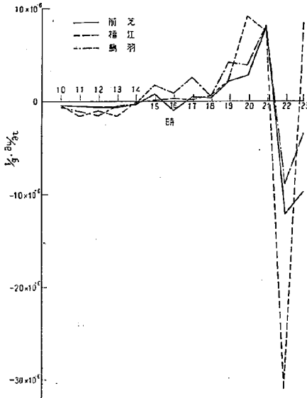
図-1.10(b) 各地点における \frac{1}{g} \frac{\partial u}{\partial t} の変動状況
