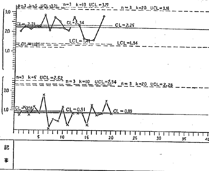
図-1 \bar{x} -R 管理図
