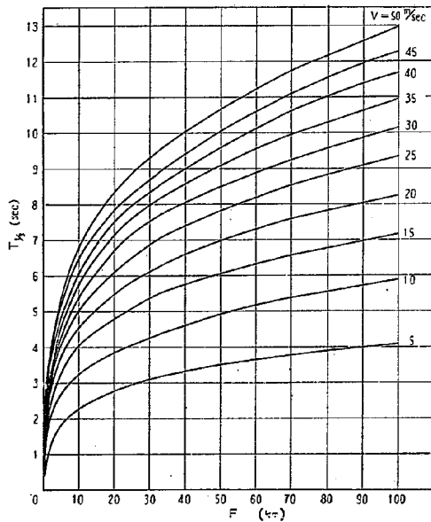
図-2.2(b) Fetch・風速・周期の関係
