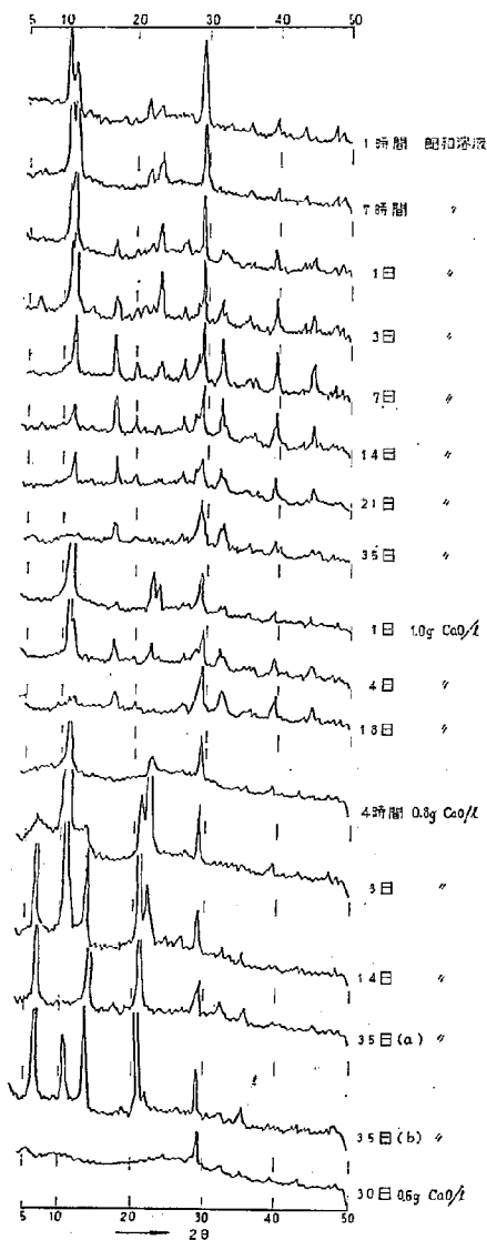
図-15 60°C における反応生成物のX線回折図 末線をのこしている。しかし18日に至ればYおよびZはほとんど見られなくなり、Vのみが認められる。0.8g CaO/lの場合は1時間では結晶性物質は生成しないが4時間でYを認め、Yの粉末線強度は漸次強くなり3日に至ってC 2 ASH n を認める。さらに時間の経過と共にC 2 ASH n の粉末線強度は大きくなる反面、Yによる強度は漸次低下する。35日の反応生成物を容器底に比較的
