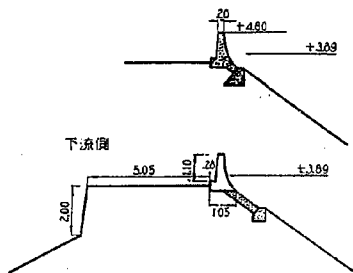
図-3.9 鍋田川左岸芝井 4.2km 地点
