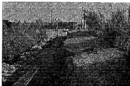
写真-3.10 裏のり肩崩壊状況
