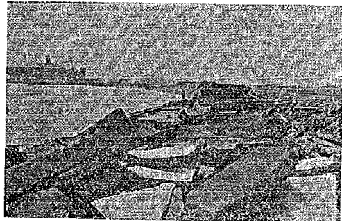
写真-3.6(a) 磯津海岸堤防
