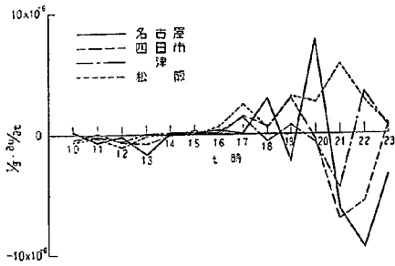
図-1.10(a) 各地点における (1/g)(\partial u/\partial t) の変動状況
