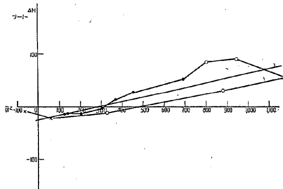
図-1.7 (c) 風力と潮位落差との関係 (津一鳥羽)
