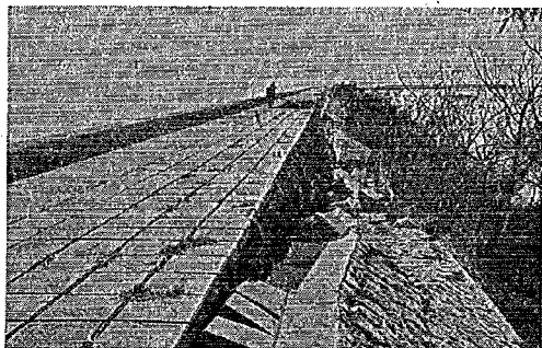
写真-3.8(c) 長島海岸堤防裏のり崩壊状況
