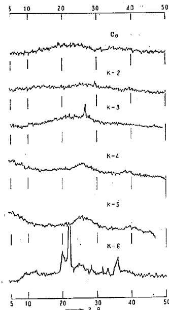
図-7 アロファン粘土のX線回折図
