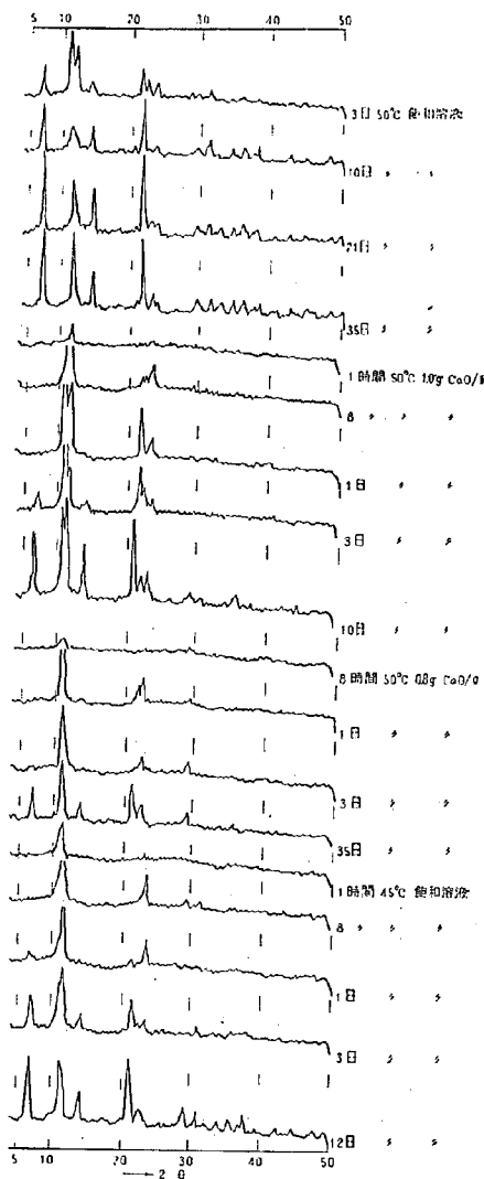
図-16 50°C, 45°C における反応生成物のX線回折図
