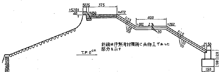
図-3.3 康衛新田海岸堤防標準断面図
