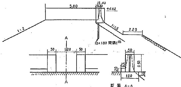
図-3.9 鍋田川左岸芝井 4.2km 地点
