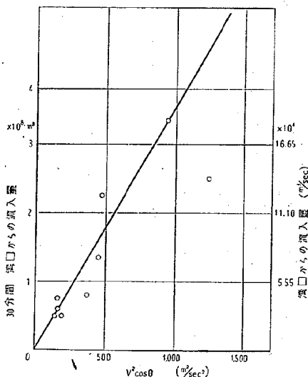
図-1.6 湾口からの流入量と風力の関係
