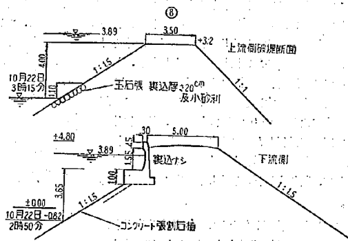
図-3.8 日光川左岸南陽町（河口）
