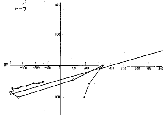
図-1.7 (f) 風力と潮位落差との関係 (島羽—福岡)
