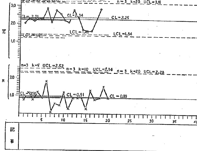
図-1 \bar{x} -R 管理図
