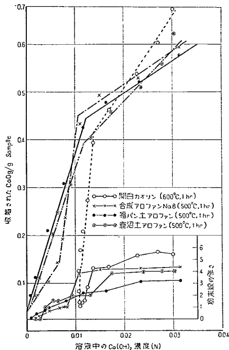
図-31 収着量と平衡濃度および固相の粉末線強度
