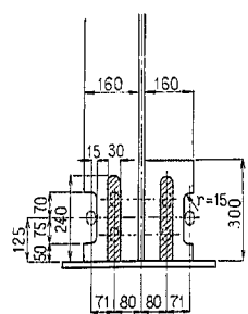
補剛材
