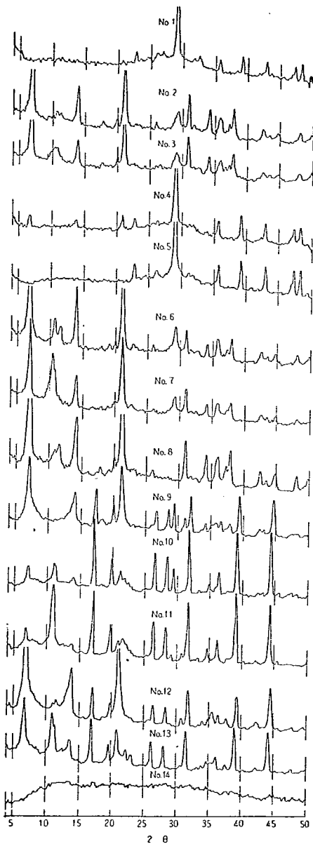
図-26 (a) \text{SiO}_2\text{-Al}_2\text{O}_3 ゲルと飽和 \text{Ca(OH)}_2 溶液との反応生成物 X 線回折図 (20°C, 14日)
