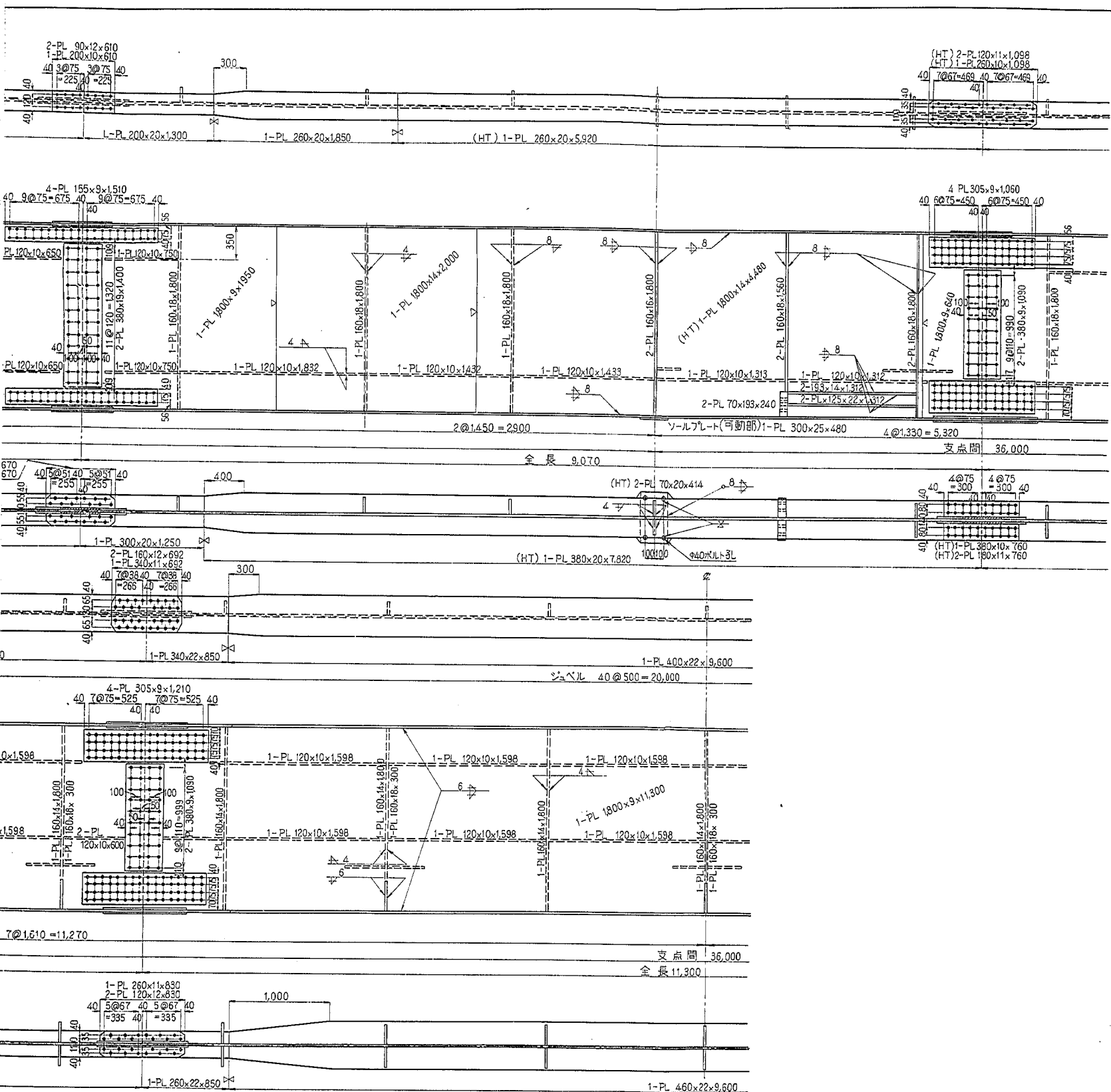
定着部詳細図
