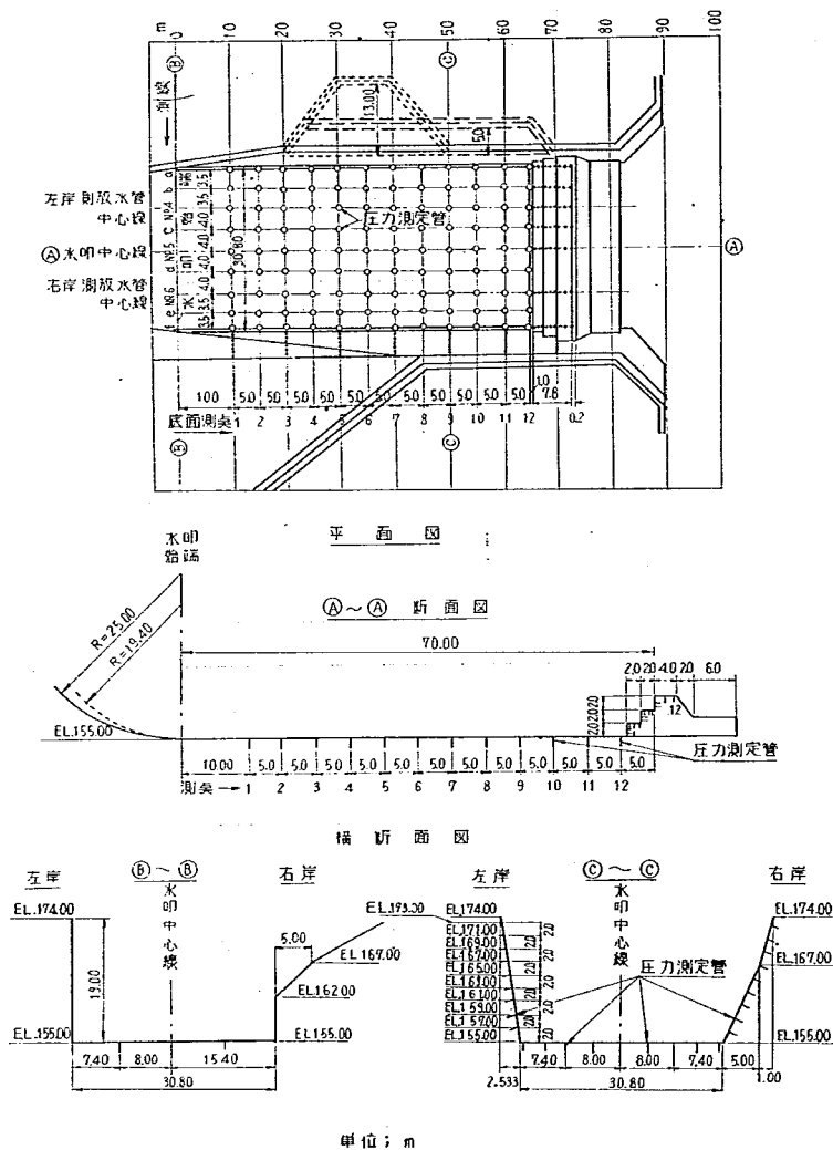
図-24 水叩 8 型 圧力測点位置図
