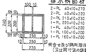
排水枋部材
