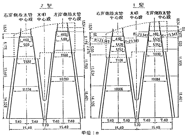
圖-50 放水管導水樋改良案
