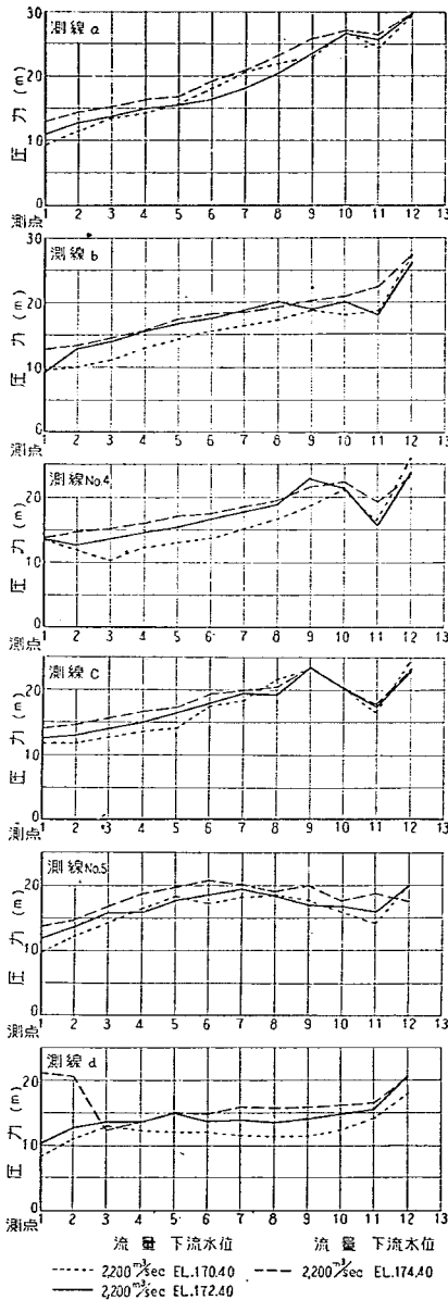
図-41-1 (1) 水門底面圧力分布図 門扉操作時 下流水位変化による圧力
