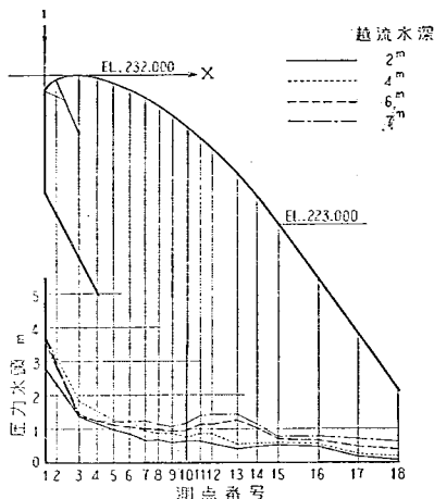
図-8 1型越流部 自由越流時圧力分布
