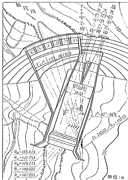
図-2 (1) 湯田ダム付近平面図
