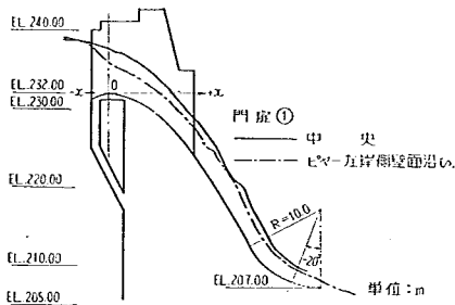
図-38 (1) 越流部水面形
