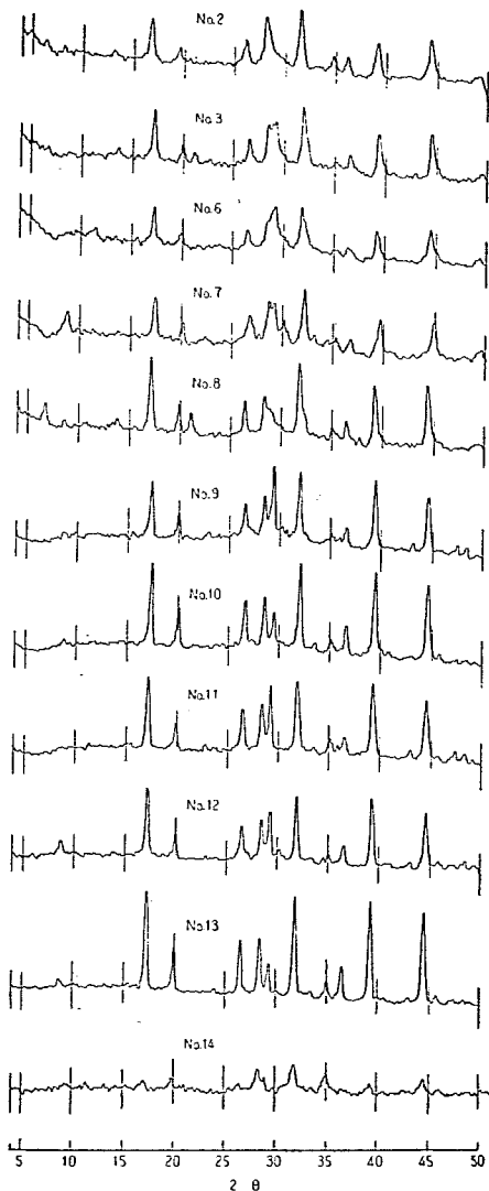
図-26 (b) \text{SiO}_2\text{-Al}_2\text{O}_3 ゲルと飽和 \text{Ca(OH)}_2 溶液との反応生成物 X 線回折図 (80°C, 14日)
