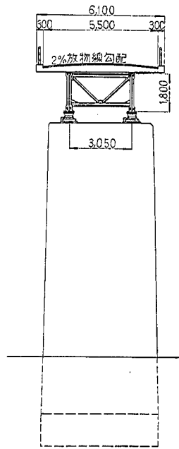
A~A'断面
