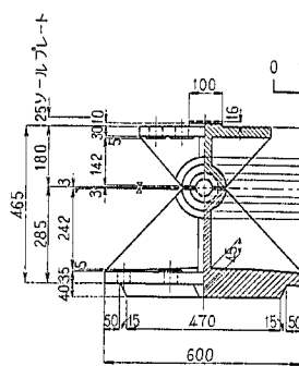
固定沓
