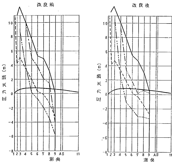
図-45 放水管ベルマウス改良案実験値
