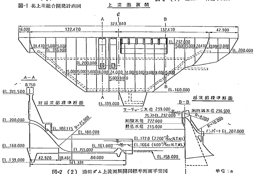
図-2 (2) 湯田ダム上流面展開図標準断面平面図
