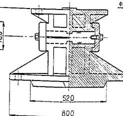
固定沓
