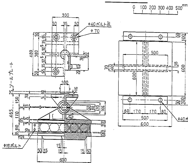
中間可動沓
