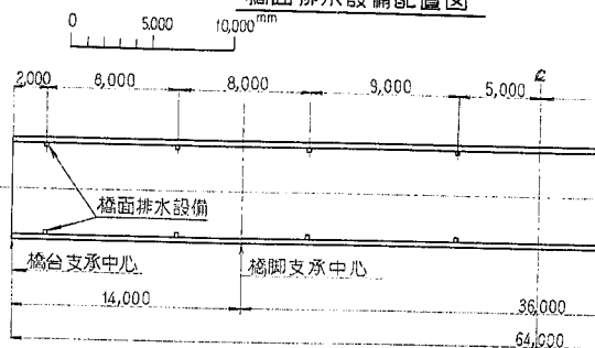
橋面排水設備配置図
