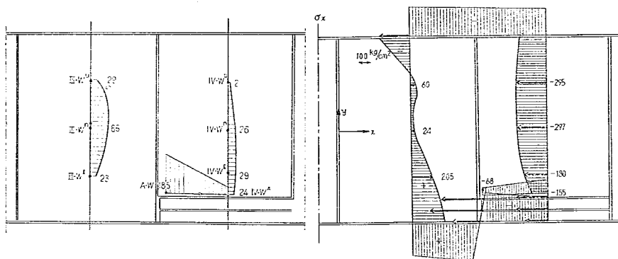
圖-22 最大剪斷應力圖
