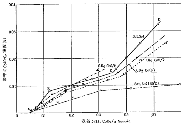
図-30 取溶量と平衡濃度（鹿沼土アロファン，20°C，35日）
