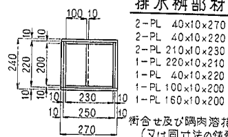
排水桷部材
