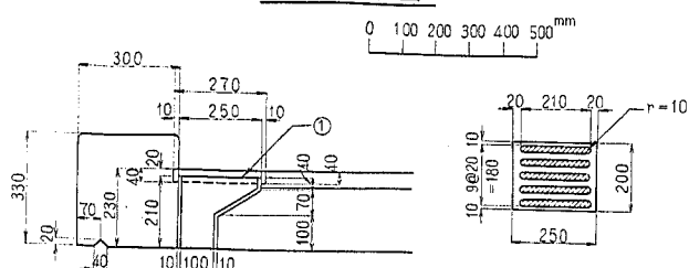
排水桝詳細図
