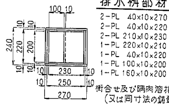
排水桝部材
