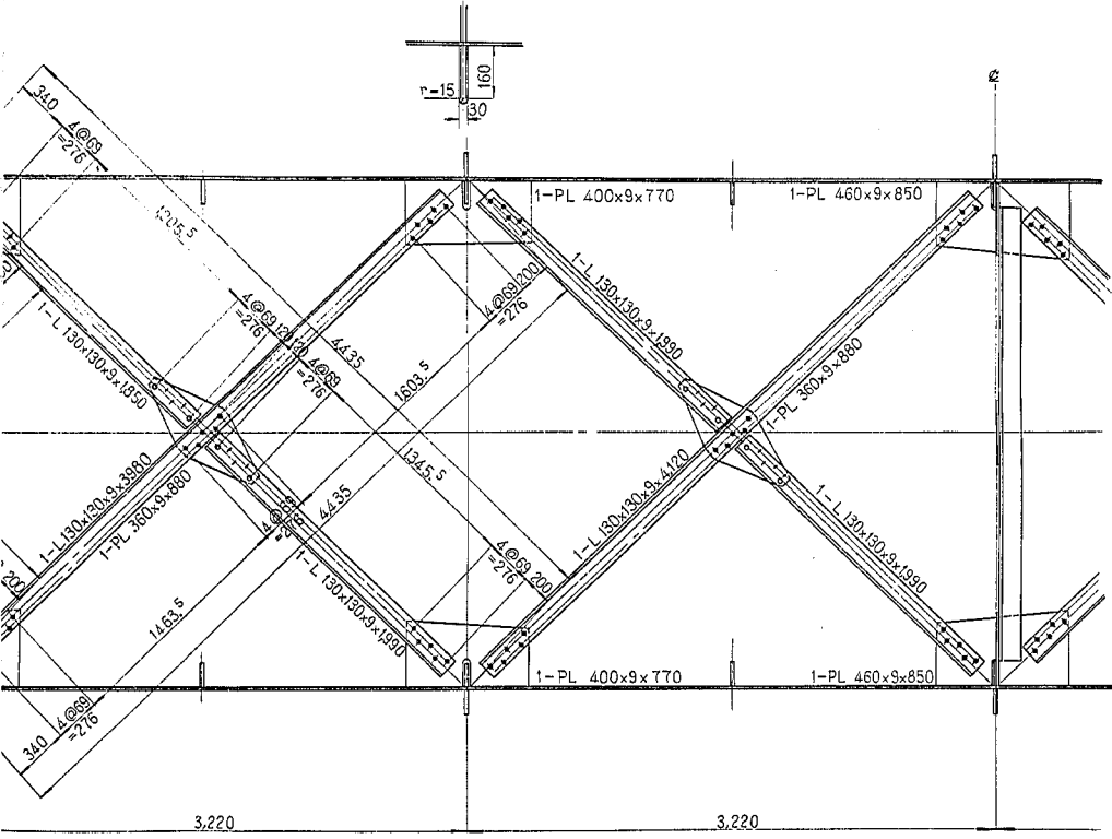
対傾構
