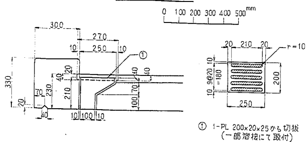
排水桝部材
