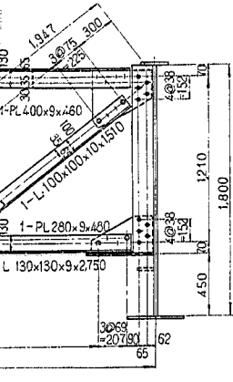
対傾構
