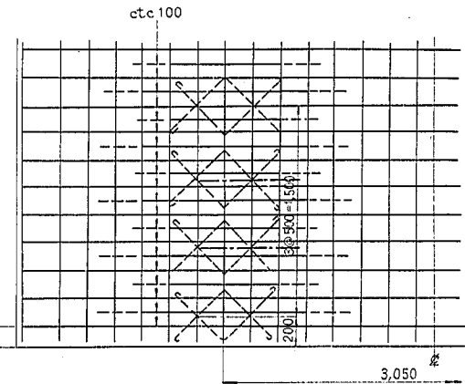
桁端部配筋図
