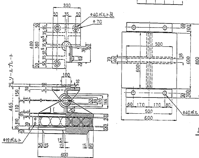
中間可動柵
