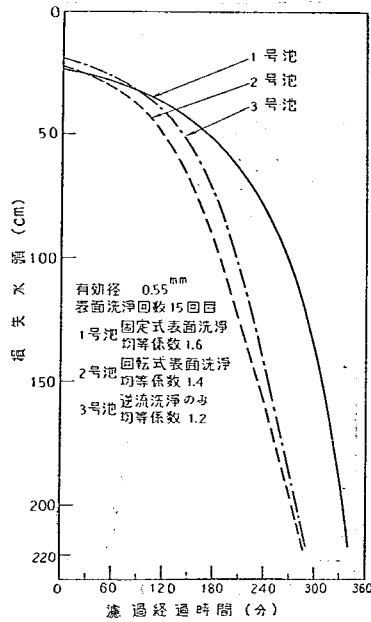
図-72A 損失水頭の比較
