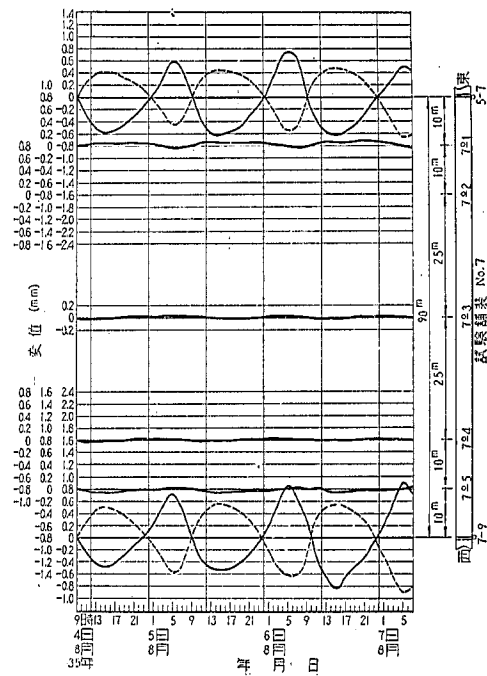
図-49 コンクリート版変位の日変化 (試験舗装 No.7)
