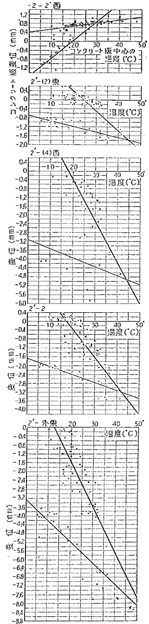
図-82 年変化におけるコンクリート版変位と温度の関係 (試験舗装 No.2)
