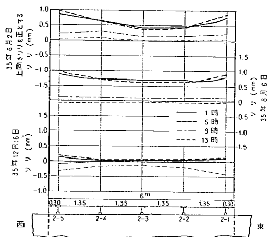
図-116 めくら目地間隔6mのコンクリート版の見掛上のそりと位置の関係
