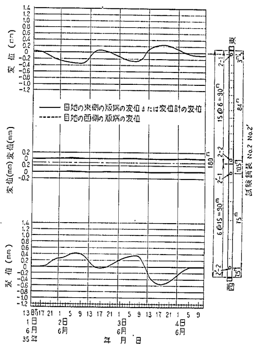
図-39 コンクリート版変位の日変化 (試験舗装 No. 2, No. 2')
