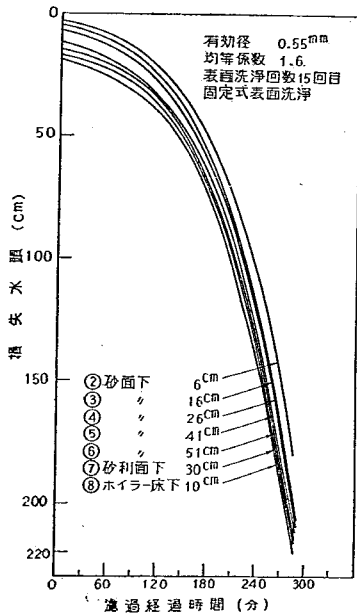
図-72B 1号池における損失水頭の変化
