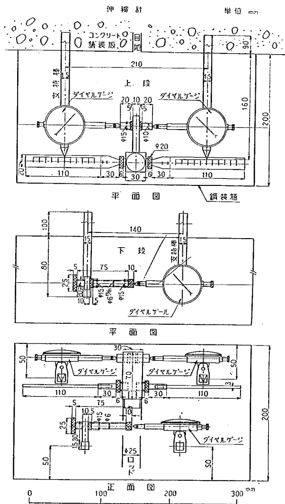
図-6 伸縮計詳細図
