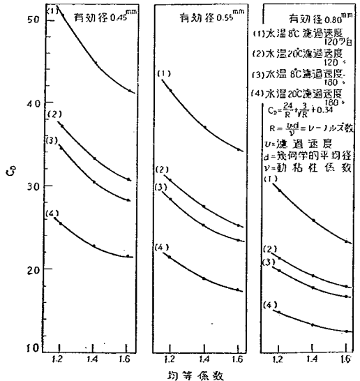
図-21 有効径別の抵抗係数 C_D (不成層の場合)
