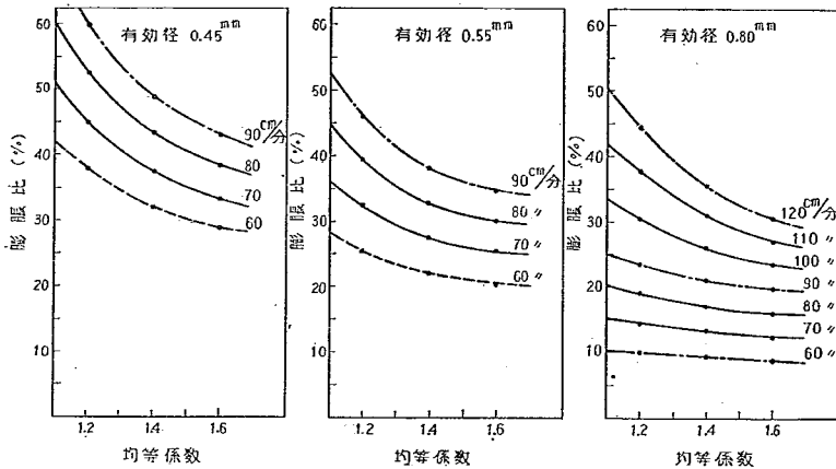
図-3 低水温時における膨脹比、洗浄速度および粒径との関係 (有効径別)
