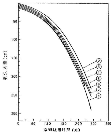
図-28D 損失水頭 (均等係数 1.2)
