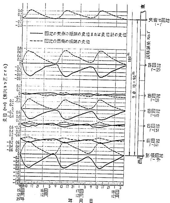
図-38 コンクリート版変位の日変化 (試験舗装 No. 1)
