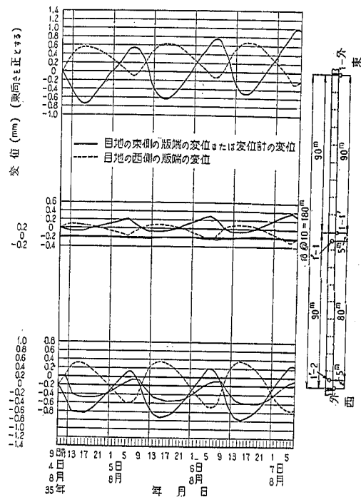
図-31 コンクリート版変位の日変化(試験舗装 No.1)
