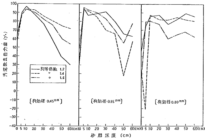
図-15B 砂層深度別汚泥量の除去百分率 (沈澱池を設置しない場合)
