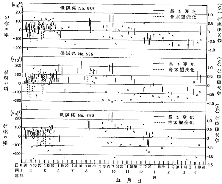
図-19 コンクリート供試体の長さ変化と含水量変化 (試験舗装 No.1)
