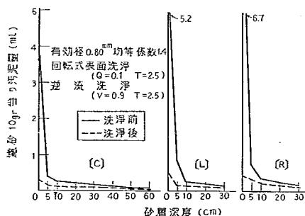
図-60B 洗浄前後の砂層深度別汚泥量
