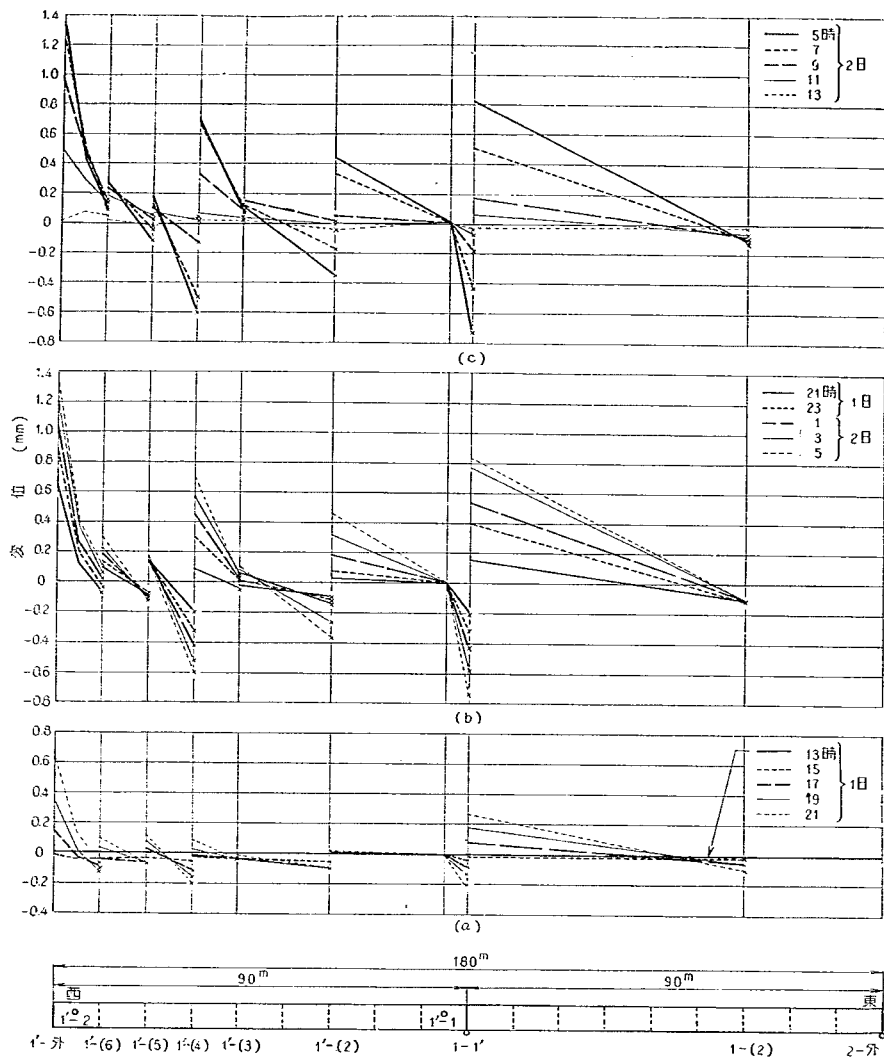
図-51 各時刻におけるコンクリート版各点の変位 (試験舗装 No.1, No.1', 35年6月)
