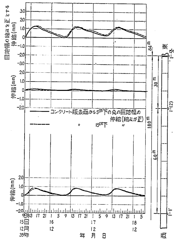
図-91 目地幅伸縮の日変化 (試験舗装 No. 1)
