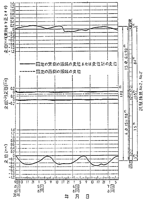
図-40 コンクリート版変位の日変化 (試験舗装 No. 2, No. 2')
