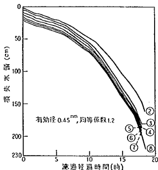
図-32B 1号池の損失水頭
