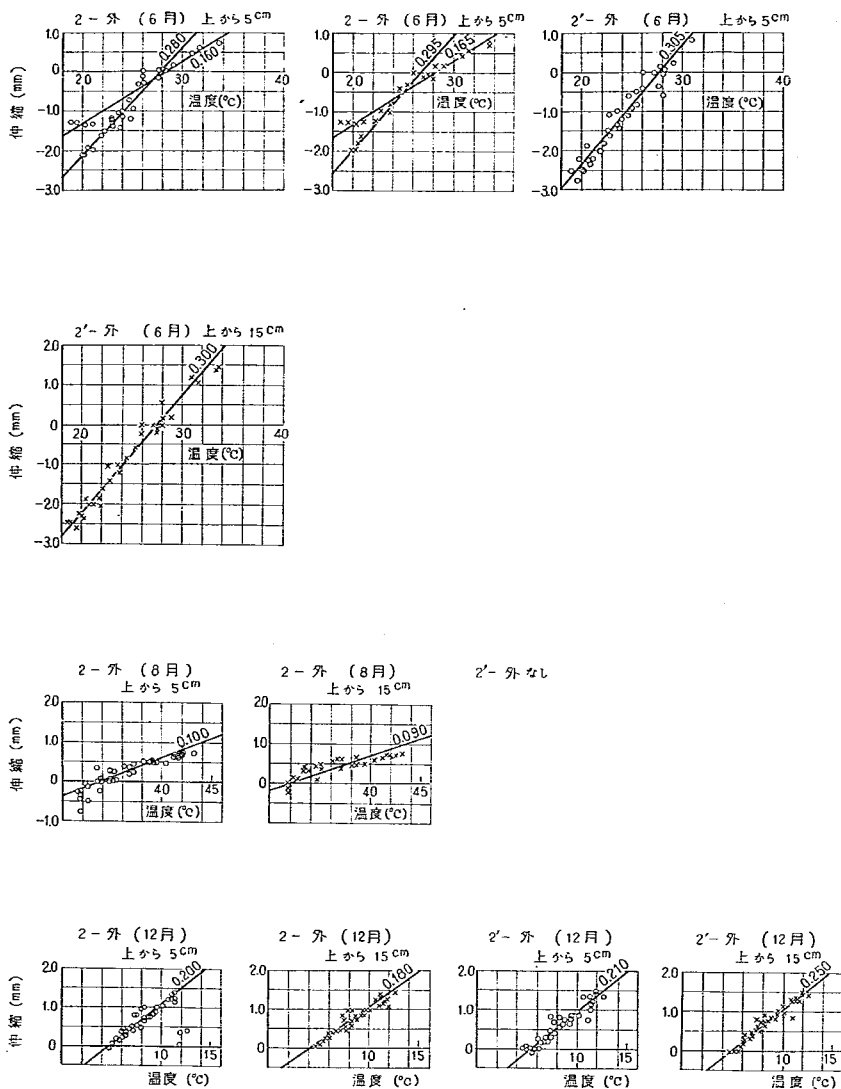
図-101 日変化における膨脹目地伸縮と温度の関係 (試験舗装 No.2)
