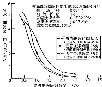
図-43 表面洗浄時間と洗浄排水汚泥量の関係
