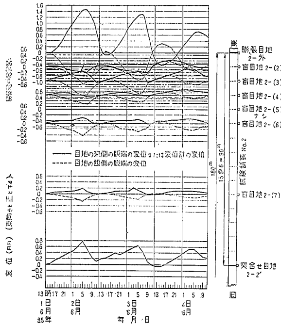
図-42 コンクリート版変位の日変化 (試験舗装 No.2)
