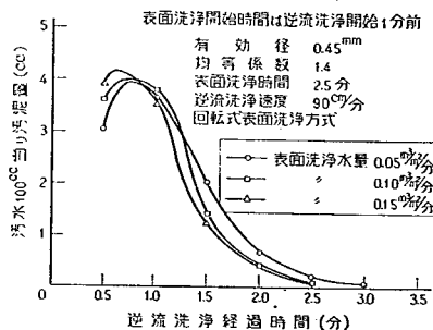
図-51 表面洗浄水量と洗浄排水汚泥量の関係
