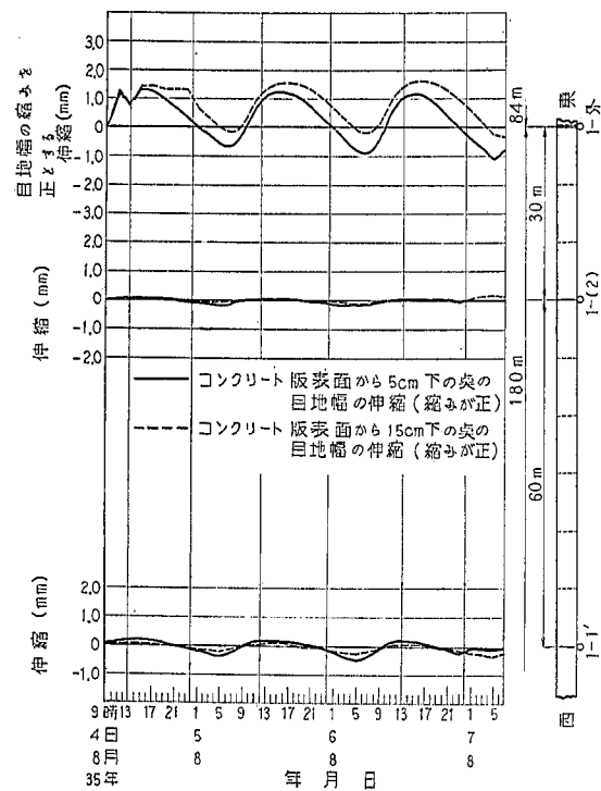
図-90 目地幅伸縮の日変化 (試験舗装 No. 1)
