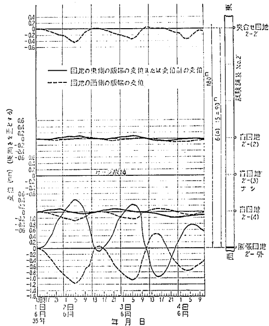
図-45 コンクリート版変位の日変化 (試験舗装 No. 2')
