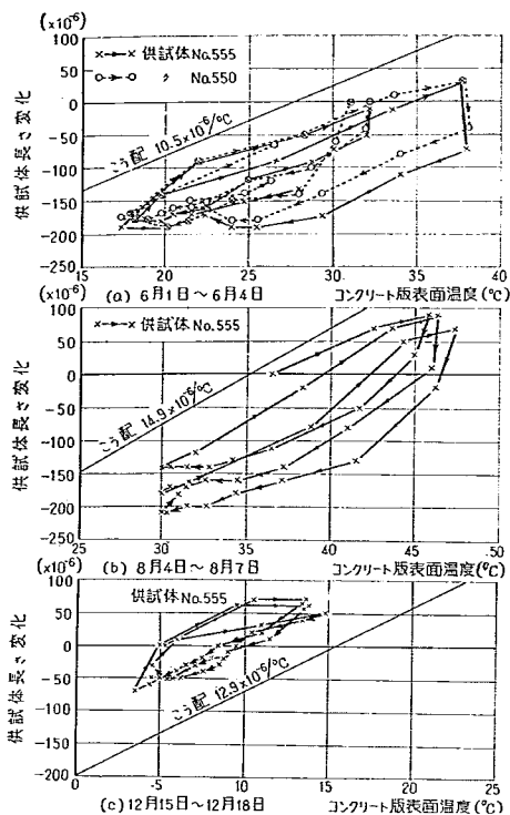
図-18 72時間連続観測における供試体長さ変化とコンクリート版表面温度の関係
