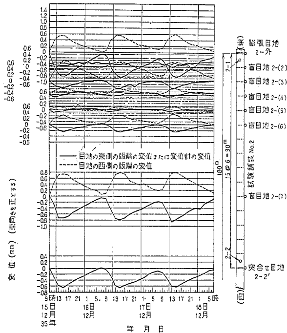
図-44 コンクリート版変位の日変化 (試験舗装 No. 2)
