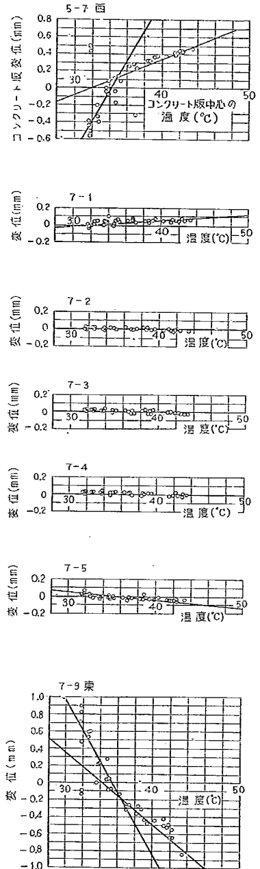
図-67 日変化におけるコンクリート版変位と温度の関係 (試験舗装 No.7, 8月)
