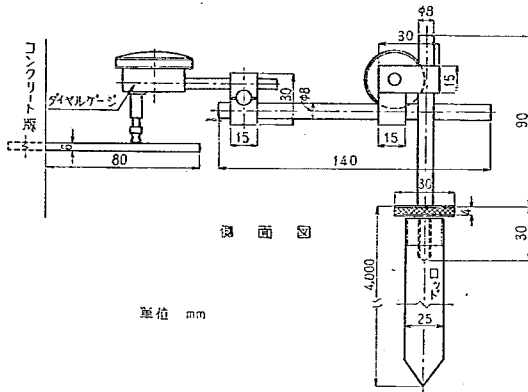
図-7 そり計詳細図
