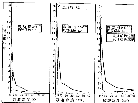
図-11 洗浄前後の砂層深度別汚泥量 (沈源池を付けない場合)
