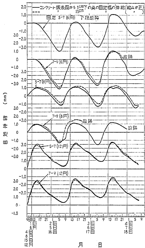
図-98 膨張目地幅伸縮の日変化 (試験舗装 No. 7)
