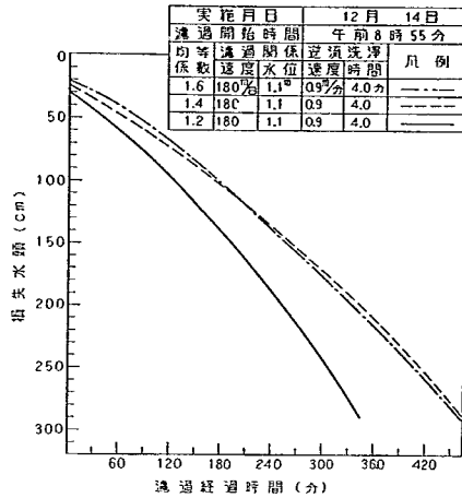
図-29A 損失水頭 (有効径 0.45 mm) の比較図
