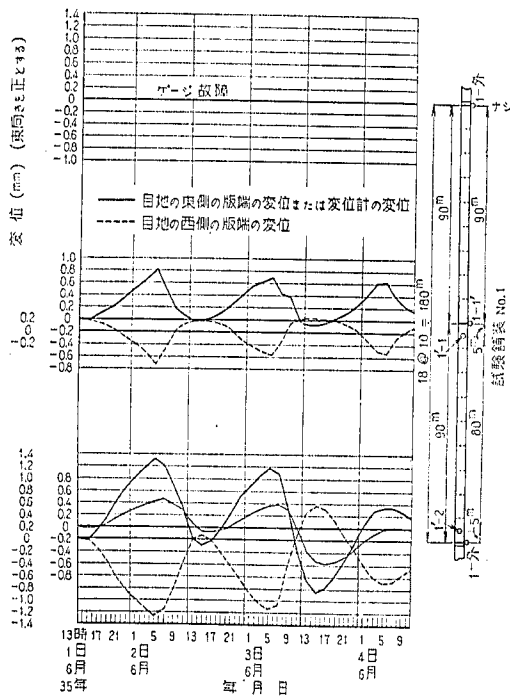
図-30 コンクリート版変位の日変化（試験舗装 No.1）
