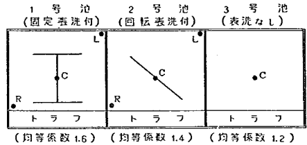
図-57 逆洗砂採取位置
