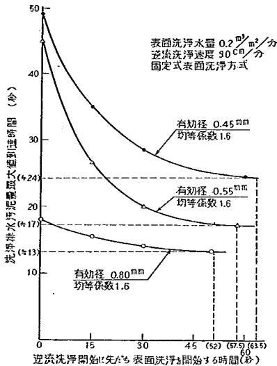
図-36 表面洗浄の開始時間
