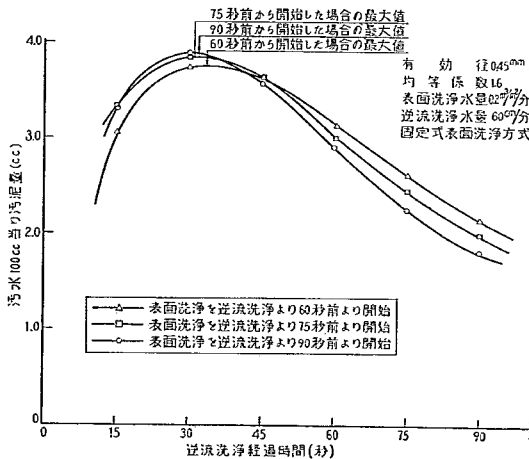
図-37 表面洗浄開始時間と洗浄排水汚泥量の関係
