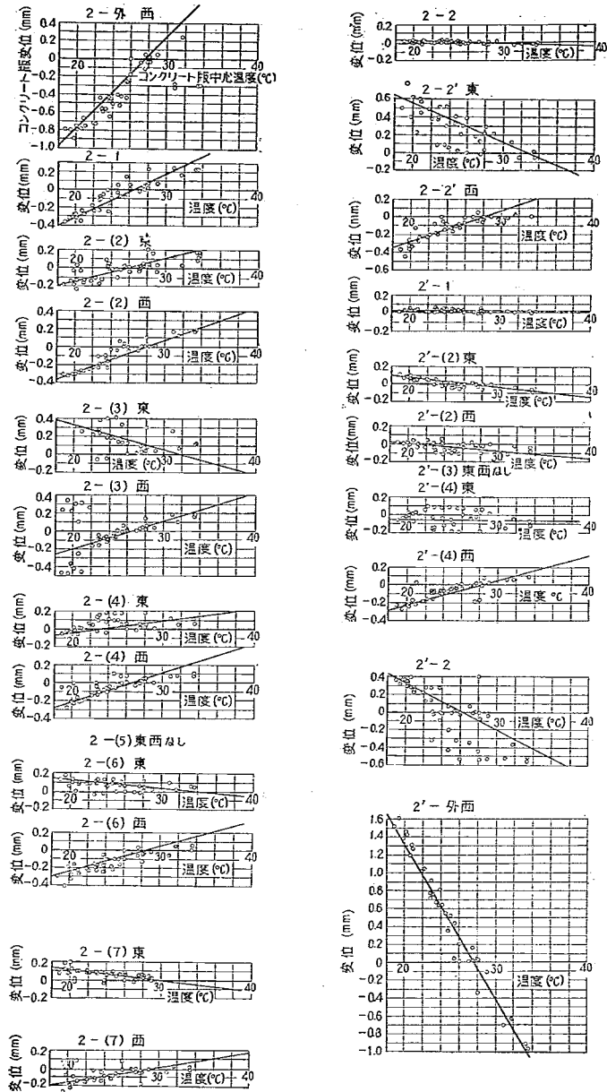
図-63 日変化におけるコンクリート版変位と温度の関係 (試験舗装 No.2, 6月)
