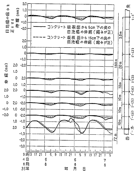
図-92 目地幅伸縮の日変化 (試験舗装 No.1')
