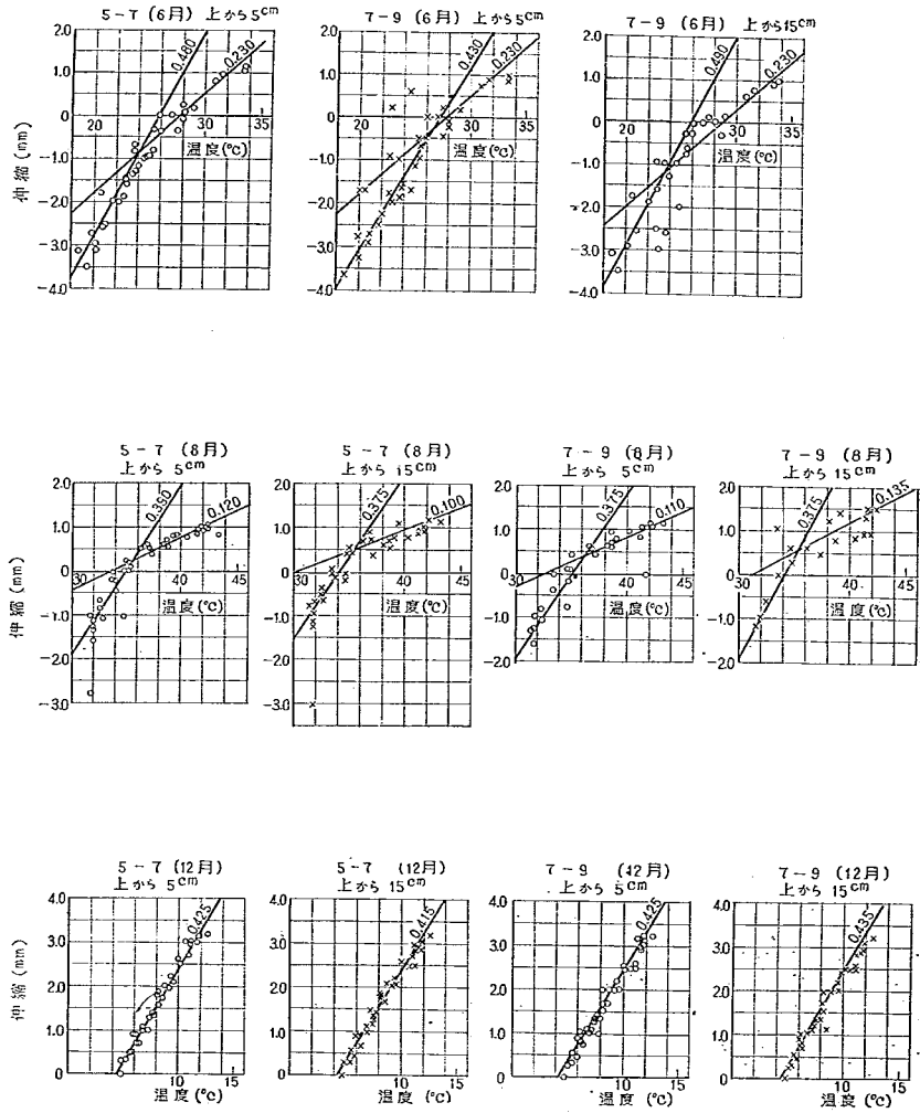
図-102 日変化における膨張目地伸縮と温度の関係 (試験舗装 No.7)
