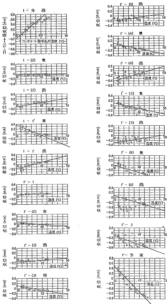
図-61 日変化におけるコンクリート版変位と温度の関係 (試験構築 No.1, 8月)
