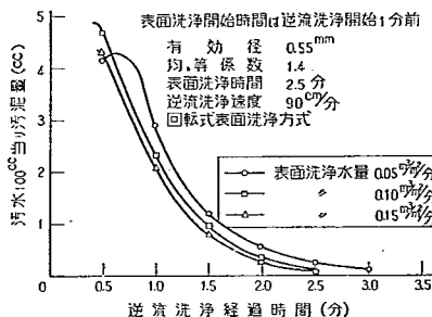
図-52 表面洗浄水量と洗浄排水汚泥量の関係
