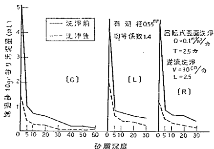
図-59B 洗浄前後の砂層深度別汚泥量
