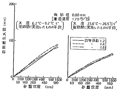
図-20 初期損失水頭
