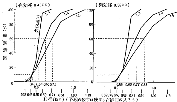
図-2 A 濕過砂の篩分け曲線
