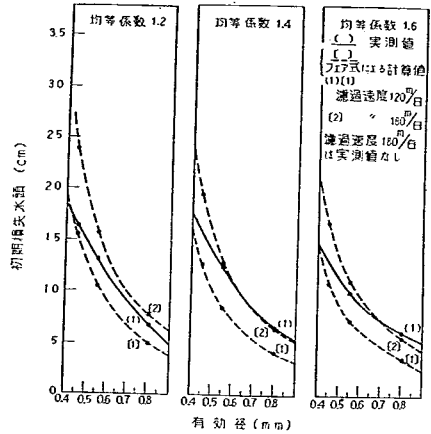
図-27 初期損失水頭の実測値とフェア式による計算値（成層 20°C）
