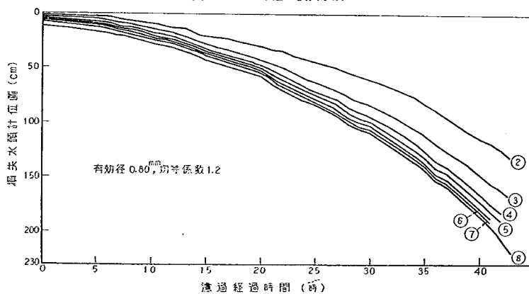
図-30D 3号池の損失水頭
