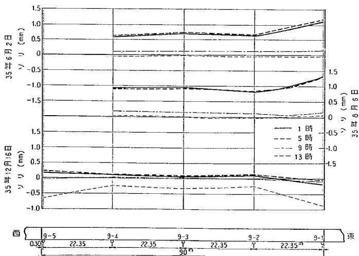
図-119 膨張目地間隔90mの連続鉄筋コンクリート版の見掛上のそりと位置の関係
