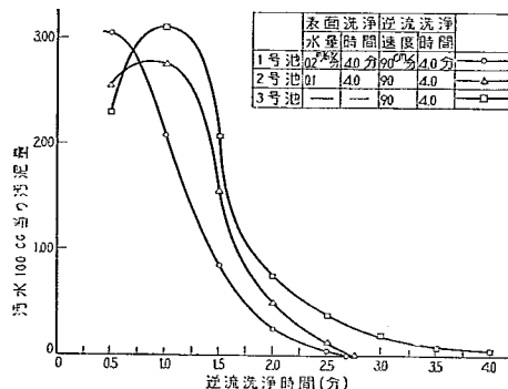
図-41 逆流洗浄のみの場合と表面洗浄併用の場合との洗浄排水汚泥量の比較
