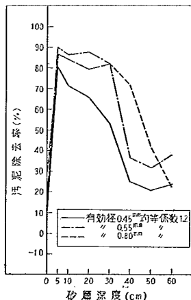
図-13 砂層深度別の汚泥量除去百分率量 (図-11の場合)
