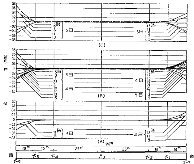
図-58 各時刻におけるコンクリート版各点の変位 (試験舗装 No. 7, 35年 8月)
