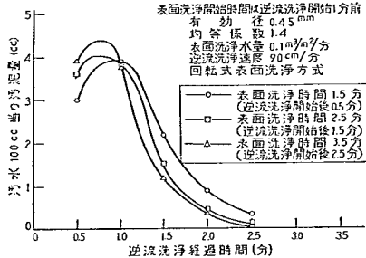
図-48 表面洗浄時間と洗浄排水汚泥量の関係
