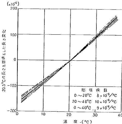
図-10 水中に養生したコンクリート供試体の膨張係数
