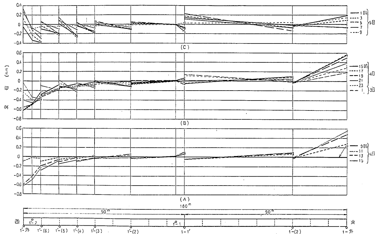
図-52 各時刻におけるコンクリート版各点の変位 (試験舗装 No.1, No.1', 35年8月)
