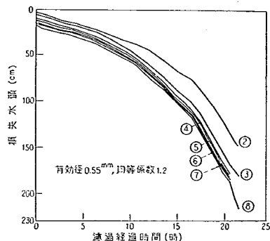
図-32C 2号池の損失水頭
