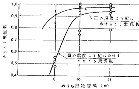
図-122 実測値から求めたコンクリート版のそり変形係数
