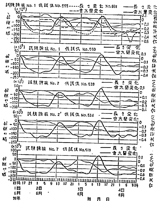
図-15 コンクリート供試体の長さ変化と含水量変化(6月・日変化)
