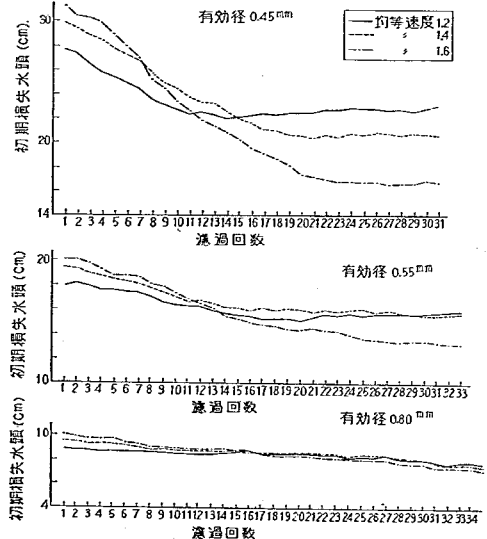
図-17 初期損失水頭 (砂面下 560 mm のもの)
