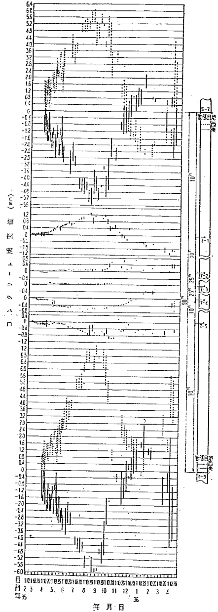
図-76 コンクリート版変位の年変化 (試験舗装 No. 7)
