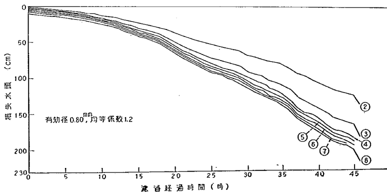
図-32D 3号池の損失水頭
