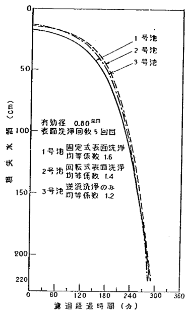
図-73A 損失水頭の比較
