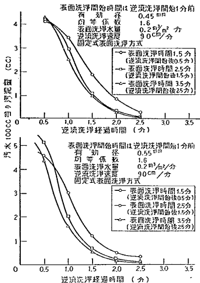
図-42 表面洗浄時間と洗浄排水汚泥量の関係
