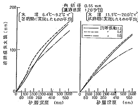
図-19 初期損失水頭
