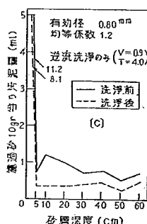
図-60C 洗浄前後の砂層深度別汚泥量
