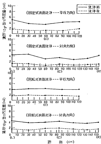
図-64 砂層表層部の汚泥分布 (有効径 0.45 mm)
