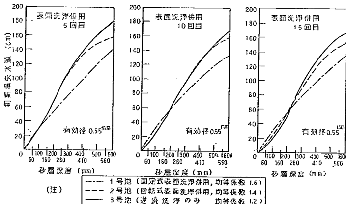
図-68 初期損失水頭の推移
