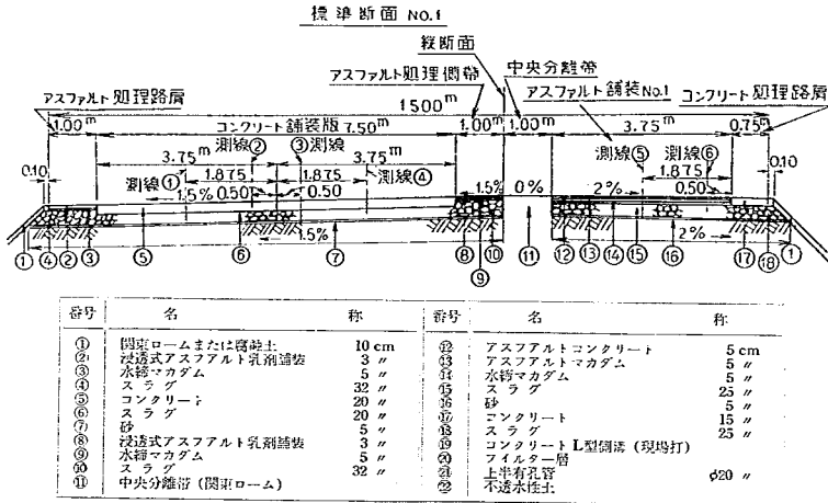
図-3 交通試験路標準断面図 No.1
