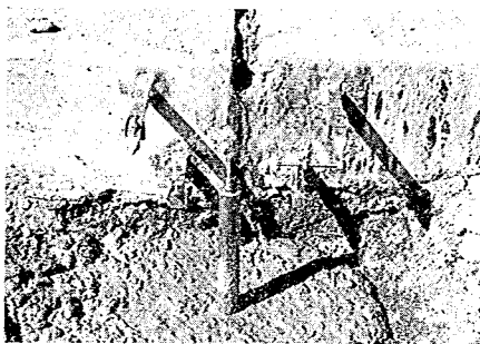
写真-8 伸縮計のロッドと鋼棒
