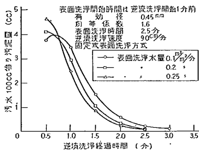
図-45 表面洗浄水量と洗浄排水汚泥量の関係
