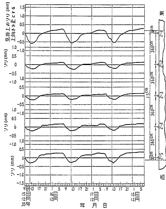
図-114 めくら日地間隔15mのコンクリート版の見掛上のそりの日変化
