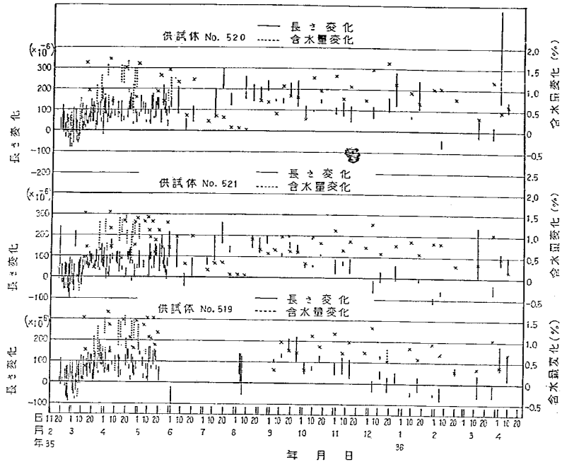
図-23 コンクリート供試体の長さ変化と含水量変化 (試験舗装 No. 7)
