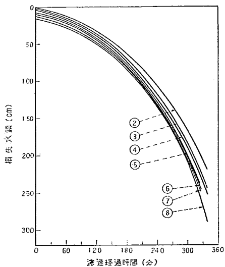
図-28B 損失水頭 (均等係数 1.6)
