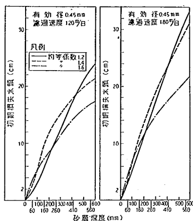
図-18 初期損失水頭
