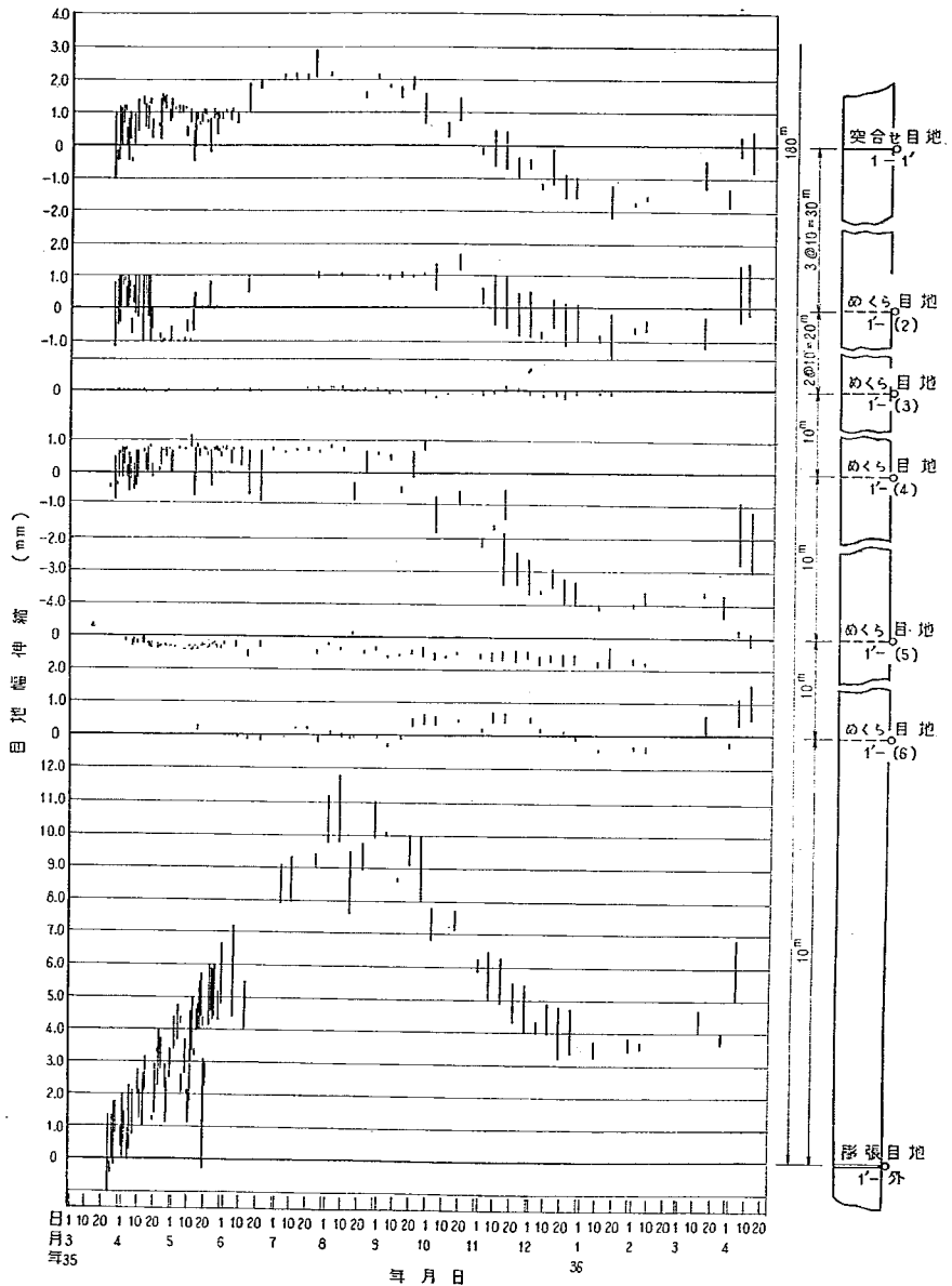
図-104 目地幅伸縮の年変化 (試験舗装 No.1')
