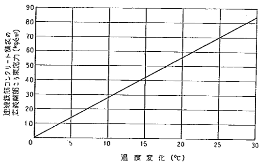
図-111 コンクリート版の広義端部こう東応力
