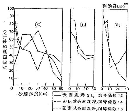
図-63 砂層の洗浄による汚泥の除去率
