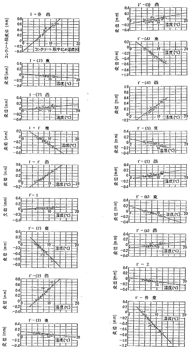
図-62 日変化におけるコンクリート版変位と温度の関係 (試験舗装 No.1, 12月)
