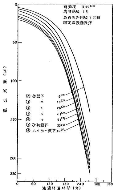
図-71B 1号池における損失水頭の変化
