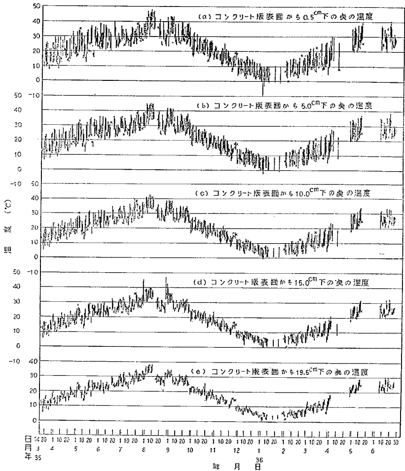
図-12 コンクリート版温度の年変化 (鉛直線は8時半の温度と13時半の温度を結んだもの)
