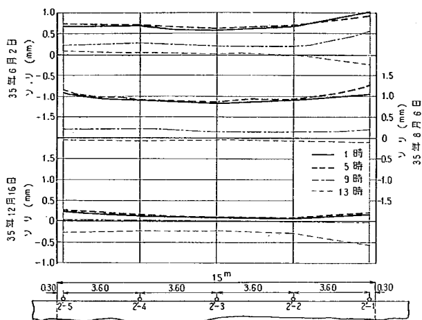
図-118 めくら目地間隔15mのコンクリート版の見掛上のそりと位置の関係
