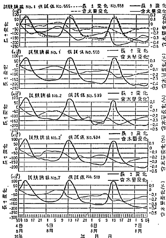
図-16 コンクリート供試体の長さ変化と含水量変化(8月・日変化)
