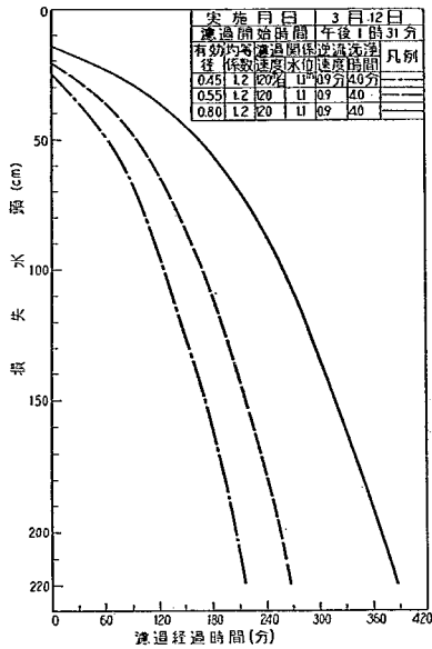
図-31A 損失水頭の比較
