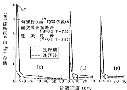
図-60A 洗浄前後の砂層深度別汚泥量
