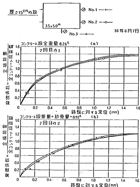
図-28 路盤摩擦係数の第2回測定値 重量変化後の測定値
