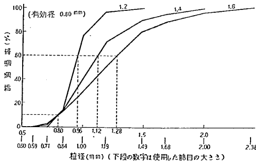
図-2 C 濾過砂の篩分け曲線
