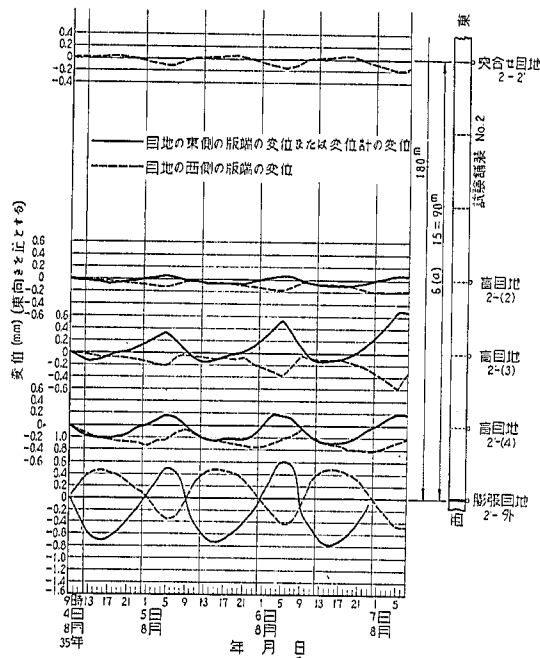
図-46 コンクリート版変位の日変化 (試験舗装 No.2')
