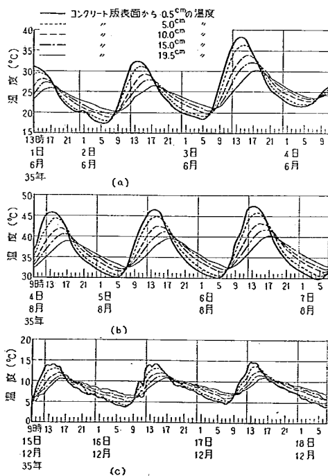
図-11 コンクリート版温度の日変化
