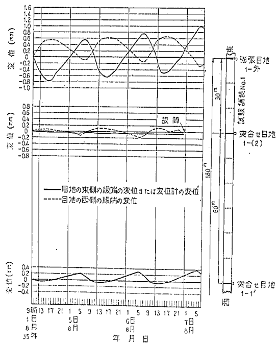
図-34 コンクリート版変位の日変化 (試験舗装 No.1)
