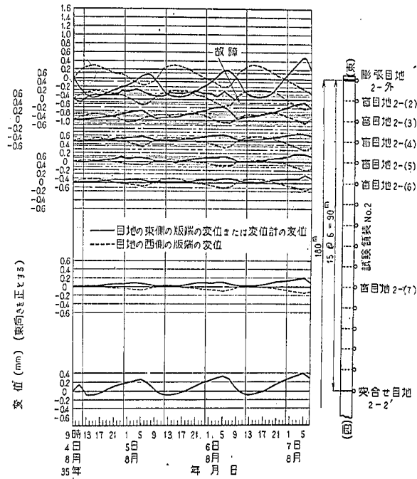
図-43 コンクリート版変位の日変化 (試験舗装 No.2)
