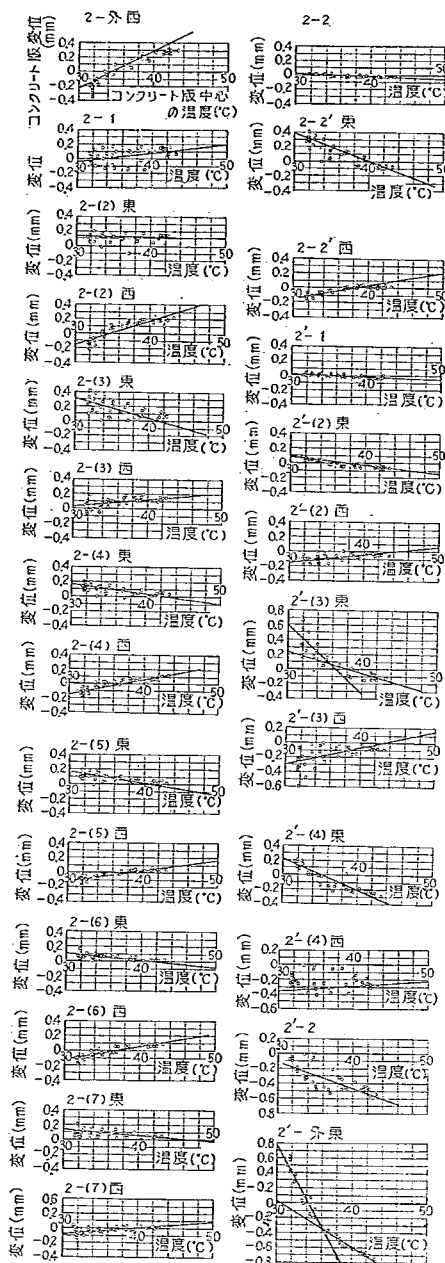
図-64 日変化におけるコンクリート版変位と温度の関係 (試験舗装 No.2, 8月)
