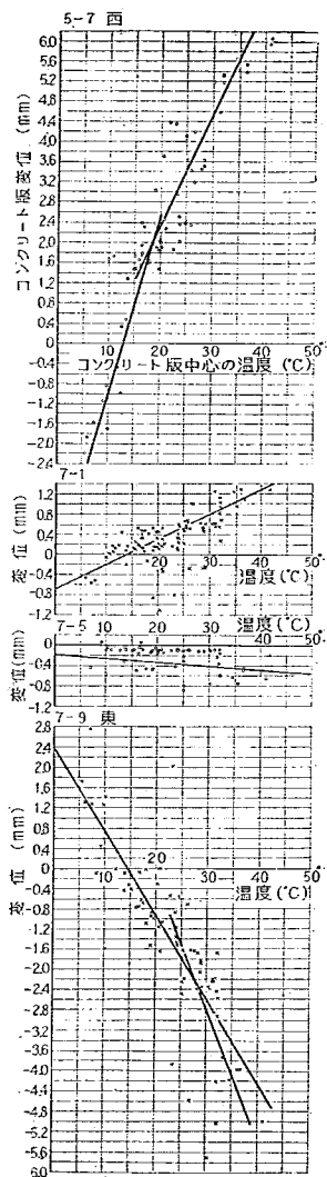
図-83 年変化におけるコンクリート版変位と温度の関係 (試験舗装 No.7)
