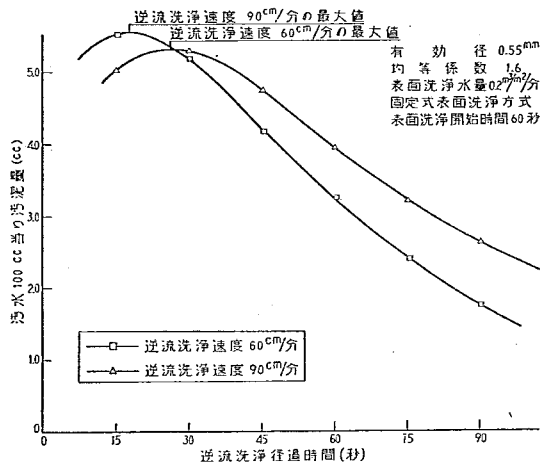
図-39 表面洗浄開始時間と洗浄排水汚泥量の関係
