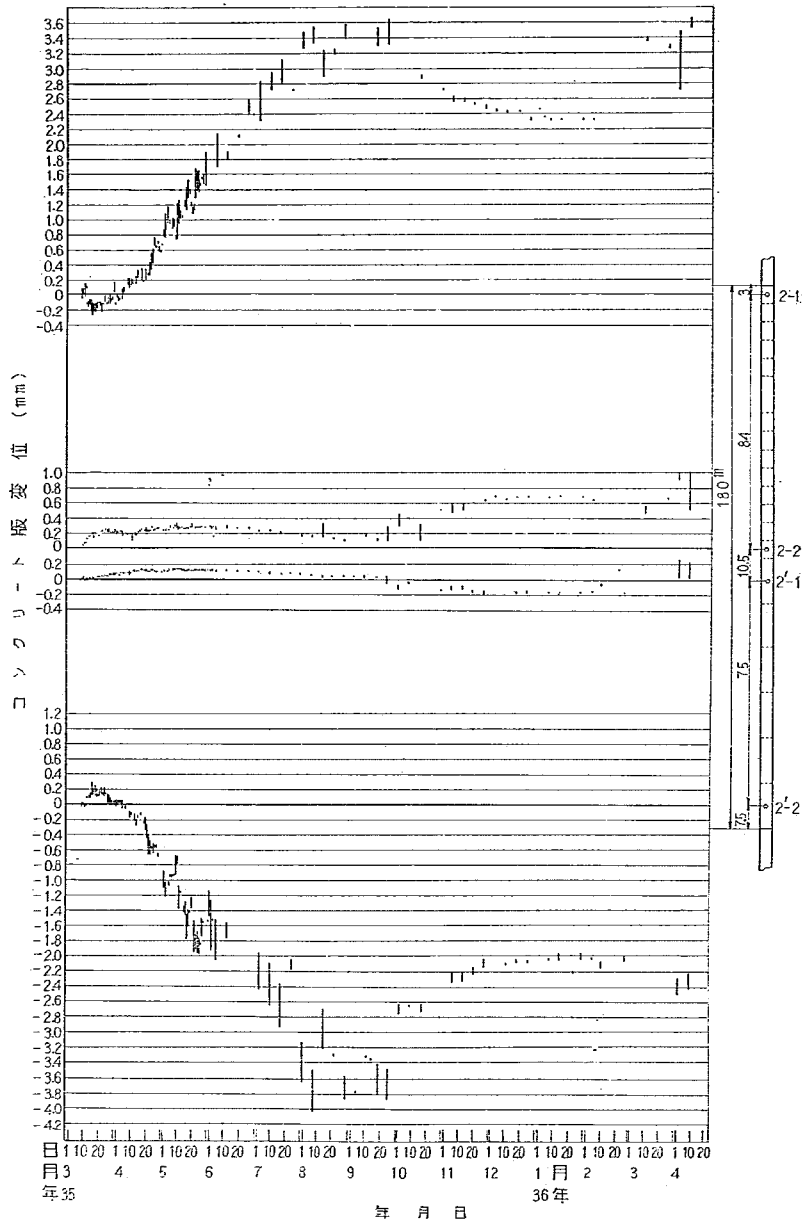
図-73 コンクリート版変位の年変化 (試験筋装 No.2)
