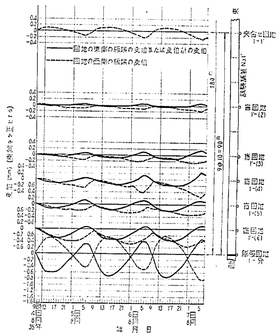
図-37 コンクリート版変位の日変化 (試験舗装 No.1)
