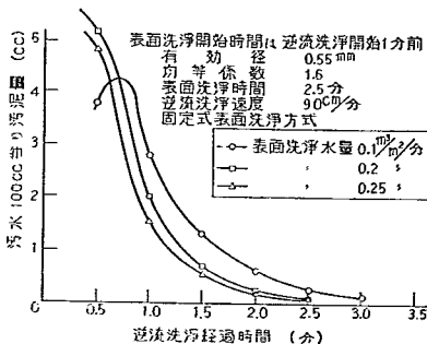
図-46 表面洗浄水量と洗浄排水汚泥量の関係
