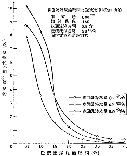
図-47 表面洗浄水量と洗浄排水汚泥量の関係
