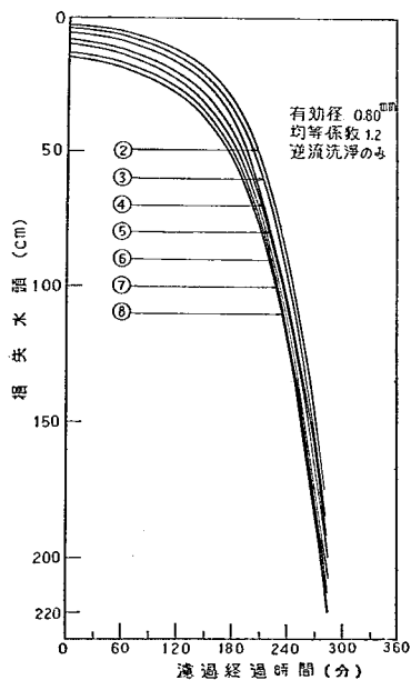
図-73D 3号池における損失水頭の変化
