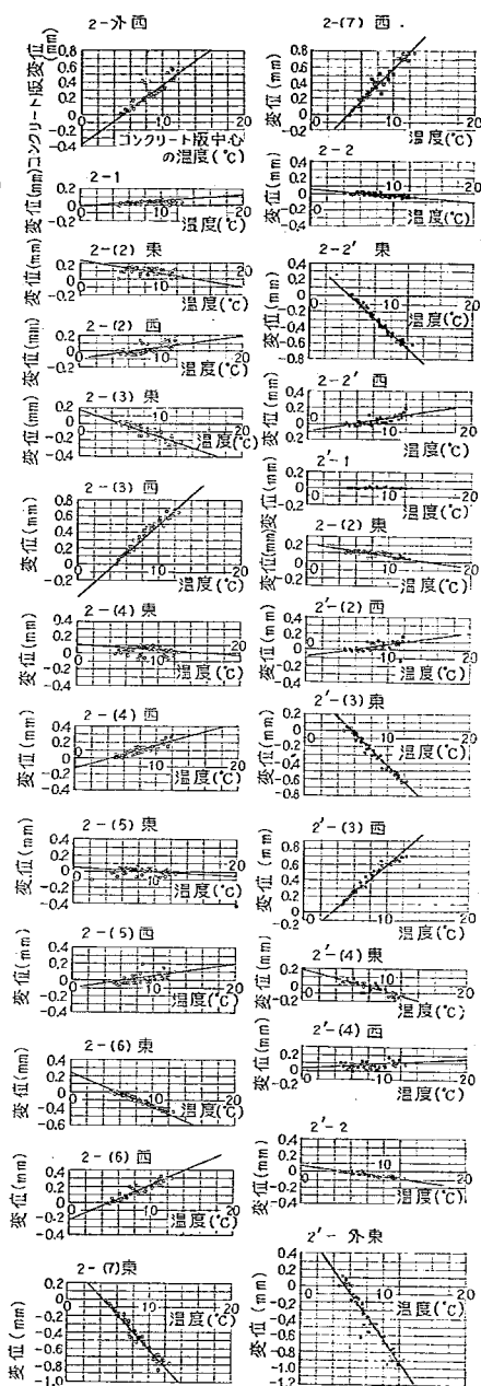
図-65 日変化におけるコンクリート版変位と温度の関係 (試験舗装 No.2, 12月)
