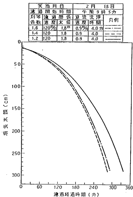
図-28A 損失水頭 (有効径 0.80 mm) の比較図
