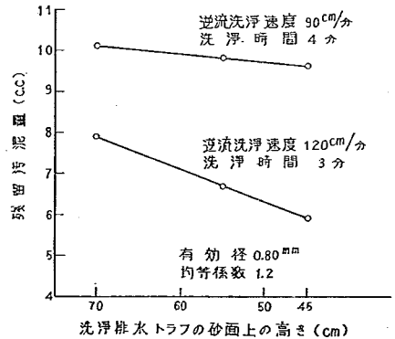
図-16 洗浄排水トラフの高さと残留汚泥量
