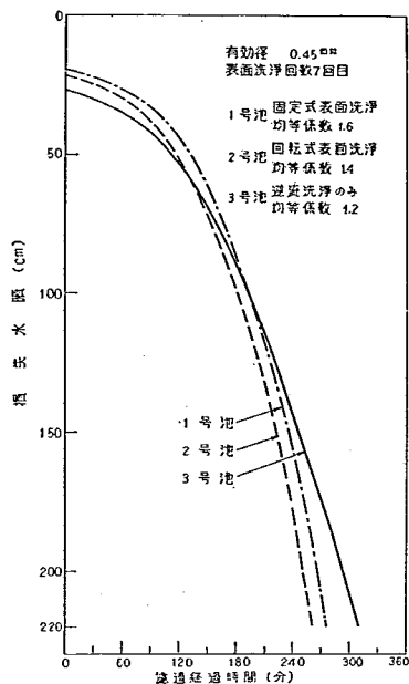
図-71A 損失水頭の比較
