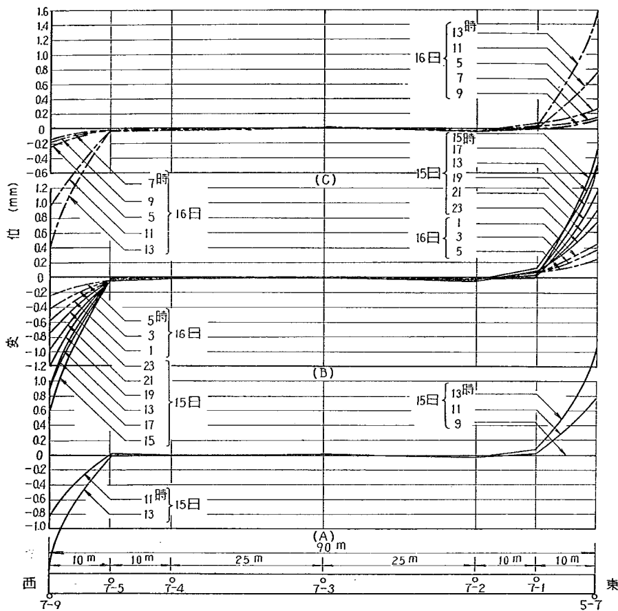
図-59 各時刻におけるコンクリート版各点の変位 (試験編號 No.7, 35年12月)
