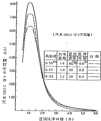
図-5 逆流洗浄時における洗浄排水の時間的変化
