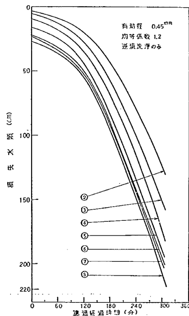
図-71D 3号池における損失水頭の変化
