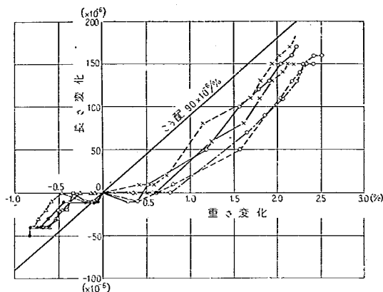
図-26 コンクリート供試体の含水量変化と長さ変化の関係
