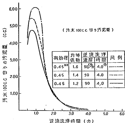
図-10 逆流洗浄時における洗浄排水の時間的変化
