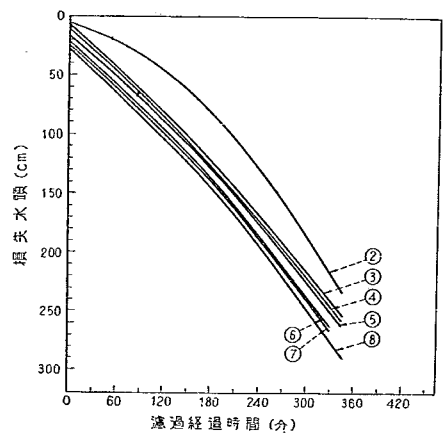
図-29D 損失水頭 (均等係数 1.2)
