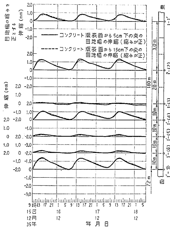
図-93 目地幅伸縮の日変化 (試験舗装 No.1')
