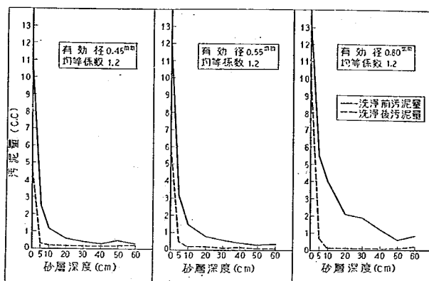
図-12 洗浄前後の砂層深度別汚泥量 (前処理としてアクセレータ使用)
