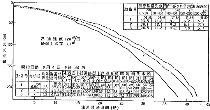
図-30A 損失水頭の比較
