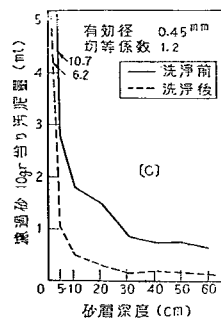
図-58C 洗浄前後の砂層深度別汚泥量
