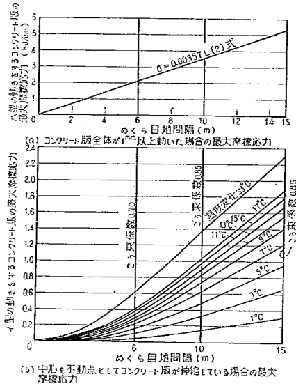
図-85 コンクリート版の最大摩擦応力度
