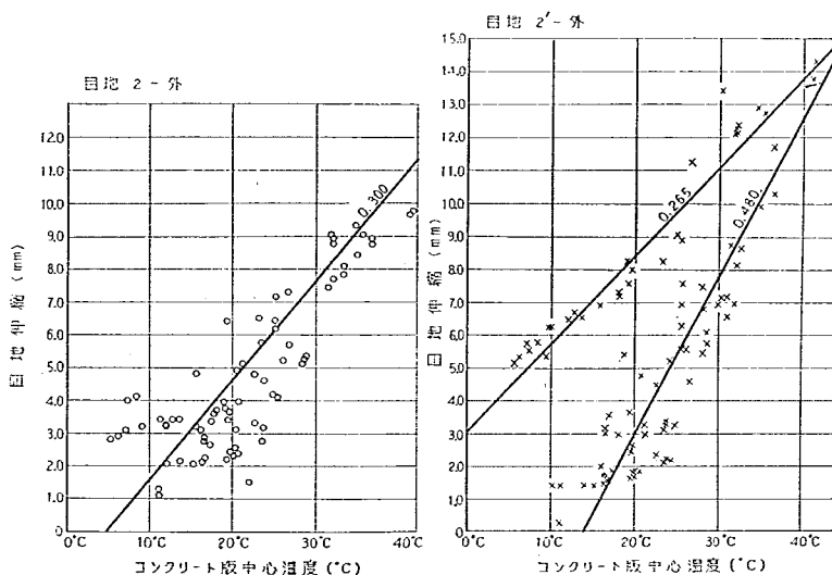
図-109 年変化における膨脹目地伸縮と温度の関係 (試験舗装 No.2)
