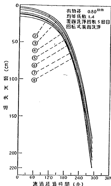
図-73C 2号池における損失水頭の変化
