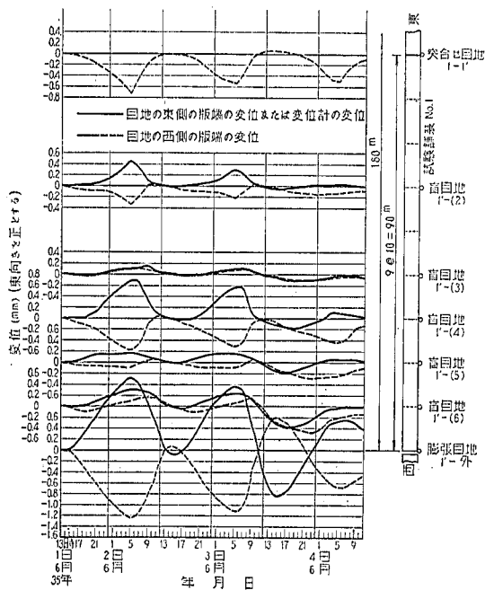
図-36 コンクリート版変位の日変化 (試験舗装 No.1)
