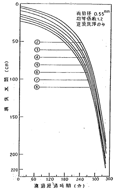
図-72D 3号池における損失水頭の変化
