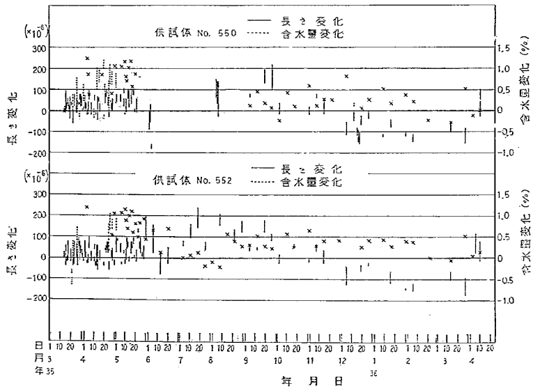
図-20 コンクリート供試体の長さ変化と含水量変化 (試験舗装 No.1')
