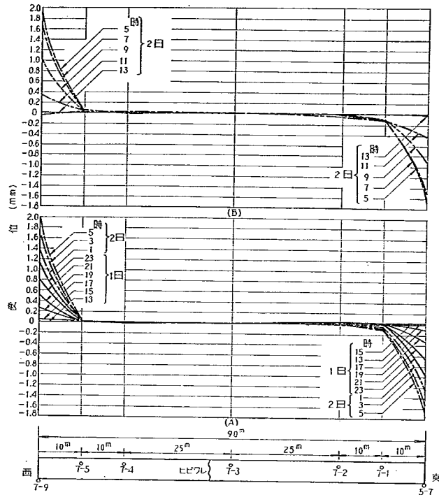
図-57 各時刻におけるコンクリート版各点の変位 (試験舗装 No. 7, 35年 6月)
