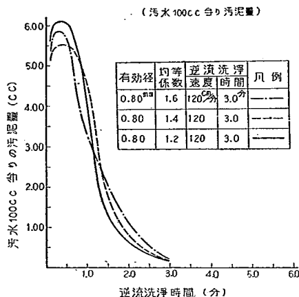
図-8 逆流洗浄時における洗浄排水の時間的変化
