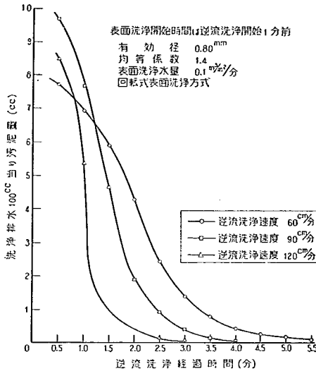
図-56 表面洗浄併用時の逆洗洗浄速度と洗浄排水汚泥量の関係
