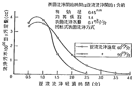
図-54 表面洗浄併用時の逆流洗浄速度と洗浄排水汚泥量の関係
