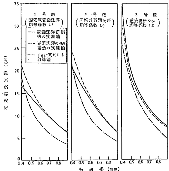
図-70 表面洗浄併用前後の初期損失水頭の変化
