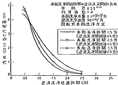
図-49 表面洗浄時間と洗浄排水汚泥量の関係
