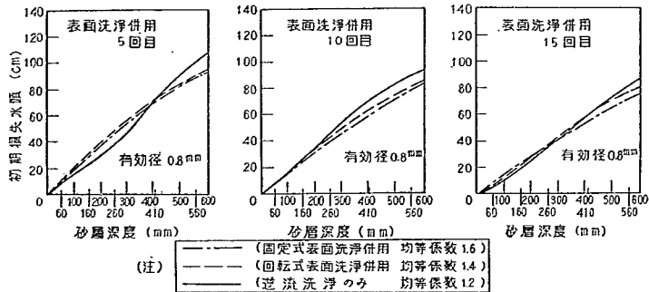
図-69 初期損失水頭の推移
