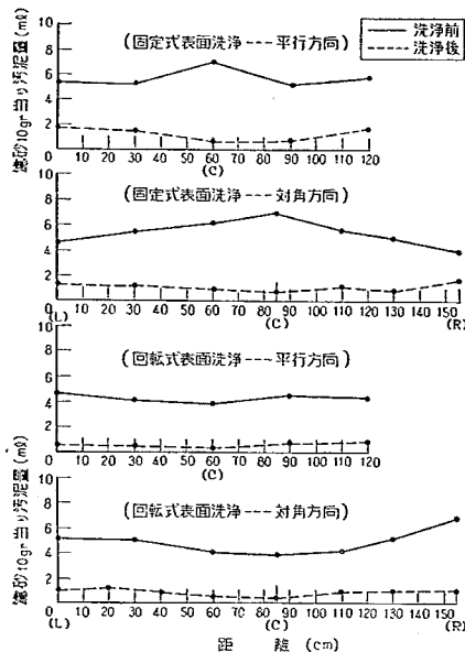
図-66 砂層表層部の汚泥分布 (有効径 0.80 mm)
