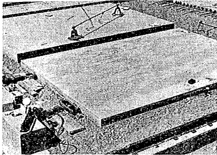
写真-1 3.5×5mのコンクリート版の摩擦試験 (ジャッキ、ひずみリング、側面にとりつけたダイヤルゲージ)
