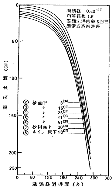
図-73B 1号池における損失水頭の変化
