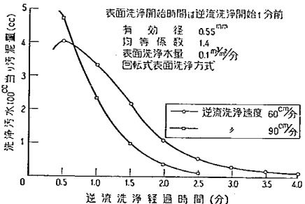
図-55 表面洗浄併用時の逆流洗浄速度と洗浄排水汚泥量の関係
