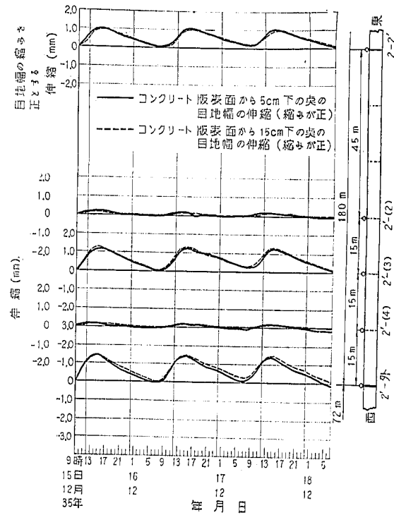
図-97 目地幅伸縮の日変化（試験舗装 No.2'）
