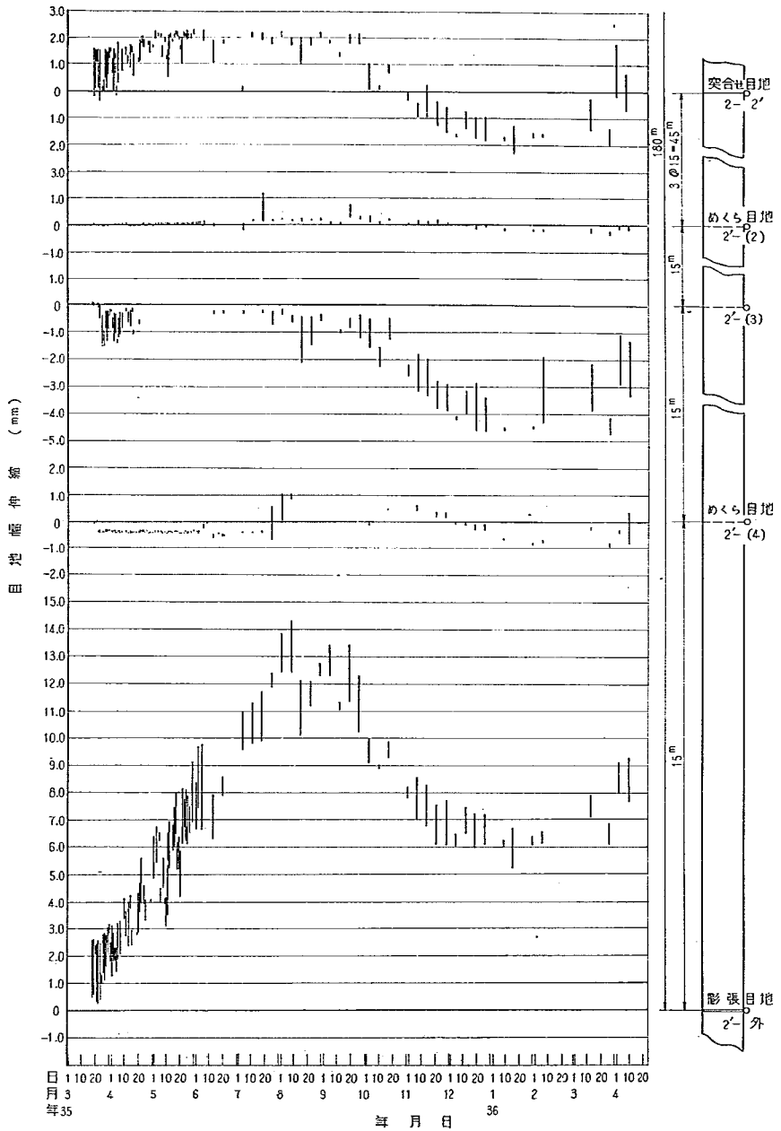
図-106 目地幅伸縮の年変化 (試験舗装 No.2')
