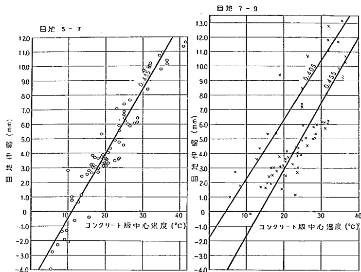
図-110 年変化における膨脹目地伸縮と温度の関係 (試験舗装 No. 7)
