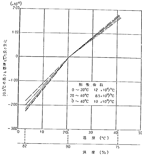
図-9 空中に養生したコンクリート供試体の膨張係数
