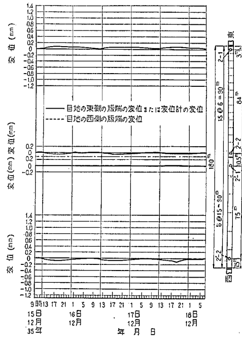
図-41 コンクリート版変位の日変化 (試験舗装 No. 2, No. 2')
