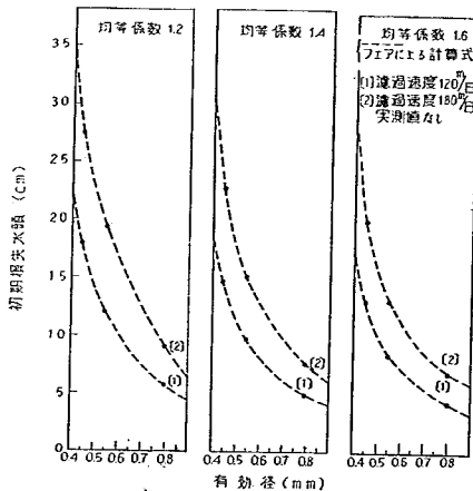
図-25 初期損失水頭のフェア式による計算値（不成層 20°C）
