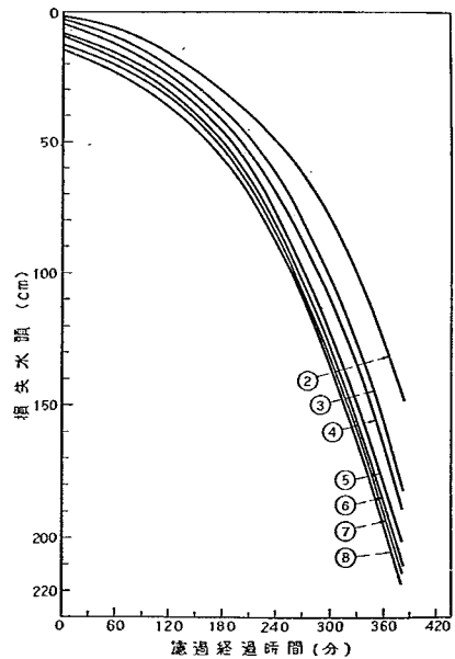
図-31D 損失水頭
