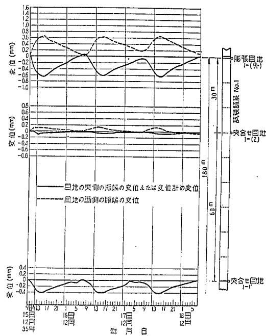
図-35 コンクリート版変位の日変化 (試験舗装 No.1)
