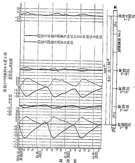
図-47 コンクリート版変位の日変化 (試験舗装 No.2')
