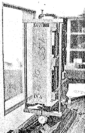
写真-12 ダイヤルゲージ法によるコンクリート供試体の長さ変化の測定
