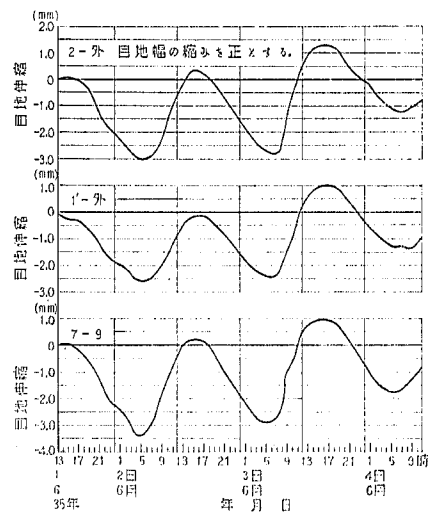
図-99 カールソン維目計による膨張目地幅伸縮 (日変化) 測定の一例
