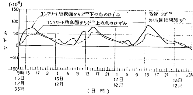
図-120 カールソンひずみ計で測定したコンクリート収縮ひずみの日変化
