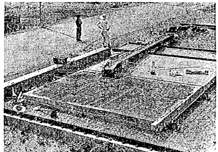
写真-3 砂を盛って重くしたコンクリート版の摩擦試験
