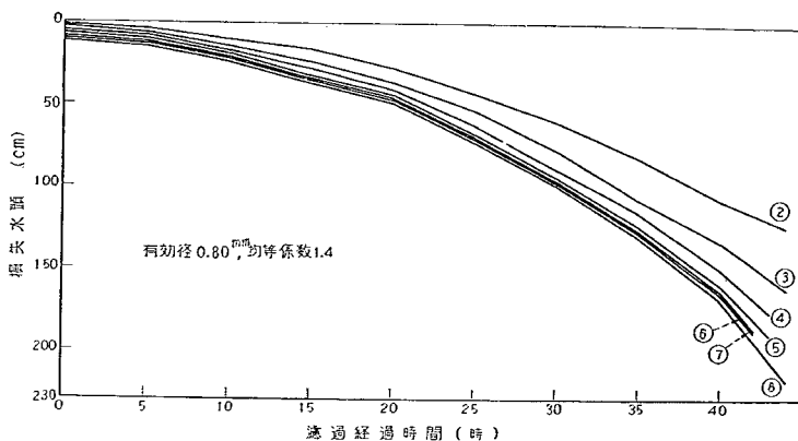
図-30C 2号池の損失水頭
