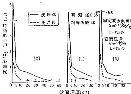
図-59A 洗浄前後の砂層深度別汚泥量
