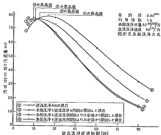
図-35 表面洗浄開始時間と洗浄排水汚泥量の関係
