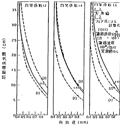
図-24 初期損失水頭の実測値とフェア式による計算値（不成層80°C）
