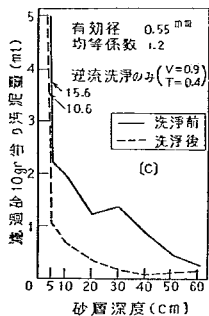
図-59C 洗浄前後の砂層深度別汚泥量
