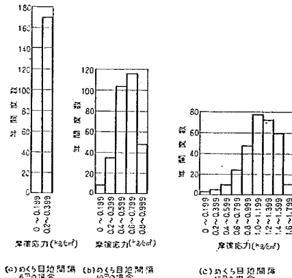
図-87 前日の昼に応力0とした場合の早朝5時ごろの摩擦応力の変数分布
