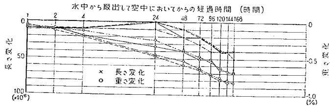
図-24 コンクリート供試体を乾燥させた場合の長さ変化と重さ変化
