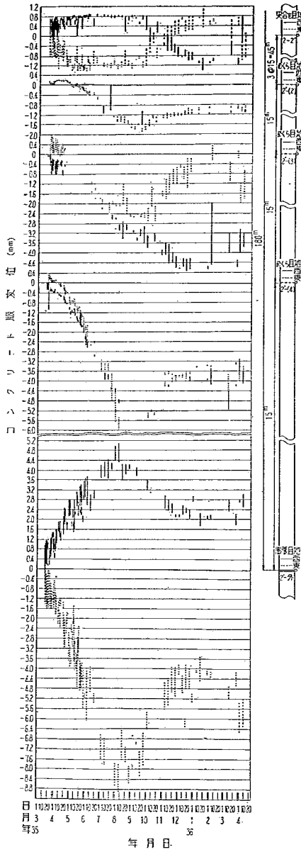
図-75 コンクリート版変位の年変化 (試験舗装 No. 2)
