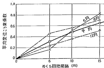
図-69 めくら目地間隔と変位係数の関係
