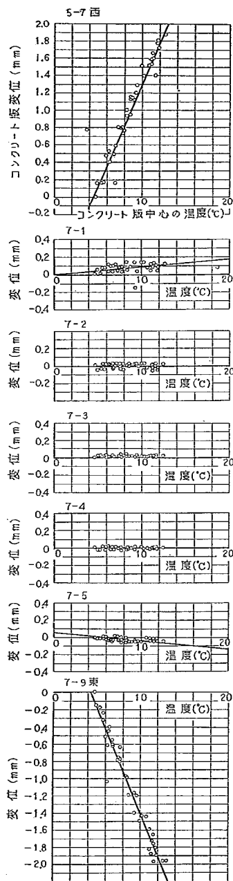
図-68 日変化におけるコンクリート版変位と温度の関係 (試験舗装 No. 7, 12月)
