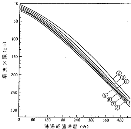
図-29B 損失水頭 (均等係数 1.6)
