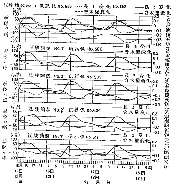
図-17 コンクリート供試体の長さ変化と含水量変化(12月・日変化)
