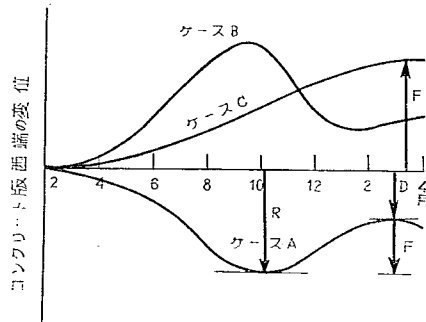
図-77 コンクリート版西端(目地の東端)変位の年変化の分類
