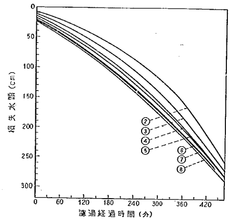
図-29C 損失水頭 (均等係数 1.4)
