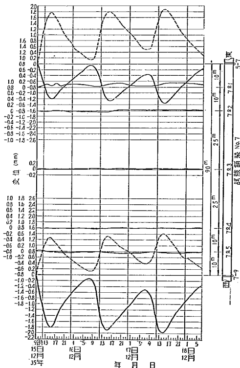
図-50 コンクリート版変位の日変化 (試験舗装 No.7)
