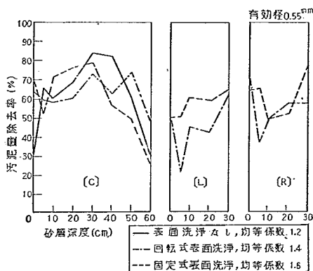
図-62 砂層の洗浄による汚泥の除去率
