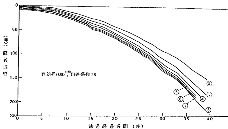
図-30B 1号池の損失水頭
