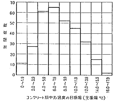
図-86 コンクリート版中心温度日振幅の度数分布
