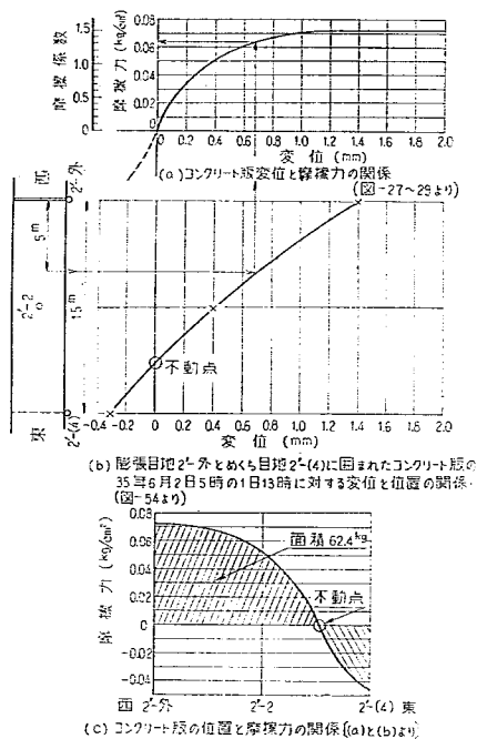
図-84 路盤摩擦力の図解法
