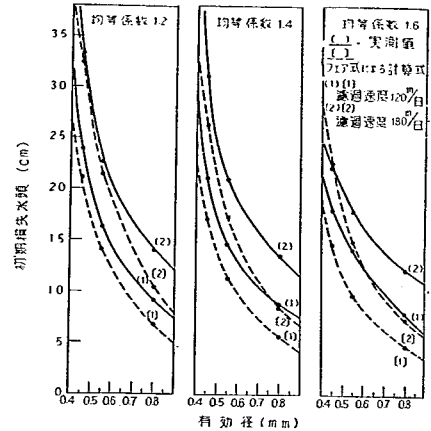
図-26 初期損失水頭の実測値とフェア式による計算値（成 8°C）
