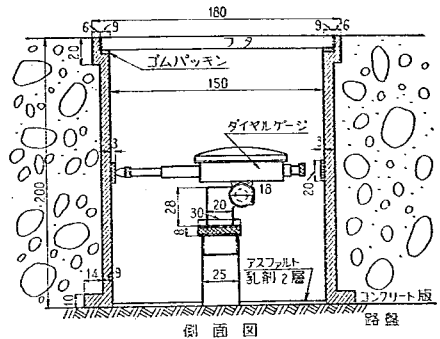
図-5 変位計詳細図
