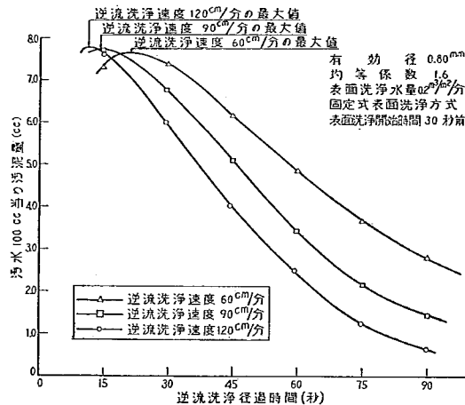
図-40 表面洗浄開始時間と洗浄排水汚泥量の関係
