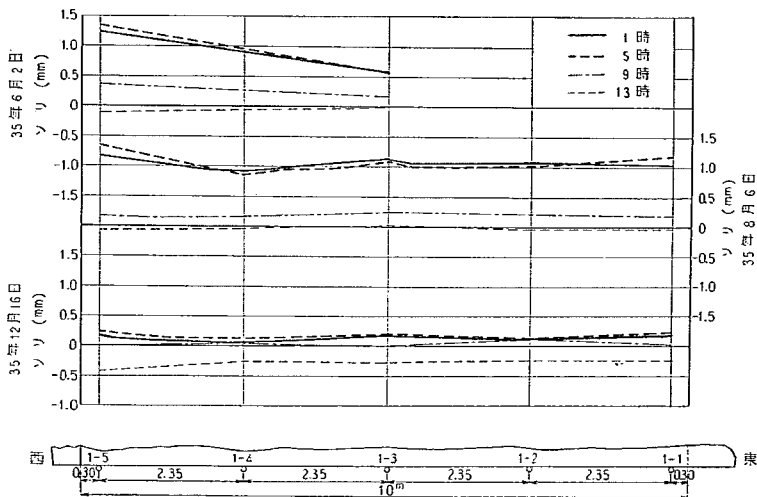
図-117 めくら目地間隔10mのコンクリート版の見掛上のそりと位置の関係
