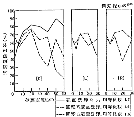
図-61 砂層の洗浄による汚泥の除去率
