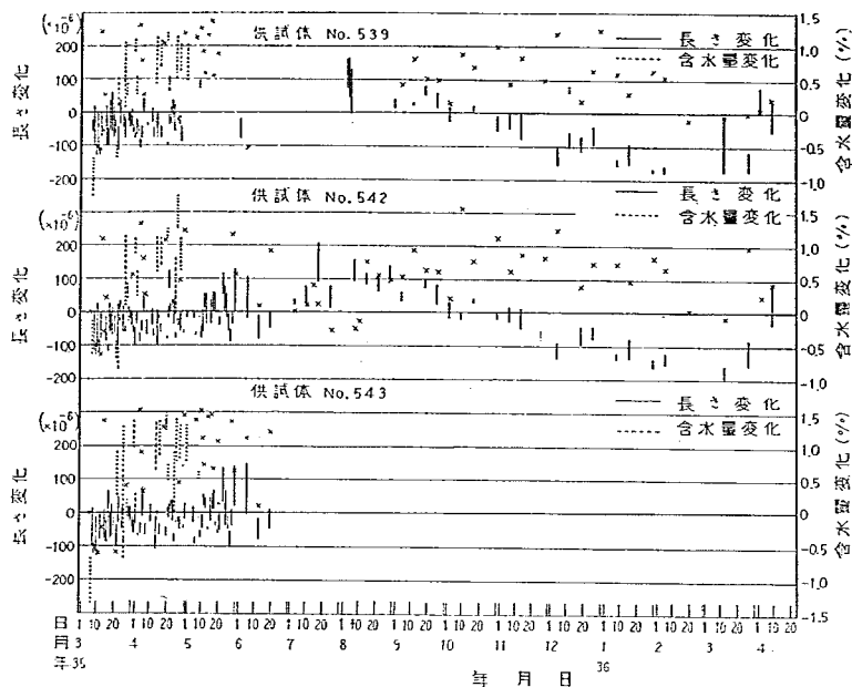
図-21 コンクリート供試体の長さ変化と含水量変化 (試験舗装 No. 2)
