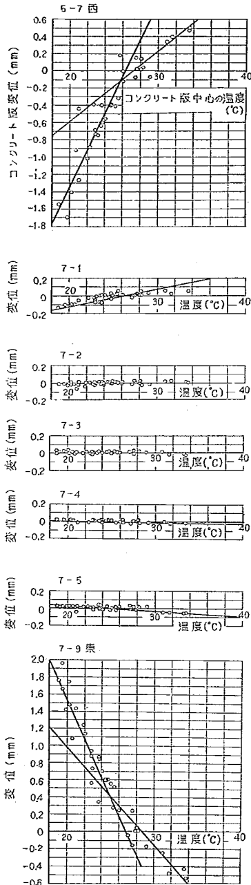
図-66 日変化におけるコンクリート版変位と温度の関係 (試験舗装 No.7, 6月)
