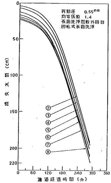
図-72C 2号池における損失水頭の変化
