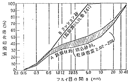
図-1 摩擦係数測定のための試験舗装の路盤材料とクッション砂の粒度
