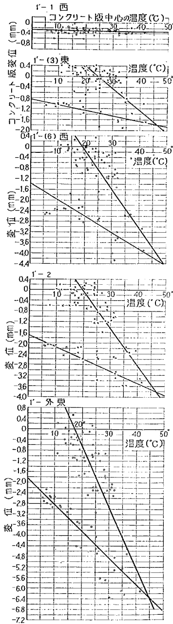
図-81 年変化におけるコンクリート版変位と温度の関係 (試験舗装 No.1)
