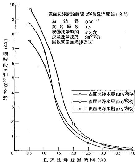
図-53 表面洗浄水量と洗浄排水汚泥量の関係
