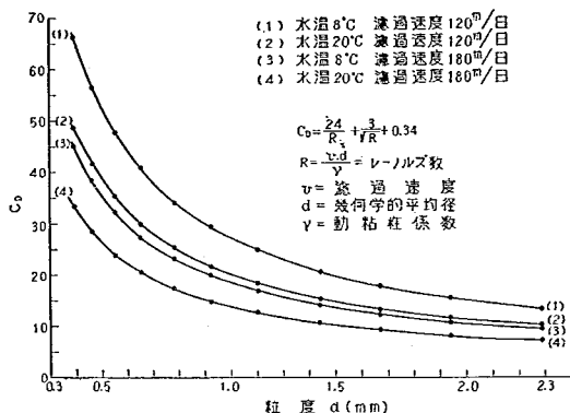
図-22 粒径と抵抗係数 C_D (成層の場合)
