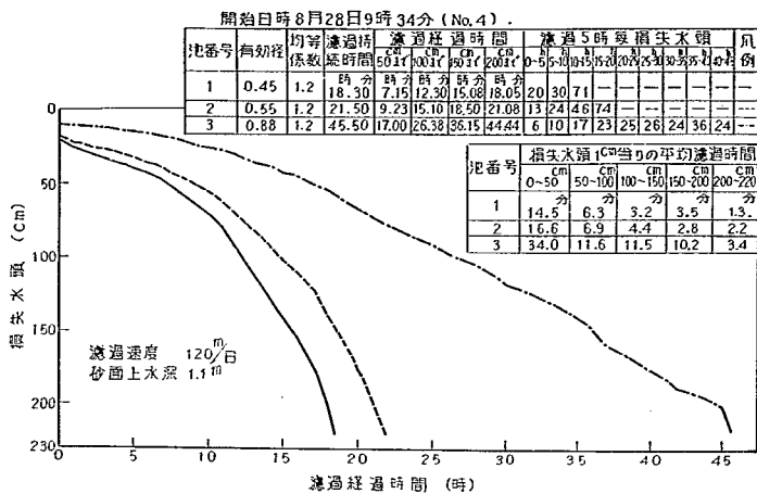
図-32A 損失水頭の比較
