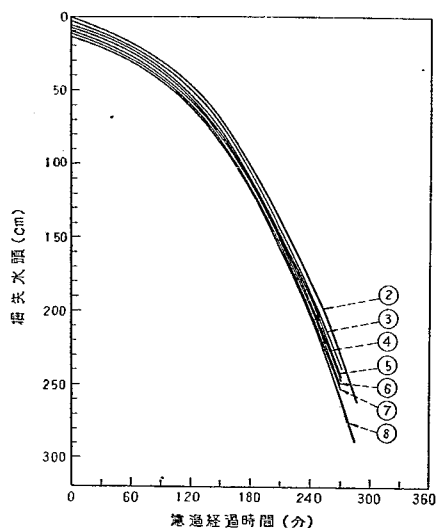
図-28C 損失水頭 (均等係数 1.4)
