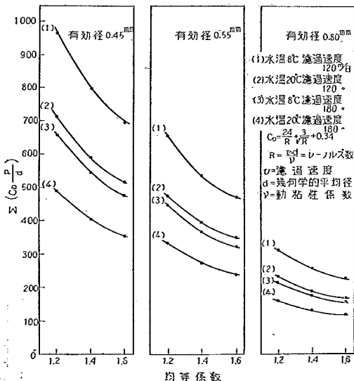
図-23 有効径別の \Sigma(C_D \frac{p}{d}) の値 (成層の場合)
