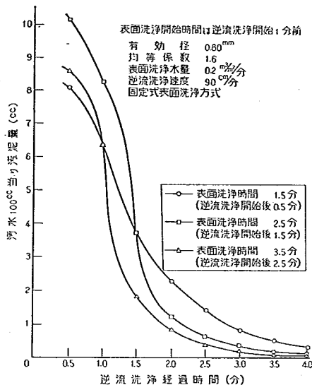
図-44 表面洗浄時間と洗浄排水汚泥量の関係
