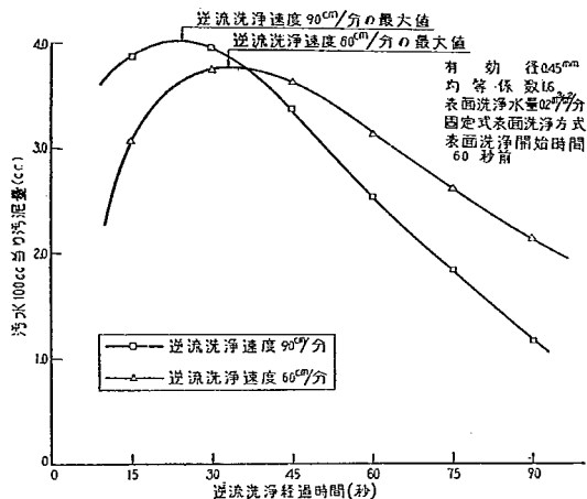
図-38 表面洗浄開始時間と洗浄排水汚泥量の関係
