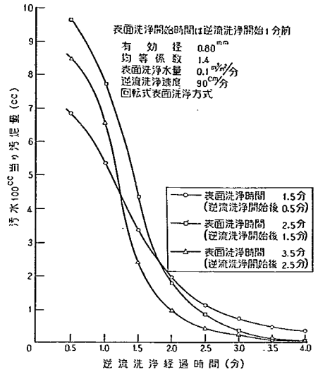
図-50 表面洗浄時間と洗浄排水汚泥量の関係
