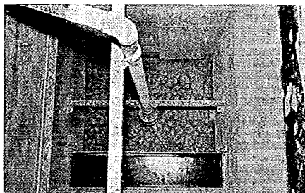
写真-5 2号池の内部（回転式表面洗浄装置付）
