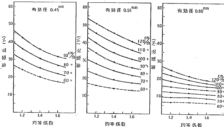
図-4 高温時における膨脹比、洗浄速度および粒径との関係 (均等係数別)
