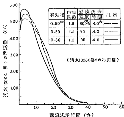
図-6 逆流洗浄時における洗浄排水の時間的変化
