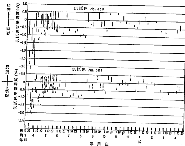
図-14 コンクリート供試体含水量の年変化
