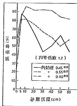
図-14 砂層深度別の汚泥除去百分率 (図-12の場合)
