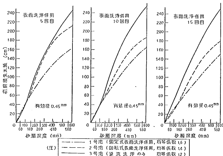
図-67 初期損失水頭の推移
