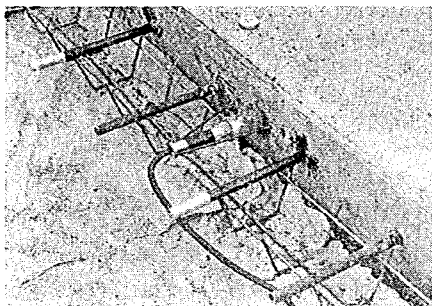
写真-11 カールソン型継目計の設置 (6mm鉄筋であらかじめ伸ばしている)
