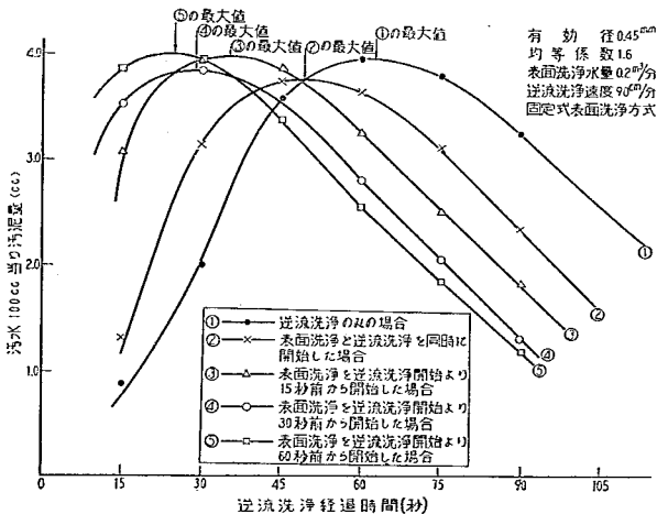
図-33 表面洗浄開始時間と洗浄排水汚泥量の関係
