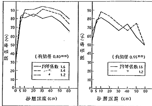
図-15A 砂層深度別汚泥量の除去百分率 (アクセレータ使用の場合)
