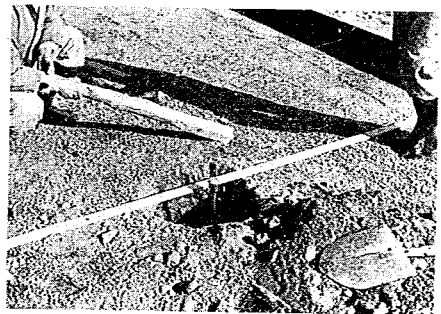
写真-4 変位計のロッドの打ち込み
