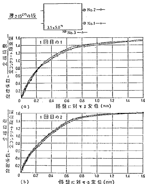
図-27 路盤摩擦係数の第1回測定値 (版厚15cm)
