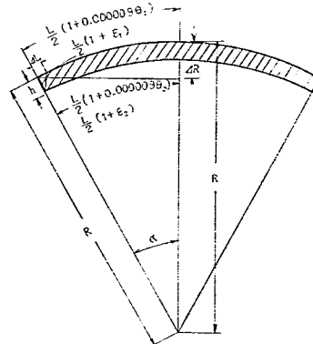
図-121 温度変化からコンクリート版中央のそりを計算する方法の説明図
