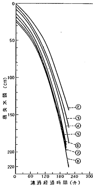
図-31B 損失水頭
