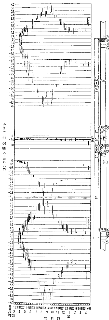
図-70 コンクリート版変位の年変化 (試験舗装 No. 1)
