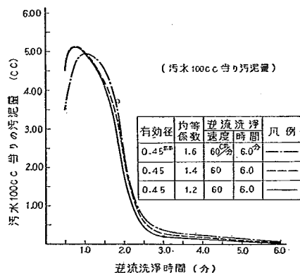
図-9 逆流洗浄時における洗浄排水の時間的変化
