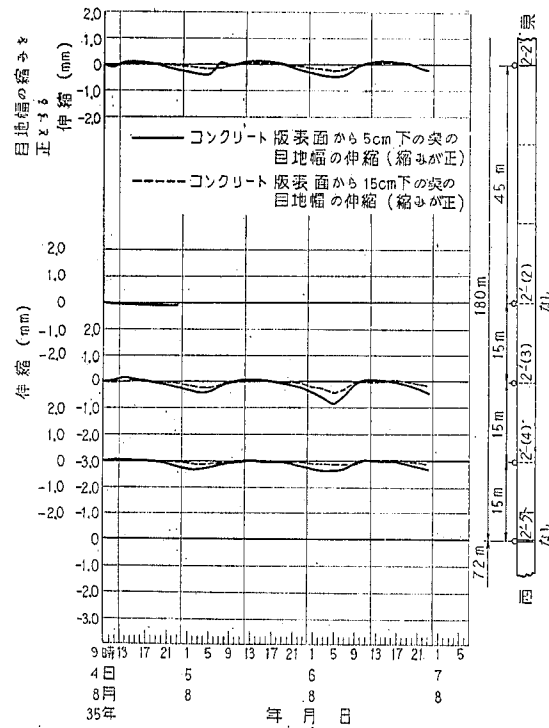
図-96 目地幅伸縮の日変化（試験舗装 No. 2'）
