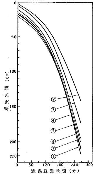
図-31C 損失水頭
