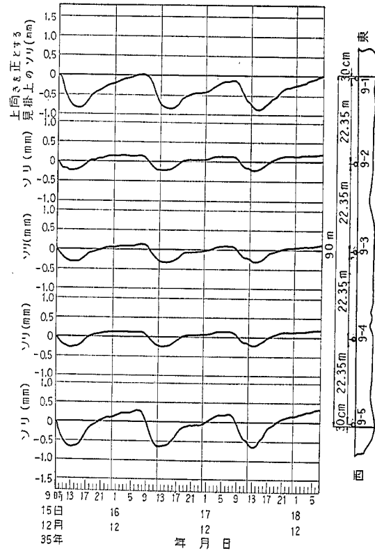
図-115 膨脹日地間隔90mの連続鉄筋コンクリート版の見掛上のそりの日変化
