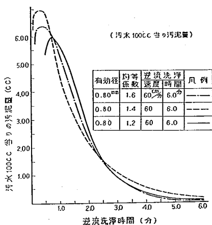
図-6 逆流洗浄時における洗浄排水の時間的変化
