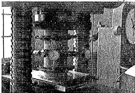
写真-15 円筒供試体のヤング率およびポアソン比の測定
