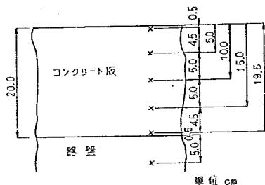
図-8 コンクリート版温度測定点位置図
