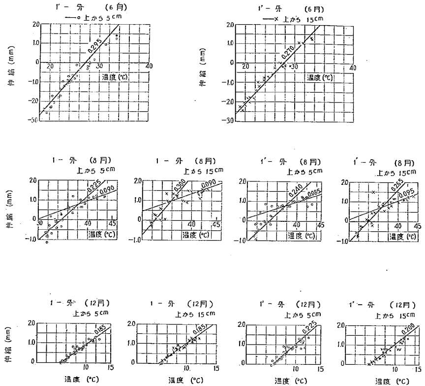
図-100 日変化における膨張目地伸縮と温度の関係 (試験舗装 No.1)
