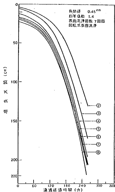
図-71C 2号池における損失水頭の変化
