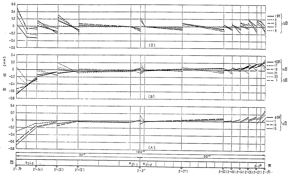
図-55 各時刻におけるコンクリート版各点の変位 (試験舗装 No.2, No.2', 35年8月)
