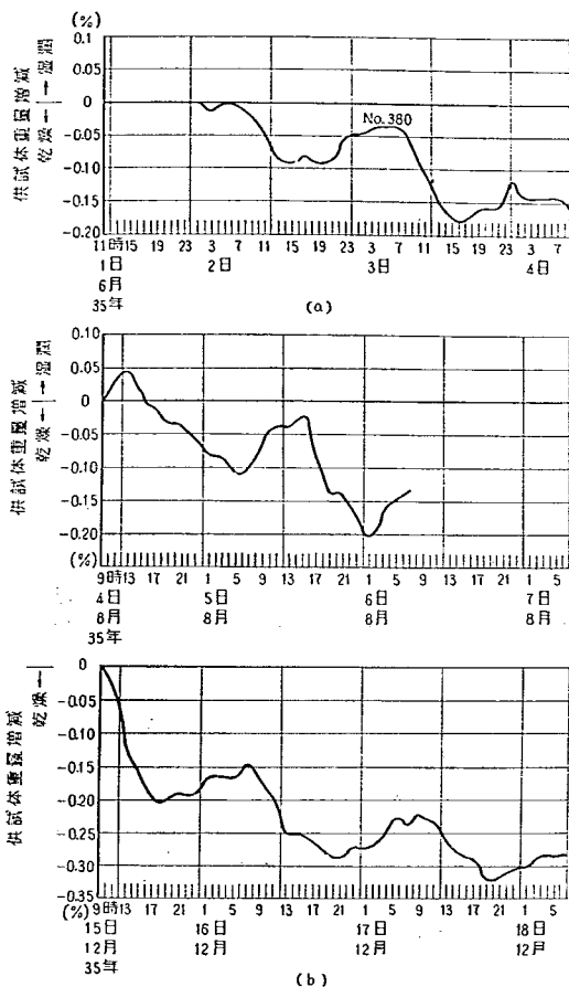
図-13 コンクリート供試体含水量の日変化
