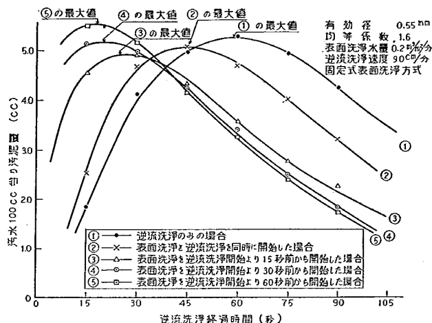
図-34 表面洗浄開始時間と洗浄排水汚泥量の関係
