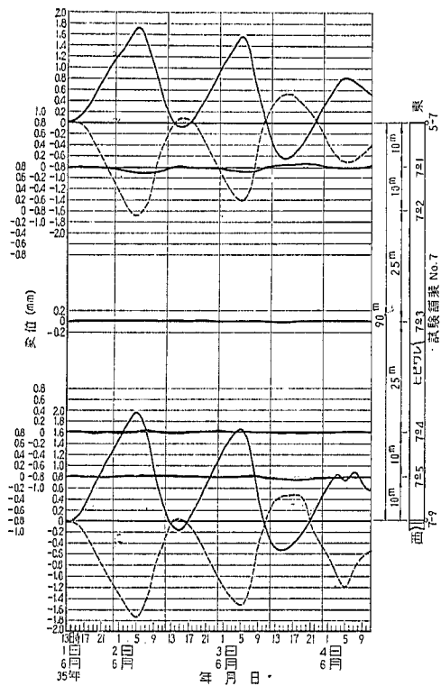
図-48 コンクリート版変位の日変化 (試験舗装 No.7)
