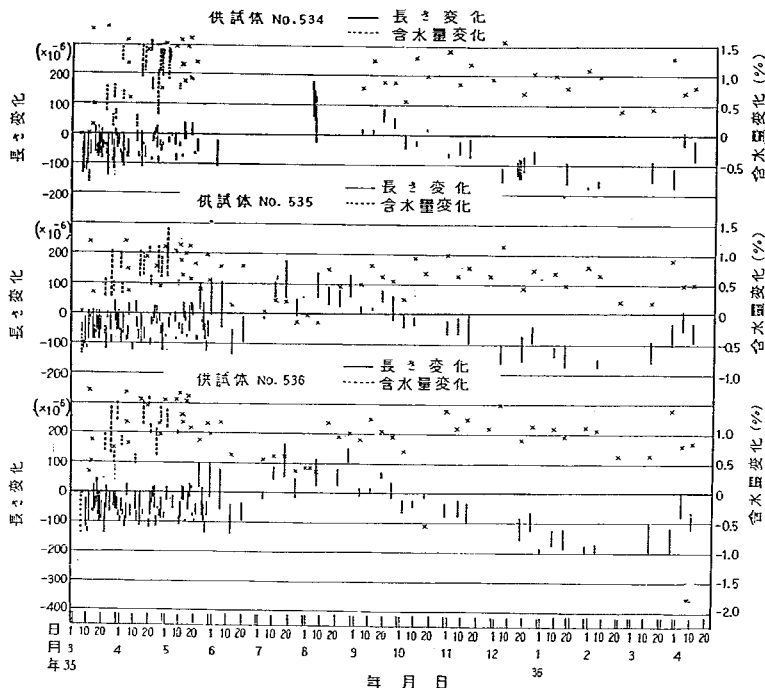
図-22 コンクリート供試体の長さ変化と含水量変化 (試験舗装 No.2')
