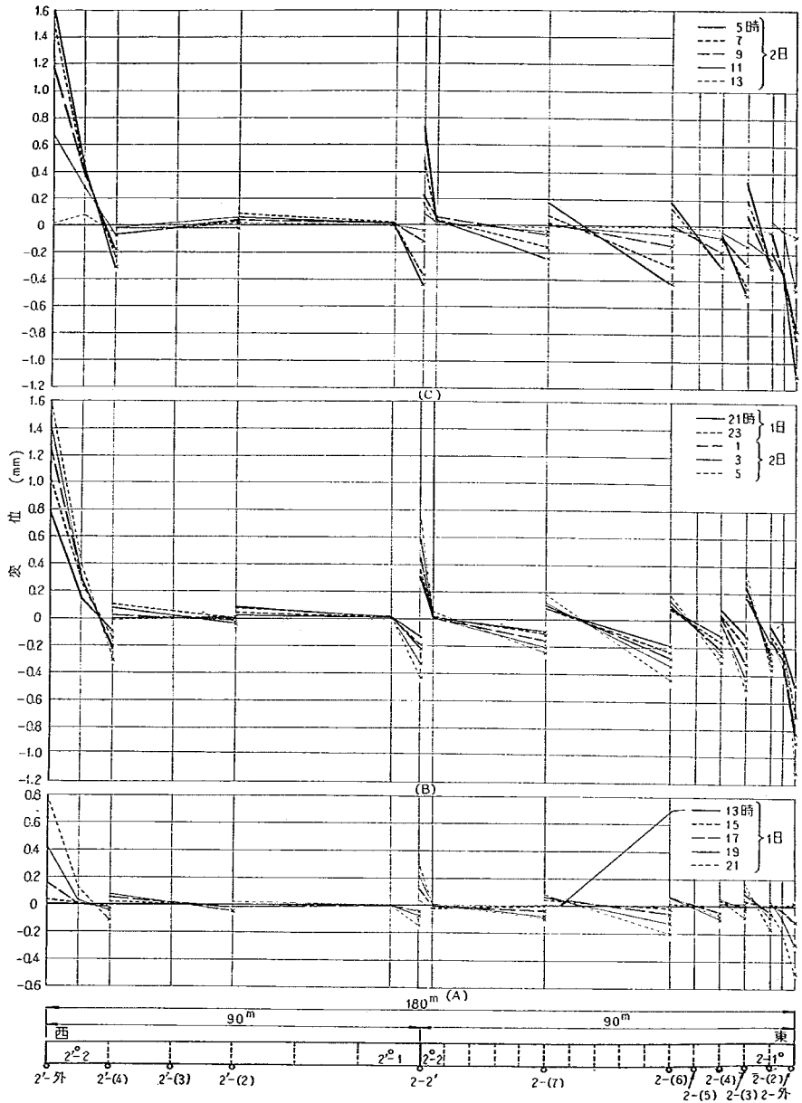
図-54 各時刻におけるコンクリート版各点の変位 (試験舗装 No.2, No.2', 35年6月)
