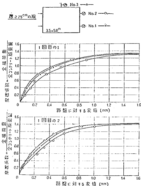
図-29 路盤摩擦係数の第1回測定値 (厚25cm)
