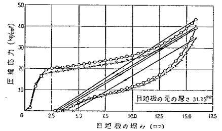
図-88 水で飽和した松目地板の圧縮復元試験結果
