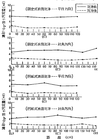
図-65 砂層表層部の汚泥分布 (有効径 0.55 mm)
