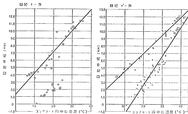
図-108 年変化における膨脹目地伸縮と温度の関係 (試験舗装 No.1)
