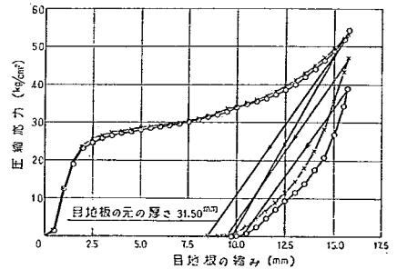
図-89 気乾状態の松目地板の圧縮復元試験結果
