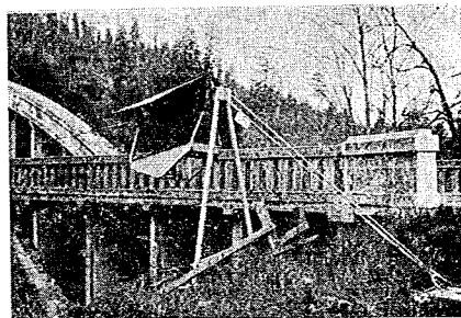
写真-15 主索のクリップ止め
