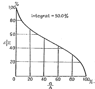
図-15 菱形流域
