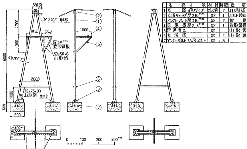
図-19 支 塔
