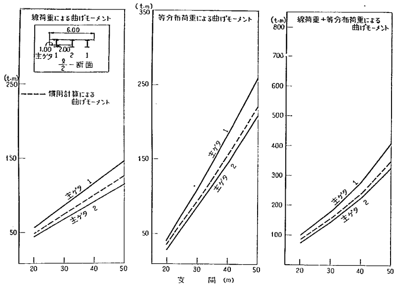
付図-2-B-1 L/2 断面の曲げモーメント
