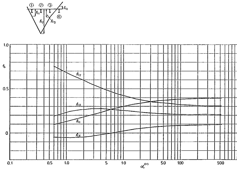
付図-1-A-16 ②ゲタの L/4 断面に対する k
