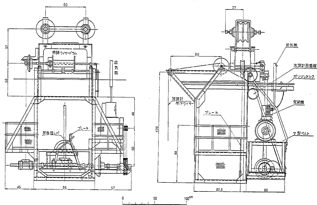
図-10 第3回吊かご
