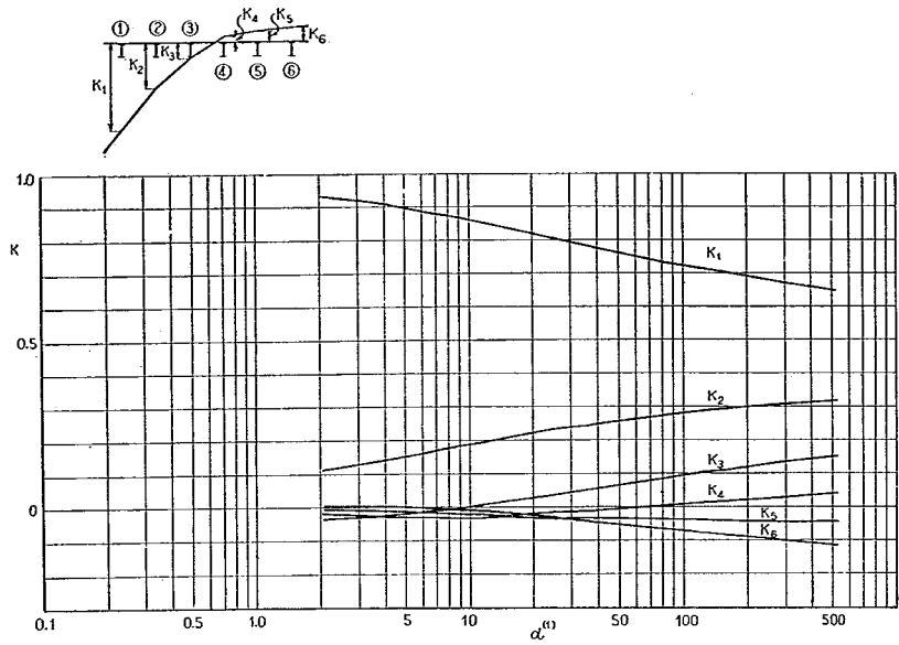
付図-1-A-31 ①ゲタの L/4 断面に対する K
