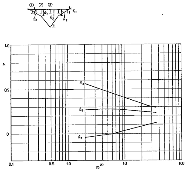
付図-1-B-14 ③ケタの L/2 断面に対する k
