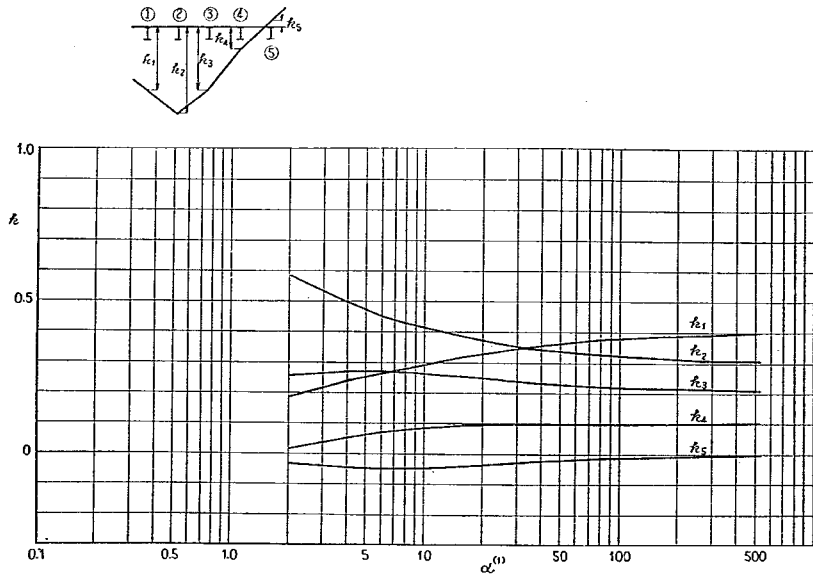
付図-1-A-24 ②ゲタの L/4 断面に対する k
