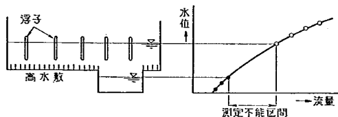
図-1 河川断面形状が複断面をしている流量観測所における水位流量曲線
