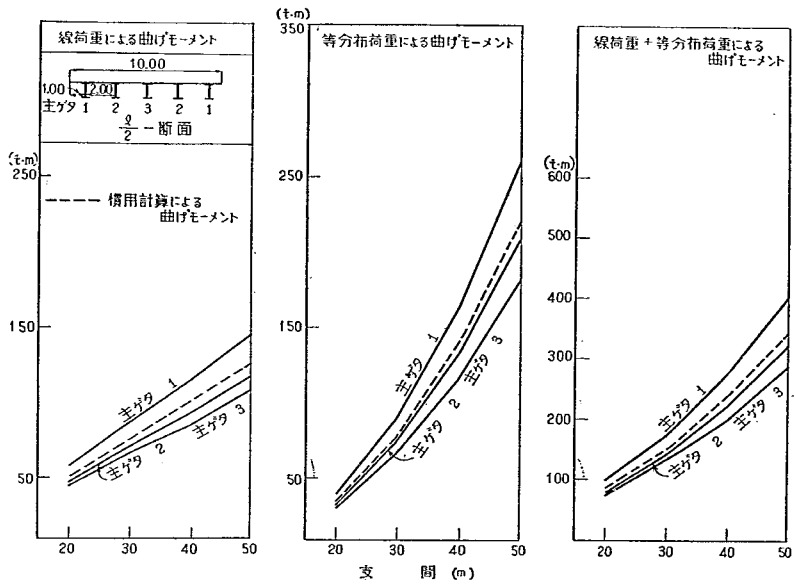
付図-2-A-7 L/2 断面の曲げモーメント
