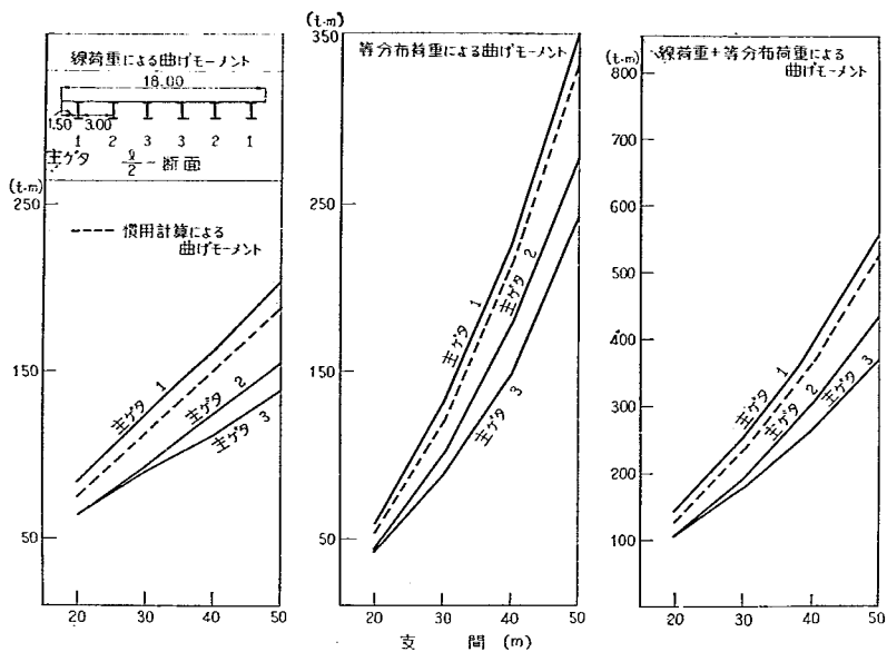
付図-2-B-10 L/2 断面の曲げモーメント
