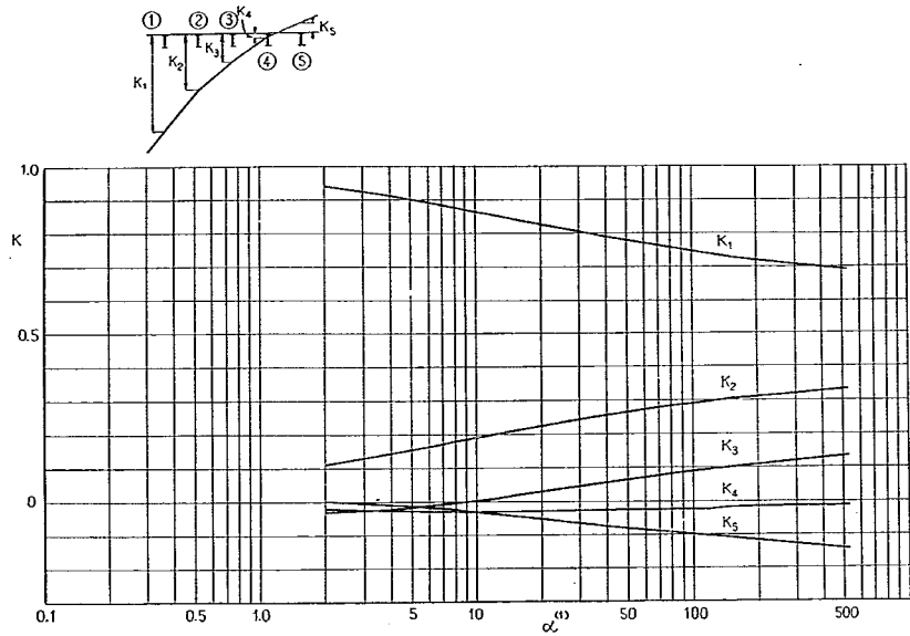
付図-1-A-19 ①ゲタの L/4 断面に対する K
