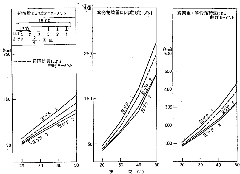
付図-2-A-10' L/4 断面の曲げモーメント
