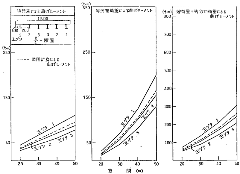
付図-2-B-9' L/4 断面の曲げモーメント
