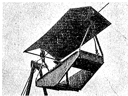
写真-16 吊 か ご
