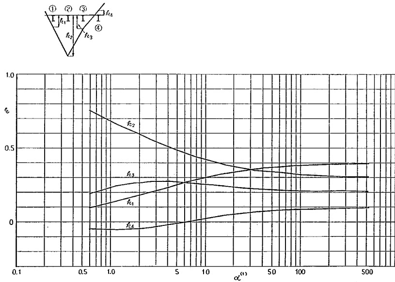
付図-1-A-16 ③ゲタの L/4 断面に対する k
