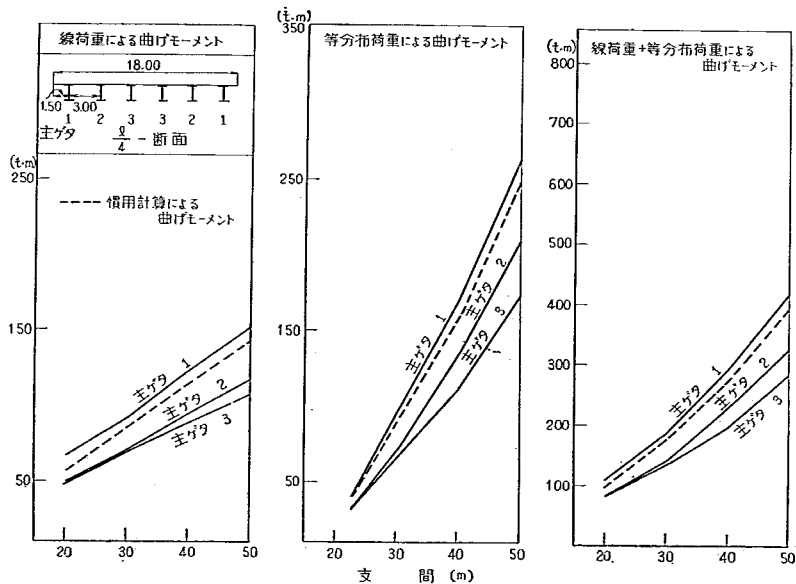
付図-2-B-10' L/4 断面の曲げモーメント
