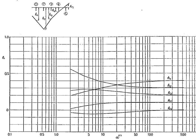
付図-1-A-22 ③ケタの L/2 断面に対する k
