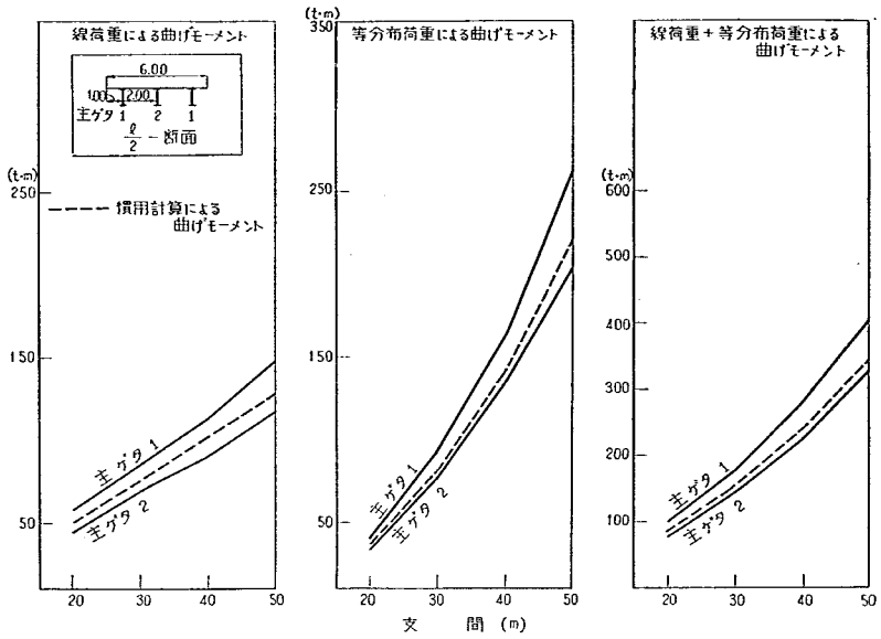
付図-2-A-1 L/2 断面の曲げモーメント
