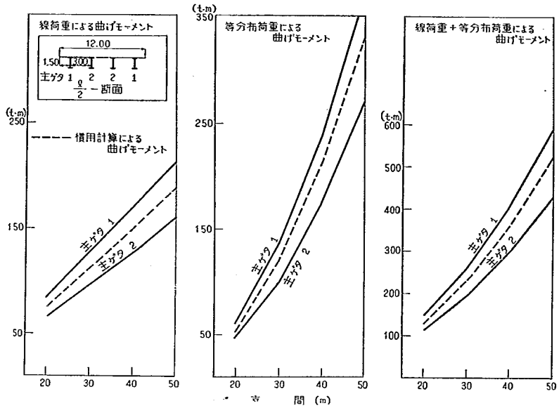
付図-2-A-5 L/2 断面の曲げモーメント
