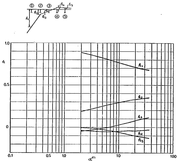
付図-1-B-10 ①ケタの L/2 断面に対する k
