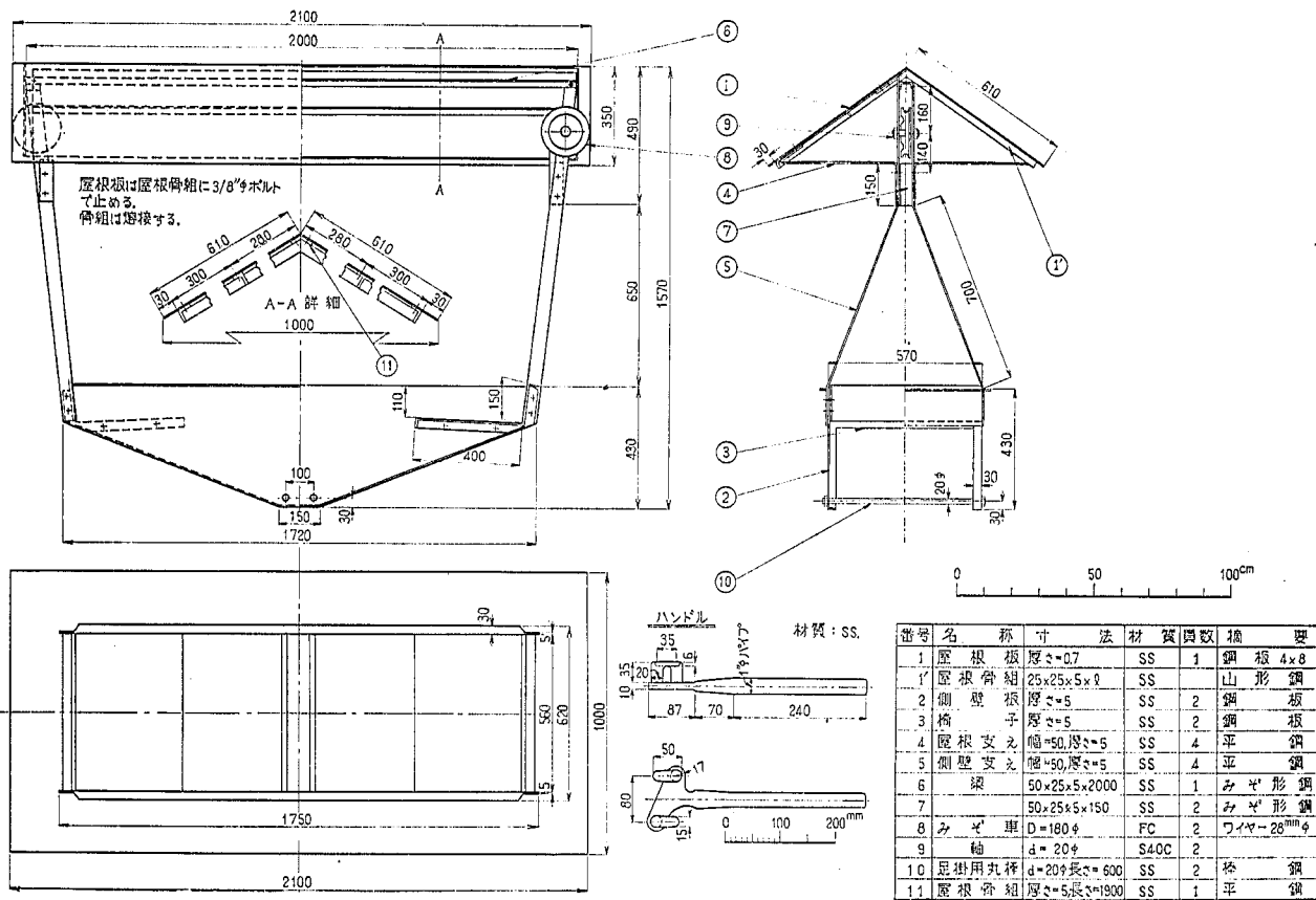
図-18 吊 か こ
