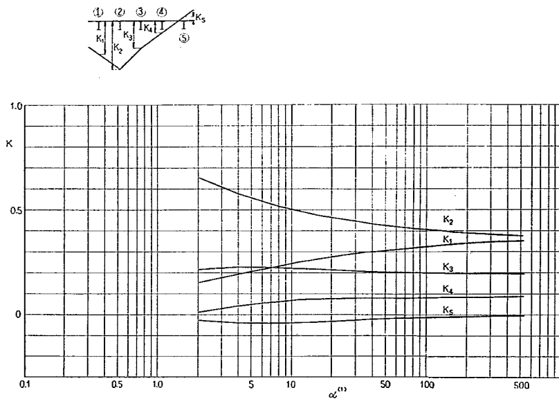
付図-1-A-21 ③ケタの L/2 断面に対する K
