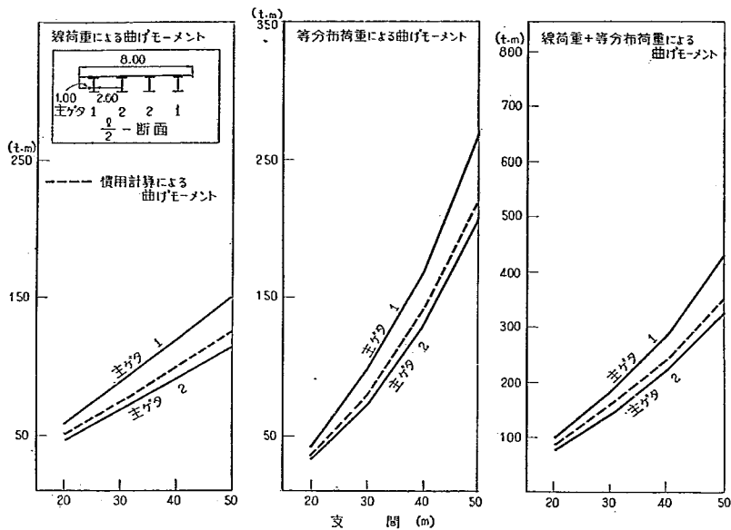
付図-2-B-4 L/2 断面の曲げモーメント
