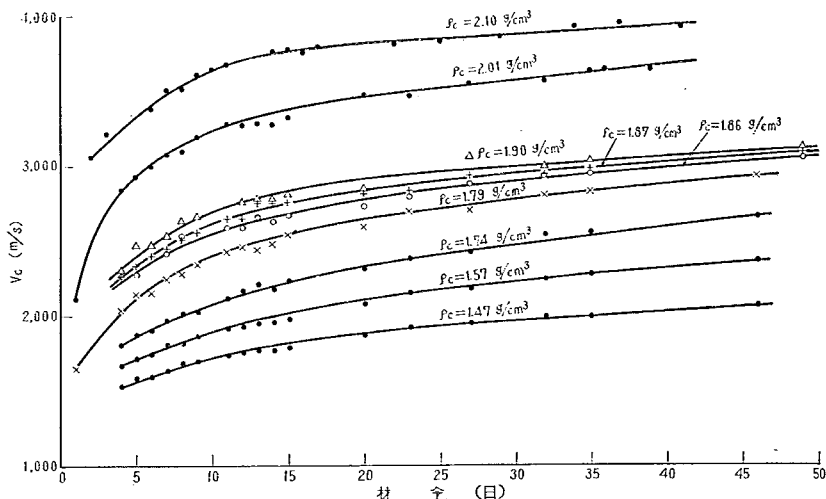
図-17 普通セメントの凝固過程における速度変化
