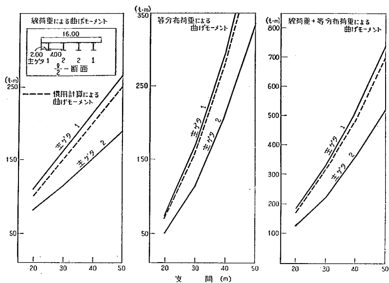
付図-2-B-6 L/2断面の曲げモーメント
