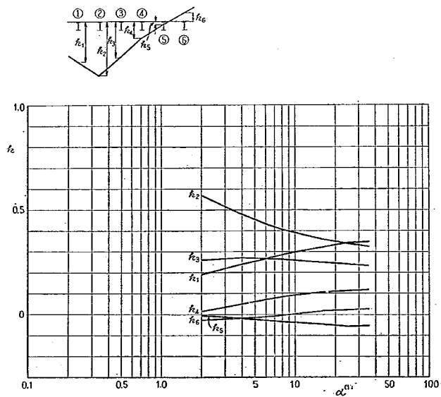
付図-1-B-18 ③ケタの L/2 断面に対する k
