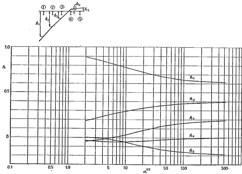
付図-1-A-20 ①ゲタの L/4 断面に対する k
