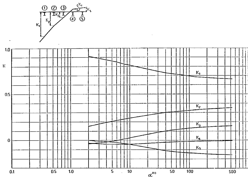
付図-1-A-17 ①ケタの L/2 断面に対する K
