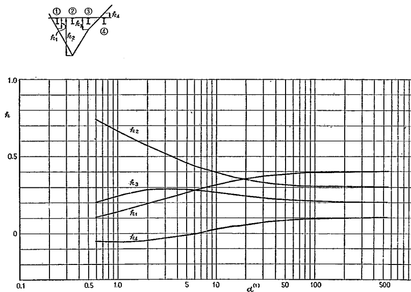
付図-1-A-14 ②ケタの L/2 断面に対する k
