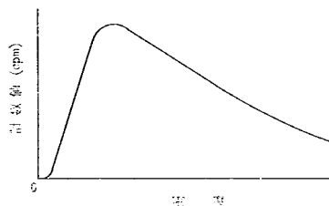
図-6 散乱 \gamma 線の計数値と密度の関係
