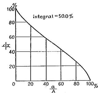
図-16 円形流域
