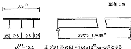
図-4 設計例にとりあげた橋
