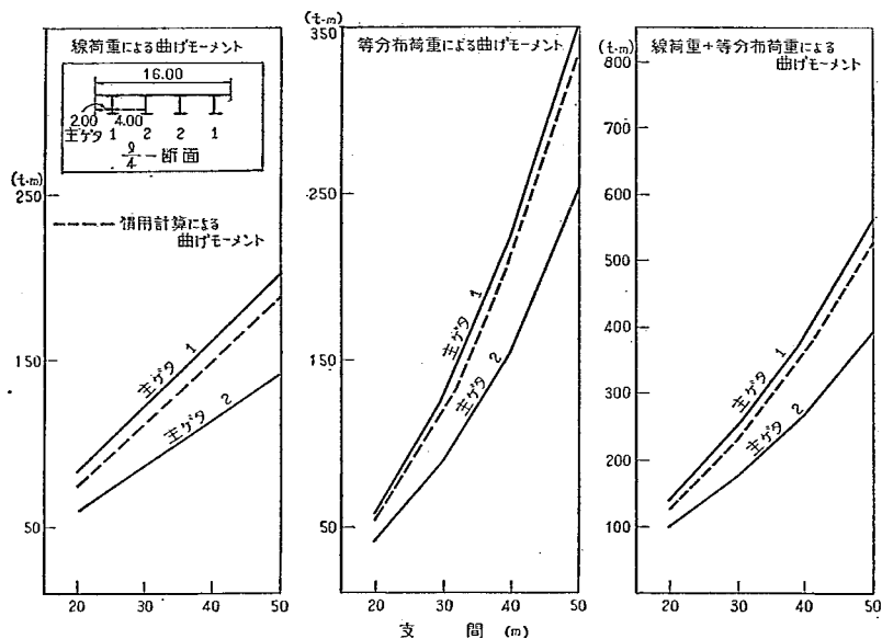
付図-2-B-6' L/4断面の曲げモーメント
