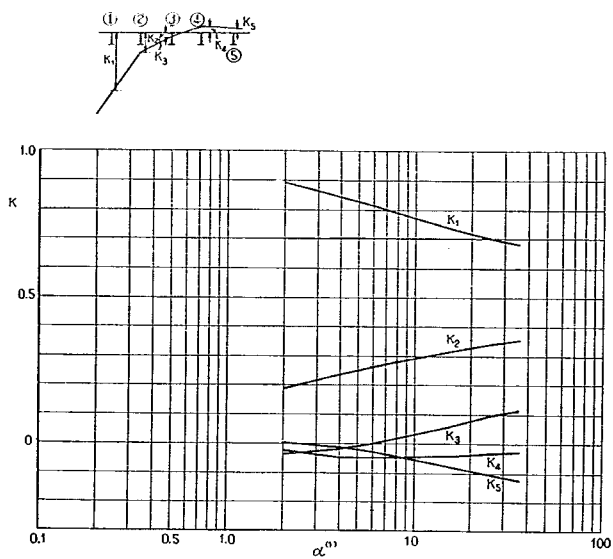
付図-1-B-9 ①ケタの L/2 断面に対する K
