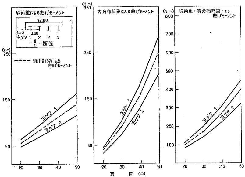
付図-2-B-5' L/4 断面の曲げモーメント
