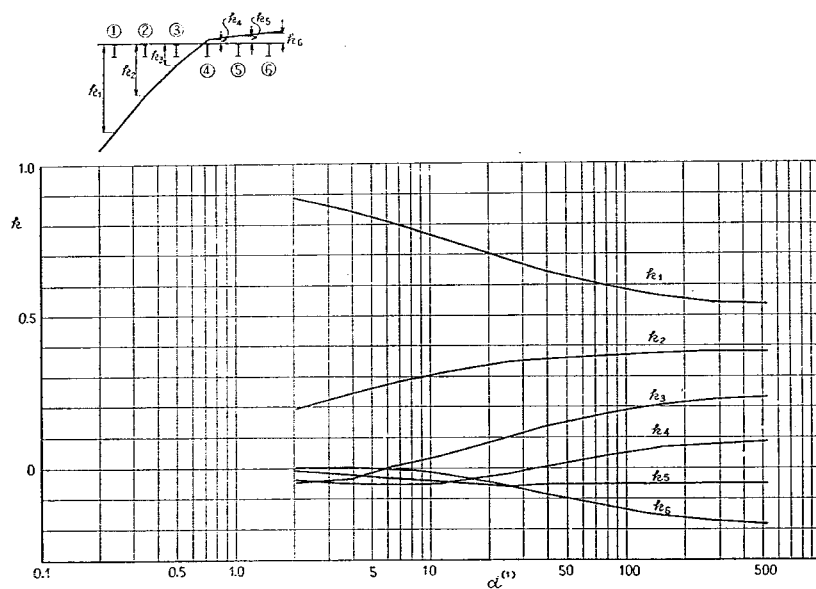
付図-1-A-30 ①ケタの L/2 断面に対する k
