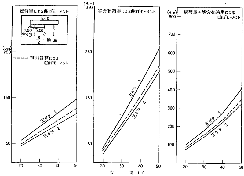
付図-2-B-1 L/2断面の曲げモーメント
