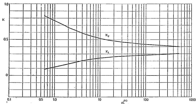
付図-1-A-5 ②ケタの L/2 断面に対する K
