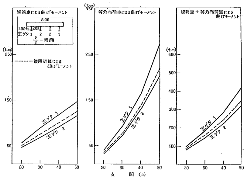
付図-2-A-4 L/2 断面の曲げモーメント
