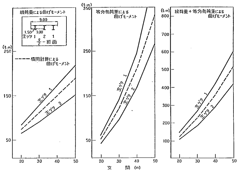
付図-2-B-2 L/2 断面の曲げモーメント
