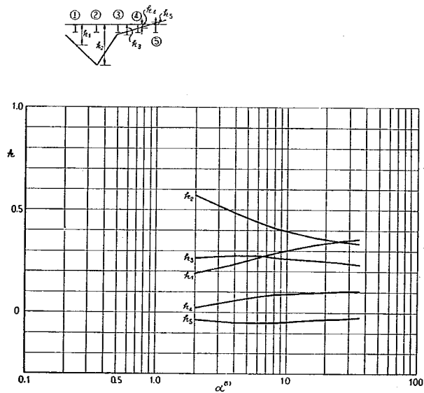
付図-1-B-12 ②ゲタの L/2 断面に対する k
