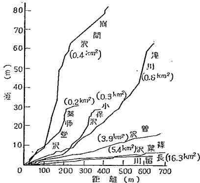
図-2 縦断図
