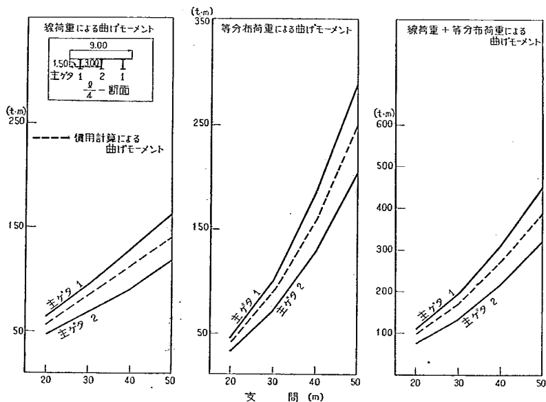
付図-2-A-2' L/4 断面の曲げモーメント
