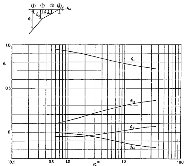
付図-1-B-6 ①ケタの L/2 断面に対する k
