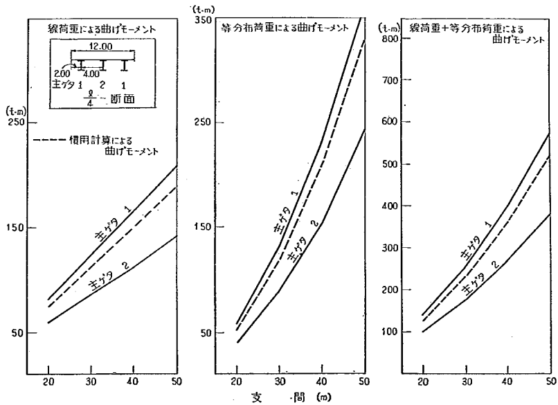
付図-2-B-3' L/4 断面の曲げモーメント
