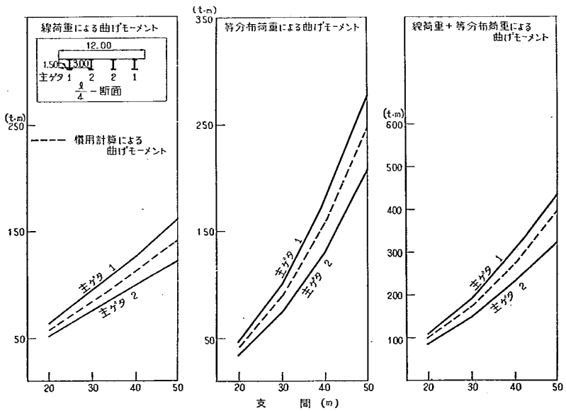
付図-2-A-5' L/4 断面の曲げモーメント
