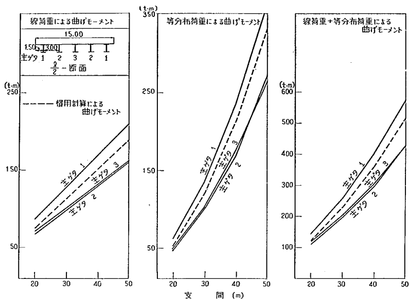
付図-2-A-8 L/2 断面の曲げモーメント
