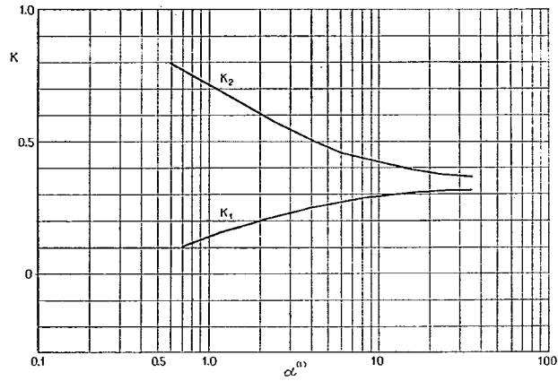
付図-1-B-3 ②ゲタの L/2 断面に対する K
