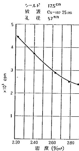
図-11 密度計カリブレーション曲線
