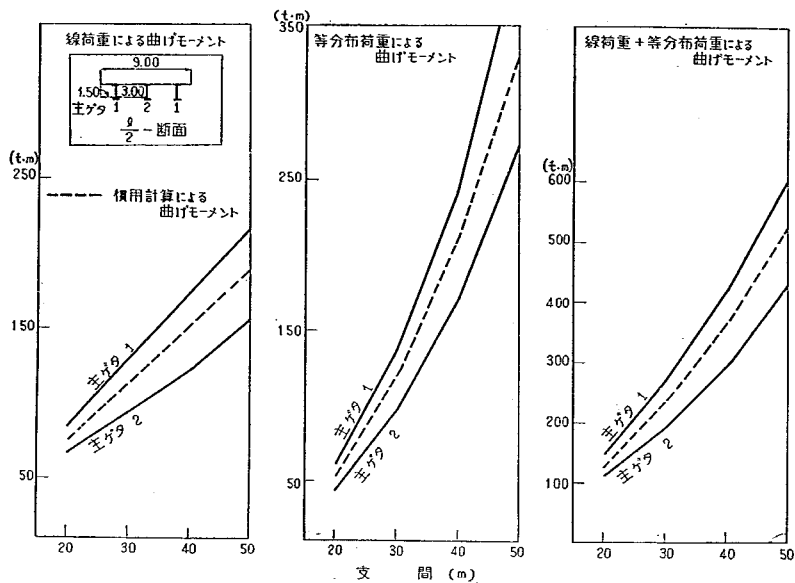
付図-2-A-2 L/2 断面の曲げモーメント
