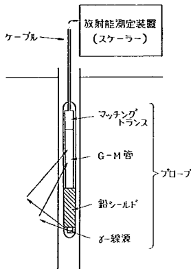
図-5 散乱型密度計
