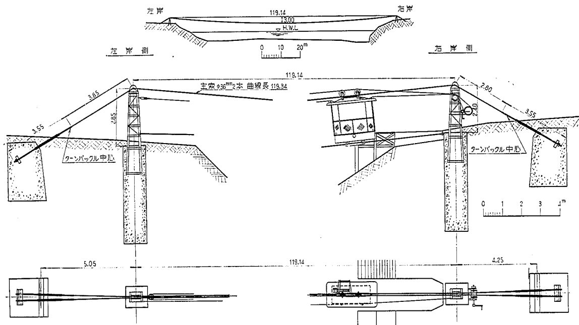
図-5 索道配置図，ただし図中の吊かごは最初のものを改造した第5回目のものである。
