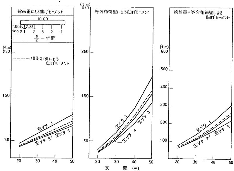
付図-2-A-7' L/4 断面の曲げモーメント
