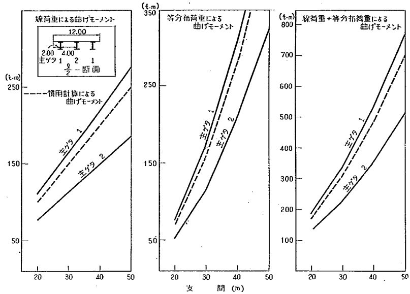
付図-2-B-3 L/2 断面の曲げモーメント
