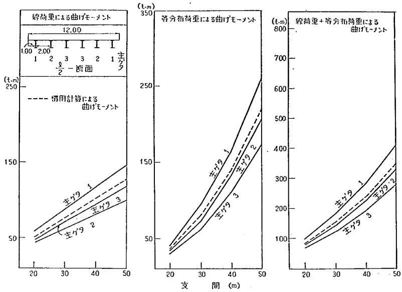
付図-2-B-9 L/2 断面の曲げモーメント
