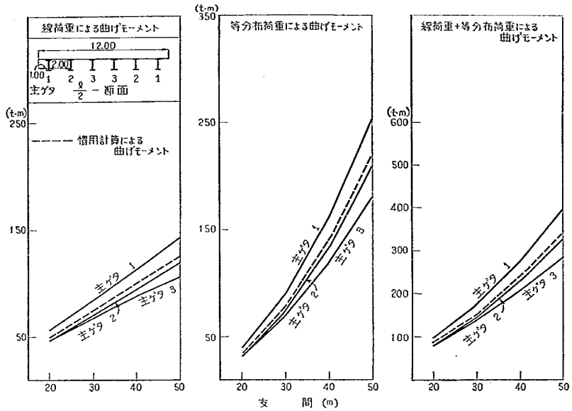
付図-2-A-9 L/2 断面の曲げモーメント
