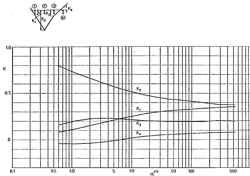
付図-1-A-13 ②ケタの L/2 断面に対する K
