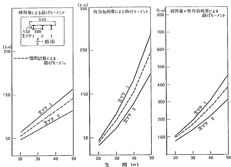
付図-2-B-2' L/4 断面の曲げモーメント
