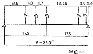
図-6 トレーラー荷重の荷荷位置
