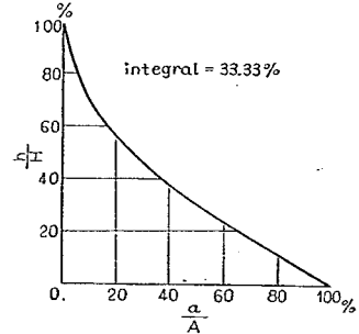
図-13 三角形流域
