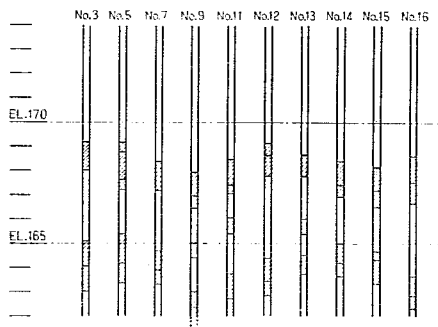
図-13 多亀裂帯分布図
