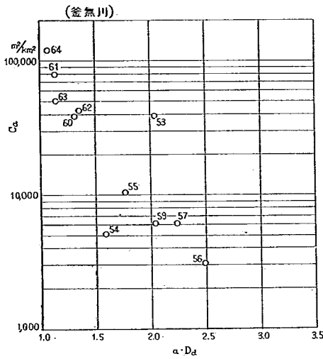
図-36 (5) 崩壊面積と流域係数
