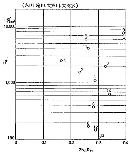
図-35 (1) 崩壊面積と流域傾斜
