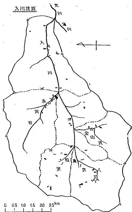
図-34 (1) 崩壊地分布図
