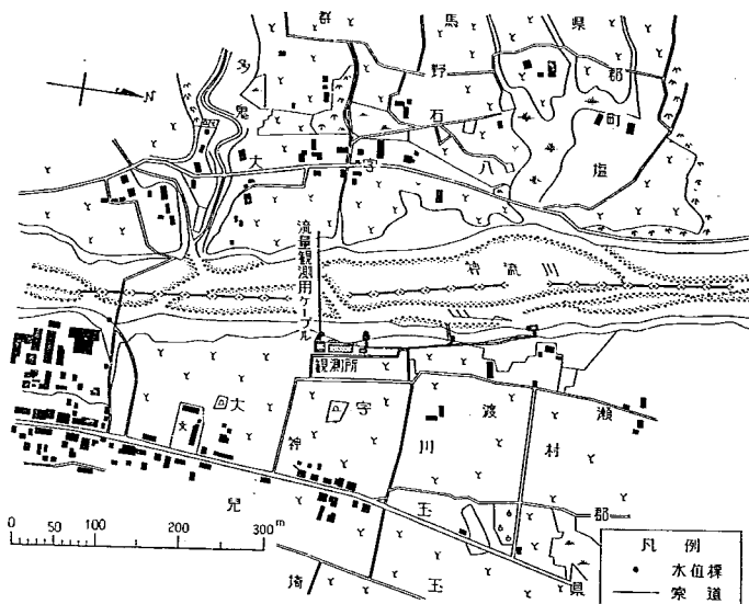
図-3 渡瀬流量観測所付近
