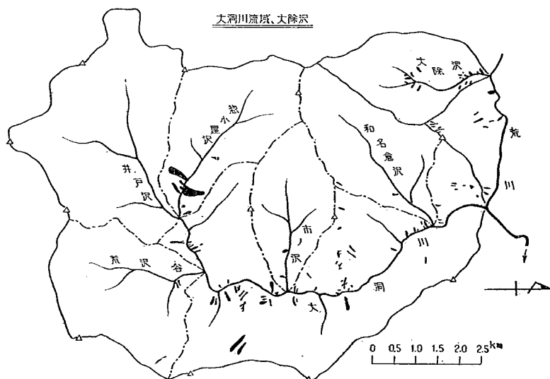
図-34 (3) 崩壊地分布図
