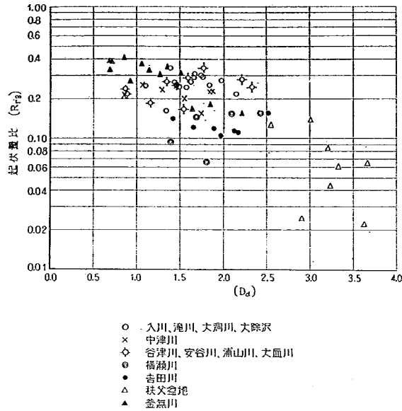
図-30 起伏量比と谷密度
