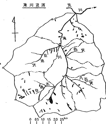
図-34 (2) 崩壊地分布図
