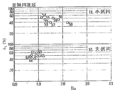
図-24 (2) hypsometric integral と谷密度
