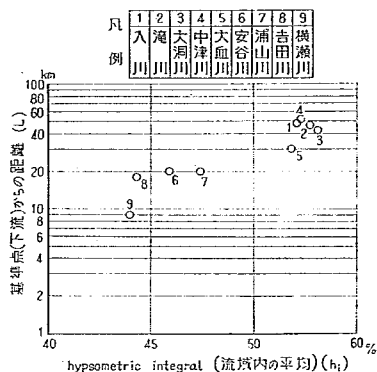
図-25 基準点からの距離と hypsometric integral の関係
