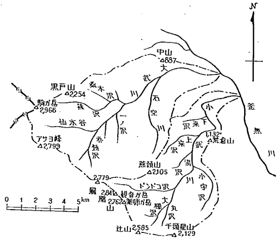
図-22 釜無川流域図
