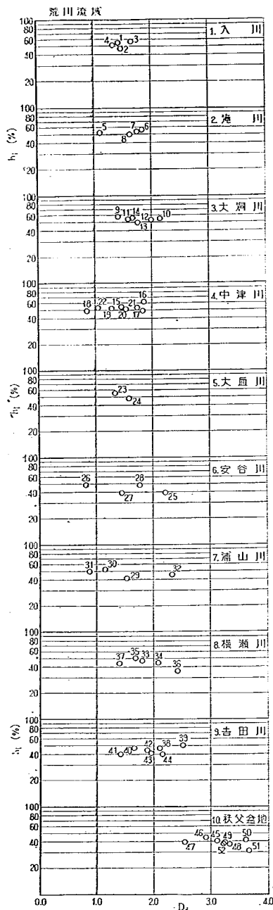
図-24 (i) hypsometric integral と谷密度
