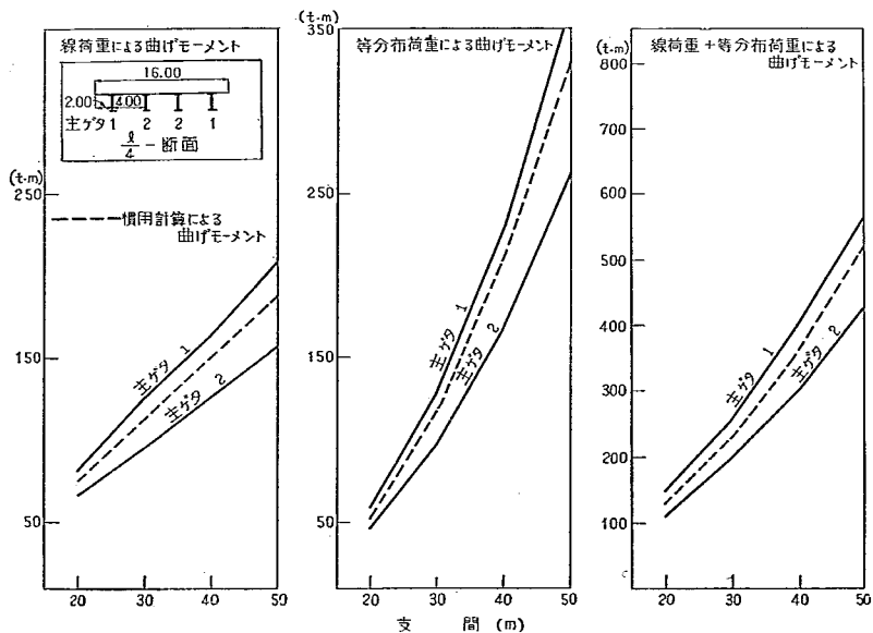
付図-2-A-6' L/4 断面の曲げモーメント
