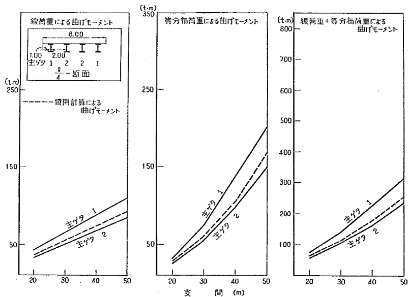
付図-2-B-4' L/4 断面の曲げモーメント
