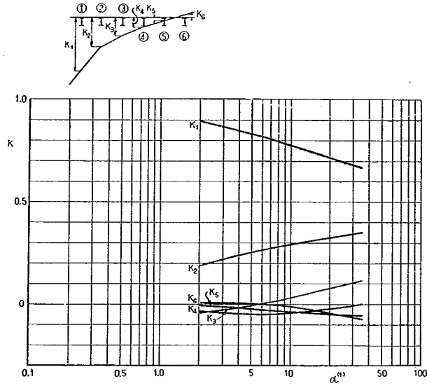
付図-1-B-15 ①ゲタの L/2 断面に対する K
