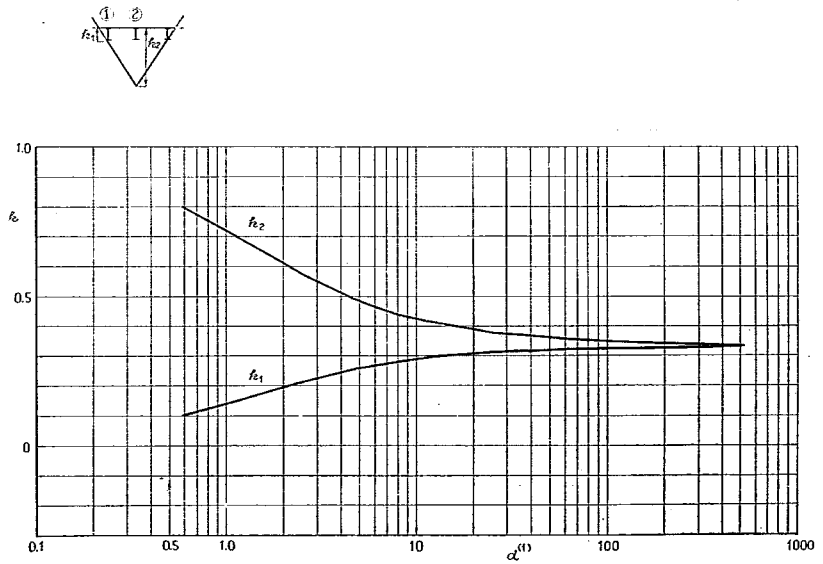
付図-1-A-8 ③ゲタの L/4 断面に対する k
