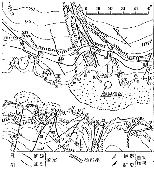
図-2(a) 原案ダム試験位置付近平面図
