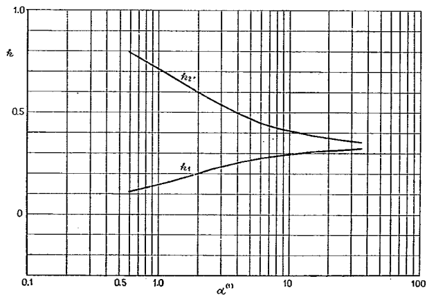
付図-1-B-4 ②ゲタの L/2 断面に対する k
