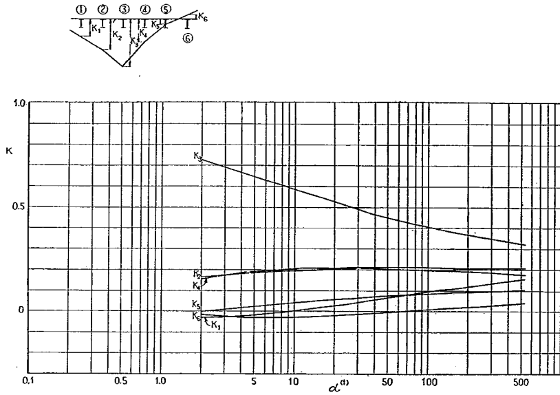
付図-1-A-39 ③ゲタの L/4 断面に対する K
