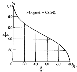
図-15 菱形流域
