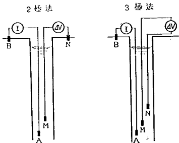
図-7 電気検層法による比抵抗の測定
