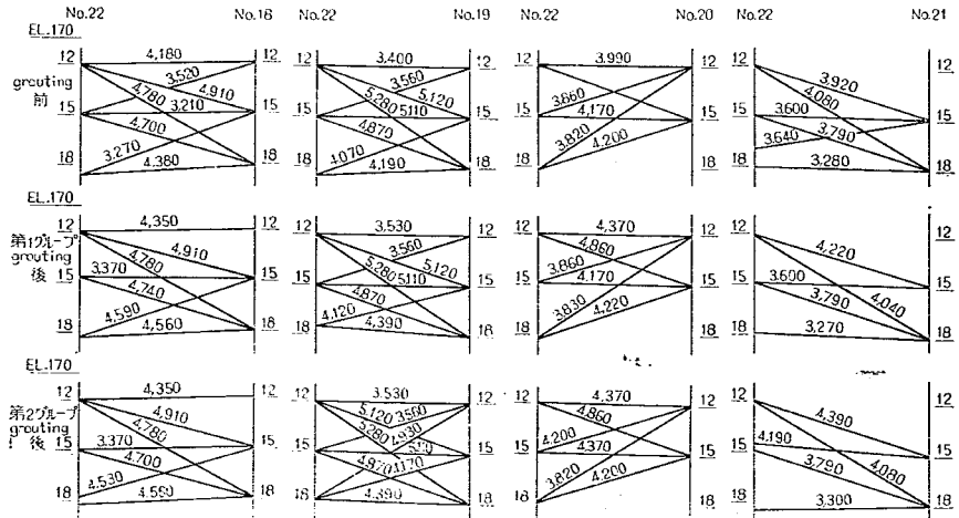
図-9 弾性波速度測定結果 (m/s)
