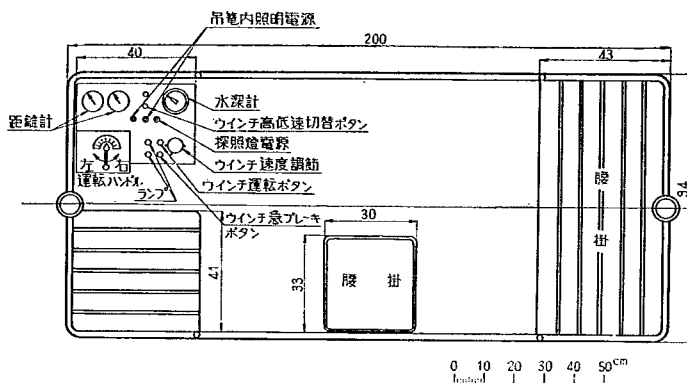
図-13 第5回吊かご内部
