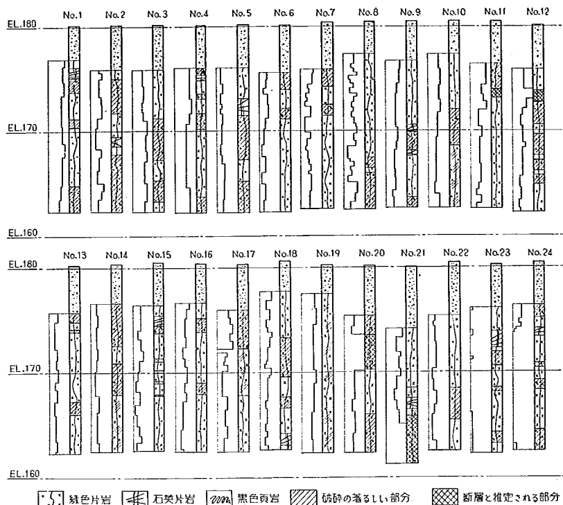
図-3 ボーリング柱状図
