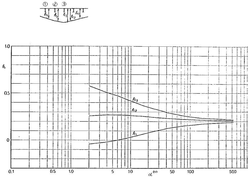
付図-1-A-28 ③ゲタの L/4 断面に対する k
