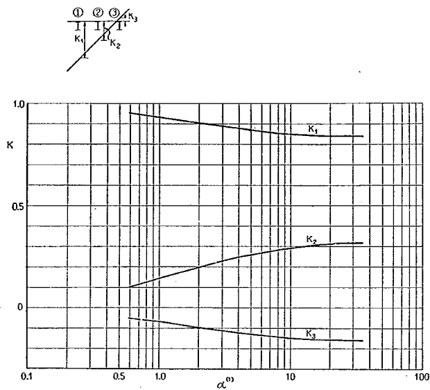
付図-1-B-1 ①ケタの L/2 断面に対する K
