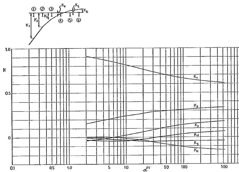
付図-1-A-29 ①ケタの L/2 断面に対する K
