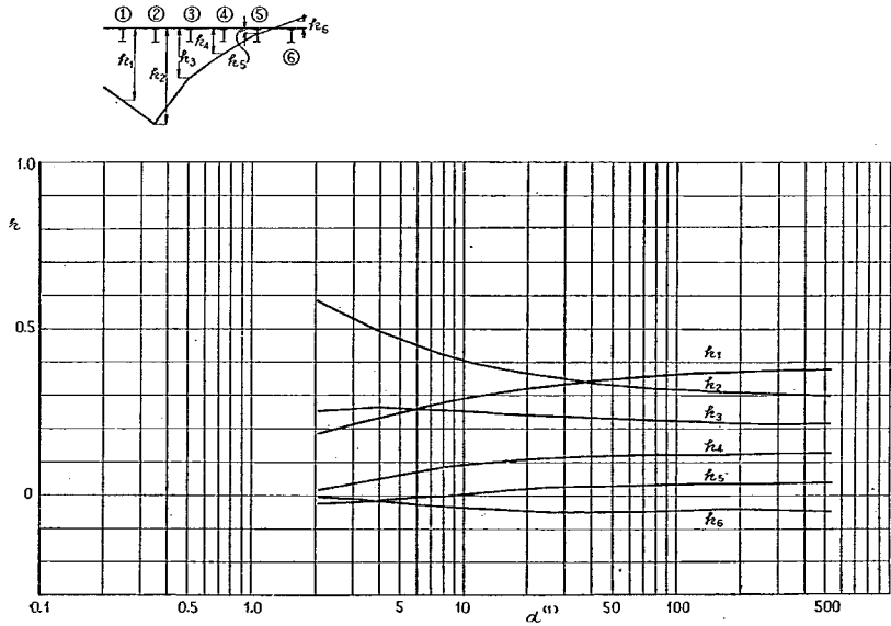
付図-1-A-36 ②ゲタの L/4 断面に対する k
