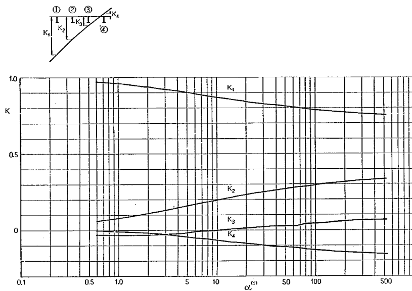
付図-1-A-11 ①ゲタの L/4 断面に対する K
