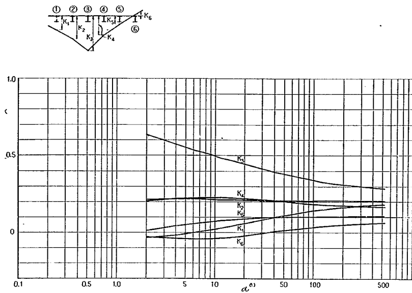
付図-1-A-37 ③ケタの L/2 断面に対する K
