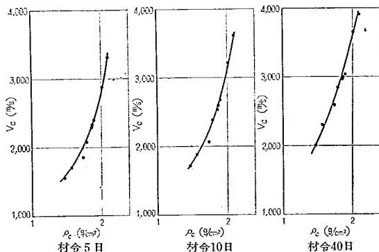
図-18 速度と密度の関係
