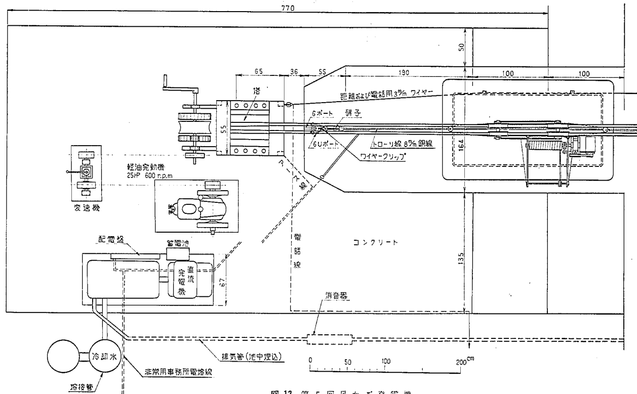
図-12 第5回吊かご発電機
