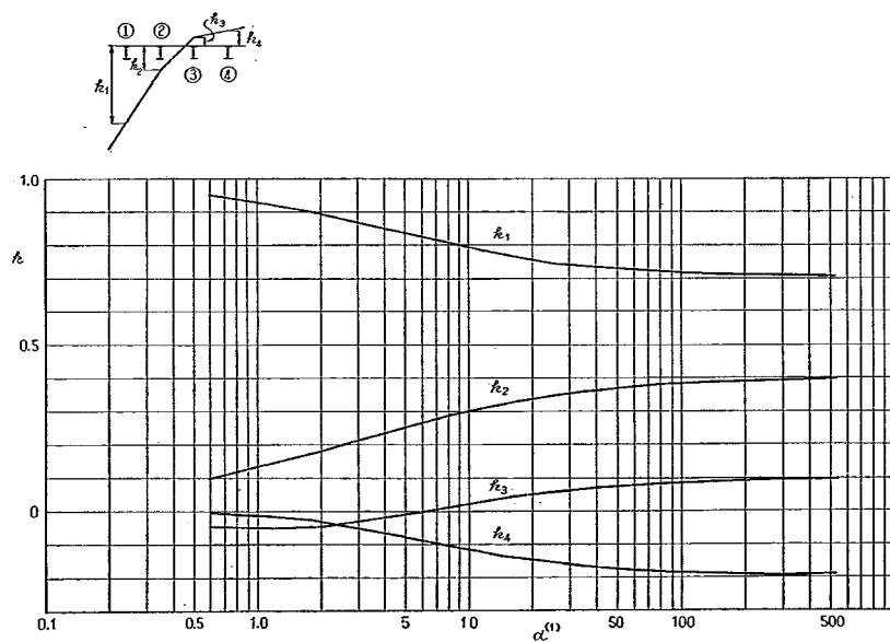
付図-1-A-12 ①ゲタの L/4 断面に対する k
