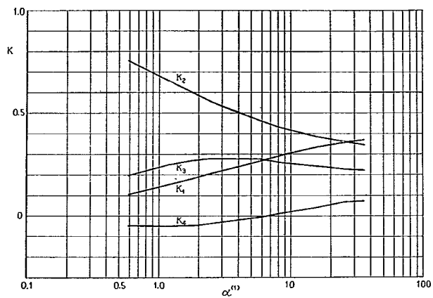
付図-1-B-7 ②ゲタの L/2 断面に対する K
