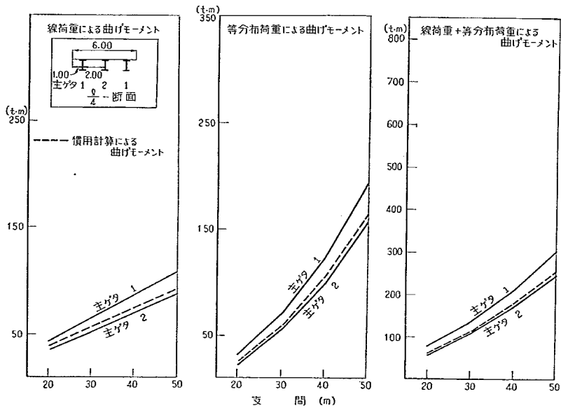
付図-2-B-1' L/4断面の曲げモーメント
