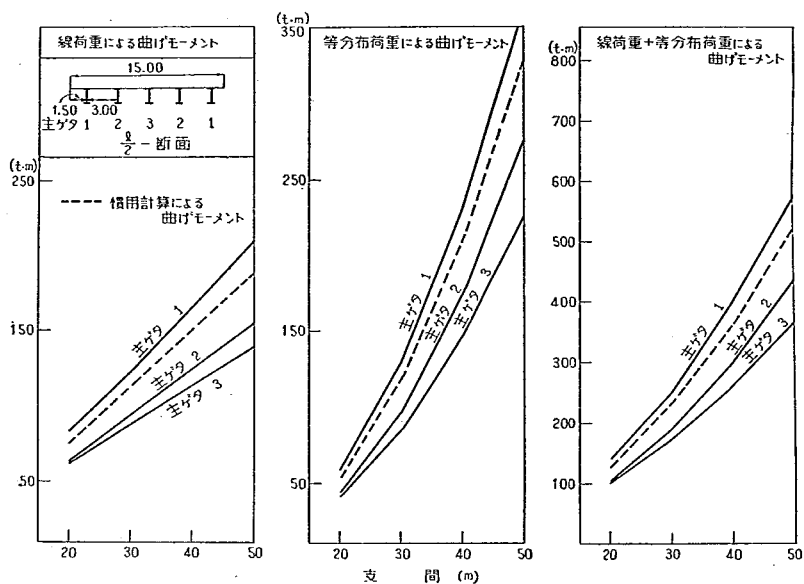
付図-2-B-8 L/2 断面の曲げモーメント
