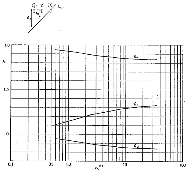
付図-1-B-2 ①ケタの L/2 断面に対する k
