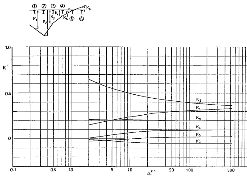
付図-1-A-33 ②ケタの L/2 断面に対する K
