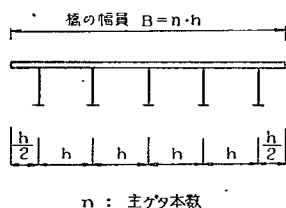
図-2 橋の幅員と主ゲタ間隔との関係
