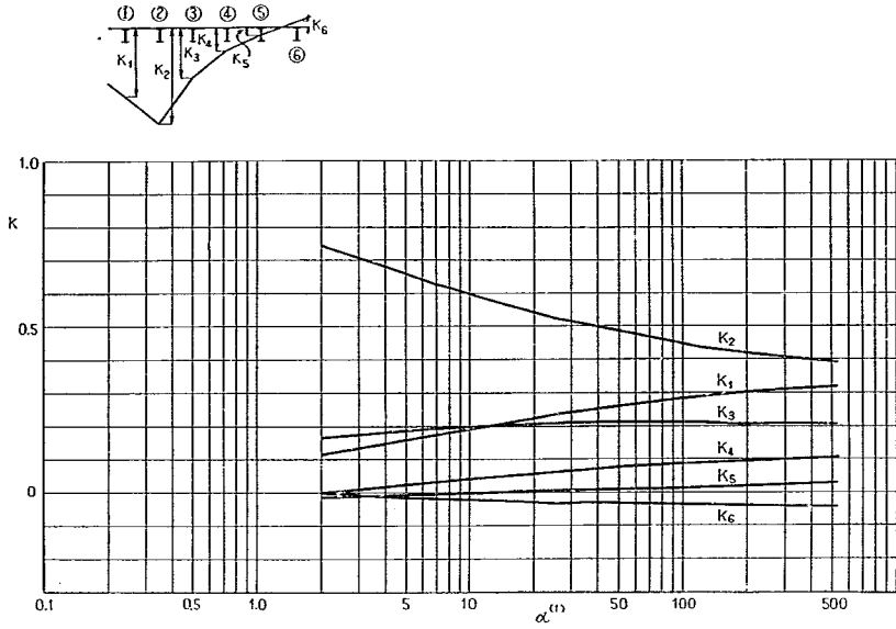
付図-1-A-35 ②ゲタの L/4 断面に対する K
