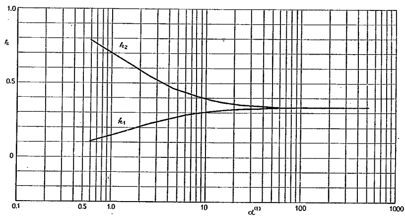
付図-1-A-6 ②ケタの L/2 断面に対する k
