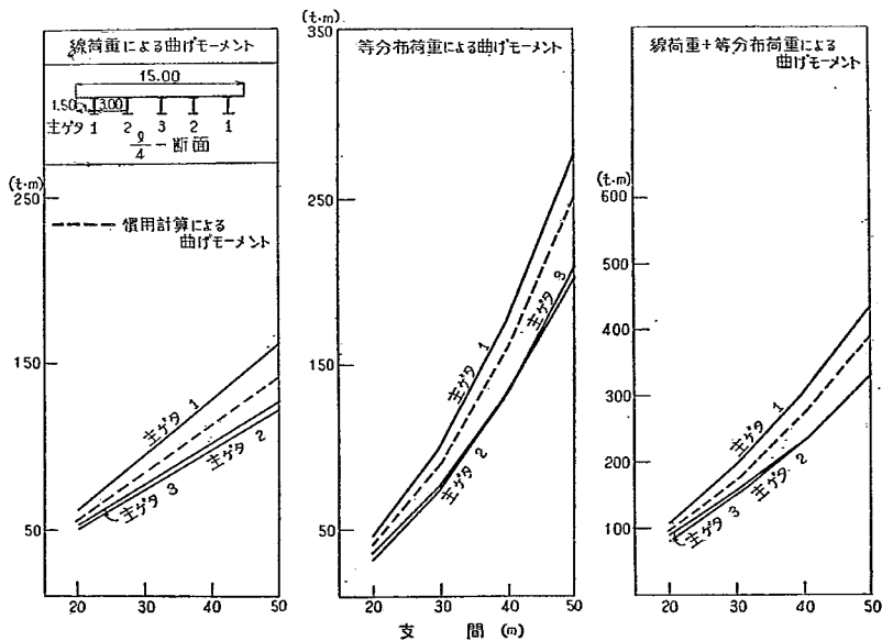
付図-2-A-8' L/4 断面の曲げモーメント
