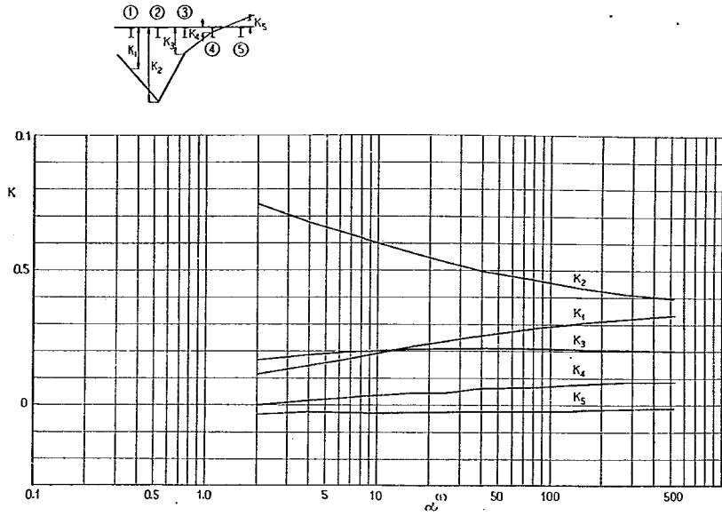
付図-1-A-23 ②ゲタの L/4 断面に対する K
