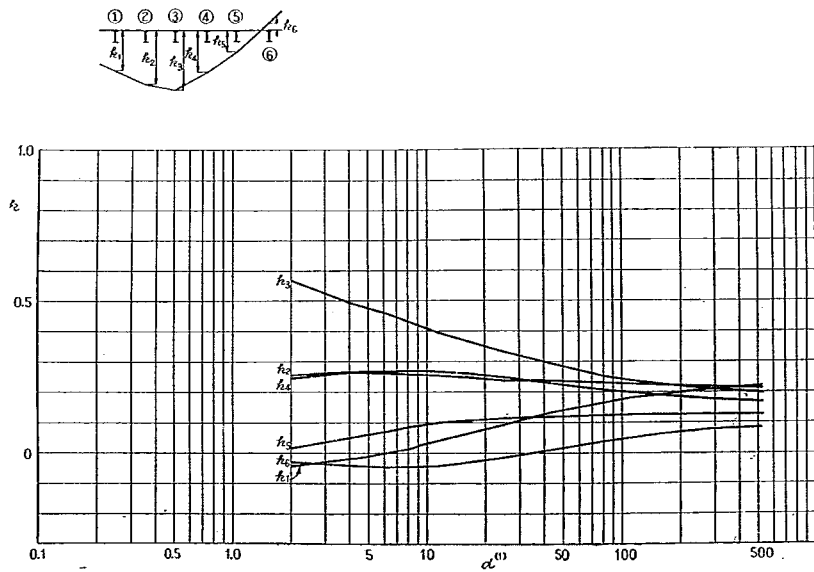
付図-1-A-40 ③ゲタの L/4 断面に対する k
