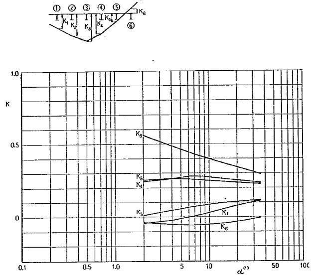
付図-1-B-19 ③ゲタの L/2 断面に対する K
