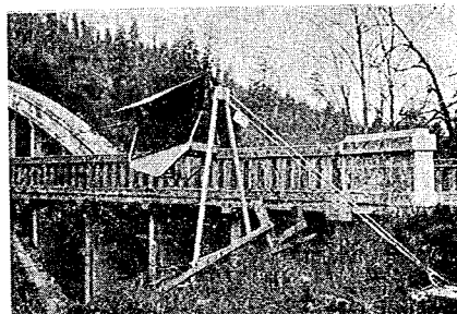
写真-15 主索のクリップ止め
