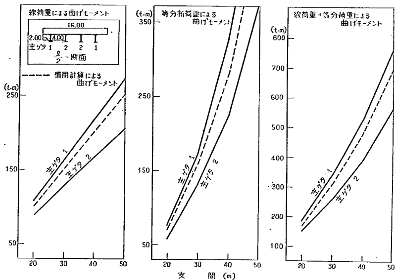
付図-2-A-6 L/2 断面の曲げモーメント
