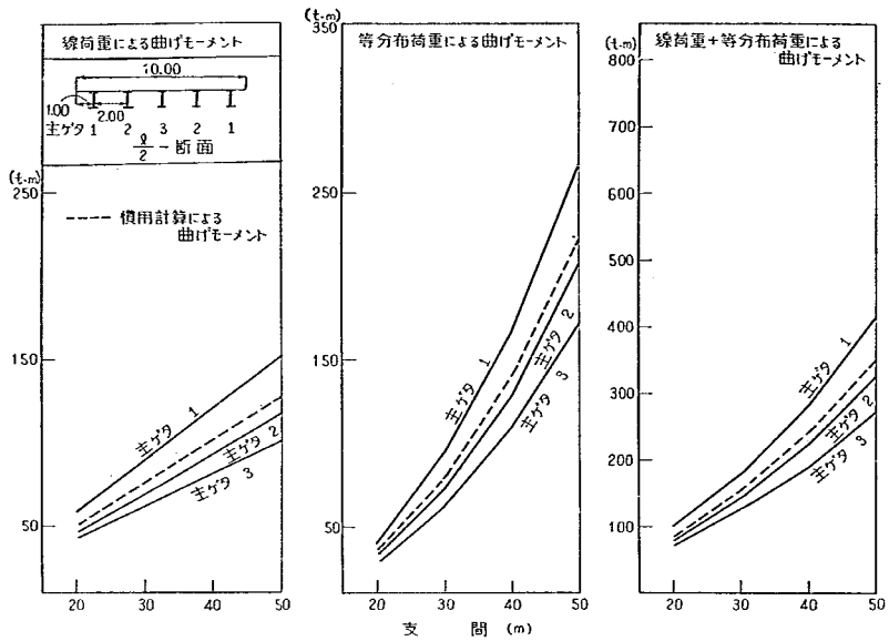
付図-2-B-7 L/2断面の曲げモーメント
