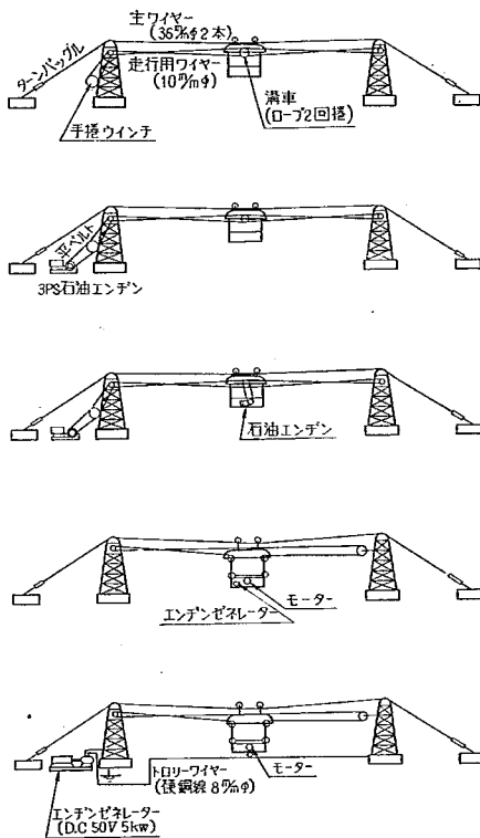
図-14 吊かご改造の変遷
