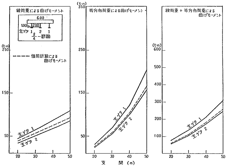
付図-2-A-1' L/4 断面の曲げモーメント
