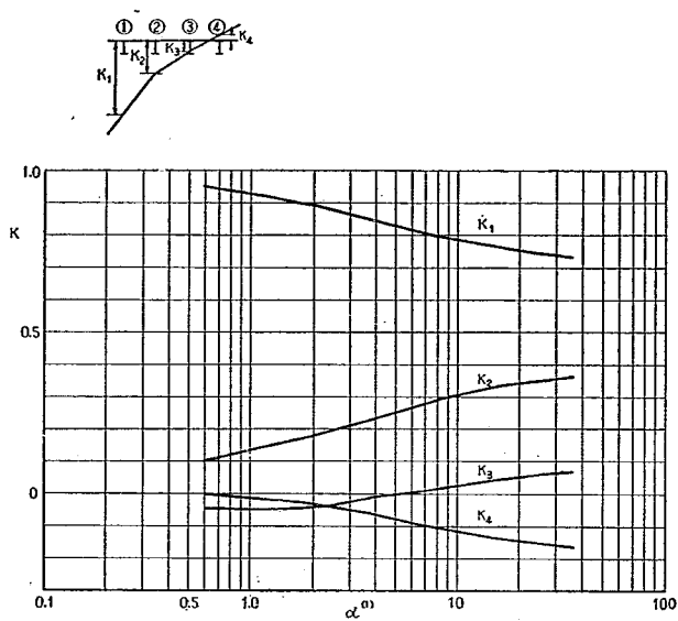
付図-1-B-5 ①ケタの L/2 断面に対する K
