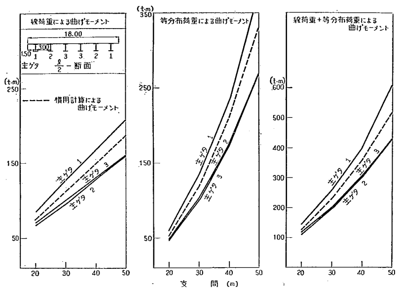
付図-2-A-10 L/2 断面の曲げモーメント
