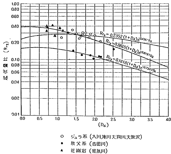
図-31 起伏量比と谷密度の関係
