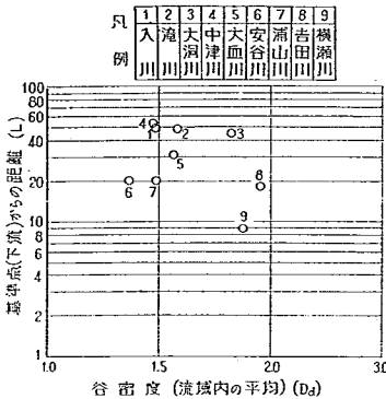
図-26 基準点からの距離と谷密度の関係
