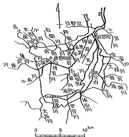
図-1 秩父盆地水系図
