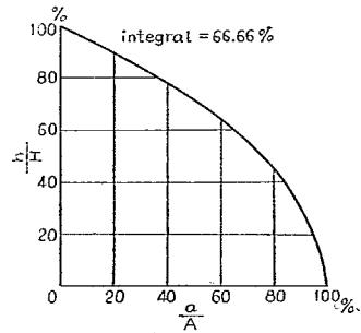
図-14 逆三角形流域
