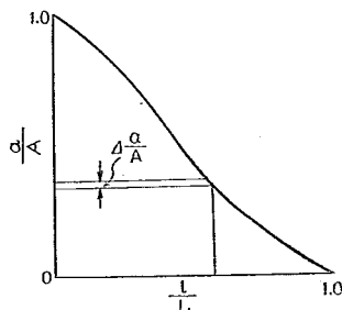
図-5 面積—距離曲線
