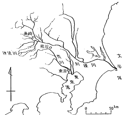
図-2 利根川支川神流川
