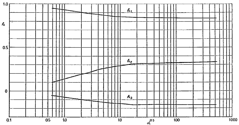
付図-1-A-4 ①ゲタの L/4 断面に対する k
