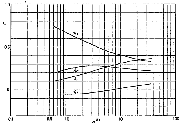
付図-1-B-8 ②ゲタの L/2 断面に対する k
