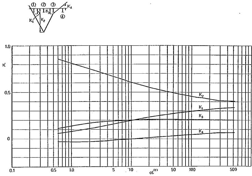
付図-1-A-15 ③ゲタの L/4 断面に対する K
