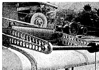
写真-8 第5回吊かご流速計用ウィンチ
