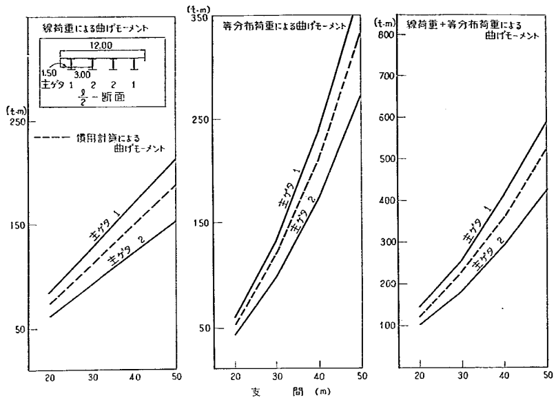
付図-2-B-5 L/2 断面の曲げモーメント
