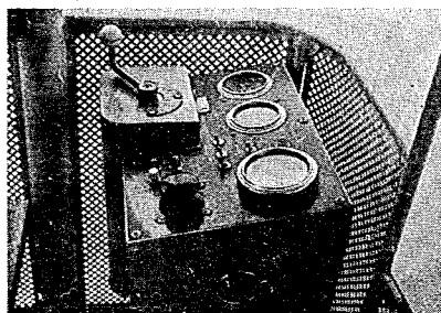
写真-7 第5回吊かご内部
