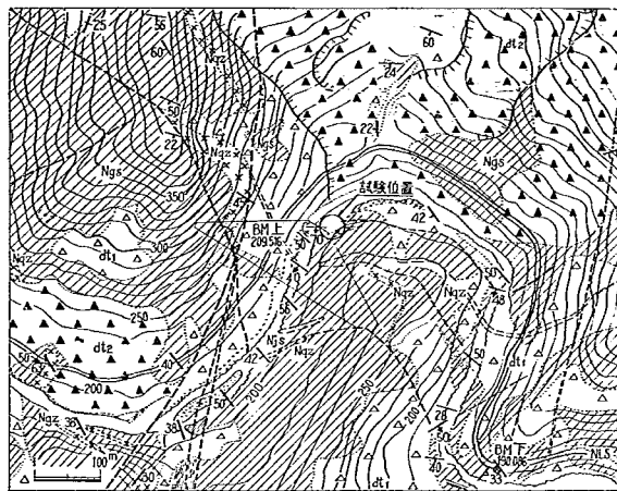
図-2(a) 原案ダム試験位置付近平面図
