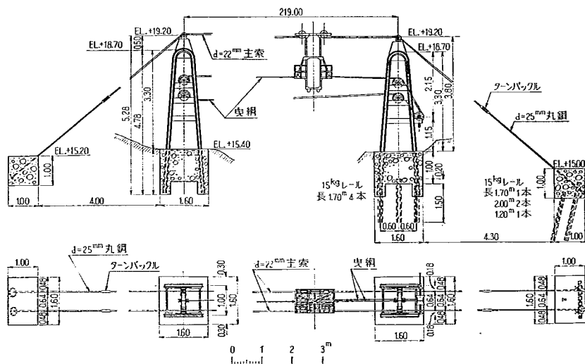
図-4 信濃川第2床固上流吊かご
