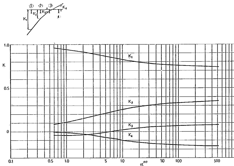
付図-1-A-9 ①ケタの L/2 断面に対する K
