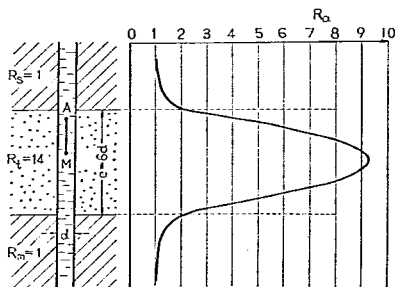
図-8 (a) 2極法特性曲線
