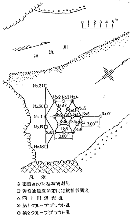
図-1 グラウト孔ならびに観測孔配置図(下久保)
