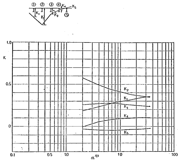
付図-1-B-11 ②ゲタの L/2 断面に対する K
