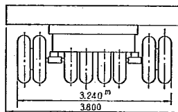
図-3 日通式180 t 積載トレーラー
