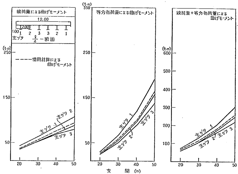
付図-2-A-9' L/4 断面の曲げモーメント
