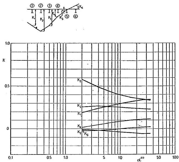
付図-1-B-17 ③ケタの L/2 断面に対する K
