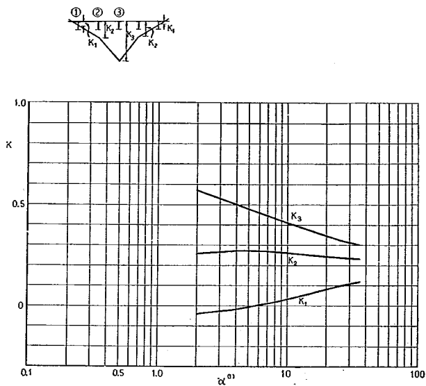
付図-1-B-13 ③ケタの L/2 断面に対する K
