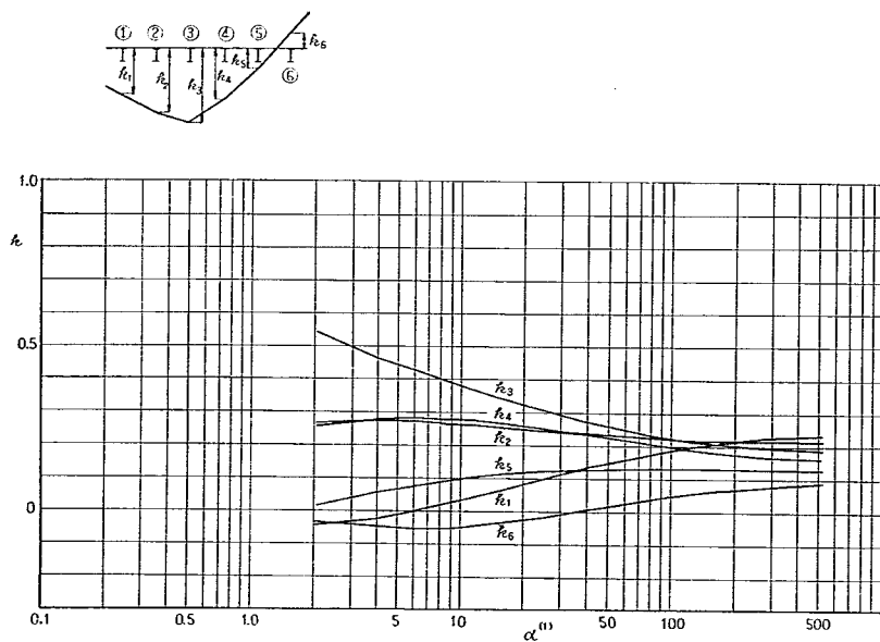
付図-1-A-38 ③ケタの L/2 断面に対する k
