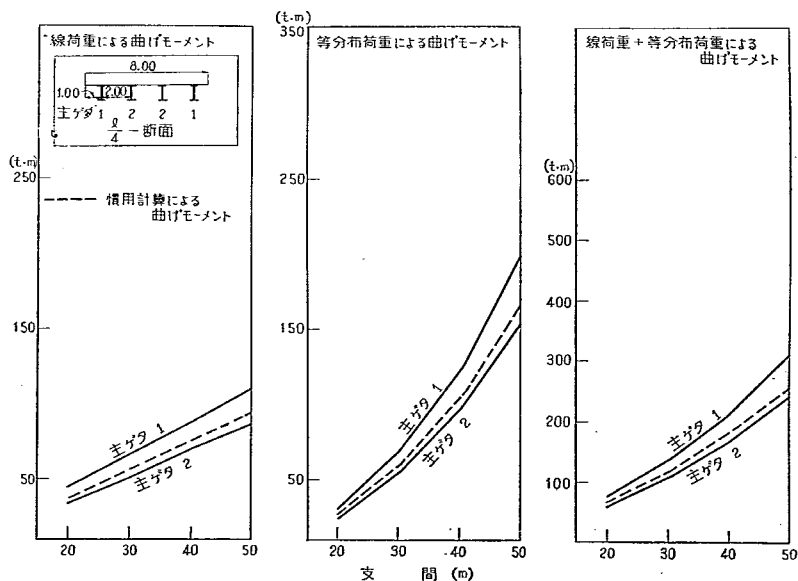
付図-2-A-4' L/4 断面の曲げモーメント
