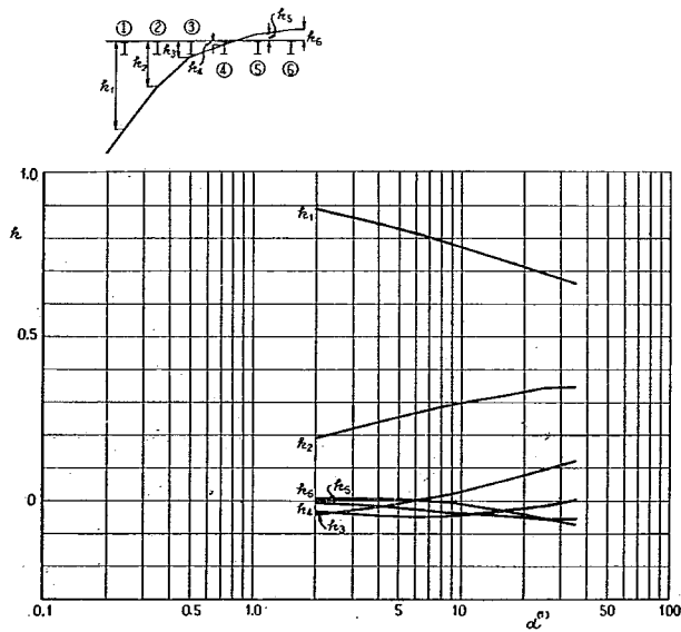
付図-1-B-16 ①ゲタの L/2 断面に対する k
