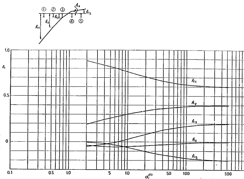
付図-1-A-18 ①ケタの L/2 断面に対する k
