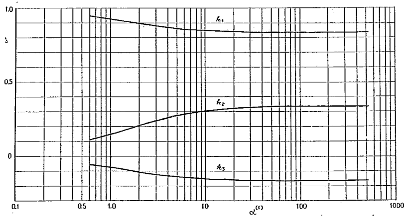
付図-1-A-2 ①ケタの L/2 断面に対する k
