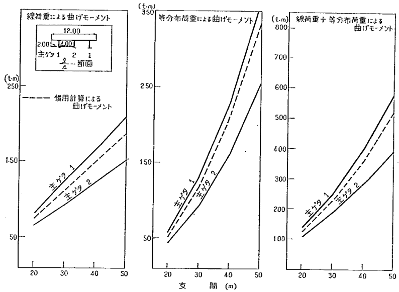
付図-2-A-3' L/4 断面の曲げモーメント
