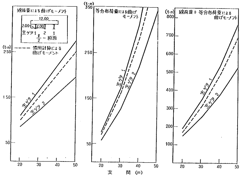
付図-2-A-3 L/2 断面の曲げモーメント
