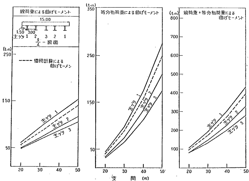
付図-2-B-8' L/4 断面の曲げモーメント
