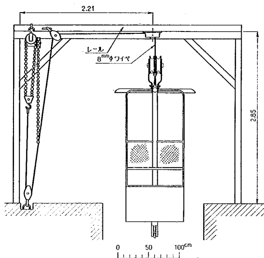
図-15 吊かご持上げ装置
