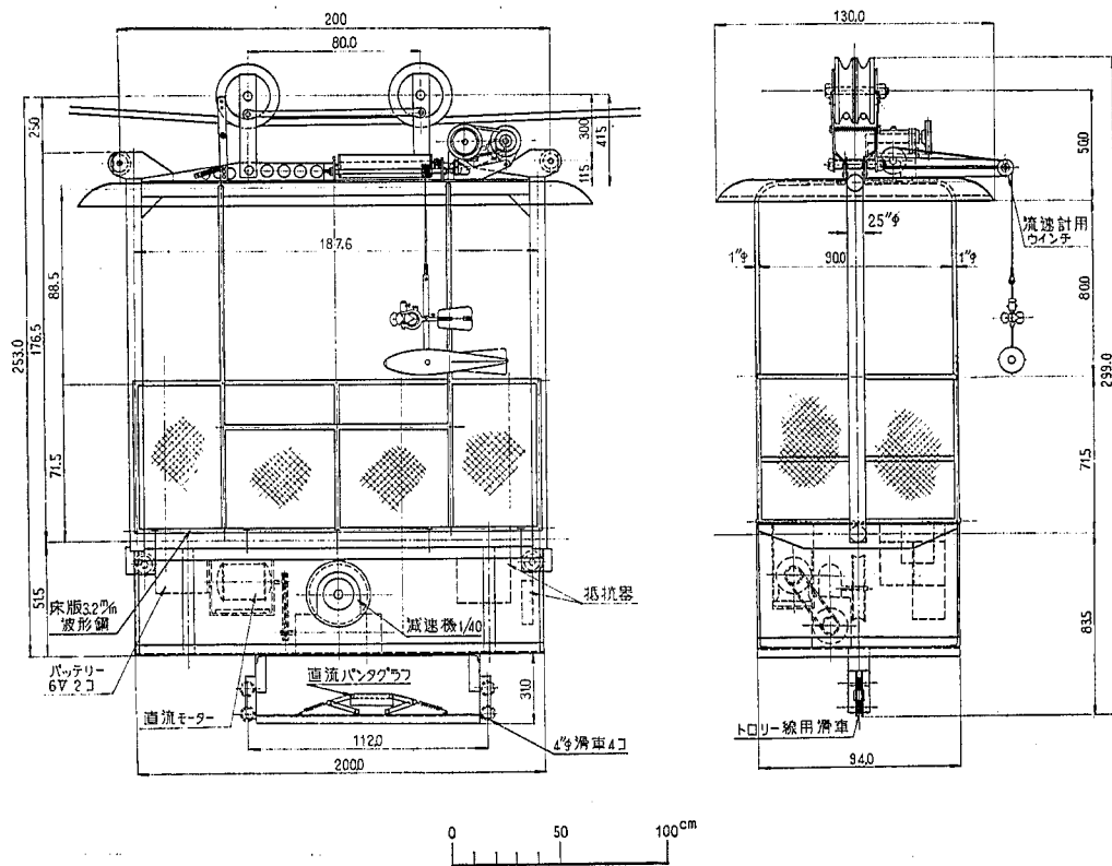
図-11 第 4 回 吊 か ど
