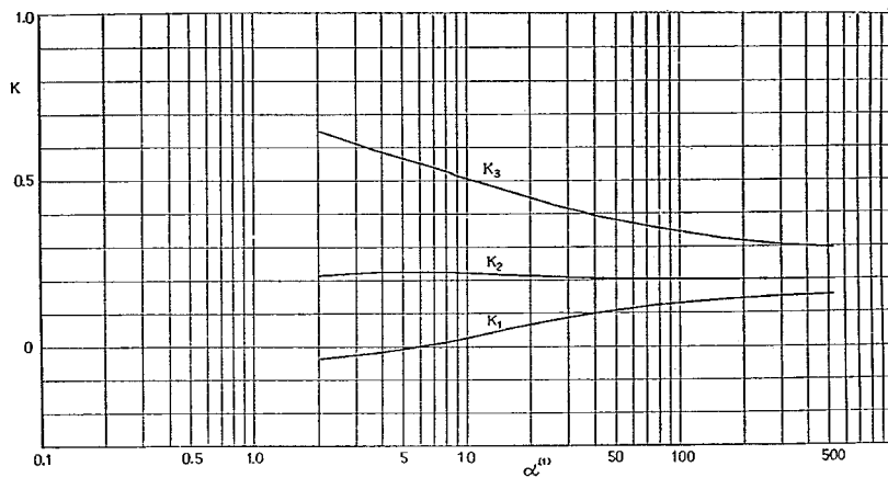
付図-1-A-25 ③ヶタの L/2 断面に対する K
