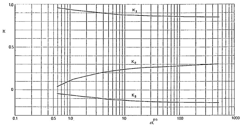
付図-1-A-1 ①ケタの L/2 断面に対する K
