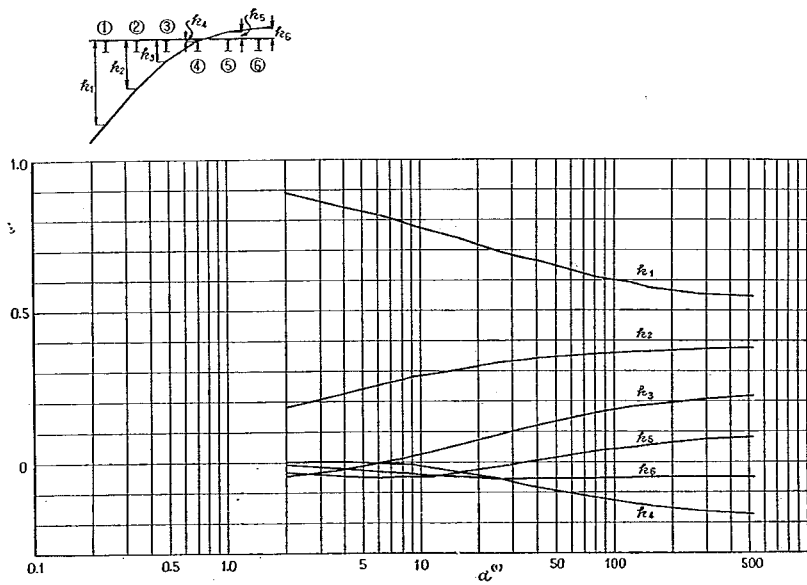
付図-1-A-32 ①ゲタの L/4 断面に対する k
