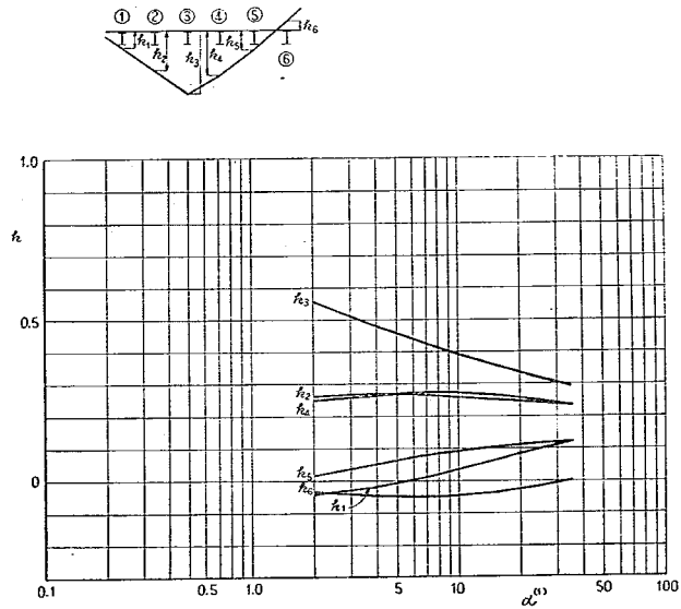
付図-1-B-20 ③ゲタの L/2 断面に対する k
