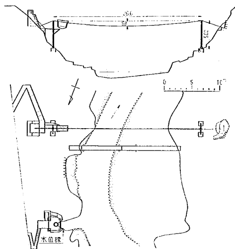
図-17 乙父地点流量観測所
