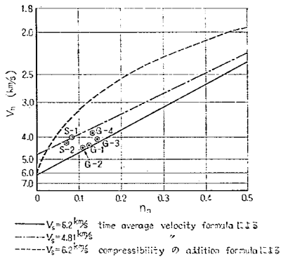
図-16 弾性波速度と空隙率の関係
