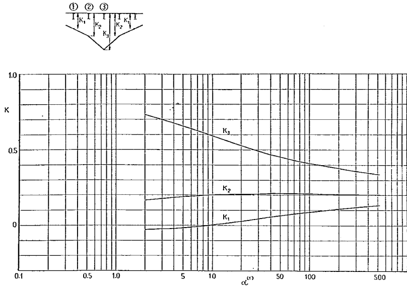
付図-1-A-27 ③ゲタの L/4 断面に対する K
