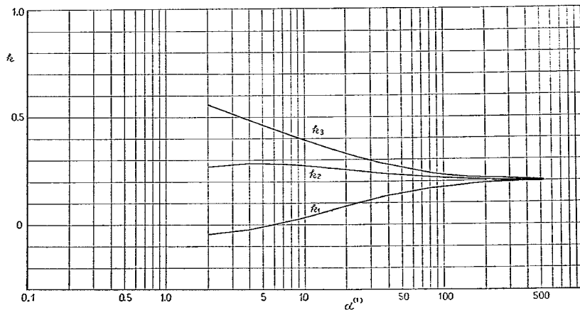
付図-1-A-26 ③ヶタの L/2 断面に対する k
