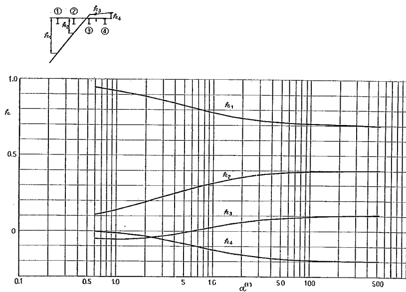
付図-1-A-10 ①ケタの L/2 断面に対する k
