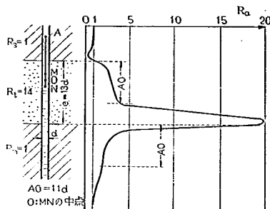
図-8 (b) 3極法特性曲線
