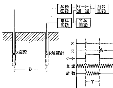
図-4 弾性波速度の測定
