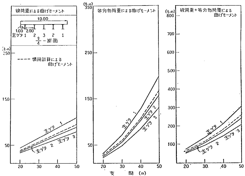
付図-2-B-7' L/4断面の曲げモーメント
