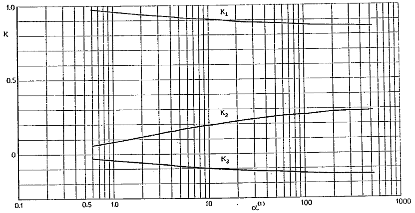
付図-1-A-3 ①ゲタの L/4 断面に対する K
