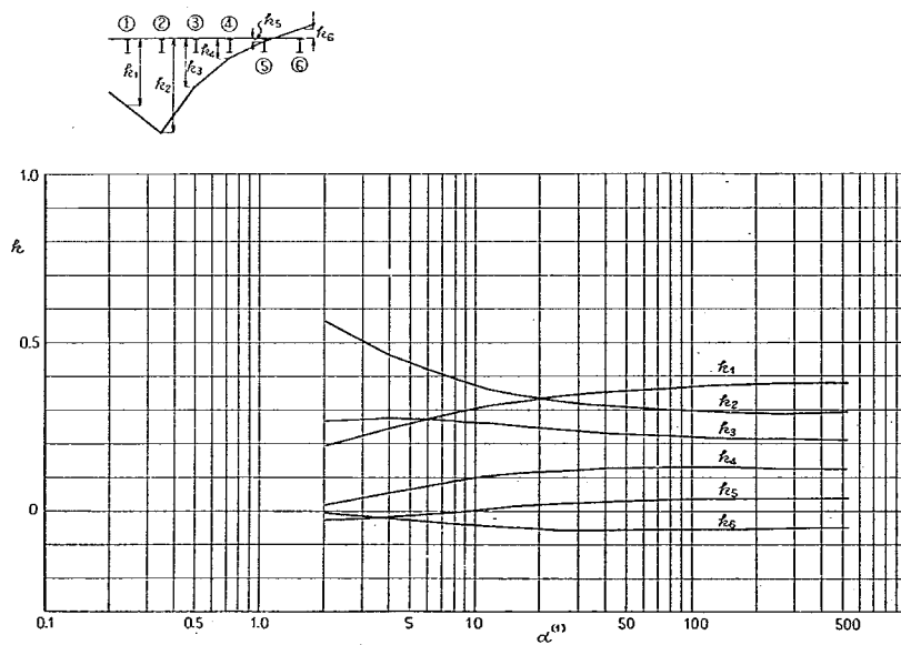
付図-1-A-34 ③ケタの L/2 断面に対する k
