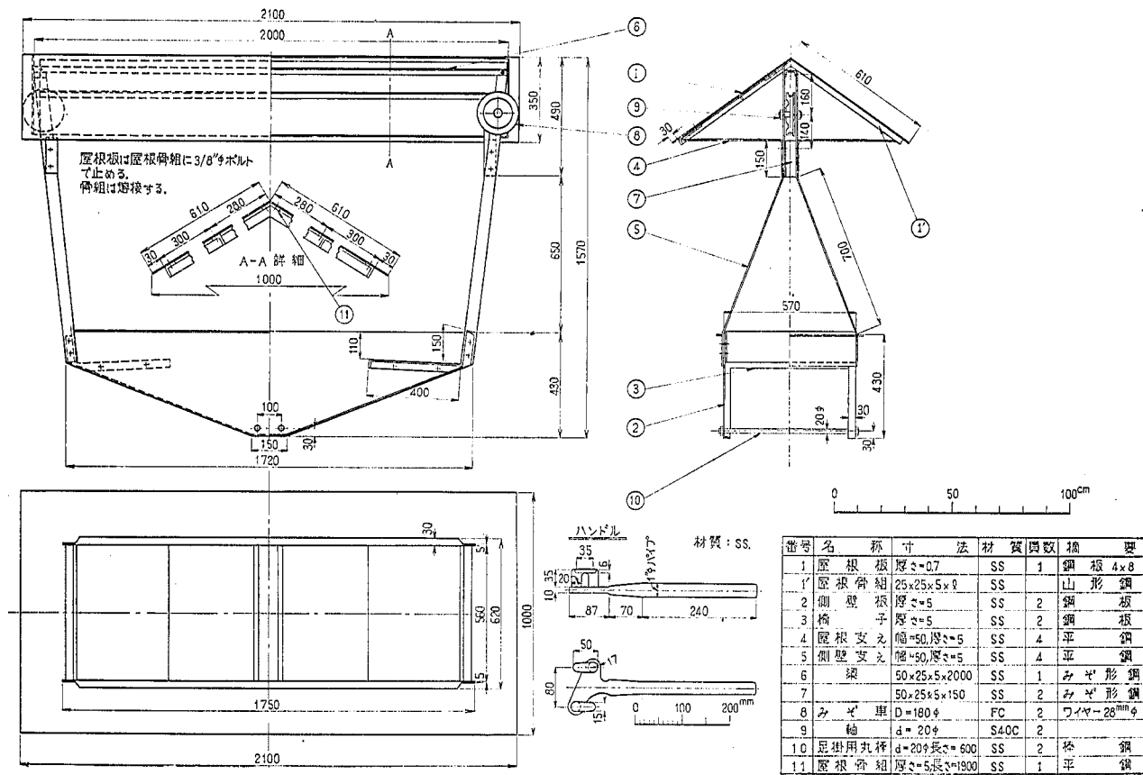
図-18 吊 か こ
