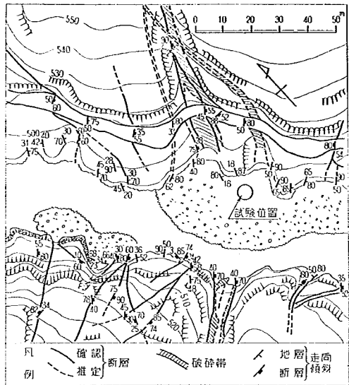
図-2(a) 原原ダム試験位置付近平面図
