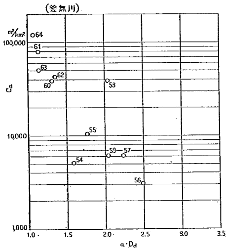
図-36 (5) 崩壊面積と流域係数
