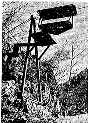
写真-11 支 塔
