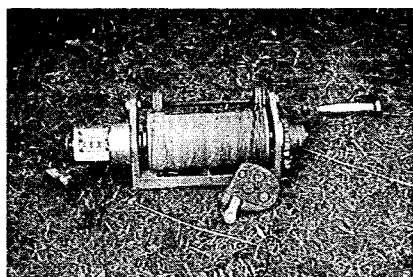
写真-20 吊かご用ウィンチ (詳細)
