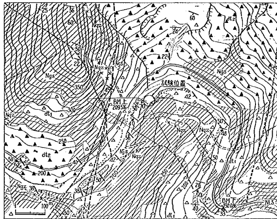
図-2(a) 原原ダム試験位置付近平面図
