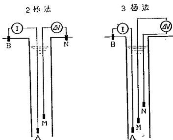
図-7 電気検層法による比抵抗の測定
