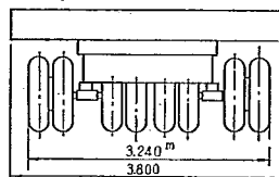
図-3 日通式180 t 積載トレーラー
