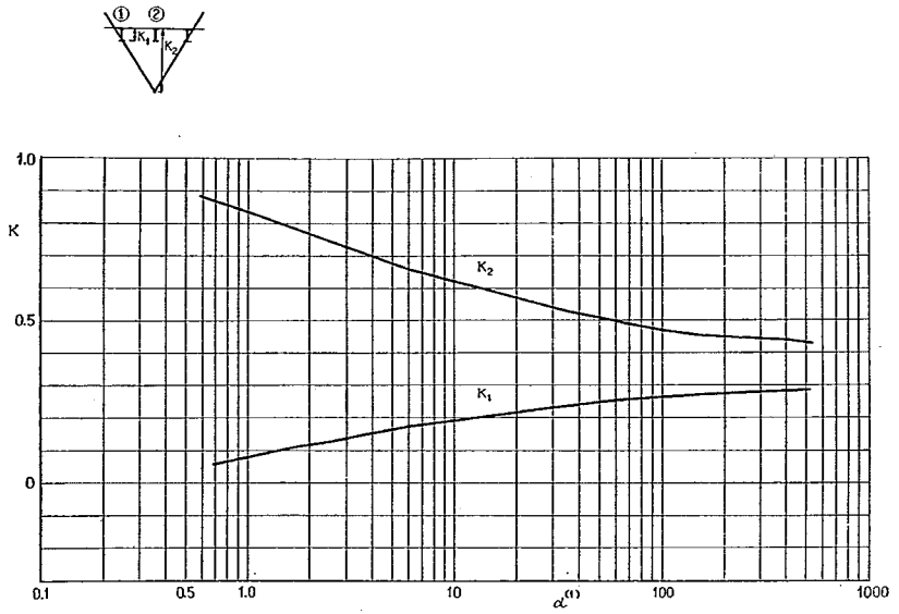
付図-1-A-7 ②ゲタの L/4 断面に対する K
