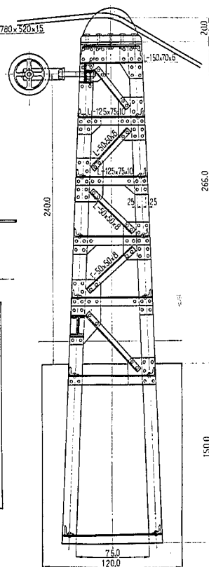
図-7 支塔
