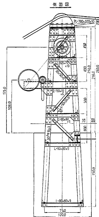
右岸側支塔
