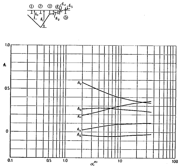
付図-1-B-12 ②ゲタの L/2 断面に対する k
