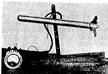
写真-31 ダイナモ流速計 (土研)
