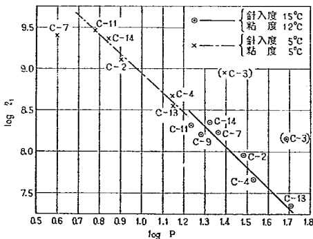
図-18 針入度と粘度との関係
