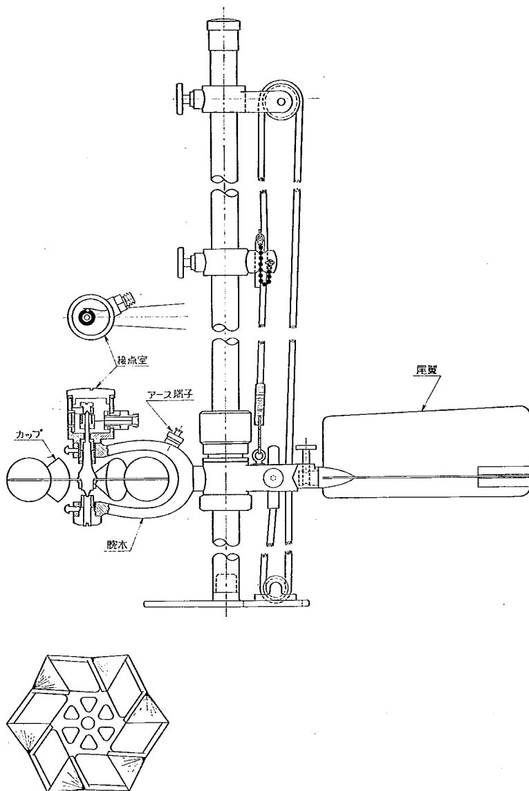
図-9 小型プライス流速計
