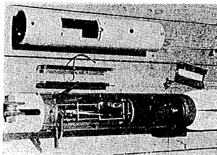
写真-21 III型水深流速計①
