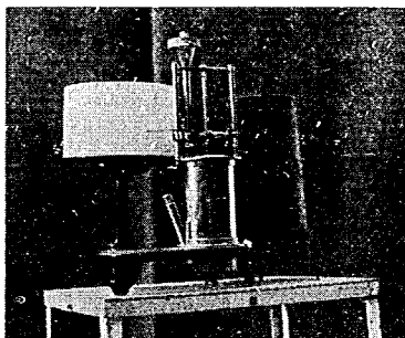
写真-3 10日巻雨量計
