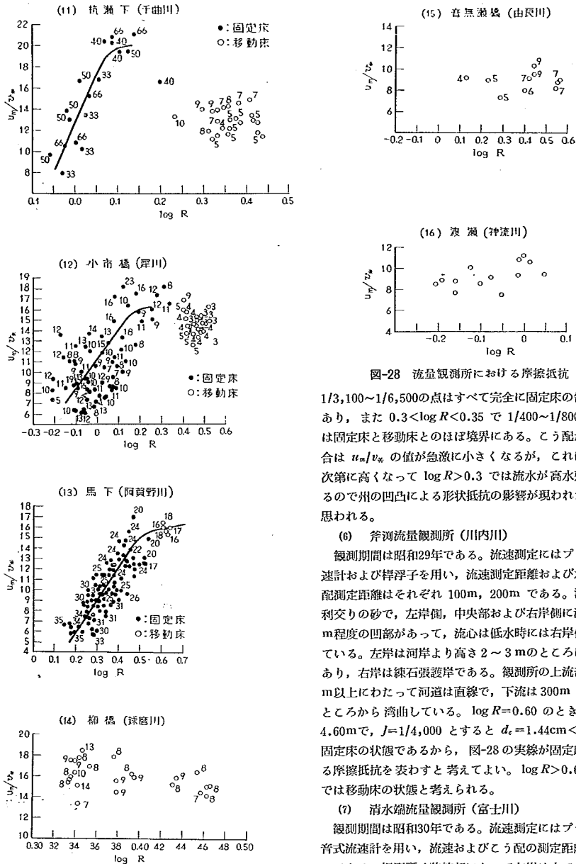
図-28 流量観測所における摩擦抵抗
