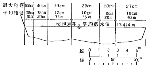
図-38 馬下観測所の砂礫の分布状態
