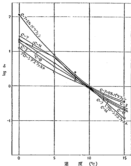
図-33 時間-温度換算の移動因子 a_T の温度依存性
