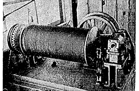
写真-28 流速計遠隔操作用ウインチ①
