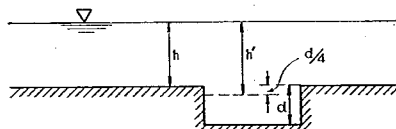
図-19 実験水路の縦断面図
