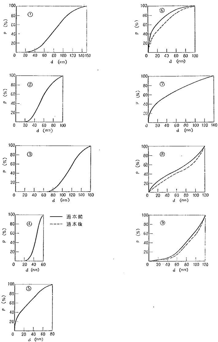
図-5 粒度累加曲線 (実線：通水前，点線：通水後)
