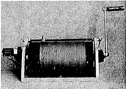
写真-26 流速計重し用ウインチ
