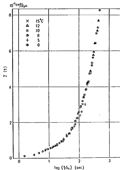
図-28 C-3のクリープコンプライアンスのマスターカーブ ( T_0=10^\circ\text{C} )
