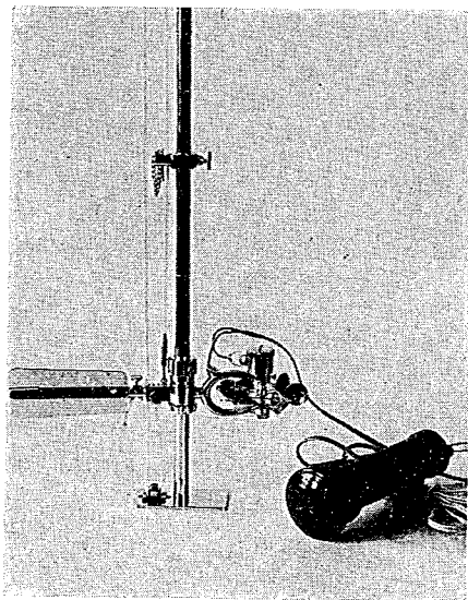
写真-30 小型ブライス流速計
