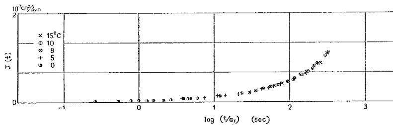
図-29 C-7 + 5%結晶性パラフィンのクリープコンプライアンスのマスターカーブ ( T_0=10^\circ\text{C} )
