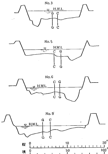
図-50 日川横断面図
