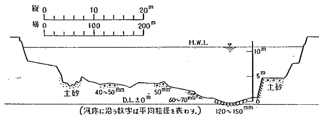
図-36 具同観測所の砂礫の分布状態
