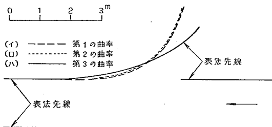
図-59 霞堤の曲率
