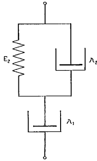
図-11 3要素粘弾性模型
