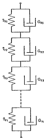
図-35 Voigt 要素の直列結合
