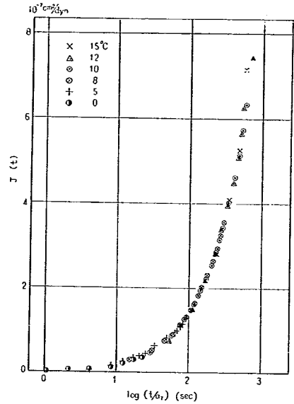
図-25 C-7のクリープコンプライアンスのマスターカーブ ( T_0=10^\circ\text{C} )
