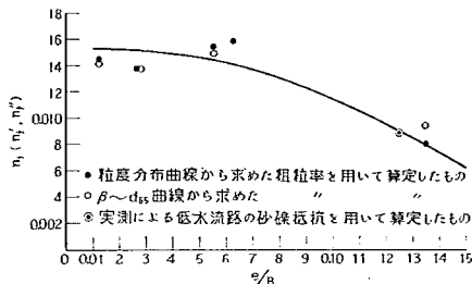
図-35 形状抵抗による粗度
