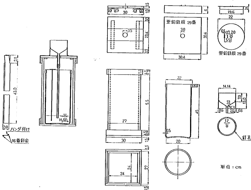
図-3 管谷式雨量計
