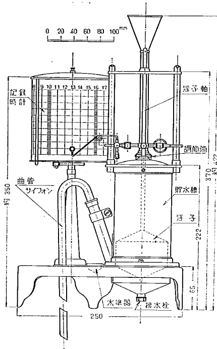
図-1 日巻雨量計(曲管サイフォン)
