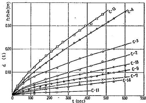
図-6 各種ストレートアスファルトのクリープ曲線 (自重による) 温度 5°C
