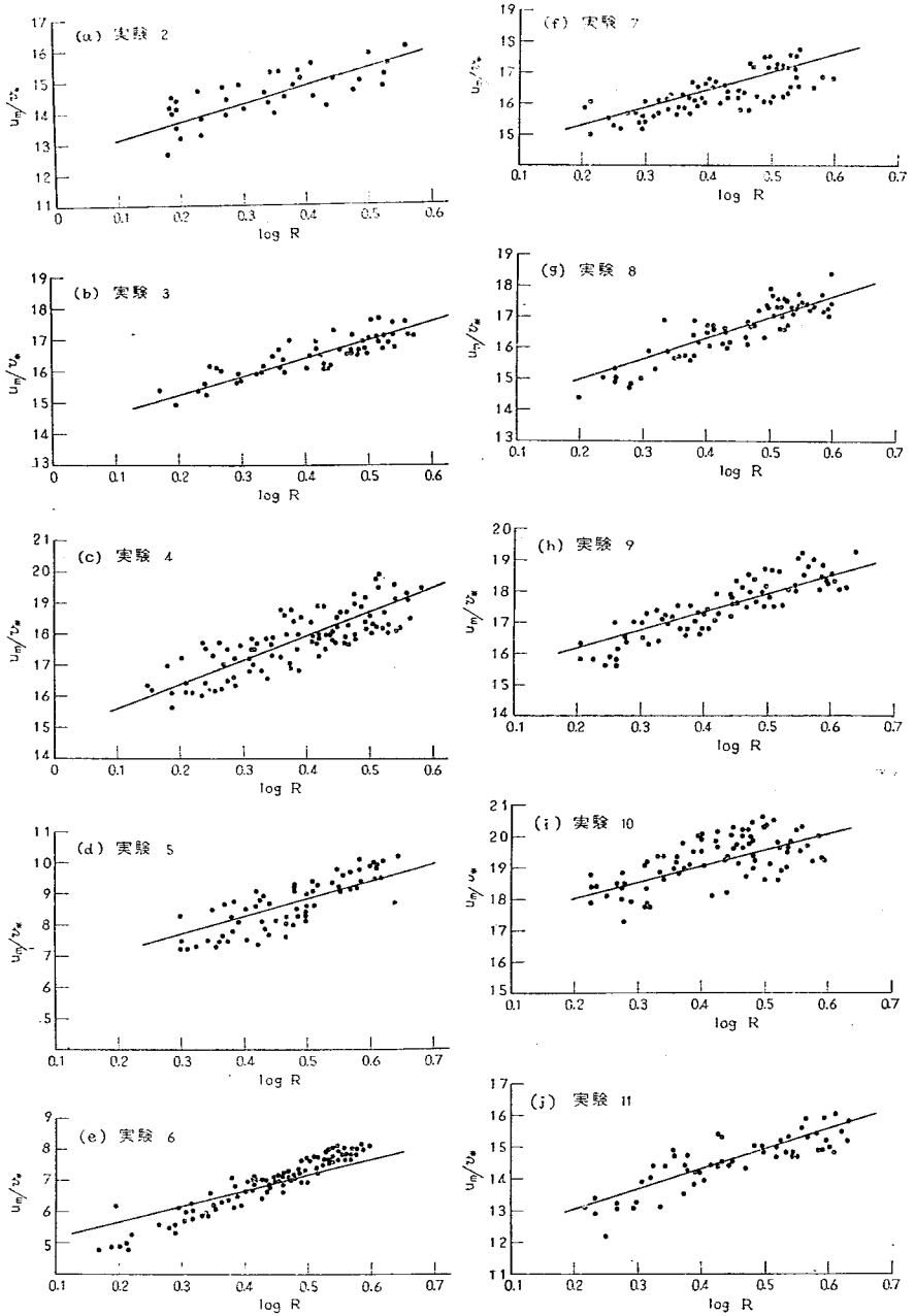
図-18 \frac{u_m}{v_*} と \log R との関係
