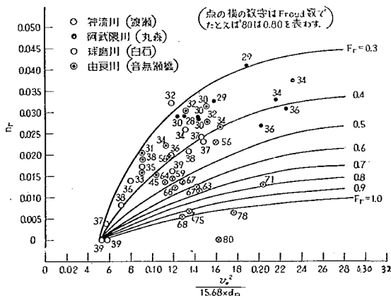
図-42 移動床の粗度係数
