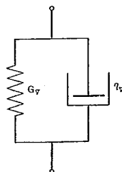
図-4 Voigt 模型
