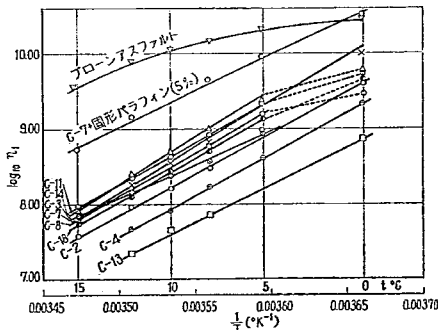
図-15 \eta_1 の温度による変化
