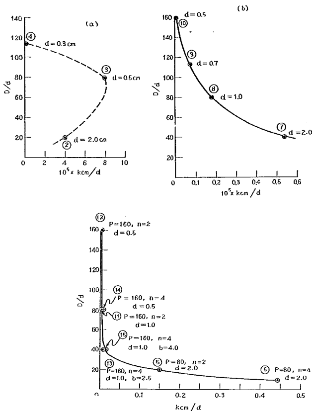
図-21 溝による粗度
