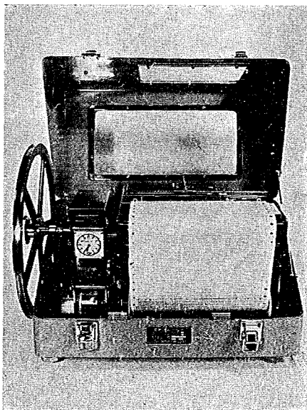
写真-15 水研式長期巻水位計
