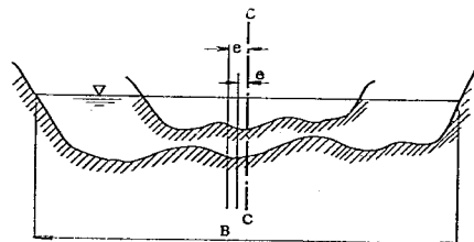
図-34 (b) 河川の横断形状
