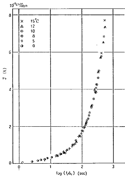
図-27 C-18のクリープコンプライアンスのマスターカーブ ( T_0=10^\circ\text{C} )
