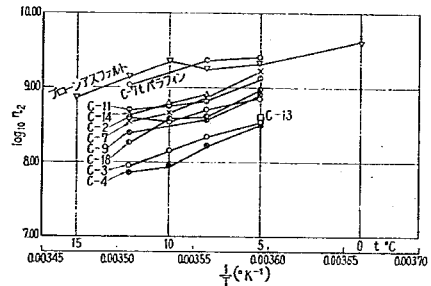
図-16 \eta_2 の温度による変化
