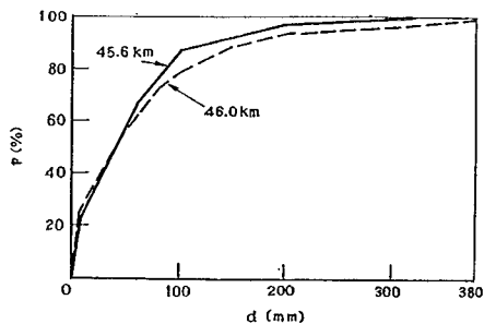
図-44 粒度分布曲線 (渡良瀬川)
