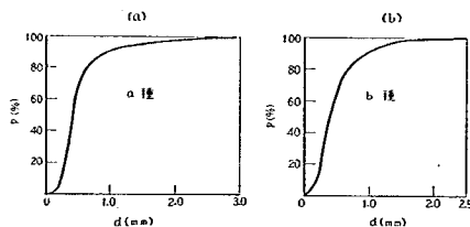
図-56 粒度分布曲線
