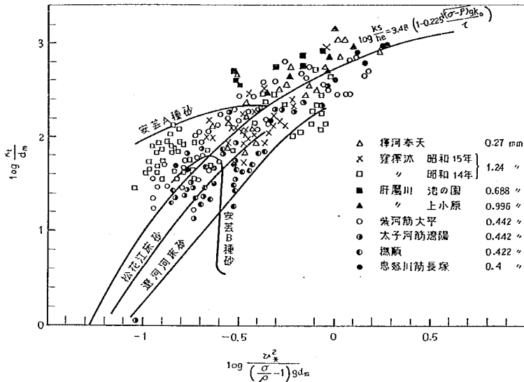
図-23 河 川 の 粗 度
