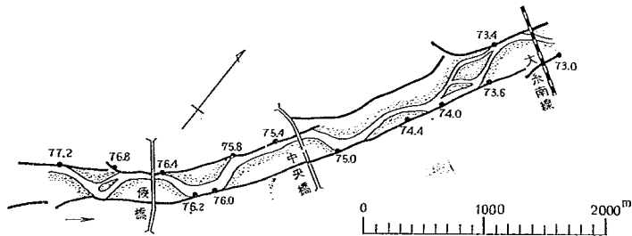
図-47 梓川平面図
