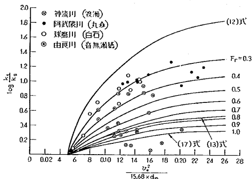
図-41 移動床の粗度
