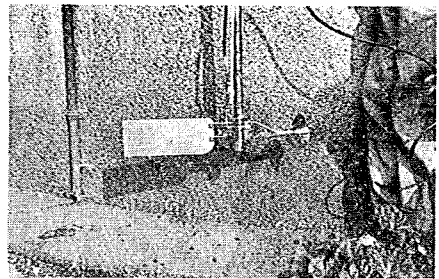
写真-1 森式流速計
