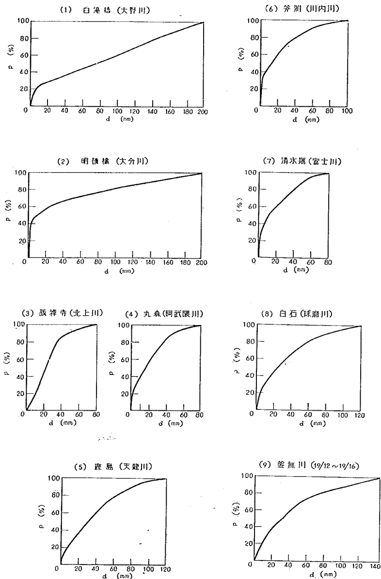
図-27 流量観測所付近の河床物質の粒度累加曲線
