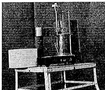
写真-4 10日巻雨量計
