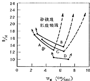
図-54 砂礫堆の形成領域
