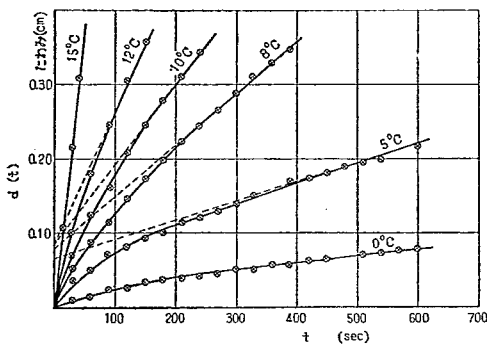
図-7.b ストレートアスファルトC-3(アラビヤ)のクリープ曲線(自重による)
