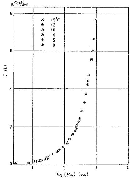
図-26 C-14のクリープコンプライアンスのマスターカーブ ( T_0=10^\circ\text{C} )
