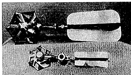
写真-24 プライス流速計、小型プライス流速計
