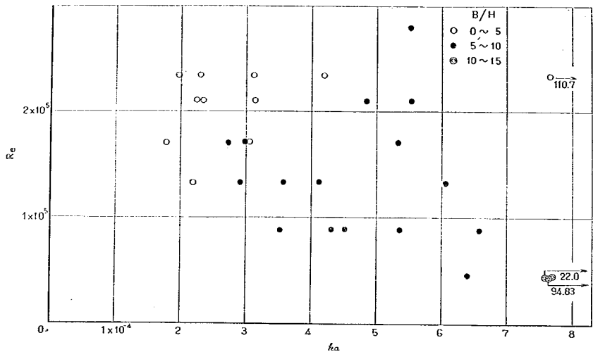
図-8 k_a に対するレイノルズ数の影響 (ゴムラバー張り水路)
