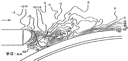
図-62 假堤付近等高線図 (水深 13cm, 通水時間 5分)
