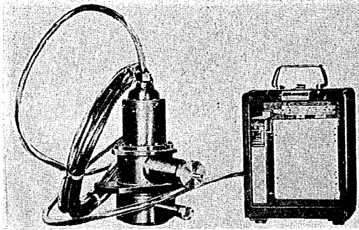
写真-16 管谷式水位計 べきである。
