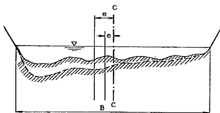
図-34 (a) 河川の横断形状
