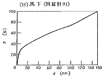
図-27 流量観測所付近の河床物質の粒度累加曲線
