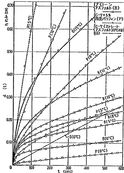
図-8 ブrownアスファルトおよび固形パラフィン添加ストレートアスファルトのクリープ曲線(中央部に528.5の荷重)
