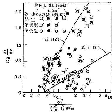
図-24 移動床の粗度
