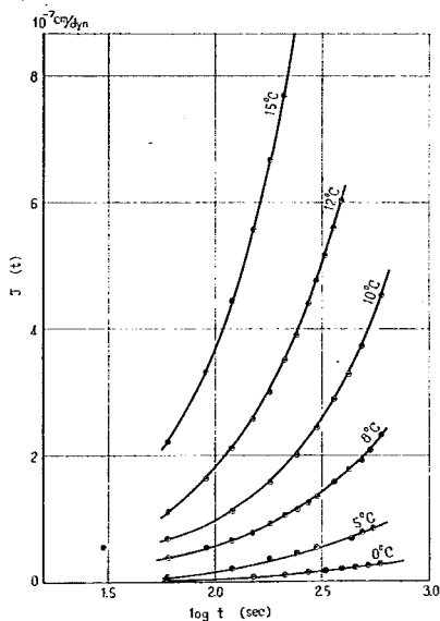
図-20 C-14のクリープコンプライアンス曲線
