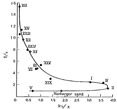
図-14 H. Schlichting の実験による粗度
