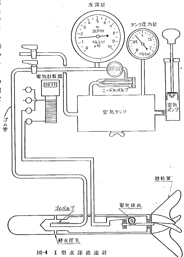
図-4 I型水深流速計
