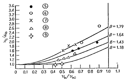
図-6 相当粗度と摩擦速度との関係
