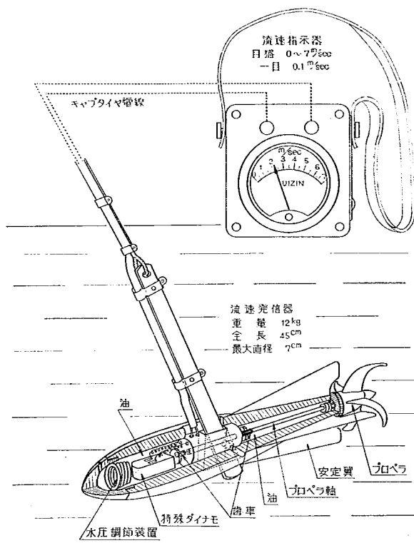
図-10 ダイナモ流速型(土研)
