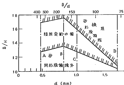
図-55 砂礫堆の形成領域
