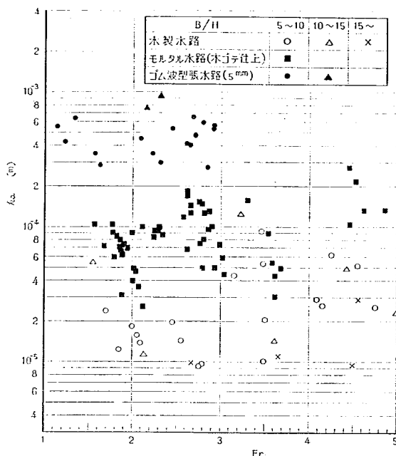
図-6 フルード数による k_a の変化
