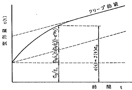
図-10 4要素粘弾性模型のクリープ曲線 (変形の時間による変化)
