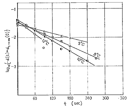
図-13 C-7のクリープ曲線の \log_{10} \{-d(t) + d_{t \rightarrow \infty}(0)\} と時間 t との関係
