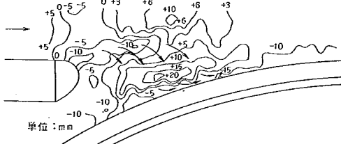
図-61 假堤付近等高線図 (水深 5cm, 通水時間 5分)
