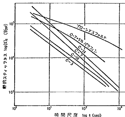
図-38 各試料の静的スティッフネス (基準温度10°C)
