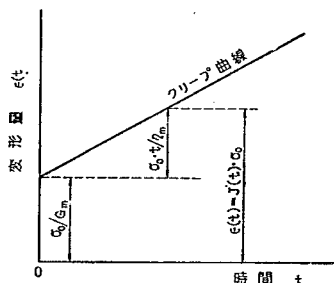
図-3 Maxwell 模型のクリープ曲線 (変形の時間による変化)
