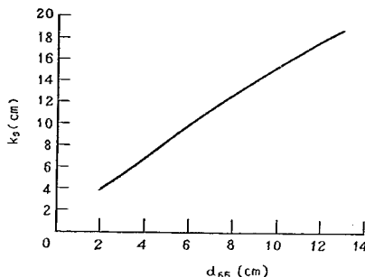
図-10 相当粗度と粒径との関係
