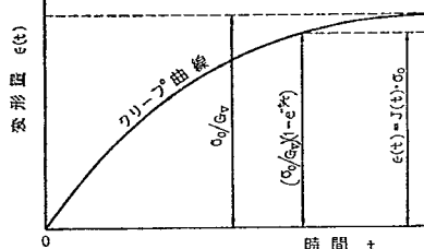
図-5 Voigt 模型のクリープ曲線 (変形の時間による変化)
