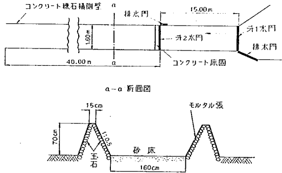
図-4 実験水路平面図
