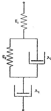
図-9 4要素粘弾性模型
