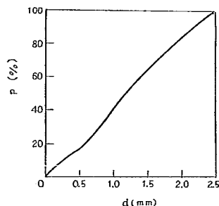
図-1 粒度累加曲線
