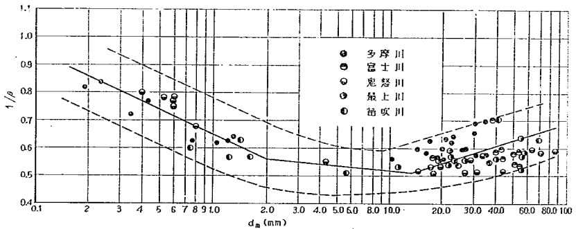
図-8 平均粒径と混合係数との関係
