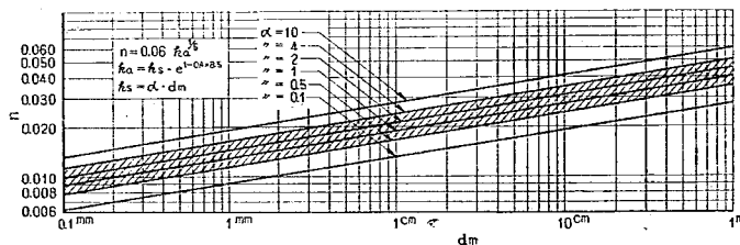
図-10 平均粒径による粗度係数の値
