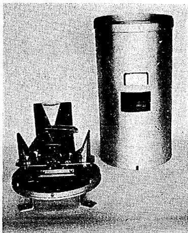
写真-8 転倒併式雨量計
