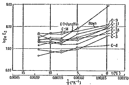
図-17 E_2 の温度による変化
