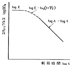
図-37 Maxwell 模型の静的スティッフネスの載荷時間による変化
