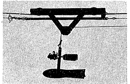
写真-29 流速計遠隔操作用ウインチ②
