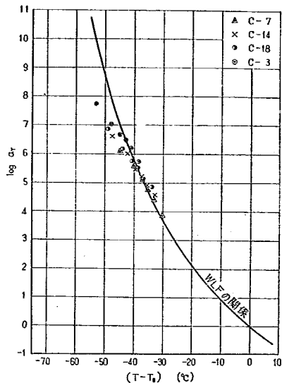
図-34 移動因子 a_T と (T - T_s) の関係 実線は WLF の式 \log a_T = -8.86(T - T_s) / \{101.6 + (T - T_s)\} をあらわす曲線
