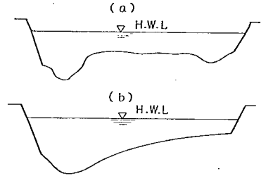
図-16 河川の横断面形状
