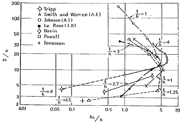
図-12 底面粗度
