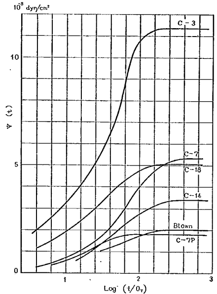
図-32 各試料のクリープ関数 (基準温度 10^\circ\text{C} )
