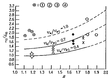
図-7 相当粗度と混合係数との関係
