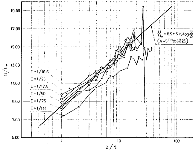
図-5 流速分布の例 (ゴムラバー張り水路, Q=0.1188\text{m}^3/\text{s} , 水路中央)
