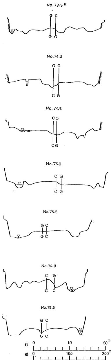
図-48 梓川横断面図
