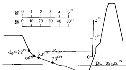
図-37 杭瀬下観測所の砂礫の分布状態
