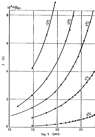
図-23 C-7 + 5%結晶性パラフィンのクリープコンプライアンス曲線
