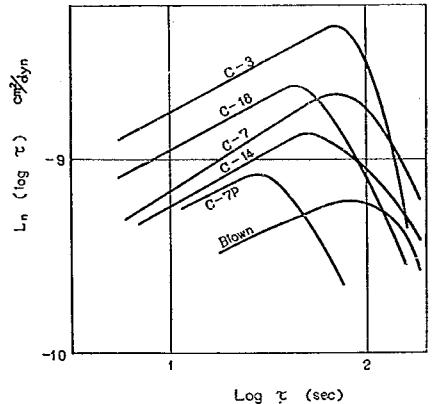
図-36 各試料の遅延スペクトル (基準温度10°C)
