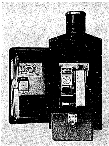
写真-2 長期巻自記雨量計
