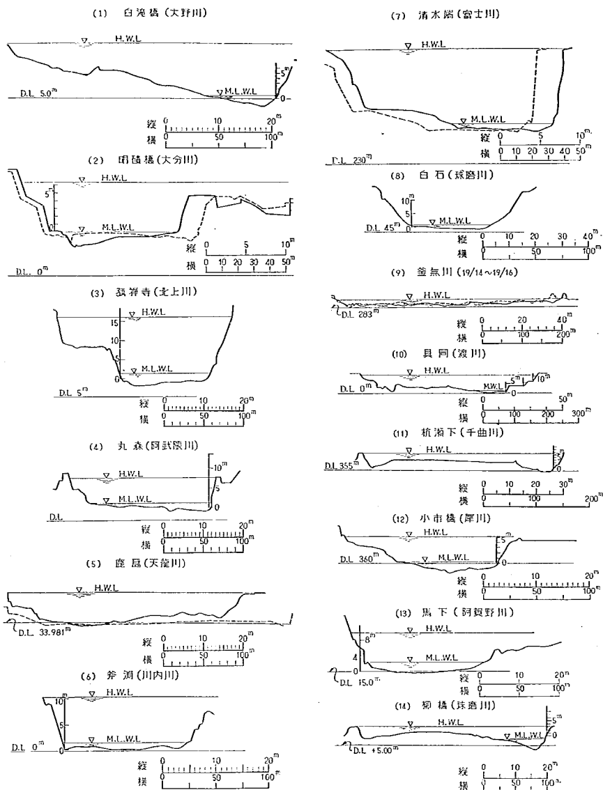
図-26 流量観測所の横断面図
