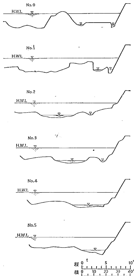
図-72 (b) 開国橋設堤部横断面図 (出水前)
