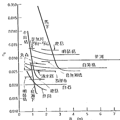
図-31 流量観測所における Manning の粗度係数 (固定床)
