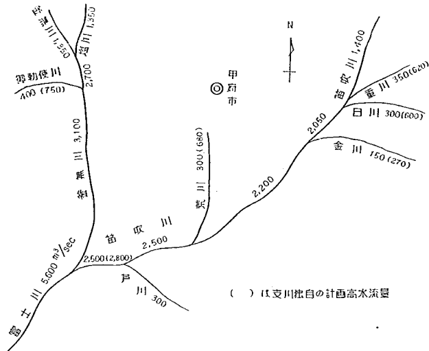
図-77 富士川流量配分図
