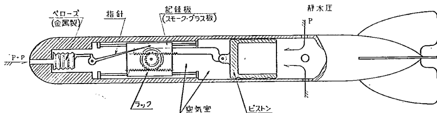
図-5 II型水深流速計
