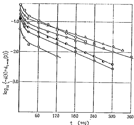
図-14 ブrownアスファルトのクリープ曲線の \log_{10}\{-d(t) + d_{\infty}(0)\} と時間 t との関係
