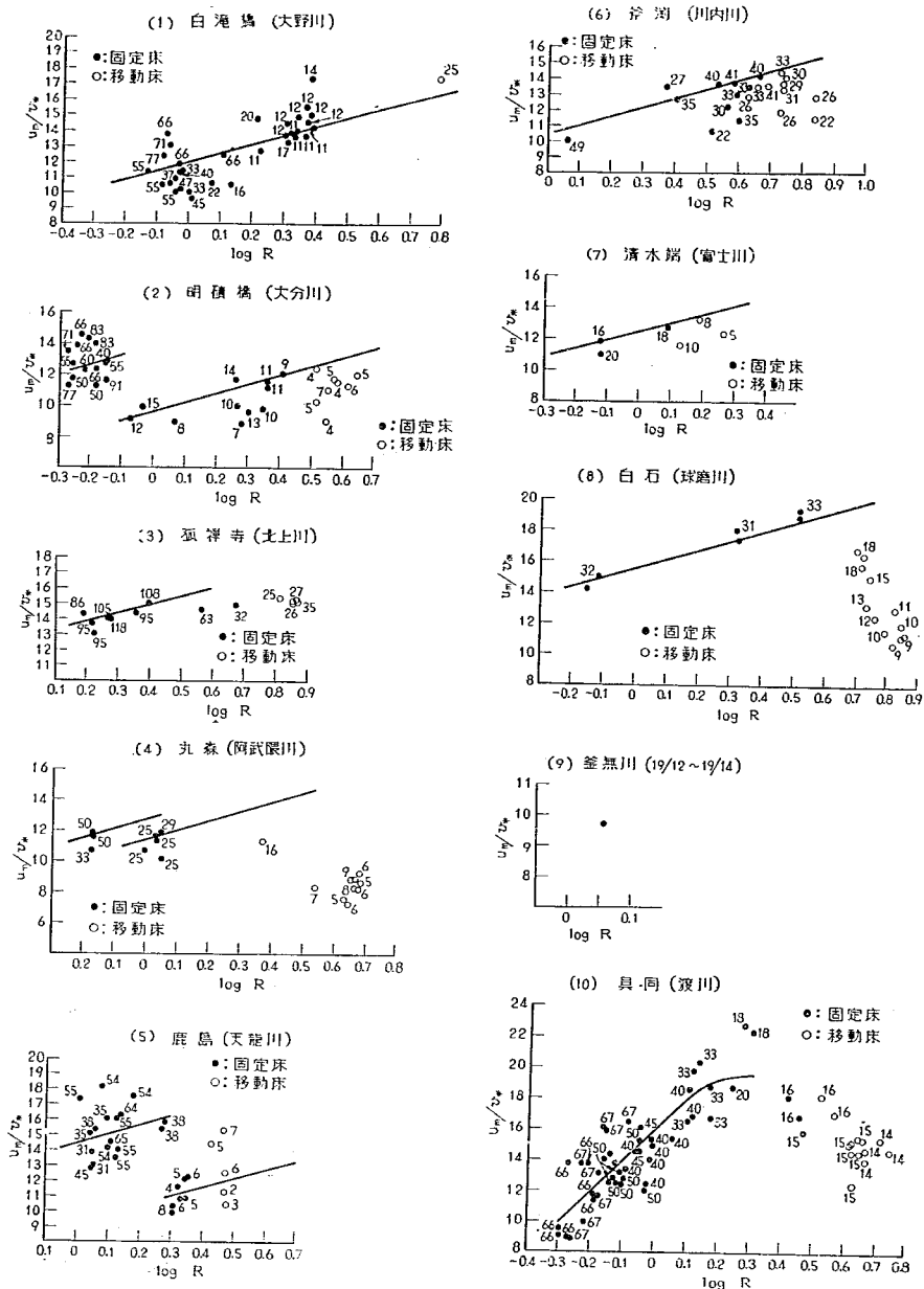
図-28 流量観測所における摩擦抵抗
