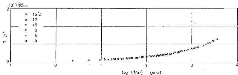
図-30 ブロームアスファルトのクリープコンプライアンスのマスターカーブ ( T_0=10^\circ\text{C} )
