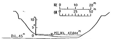
図-40 白石流量観測所横断面図
