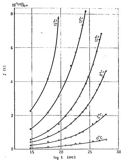
図-21 C-18のクリープコンプライアンス曲線
