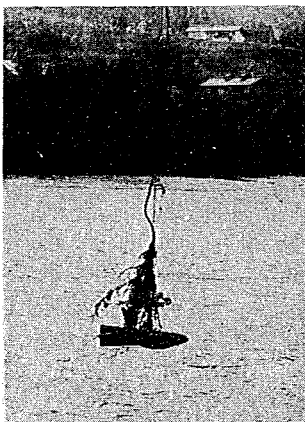
写真-17 ごみの巻きついた プライス流速計
