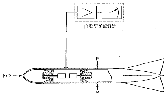
図-8 IV型水深流速計 ②
