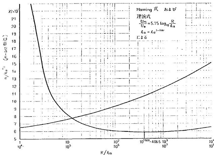
図-9 粗度係数 (n) の変化
