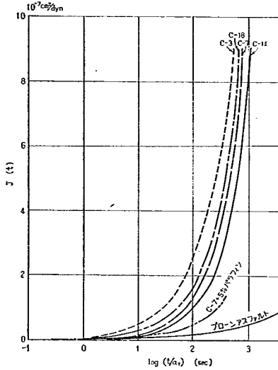
図-31 各試料のクリープコンプライアンスのマスターカーブ ( T_0=10^\circ\text{C} )
