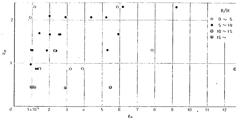
図-7 k_a に対するレイノルズ数の影響 (木製水路)
