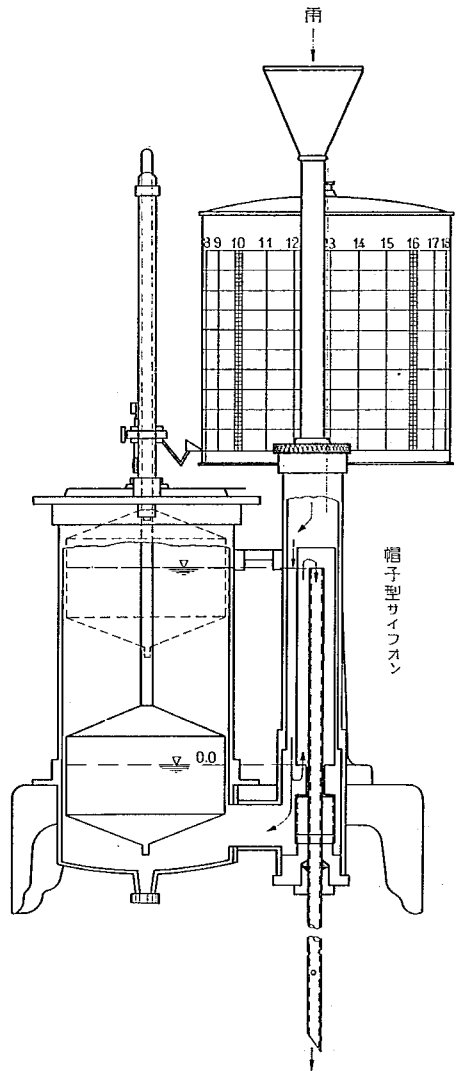
図-2 日巻自記雨量計(帽子型サイフォン)
