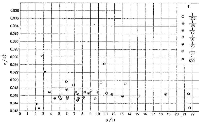
図-4 粗度係数におよぼす側壁の影響 (木製水路)
