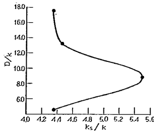
図-13 底面粗度（著者の実験による）
