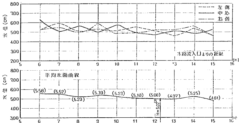
図-2 水面曲線の例 (木製水路, Q=0.0748 m 3 /s, I=1/16.6^\circ=0.06 )
