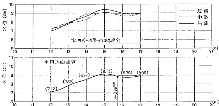
図-3 水面曲線の例 (ゴムラバー張り水路, Q=0.1188 \text{ m}^3/\text{scc} , I=1/12.5 )
