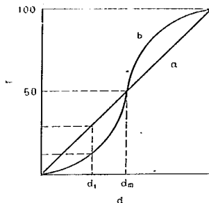
図-2 粒度累加曲線
