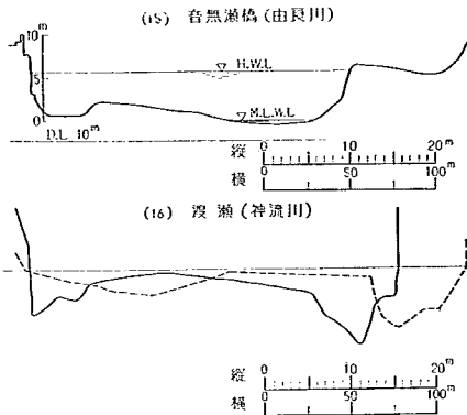
図-26 流量観測所の横断面
