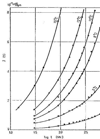
図-22 C-3のクリープコンプライアンス曲線
