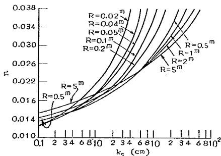
図-22 n と k_s との関係
