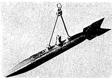
写真-23 IV型水深流速計 ①
