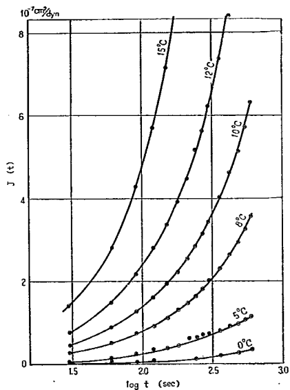
図-19 C-7のクリープコンプライアンス曲線
