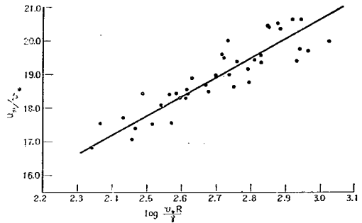
図-17 滑面の摩擦抵抗
