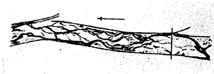
図-85 釜無川の乱流
