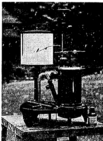
写真-1 日巻雨量計（曲管サイフォン式）
