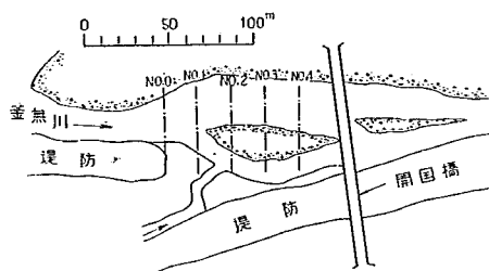
図-72 (a) 開国橋設堤平面図 (出水前)
