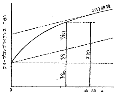
図-1 クリープコンプライアンス J(t) (単位応力を与えたときの変位) とその他の粘弾性諸量との関係
