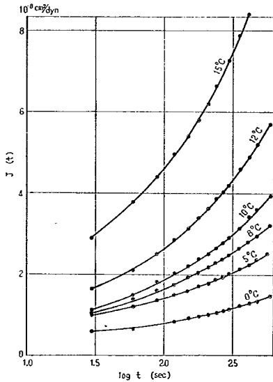
図-24 ブラウンアスファルトのクリープコンプライアンス曲線
