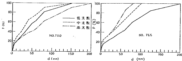
図-46 粒度分布曲線 (梓川)
