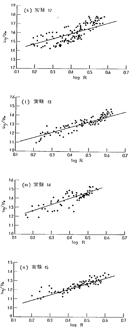
図-18 \frac{u_m}{v_*'} と \log R との関係
