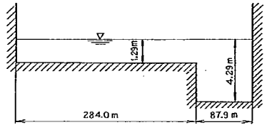
図-51 横断面図
