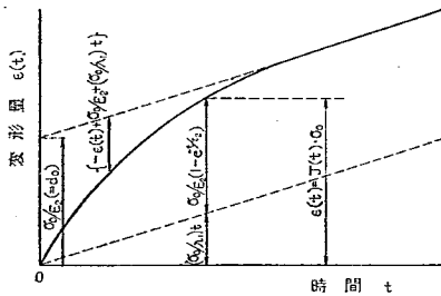
図-12 3要素粘弾性模型のクリープ曲線 (変形の時間による変化)
