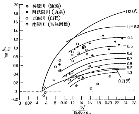
図-39 移動床の粗度
