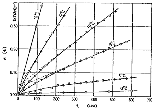
図-7.a ストレートアスファルトC-7(コーニング)のクリープ曲線(自重による)
