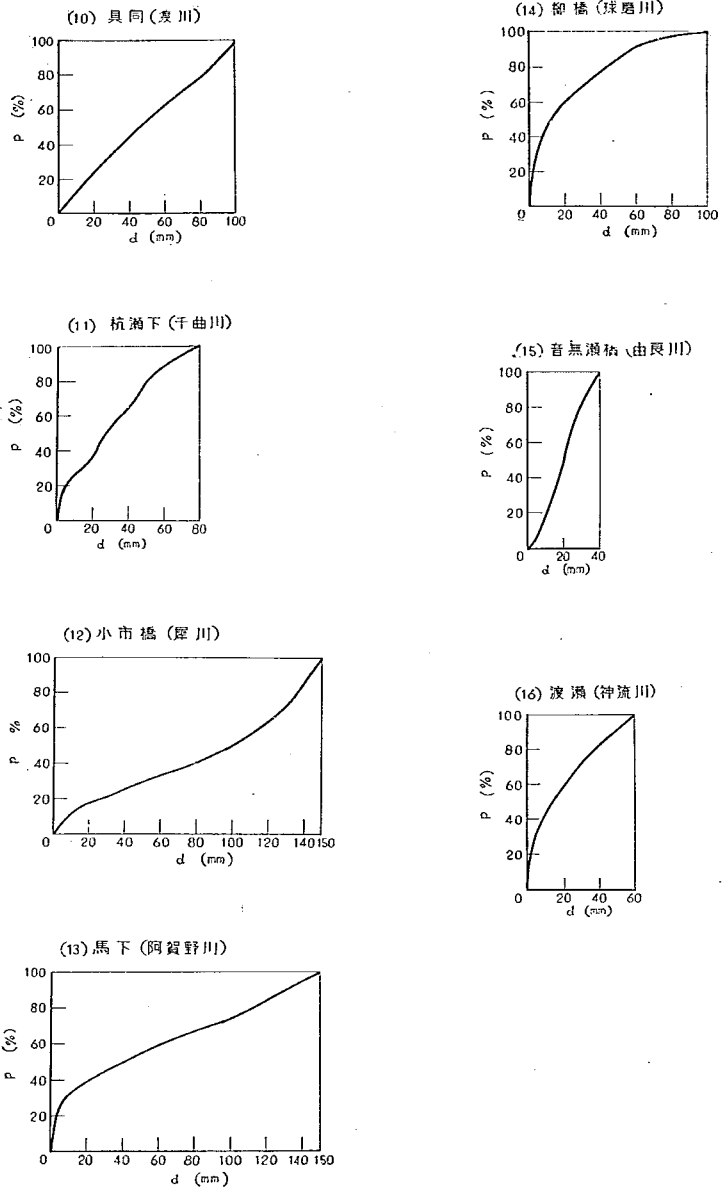
図-27 流量観測所付近の河床物質の粒度累加曲線
