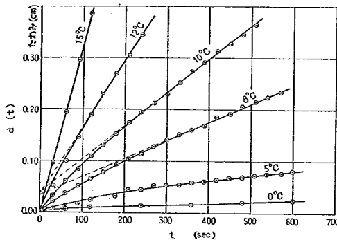
図-7.a ストレートアスファルトC-7(コーリング)のクリープ曲線(自重による)
