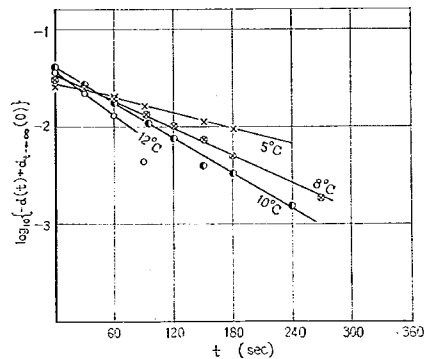
図-13 C-7のクリープ曲線の \log_{10} \{ -d(t) + d_{t \rightarrow \infty}(0) \} と時間 t との関係
