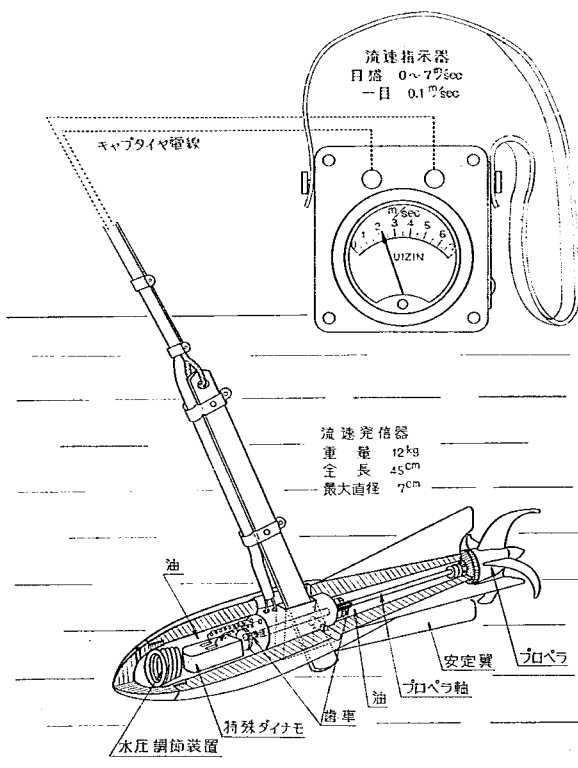
図-10 ダイナモ流速型(土研)
