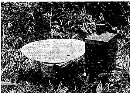
写真-7 風よけ（左側）右側は長期雨量計
