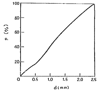
図-1 粒度累加曲線
