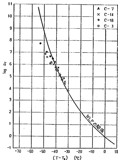
図-34 移動因子 a_T と (T - T_g) の関係 実線は WLF の式 \log a_T = -8.86(T - T_g) / \{101.6 + (T - T_g)\} をあらわす曲線
