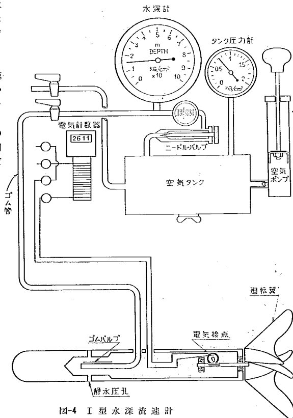
図-4 I型水深流速計
