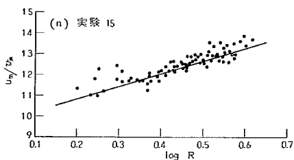
図-18 \frac{u_m}{v_*} と \log R との関係
