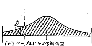
(e) ケーブルにかかる風荷重
