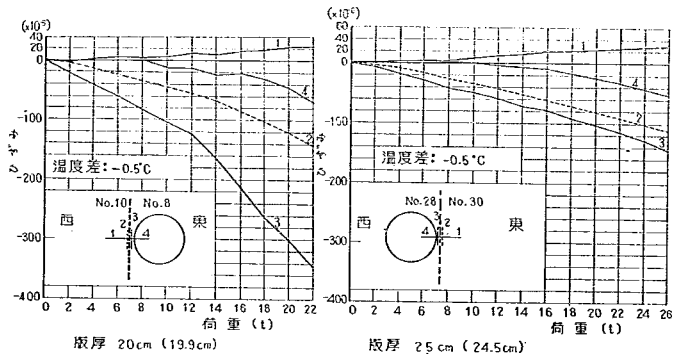
図-127 スリッパのあるめくら目地縁における荷重~ひずみ関係の1例
