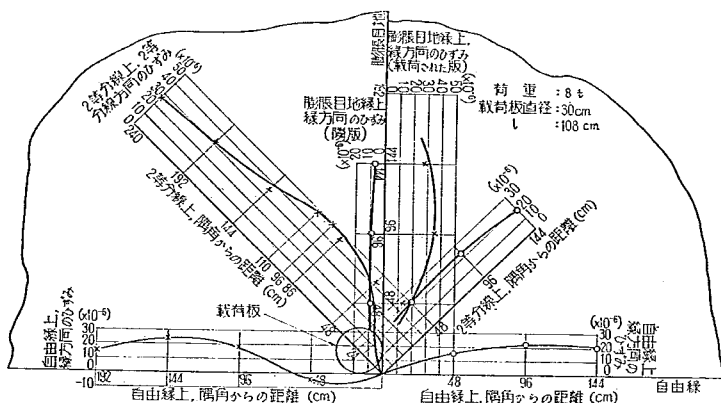
図-72 膨脹目地隅角部表面における平均ひずみ (第1回試験舗装, 版厚 25cm)
