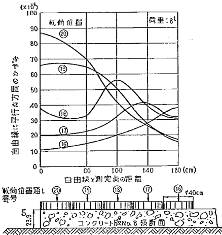
図-109 自由縁部におけるひずみと载荷位置の 関係の1例 (第2回試験舗装)
