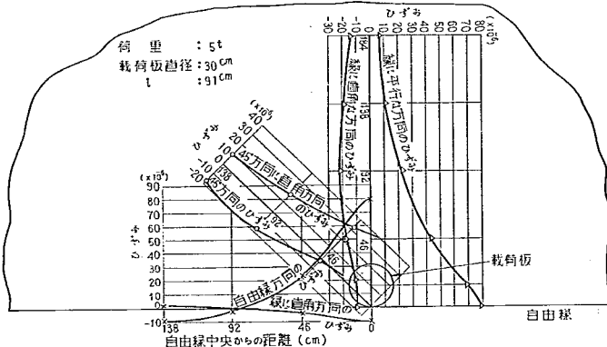
図-79 自由縁部底面における平均ひずみ (第1回試験舗装, 版厚20cm)
