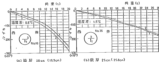
図-131 中央部における荷重～ひずみ関係の一例
