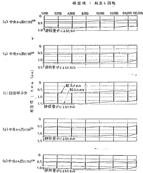
図-149 ひびわれ発生後の繰返し荷重による自由縁部の平均たわみと繰返し回数の関係
