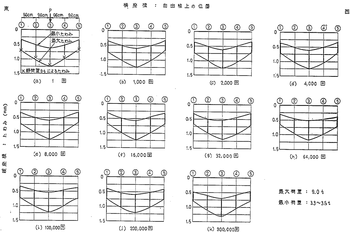
図-137 繰返し荷重による自由縁部の平均たわみ
