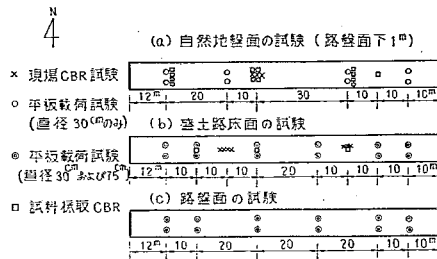
図-9 路床路盤試験位置図 (第1回試験舗装)
