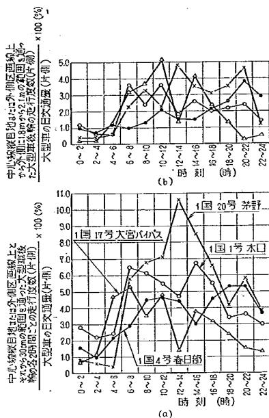
図-158 傾度極大の位置における大型車走行度数の時間変化
