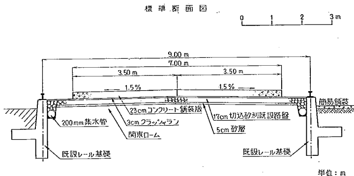
図-6 第2回試験舗装標準断面図
