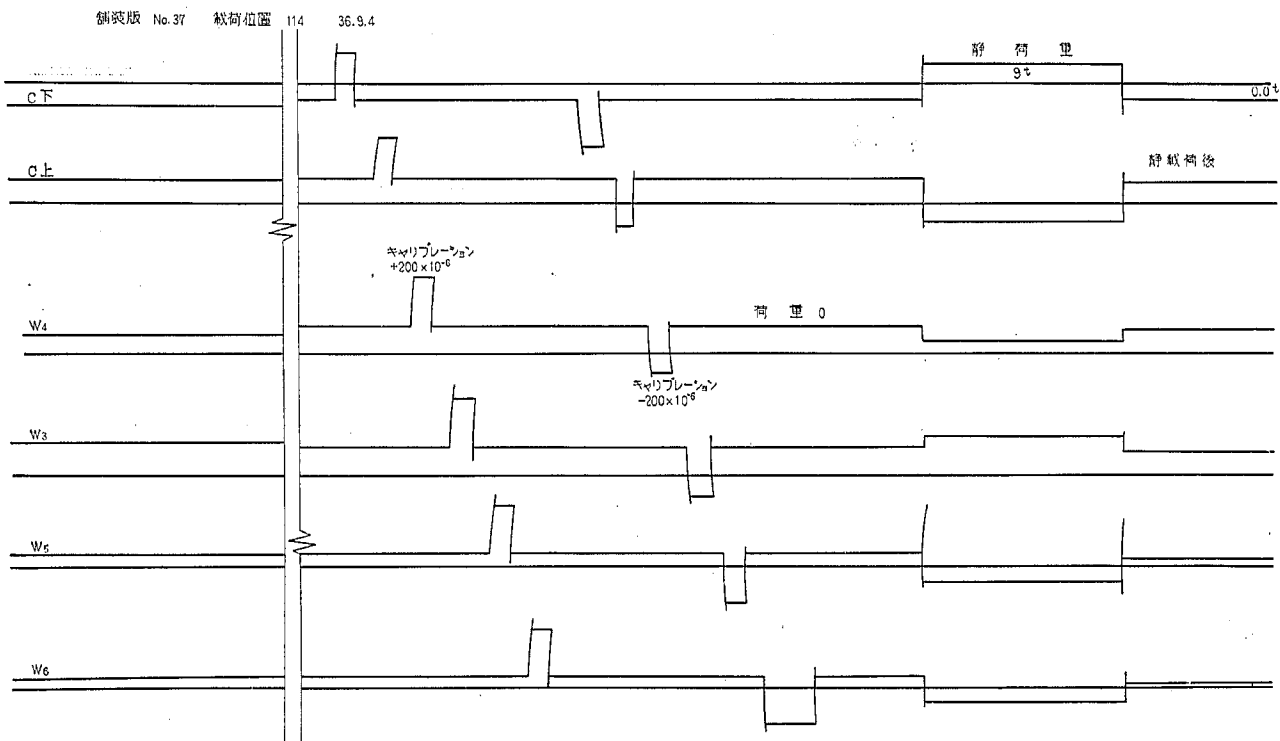
図-35 (1) オッシログラフ記録の 1 例
