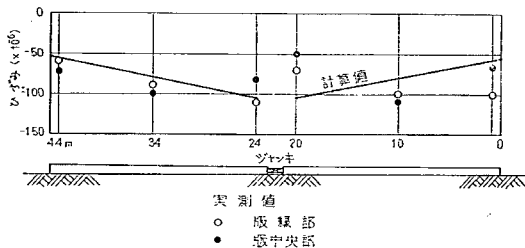
図-14 一次緊張によるひずみ (B版)
