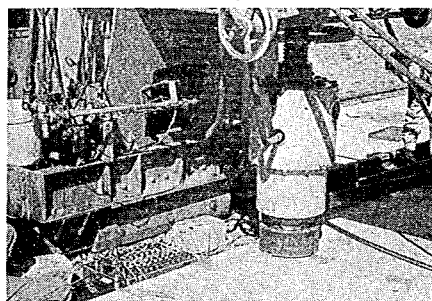
写真-16 30t ジャッキとワイヤストレインゲージによるびずみ測定状況
