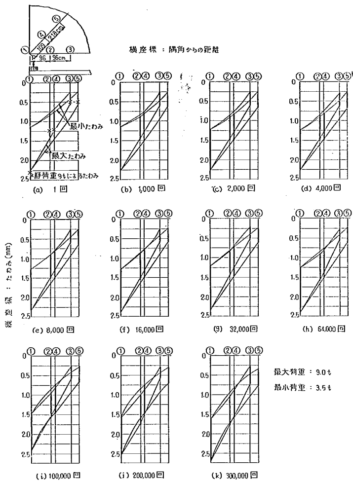
図-134 繰返し荷重による自由隅角部の平均たわみ
