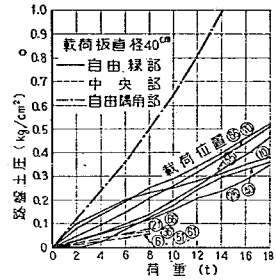
図-44 第2回試験舗装における路盤土圧と荷重の関係 (版厚23.9cm)
