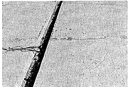
写真-15 舗装版縁部載荷による舗装版表面の ひびわれ
