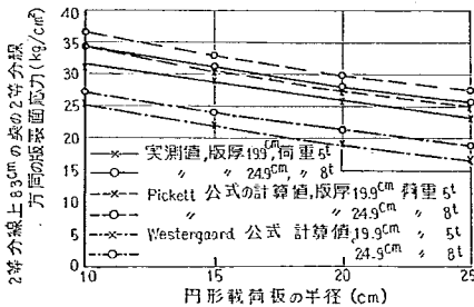
図-96 自由隅角部における載荷板半径と 応力の平均的關係
