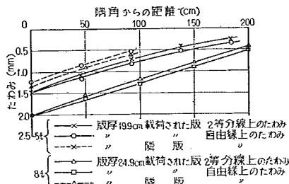
図-55 膨脹目地隅角部における平均たわみ (第1回試験舗装)
