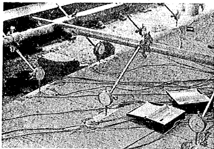
写真-26 鋼製ワグとダイヤルゲージによるたわみの測定状況
