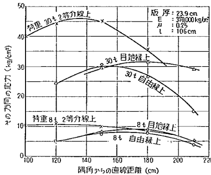
図-77 スリッパを用いためくら目地隅角部における平均応力(第2回試験舗装)
