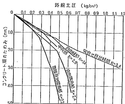
図-50 路盤土圧とコンクリート版たわみの関係 (第1回試験舗装, 版厚25cm)
