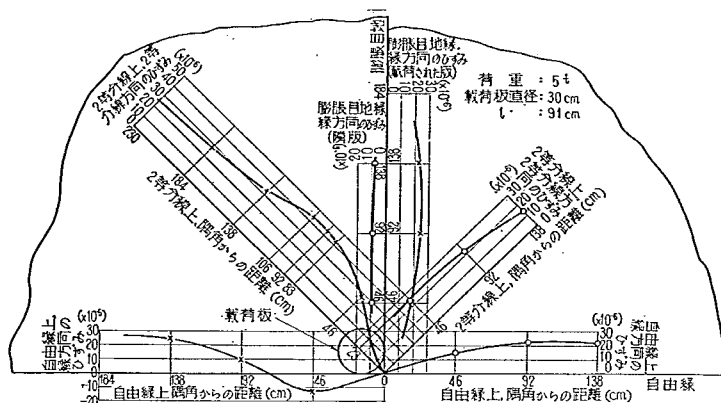
図-71 膨張目地隅角部表面における平均ひずみ (第1回試験舗装, 版厚 20cm)
