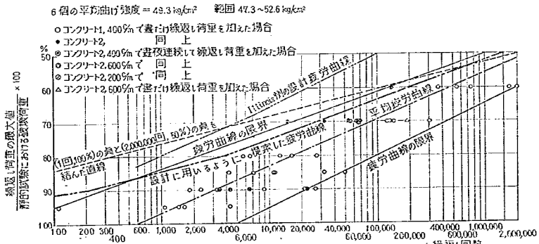
図-132 コンクリートハリ供試体の疲労曲線
