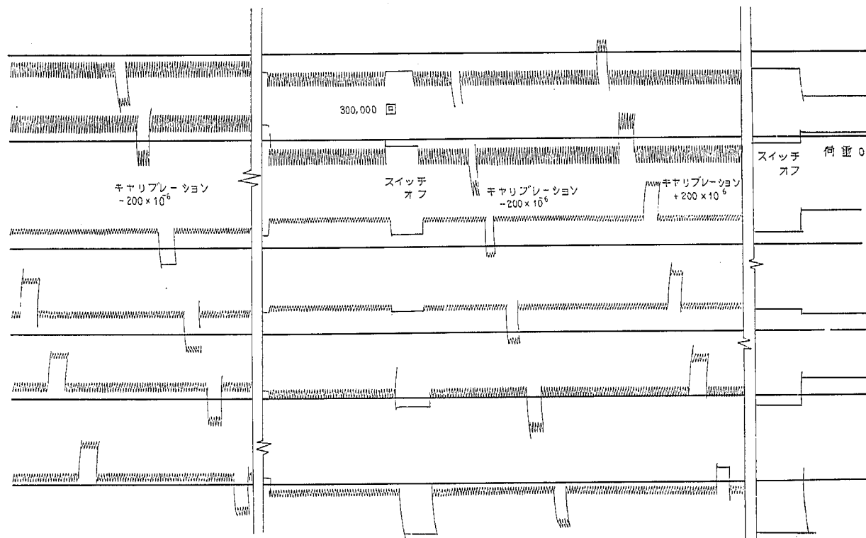
図-53(6) オッシログラフ記録の1例
