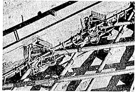
写真-2 A 版縁部構造
