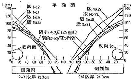
図-116 自由隅角部におけるひびわれのスケッチ (第1回試験舗装)
