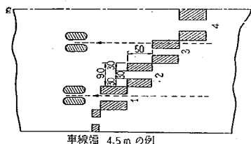
図-38 走行位置調査のためのマーキングの一例
