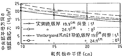
図-101 中央部における載荷板半径と応力の平均的關係
