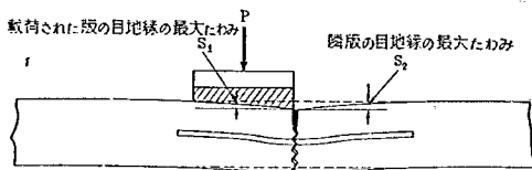
図-64 コンクリート版目地縁部のたわみの説明図
