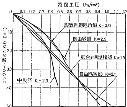
図-48 路盤土圧とコンクリート版たわみの関係 (第1回試験舗装, 版厚20cm)
