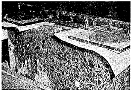
写真-39 切り取りハリ供試体のキャッピング
