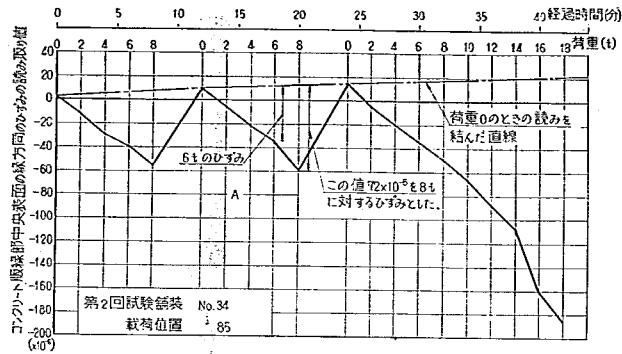
図-33 ワイヤストレインゲージひずみと時間、荷重の関係の一例 (自由縁部)
