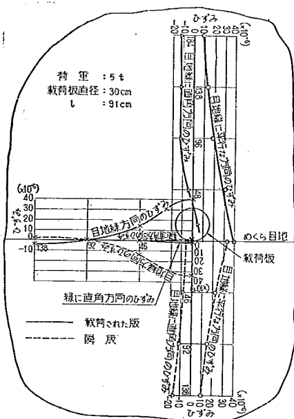
図-88 スリッパを用いためくら目地縁部底面における平均ひずみ (第1回試験舗装, 版厚20cm)
