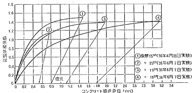
図-8 コンクリートブロック版による路盤摩擦係数と変位の関係
