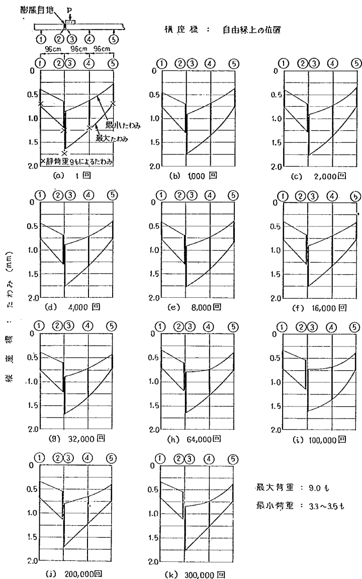
図-135 繰返し荷重による膨脹自地隅角部の平均たわみ
