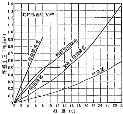
図-41 第1回試験舗装における荷重と路盤土圧の関係 (版厚19.9cm)
