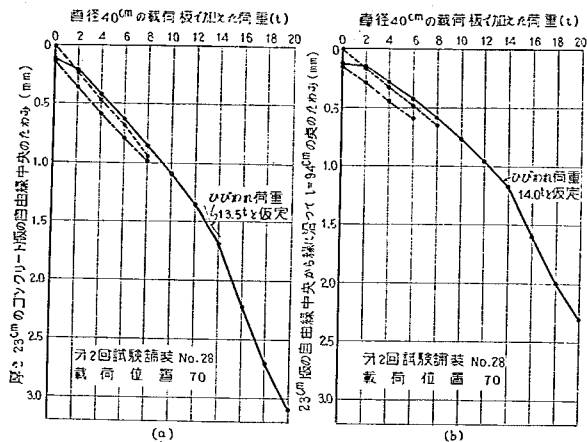
図-17 自由縁部載荷の場合の荷重～たわみ曲線の1例
