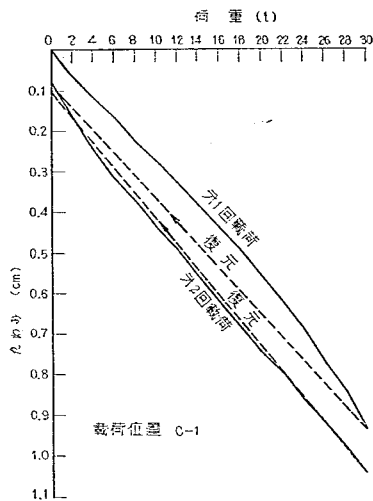
図-32 縁部のたわみ
