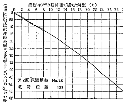
図-52 めくら目地隅角載荷の場合の荷重～沈下曲線の 1 例
