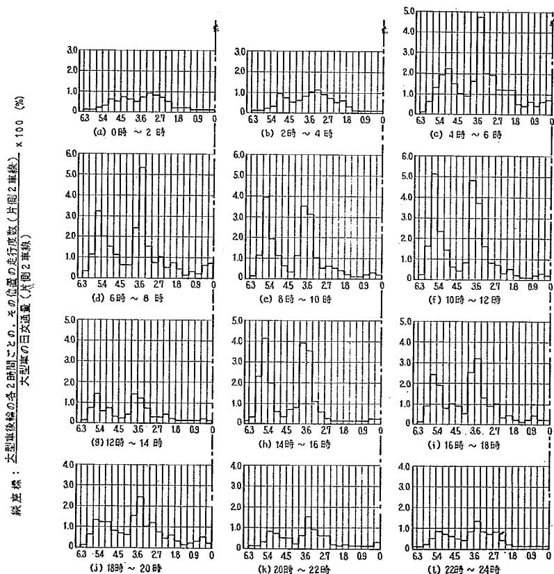
図-157 大型車走行位置分布の24時間内変化 (4車線、1級国道17号 大宮バイパス)
