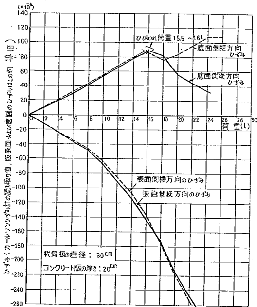
図-22 中央部載荷における荷重～ひずみ関係の1例 (カルソンひずみ計, 第1回試験舗装破壊試験)
