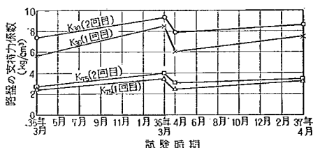
図-39 路盤の支持力係数の経年度化
