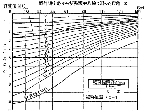
図-30 P C舗装版縁部のたわみ位置曲線
