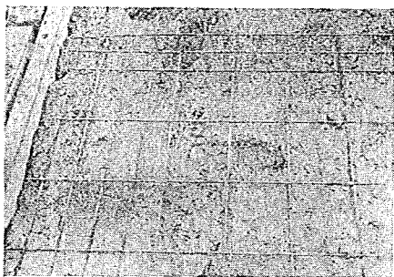
写真-7 鉄網の埋設状況 (第1回試験舗装)
