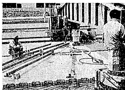
写真-11 静荷重載荷試験 (1 次プレストレス時)
