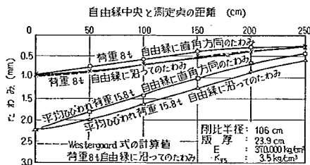
図-62 自由縁部における平均たわみ (第2回試験舗装)
