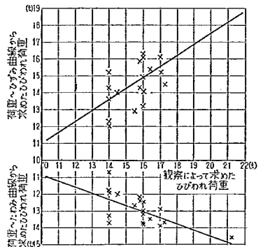
図-124 自由縁部における各種ひびわれ荷重の関係
