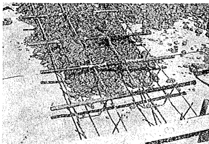
写真-5 めくら目地付近のコンクリート打ち込み
