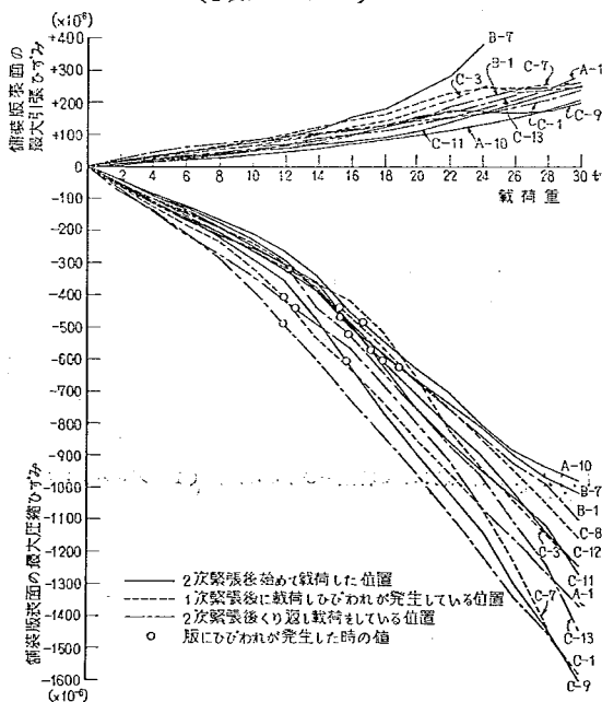
図-25 縁部載荷による荷重—ひずみの関係 (2次プレストレス, 版厚12cm)
