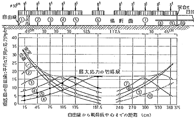
図-114 自動車走行位置 (載荷位置) と応力の平均的關係 (第1回試験舗装, 版厚25cm)
