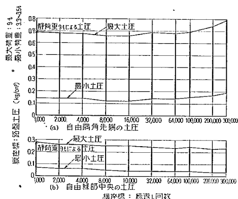
図-133 繰返し荷重試験における路盤土圧と繰返し回数の関係
