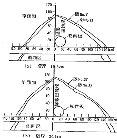
図-118 膨脹目地隅角部におけるひびわれのスケッチ (第1回試験舗装)
