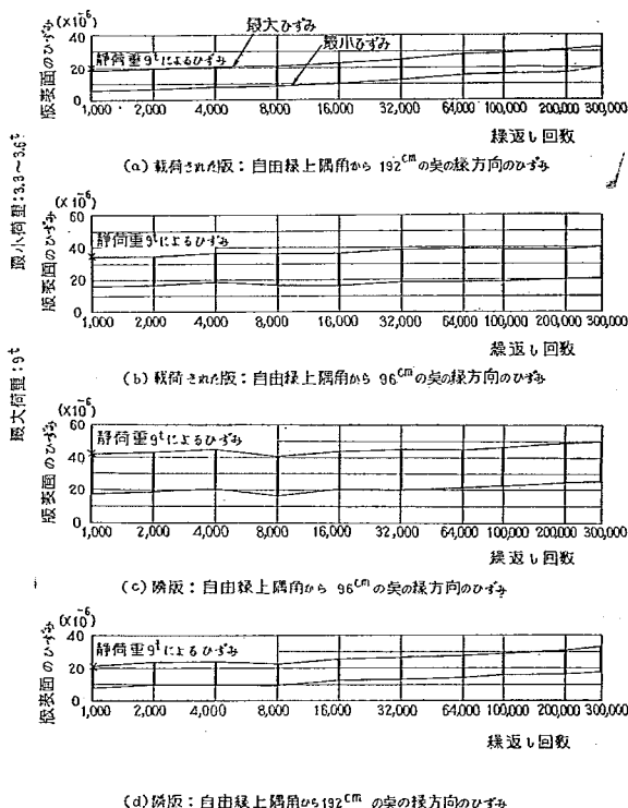
図-143 繰返し載荷試験におけるめくら目地隅角部の平均ひずみと繰返し回数の関係
