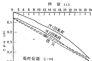
図-33 中央部のたわみ
