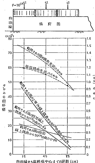
図-102 膨眼目地隅部における載荷位置とたわみおよび版表面ひずみの平均的關係 (第1回試験舗装、版厚20cm)
