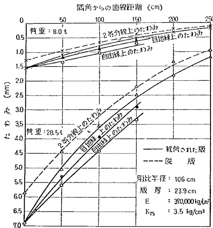
図-56 膨脹目地隅角部における平均たわみ (第2回試験舗装)
