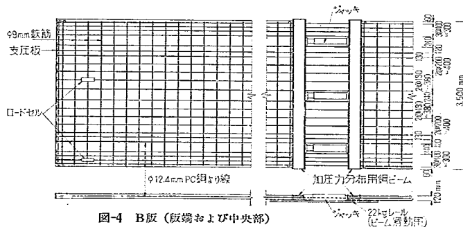
図-4 B版 (版端および中央部)
