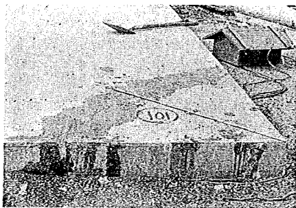
写真-42 コンクリート版自由隅角のひびわれ
