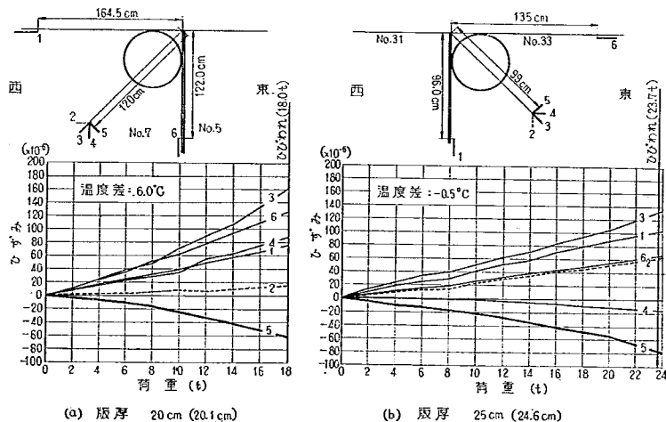
図-119 膨脹目地隅角部における荷重～ひずみ関係の1例
