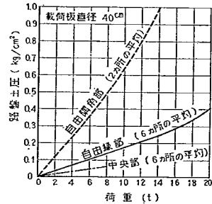
図-45 第2回試験舗装における荷重と平均路盤土圧の関係 (版厚23.9cm)
