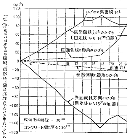
図-19 膨脹目地縁部における荷重～ひずみ関係の1例 (カルソンひずみ計, 第1回試験舗装破壊試験)
