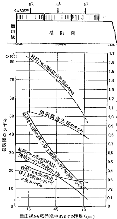
図-103 膨脹目地隅角部における荷役位置とたわみおよび版表面ひずみの平均的關係 (第1回試験舗装, 版厚25cm)
