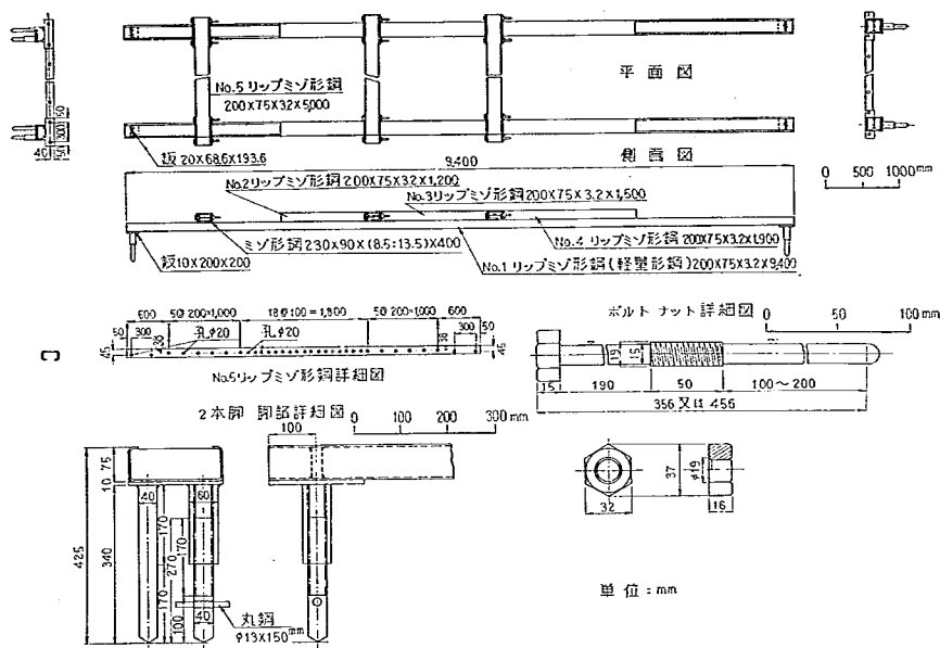
図-25 繰返し載荷試験用ダイヤルゲージ支持枠設計図
