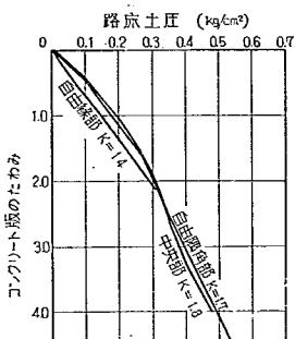
図-47 路床土圧とコンクリート版たわみの関係 (第1回試験舗装, 版厚20cm)
