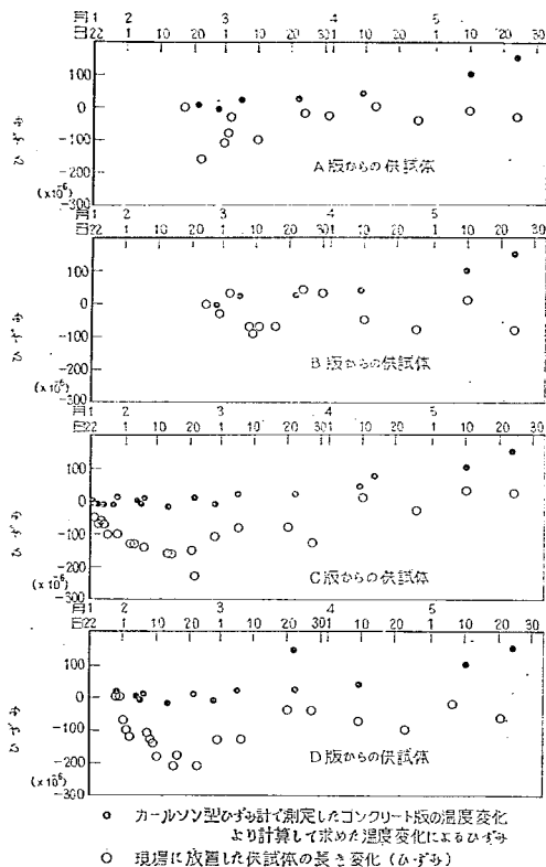
図-13 コンクリート供試体 (10×10×50cm) の長さ変化
