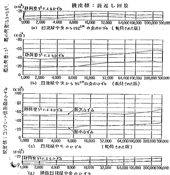
図-145 繰返し載荷試験における縦目地縁部の平均ひずみと繰返し回数の関係
