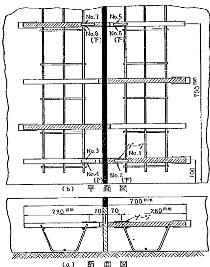
図-37 スリップバーのひずみ測定位置 (膨脹目地) (めくら目地の場合も貼付位置は同じ)
