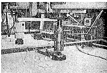
写真-13 くり返し載荷試験
