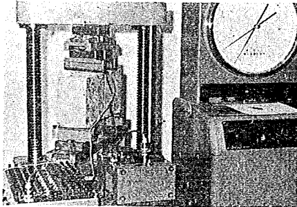
写真-37 ワイヤストレーンゲージによる曲げヤング率の測定
