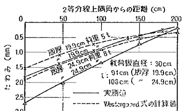
図-53 自由隅角部 2 等分線上の平均たわみ (第 1 回試験舗装)
