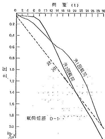
図-34 路盤表面の土圧
