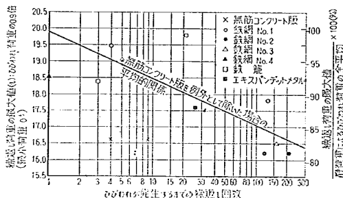
図-151 人力による繰返し載荷試験における、繰返し荷重の最大値とひびわれ発生回数との関係
