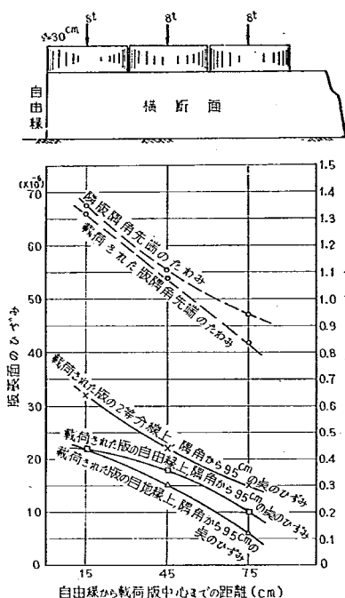
図-105 スリッパのあるめくら目地隅部における荷役位置とたわみおよび版表面ひずみの平均的關係 (第1回試験舗装, 版厚25cm)
