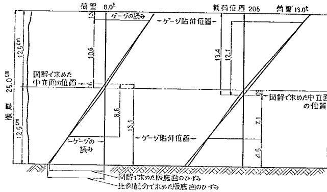
図-85 図解法によるコンクリート版中立面の決定
