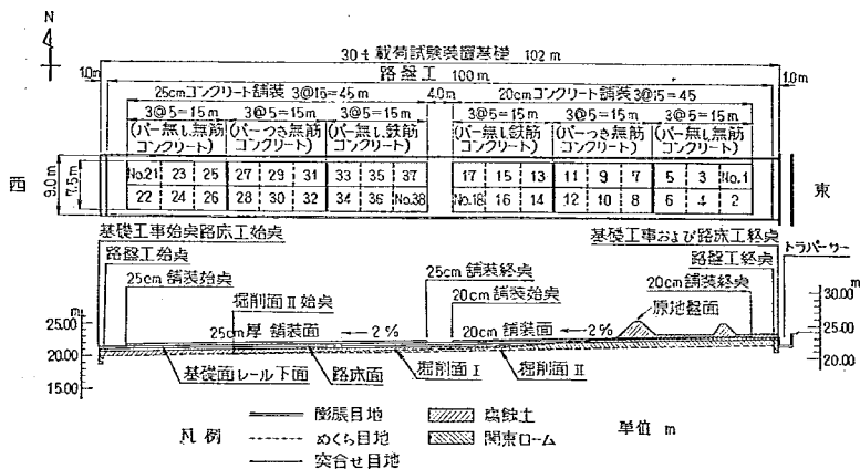
図-1 第1回試験舗装一様図
