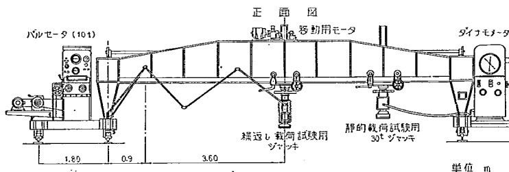
図-13 30t 載荷試験機およびバルセータ
