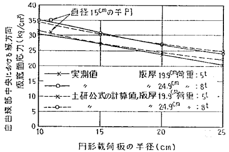
図-97 自由縁部における載荷板形状と 応力の平均的關係
