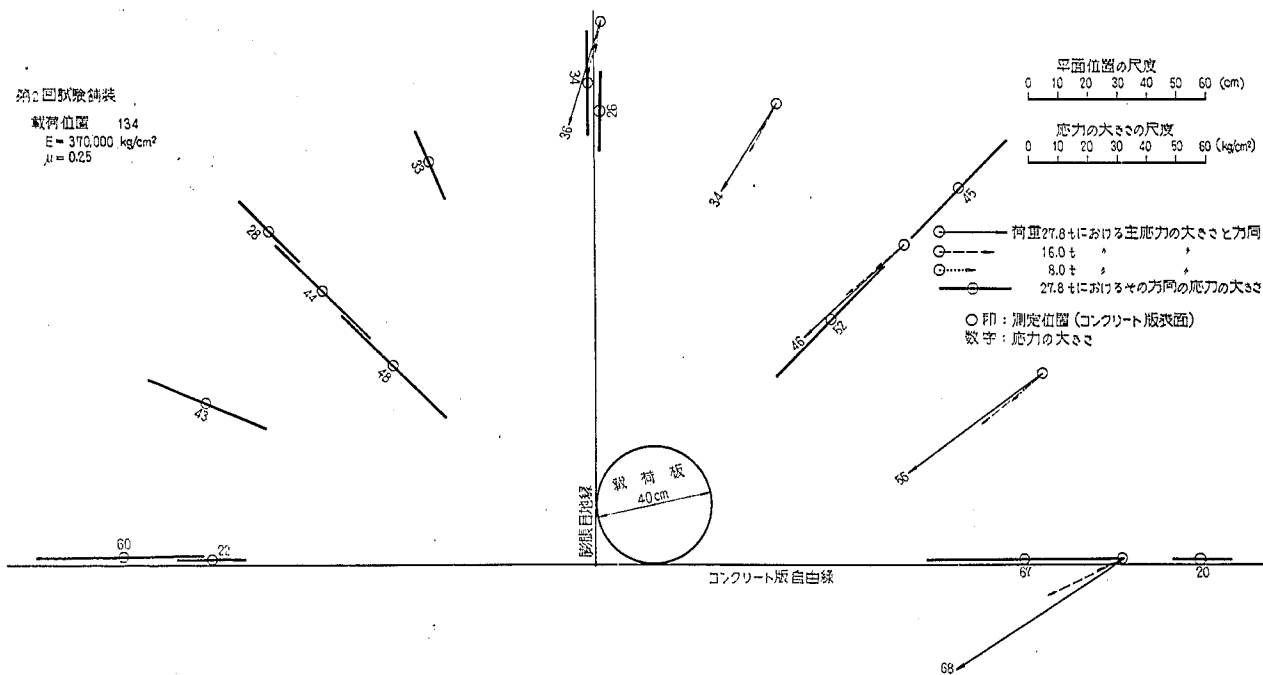
図-74 膨張目地隅角部における主応力の大きさと方向の測定例 (第2回試験舗装)
