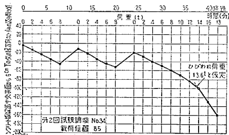
図-18 自由縁部載荷の場合の荷重～ひずみ曲線の1例
