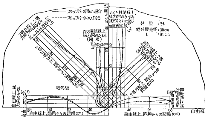
図-75 めくら目地隅角部表面における平均ひずみ（第1回試験舗装、版厚20cm）
