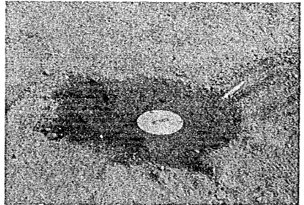
写真-23 土圧計の埋設状況
