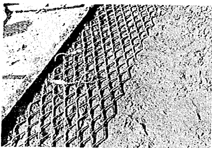
写真-12 第2回試験舗装エキスパンデッドメタル埋設状況
