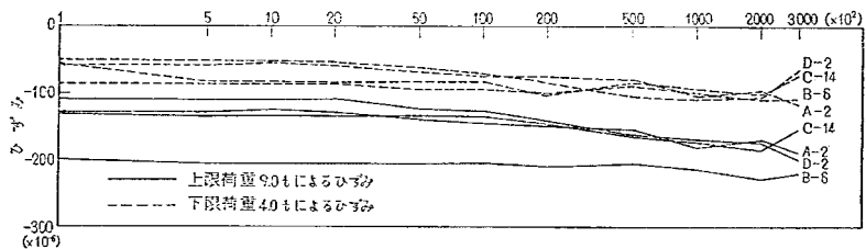
図-39 くり返し载荷回数と舗装版表面のひずみ (舗装版中央部)
