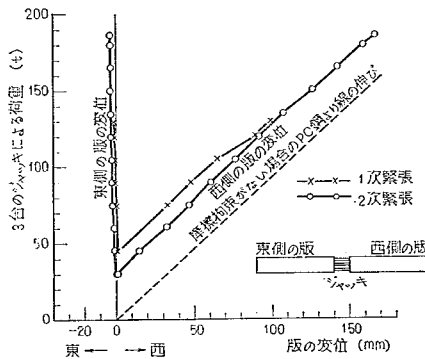
図-9 B版の緊張による変位
