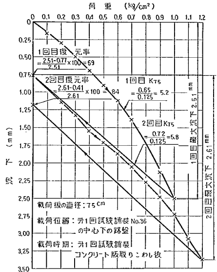
図-10 平板載荷試験結果の1例
