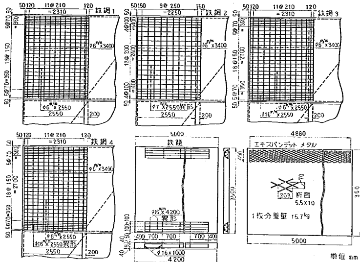
図-8 第2回試験舗装鉄筋類詳細図
