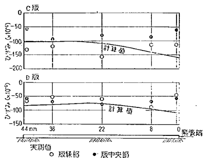
図-16 1次緊張によるひずみ
