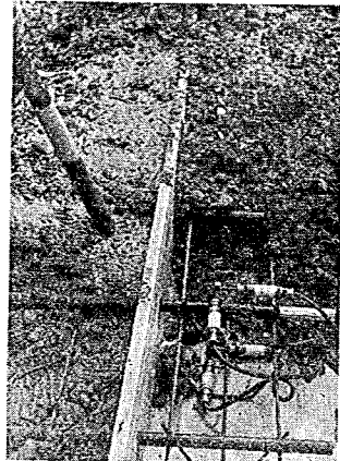
写真-4 膨脹目地付近のコンクリート打ち込み
