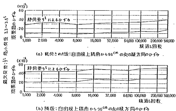
図-142 繰返し載荷試験における膨脹目地隅角部の平均ひずみと繰返し回数の関係
