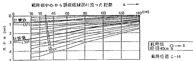
図-31 PC舗装版中央部のたわみ位置曲線
