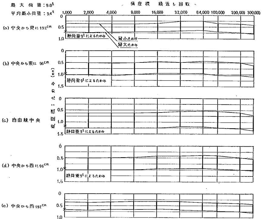
図-138 繰返し荷重による自由縁部の平均たわみと繰返し回数の関係
