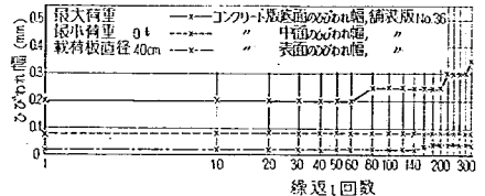
(g) エキスパート・メタルで補強した版
