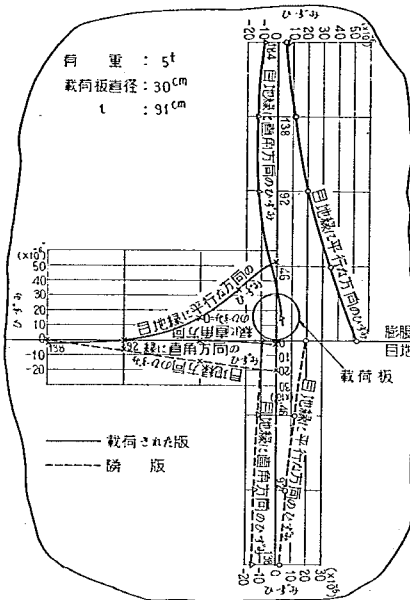
図-86 膨脹目地縁部底面における平均ひずみ (第1回試験舗装, 版厚20cm)
