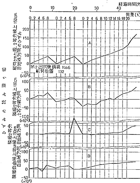
図-34 ワイヤストレインゲージひずみと時間、荷重の関係の一例 (めくら目地隅角部)
