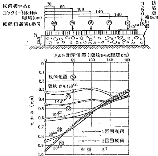
図-107 自由縁部におけるたわみと载荷位置の関係の1例 (第2回試験舗装)
