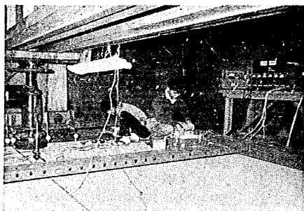
写真-20 夜間繰返し載荷試験状況
