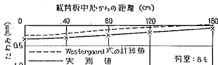
図-65 中央部の平均たわみ (第2回試験舗装)
