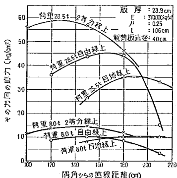
図-73 膨脹目地隅角部における平均応力 (第2回試験舗装)
