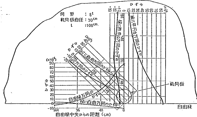
図-80 自由縁部底面における平均ひずみ (第1回試験舗装, 版厚25cm)
