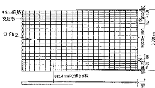
図-5 C版(版端部)
