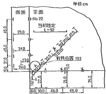
図-28 自由隅角部におけるワイヤストレングージ貼付位置の1例(第1回試験舗装)
