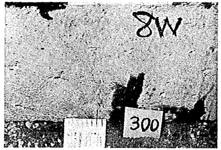
写真-22 シックネスゲージによるひびわれ幅の測定 (繰返し回数300)
