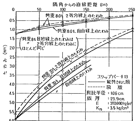
図-58 めくら目地隅角部の平均たわみ (第2回試験舗装)
