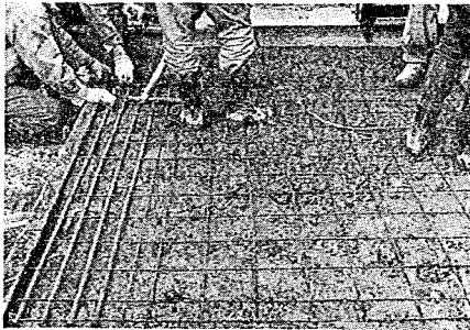
写真-10 第2回試験舗装鉄網 No. 3 埋設状況
