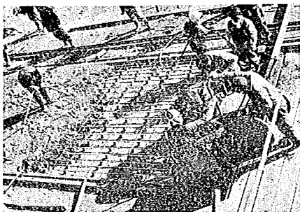
写真-7 コンクリート打設
