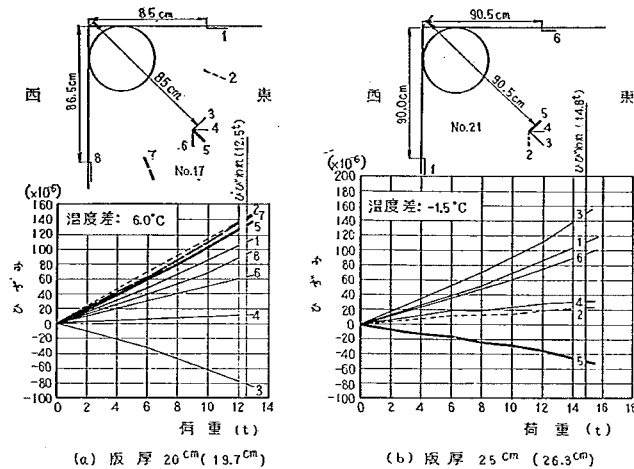
図-117 自由隅角部における荷重～ひずみ関係の1例
