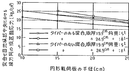
図-100 突合せ目地縁部における載荷板半径と応力の平均的關係
