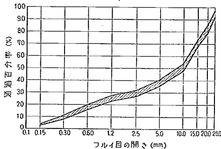
図-3 込切り砂利(路盤材料)の粒度の範囲(実測値)
