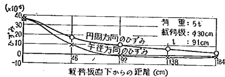
図-93 中央部底面における平均ひずみ (第1回試験舗装、版厚20cm)
