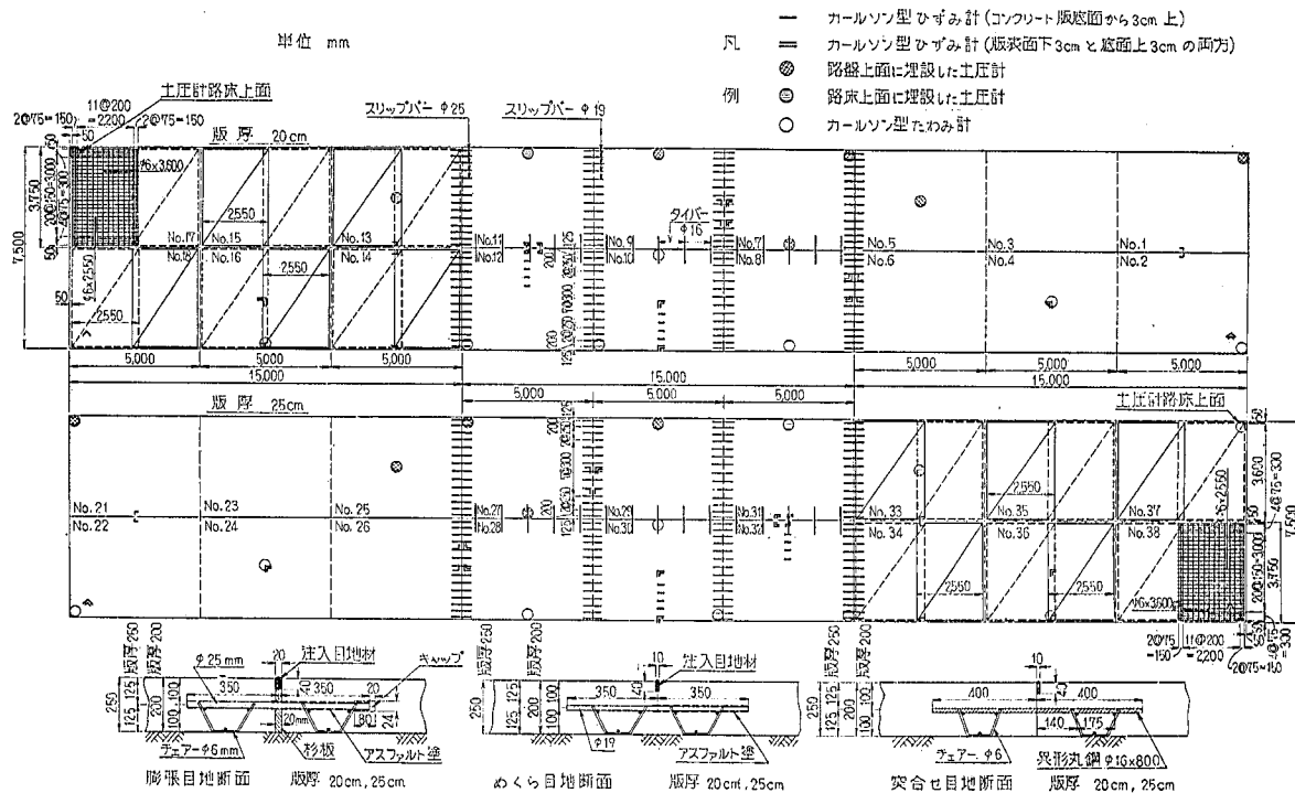
図-4 第1回試験補装詳細および計器埋設位置図
