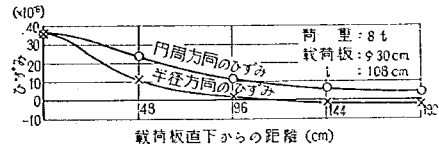
図-94 中央部底面における平均ひずみ (第1回試験舗装、版厚25cm)
