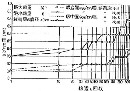
(c) 鉄網 No. 2 (φ7 mm異形丸鋼) で補強した版
