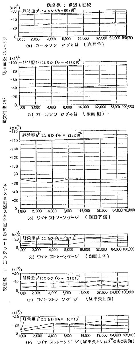
図-150 ひびわれ発生後の繰返し荷重による自由縁部の平均ひずみと繰返し回数の関係
