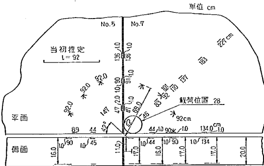
図-29 目地隅角部におけるワイヤストレングージ貼付位置の1例(第1回試験舗装)
