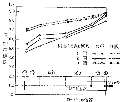
図-11 緊張荷重の伝達
