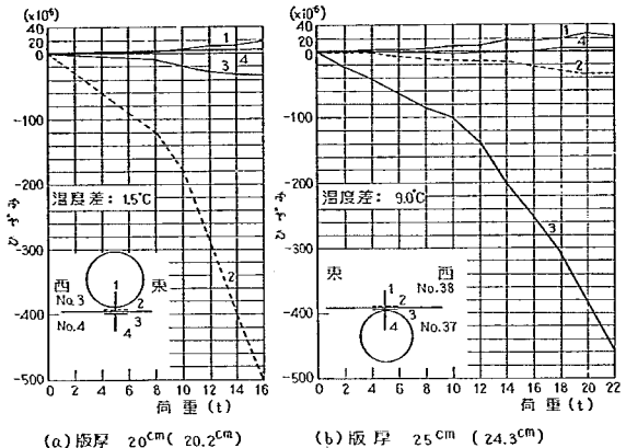
図-130 タイバーのない突合せ目地縁における荷重～ひずみ関係の一例
