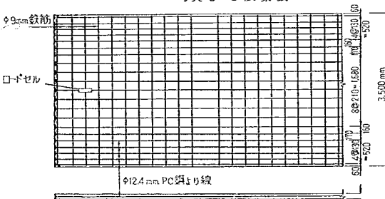
図-6 D版(版端部)
