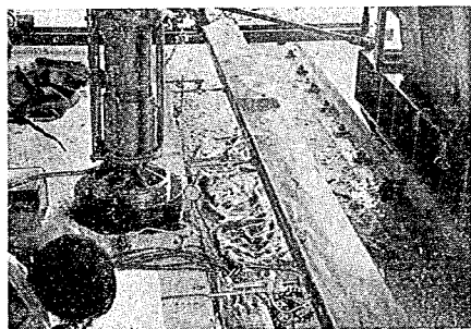
写真-29 繰返し載荷試験におけるたわみの測定状況
