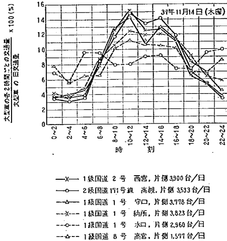
図-160 大型車交通量の日変化 (日本道路公団高速道路試験所“名神間交通量調査報告書”より複製)
