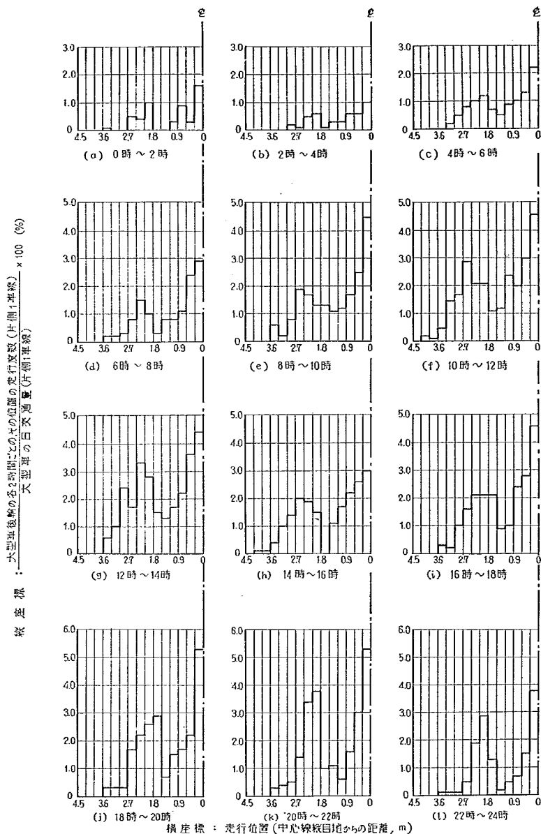
図-156 大型車走行位置分布の24時間内変化(2車線, 1級国道4号 春日部)
