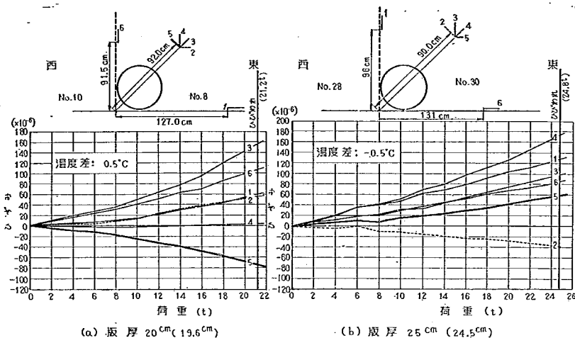
図-121 スリッパのあるめくら目地隅角部の荷重～ひずみ関係の1例
