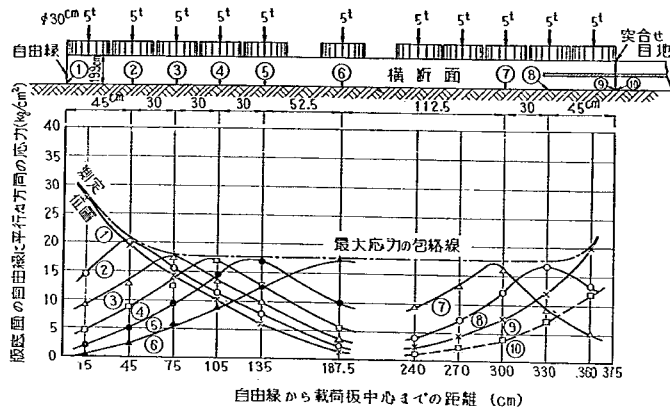
図-113 自動車走行位置 (載荷位置) と応力の平均的關係 (第1回試験舗装, 版厚20cm)
