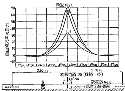
図-83 自由縁部における応力の測定例 (第2回試験舗装)
