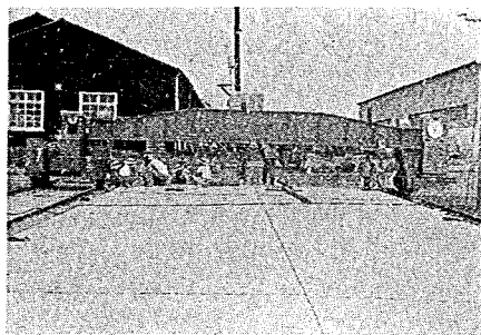
写真-15 30t 載荷試験装置の全景(右側のジャッキは静的載荷試験用で能力30tのもの、中央のジャッキは動的載荷試験用で能力10tのもの)
