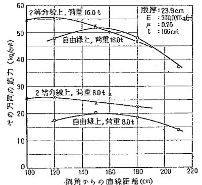
図-69 自由隅角における平均応力 (第2回試験舗装)
