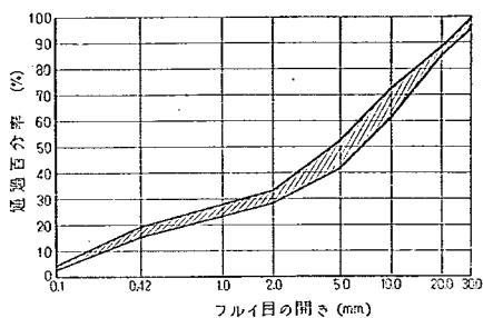
図-5 クラッシャーランの粒度の範囲 (実測値)
