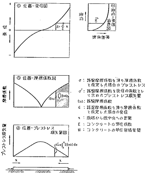
図-12 路盤摩擦拘束によるプレストレス損失量の図解
