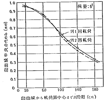
自由縁部におけるたわみと 载荷位置の平均的關係
