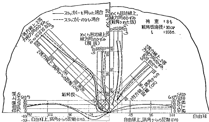
図-76 めくら目地隅角部表面における平均ひずみ（第1回試験舗装、版厚25cm）
