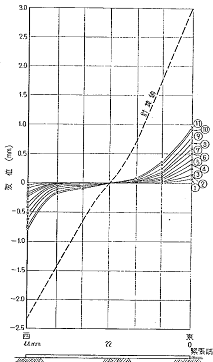
図-17 1次緊張による変位 (C版)
