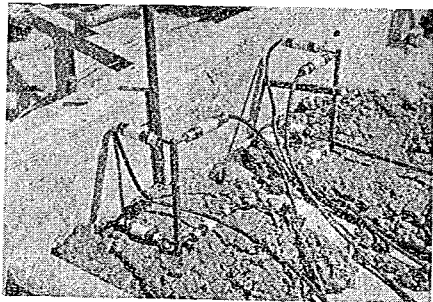
写真-6 縦突合せ目地付近のコンクリート打ち込みおよびカーソンひずみ計の埋設状況
