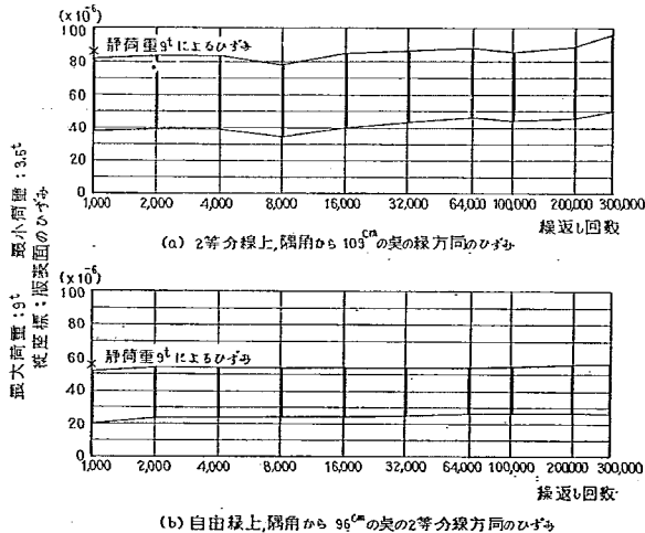
図-141 繰返し載荷試験における自由隅角部の平均ひずみと繰返し回数
