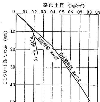
図-49 路床土圧とコンクリート版たわみの関係 (第1回試験舗装, 版厚25cm)
