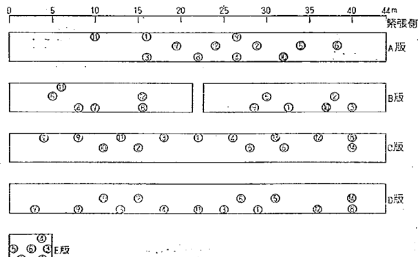
図-20 載荷位置
