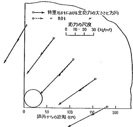
図-70 自由隅角部における主応力の大きさと方向の測定例
