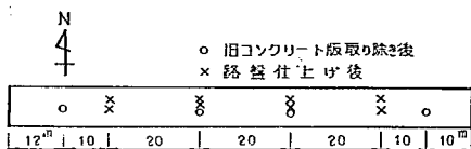
図-11 第2回試験舗装前における平板載荷試験位置図(路盤面)
