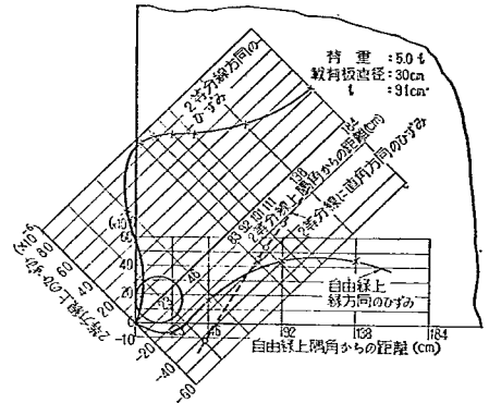
図-67 自由隅角部表面における平均ひずみ (第1回試験舗装, 版厚20cm)
