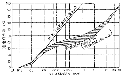
図-2 敷砂および路盤材料の粒度
