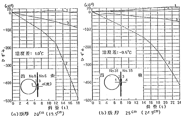
図-126 膨脹目地縁部における荷重～ひずみ関係の1例
