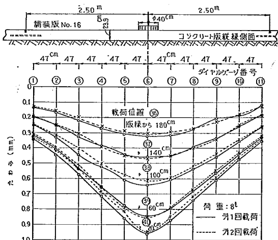
図-106 自由縁部におけるたわみと荷役位置の關係の測定例 (第2回試験舗装)
