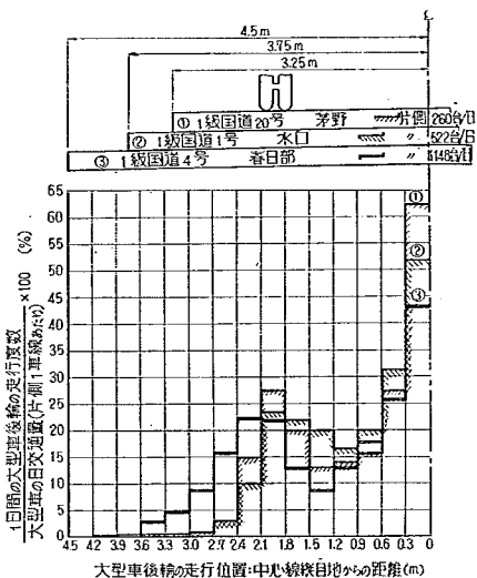
図-154 2車線コンクリート舗装における大型車走行位置の観測例
