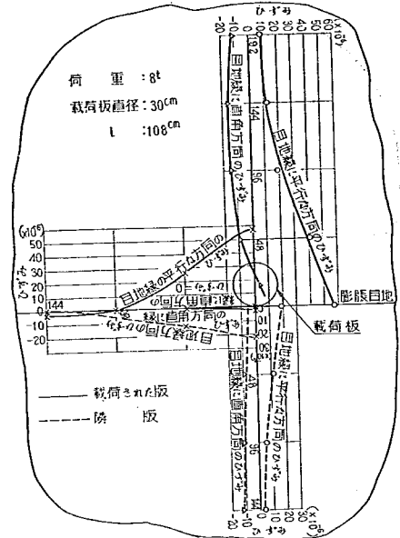
図-87 膨脹目地縁部底面における平均ひずみ (第1回試験舗装, 版厚25cm)
