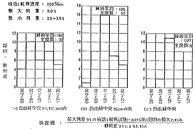
図-140 繰返し載荷試験におけるたわみと静的載荷試験におけるたわみの比較
