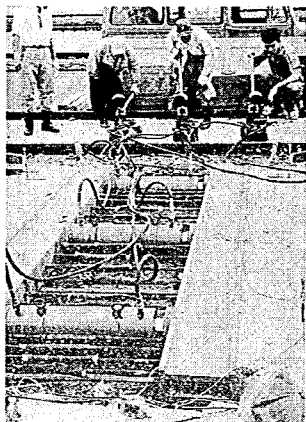
写真-4 B版緊張
