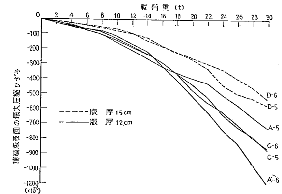
図-22 中央部荷重による荷重-ひずみの関係 (1次プレストレス)
