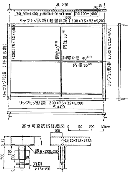
図-23 静的載荷試験用ダイヤルゲージ支持枠
