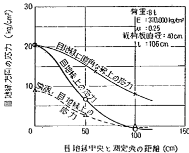
図-92 タイバーつき突合せ目地縁部における平均応力 (第2回試験舗装)
