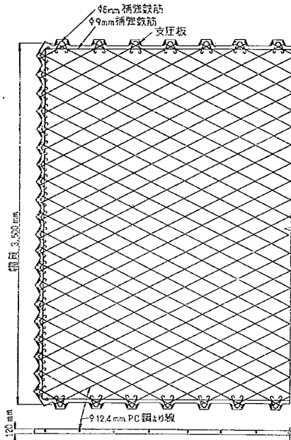
図-3 A版 (版端部)
