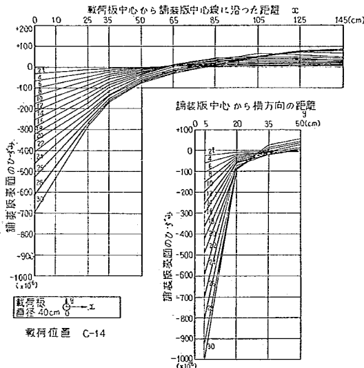
図-28 PC舗装版中央部のひずみ—位置曲線
