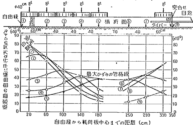
図-112 自由縁部、中央部および突合せ目地縁部における載荷位置とひずみの平均的関係 (第2回試験舗装, 平均値)
