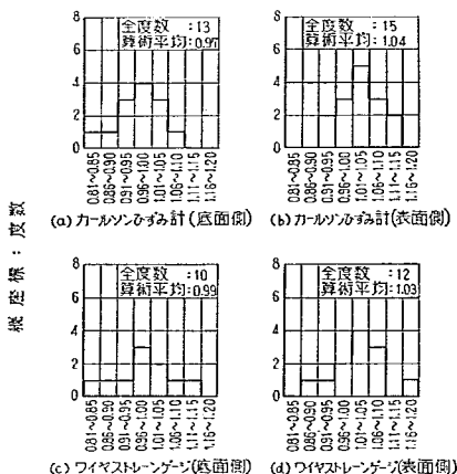
図-146 繰返し載荷試験におけるひずみと静的載荷試験におけるひずみの比較
