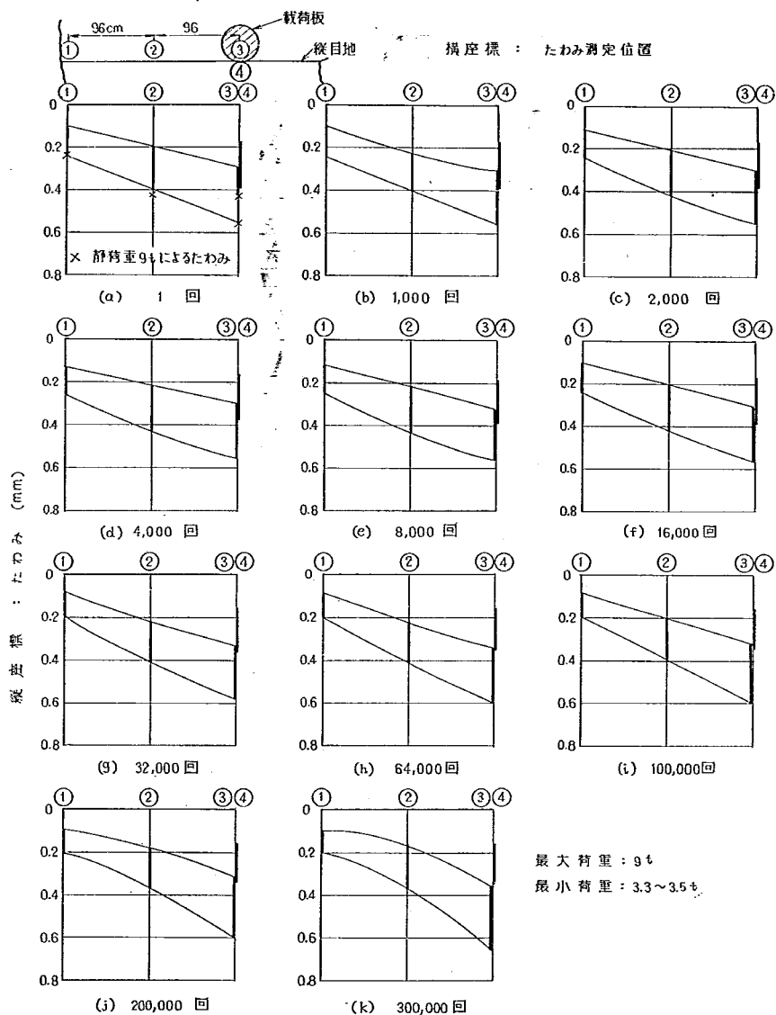
図-139 繰返し載荷試験における縦目地縁部(タイバーつき)の平均たわみ
