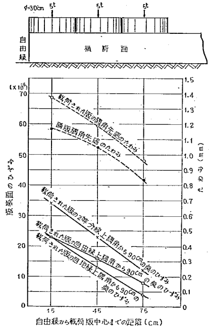
図-104 スリップバーのあるめくら目地隅角部における荷役位置とたわみおよび版表面ひずみの平均的關係 (第1回試験舗装, 版厚20cm)
