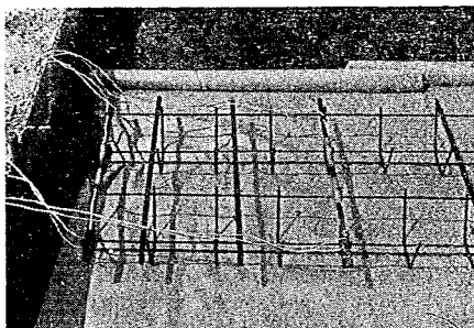
写真-35 ワイヤストレインゲージによるスリップバーひずみの測定 (めくら目地)
