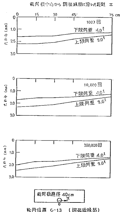
図-40 くり返し載荷によるたわみ一位置図
