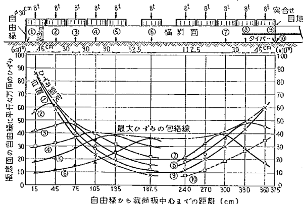
図-111 自由縁部、中央部および突合せ目地縁部における載荷位置と板底面ひずみの平均的関係 (第1回試験舗装, 版厚25cm)
