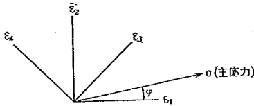
図-66 ひずみ測定用の45°ローゼットから主応力の計算
