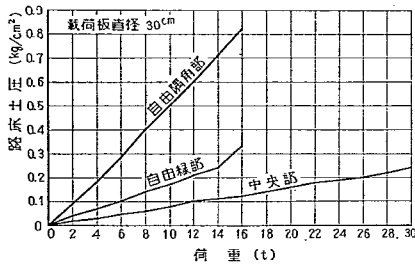
図-42 第1回試験舗装における荷重と路床土圧の関係 (版厚24.9cm)
