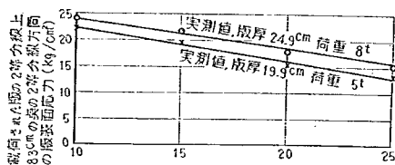
図-98 膨眼目地縁部における載荷板半径と応力の平均的關係
