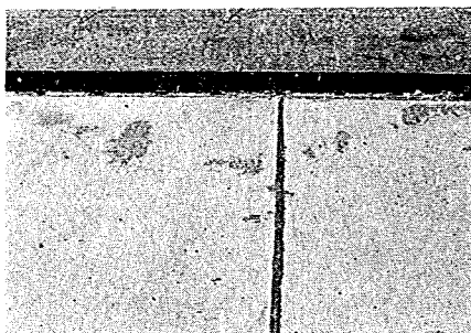
写真-44 コンクリート版膨脹目地隅角のひびわれ
