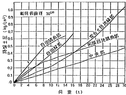
図-43 第1回試験舗装における荷重と路盤土圧の関係 (版厚24.9cm)
