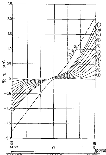
図-18 1次緊張による変位 (D版)
