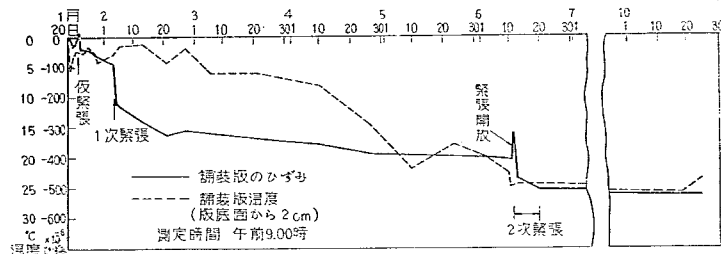
図-19 カーソン型ひずみ計による長期観測
