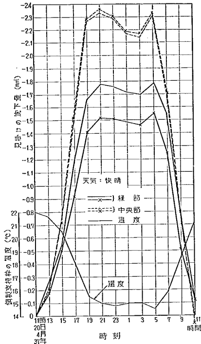
図-26 鋼製支持棒とダイヤルゲージによる見掛け上のたわみの測定例(快晴の場合)
