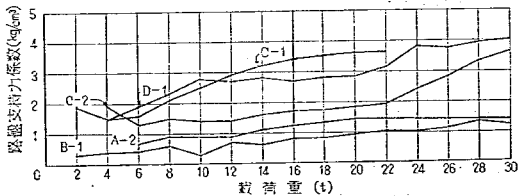
図-35 土圧計による路盤支持力係数
