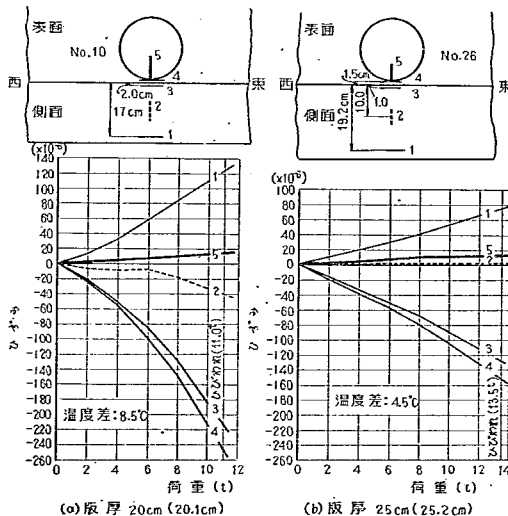
図-123 自由縁部における荷重~ひずみ関係の1例
