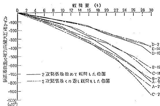
図-24 中央部載荷による荷重—ひずみの関係 (2次プレストレス)
