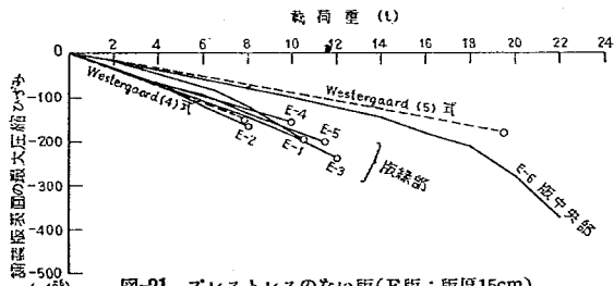
図-21 プレストレスのない版 (E 版 : 版厚 15cm) の荷重—ひずみの関係
