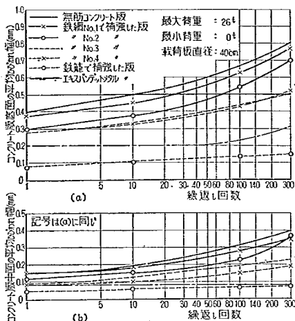
図-153 26t繰返し荷重による自由縁部ひびわれ発達の平均的関係
