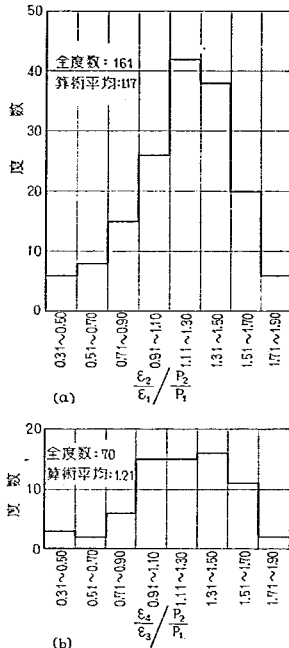
図-36 繰返し載荷試験における最大、最小ひずみの比と最大、最小荷重の比の関係
