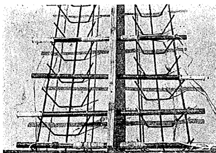
写真-34 ワイヤストレインゲージによるスリップバーひずみの測定 (膨脹目地)
