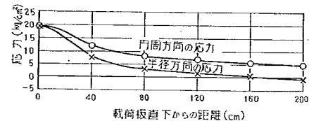
図-95 中央部底面における平均応力 (第2回試験舗装)
