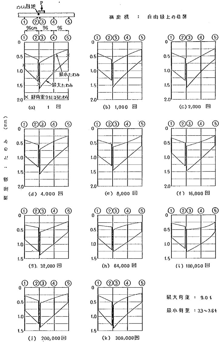
図-136 繰返し荷重によるめくら目地隅角部の平均たわみ
