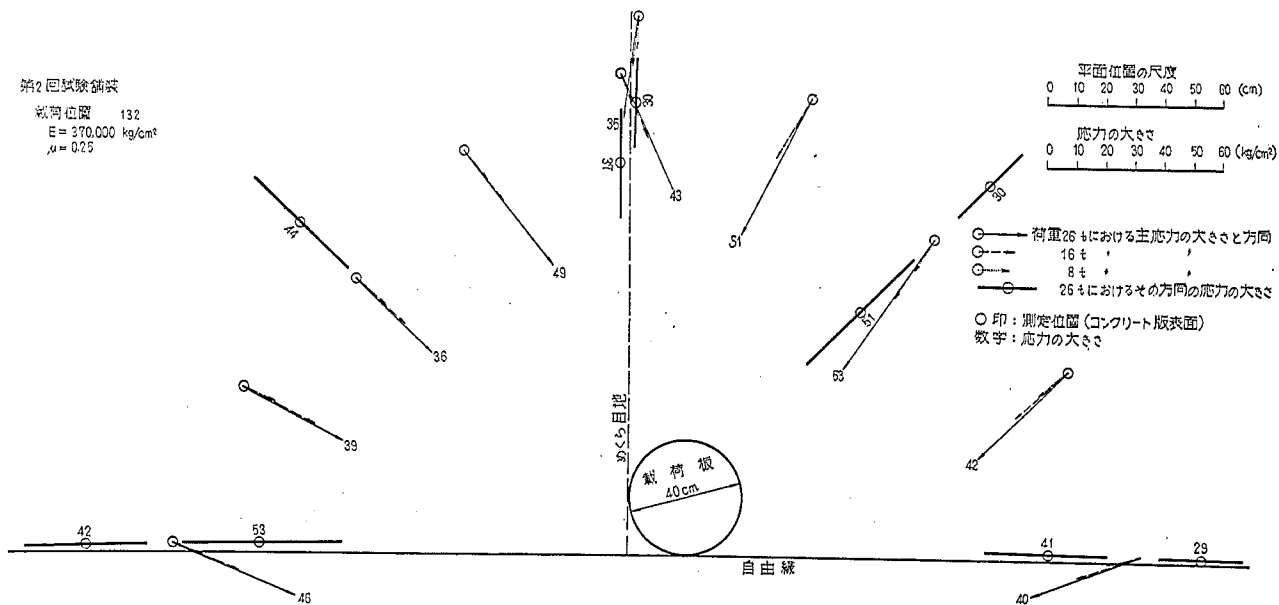
図-78 めくら目地隅部における主応力の大きさと方向の測定例（第2回試験鋪装）
