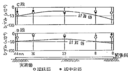
図-15 単緊張によるひずみ
