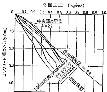
図-51 路盤土圧とコンクリート版たわみの関係 (第2回試験舗装)
