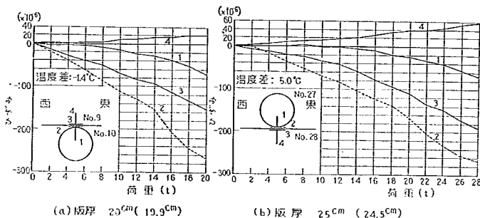
図-129 タイバーのある突合せ目地における荷重~ひずみ関係の1例
