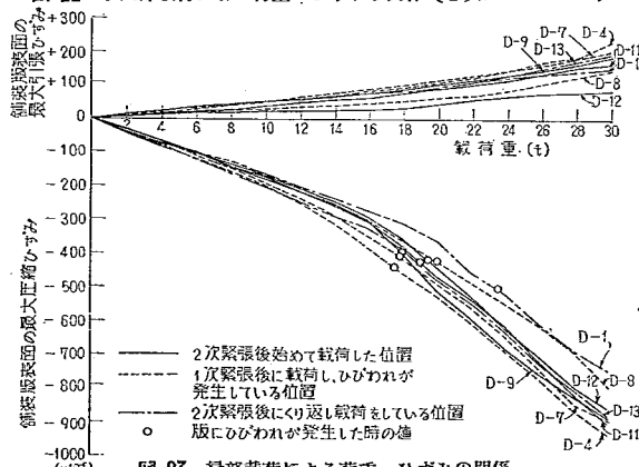
図-23 縁部荷重による荷重-ひずみの関係 (2次プレストレス, 版厚15cm)
