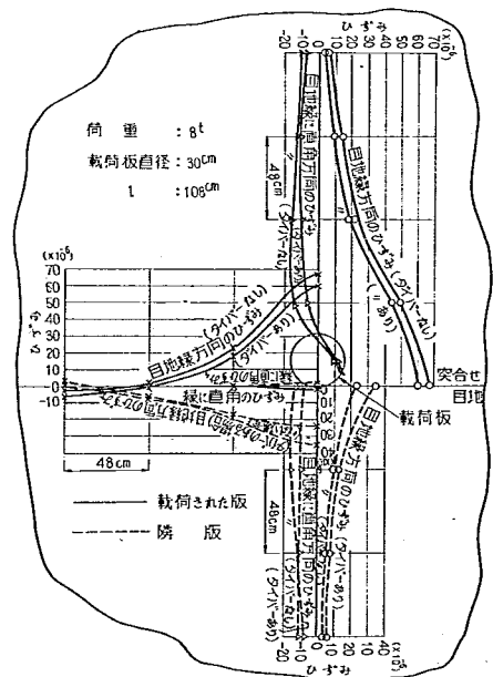
図-91 突合せ目地縁部底面における平均ひずみ (第1回試験舗装, 版厚25cm)
