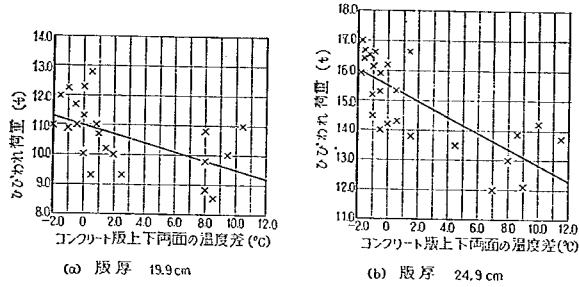
図-125 コンクリート版上下両面の温度差とひびわれ荷重の関係
