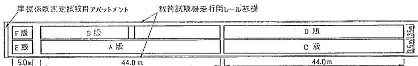
図-1 P C試験舗装一般図
