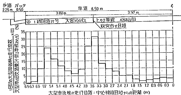
図-155 4車線コンクリート舗装における大型車走行位置の観測例
