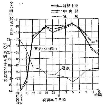
図-27 鋼製支持棒とダイヤルゲージによる見掛け上のたわみの測定例(曇後雨の場合)
