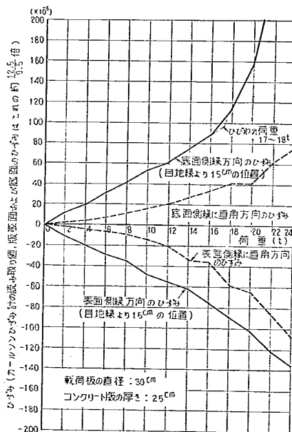
図-20 スリップバーのあるめくら目地縁部における荷重～ひずみ関係の1例 (カルソンひずみ計, 第1回試験舗装破壊試験)
