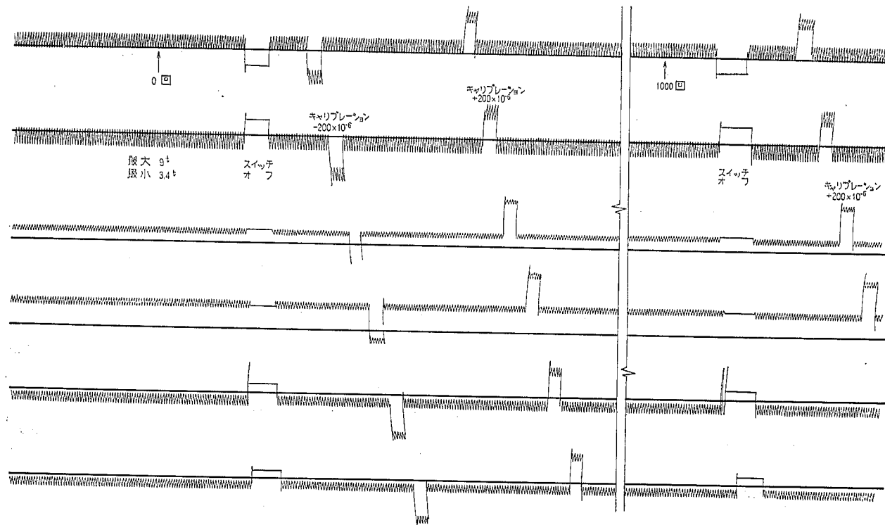
図-35 (3) オッシログラフ記録の 1 例
