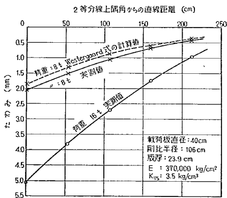
図-54 自由隅角部の平均たわみ (第 2 回試験舗装)
