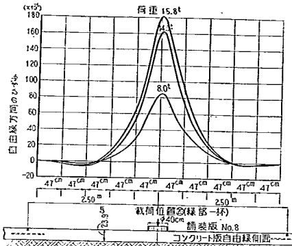
図-81 自由縁部におけるひずみの測定例 (第2回試験舗装)
