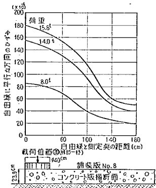
図-82 自由縁部におけるひずみの測定例 (第2回試験舗装)
