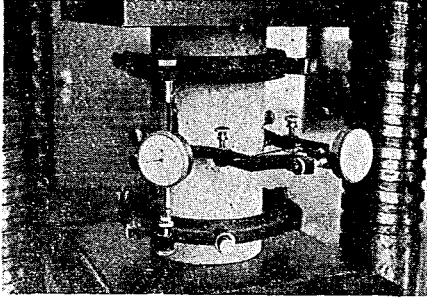
写真-36 コンプレッソメータおよびエキステンソメータによる圧縮ヤング率およびポアソン比の測定
