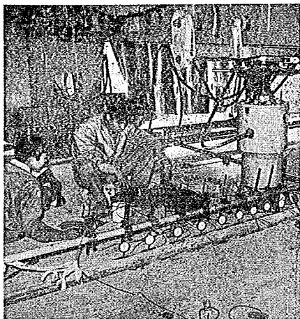
写真-12 静荷重載荷試験(2次プレストレス時)
