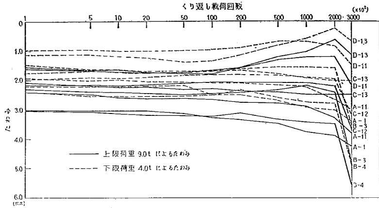
図-36 くり返し载荷回数とたわみ (舗装版露部)
