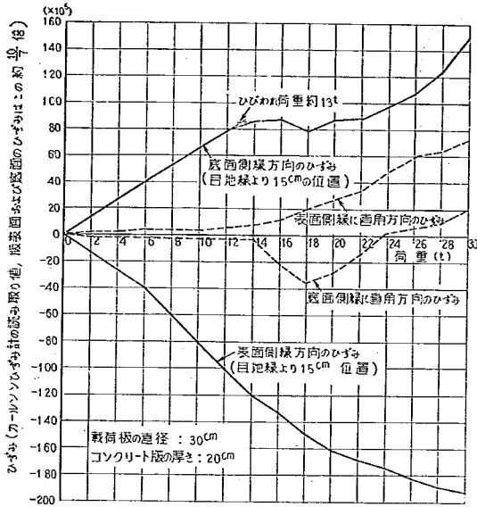
図-21 タイバーのある突合せ目地線部における荷重～ひずみ関係の1例 (カルソンひずみ計, 第1回試験舗装破壊試験)
