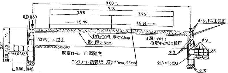
図-2 第1回試験舗装標準断面図ならびにレール基礎断面図
