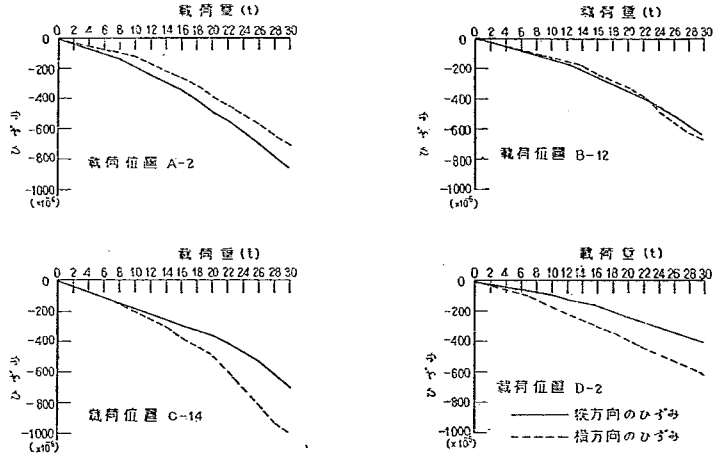
図-29 中央部荷重による舗装版表面のひずみ
