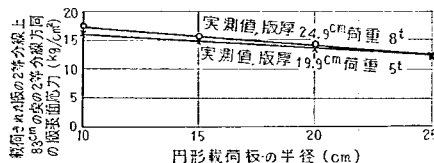
図-99 スリッパを用いたため目地縁部における載荷板半径と応力の平均的關係
