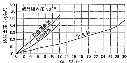
図-40 第1回試験舗装における荷重と路床土圧の関係 (版厚19.9cm)
