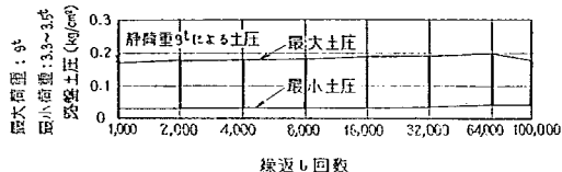
図-147 ひびわれ発生後の繰返し載荷試験における自由縁部中央の路盤土圧と繰返し回数との関係
