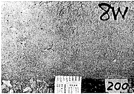
写真-21 シックネスゲージによるひびわれ幅の測定 (繰返し回数200)
