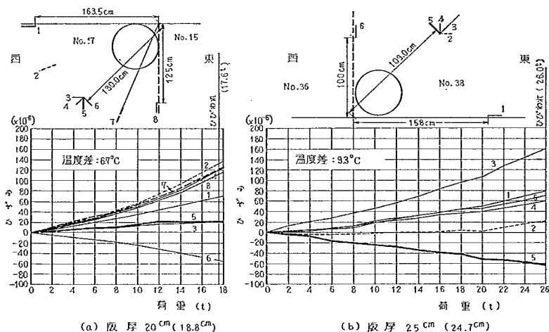
図-122 スリッパのないめくら目地隅角部における荷重～ひずみ関係の1例
