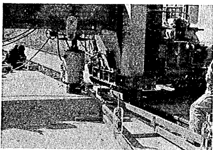
写真-25 ベンケルマンビームによるたわみの測定状況
