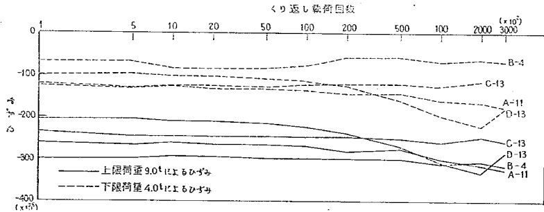
図-38 くり返し载荷回数と舗装版表面のひずみ (舗装版露部)
