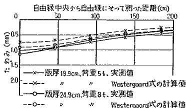
図-61 自由縁部上の平均たわみ (第1回試験舗装)
