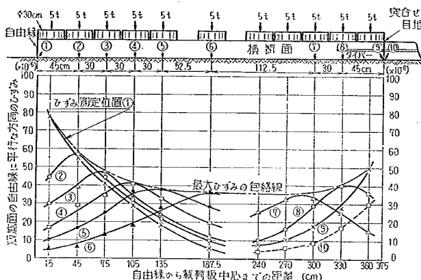
図-110 自由縁部、中央部および突合せ目地縁部における載荷位置と板底面ひずみの平均的関係 (第1回試験舗装, 版厚20cm)
