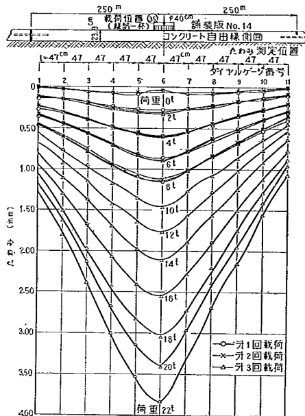
図-59 自由縁部におけるたわみの測定例 (第2回試験舗装)
