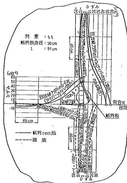
図-90 突合せ目地縁部底面における平均ひずみ (第1回試験舗装, 版厚20cm)
