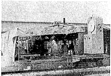
写真-18 テントを張った載荷試験の状況
