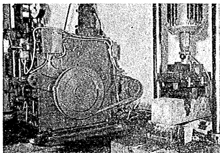
写真-40 アムスラー型パルセータによる曲げ疲労試験
