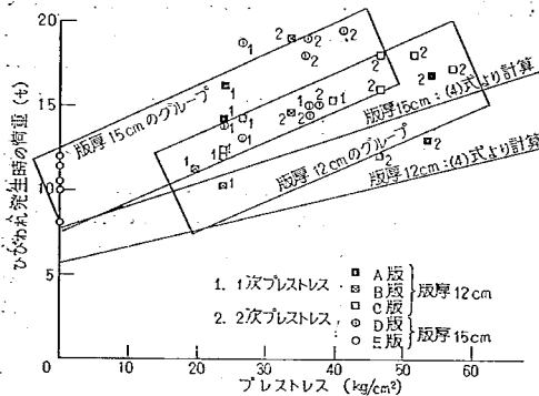
図-26 プレストレスと縁部におけるひびわれ発生時の荷重 ス量だけ増加するとして求めた。計算に用いた諸数値は 表-19 の値を用いた。
