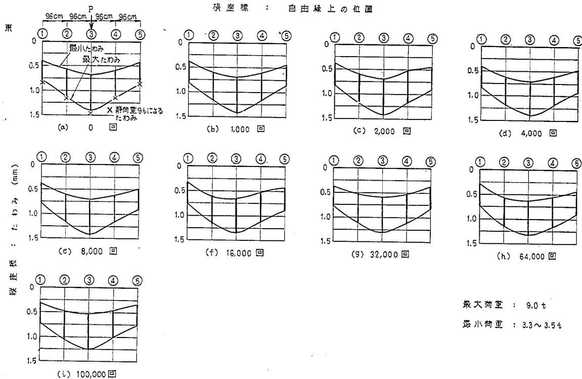
図-148 ひびわれ発生後の繰返し荷重による自由縁部の平均たわみ
