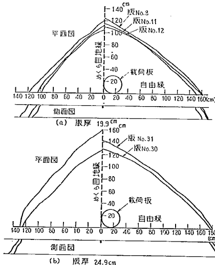
図-120 スリッパーを用いた、めくら目地隅角部におけるひびわれのスケッチ (第1回試験舗装)
