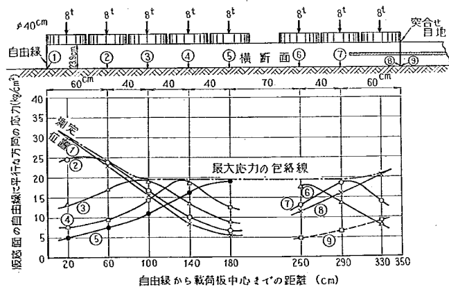
図-115 自動車走行位置 (載荷位置) と応力の平均的關係 (第2回試験舗装, 平均値)
