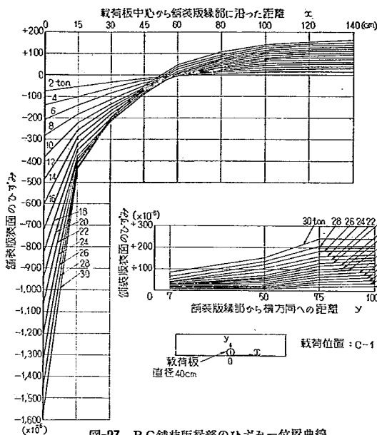
図-27 PC舗装版縁部のひずみ—位置曲線
