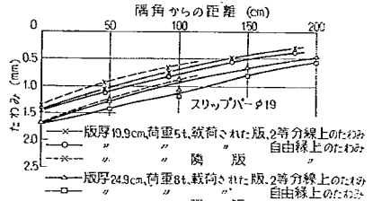
図-57 スリッバーを用いためくら目地隅角部における平均たわみ(第1回試験舗装)
