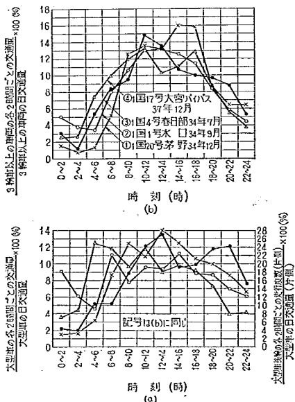
図-159 交通量の時間変化の観測例
