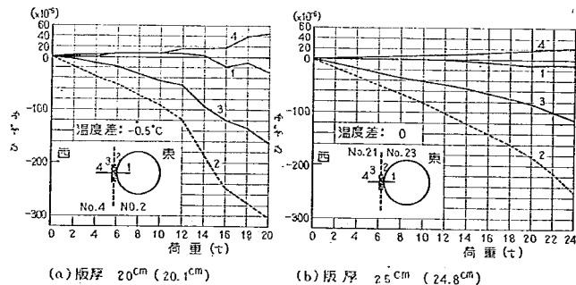
図-128 スリッパのないめくら目地における荷重~ひずみ関係の1例
