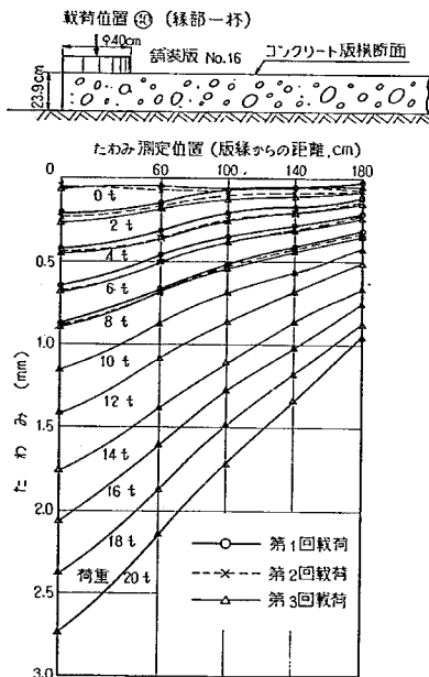
図-60 自由縁部におけるたわみの測定例 (第2回試験舗装)
