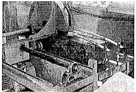
写真-38 ダイヤモンドソーによる切り取りハリ供試体の作成
