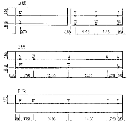
図-10 ロードセル位置図 (単位m)
