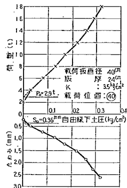
図-46 コンクリート版と路盤が離れていた場合の路盤土圧と荷重および沈下の関係の1例
