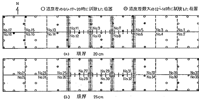
図-16 第1回試験舗装破壊試験位置図 (載荷板直径30cm)
