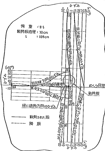
図-89 スリッパを用いためくら目地縁部底面における平均ひずみ (第1回試験舗装, 版厚25cm)
