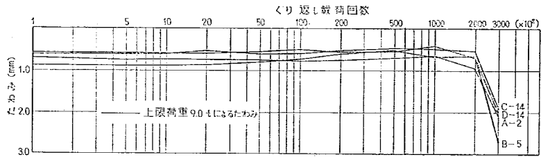
図-37 くり返し载荷回数とたわみ (舗装版中央部)
