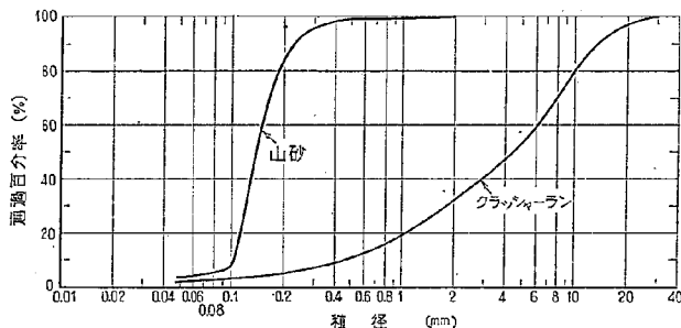
図-9 昭和36年度に施工した路床路盤材料の粒度
