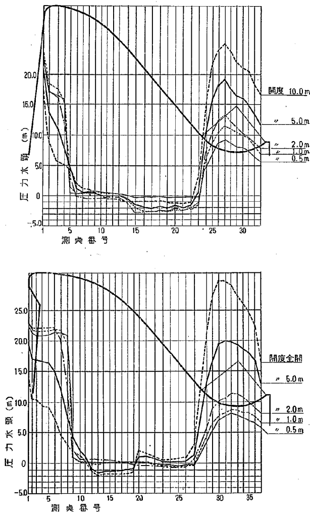
図-23 2型越流部門扉操作時圧力分布図
