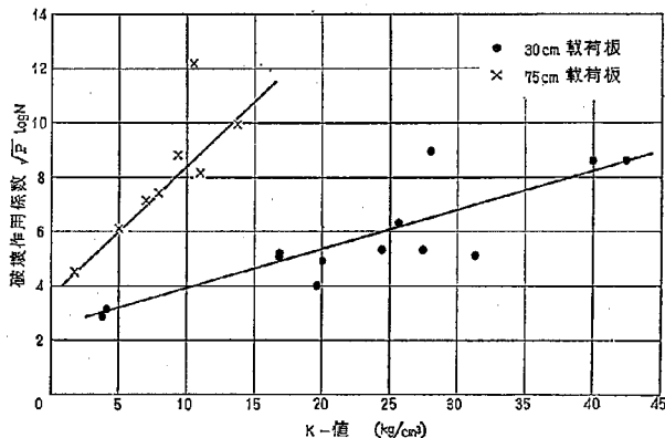
図-29 K 値と \sqrt{P} \log N の関係
