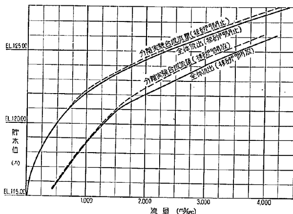
図-47 水位—流量曲線の比較
