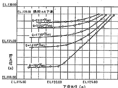
図-38 (2) 中央越流部下流水位の変化にともなう貯水位の変動
