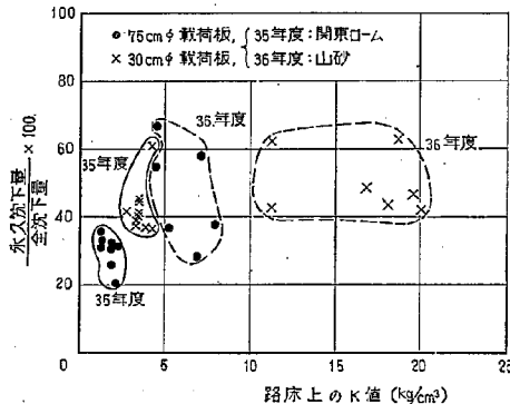
図-16 路床上での載荷試験結果
