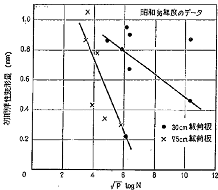
図-35 \sqrt{p} \log N と初期弾性変形量の関係
