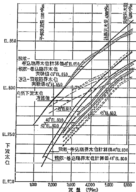
図-9 跳水水位の比較
