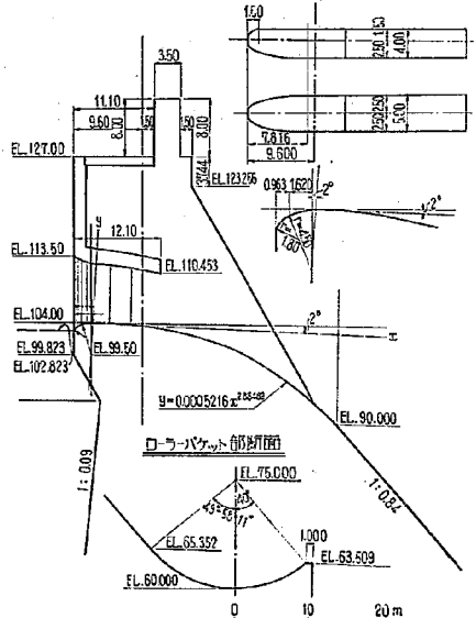
図-19 (2) 2型余水吐越流部定規図
