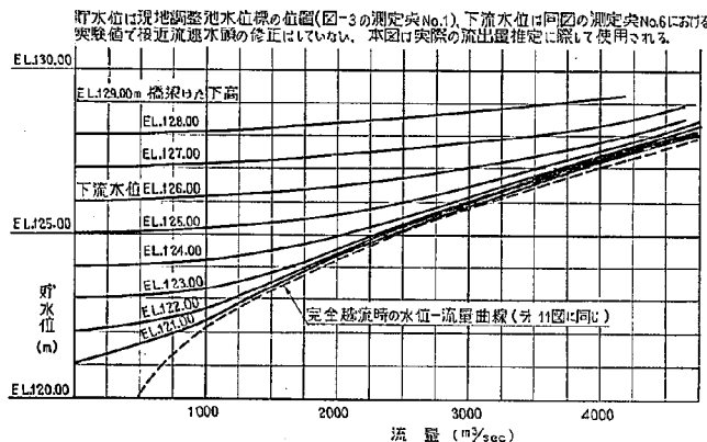
図-34 (2) 下流水位の変化にともなう水位-流量曲線 (排砂門閉止)
