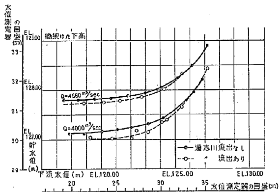
図-31 道志川流出が貯水位におよぼす影響の比較
