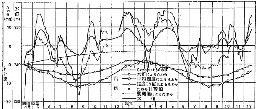
図-2.11 鴨子ダムたわみ解析図
