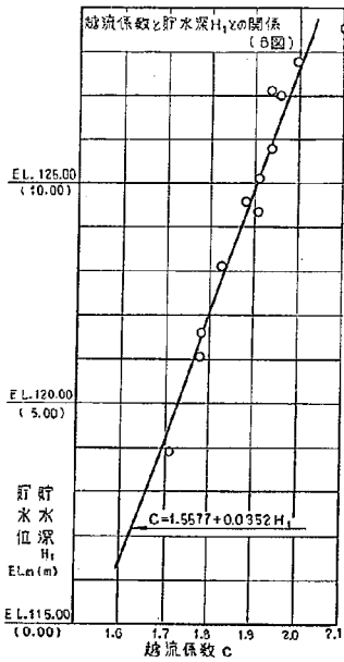
図-39 中央越流部越流係数と貯水深との関係
