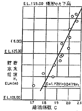
図-40 左岸固定せき越流係数と貯水深との関係
