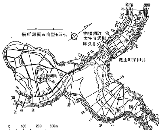
図-29 津久井ダム付近平面図
