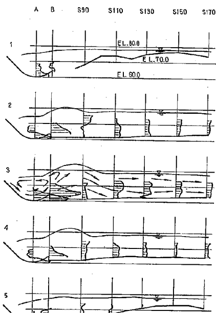
圖-26 (3) 減勢池內流速分布, 水面形 Q=2,000\text{m}^3/\text{sec}
