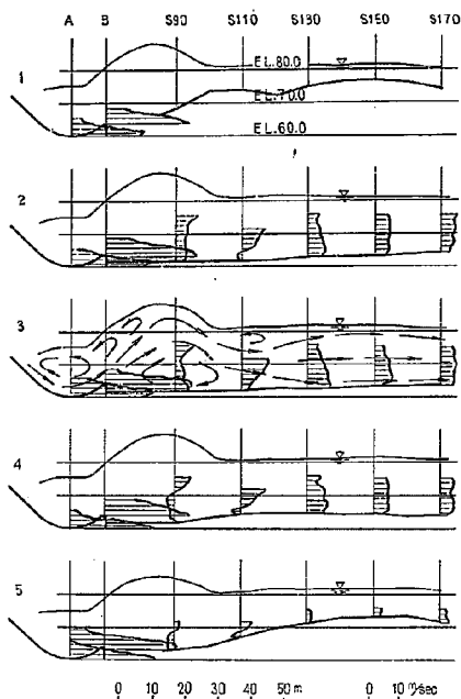
図-26 (5) 減勢池内流速分布, 水面形 Q=4,200\text{m}^3/\text{sec}
