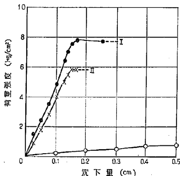
図-27 ソイルセメント層の載荷試験結果
