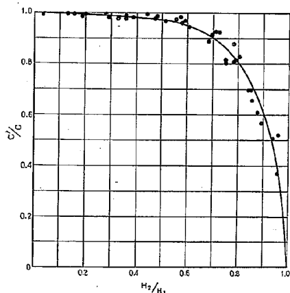
図-50 右岸固定せきの H_2/H_1 と C/C の関係
