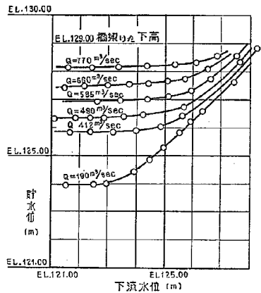
図-41 (1) 左岸固定せき下流水位の変化にともなう貯水位の変動
