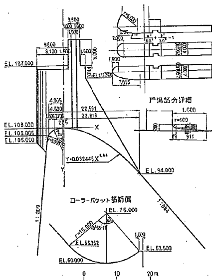
図-19 (1) 2型余水吐越流部定規図
