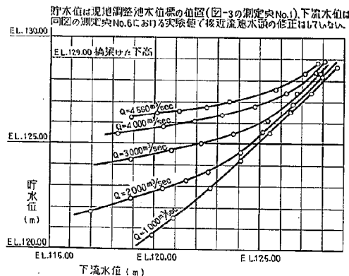
図-35 (1) 下流水位の変化にともなう貯水位の変動 (排砂門開放時)
