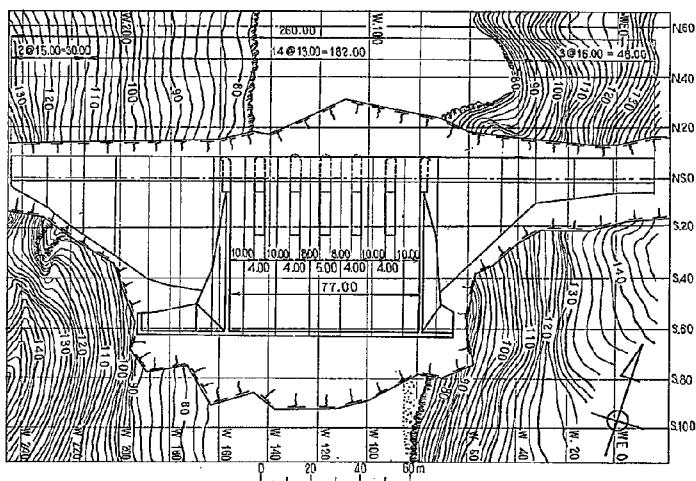
図-18 (1) 2 型余水吐平面
