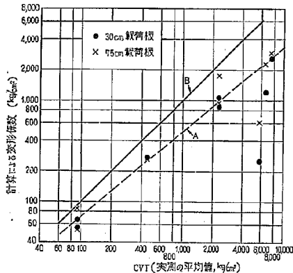
図-20 弾性理論より求めた変形係数と実測による CVT の関係 (路盤材料の場合)
