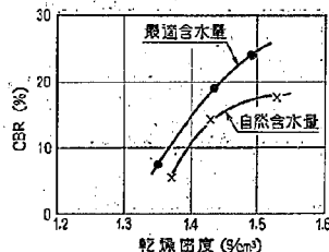
図-11 路床土(山砂)のCBR試験結果
