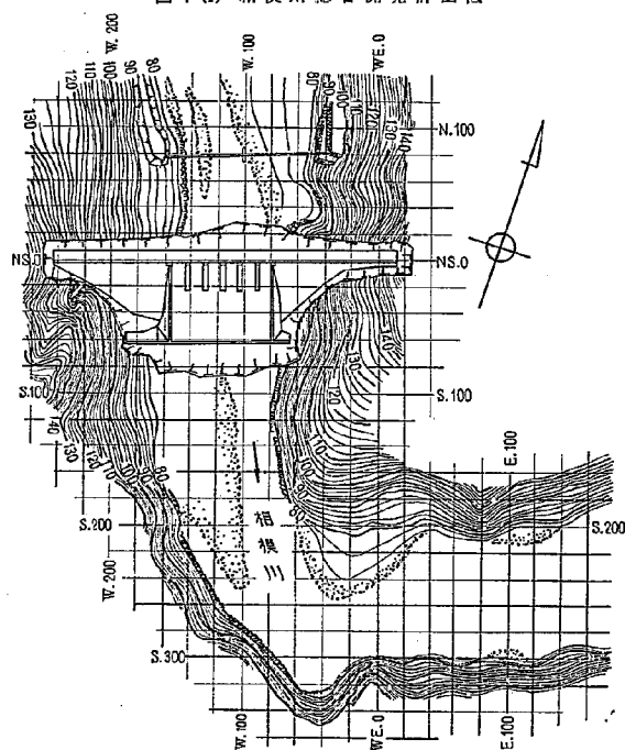
図-1 (1) 相模川総合開発計画図
