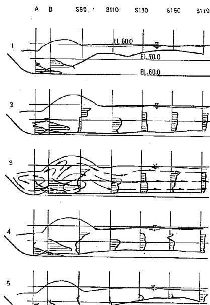
圖-26 (4) 減勢池內流速分布, 水面形 Q=3,000\text{m}^3/\text{sec}
