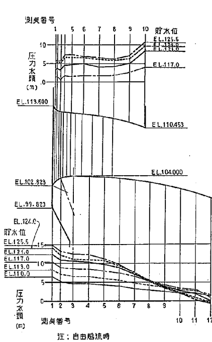
図-17 (1) オリフィス 3 型圧力分布図
