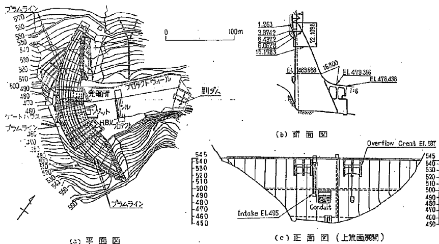
図-2.8 二瀬ダム
