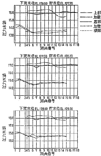
図-38 (8) 排砂門圧力分布図
