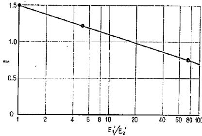
図-24 \zeta と E_1'/E_2' の関係
