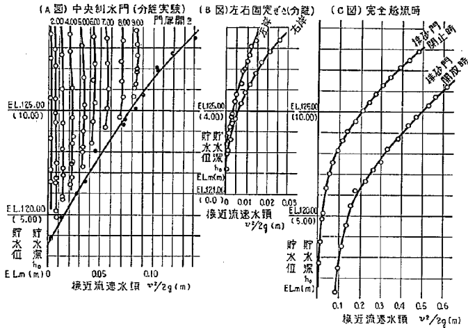
図-52 模型における貯水位と接近流速水頭の関係
