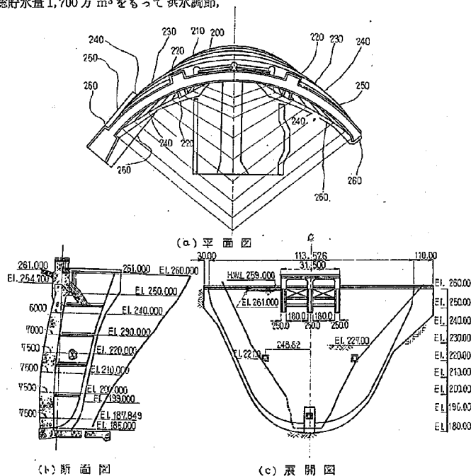
図-2.12 室牧ダム一般図
