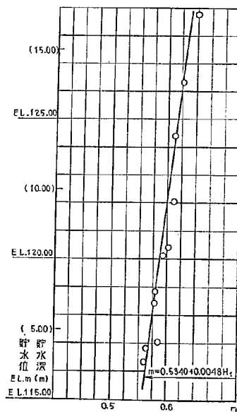
図-44 (2) 流量係数と貯水深との関係
