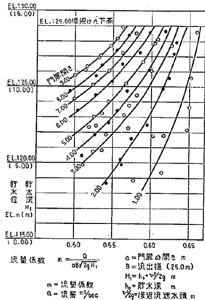
図-46 門扉等高操作時の流量係数（完全流出）
