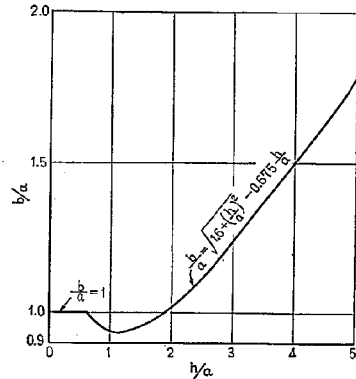
図-26 Westergaard の式における b と a の関係
