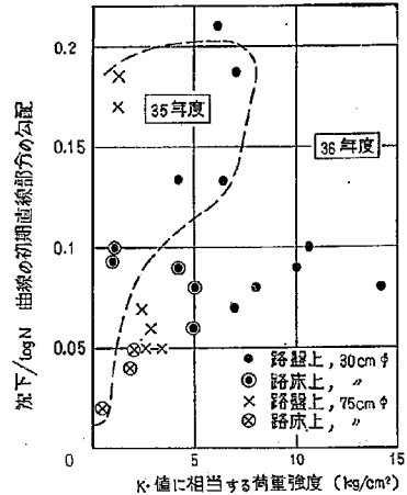
図-32 路床路盤の支持力の大小と初期直線部分のこう配
