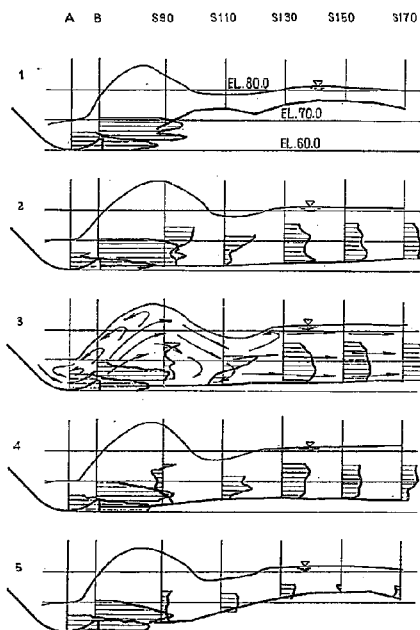
図-26 (7) 減勢池内流速分布, 水面形 Q=5,900\text{m}^3/\text{sec}
