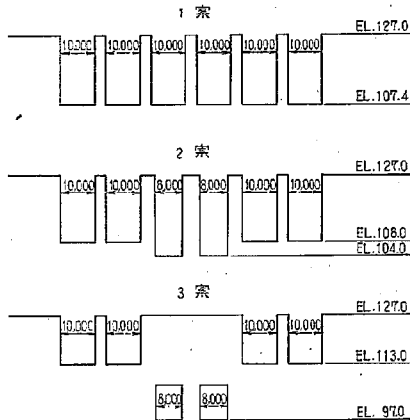
図-3 余水吐比較案
