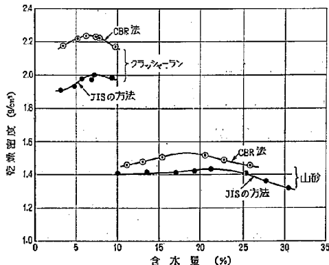
図-10 路床路盤材料の突固め試験結果
