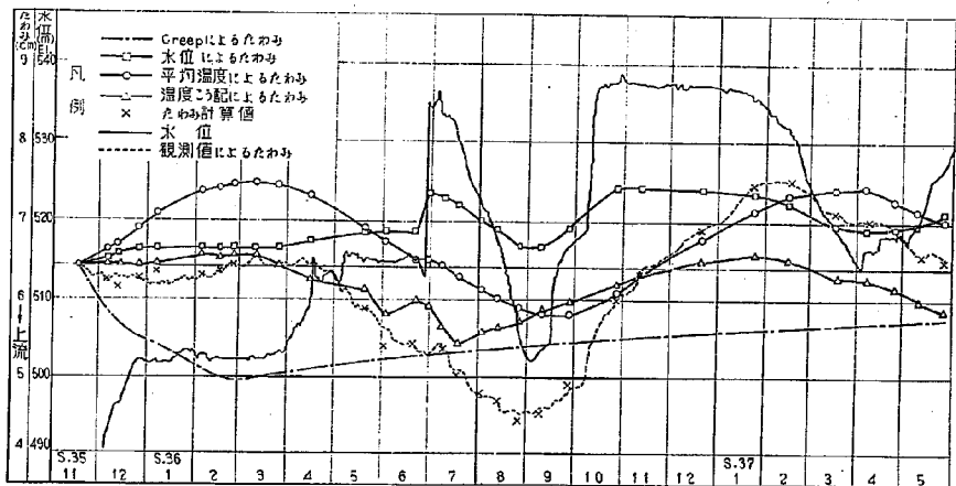
図-2.9 二瀬ダムのたわみ解析
