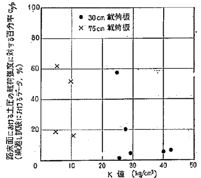
図-33 K 値と繰返し載荷による \sigma_n/p との関係
