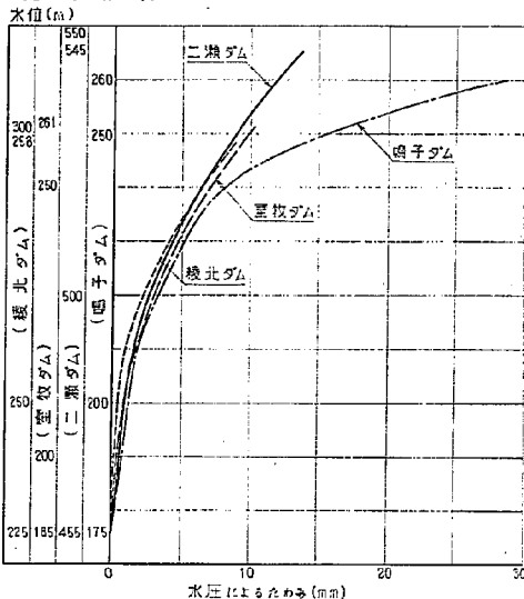
図-2.16 水深たわみ曲線図
