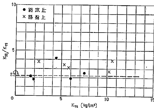
図-18 K_{30} と K_{15} の関係
