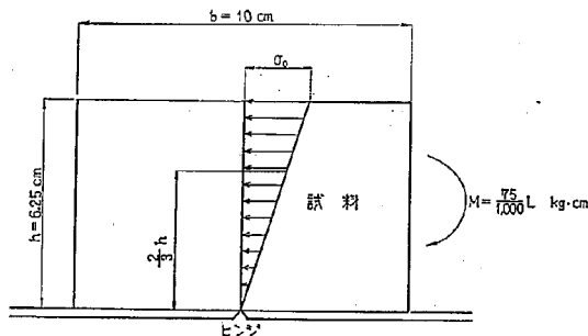
図-28 コヘイジョメーターの説明図
