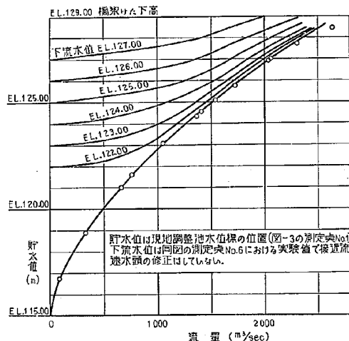
図-38 (1) 中央越流部下流水位の変化にともなう水位-流量曲線
