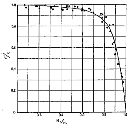
図-49 左岸固定せきの H_2/H_1 と C/C の関係
