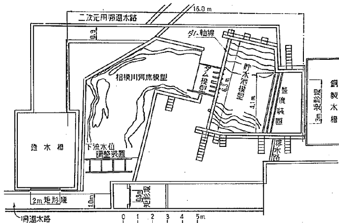
図-2 城山ダム模型配置図
