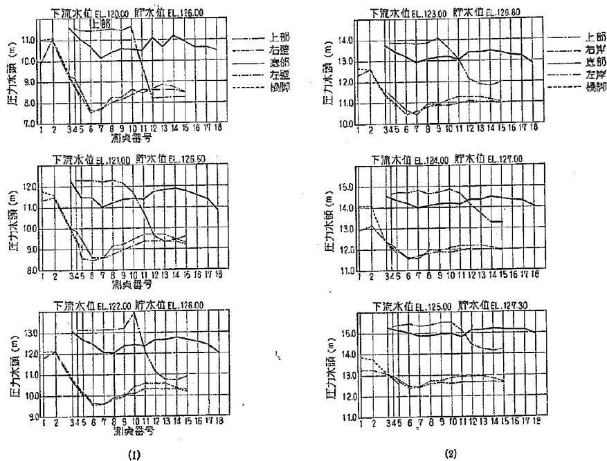
圖-37 排砂門壓力分布圖
