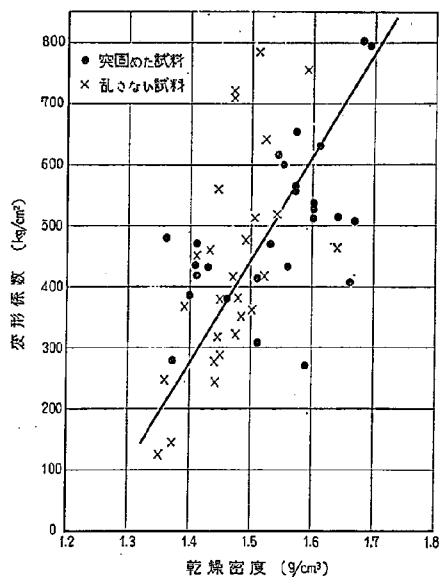
図-12 路床土（山砂）に関する CVT 試験結果
