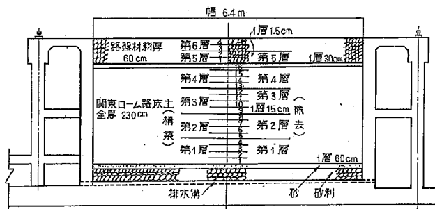
図-14 テストピット中央付近断面図
