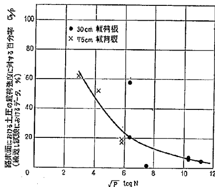
図-36 \sqrt{p} \log N と \sigma_a/p の関係
