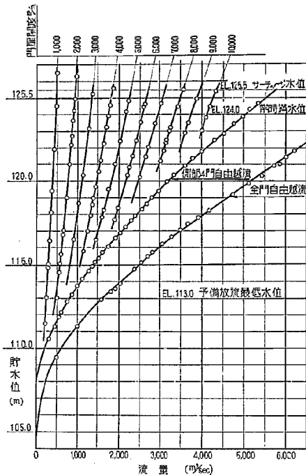
図-7 1型余水吐水位—流量曲線
