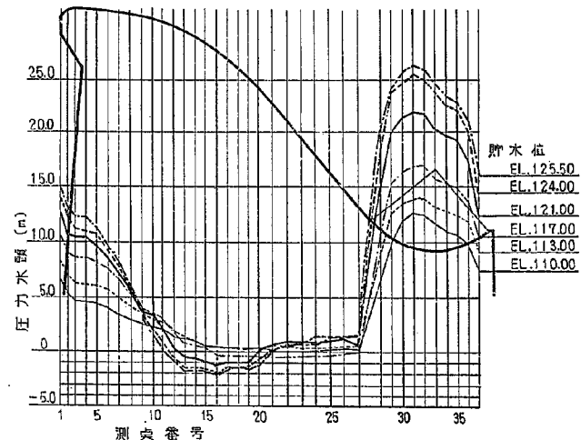
図-22 2 型越流部自由越流時圧力分布図
