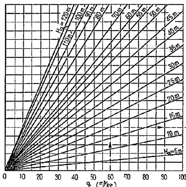
図-5 跳水共軛水深と飛散巻込臨界水深との関係
