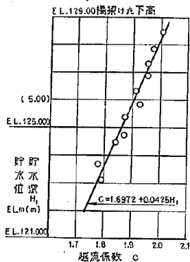
図-42 右岸固定せきの越流係数と貯水深との関係
