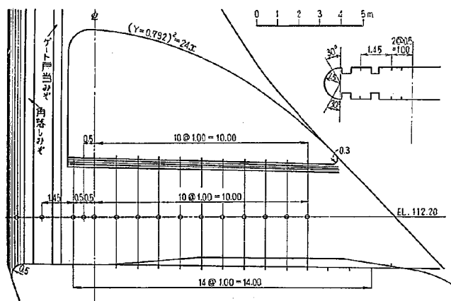
圖-36 排砂門壓力測定点配置圖
