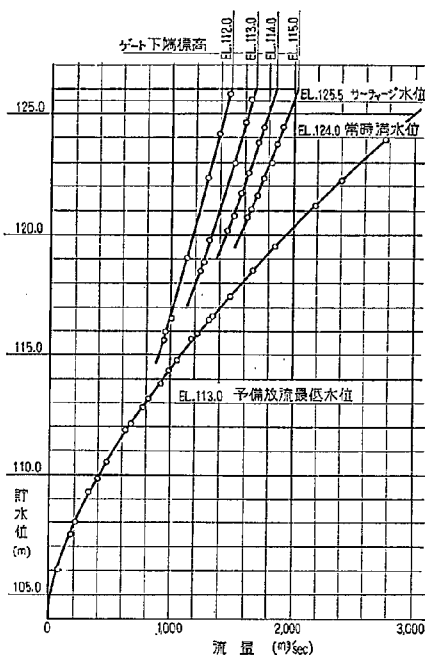
図-8 1型余水吐中央部水位—流量曲線
