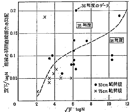
図-34 \sqrt{p} \log N と沈下/ \log N 曲線の初期直線部分のこう配
