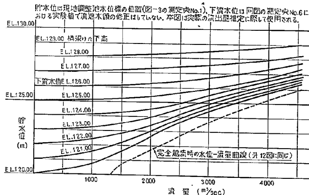
図-35 (2) 下流水位の変化にともなう水位-流量曲線 (排砂門開放)
