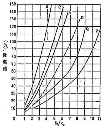
図-22 路盤厚と K_1/K_2 の関係 (30 cm 載荷板を使用する場合)
