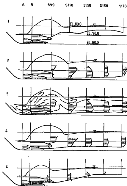
図-26 (6) 減勢池内流速分布, 水面形 Q=4,900\text{m}^3/\text{sec}
