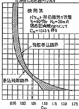
図-5 跳水共軛水深と飛散巻込臨界水深との関係
