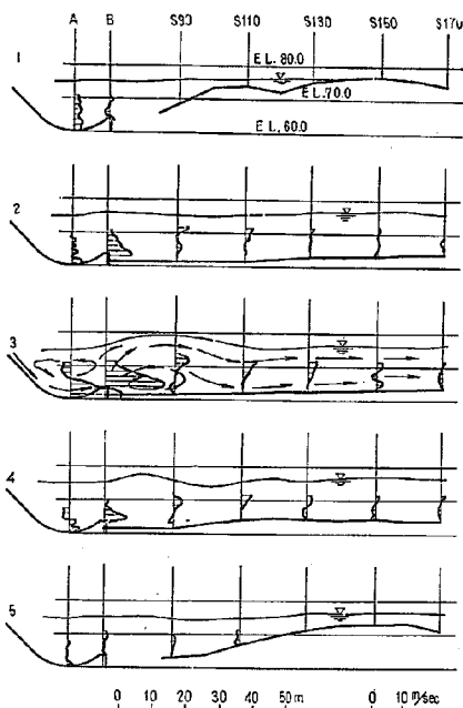
圖-26 (1) 減勢池內流速分布, 水面形 Q=700\text{m}^3/\text{sec}
