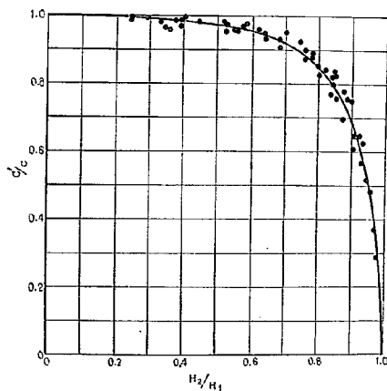
図-48 (1) 中央越流部の H_2/H_1 と C'/C の関係
