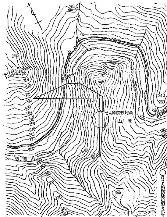
図-4.2 下久保ダムサイト一般平面図
