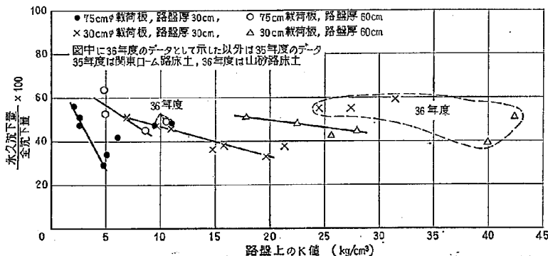
図-17 路盤上での載荷試験結果
