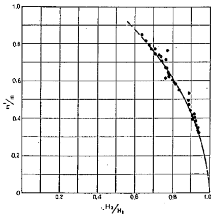
図-51 排砂門の H_2/H_1 と m'/m の関係
