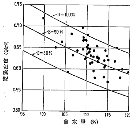
図-4 路床土の施工管理試験結果 (乱さない試料による)
