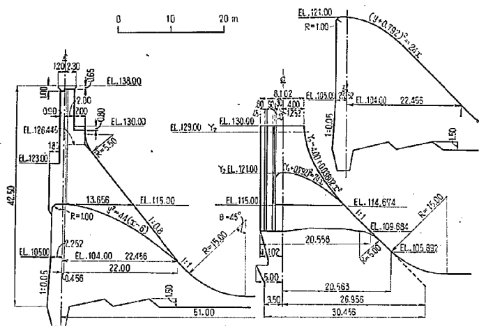
図-28 (3) 越流都定規圖
