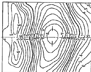
流量 4300 貯水値 125.5 下流水値 81.1 門扉操作 全門扉操作で均等に放流した場合
