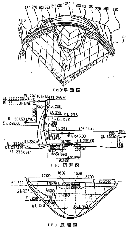
図-2.14 綾北ダム一般図
