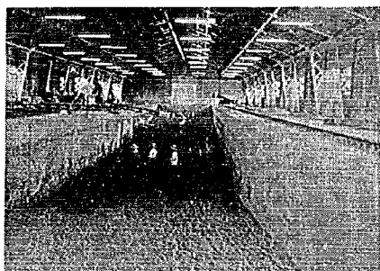
写真-3 路床材料の運搬と締固め
