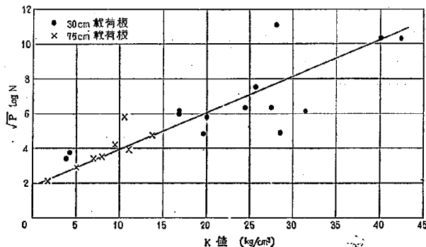
図-30 K 値と \sqrt{p} \log N の関係
