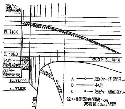
図-10 オリフィス抽出実験越流水脈水面形状
