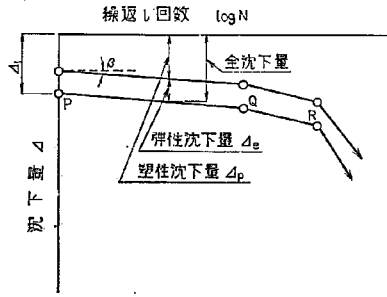
図-31 繰返し載荷試験結果の模型図
