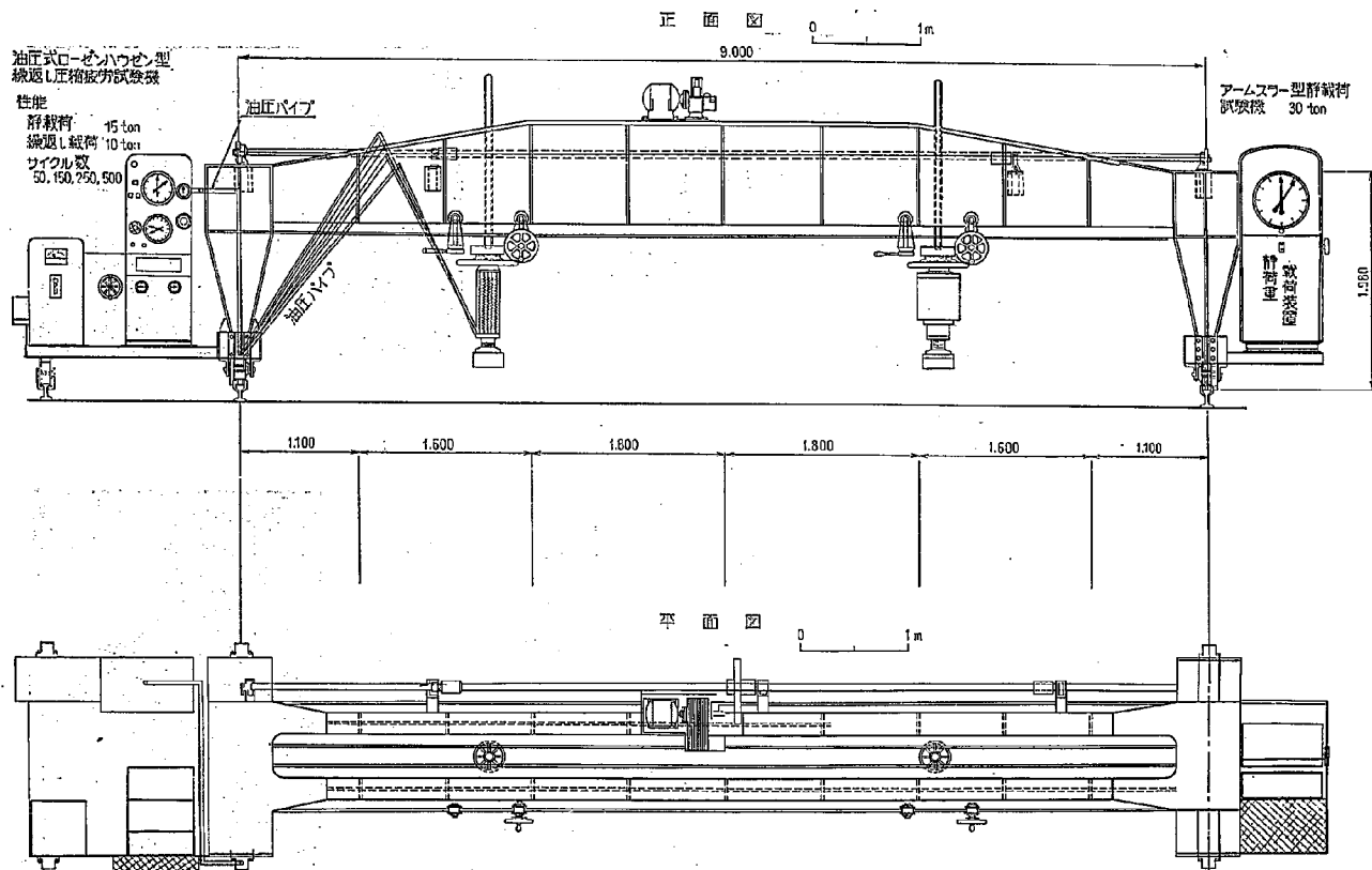
図-2 30 ton 載荷試験機
