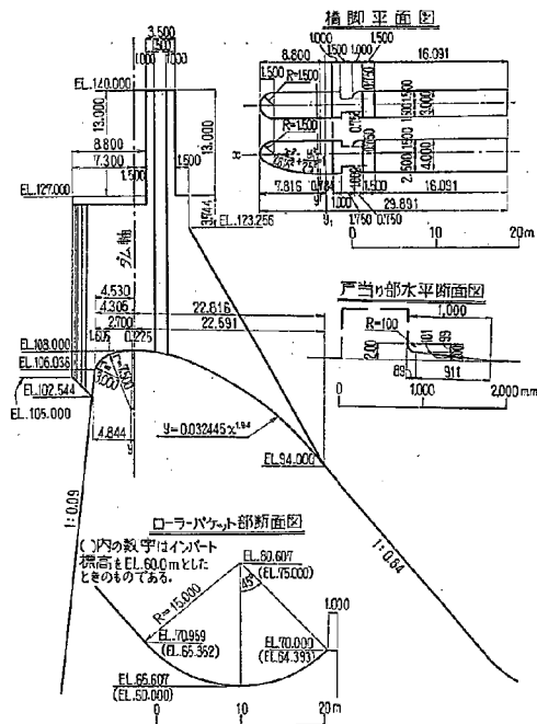
図-6 (a) 越流部定規図 (側部)
