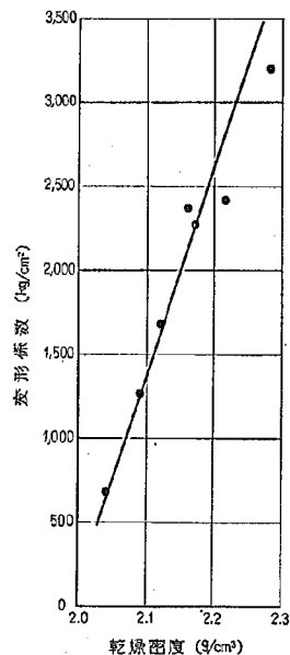
図-13 路盤材料（クラッシャーラン）の CVT 試験結果
