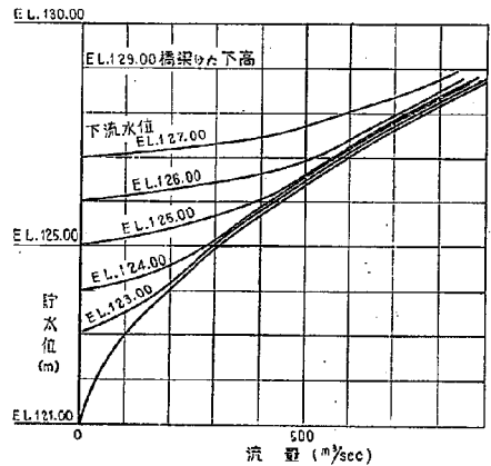
図-41 (2) 下流水位の変化にともなう水位-流量曲線
