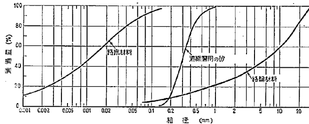
図-3 昭和35年度に施工した路床路盤材料の粒度
