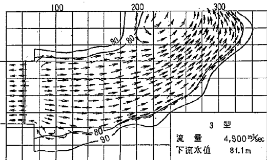
図-25 減勢池内流線図
