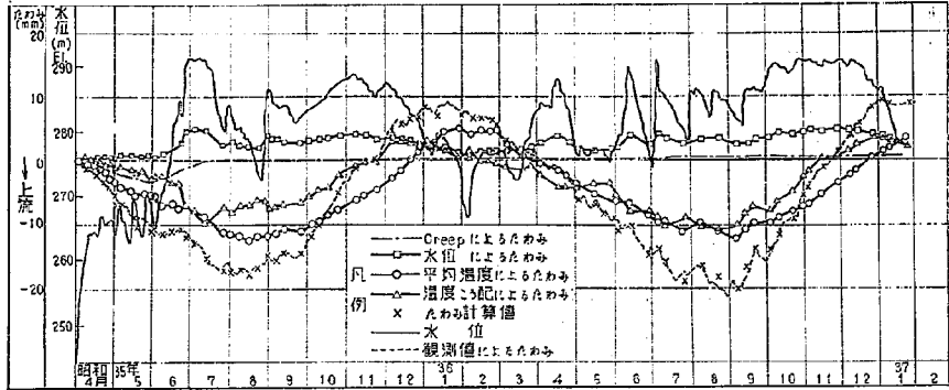
図-2.15 綾北ダムたわみ解析
