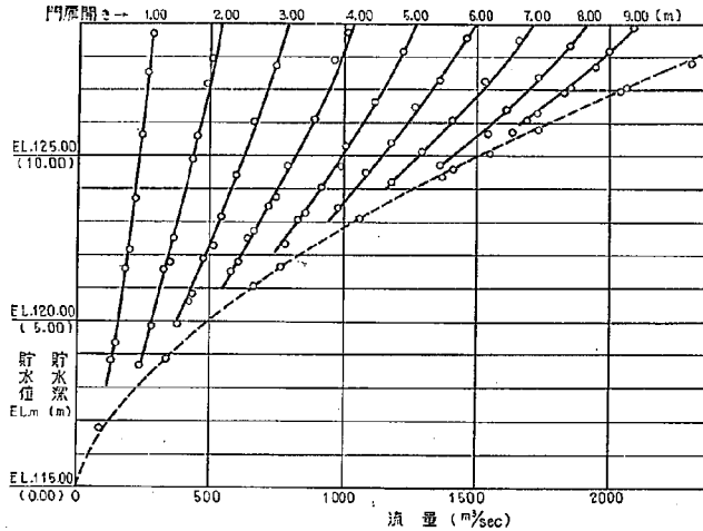
図-45 門扉等高操作時の水位-流量曲線（完全流出）
