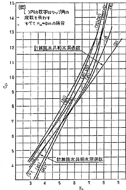
図-4 フルード数-飛散巻込臨界水深係数関係曲線
