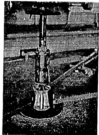
写真-2 載荷試験中の載荷板の沈下測定
