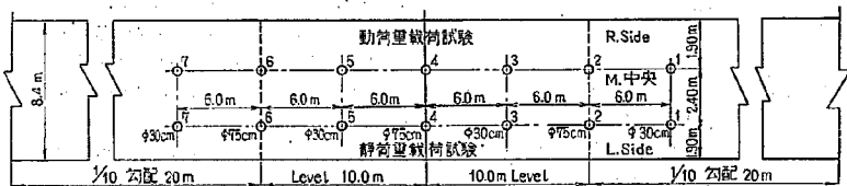
図-15 テストピット平面図 (載荷試験位置を示す)
