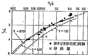
図-25 土研報告 95 号の図-17 より複製
