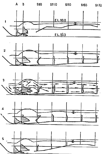
圖-26 (2) 減勢池內流速分布, 水面形 Q=1,500\text{m}^3/\text{sec}
