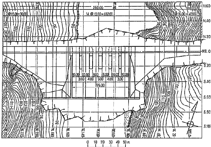
図-6 (1) 1 型余水吐平面
