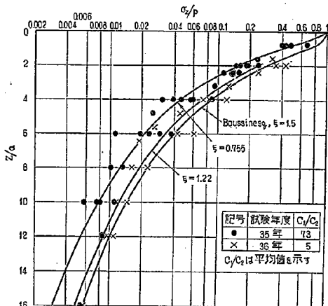
図-23 \sigma_z/p と z/a の関係
