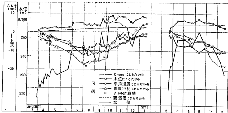
図-2.13 室牧ダムたわみ解析図
