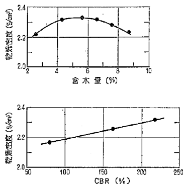
図-7 路盤材料についての CBR 試験結果
