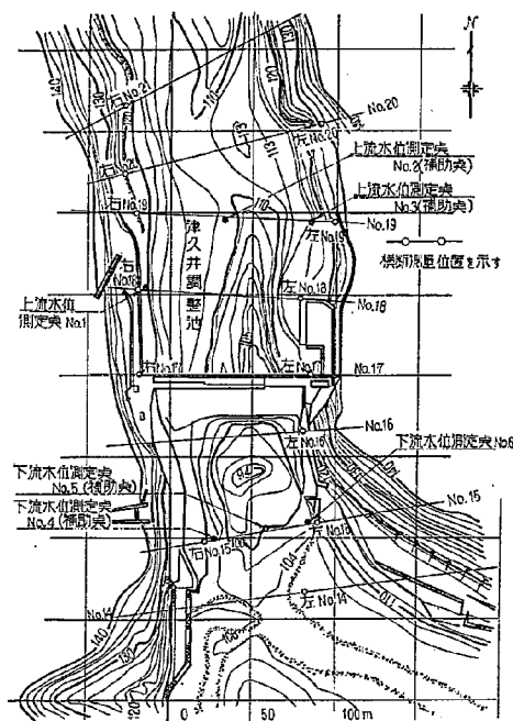
図-30 水位測定点位置図
