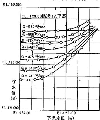
図-43 (1) 右岸固定せき下流水位の変化にともなう貯水位の変動
