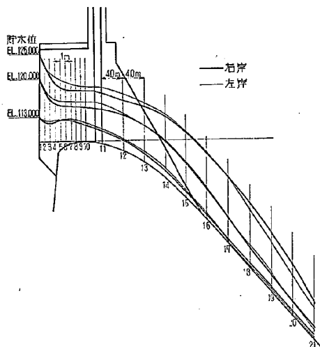
図-24 越流水脈水面形状
