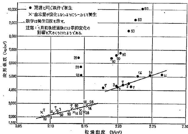
図-8 路盤材料の CVT 試験結果
