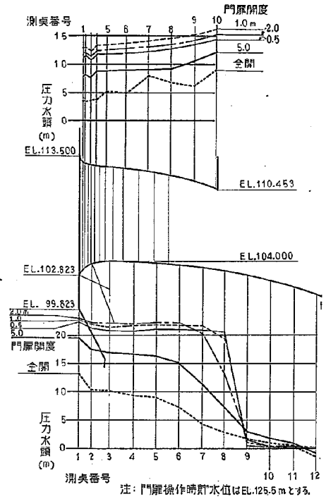
図-17 (2) オリフィス 3 型圧力分布図
