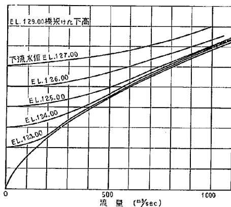
図-43 (2) 右岸固定せき下流水位の変化にともなう水位—流量曲線
