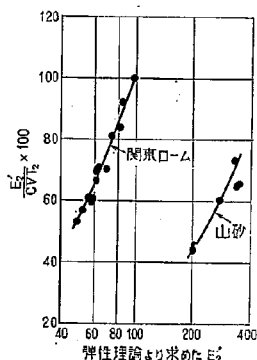
図-19 弾性理論より求めた変形係数と乱さない試料による CVT の関係(路床土の場合)
