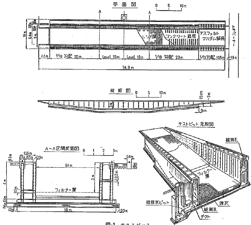
図-1 テストピット
