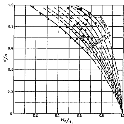
図-48 (2) 門扉等高操作時
