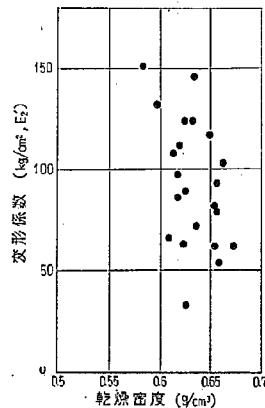
図-5 乱さない試料による CVT 試験結果 (関東ローム路床土)
