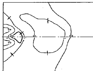
流量 700 貯水位 113.0 下流水位 74.2 門扉操作 中央2門で放流した場合
