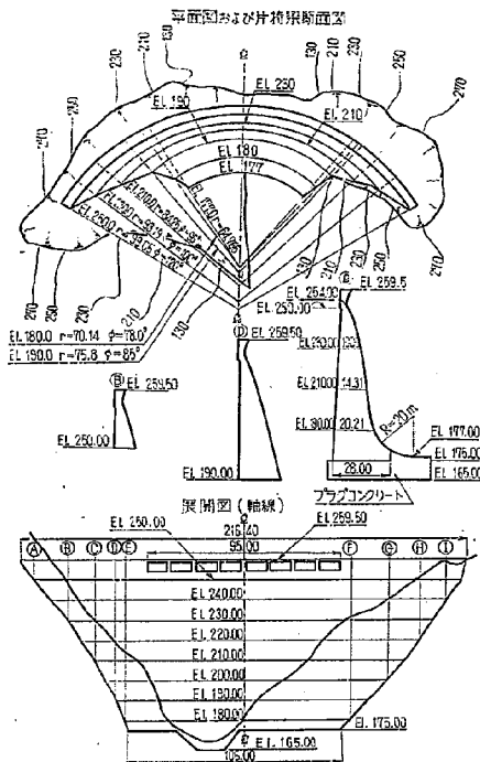
図-2.10 鳴子ダム一般図
