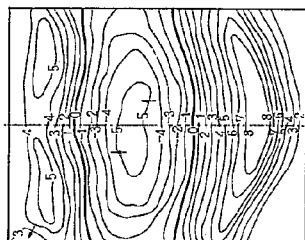
流量 3000 貯水値 124.0 下流水値 79.2 門扉操作 全門扉操作で均等に放流した場合
