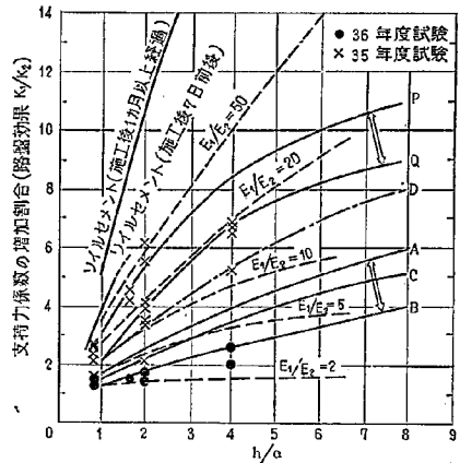
図-21 路盤厚と路盤効果の関係 (ソイルセメントの曲線は暫定的なもの)
