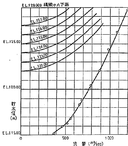
図-44 (1) 排砂門下流水位の変化にともなう水位—流量曲線
