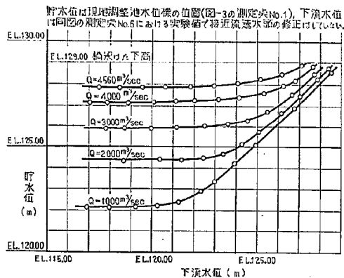
図-34 (1) 下流水位の変化にともなう貯水位の変動 (排砂門閉止時)
