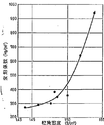
図-6 砂の乾燥密度と CVT 試験結果
