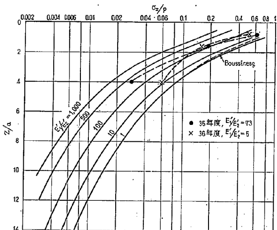
図-37 繰返し載荷試験結果
