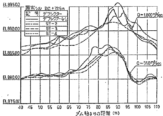
図-45 右岸導流壁沿い水面形状
