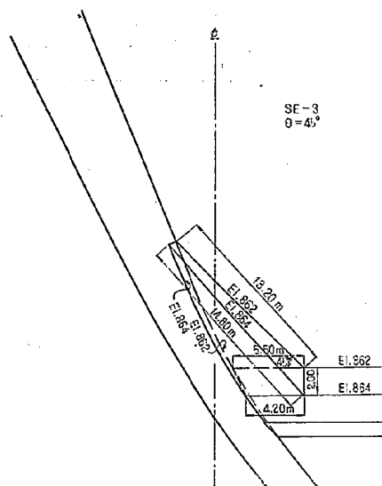
図-46(2) シルデフレクター形状
