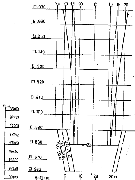
図-23 越流部落下水脈軌跡
