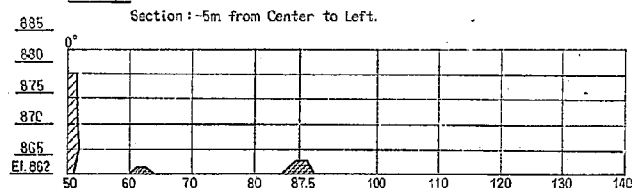
図-54(1) 水叩き内流速分布図 (R. W. L. 976.00 m 放水管 2 門)
