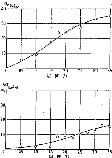
図-15 F-7 沿いの応力増加曲線 (Wall 入り模型)
