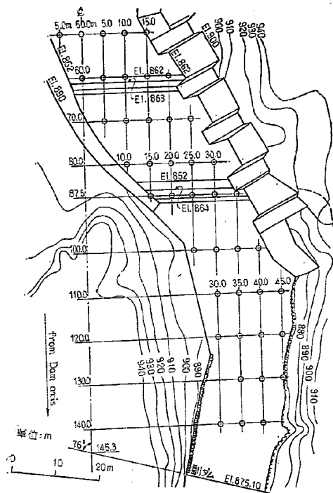
図-53 流速測定点配置図
