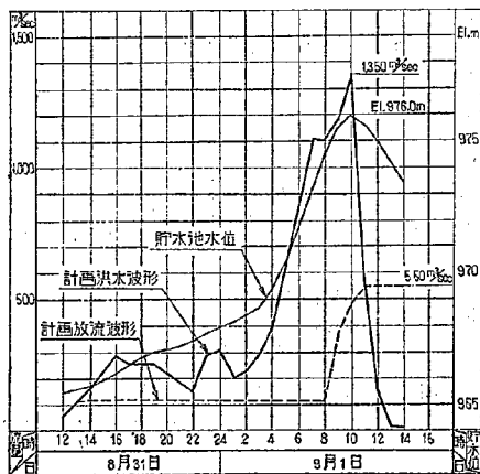
図-2 洪水調節計画図
