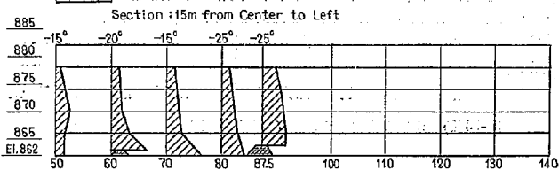
図-54(3) 水叩き内流速分布図 (R. W. L. 976.00 m 放水管 2 門)
