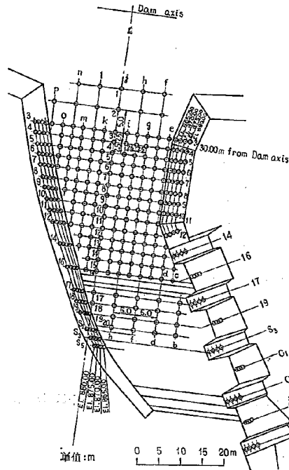
図-56 水叩き部圧力測定点配置図
