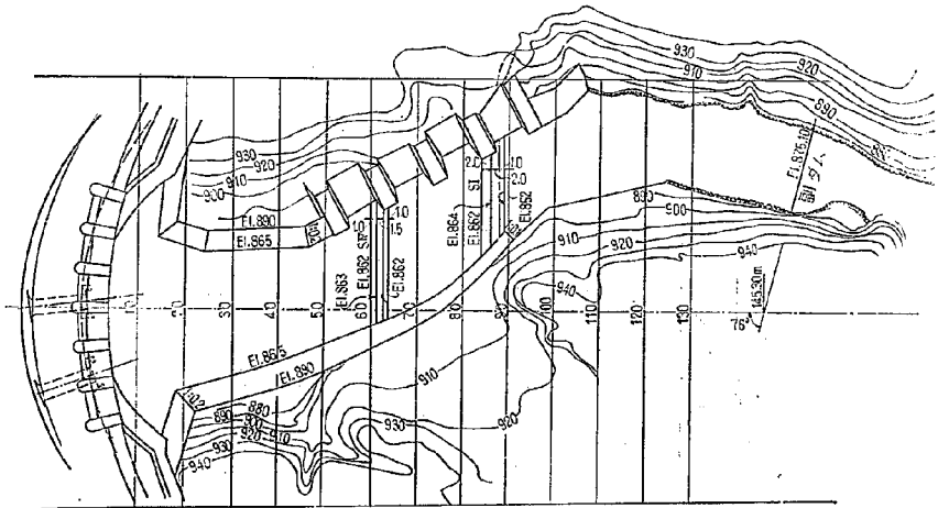
図-50 最終案水じょく池平面形状
