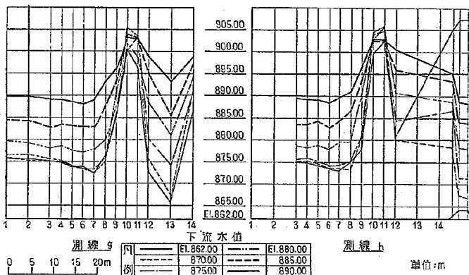
図-10(4) 水叩面圧力測定 縦断面 貯水位 El. 979.00 m
