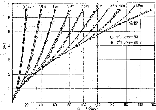
図-20 越流部貯水位-流量関係図 (1 径間)
