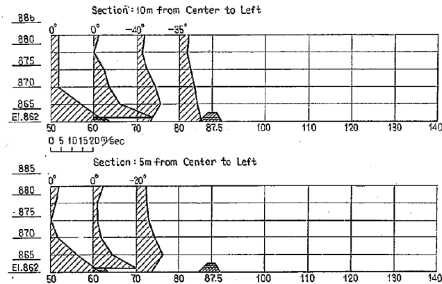
図-55(2) 水叩き内流速分布図 (R. W. L. 979.00 m Over lap)
