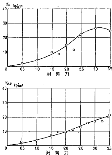
図-14 F-9 沿いの応力増加曲線 (Wall 入り模型)
