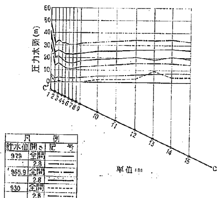
図-34 放水管内圧力分布図
