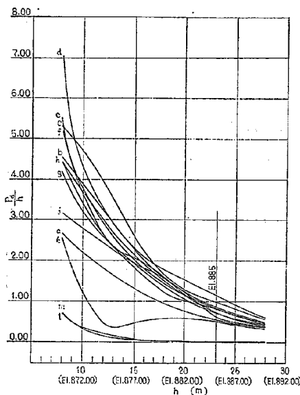
図-11 P_a/h-h 曲線
