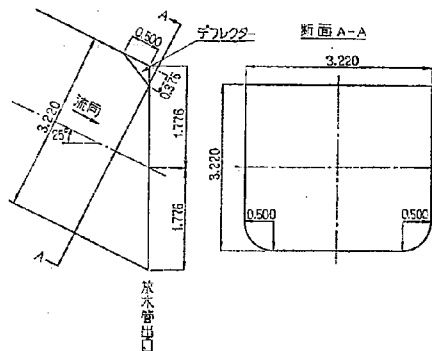
图-13 放水管出口断面形状
