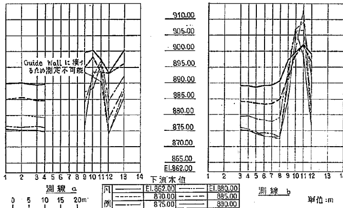
図-10(1) 水叩面圧力測定、縦断面 貯水位 El. 979.00 m
