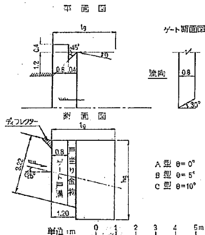
図-28 放水管ゲート記号図
