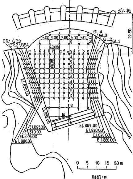
図-9 第一案水じょく池圧力パイプ配置図
