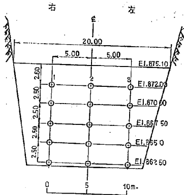
図-58 副ダム圧力測定点配置図
