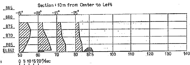
図-54(1) 水叩き内流速分布図 (R. W. L. 976.00 m 放水管 2 門)
