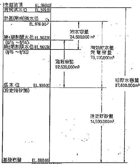
図-3 川俣ダム貯水池使用計画図
