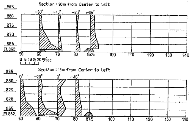
図-55(3) 水叩き内流速分布図 (R. W. L. 979.00 m Over lap)
