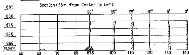
図-54(4) 水叩き内流速分布図 (R. W. L. 976.00 m 放水管 2 門)
