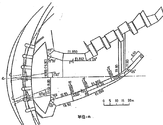
図-12 余水吐水じょく池平面図
