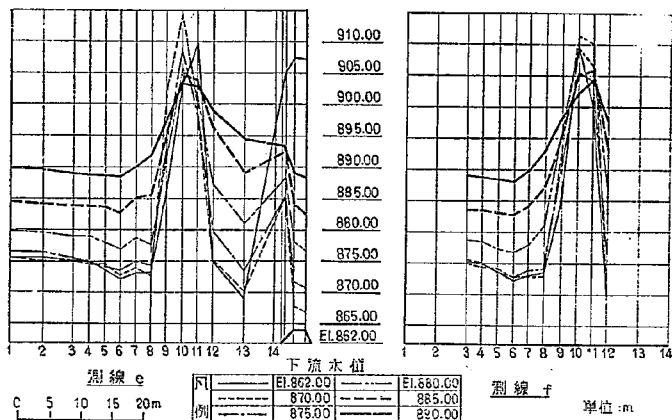
図-10(3) 水叩面圧力測定 縦断面 貯水位 El. 979.00 m
