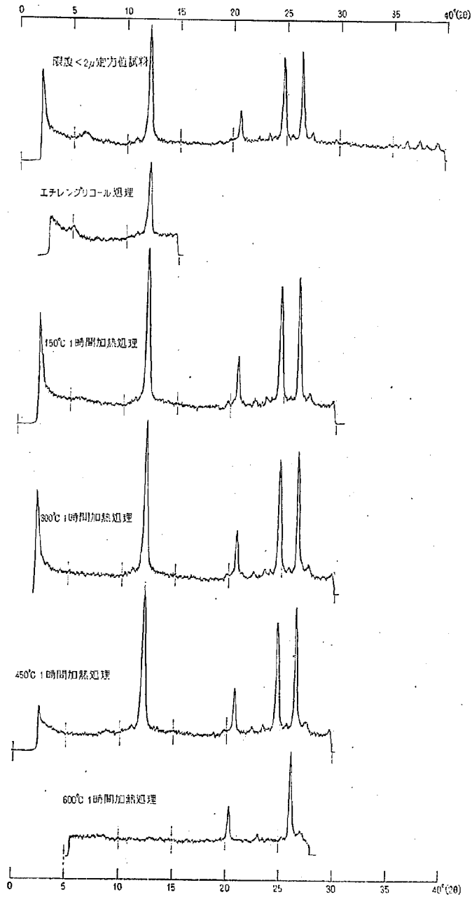
図-9 断層(30)の粘土X線分析図(測定 金子幸子)
