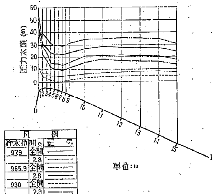
図-35 放水管内圧力分布図
