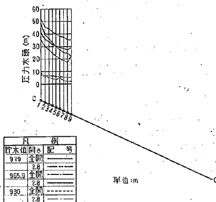
図-33 放水管内圧力分布図
