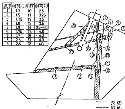
図-7 最終案の幅3.5m Wall入り模型の破壊状況
