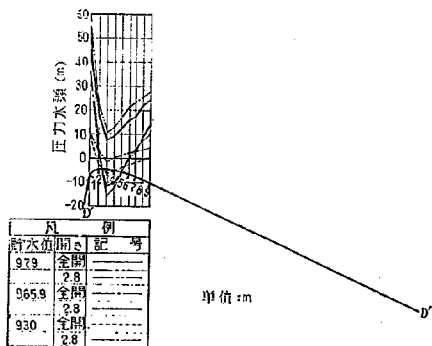
図-36 放水管内圧力分布図
