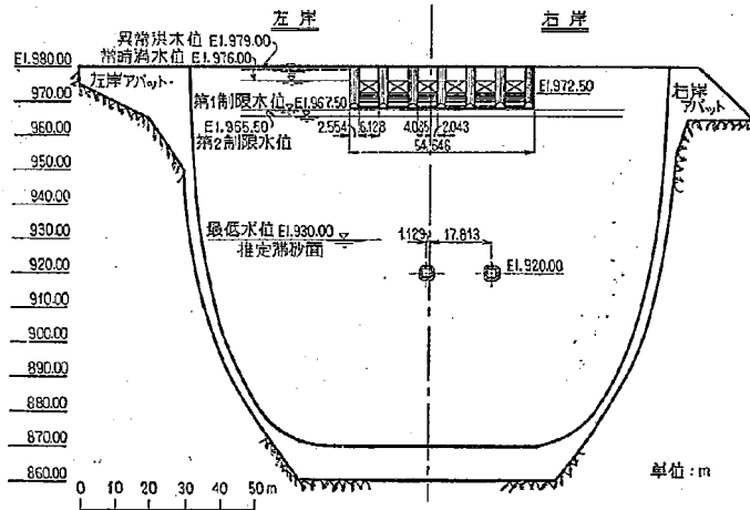
図-5(2) 上流面展開図 (ダム本体)
