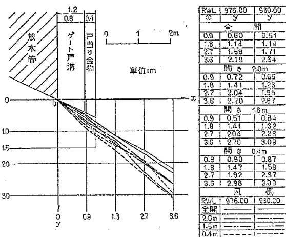
図-44 放水管放出水取下面軌跡
