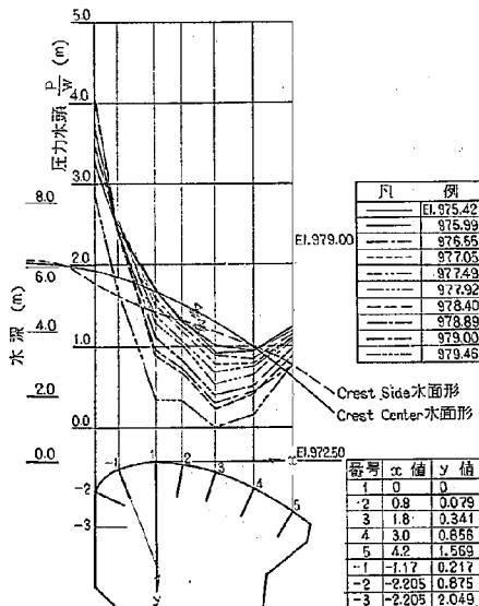
図-8 堤頂越流部水面形および圧力分布図
