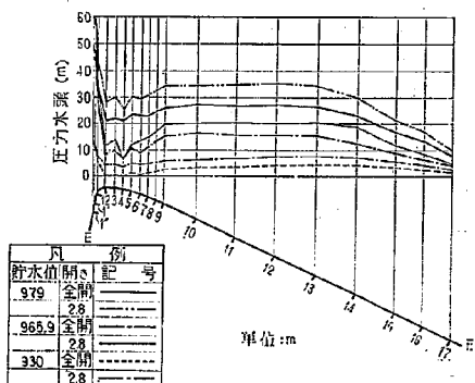
図-37 放水管内圧力分布図
