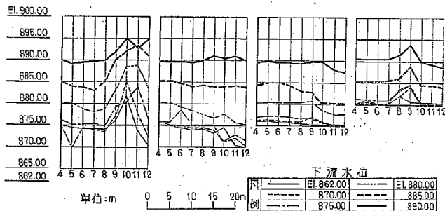
圖-10(8) 左岸側壁压力測定 縦断面 貯水位 EL. 979.00 m
