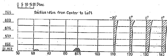
図-55(6) 水叩き内流速分布図 (R.W.L. 979.00 m Over lap)
