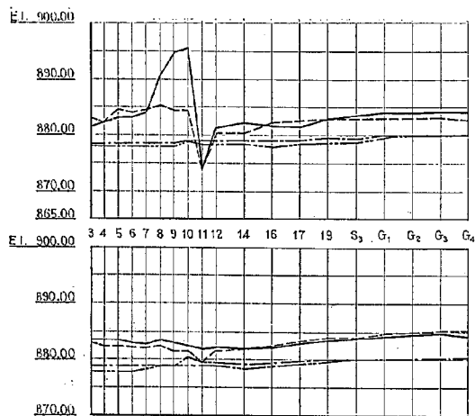
圖-57(11) 左岸側導流壁壓力分布圖
