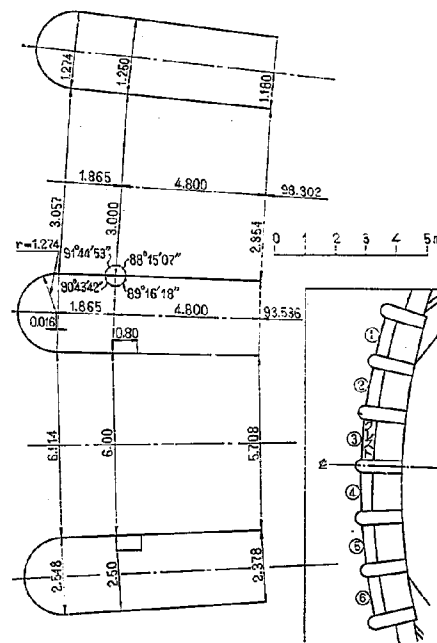
図-16 越流部模型平面図
