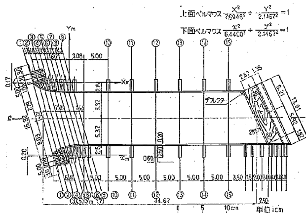
図-25 放水管模型図 (側面)
