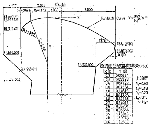
図-7 越流面標準断面図
