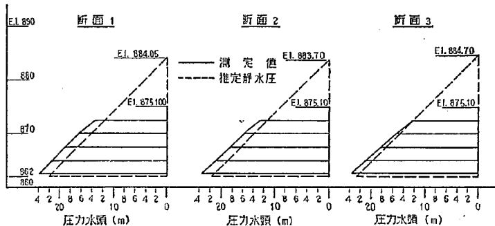
図-59 副ダム圧力分布図 ( Q=1,800 \text{ m}^3/\text{sec} )
