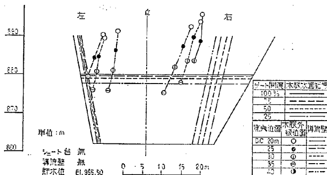
図-42 放水管放出水脈軌跡
