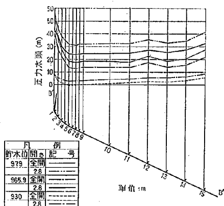
図-32 放水管内圧力分布図
