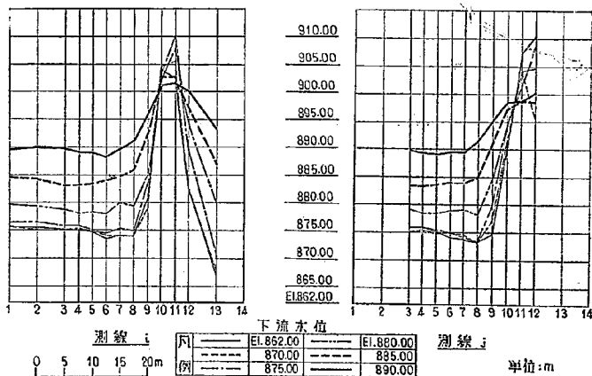
図-10(5) 水叩面圧力測定 縦断面 貯水位 El. 979.00 m
