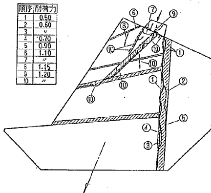
図-3 基礎処理前の模型の破壊状況
