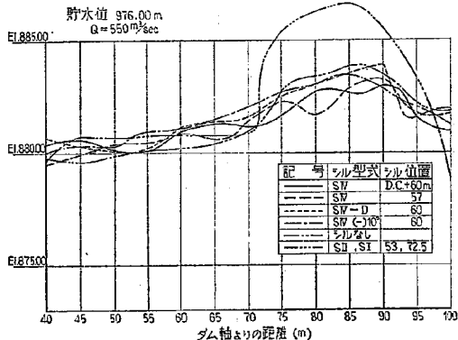
図-46 右岸導流壁沿い水面形状
