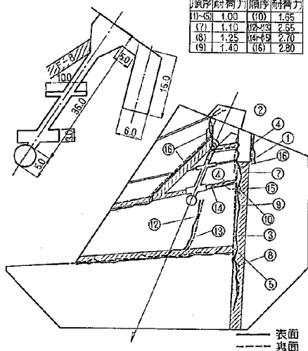
図-6 幅2m Wall (応力集中を防止したもの) 入り模型の破壊状況
