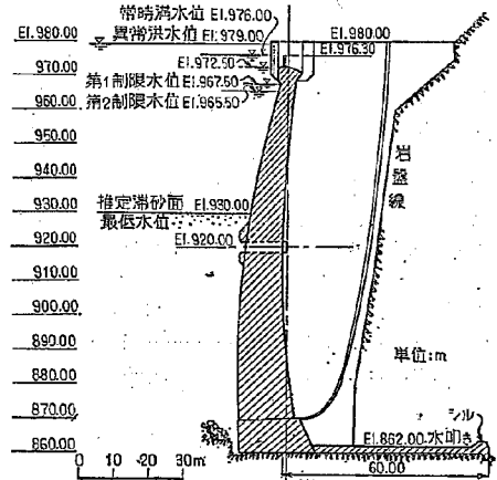
図-5(3) 標準断面図 (ダム本体)
