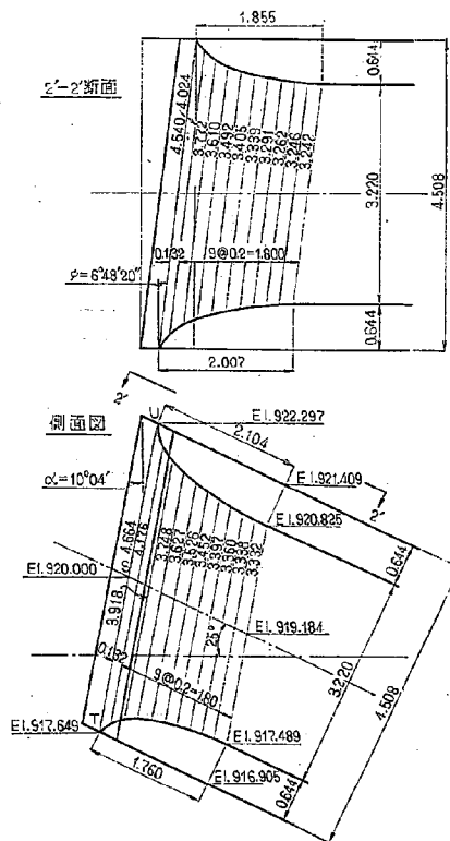
図-15(2) ヘルマウス形状 (左岸放水管)
