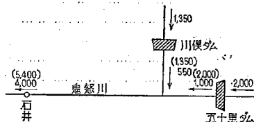
図-1 流量配分図
