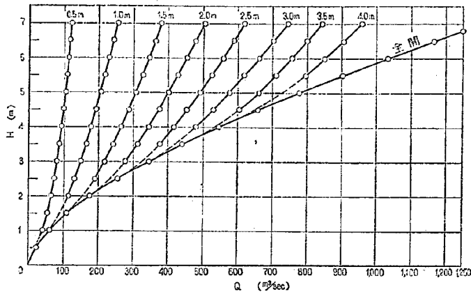
図-21 越流部貯水位一流量関係図(金門等高半開操作)
