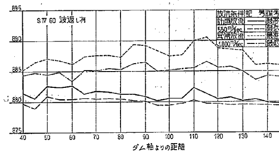
図-52(1) 左岸側導流壁沿い水面形
