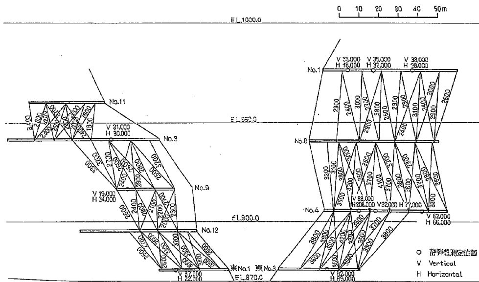
図-19 川俣ダムサイト弾性波速度、弾性係数表示図
