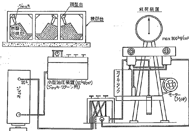
図-2 加圧装置略図
