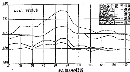
図-52(2) 右岸側導流壁沿い水面形
