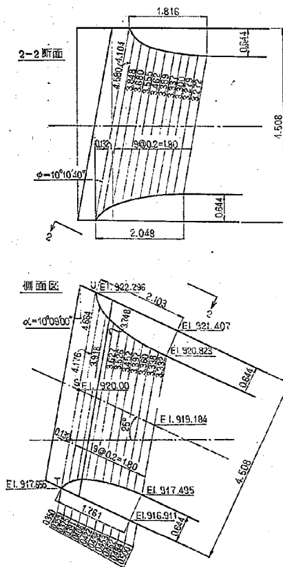
図-15(1) ヘルマウス形状 (右岸放水管)
