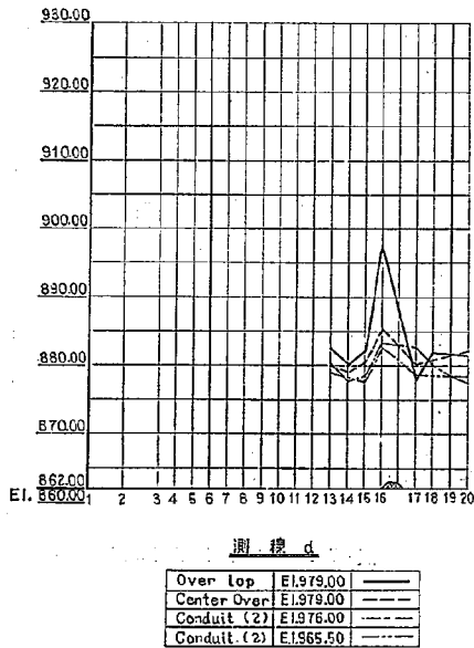
図-57(1) 水叩き面圧力分布図
