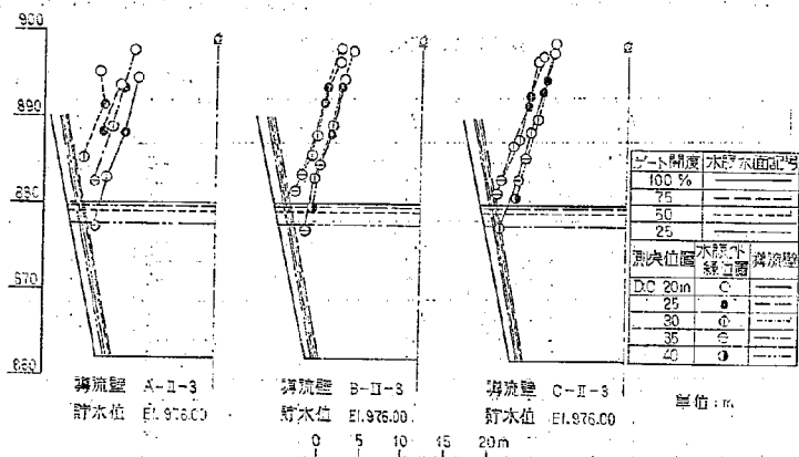
図-40 左岸側放水管放出水脈軌跡
