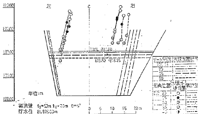
図-41 放水管水脈外縁軌跡
