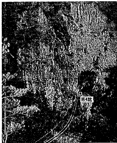
写真-2 右岸全景 (中央部第4坑付近の洞から左上へ延びるのは割れ目(20)、右上へ延びるのは噴気ガスによる変質部を伴う割れ目)
