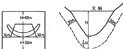
図-4 ダム地点決定調査地質調査範囲
