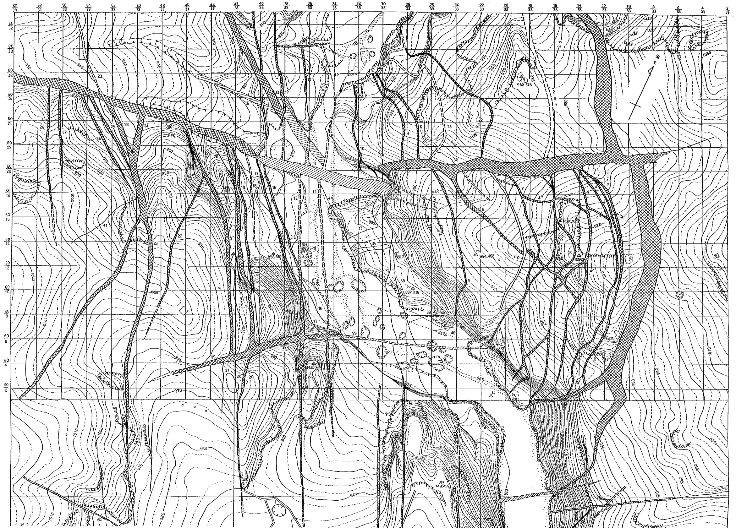
図-8 川俣ダムサイト地質図(クラック マップ)
