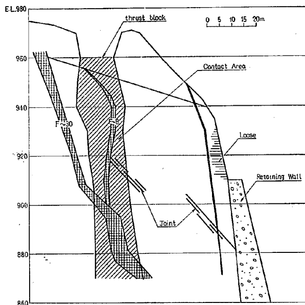
図-13 (g) 地質垂直断面図 (左岸アバットメント)
