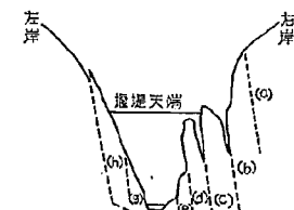
図-3 川俣ダムサイト地質断面図
