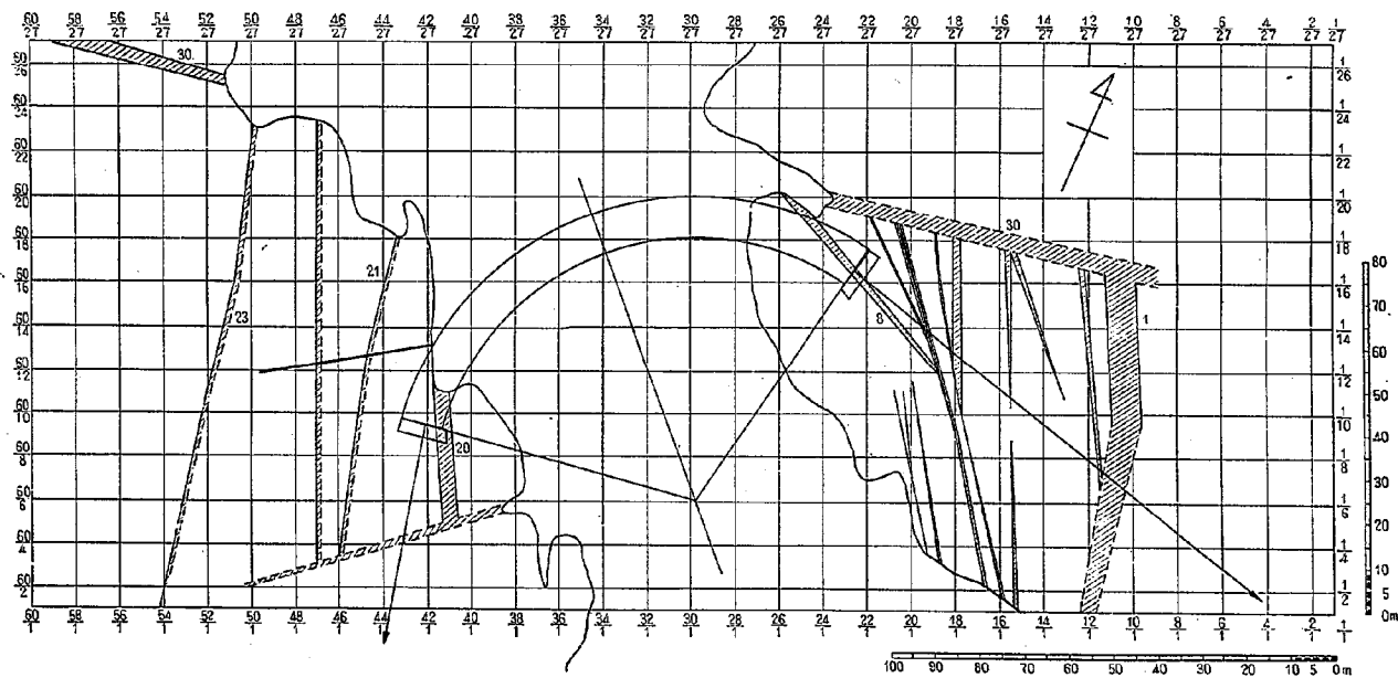
図-13 (d) 川俣ダムサイト水平地質断面図 (E.L.930m)
