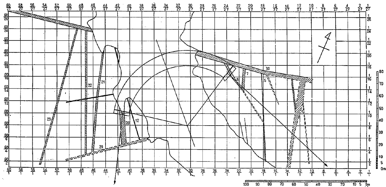
図-13(c) 川俣ダムサイト水平地質断面図 (E.L.910m)
