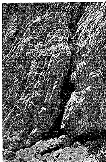
写真-4 左岸下流側 (中央の溝は断層(1)の河床部)
