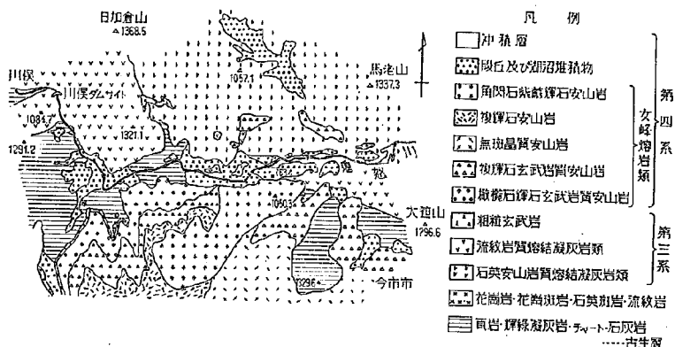
図-5 鬼怒川上流地域地質図
