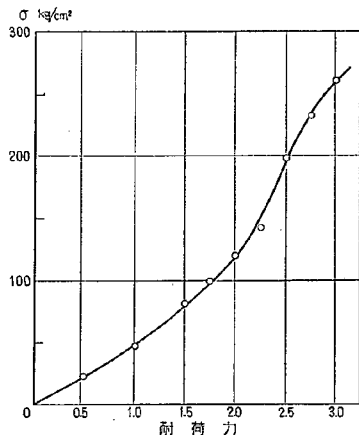
図-13 Wall 内の応力増加曲線
