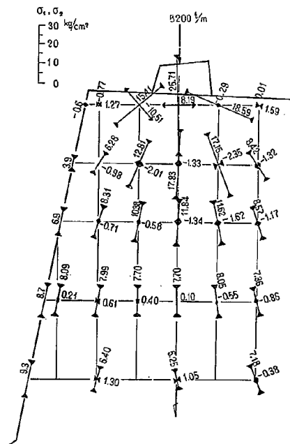
図-8 風化帯のない場合の主応力 (Aタイプ)
