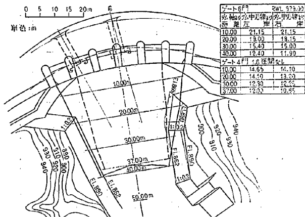
図-24 越流部落水 脈幅平面図
