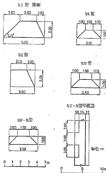
図-47 実験シル断面形状図(原寸)
