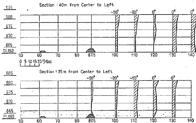
図-55(5) 水叩き内流速分布図 (R.W.L. 979.00 m Over lap)
