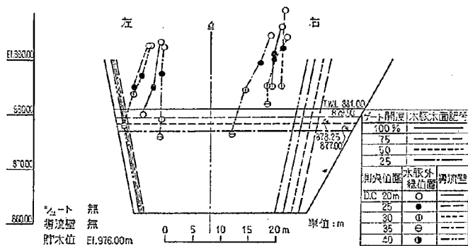
図-43 放水管水取外縁軌跡
