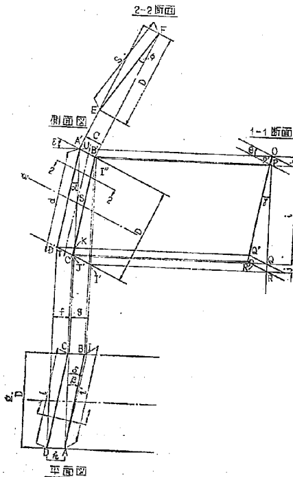
図-14 放水管呑口部設計記号説明図
