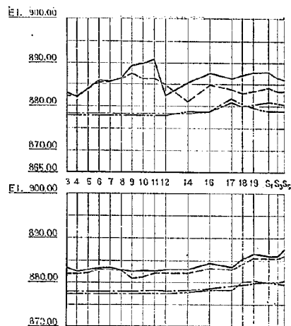
圖-57(13) 右岸側導流壁壓力分布圖
