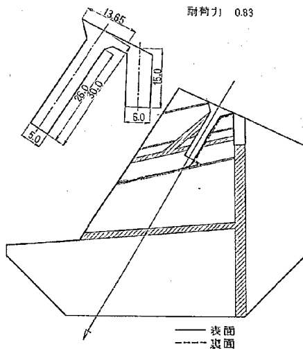
図-4 幅5m Wall入り模型の破壊状況
