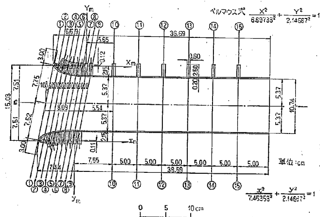
図-26 放水管模型図 (平面)
