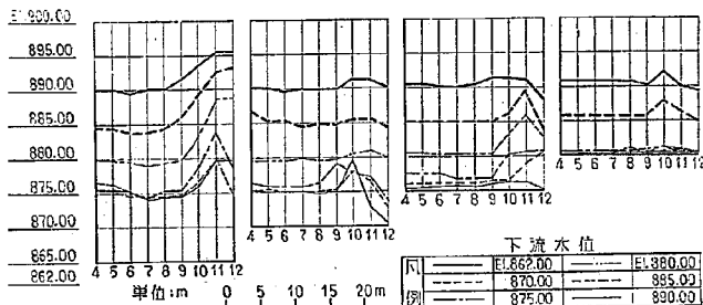
圖-10(9) 右岸側壁压力測定 縦断面 貯水位 EL. 979.00 m
