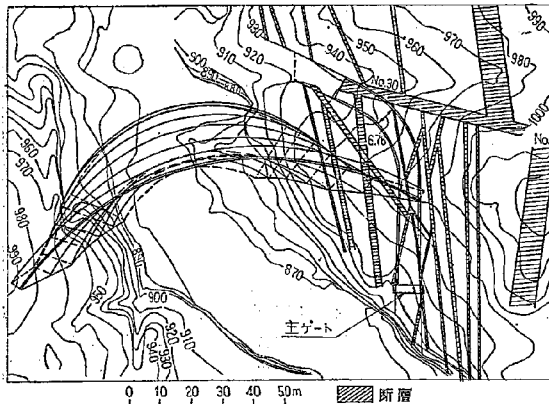
図-4 左岸トンネル余水吐案
