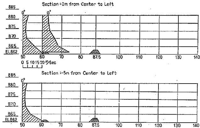
図-55(1) 水叩き内流速分布図 (R. W. L. 979.00 m Over lap)
