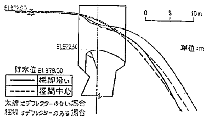
図-22 越流水面形状
