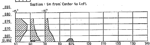
図-54(2) 水叩き内流速分布図 (R. W. L. 976.00 m 放水管 2 門)
