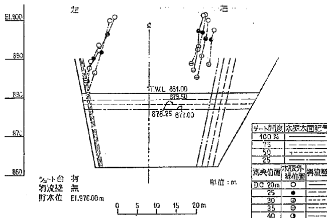
図-39 放水管水脈外縁軌跡
