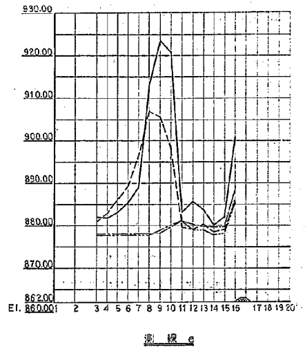
図-57(2) 水叩き面圧力分布図
