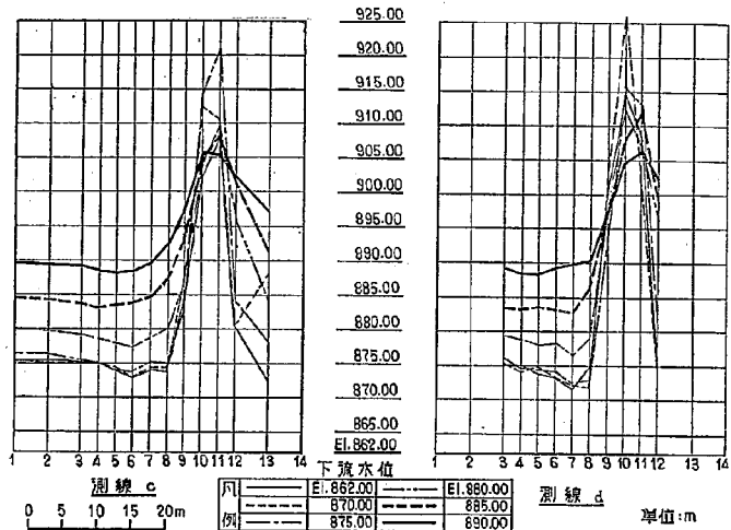
図-10(2) 水叩面圧力測定縦断面 貯水位 El. 979.00 m
