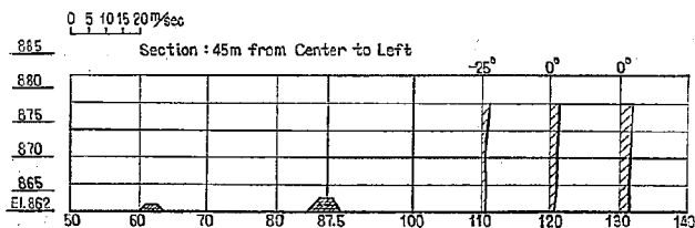
図-54(6) 水叩き内流速分布図 (R. W. L. 976.00 m 放水管 2 門)
