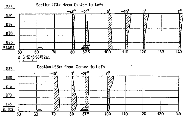
図-55(4) 水叩き内流速分布図 (R.W.L. 979.00 m Over lap)
