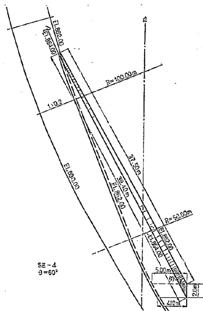
図-46(3) シルデフレクター形状
