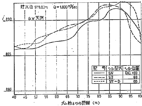
図-49 右岸導流壁沿い水面形状
