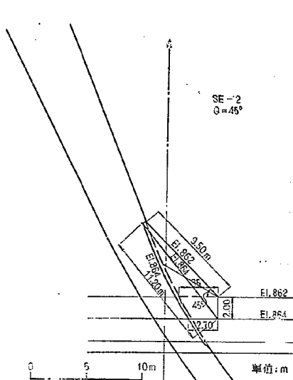
図-46(1) シルデフレクター形状
