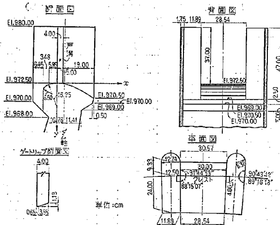
図-19 越流部模型形状図
