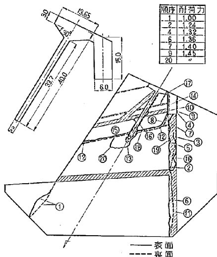
図-5 幅2m Wall入り模型の破壊状況
