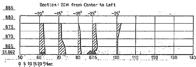
図-54(2) 水叩き内流速分布図 (R. W. L. 976.00 m 放水管 2 門)
