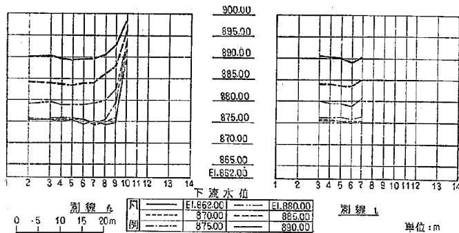
圖-10(6) 水叩面压力測定 縦断面 貯水位 EL. 979.00 m
