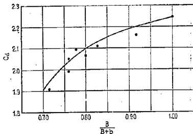
図-6 標準型越流部 C_d \sim B/(B+b) 関係
