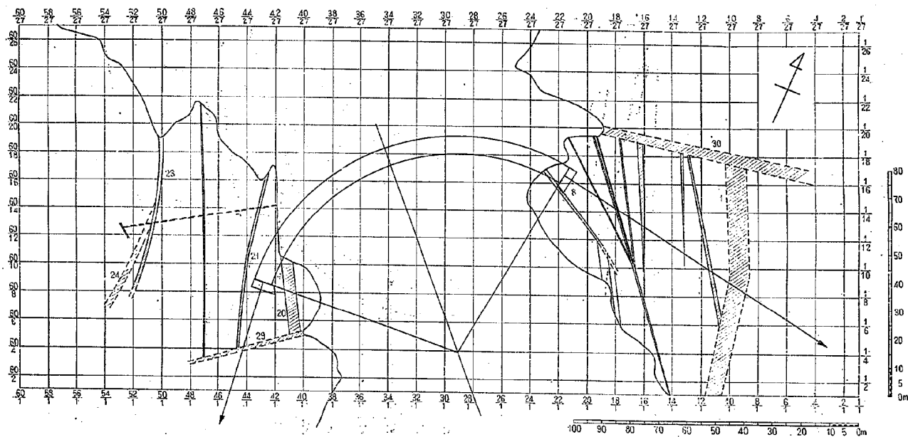
図-13 (e) 川俣ダムサイト水平地質断面図 (E.L.950m)
