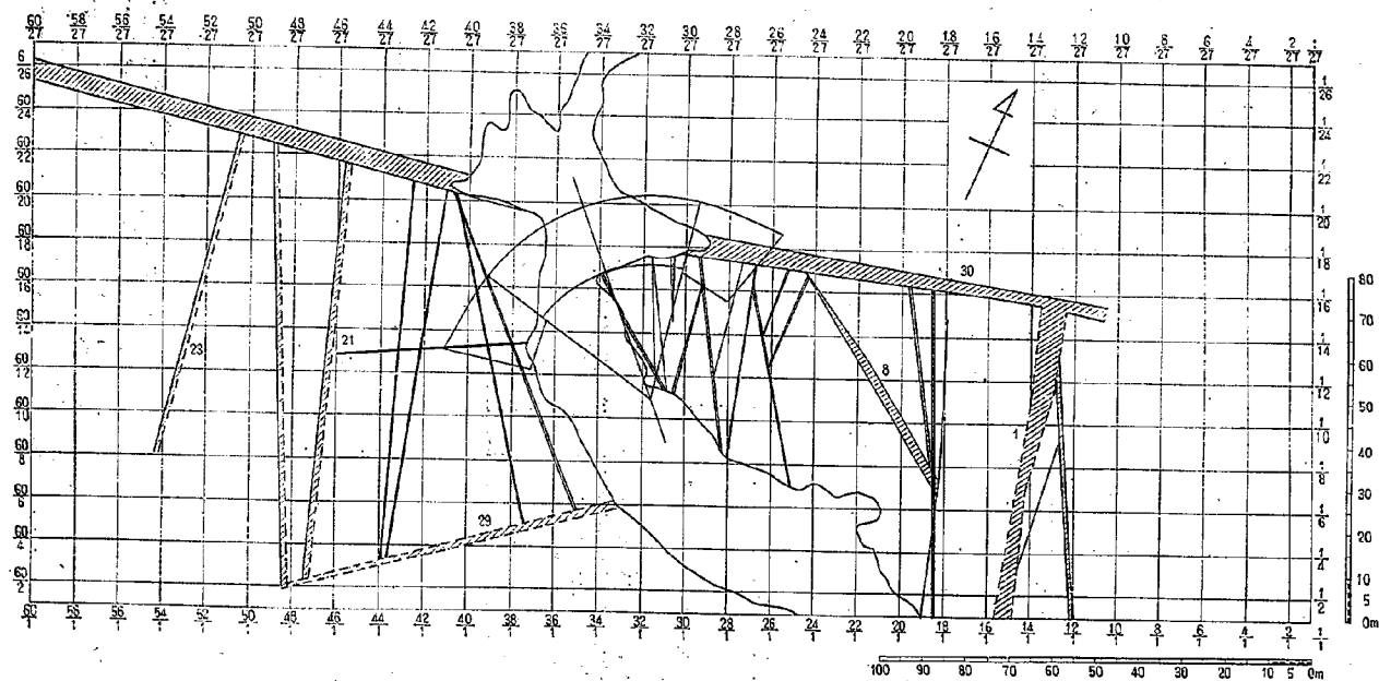
図-13 (a) 川俣ダムサイト水平地質断面図 (E.L.870m)
