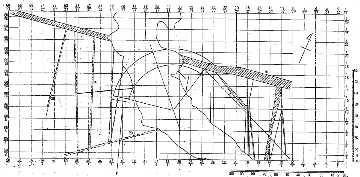
図-13 (b) 川俣ダムサイト水平地質断面図 (E.L.890m)
