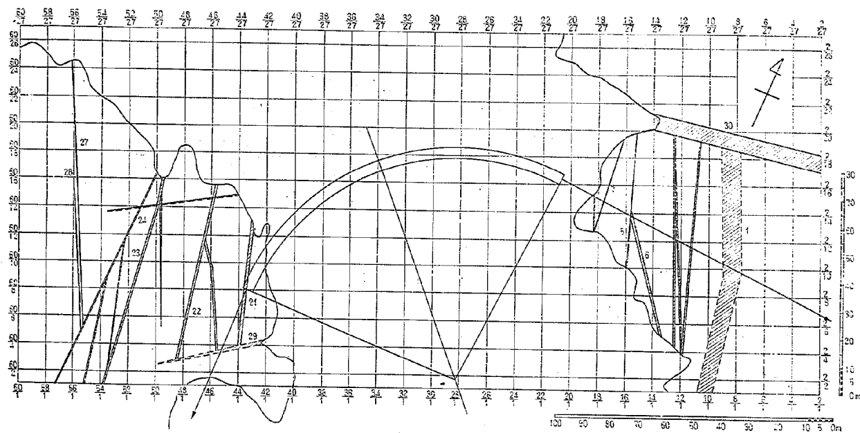
図-13 (f) 川俣ダムサイト水平地質断面図 (E L. 970m)
