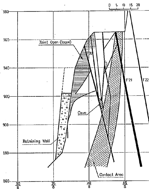
図-13 (h) 地質垂直断面図 (右岸アバットメント)
