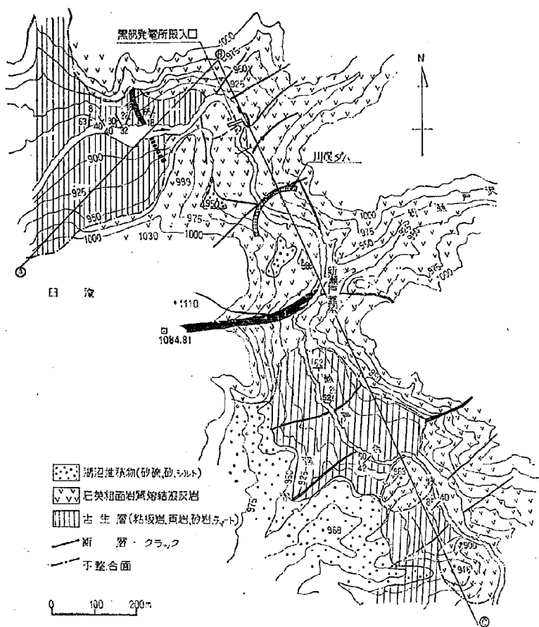
図-6 川俣ダム予定地点地質図
