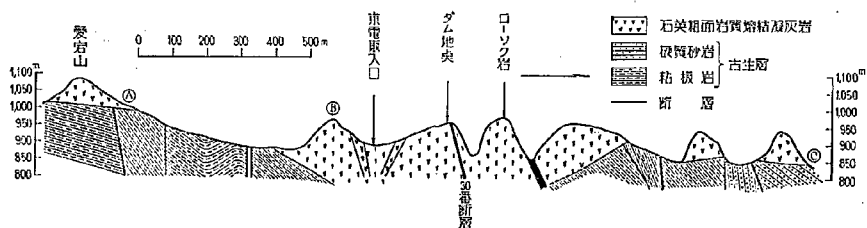
図-7 川俣ダム予定地点地質断面図
