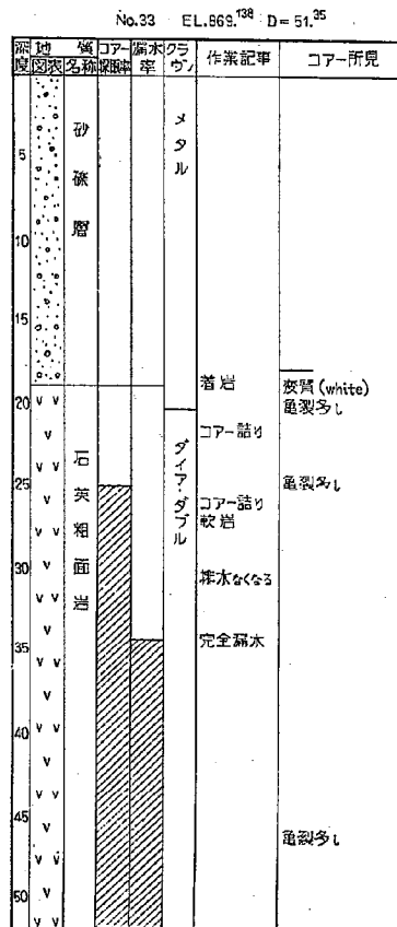
図-12(4) 川俣ダムサイトボーリング柱状図
