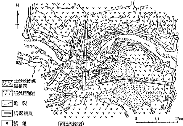
図-2 川俣ダムサイト地質図
