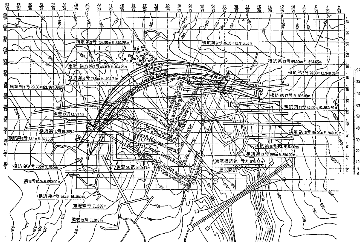
図-10 川俣ダムサイト地質調査箇所位置図
