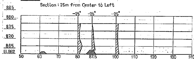
図-54(5) 水叩き内流速分布図 (R. W. L. 976.00 m 放水管 2 門)
