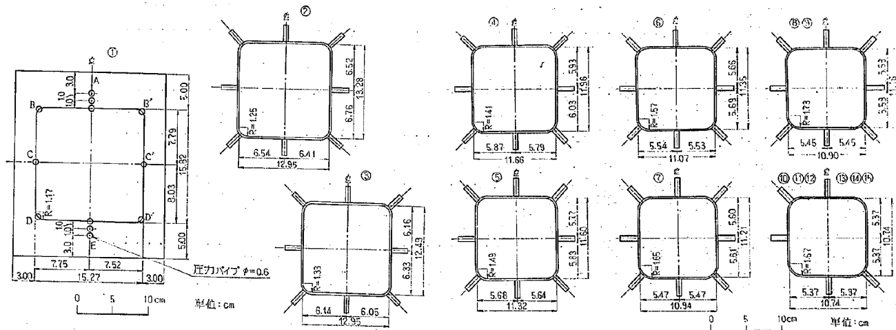
図-27 放水管模型図(断面)
