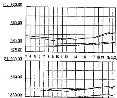
圖-57(14) 右岸側導流壁壓力分布圖
