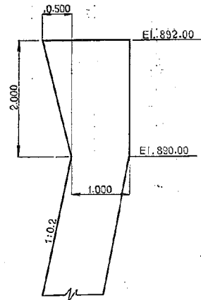
図-51 波がえし
