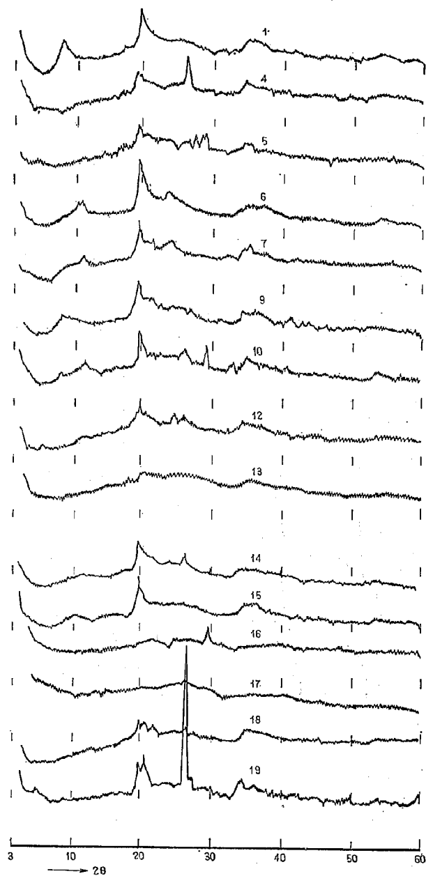
図-17 土壤コロイドのX線回折図 (群馬県路床土)
