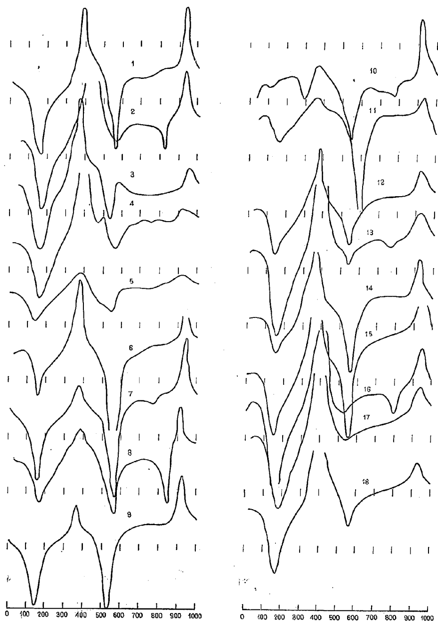
図-18 土壌コロイドの DTA 曲線 (群馬県路床土)
