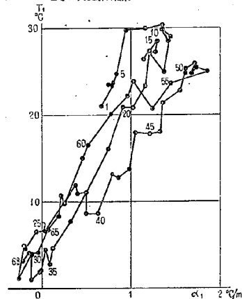
図-4.20 綾北ダム T_1 と等置直線温度こう配 \alpha_1 の相関図
