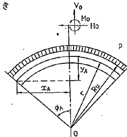
図-5.14 (2) 簡易荷重分割計算説明図
