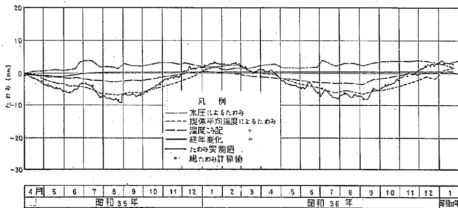
図-5.2 (4) 綾北ダム中間標高たわみの実測解析図
