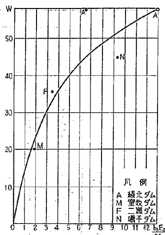
図-5.16 水圧による換算たわみ \delta_0 と形状因子 W との関係
