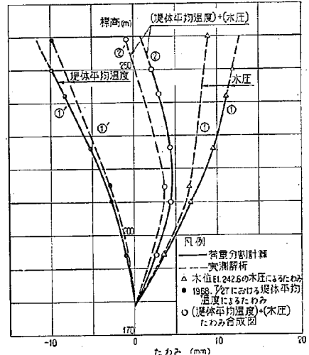
図-5.19 鳴子ダムの水压および堤体平均温度によるたわみおよびその合成図(荷重分割計算比較図)
