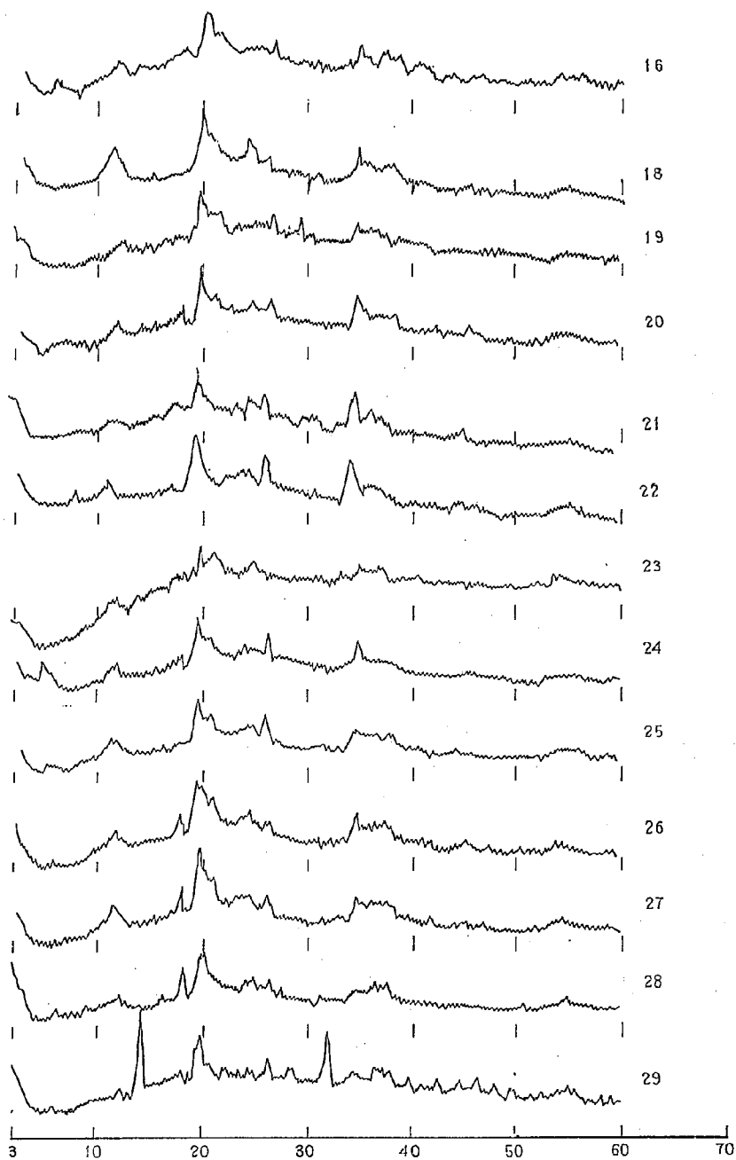
図-21 (2) 土壤コロイドのX線回折図 (三重県路床土)
