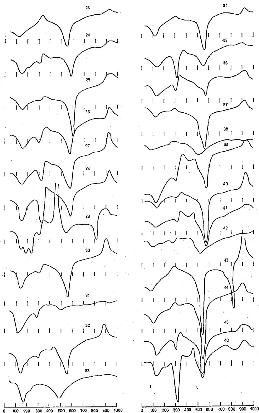
図-22 (2) 土壌コロイドの DTA 曲線 (三重県路床土)
