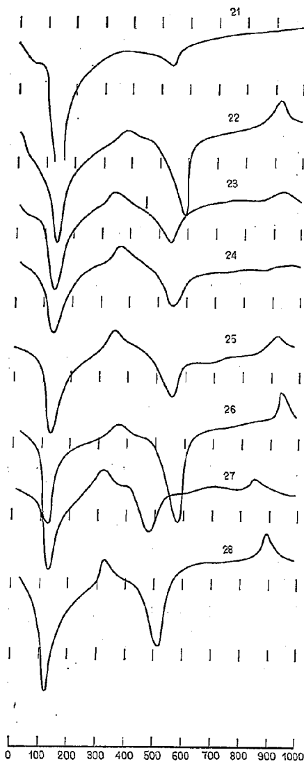
図-32 (2) 土壌コロイドの DTA 曲線 (福島県路床土)
