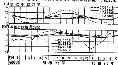
図-4.14 二瀬ダム堤体平均温度，等置直線温度こう配変動図
