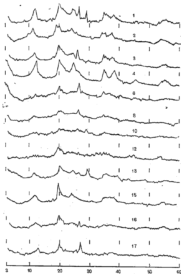
図-24 土壤コロイドのX線回折図 (愛知県路床土)
