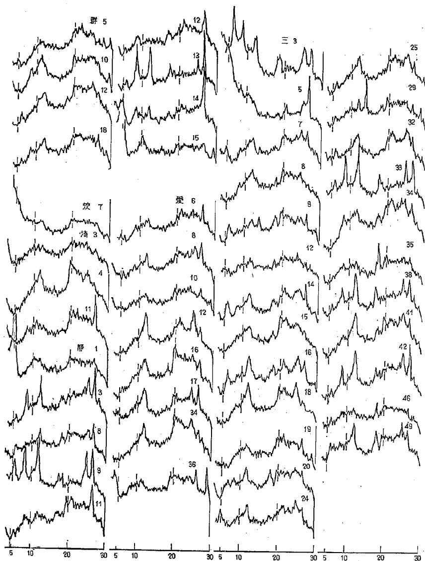
図-23 エチレングライコール処理粘土のX線回折図
