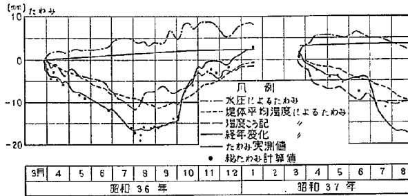
図-5.4 (1) 室牧ダムのたわみの実測解析図
