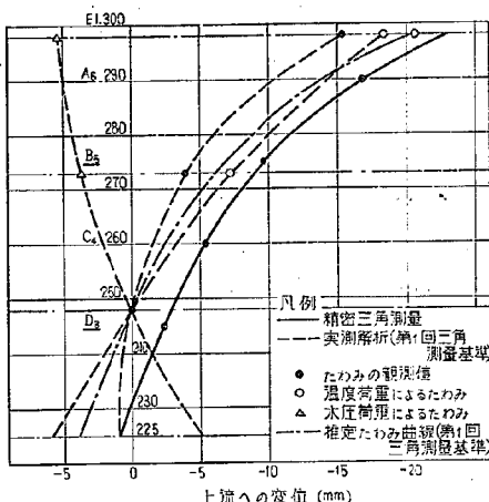
図-5.21 綾北ダムのたわみ曲線
