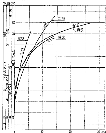
図-5.11 水位～水圧によるたわみ曲線
