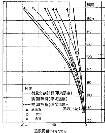
図-5.18 鳴子ダムの温度荷重によるたわみ(荷重分割計算比較図)
