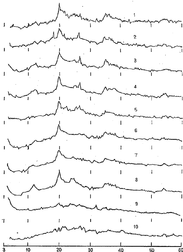
図-33 土壌コロイドのX線回折図(岩手県路床土)
