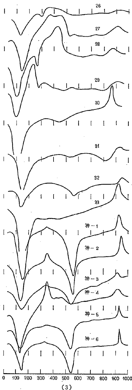
図-12 土壤コロイドの DTA 曲線 (東京都路床土, 神奈川県路床土)
