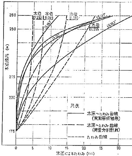
図-5.10 鳴子ダム水位～水圧によるたわみ曲線 クラウンたわみ曲線
