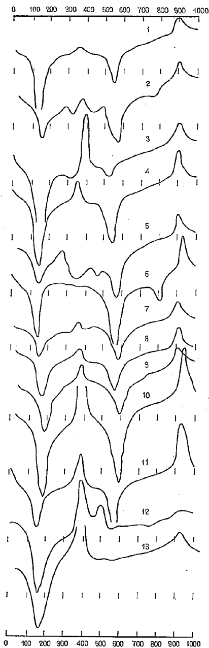
図-20 土壤コロイドのDTA曲線(茨城県路床土)
