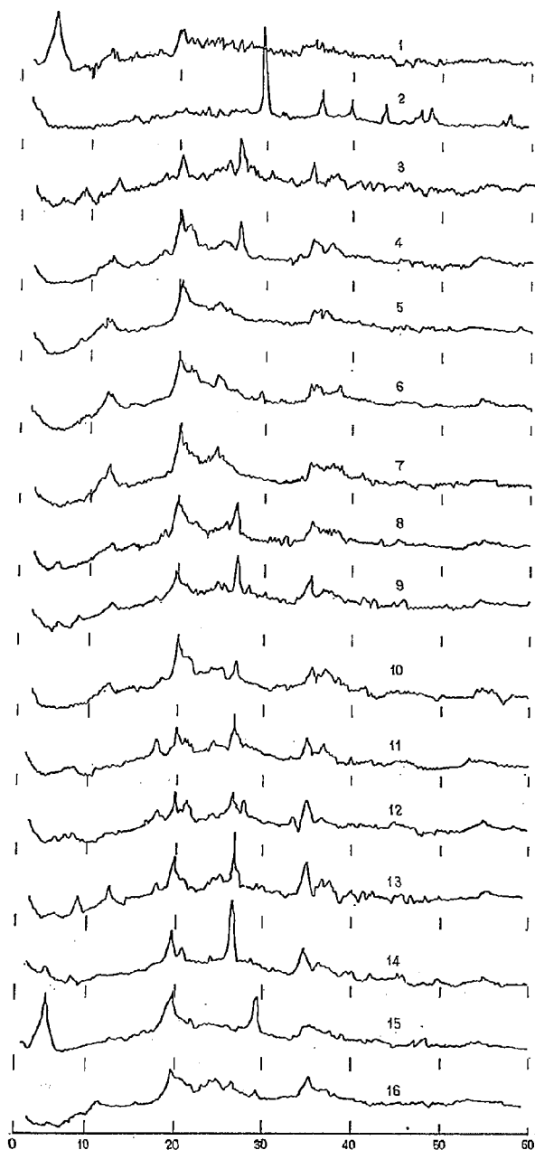
図-26 土壌コロイドのX線回折図 (静岡県路床土)
