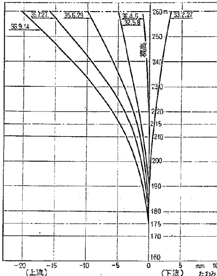
図-5.13 鳴子ダムの温度荷重によるたわみの変動
