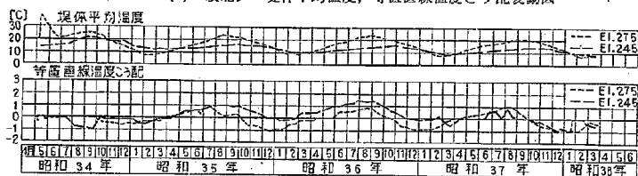
図-4.12 (2) 綾北ダム右岸堤体平均温度，等置直線温度こう配変動図
