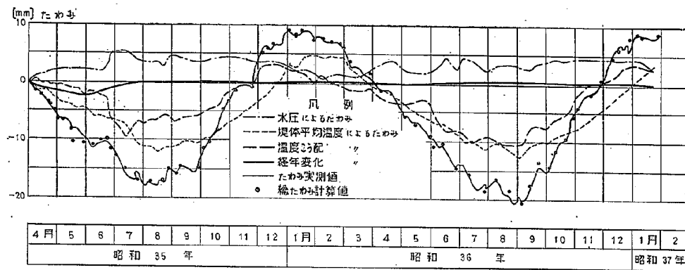
図-5.2 (1) 綾北ダム実測解析図
