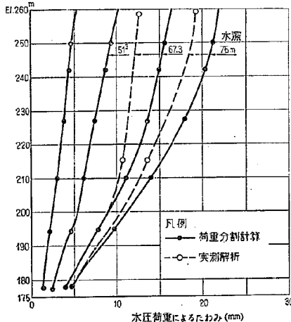
図-5.17 鳴子ダムの水压荷重によるたわみ(荷重分割計算比較図)
