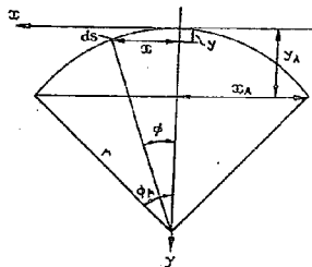
図-5.14(3) 簡易荷重分割計算説明図 (アーチ形状)
