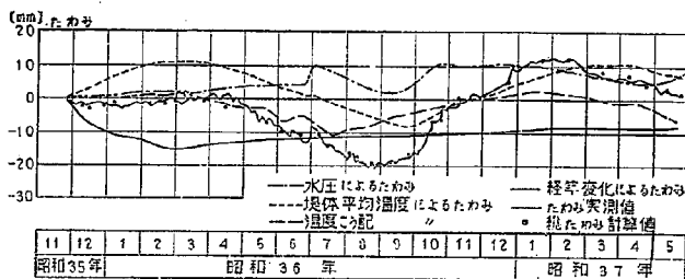
図-5.6 二瀬ダムのたわみの実測解析図
