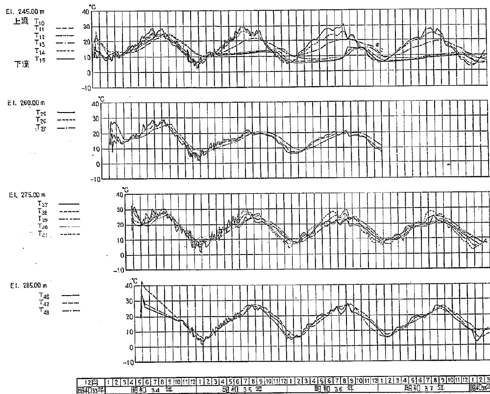
図-4.3 綾北ダム堤体温度変動図
