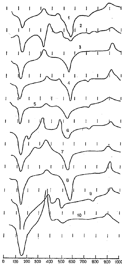
図-34 土壤コロイドの DTA 曲線 (岩手県路床土)
