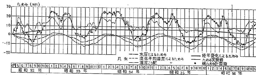
図-5.8 (1) 鳴子ダムのたわみの実測解析図
