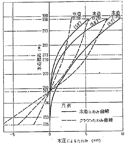
図-5.9 綾北ダム水位～たわみ曲線、クラウンたわみ曲線
