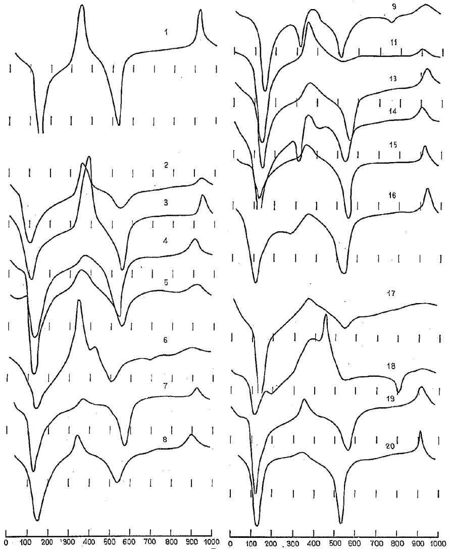
図-32 (1) 土壌コロイドの DTA 曲線 (福島県路床土)
