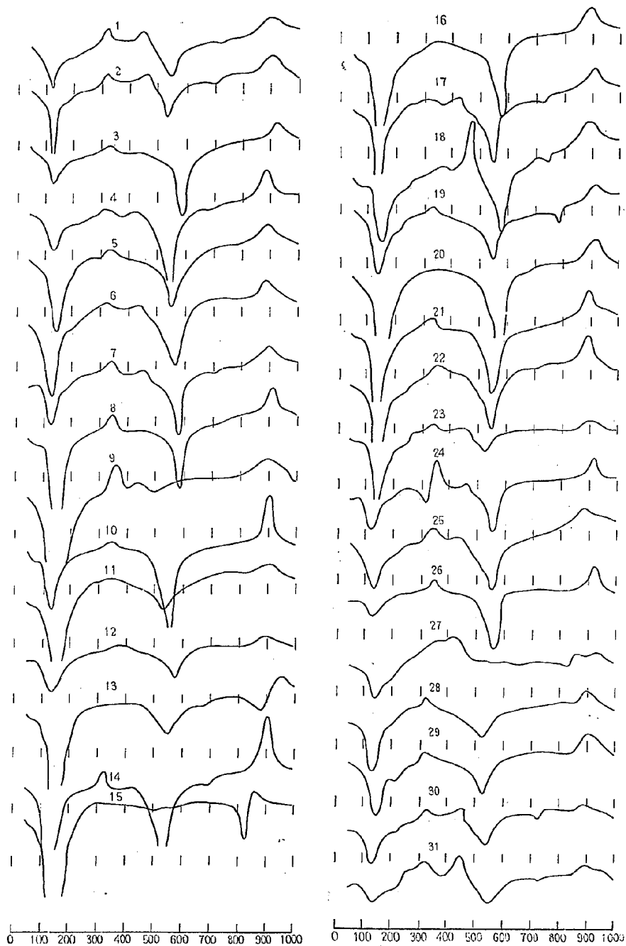
図-29 (1) 土壤コロイドのDTA曲線(宮城県床土)
