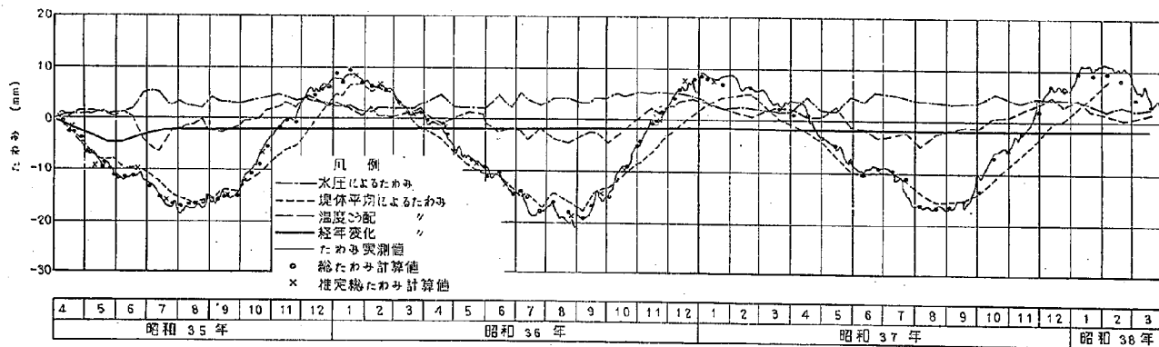
図-5.2 (2) 綾北ダムたわみの実測解析図
