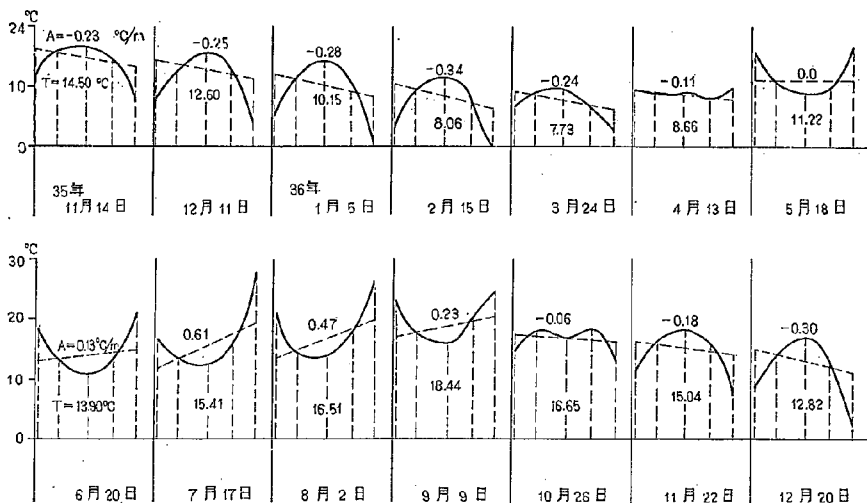
図-4.18 二瀬ダム半径方向温度分布変動図 (Bl. 515m クラウンカンティレバー)
