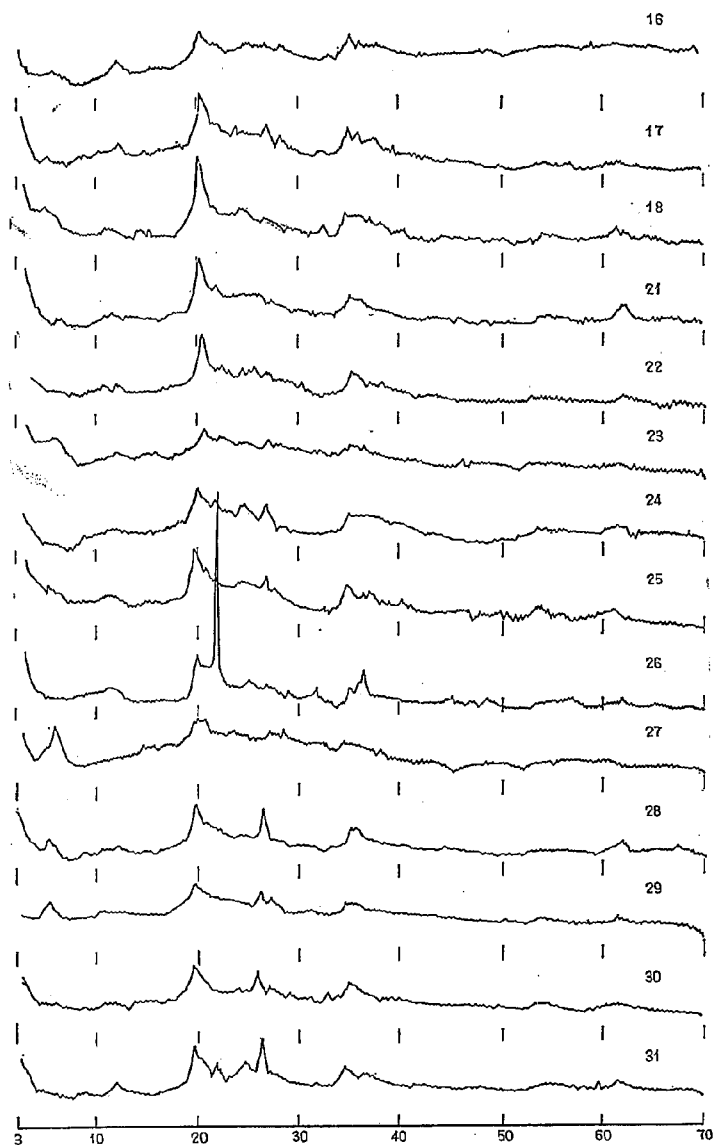
図-28 (2) 土壌コロイドのX線回折図 (宮城県路床土)
