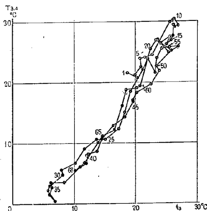
図-4.19 綾北ダム T_{3.4} と堤体平均温度 t_3 の相関図
