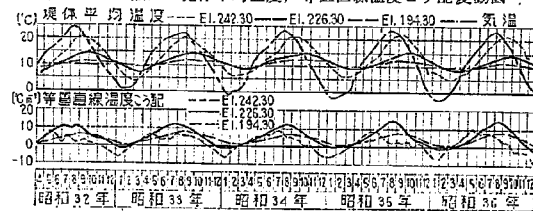
図-4.15 鴫子ダム堤体平均温度，等置直線温度こう配変動図
