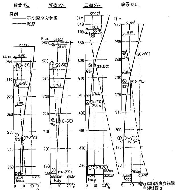
図-4.16 クラウンキャンティレバー断面における堤体平均温度変動幅分布図
