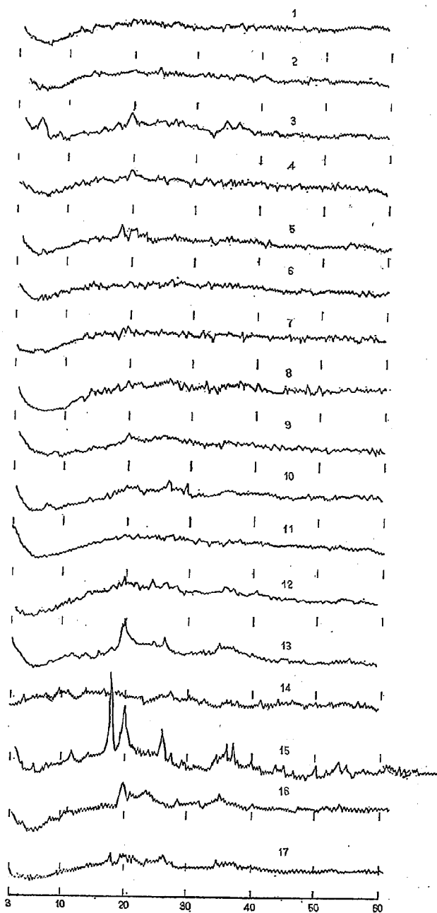
図-11 土壌コロイドのX線回折図（東京都路床土，神奈川県路床土）
