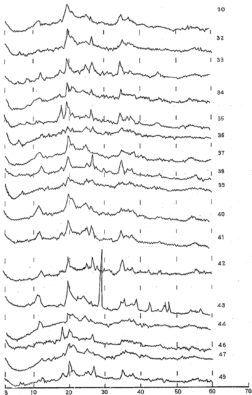
図-21 (3) 土壌コロイドのX線回折図 (三重県路床土)
