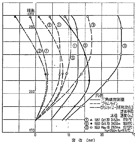
図-5.20 鳴子ダムたわみ曲線
