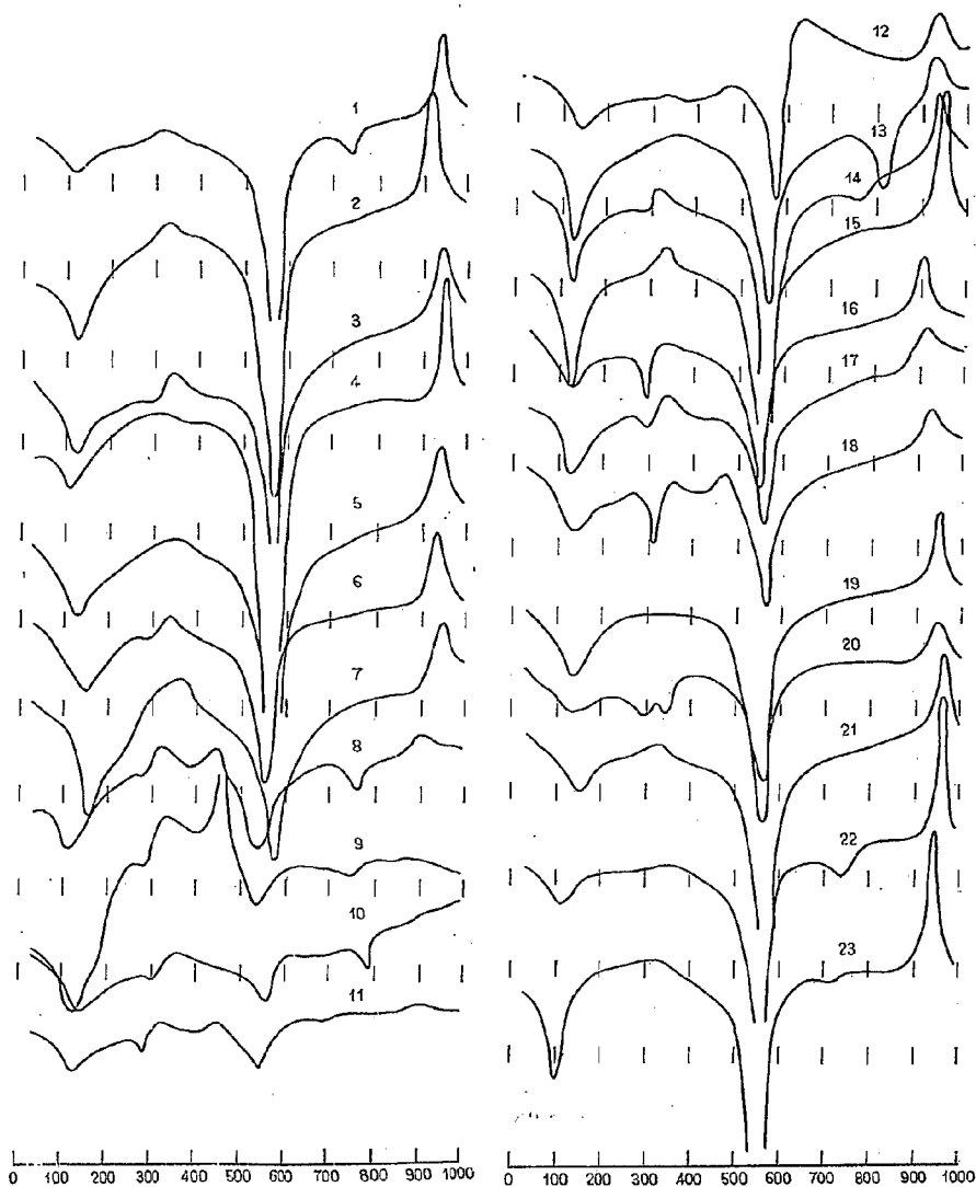
図-25 (1) 土壌コロイドの DTA 曲線 (愛知県路床土)
