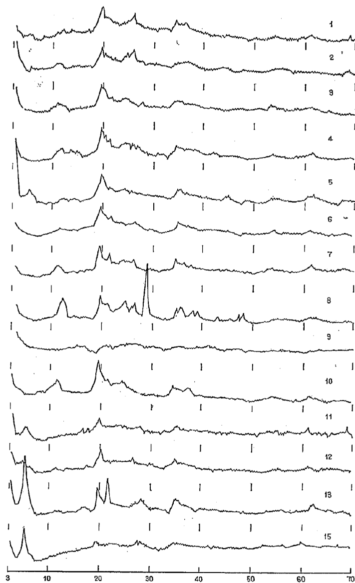
図-28(1) 土壌コロイドのX線回折図(宮城県路床土)
