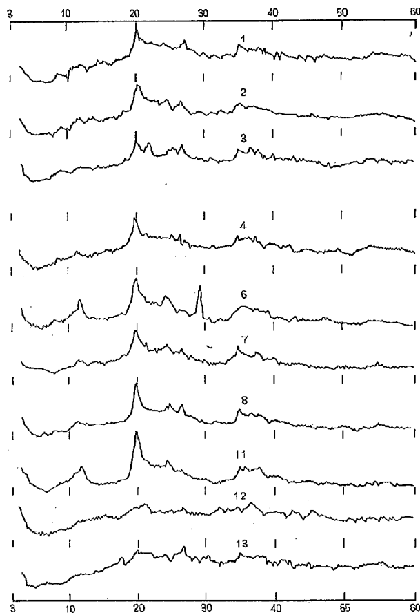
図-19 土壌コロイドのX線回折図 (茨城県路床土)
