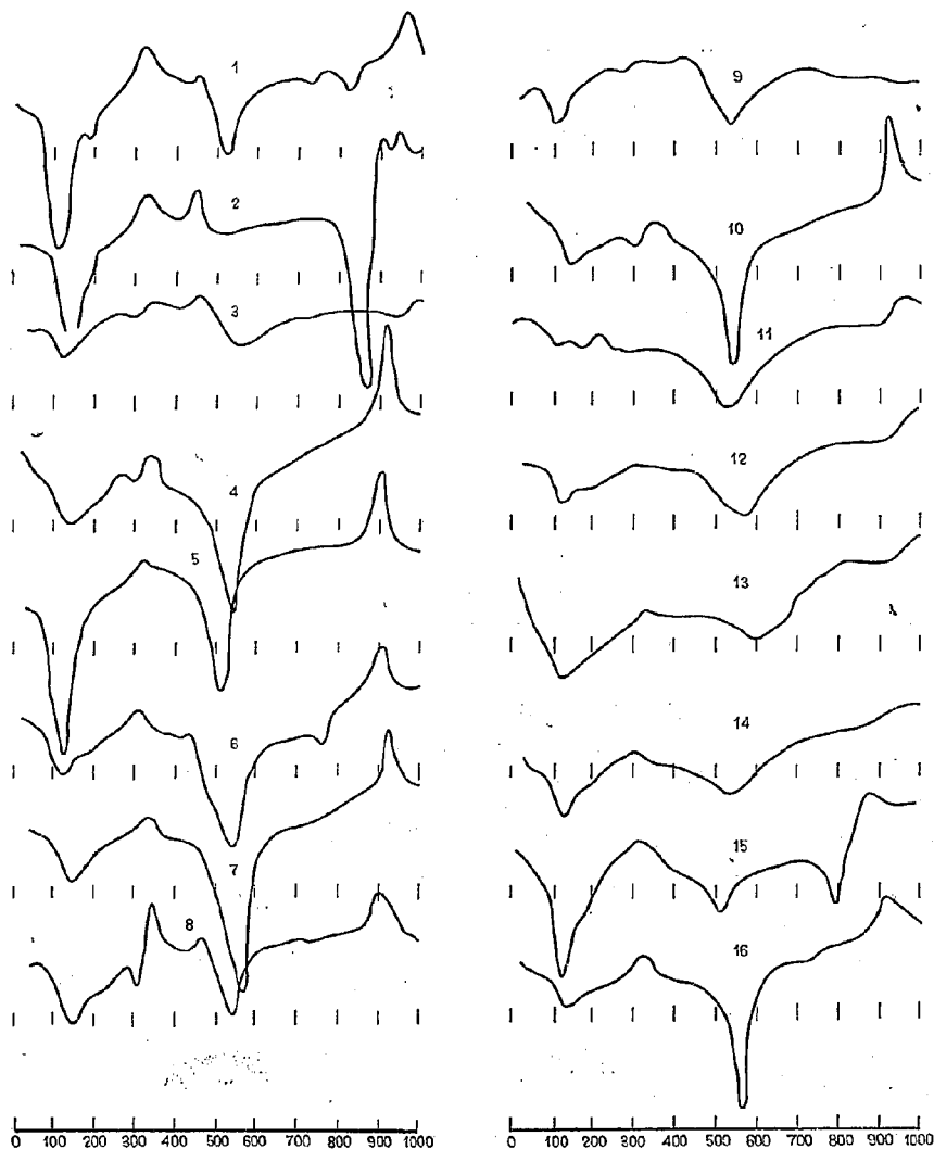
図-27 土壌コロイドの DTA 曲線 (静岡県路床土)
