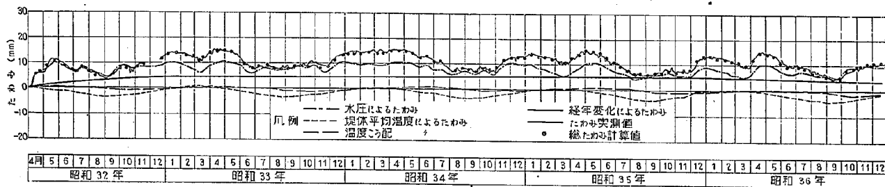
図-5.8 (2) 鳴子ダムの中間標高のたわみの実測解析図
