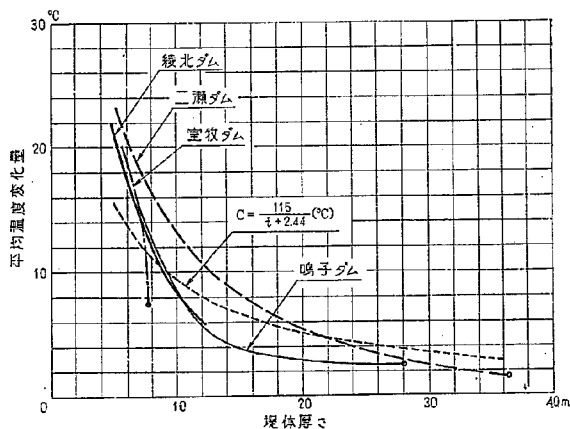
図-4.17 堤体厚さと平均温度変化量との関係
