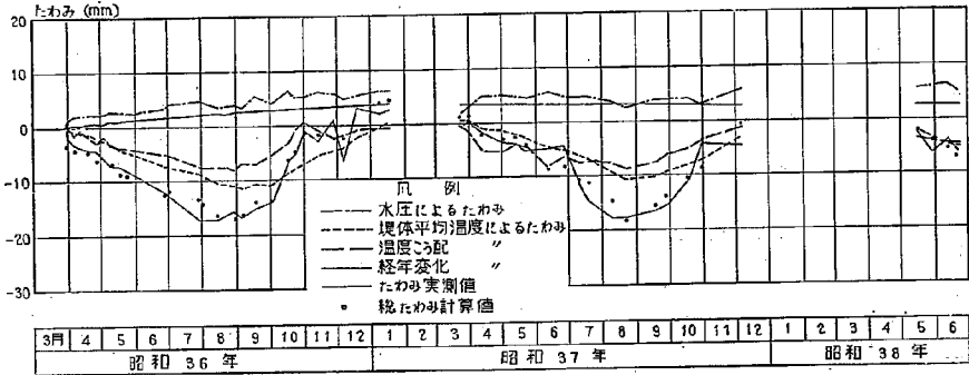
図-5.4 (2) 室牧ダムのたわみの実測解析図
