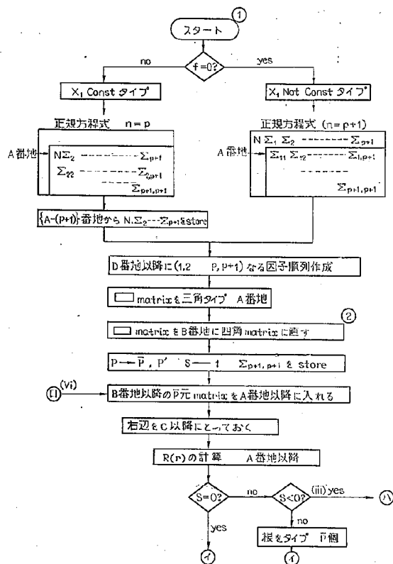
図-2.1 多変量解析フローチャート
