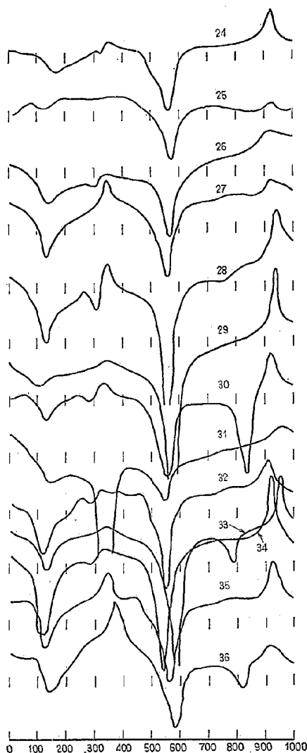
図-25 (2) 土壌コロイドのDTA曲線(愛媛県路床土)
