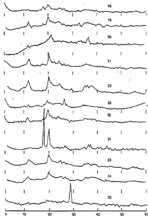
図-24 土壤コロイドのX線回折図 (愛知県路床土)
