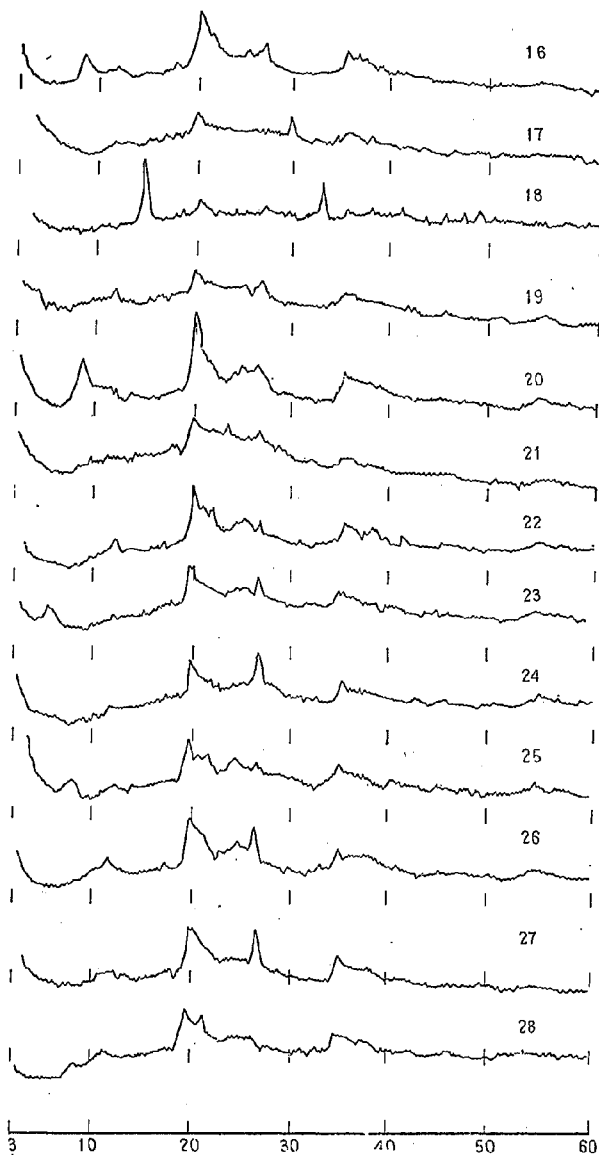
図-31(2) 土壌コロイドのX線回折図(福島県路床土)
