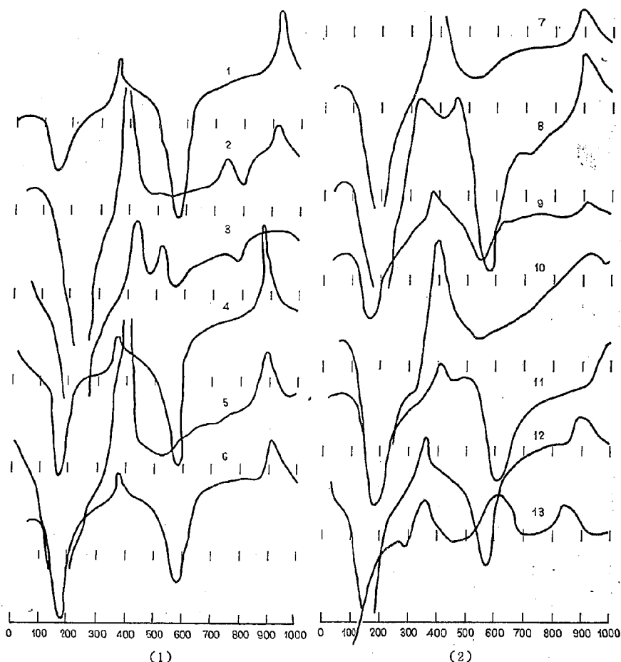
図-16 土壤コロイドの DTA 曲線 (埼玉県路床土)
