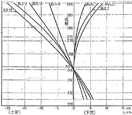
図-5.12 綾北ダムの温度荷重によるたわみの変動
