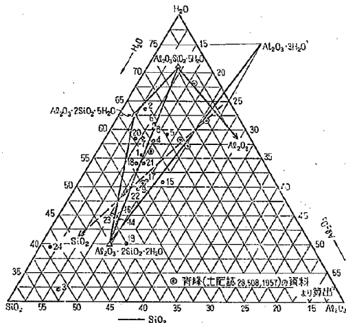
図-14 \text{Al}_2\text{O}_3\text{-SiO}_2\text{-(H}_2\text{O)}^+ 三成分系図
