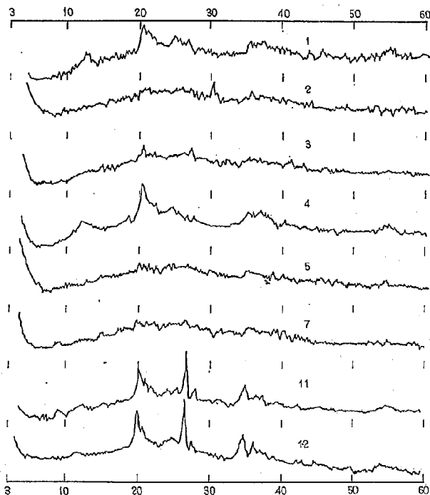
図-15 土壌コロイドのX線回折図 (埼玉黒路床土)
