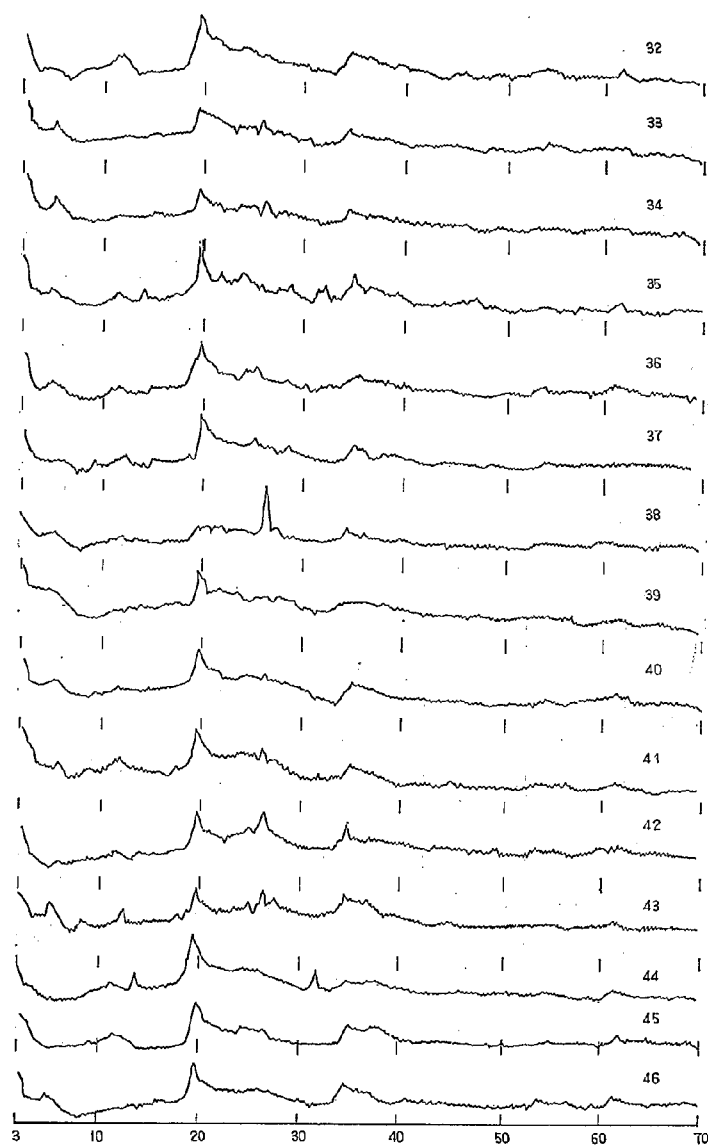
図-28 (3) 土壌コライトのX線回折図 (宮城県路床土)
