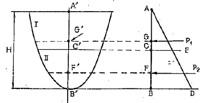
図-5.14 (1) 簡易荷重分割計算説明図 (水圧荷重)
