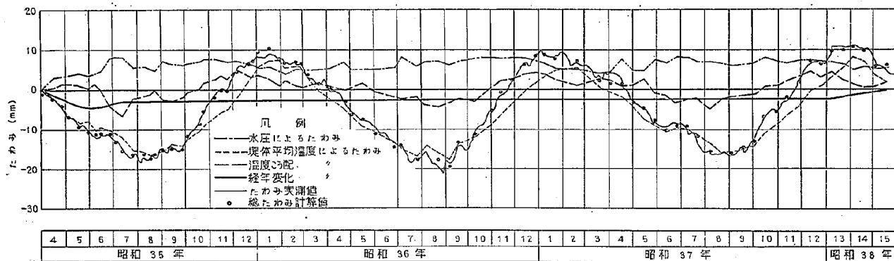
図-5.2 (3) 綾北ダムのたわみの実測解析図
