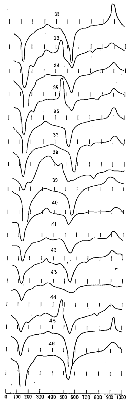
図-29 (2) 土壌コロイドのDTA曲線(宮城県路床土)
