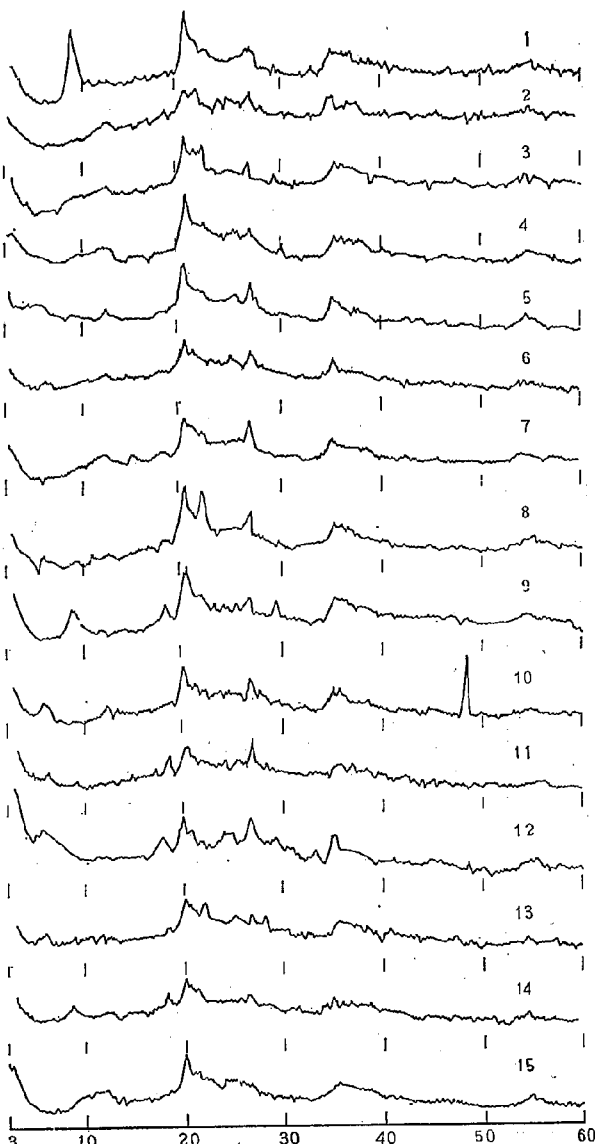
図-31 (1) 土壌コロイドのX線回折図 (福島県赤床土)
