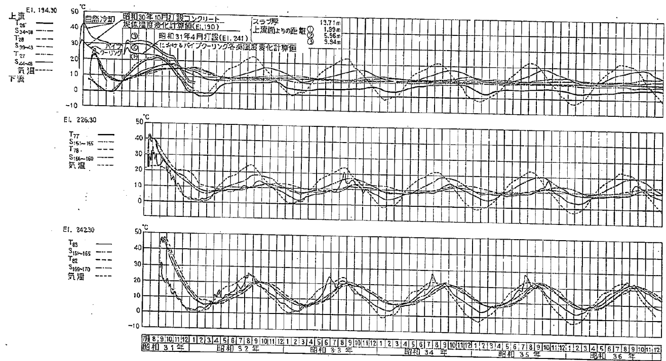
図-4.6 鳴子ダム堤体温度変動図
