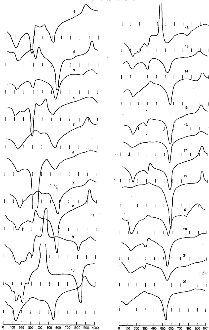
図-22 (1) 土壌コロイドの DTA 曲線 (三重県路床土)
