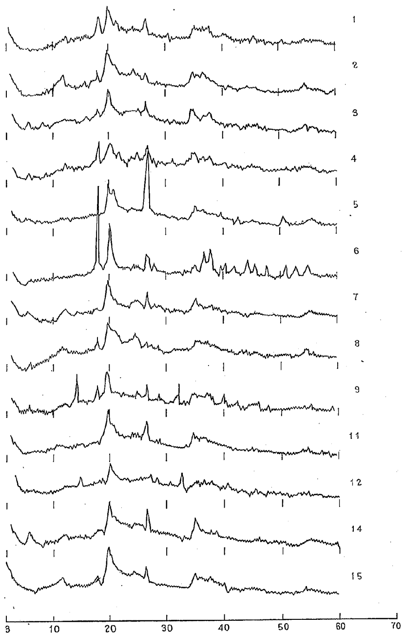
図-21 (1) 土壌コロイドのX線回折図 (三重県路床土)
