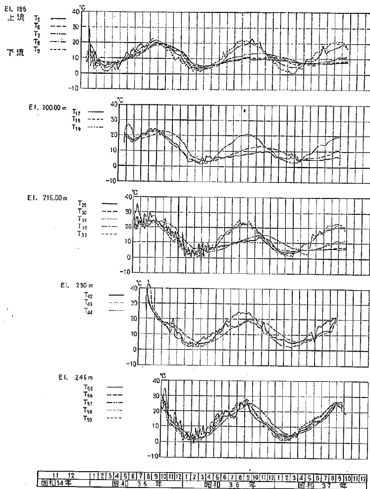
図-4.4 室牧ダム堤体温度変動図
