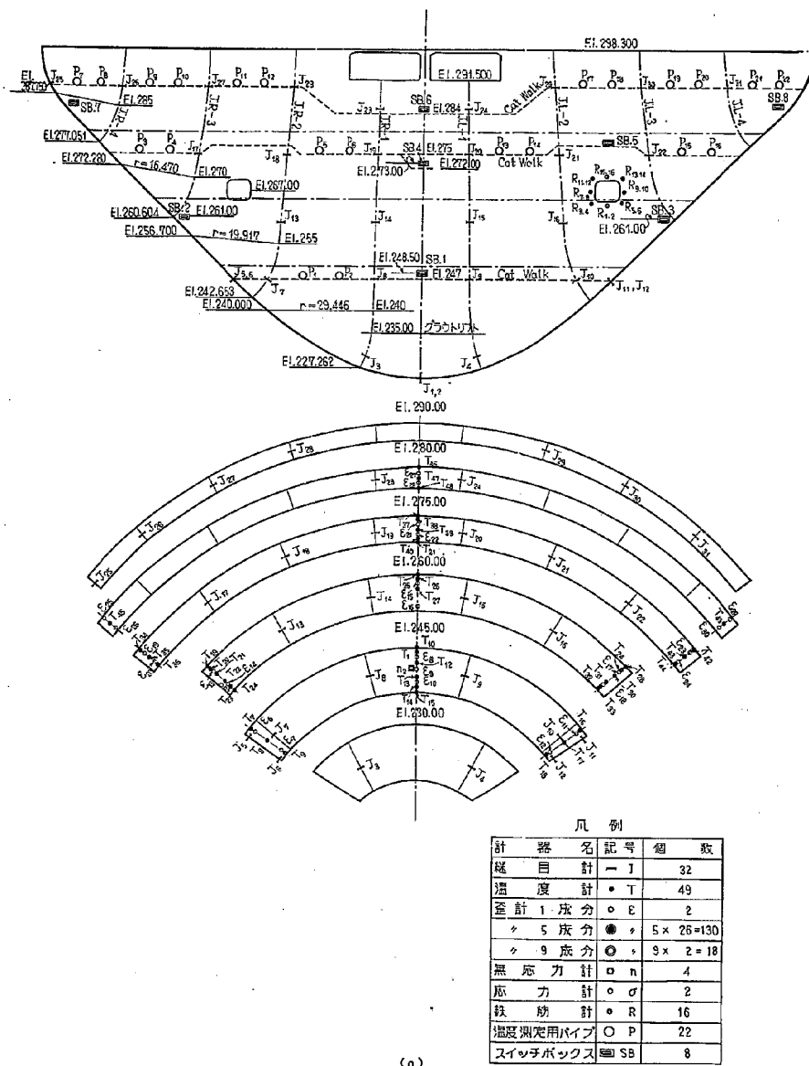
図-4.1(a) 綾北ダム計器埋込図
