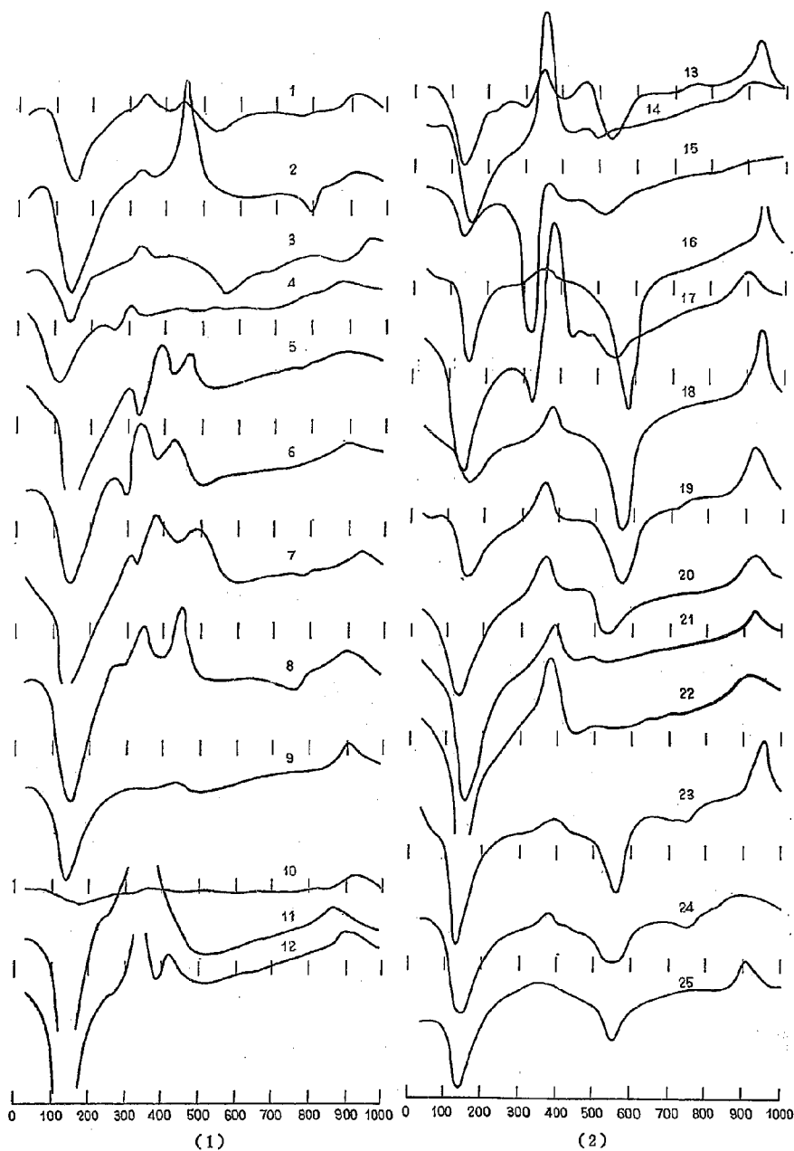
図-12 土壌コロイドのDTA曲線(東京都路床土, 神奈川県路床土)
