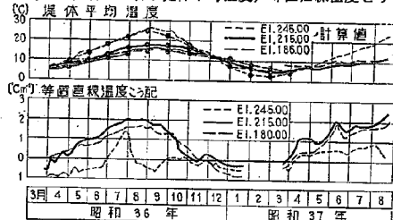
図-4.13 室牧ダム堤体平均温度，等置直線温度こう配変動図
