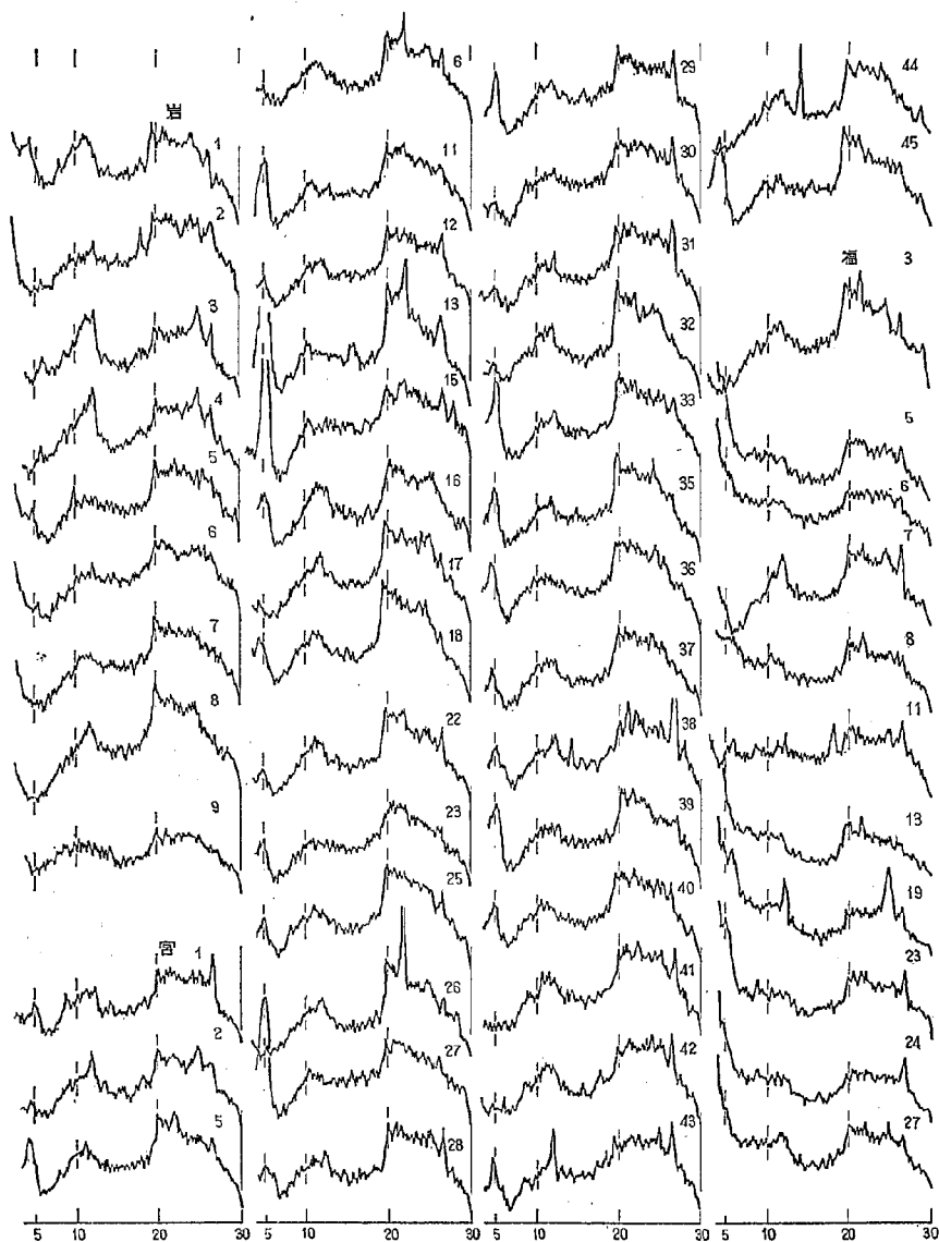
図-30 エチレングライコール処理粘土のX線回折図
