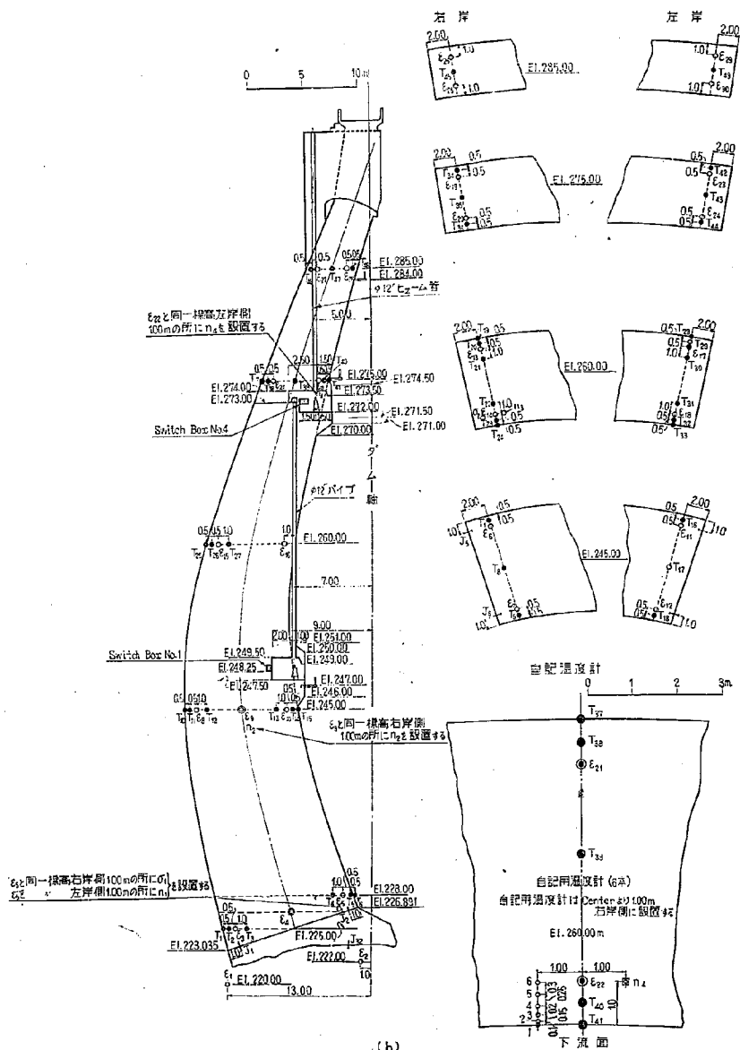
図-4.1(b) 綾北ダム計器埋込面
