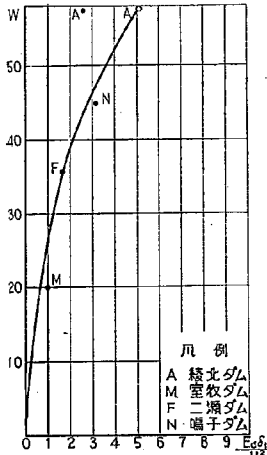
図-5.15 水圧による換算たわみ \delta_0 と形状因子 W との関係
