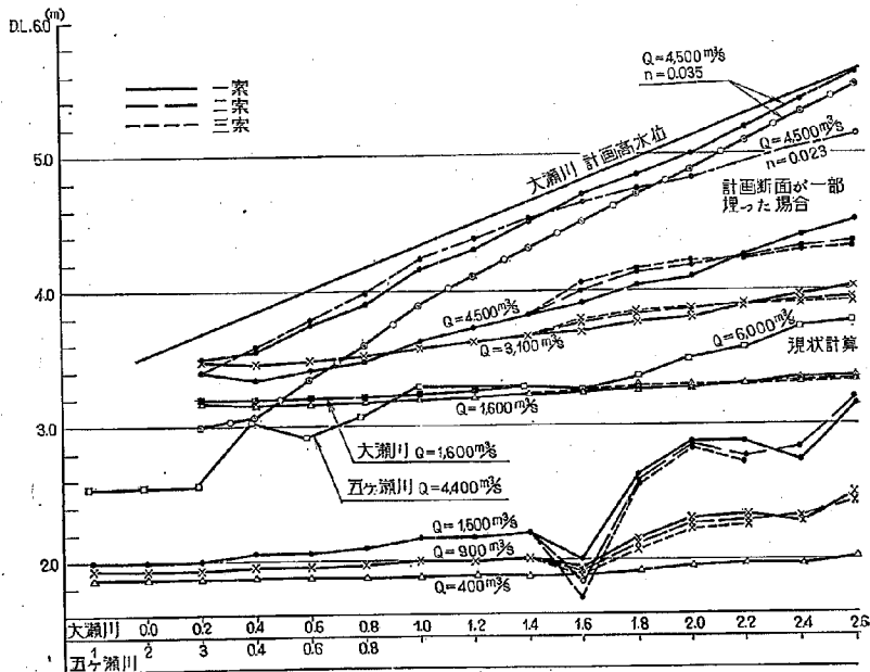
図-41 水位縦断面図
