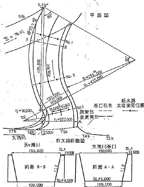
図-68 第3案新水路図
