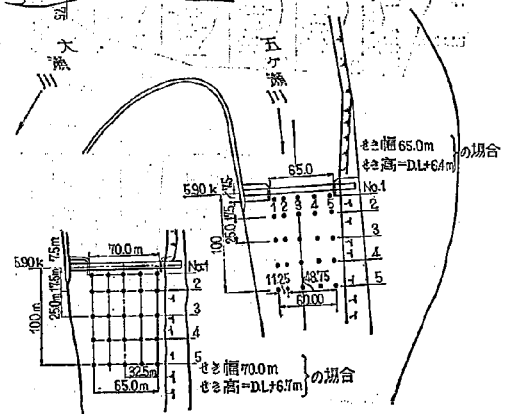
図-58 分流量せき下流速測定箇所図
