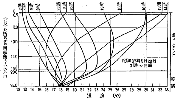
図-57 コンクリート版の深さ方向の温度変化の1例
