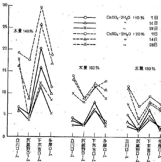
図-18 関東ローム層別のモルタル強度 ( \text{Ca}(\text{OH})_2 20%)
