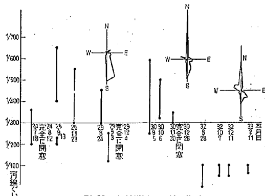
図-28 大瀬川河口洲開口状況
