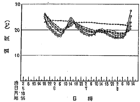
図-4 雨が続いた場合のコンクリート版の温度変化の1例(Ⅱ型)
