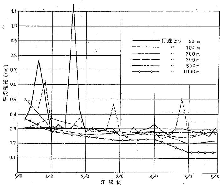
図-10 海底砂の平均粒径 (昭和35年12月21日観測)
