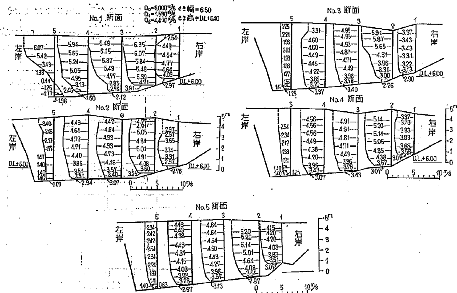
図-59(1) 第1案㊟せきの場合の流速分布図
