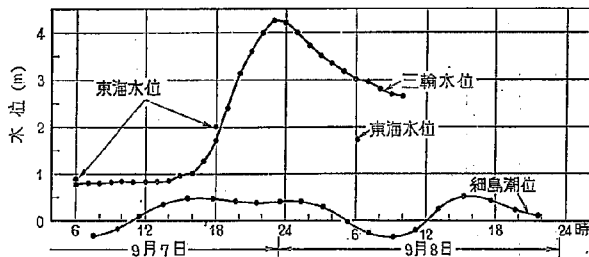
図-33 昭和29年13号台風水位曲線
