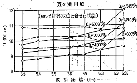
図-55 第1案①せき水位縦断面
