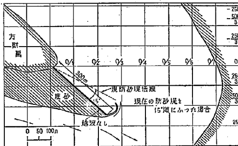
図-20(4) 防砂堤改良案2 堆砂状況 (SSE 波)
