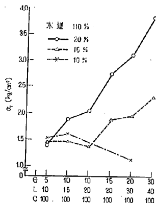
図-20 立川ロームに \text{Ca}(\text{OH})_2 — \text{CaSO}_4 \cdot 2\text{H}_2\text{O} —セメントを添加した場合の圧縮強度
