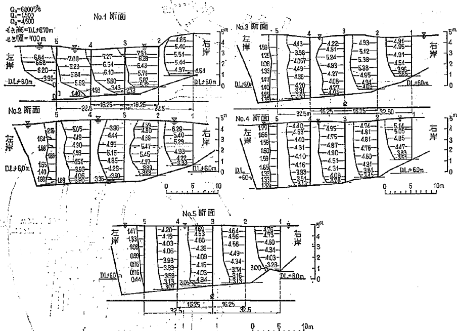
図-59(2) 第1案㊟せきの場合の流速分布図
