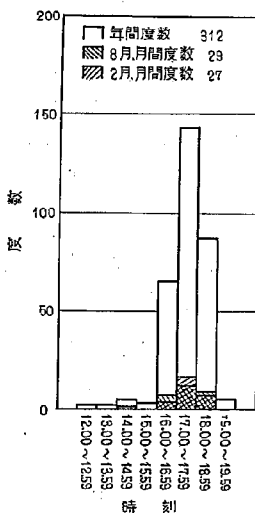
図-28 昭和36年4月～昭和37年3月1カ年間のコンクリート版底面の日最高温度時刻度数分布
