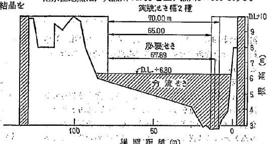
図-62 第 2 案分流せき
