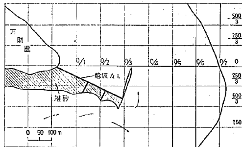
図-19(2) 防砂堤改良案1 堆砂状況 (SSE 波)
