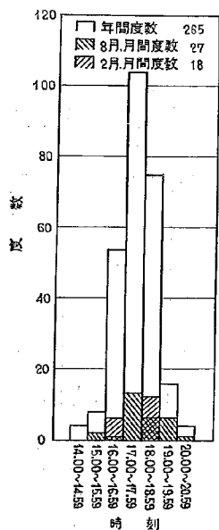
図-29 昭和37年4月～昭和38年3月1カ年間のコンクリート版底面の日最高温度時刻度数分布
