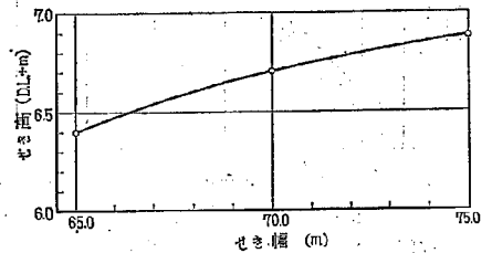
図-50 第1案分流量のせき高とせき幅の関係
