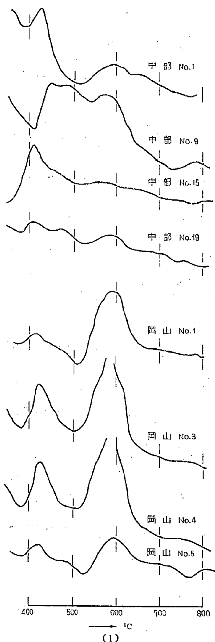
図-10 (1) ビベリンゲン処理粘土上の熱分析曲線
