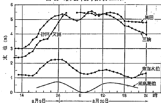
図-34 昭和32年7号台風水位曲線
