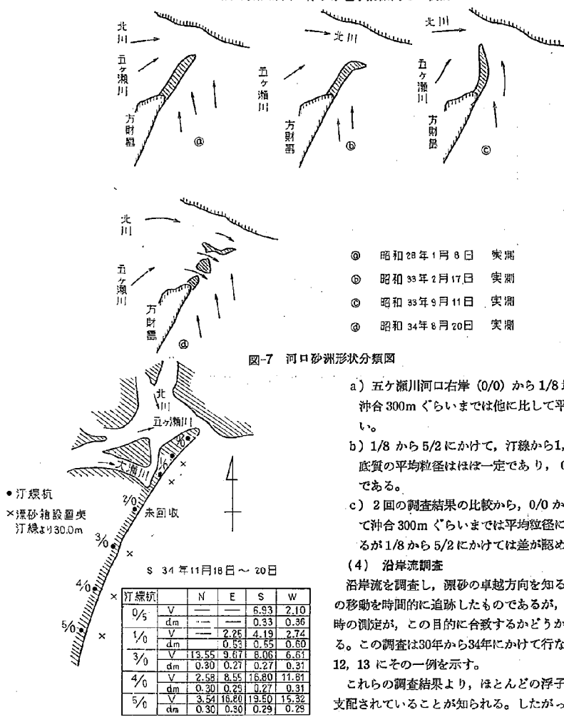
図-8 漂砂調査結果
