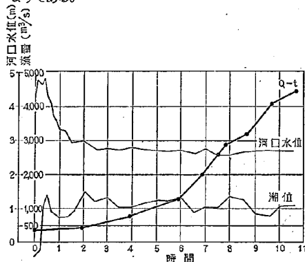
図-38 河口水位 (二次元実験)
