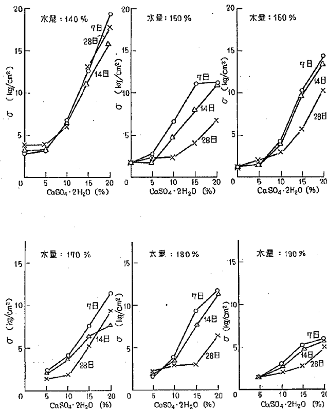
図-15 モルタルの圧縮強度と \text{CaSO}_4 \cdot 2\text{H}_2\text{O} 量の関係 ( \text{Ca}(\text{OH})_2 20%)
