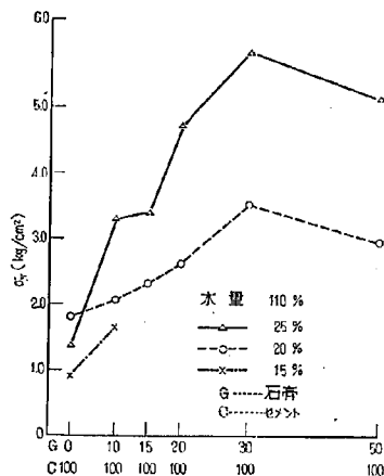
図-19 立川ロームに \text{CaSO}_4 \cdot 2\text{H}_2\text{O} —セメントを添加した場合の圧縮強度
