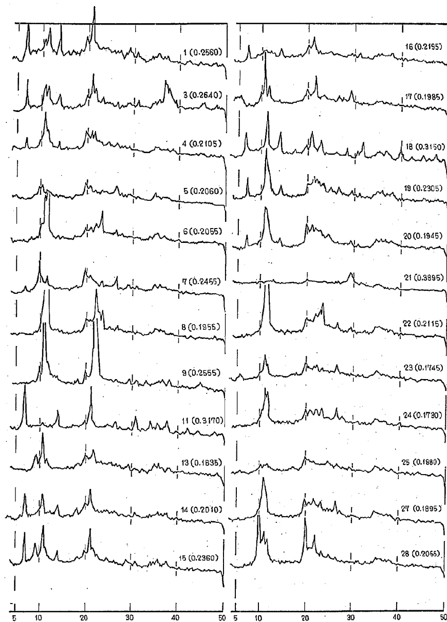
図-9 路床土中のコロイドと \text{Ca}(\text{OH})_2 溶液との反応生成物のX線回折図 (福島県路床土)
