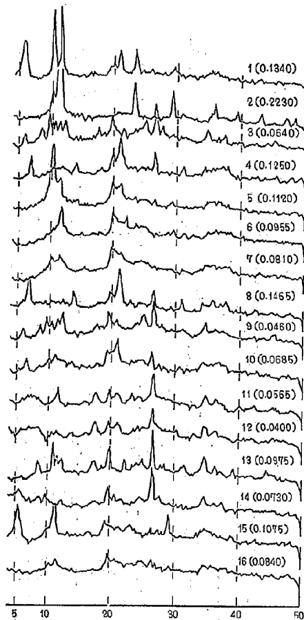
図-7 路床土中のコロイドと \text{Ca}(\text{OH})_2 溶液との反応生成物のX線回折図 (静岡県路床土)
