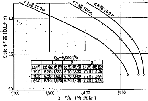
図-51 第1案分流量のせき高と分流量との関係
