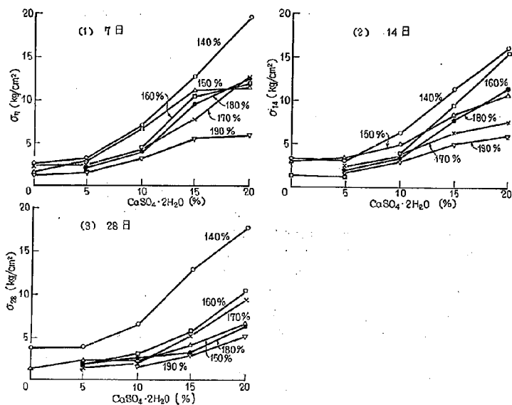
図-17 モルタルの圧縮強度と \text{CaSO}_4 \cdot 2\text{H}_2\text{O} 量および水量の関係 ( \text{Ca}(\text{OH})_2 20%)
