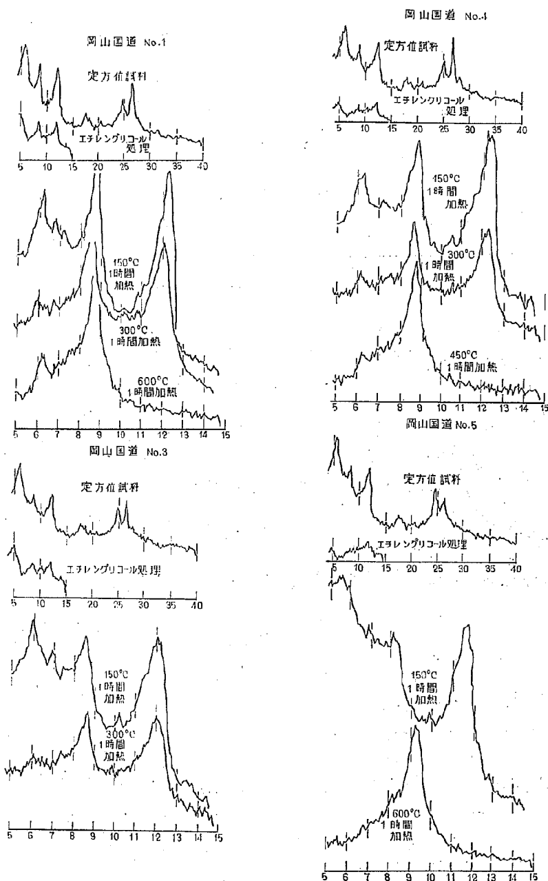
図-3 処理粘土のX線回折図 (岡山国道粘土)
