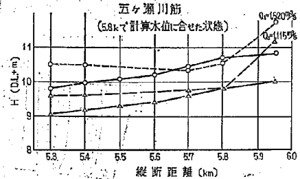
図-56 第1案②せき水位縦断面
