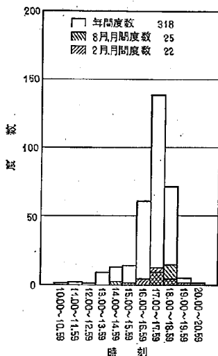
図-27 昭和35年4月～昭和36年3月1カ年間のコンクリート版底面の日最高温度時刻度数分布
