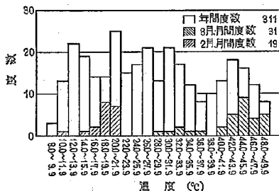
図-11 昭和37年4月～昭和38年3月1カ年間のコンクリート版表面の日最高温度の度数分布
