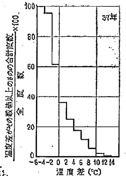
(c) 昭和37年4月~昭和38年3月
