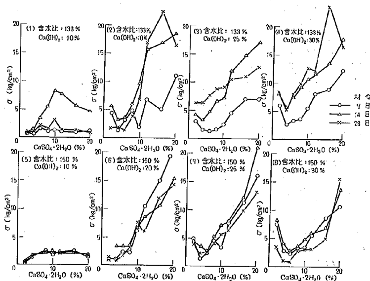
図-6(B) 圧縮強度と配合、材令との関係
