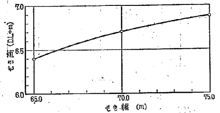
図-51 第1案分流量のせき高とせき幅の関係
