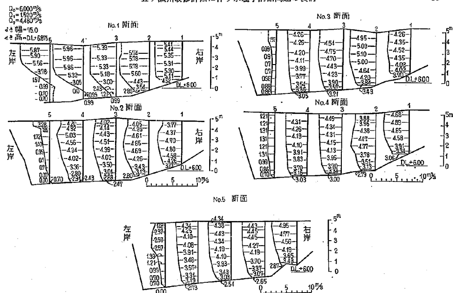
図-59.(3)第1案㊦ぎの場合の流速分布図
