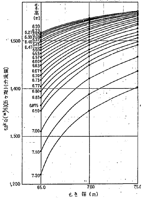
図-50 第1案分流量の分流量
