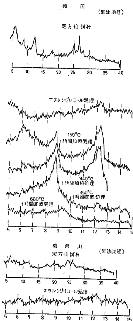
図-4 処理粘土のX線回折図 (梅田粘土, 堀荷山粘土)
