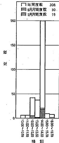
図-23 昭和37年4月~昭和38年3月1カ年間のコンクリート版表面の日最高温度時刻度数分布
