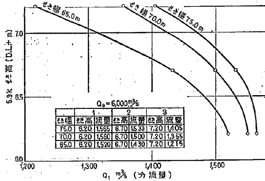
図-49 第1案分流量のせき高と分流量との関係
