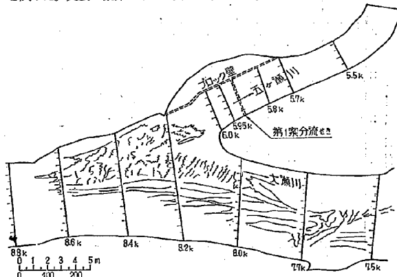
図-60 堆砂状況図
