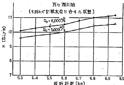
図-46 現状分流水位縦断面
