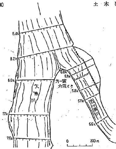
図-61 流線図
