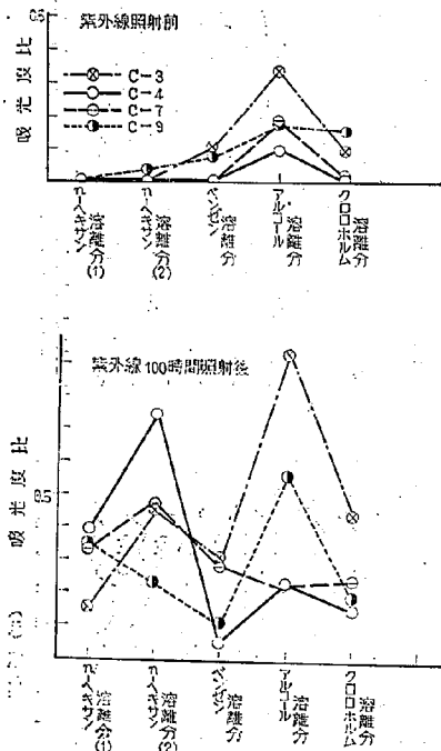
図-12 アスファルト組成成分の IR スペクトルにおける 5.86 (C=O による) 吸光度比
