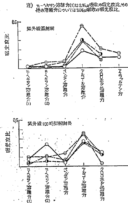
図-14 アスファルト組成成分の IR スペクトルにおける 3μ 付近の吸収 (OH, NH または NH 2 による) の吸光度比
