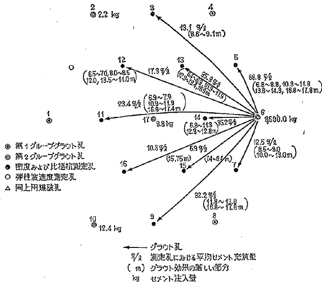
図-13 グラウト効果の平面分布 (下久保ダム第2グラウト)
