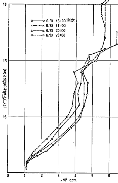
図-30 (k) 利根川河床洗掘測定結果 (1961.6.28~7.20)
