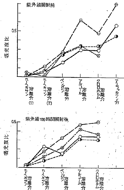
図-13 アスファルト組成成分の IR スペクトルにおける 6.25μ 吸収 (C=C による) 吸光度比
