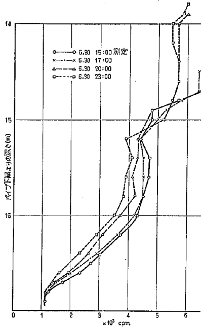
図-30 (k) 利根川河床洗掘測定結果 (1961.6.28~7.20)
