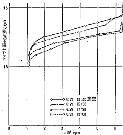
図-30 (f) 利根川河床洗掘測定結果 (1961. 6. 28 ~ 7. 20)
