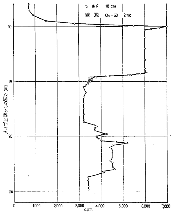
図-28 増水時における測定結果 (1960.8.21, 16:00)
