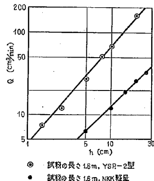
図-8 (b) 海岸砂に矢板が埋め込まれた場合の水位差 (h) と流量 (Q) の関係
