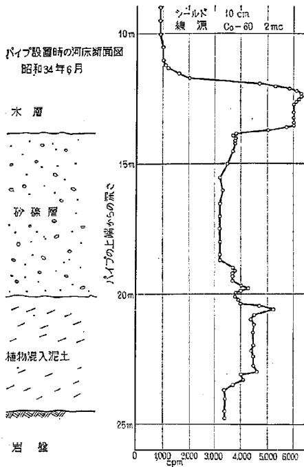
図-22 平時における測定結果 (1960.5.7)
