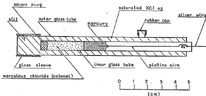
図-4 電極の構造
