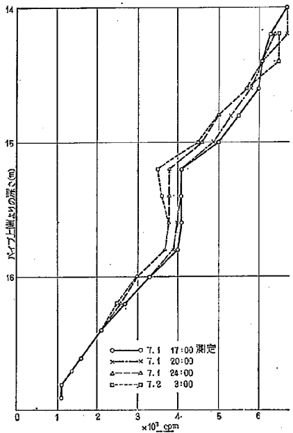
図-30 (n) 利根川河床洗掘測定結果(1961.6.28~7.20)
