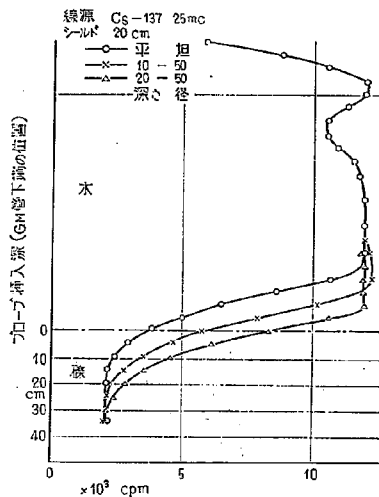
図-16 パイプの周囲の穴の生成による応答数の変化 (11)
