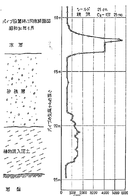
図-21 平時における測定結果 (1960.4.6)
