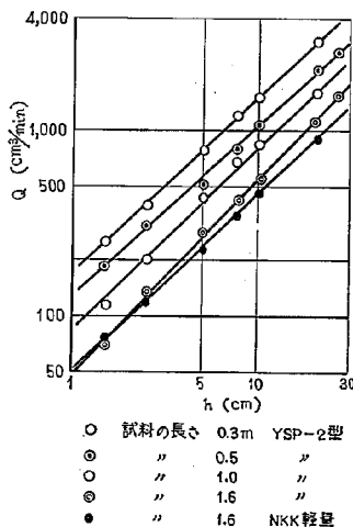
図-8 (a) 川砂に矢板が埋め込まれた場合の水位差 (h) と流量 (Q) の関係
