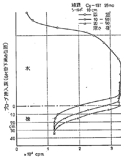
図-15 パイプの周囲の穴の生成による応答数の変化 (10)
