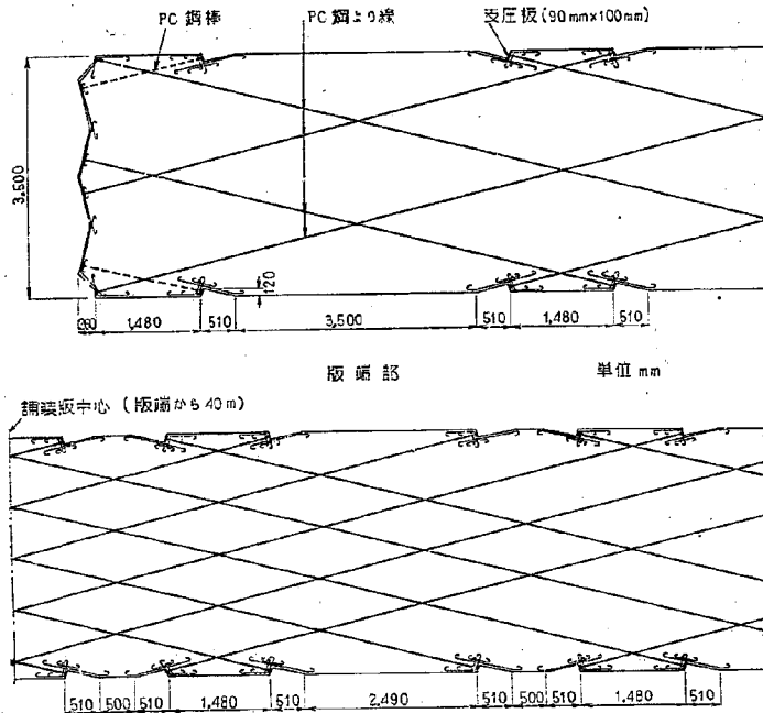
図-3 斜め方向版の PC 鋼より線配置 (単位 mm)
