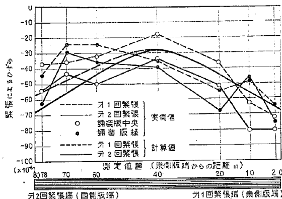
図-19 縦方向版緊張によるひずみ (木緊張)
