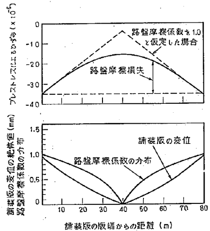
図-5 斜め方向版の設計プレストレスの計算
