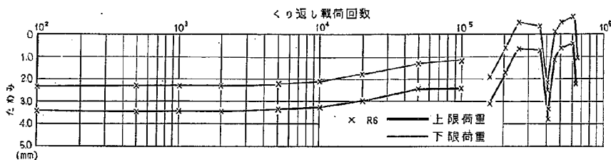
図-29 くり返し載荷による簡装版縁部のたわみ (その2)
