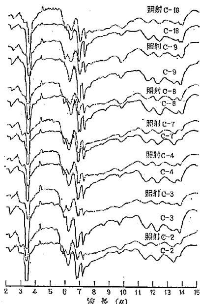
図-10 アスファルト試料の紫外線照射前後の赤外線吸収スペクトル
