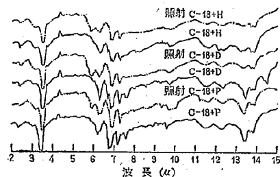
図-15 各種薬剤を添加したアスファルトの紫外線照射前後の赤外線吸収スペクトル
