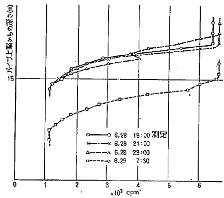
図-30 (c) 利根川河床洗掘測定結果 (1961. 6. 28~7. 20)
