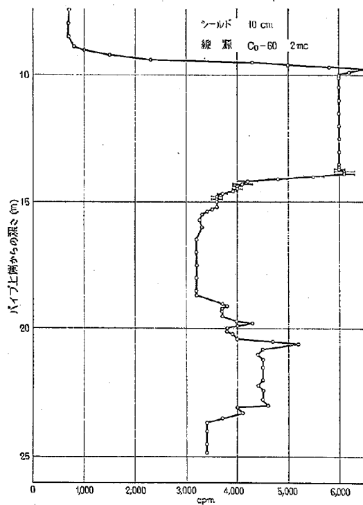
図-25 増水時における測定結果 (1960.8.13, 9:00)
