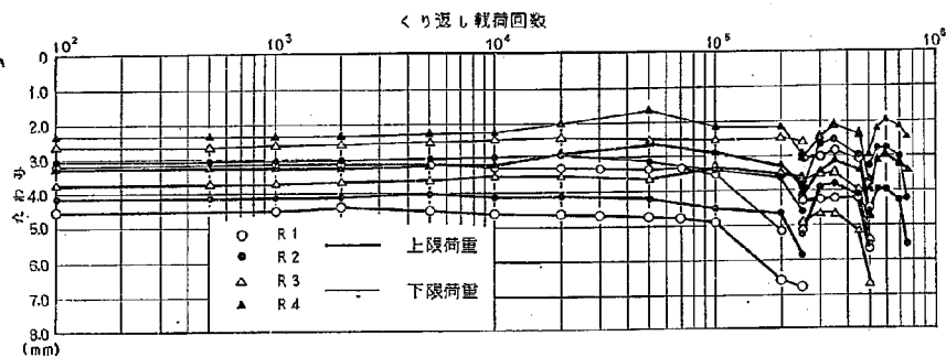
図-28 くり返し載荷による舗装版縁部のたわみ (その1)
