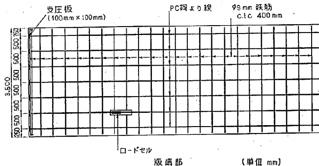
図-2 縦方向版のPC鋼より線配置 (単位 mm)
