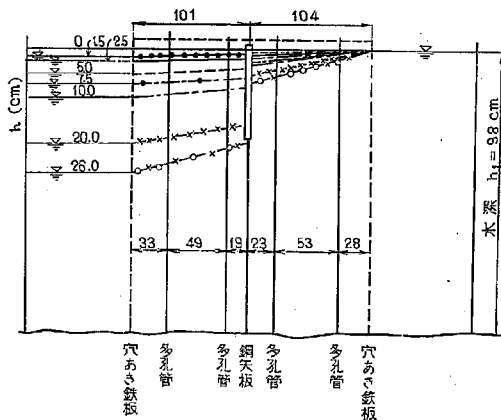
図-9 (a-2) 実験水槽内の水位 川砂とYSP-2型の組み合わせ
