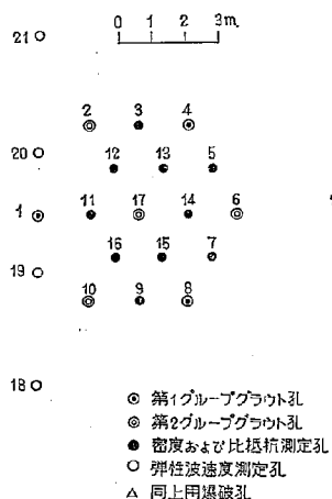
図-4 下久保ダム グラウト試験測定孔配置
