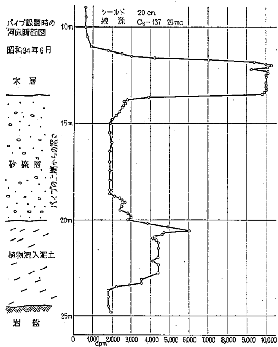
図-23 平水時における測定結果 (1960.5.7)
