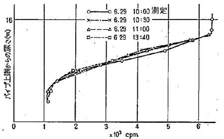
図-30 (e) 利根川河床洗掘測定結果 (1961. 6. 28~7. 20)
