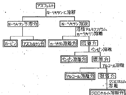
図-1 アスファルト試料の組成分別系統図
