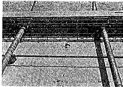
写真-3 縦方向版緊張端の補強鉄筋
