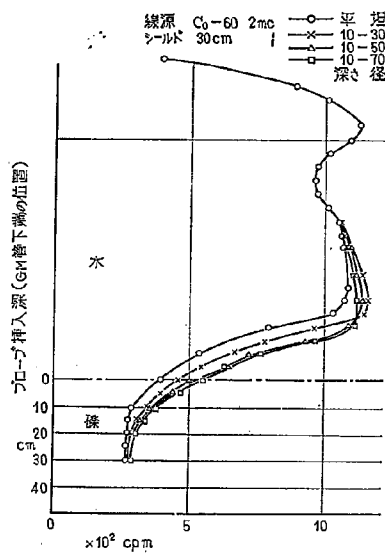
図-8 パイプの周囲の穴の生成による応答数の変化 (3)
