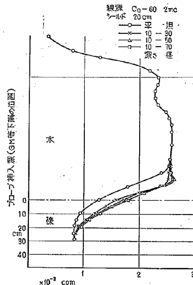
図-7 パイプの周囲の穴の生成による応答数の変化 (2)
