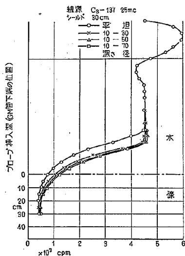
図-11 パイプの周囲の穴の生成による応答数の変化 (6)
