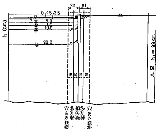
図-9 (a-4) 実験水槽内の水位 川砂とYSP-2型の組み合わせ
