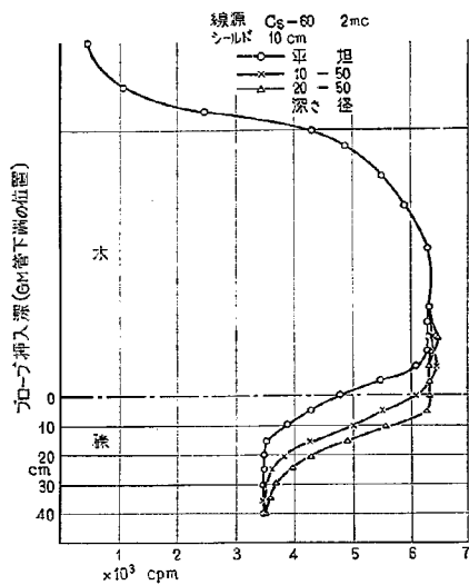
図-12 パイプの周囲の穴の生成による応答数の変化 (7)
