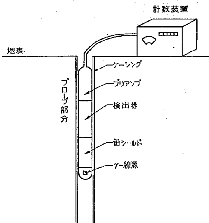
図-1 γ線密度計の概略図
