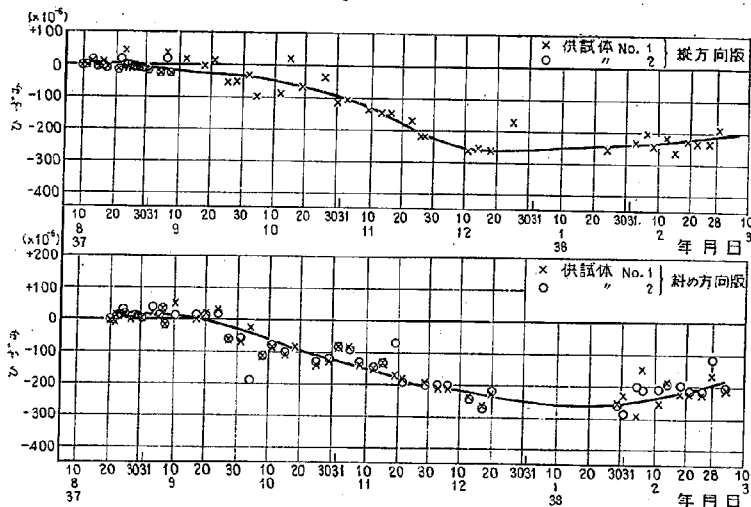
図-8 温度変化による供試体のひずみ（温度膨脹係数を 10 \times 10^{-6}/^{\circ}\text{C} と仮定）午前9時測定
