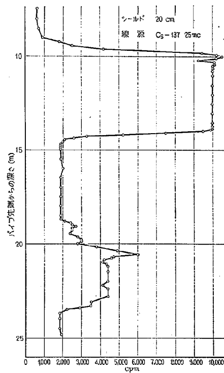
図-26 増水時における測定結果 (1960.8.13, 9:30)
