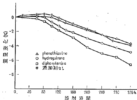
図-2 C-2の紫外線照射過程の重量変化
