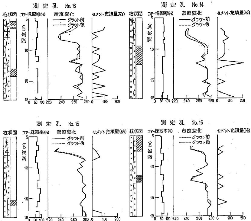
図-11 (b) 下久保ダムセメントグラウト調査結果
