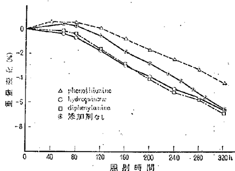
図-5 C-7の紫外線照射過程の重量変化
