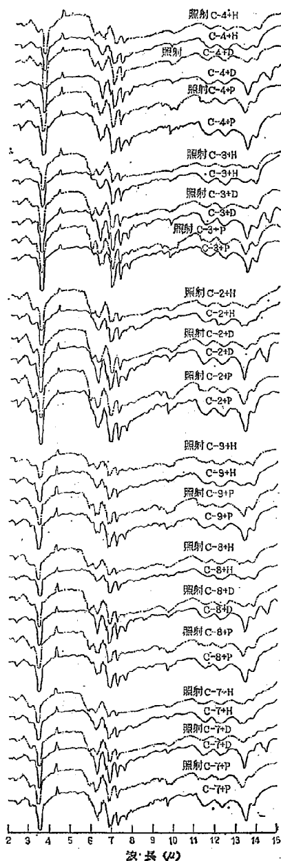
図-15 各種薬剤を添加したアスファルトの紫外線照射前後の赤外線吸収スペクトル
