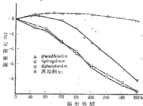
図-3 C-3の紫外線照射過程の重量変化
