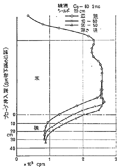
図-13 パイプの周囲の穴の生成による応答数の変化 (8)
