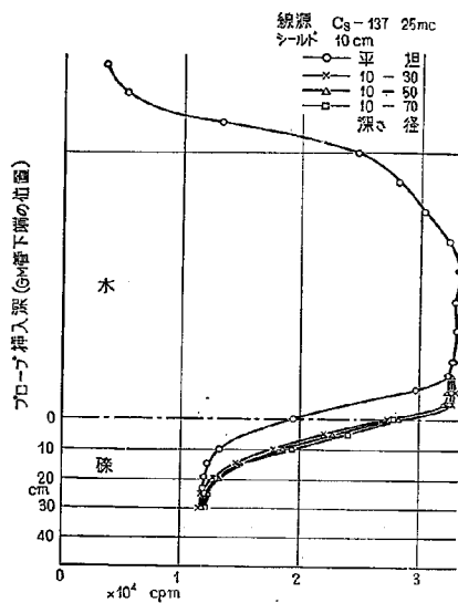
図-9 パイプの周囲の穴の生成による応答数の変化 (4)
