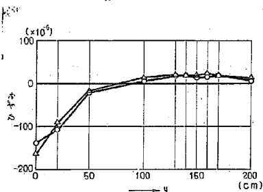
図-21 中央部載荷8 t によるひずみ (縦方向版)
