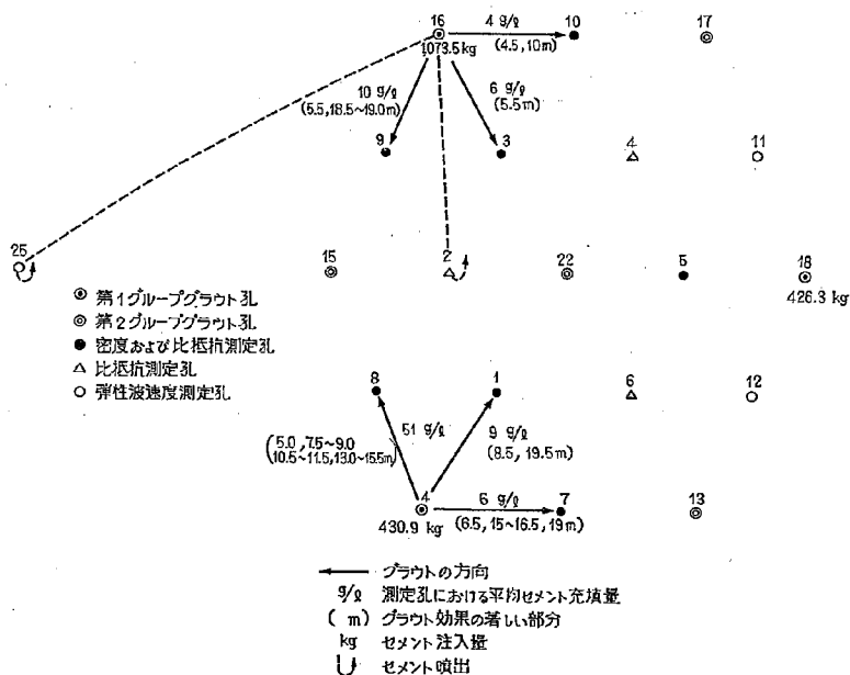
図-9 グラウト効果の平面分布 (園原ダム第3グラウト)
