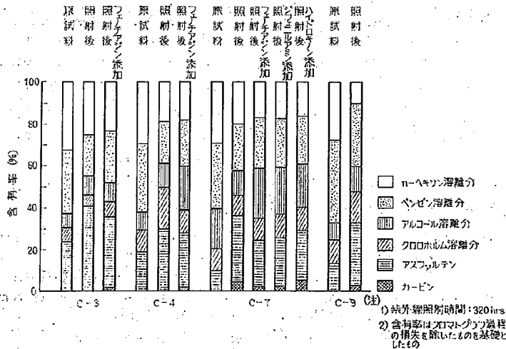
図-9 紫外線照射による組成含量の変化
