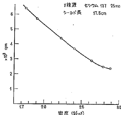
図-2 密度計カリブレーション曲線
