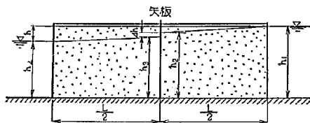
図-11 透水層内の浸透
