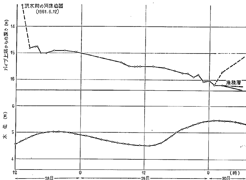
図-31 利根川河床測定結果(1961.6.28~30) 水位と河床位置の関係
