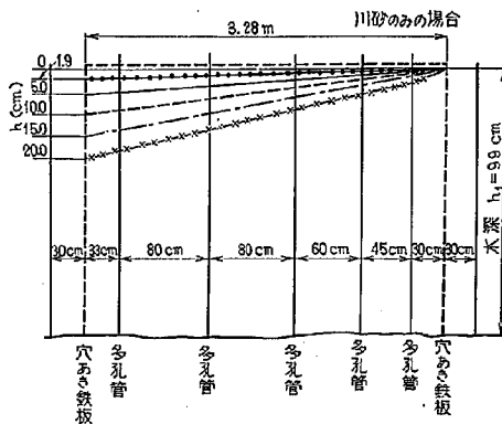
図-5 実験水槽内の水位
