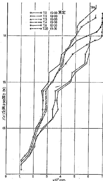
図-30 (P) 利根川河床洗掘測定結果 (1961.6.28~7.20)
