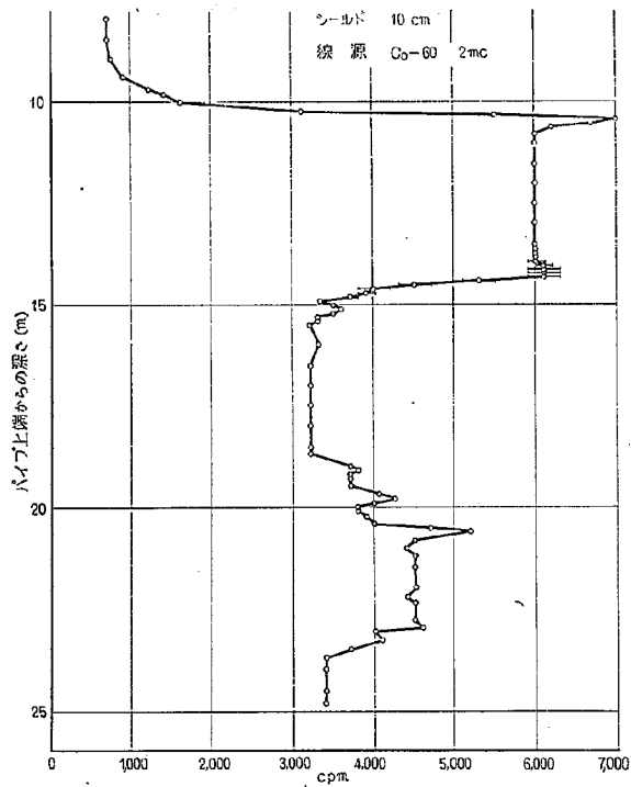
図-27 増水時における測定結果 (1960.8.21, 11:00)
