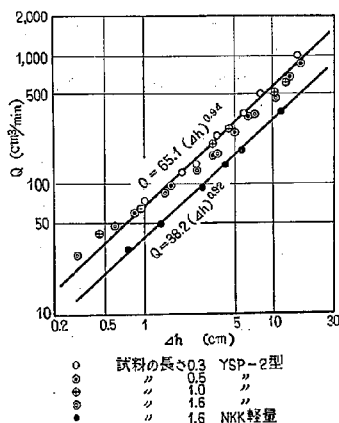
図-10 (a) 鋼矢板縫目 1m 当りの浸透流量 (川砂の場合)
