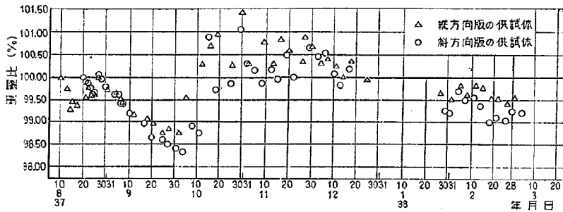
図-9 コンクリート供試体の重量変化 午前9時測定
