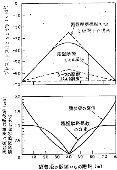
図-4 縦方向版の設計プレストレスの計算
