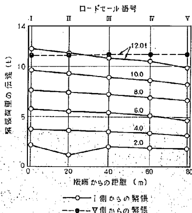
図-12 ロードセルによる緊張荷重の測定結果
