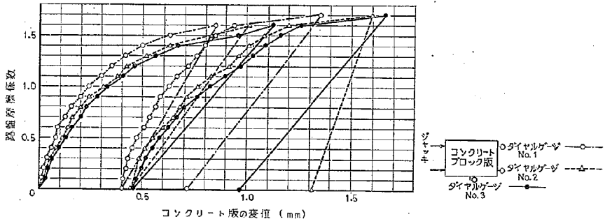
図-13 敷砂厚1cmの場合のコンクリートブロック版の路盤摩擦係数
