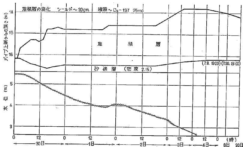
圖-32 利根川河床測定結果 (1961. 6. 30~7. 20)
