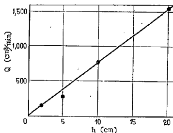
図-6 砂のみの透水実験の流量 (Q) と水位差 (h) の関係
