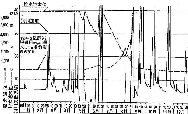
図-13 貯水池の塩分濃度の変化
