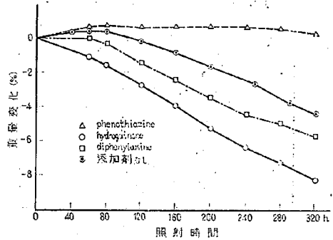
図-8 C-18の紫外線照射過程の重量変化
