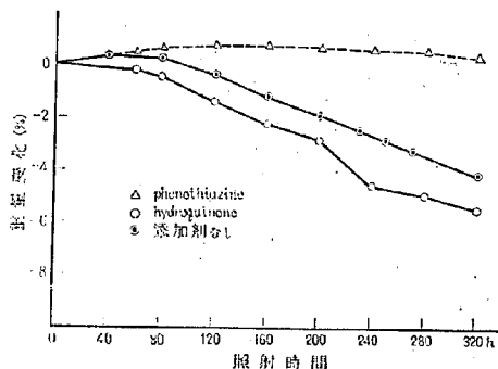
図-7 C-9の紫外線照射過程の重量変化
