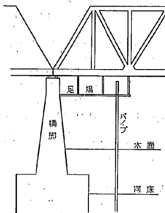
図-18 利根川パイプ設置図
