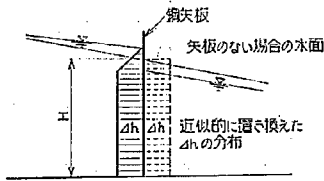
図-14 矢板の位置の水位差
