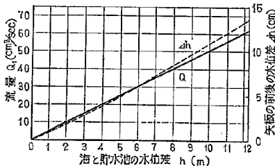
図-15 矢板の止水効果計算例
