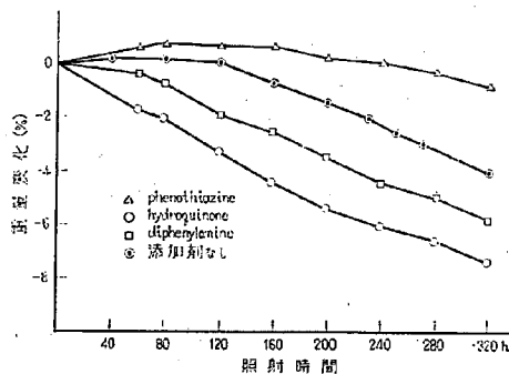
図-4 C-4の紫外線照射過程の重量変化
