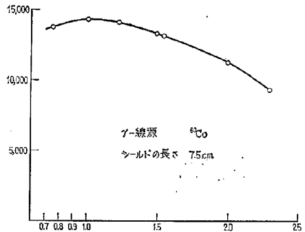
図-3 γ線密度計のカリブレーションカーブ
