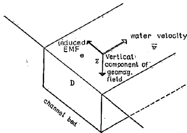
図-3 水路の流れに誘起される起電力
