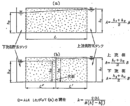
図-4 透水係数の算出
