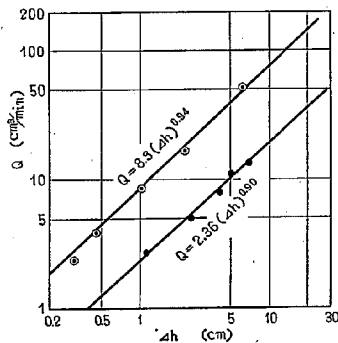
図-10 (b) 鋼矢板縫目 1m 当りの浸透流量 (海岸砂の場合)
