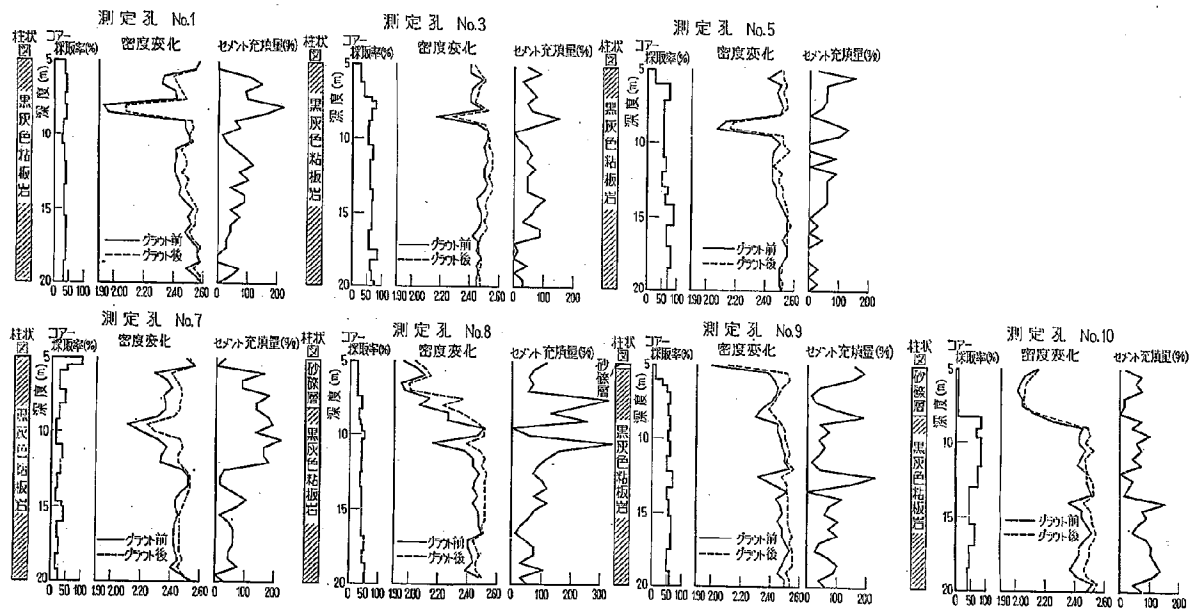
図-5 圓原ダム セメントグラウト調査結果 (1)
