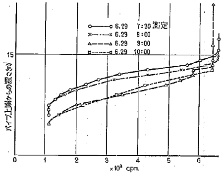
図-30 (d) 利根川河床洗掘測定結果 (1961. 6. 28~7. 20)
