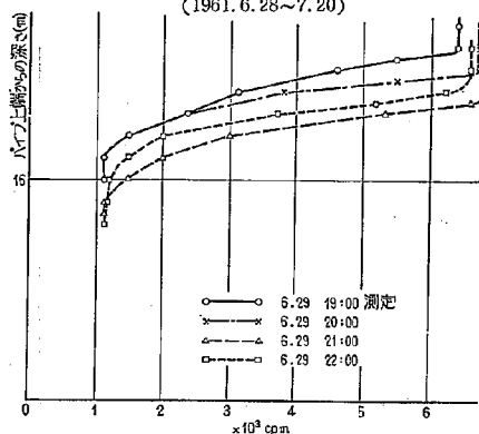
図-30 (g) 利根川河床洗掘測定結果 (1961. 6. 28 ~ 7. 20)
