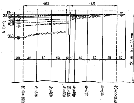
図-9 (b) 実験水槽内の水位 川砂とNKK軽量の組み合わせ
