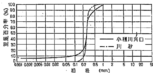
図-3 粒度加積曲線
