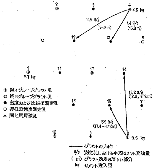
図-12 グラウト効果の平面分布 (下久保ダム第1グラウト)
