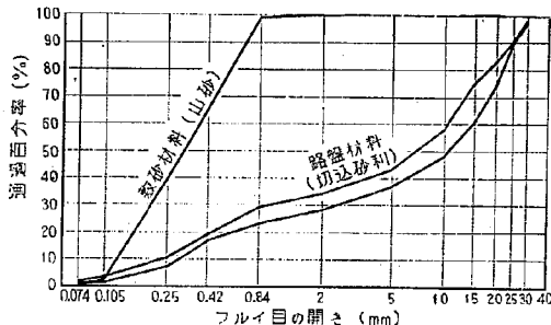
図-7 路盤と敷砂材料の粒度
