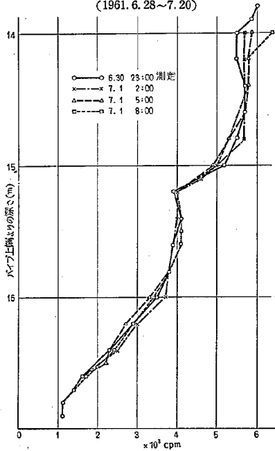
図-30 (l) 利根川河床洗掘測定結果 (1961.6.28~7.20)
