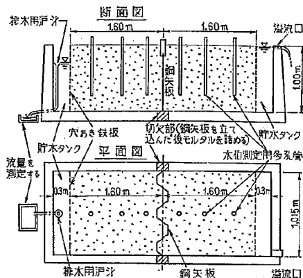
図-1 実験水槽
