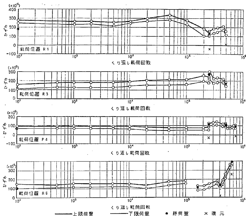
図-30 くり返し载荷による舗装版縁部表面のひずみ
