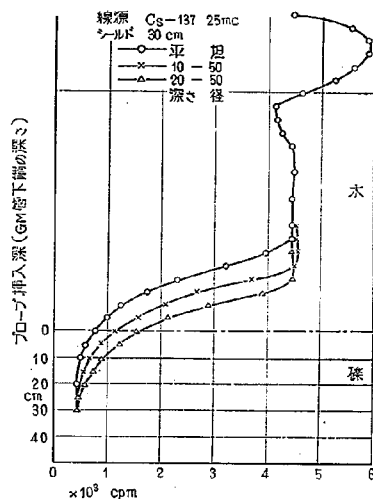
図-17 パイプの周囲の穴の生成による応答数の変化 (12)
