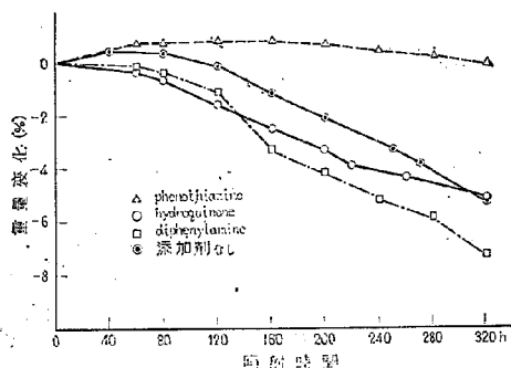
図-6 C-8の紫外線照射過程の重量変化
