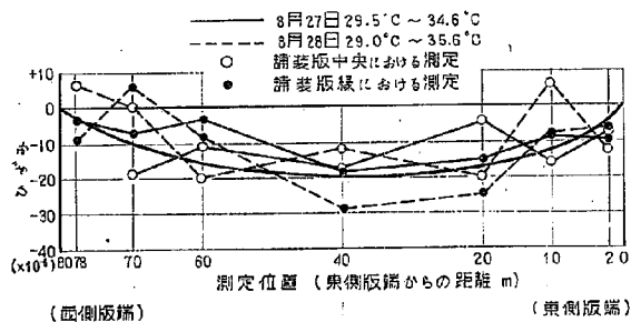
図-17 縦方向版の温度変化によるひずみ
