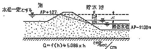
図-12 堤防の浸透流
