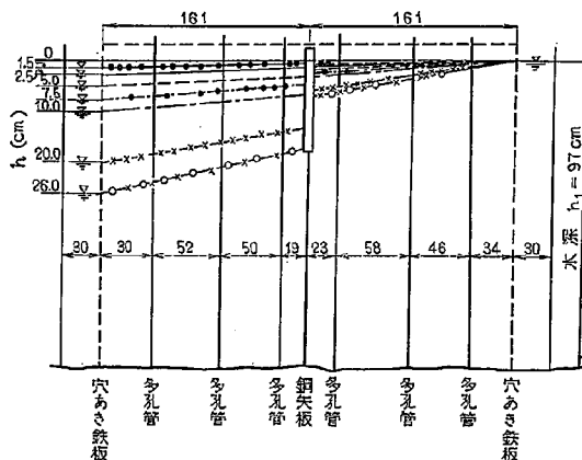
図-9 (a-1) 実験水槽内の水位 川砂とYSP-2型の組み合わせ
