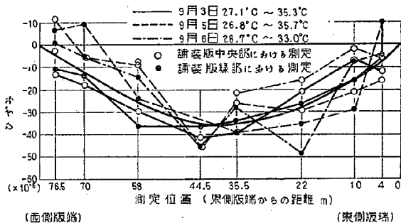
図-18 斜め方向版の温度変化によるひずみ
