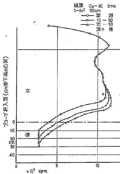
図-14 パイプの周囲の穴の生成による応答数の変化 (9)
