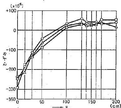
図-22 縁部載荷8 t によるひずみ (縦方向版)
