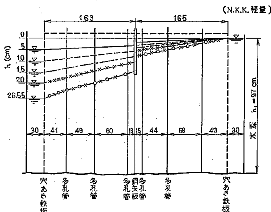
図-9 (d) 実験水槽内の水位 海岸砂とNKK軽量の組み合わせ
