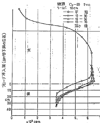
図-6 パイプの周囲の穴の生成による応答数の変化 (1)
