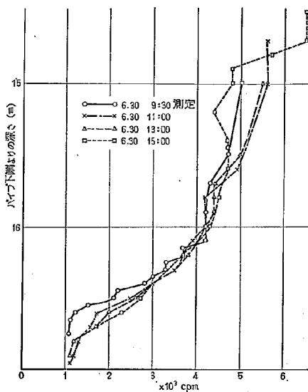
図-30 (j) 利根川河床洗掘測定結果 (1961. 6. 28 ~ 7. 20)
