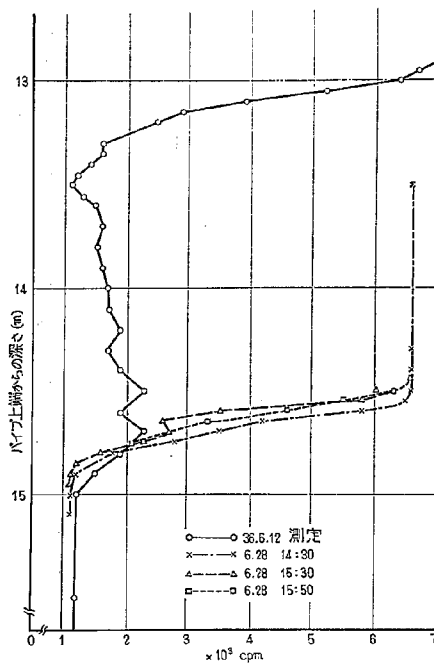
図-30 (a) 利根川河床洗掘測定結果 (1961. 6. 28~7. 20)
