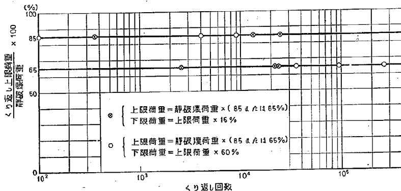
図-27 コンクリート供試体の曲げ疲労試験結果
