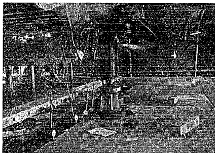
写真-9 くり返し荷重による載荷試験
