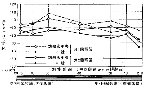
図-15 縦方向版緊張によるひずみ (仮緊張)
