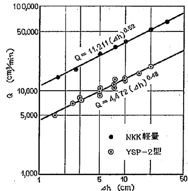
図-7 矢板のみの場合の矢板継目からの滲水量
