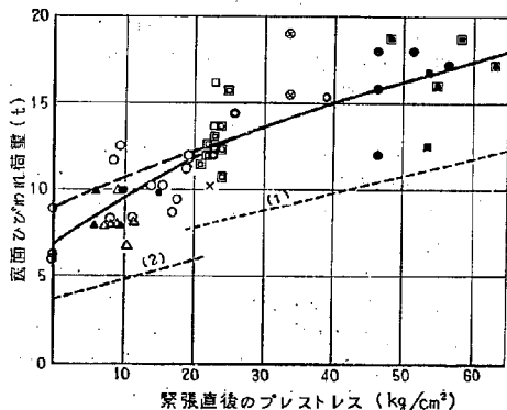
図-26 緊張直後のプレストレスと舗装版綫部の底面ひびわれ荷重との関係 (版厚 12cm)
