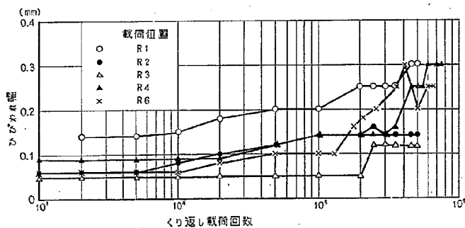
図-31 くり返し载荷によるひびわれ幅の変化
