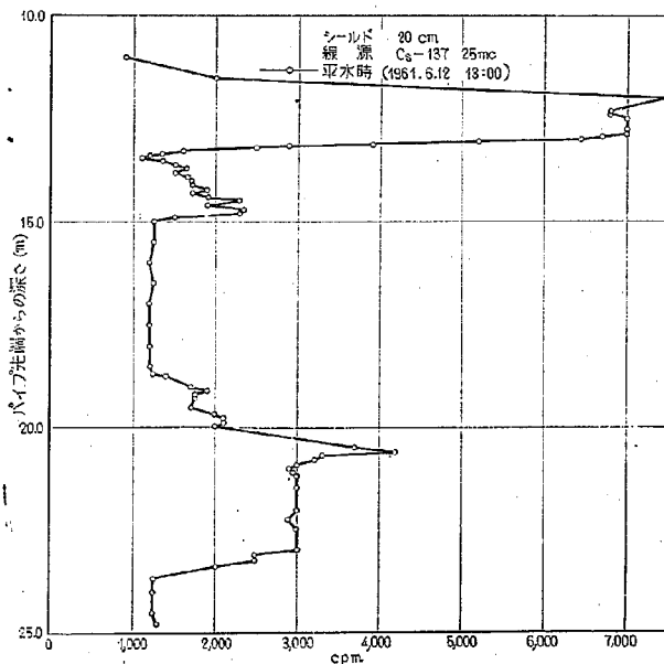
図-29 利根川河床測定結果 (1961.6.12)
