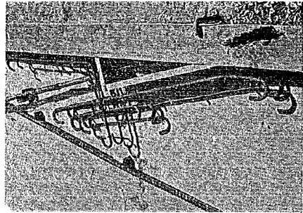
写真-4 斜め方向版緊張端の補強鉄筋
