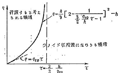
図-5 \eta_{\tau} > 0 のときの波形の区別
