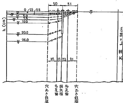
図-9 (a-3) 実験水槽内の水位 川砂とYSP-2型の組み合わせ
