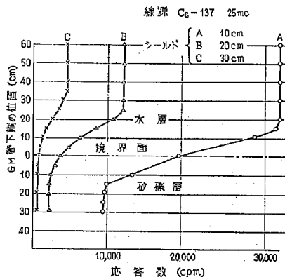
図-5 水-礫層境界における深さと応答数間の関係 前に述べた検出器と \gamma -線源との距離 r とだいたい次のような関係にある。
