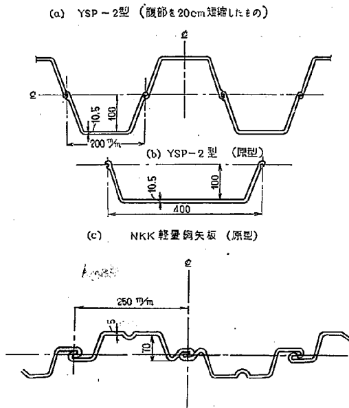
図-2 実験に使用した鋼矢板
