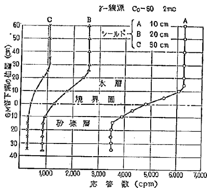
図-4 水-礫層境界における深さと応答数間の関係
