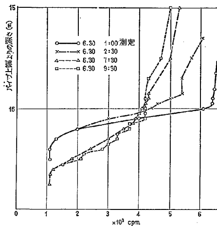
図-30 (i) 利根川河床洗掘測定結果 (1961. 6. 28 ~ 7. 20)
