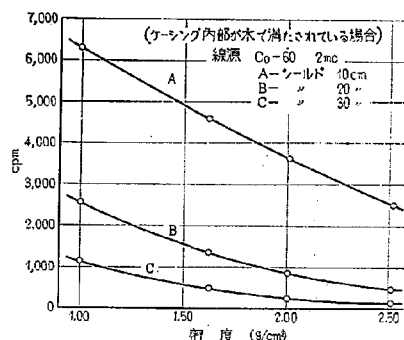
図-19 カリブレーション曲線
