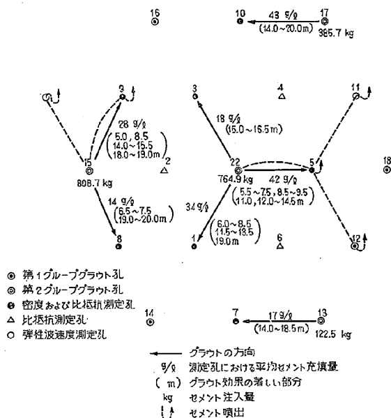
図-10 グラウト効果の平面分布 (箇原ダム第4グラウト)
