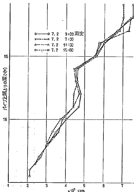
図-30 (O) 利根川河床洗掘測定結果 (1961.6.28~7.20)
