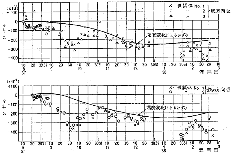
図-10 コンクリート供試体の長さ変化 午前9時測定
