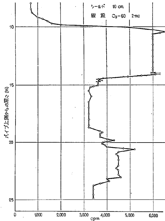
図-24 増水時における測定結果 (1960.8.12, 19:00)
