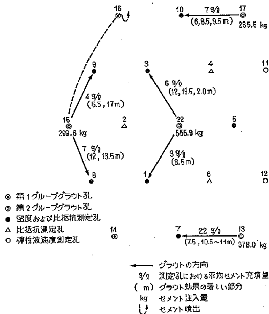
図-8 グラウト効果の平面分布 (園原ダム 第2グラウト)
