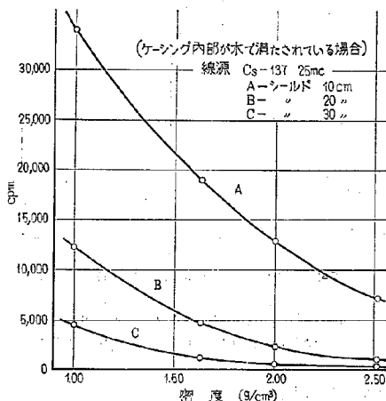
図-20 カリブレーション曲線
