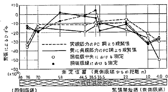
図-16 斜め方向版緊張によるひずみ (仮緊張)
