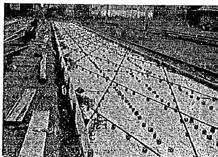
写真-2 斜め方向版の PC 鋼より線配置
