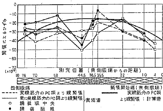
図-20 斜め方向版緊張によるひずみ (木緊張)
