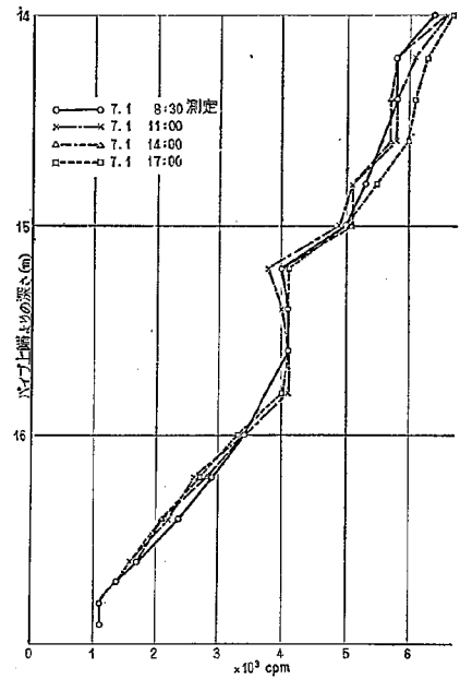
図-30(m) 利根川河床洗掘測定結果(1961.6.28~7.20)
