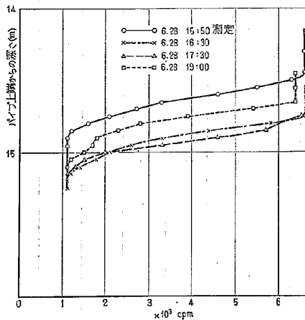
図-30 (b) 利根川河床洗掘測定結果 (1961. 6. 28~7. 20)
