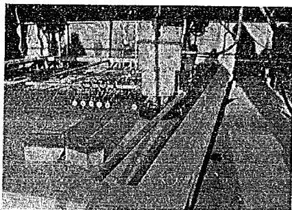
写真-8 静荷重による載荷試験
