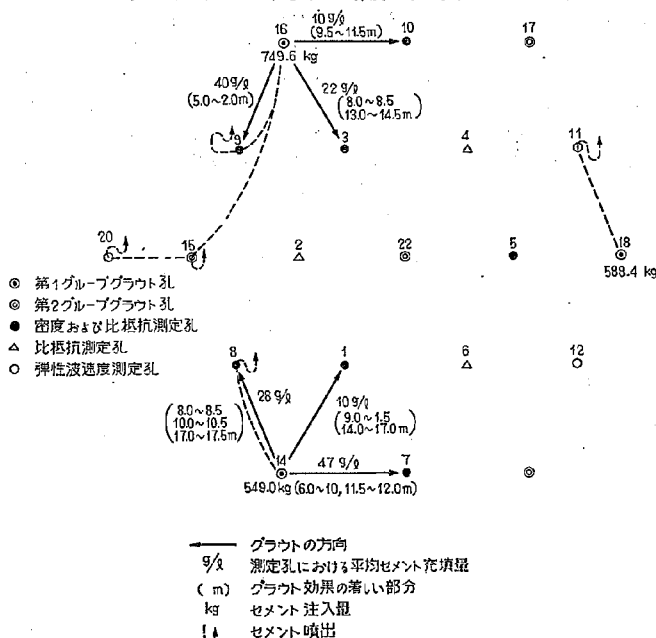
図-6 グラウト効果の平面分布 (断原ダム第 1 グラウト)
