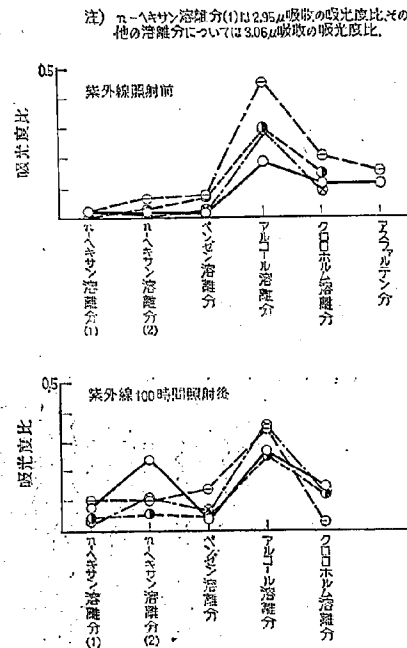
図-14 アスファルト組成分の IR スペクトルにおける 3\mu 付近の吸収 ( OH , NH または NH_2 による) の吸光度比
