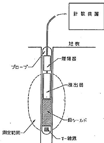
図-1 γ線背面散乱型密度計概略図
