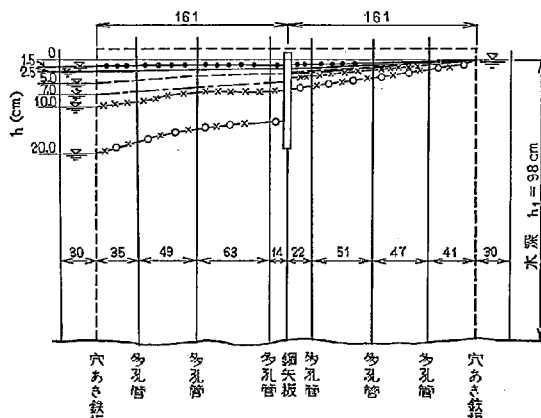
図-9 (c) 実験水槽内の水位 海岸砂とYSP-2型の組み合わせ
