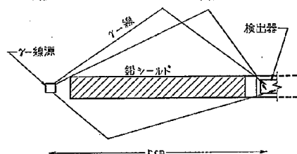
図-2 \gamma -線源と検出器との相対的位置
