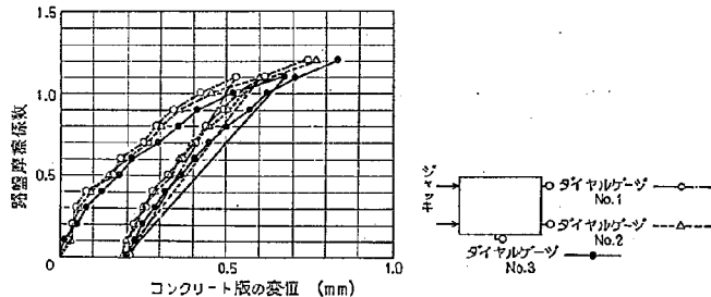
図-14 敷砂厚2cmの場合のコンクリートブロック版の路盤摩擦係数
