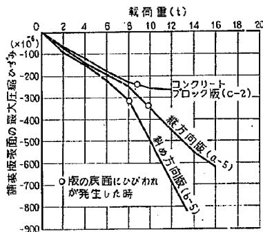
図-23 縁部載荷による荷重-最大圧縮ひずみの関係の例
