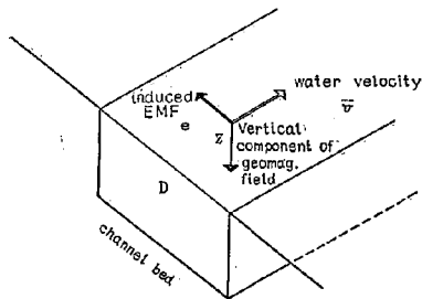
図-3 水路の流れに誘起される起電力
