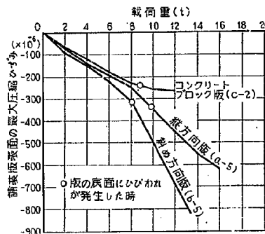
図-23 縁部載荷による荷重-最大圧縮ひずみの関係の例
