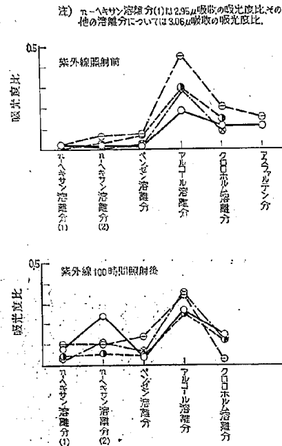
図-14 アスファルト組成分の IR スペクトルにおける 3μ 付近の吸収 (OH, NH または NH 2 による) の吸光度比
