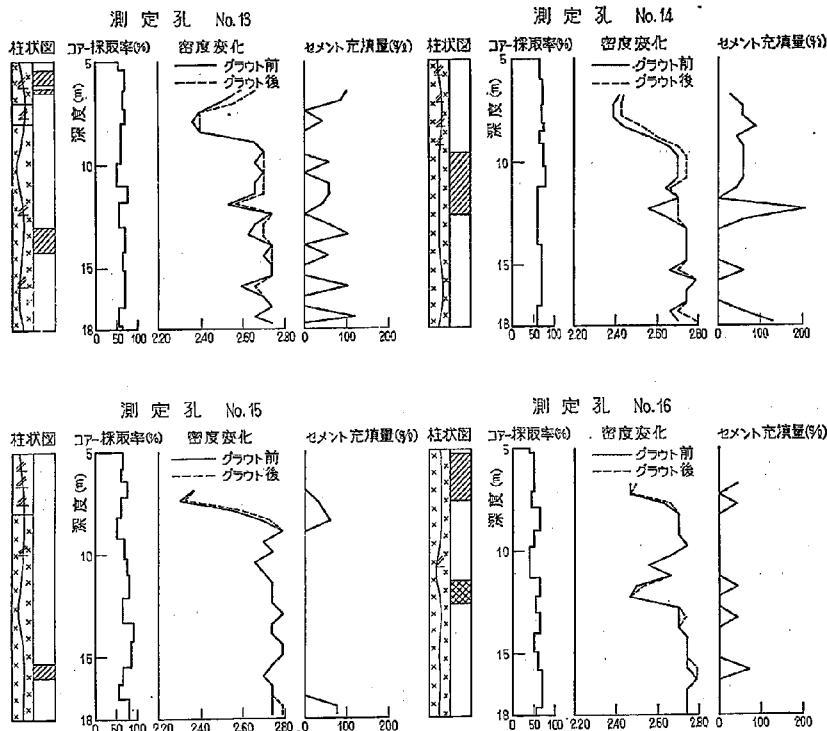
図-11 (b) 下久保ダムセメントグラウト調査結果
