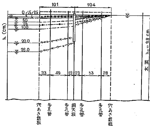
図-9 (a-2) 実験水槽内の水位 川砂とYSP-2型の組み合わせ
