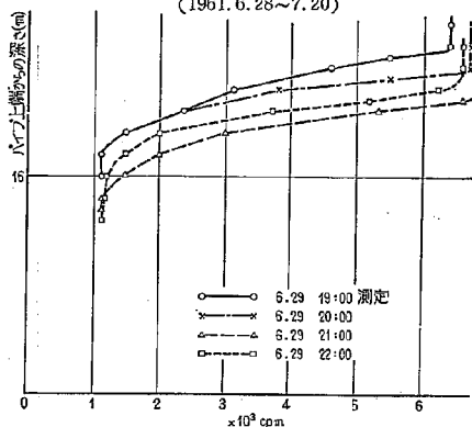
図-30 (g) 利根川河床洗掘測定結果 (1961.6.28~7.20)
