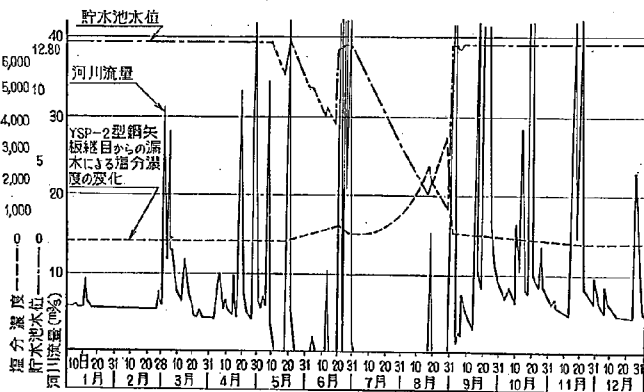
図-13 貯水池の塩分濃度の変化
