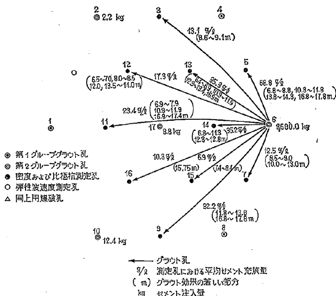
図-13 グラウト効果の平面分布（下久保ダム第2グラウト）
