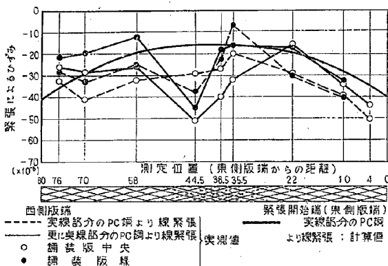
図-20 斜め方向版緊張によるひずみ (本緊張)
