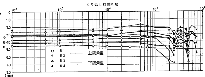
図-28 くり返し載荷による舗装版縁部のたわみ (その1)
