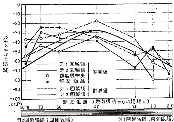
図-19 縦方向版緊張によるひずみ (本緊張)
