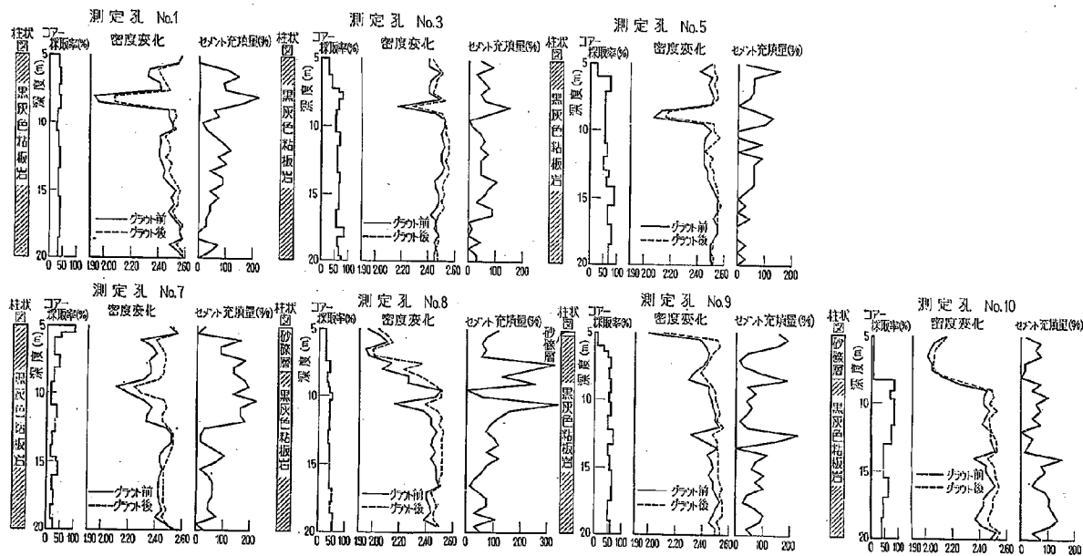
図-5 黒原ダム セメントグラウト調査結果(1)
