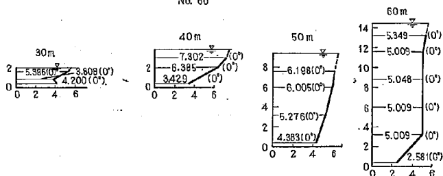
図-21(5) 2-17 型における流速図
