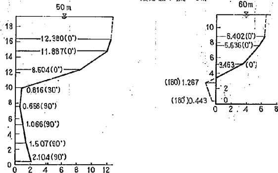
図-7(2) 2-12 型における流速図
