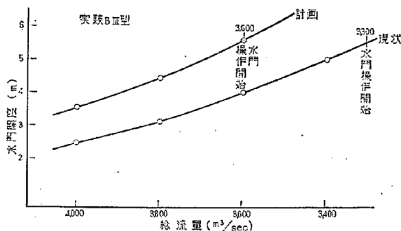
図-37 水門開度、総流量曲線
