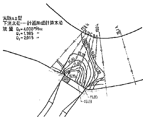
図-30 水位等高図
