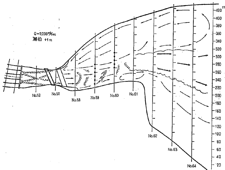
図-37(10) 流線スケッチ 模型形状 2-16 型
