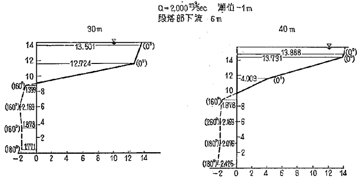
図-16(2) 2-15 型における流速図
