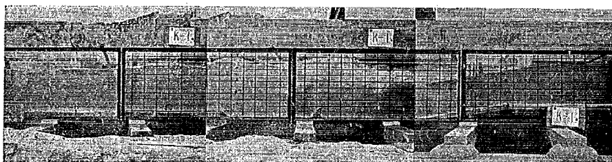
写真-1 1-3型 模型における流況 (流量 2,000 \text{m}^3/\text{sec} , 潮位 -1m, シル高 0m の場合)
