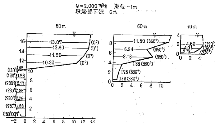
図-26(2) 2-19 型における流速図
