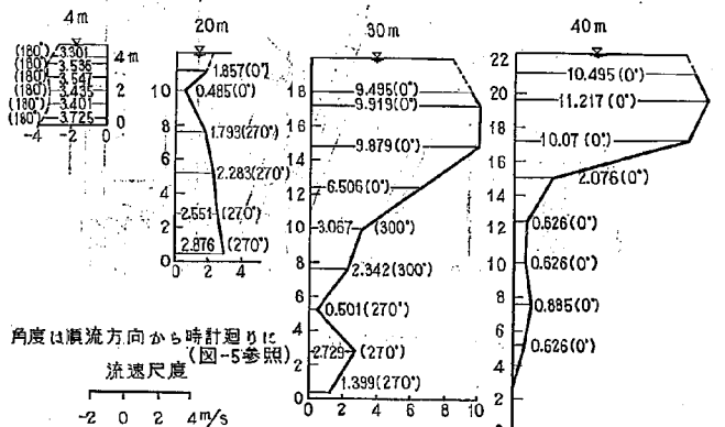
図-7(1) 2-12 型における流速図
