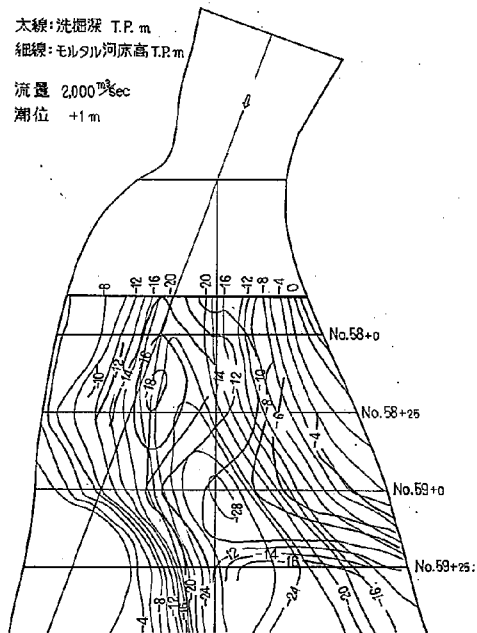
図-35(1) 段落下流側ほどこまで洗掘されるか。 10分(模型で)通水後の河床高
