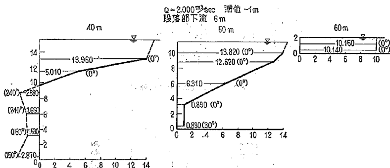
図-18(2) 2-16 型における流速図
