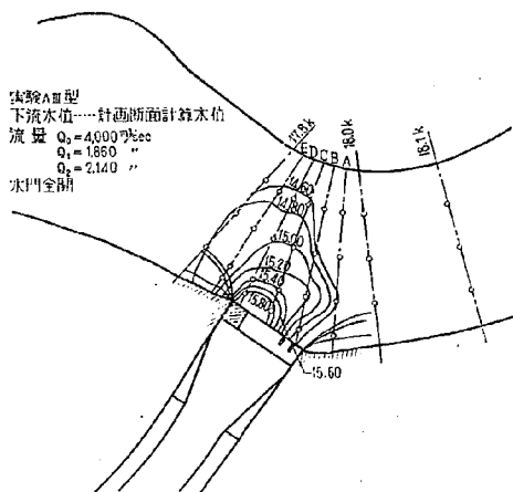
図-32 水位等高図
