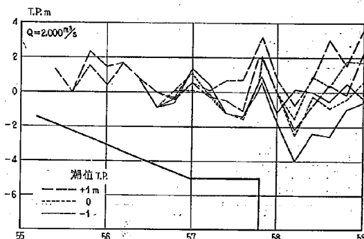
図-3.15 2-14 型 模型水位の縦断
