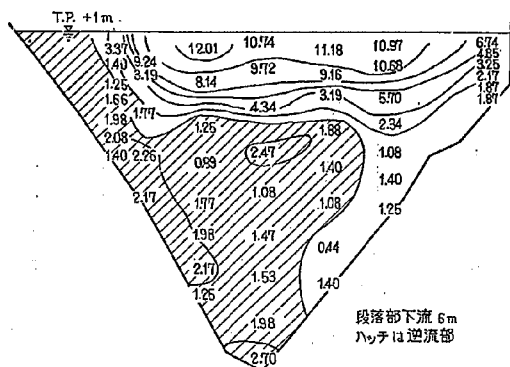
図-5.5 2-14 型 流量 2,000 m³/sec, 潮位 T.P. +1m
