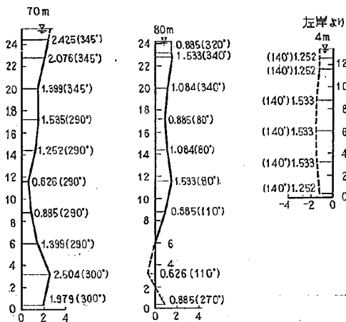
図-18(4) 2-16 型における流速図
