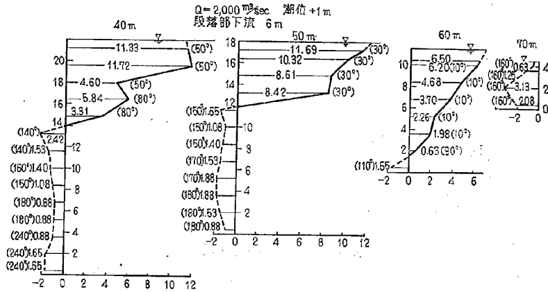
図-27(2) 2-20 型における流速図
