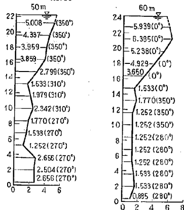
図-31(5) 2-21 型における流速図
