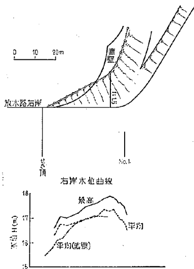
図-38 せき右岸形状変化による水位変化比較図
