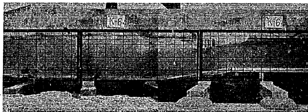
写真-6 1-3 型 模型における流況 (流量 2,000 \text{ m}^3/\text{sec} , 潮位 0 \text{ m} , シル高 1 \text{ m} の場合)
