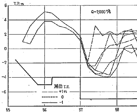
図-3.4 2-5 型 模型の水位縦断
