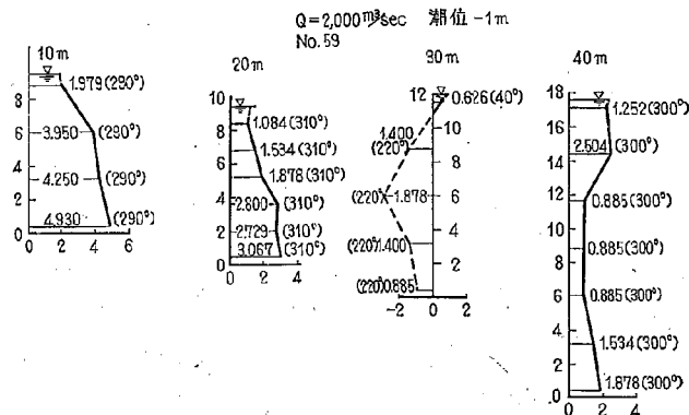
図-24(4) 2-18 型における流速図
