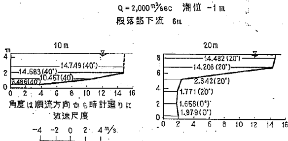
図-16(1) 2-15 型における流速図
