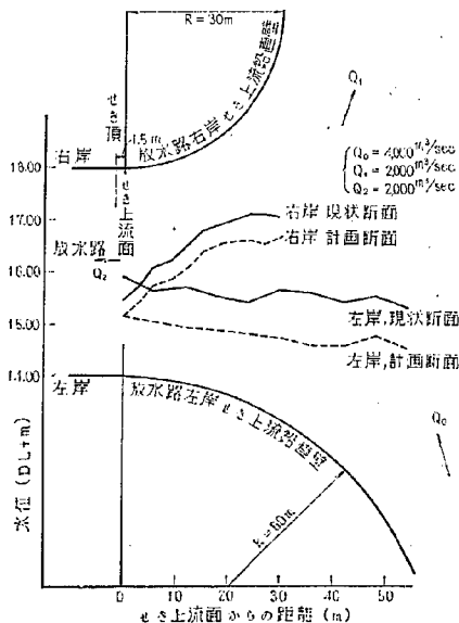
図-34 せき直上流右岸水位比較図
