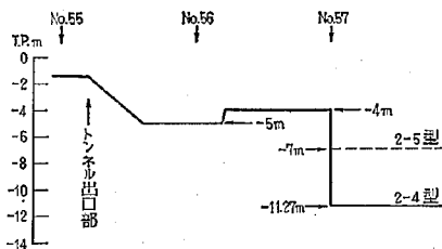
図-2.3 2-4 型, 2-5 型 縦断面図
