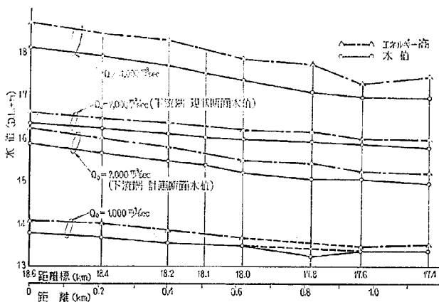
図-9 検証実験縦断水位およびエネルギー高図
