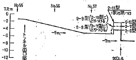
図-2.4 2-6 型, 2-7 型, 2-8 型, 2-9 型, 2-10 型, 2-11 型 縦断面図
