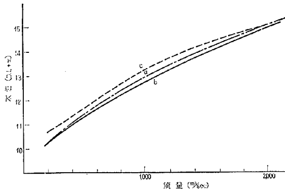
図-5 No. 17.6km 断面の水位流量曲線 (計画断面)
