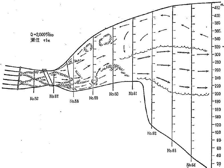
図-37(16) 流線スケッチ 模型形状 2-19 型
