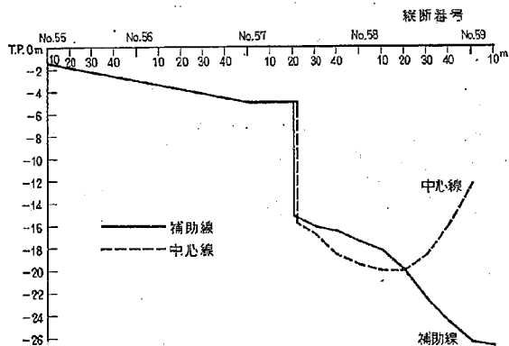
図-14 模型河床縦断
