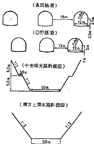
図-2 放水路断面図
