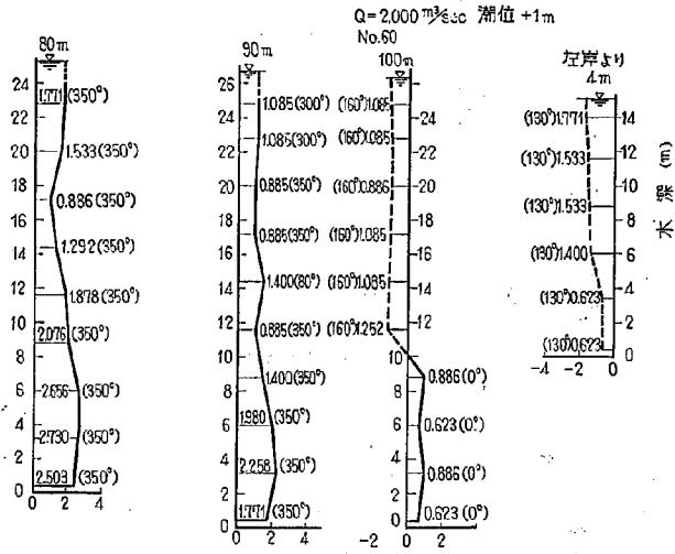
図-15(6) 2-15 型における流速図
