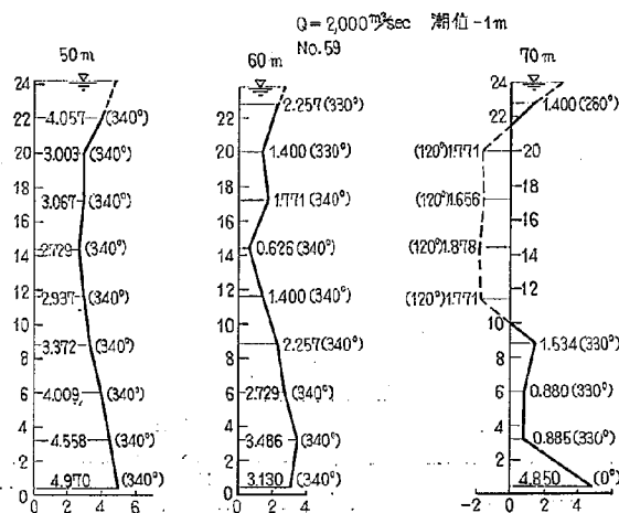
図-22(4) 2-17 型における流速図
