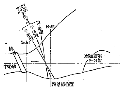
図-2.9 2-19型、2-20型、2-21型 平面図
