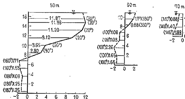
図-25(2) 2-19 型における流速図
