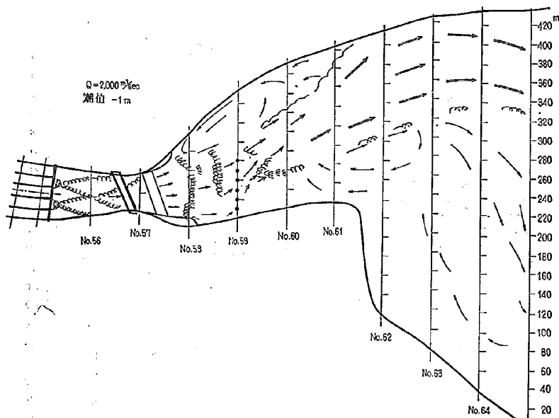
図-37(11) 流線スケッチ 模型形状 2-16 型
