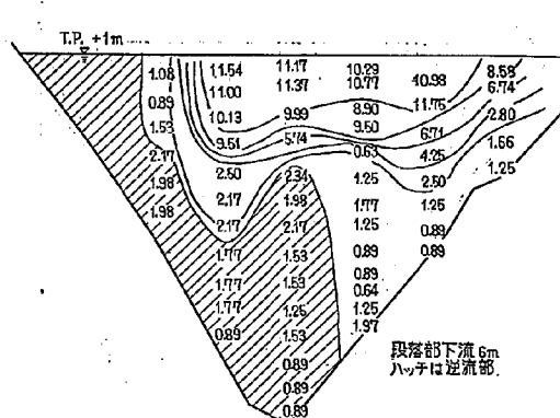
図-5.9 2-21 型 流量 2,000 m³/sec, 潮位 T.P. +1 m
