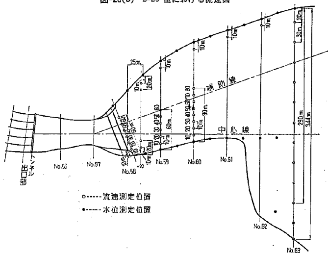
図-29 2-21 型における流速、水位測定位置平面図
