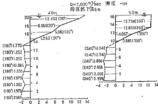
図-31(2) 2-21 型における流速図
