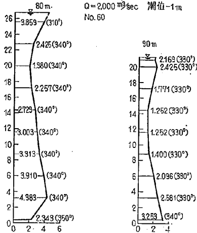
図-22(6) 2-17 型における流速図
