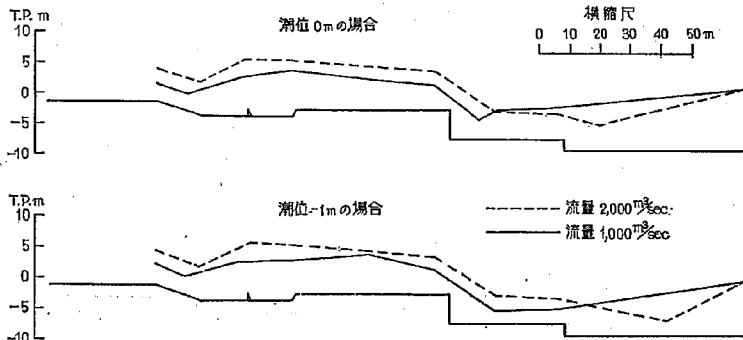
図-1.3.2 シル高 0m の 1-3 型 模型における水位縦断
