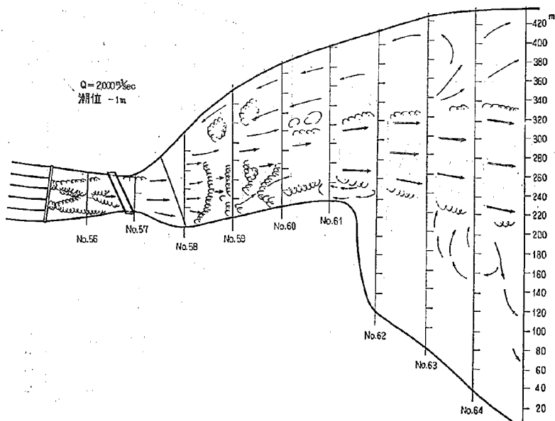
図-37(22) 流線スケッチ 模型形状 2-21 型 (右岸岩礁掘削 T.P. -4.0 m)
