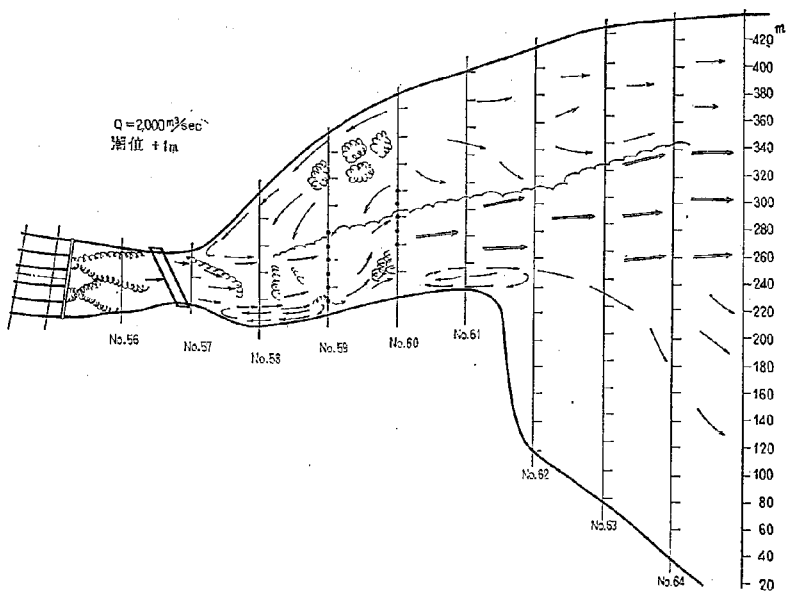
図-37(14) 流線スケッチ 模型形状 2-18 型
