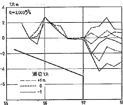
図-3.2 2-2 型模型の水位縦断
