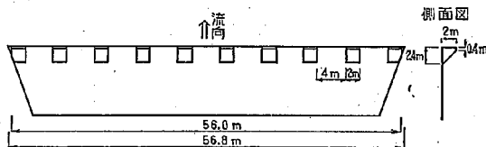
図-3.11 2-13 型パフフルビア
