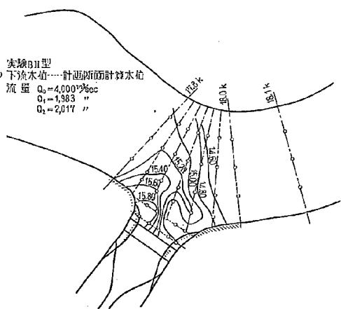
図-31 水位等高図
