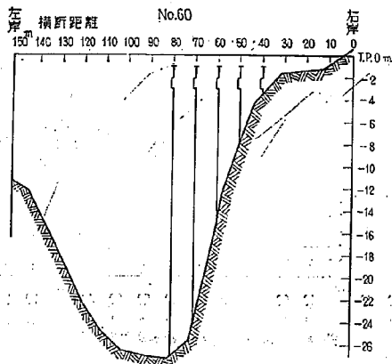
図-6(2) 流速測定位置横断面図
