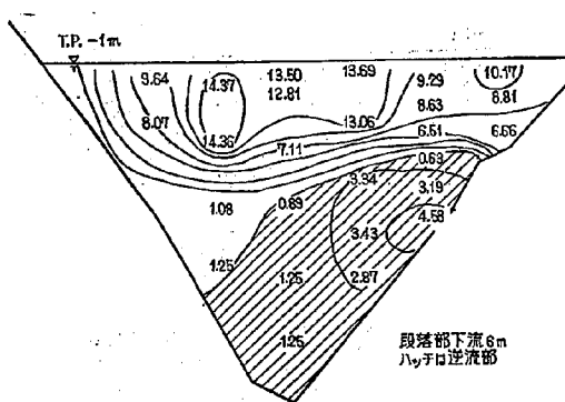
図-5.8 2-18 型 流量 2,000 m 3 /sec, 潮位 T.P. -1m
