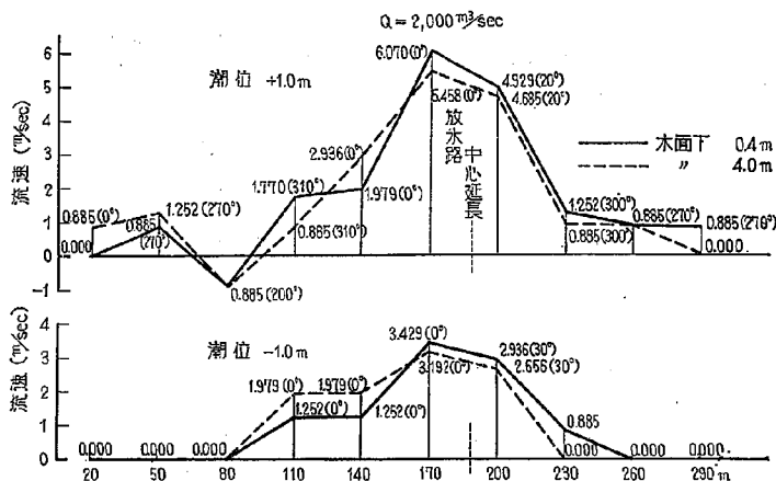
図-32 2-21 型 No. 63 表層流速
