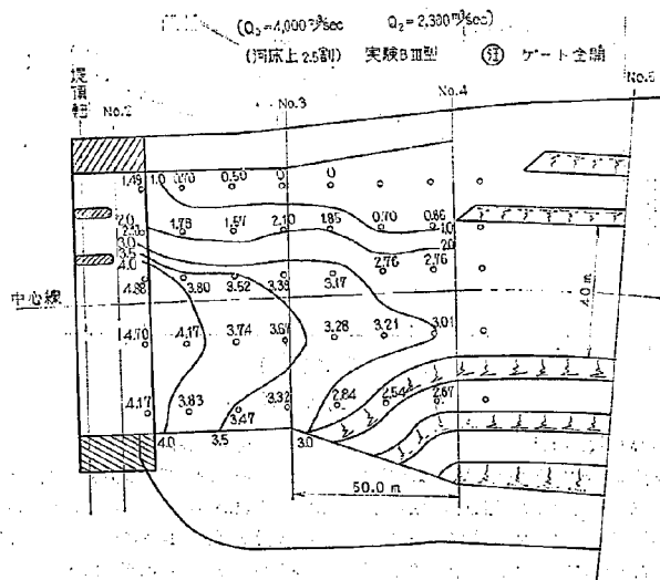
図-35 せき下流流速分布図
