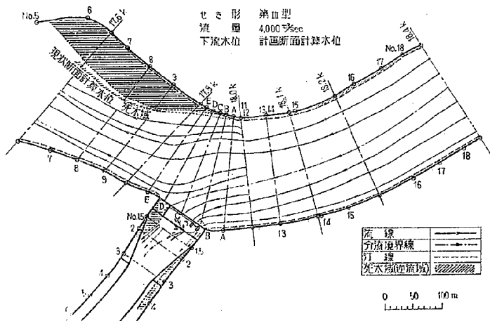
図-25 分流せき付近流向図
