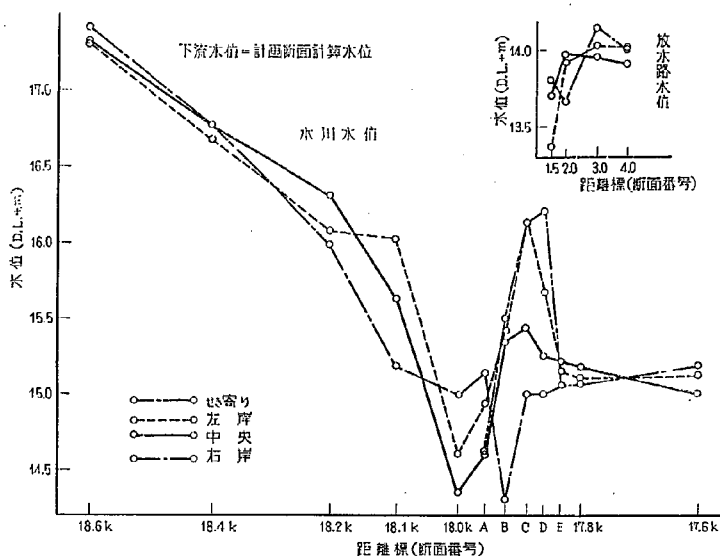
図-20 水位縦断面図 Q_0=4,000\text{m}^3/\text{sec} (Ⅱ型)
