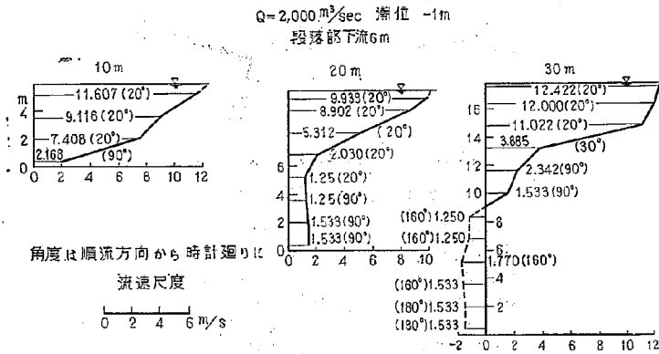
図-31(1) 2-21 型における流速図
