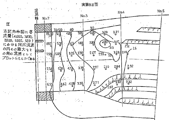
図-36 せき下流部流速分布図(河床最大流速)
