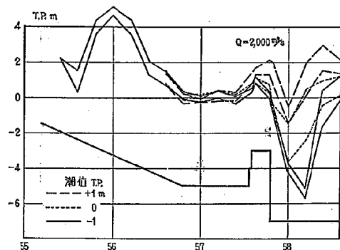
図-3.7 2-8 型 模型の水位縦断
