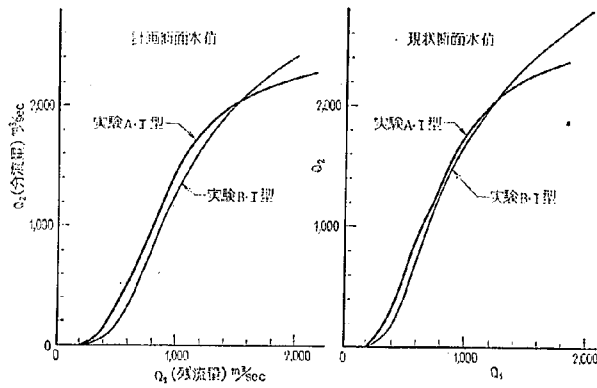
図-17 分流量 ( Q_2 ) と本川残流量 ( Q_1 ) I 型
