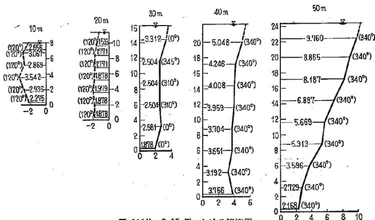
図-16(4) 2-15 型における流速図
