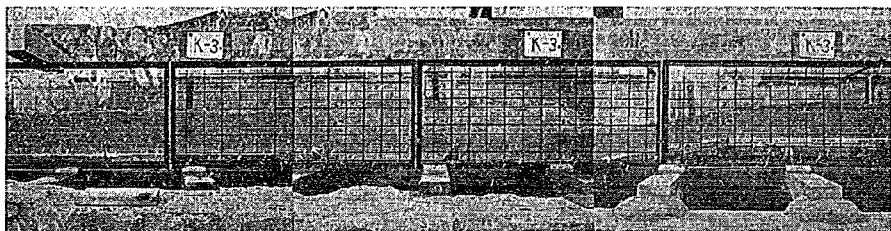
写真-3 1-3 型 模型における流況 (流量 1,000 \text{ m}^3/\text{sec} , 潮位 -1 \text{ m} , シル高 0 \text{ m} の場合)
