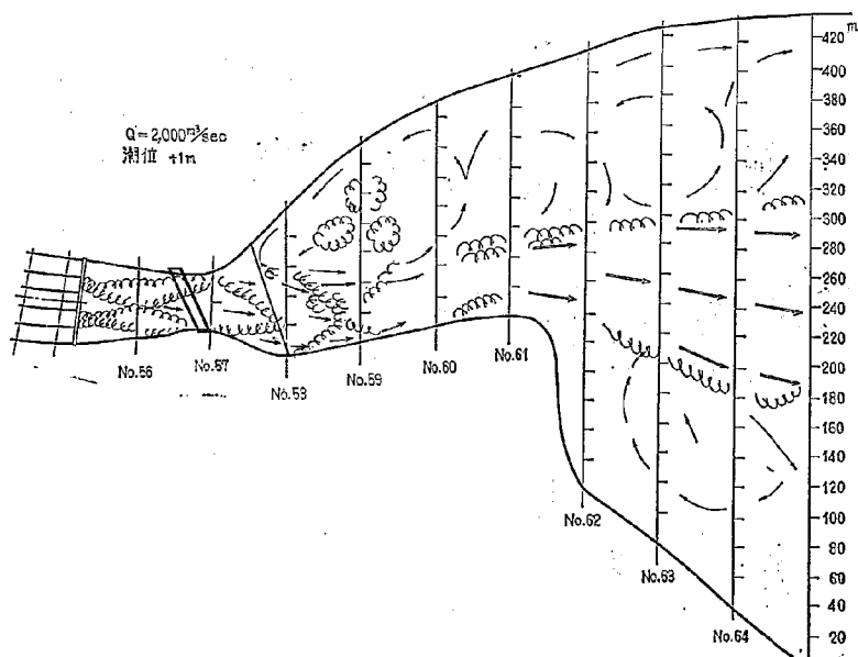
図-37(20) 流線スケッチ 模型形状 2-21 型 (右岸岩礁掘削 T.P-4.0m)
