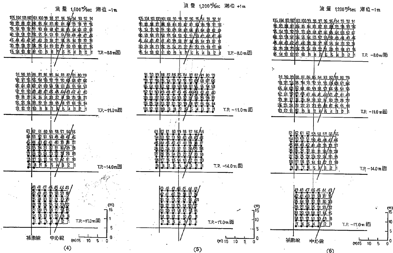
図-36 段落部下流側はどこまで洗掘されるか。黒丸は10分(模型で)通水後残存した標識立方体
