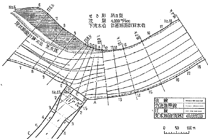
図-21 分流域せき付近流向図
