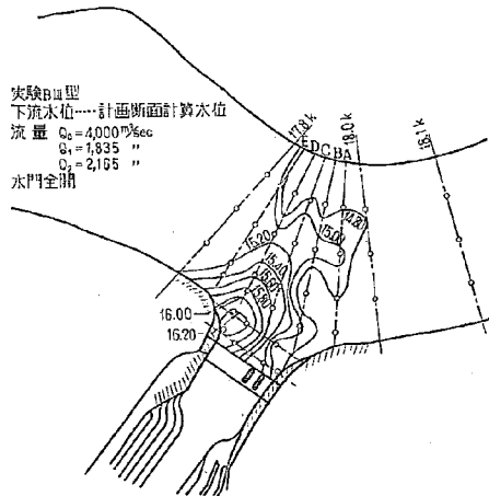
図-33 水位等高図
