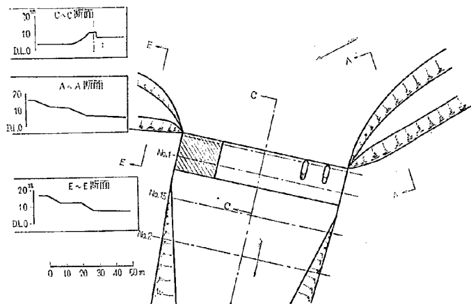
図-11 分流せき取付部形状図
