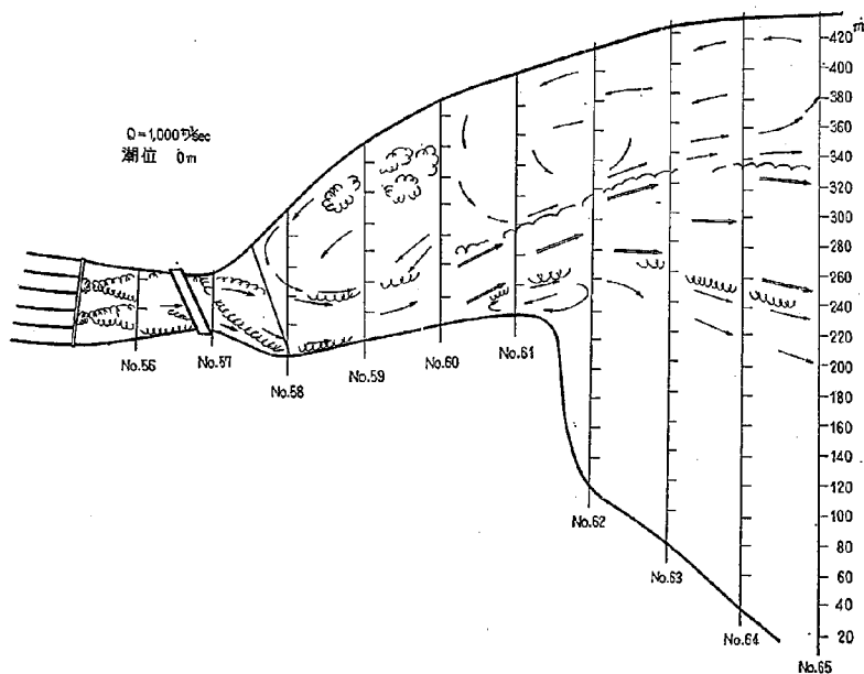
図-37(24) 流線スケッチ 模型形状 2-21 型 (右岸岩礁掘削 T.P-4.0m)
