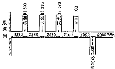
図-4 計画流量配分図
