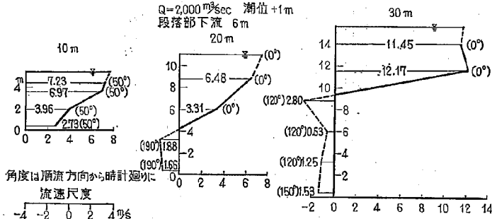
図-17(1) 2-16 型における流速図
