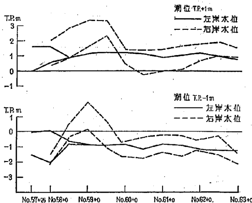
図-8 段落部下流海部両岸の水位
