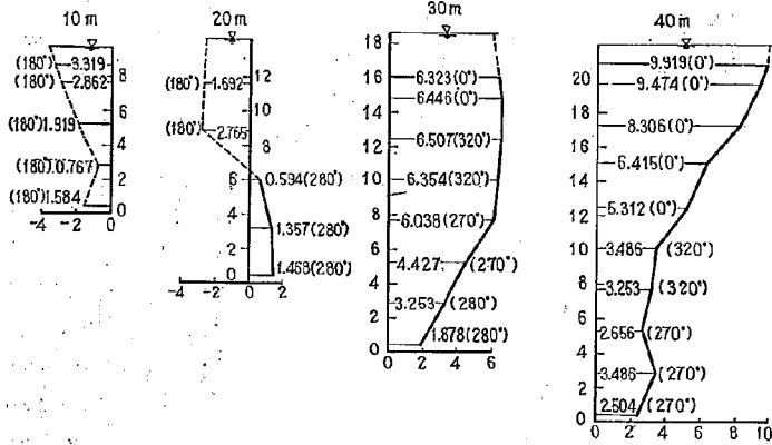
図-7(3) 2-12 型における流速図
