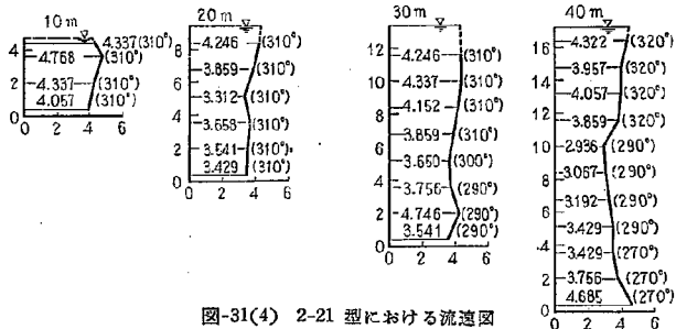
図-31(4) 2-21 型における流速図
