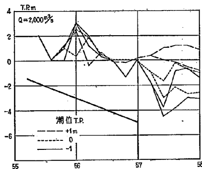
図-3.1 2-1 型模型の水位縦断
