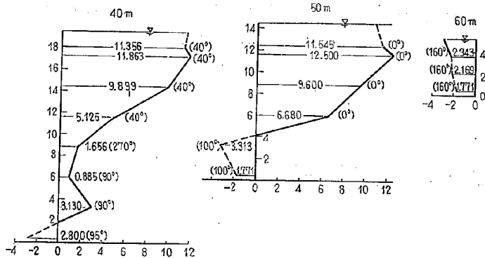
図-23(2) 2-18 型における流速図
