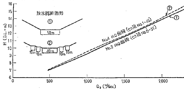
図-6 狩野川放水路 No. 2 (実験A), No. 4 (実験B) H, Q 曲線
