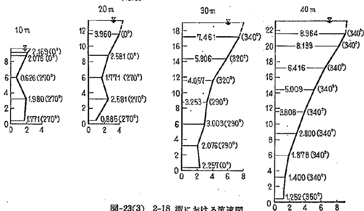
図-23(3) 2-18 型における流速図
