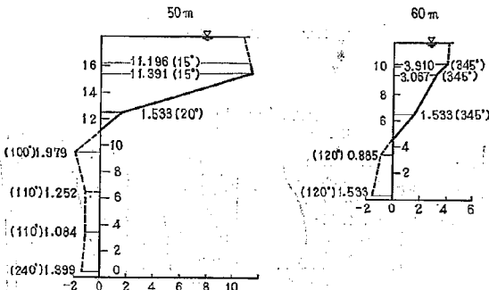
図-9(2) 2-13 型における流速図
