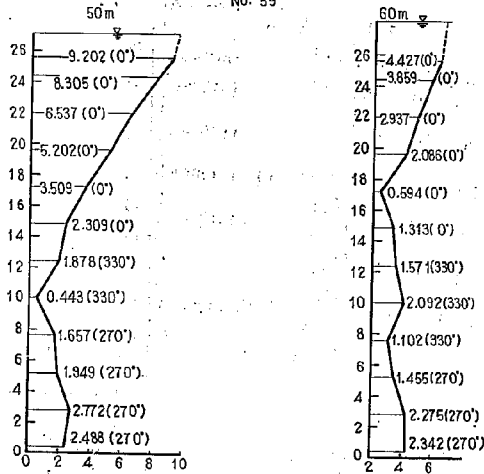
図-7(4) 2-12 型における流速図
