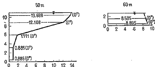
図-16(3) 2-15 型における流速図
