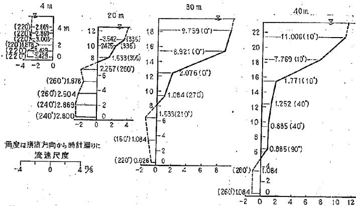
図-9(1) 2-13 型における流速図
