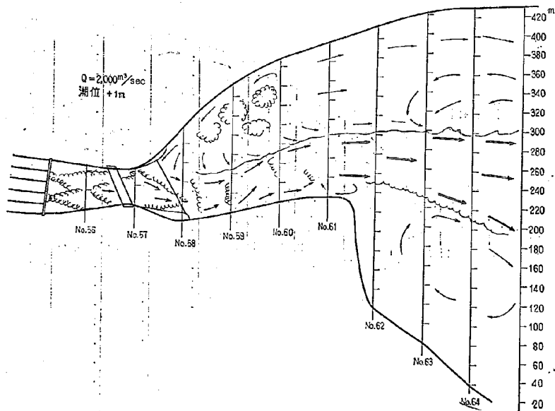
図-37(18) 流線スケッチ 模型形状 2-20 型
