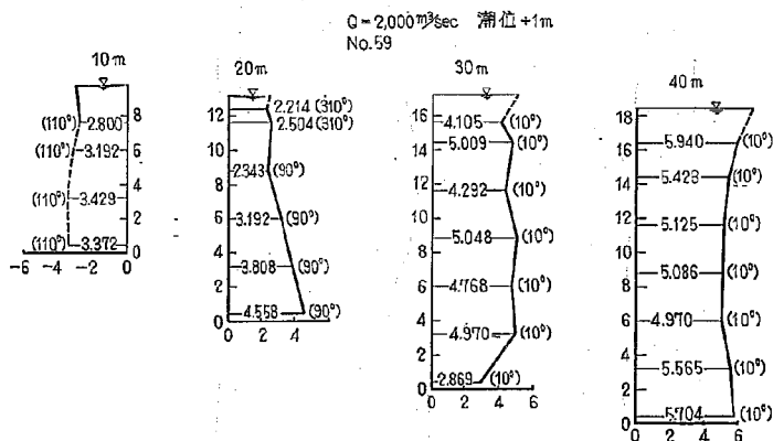
図-21(3) 2-17型における流速図
