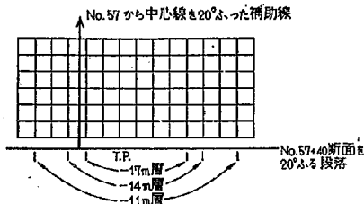
図-10.1 洗掘実験 (2-21 型)
