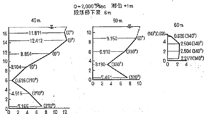
図-21(2) 2-17型における流速図
