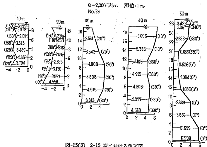
図-15(3) 2-15 型における流速図
