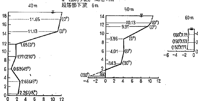
図-17(2) 2-16 型における流速図
