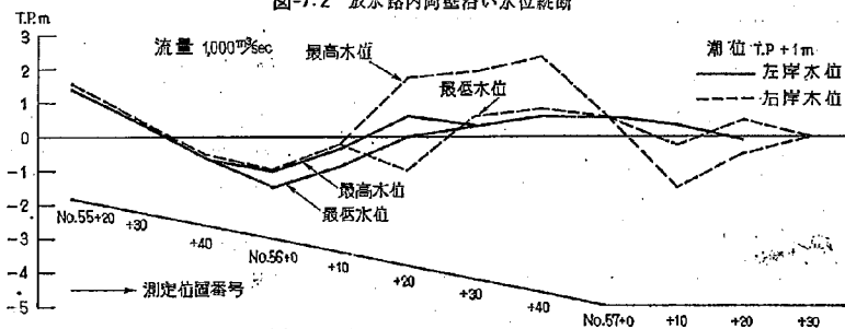
図-7.3 放水路内両壁沿い水位縦断
