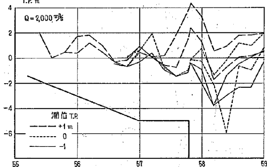
図-3.14 2-13 型 模型水位の縦断
