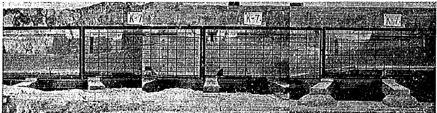
写真-7 1-3 型 模型における流況 (流量 1,000 \text{ m}^3/\text{sec} , 潮位 -1 \text{ m} , シル高 1 \text{ m} の場合)
