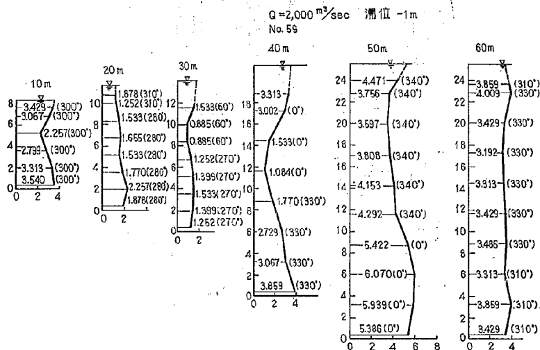
図-18(3) 2-16 型における流速図
