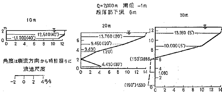
図-18(1) 2-16 型における流速図
