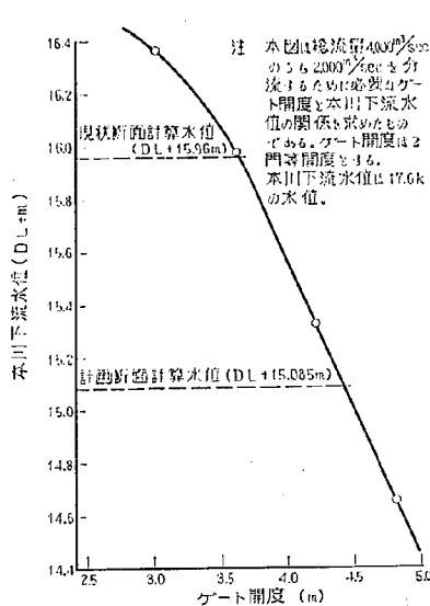
図-29 下流水位とゲート開度
