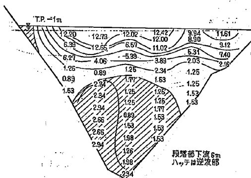
図-5.10 2-21 型 流量 2,000 m³/sec, 潮位 T.P. -1 m
