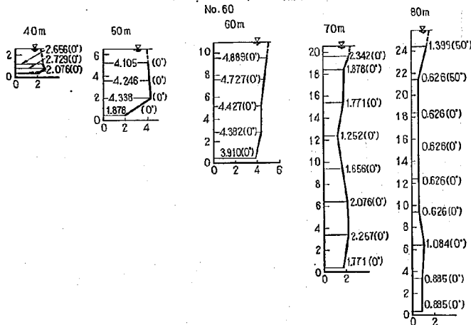
図-10(5) 2-13 型における流速図
