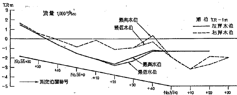
図-7.4 放水路内両壁沿い水位変動
