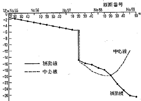
図-20 模型河床縦断
