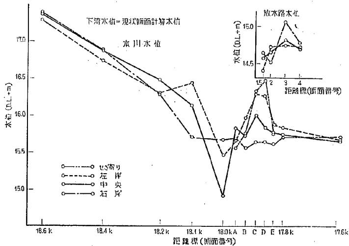
図-19 水位縦断面 Q_0=1,000\text{m}^3/\text{sec} (II 型)
