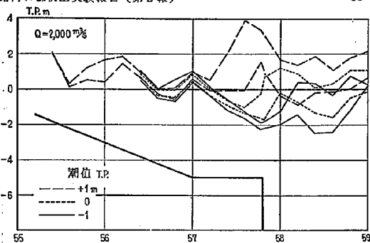
図-3.13 2-12 型 模型水位の縦断
