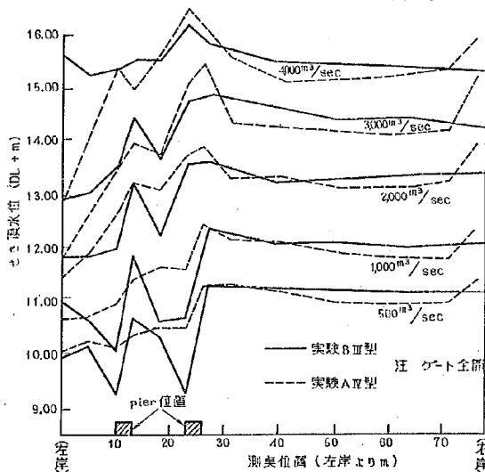
図-23 (2) せき頂横断水位 (現状断面計算水位)
