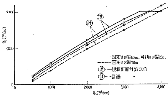
図-22(2) Q_0-Q_2 曲線(実験A-II, III型)
