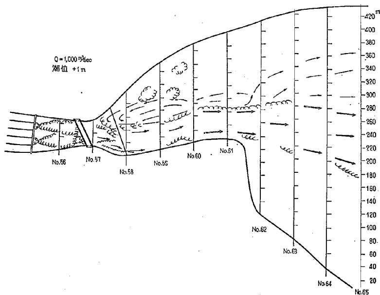
図-37(23) 流線スケッチ 模型形状 2-21 型 (右岸岩礁掘削 T.P-4.0m)
