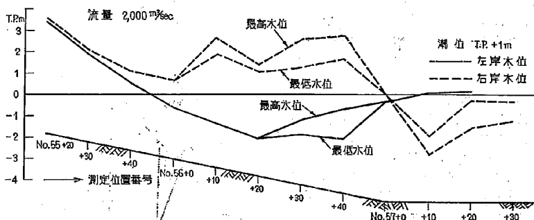
図-7.1 放水路内両壁沿い水位縦断
