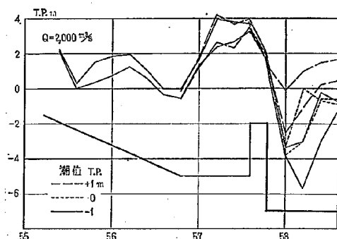
図-3.9 2-10 型 模型の水位縦断
