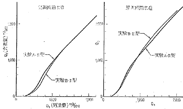
図-18 分流量 ( Q_2 ) と本川残流量 ( Q_1 ) II 型
