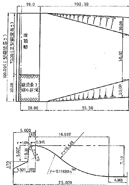
図-10 分流せき形状図 (I型, II型)
