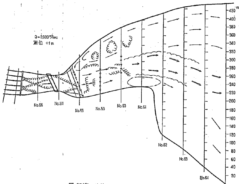
図-37(6) 流線スケッチ 模型形状 2-14 型
