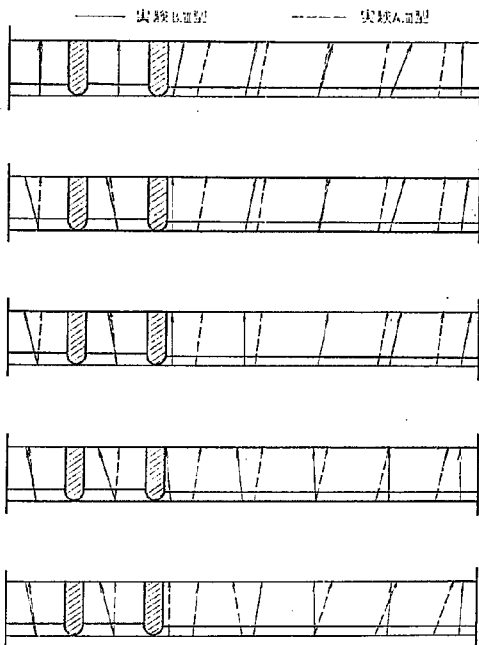
図-24 せき頂流向比較図
