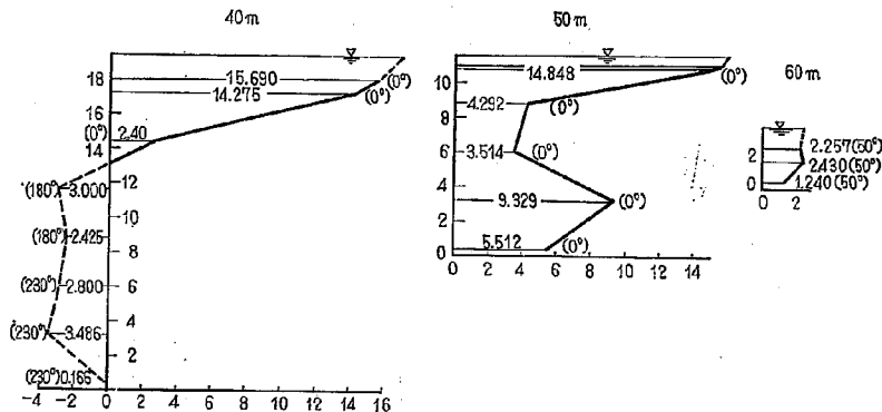
図-22(2) 2-17 型における流速図
