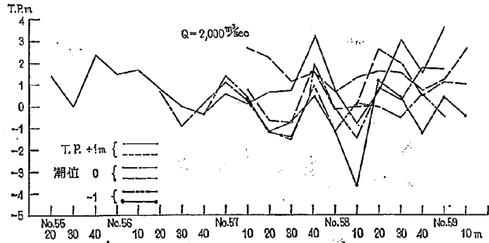
図-4 2-14 型模型における水位縦断面図
