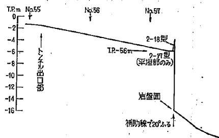
図-2.8 2-17型、2-18型 縦断面
