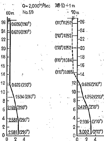
図-17(4) 2-16型における流速図
