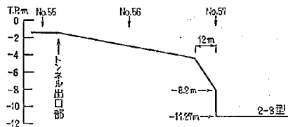
図-2.2 2-3 型 縦断面図
