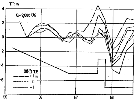
図-3.6 2-7 型 模型の水位縦断
