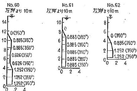
図-30(7) 2-21 型における流速図
