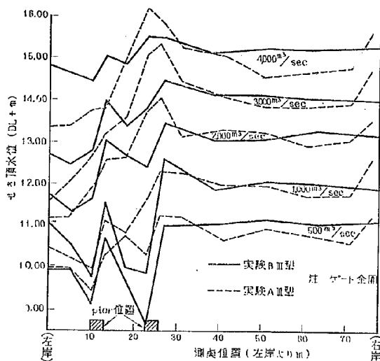
図-23 (1) せき頂横断水位 (計画断面計算水位)
