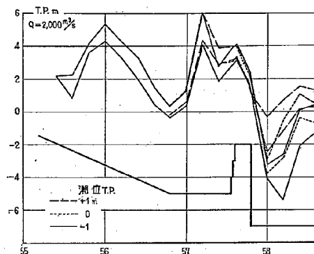
図-3.8 2-9 型 模型の水位縦断
