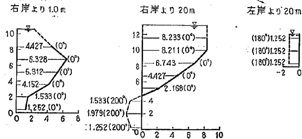
図-31(9) 2-21 型における流速図 (No. 58, 59 両岸近くの流速)
