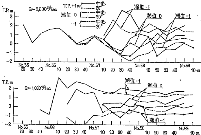
図-2 2-12型模型における水位縦断面図
