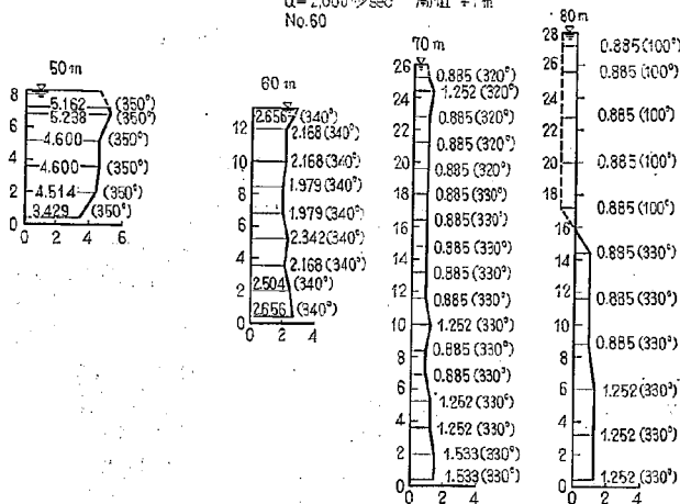
図-30(6) 2-21 型における流速図
