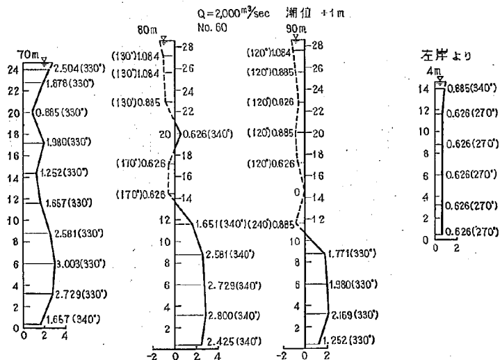
図-17(6) 2-16 型における流速図
