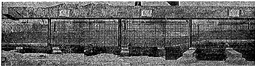
写真-4 1-3 型 模型における流況 (流量 1,000 \text{ m}^3/\text{sec} , 潮位 0 \text{ m} , シル高 0 \text{ m} の場合)
