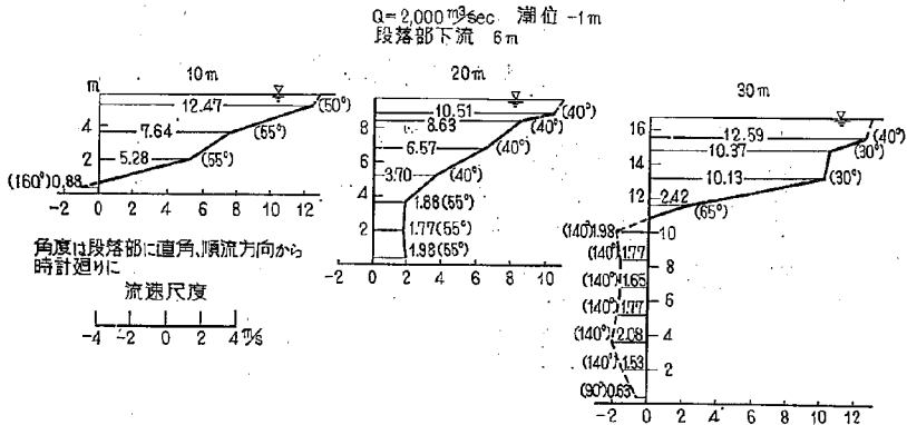
図-28(1) 2-20 型における流速図
