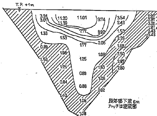
図-5.3 2-13 型 流量 2,000 m³/sec, 潮位 T.P. +1m
