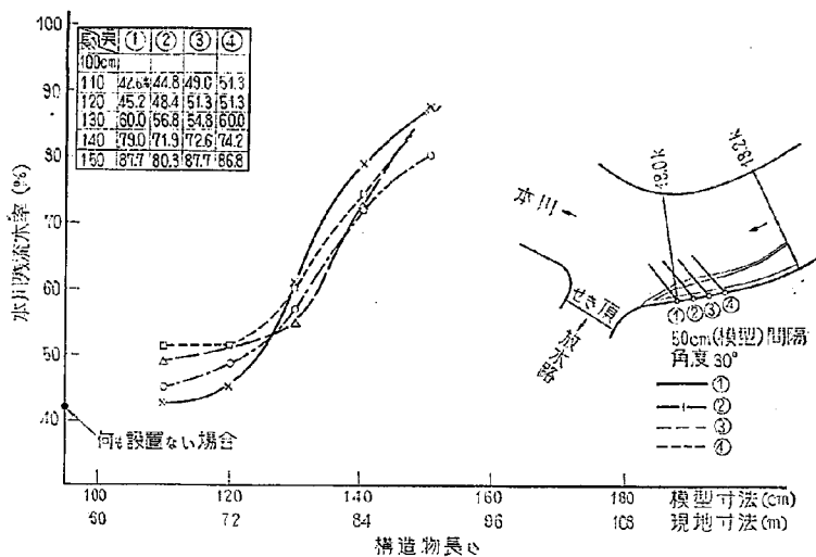
図-39 流木対策関係図
