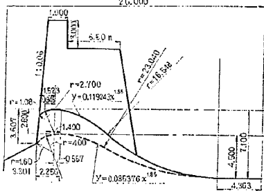
図-15 分流せき形状図(Ⅲ型)
