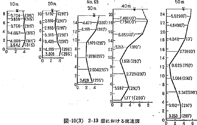
図-10(3) 2-13型における流速図
