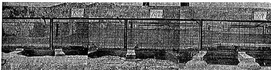
写真-9 1-3 型 模型における流況 (流量 815 \text{ m}^3/\text{sec} , 潮位 -1 \text{ m} , シル高 2 \text{ m} の場合)
