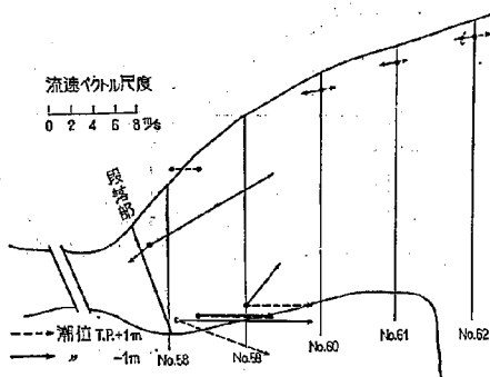
図-9 2-21 型, 2,000 m³/sec, 岸ぞい測点における最大流速ベクトル
