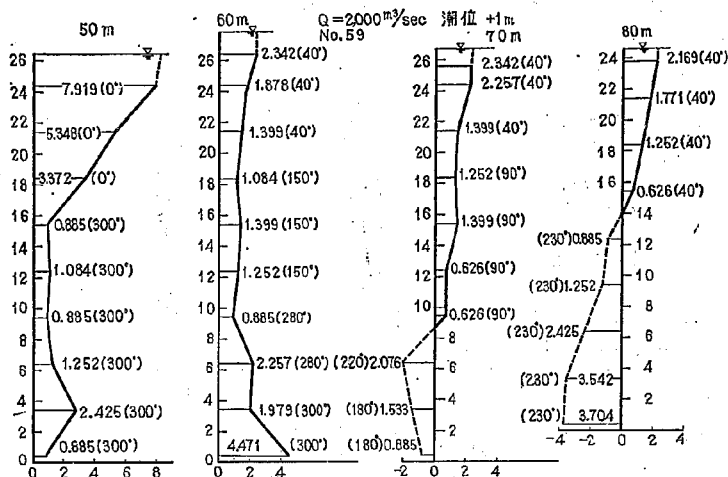
図-9(4) 2-13 型における流速図
