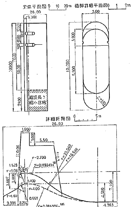
図-12 分流せき形状図(Ⅲ型)
