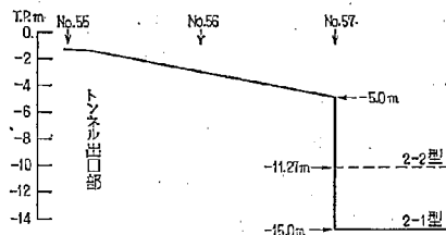
図-2.1 2-1 型、2-2 型 縦断面図
