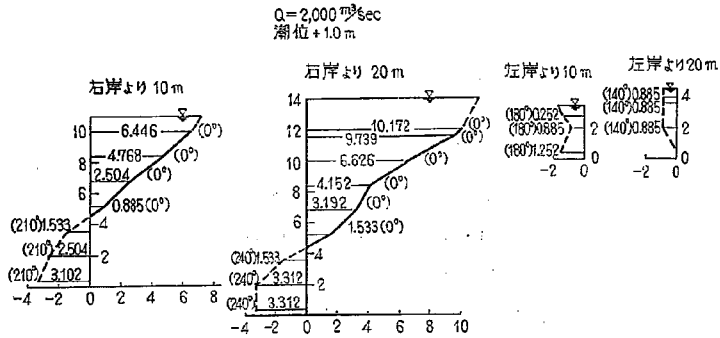
図-30(8) 2-21 型における流速 (No. 58, 両岸近くの流速)
