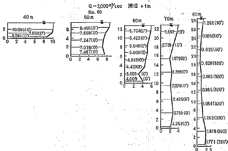
図-9(5) 2-13 型における流速図
