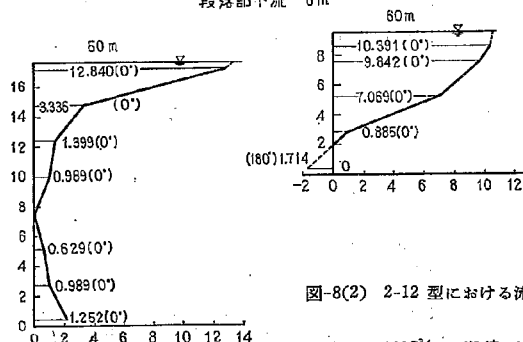
図-8(1) 2-12 型における流速図
