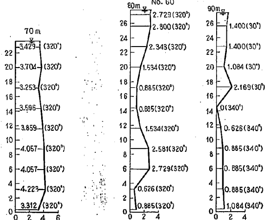
図-21(6) 2-17 型における流速図
