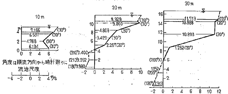
図-23(1) 2-18 型における流速図
