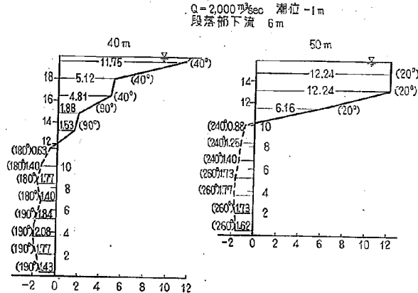
図-28(2) 2-20 型における流速図
