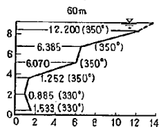
図-31(3) 2-21 型における流速図
