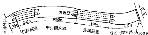
図-3 放水路略図
