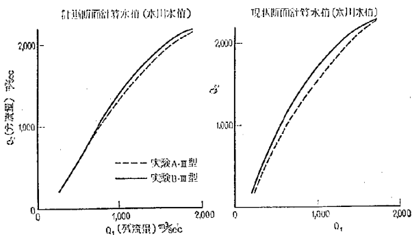
図-22(1) 分流量( Q_2 )と本川残流量( Q_1 ) III型
