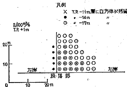
図-10.2 流量 2,000 m³/sec, 潮位 T.P. +1m
