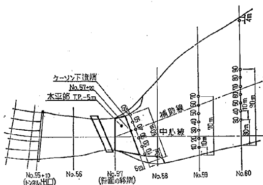
図-13 2-15 型, 2-16 型流速測定位置平面図
