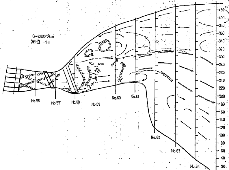
図-37(2) 流線スケッチ 模型形状 2-12 型
