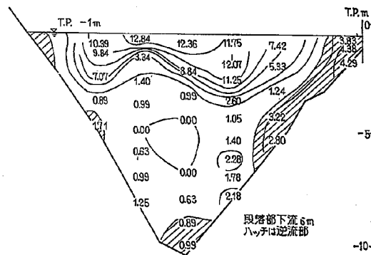
図-5.2 2-12 型 流量 2,000 m³/sec, 潮位 T.P. -1m
