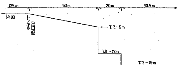
図-1.4 1-4型模型
