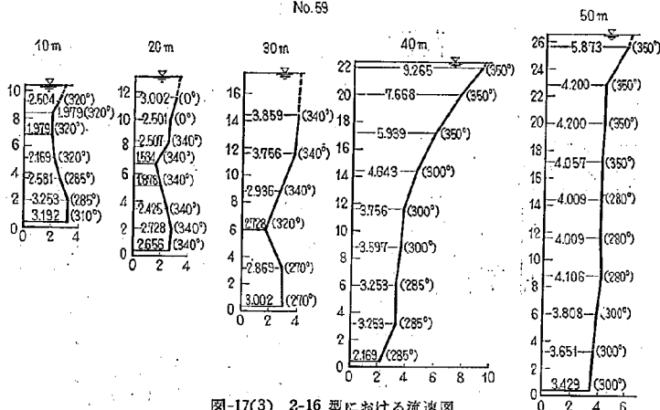
図-17(3) 2-16型における流速図
