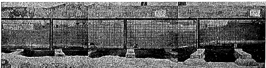
写真-5 1-3 型 模型における流況 (流量 2,000 \text{ m}^3/\text{sec} , 潮位 -1 \text{ m} , シル高 1 \text{ m} の場合)
