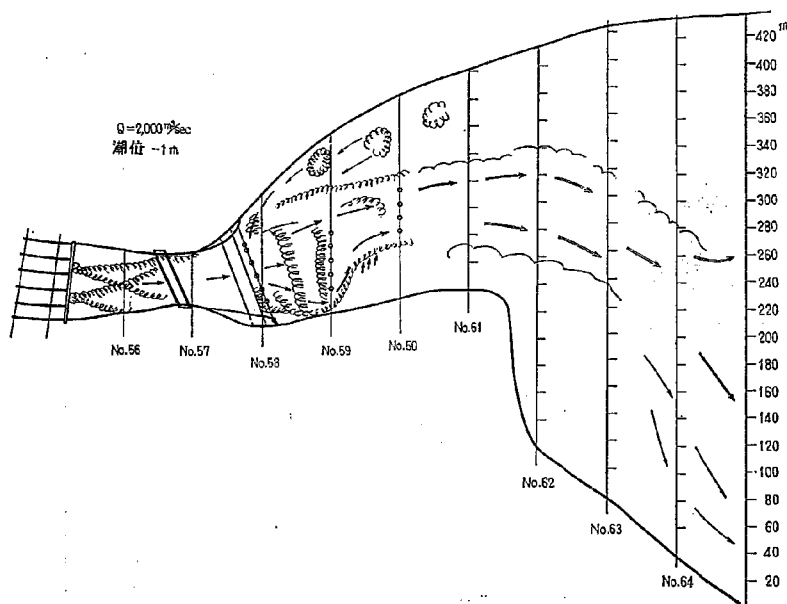
図-37(7) 流線スケッチ 模型形状 2-14 型
