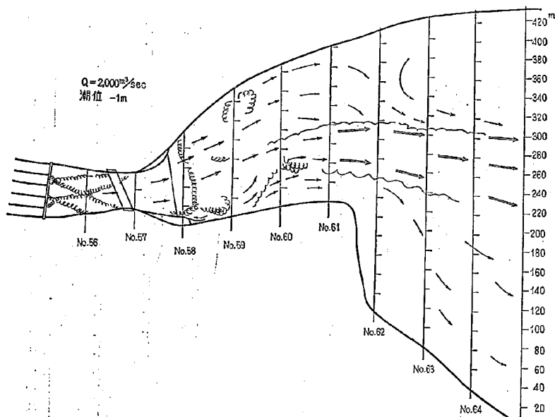
図-37(17) 流線スケッチ 模型形状 2-19 型
