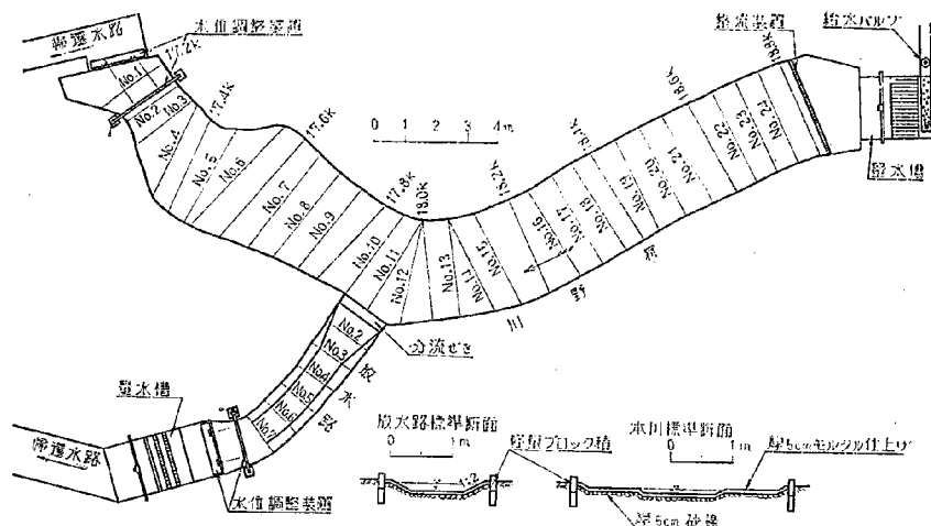
図-8 狩野川分流せき水理実験模型図
