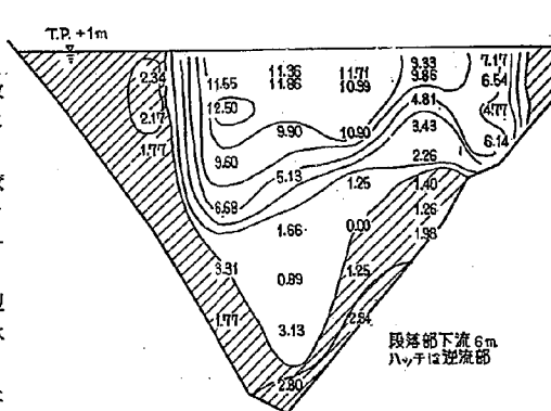
図-5.7 2-18 型 流量 2,000 m 3 /sec, 潮位 T.P. +1m
