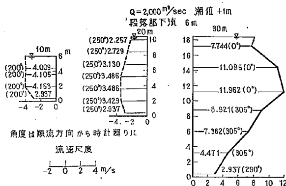
図-21(1) 2-17型における流速図
