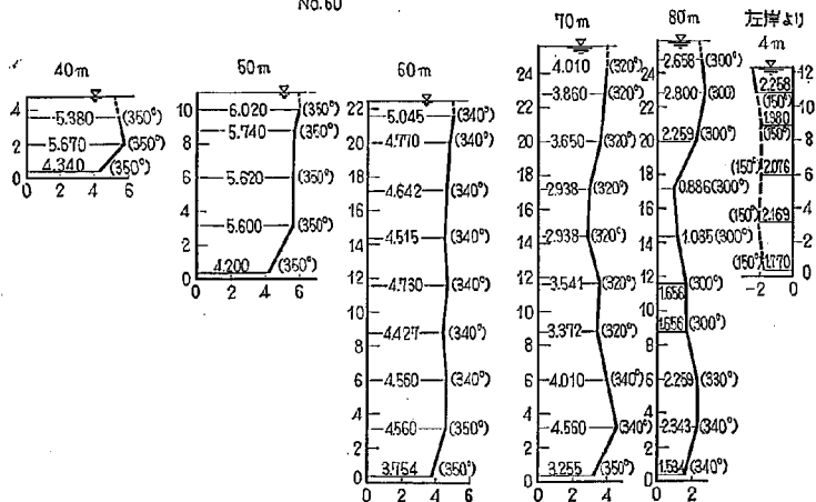
図-16(6) 2-15 型における流速図
