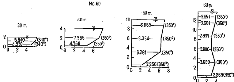
図-23(5) 2-18 型における流速図
