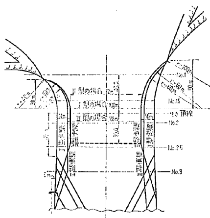
図-14 分流せき上・下流取付形状(Ⅱ型) 側壁比較 I型(固定せきのみ長さ100m) Ⅲ型(橋脚部省略)
