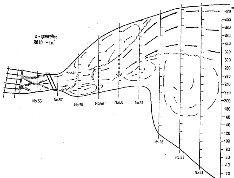
図-37(13) 流線スケッチ 模型形状 2-17 型
