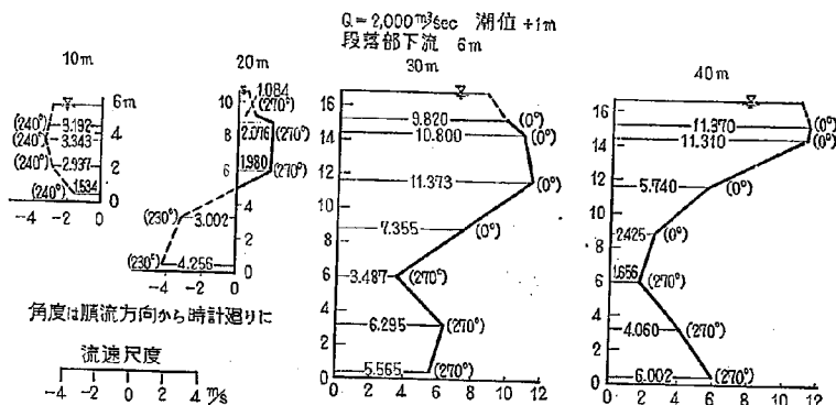
図-15(1) 2-15 型における流速図
