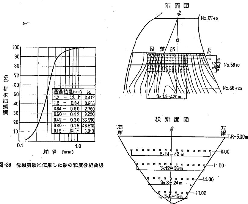
図-34 段落部下流側洗掘実験の標識立方体配置図
