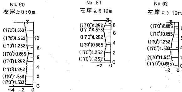
図-31(8) 2-21 型における流速図
