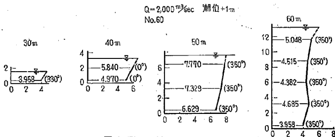
図-17(5) 2-16型における流速図
