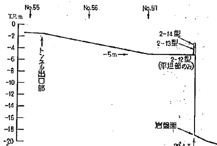
図-2.6 2-12 型, 2-13 型, 2-14 型 縦断面図
