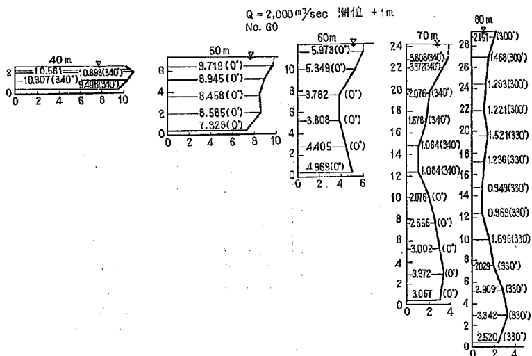
図-7(5) 2-12 型における流速図
