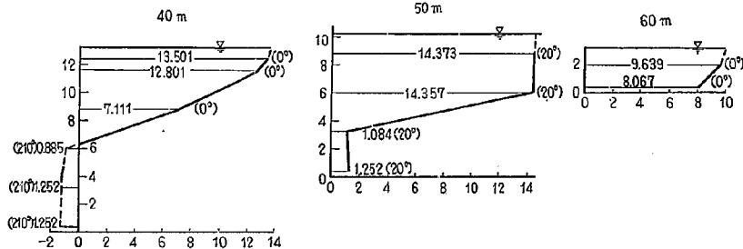
図-24(3) 2-18 型における流速図
