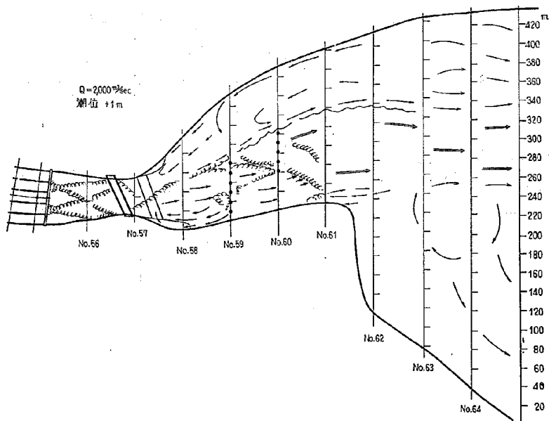
図-37(8) 流線スケッチ 模型形状 2-15 型
