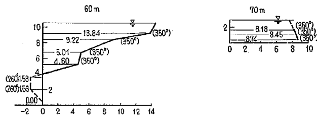
図-28(3) 2-20 型における流速図
