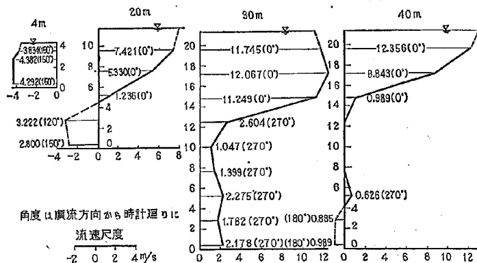
図-8(1) 2-12 型における流速図
