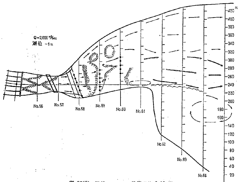
図-37(5) 流線スケッチ 模型形状 2-13 型
