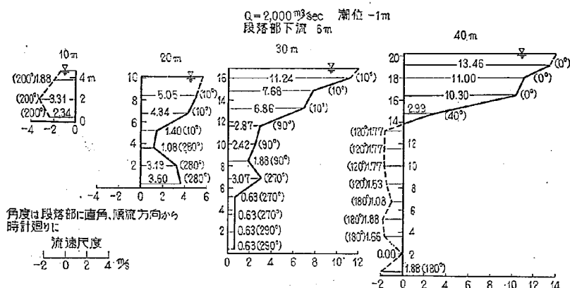
図-26(1) 2-19 型における流速図
