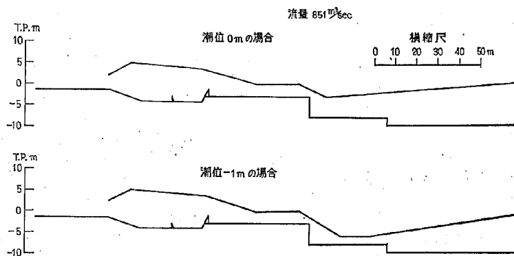
図-1.3.4 シル高 2m の 1-3 型 模型における水位縦断
