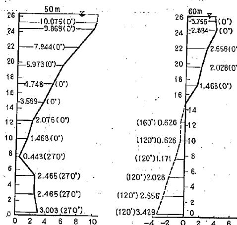
図-8(4) 2-12 型における流速図
