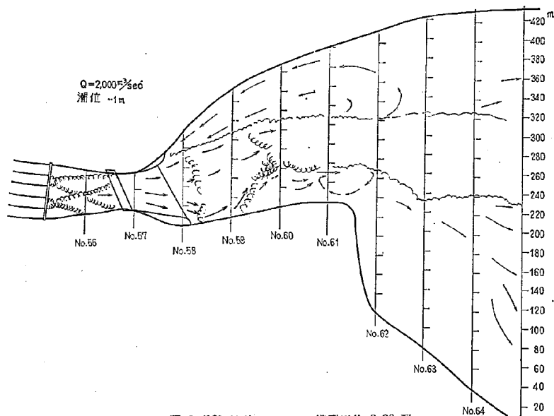
図-37(19) 流線スケッチ 模型形状 2-20 型
