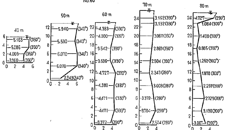
図-24(6) 2-18 型における流速図
