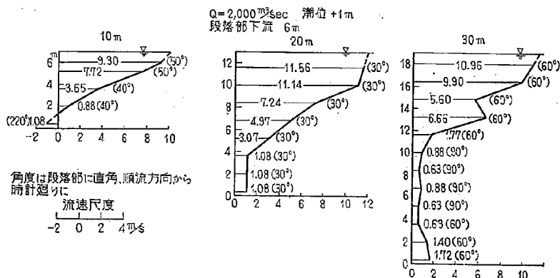
図-27(1) 2-20 型における流速図
