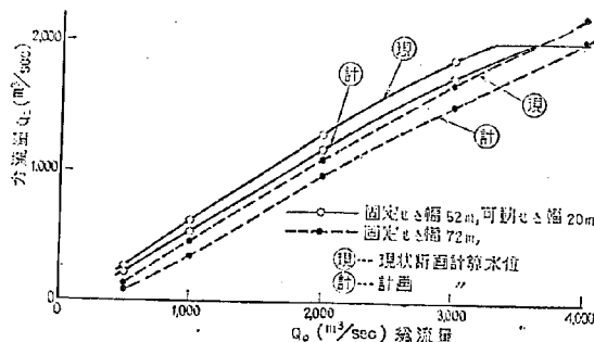
図-40 Q_0 - Q_2 曲線 (実験B-I, Ⅲ型)
