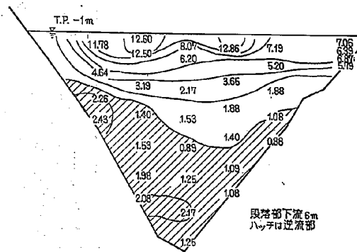
図-5.4 2-13 型 流量 2,000 m³/sec, 潮位 T.P. -1m
