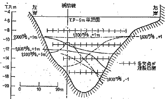
図-11 段落部直下における立方体の残存状況
