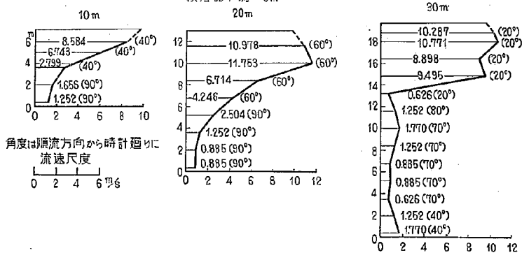
図-30(1) 2-21 型における流速図 (岩礁掘削 T. P. -4m)
