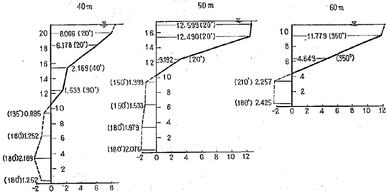
図-10(2) 2-13型における流速図
