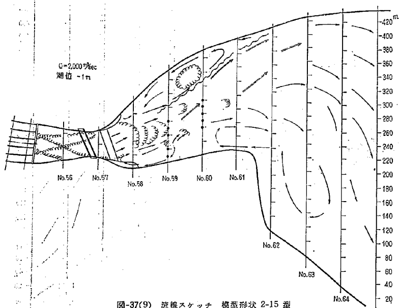
図-37(9) 流線スケッチ 模型形状 2-15 型
