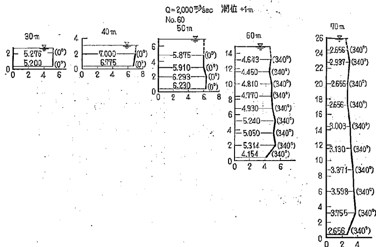
図-15(5) 2-15 型における流速図
