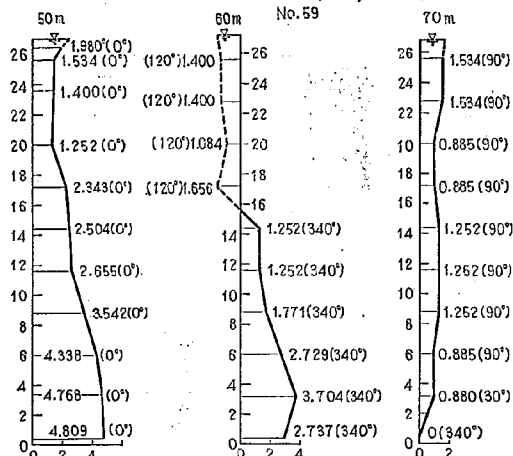
図-21(4) 2-17 型における流速図
