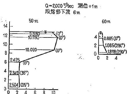
図-15(2) 2-15 型における流速図
