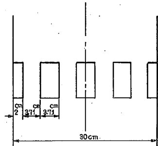
図-1.3.1 バッフルピア配置平面図(模型)
