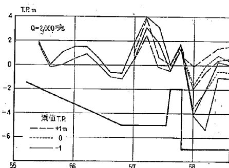
図-3.10 2-11 型 模型水位の縦断
