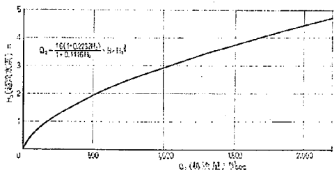
図-7 狩野川放水路越流せき、水位—越流量曲線
