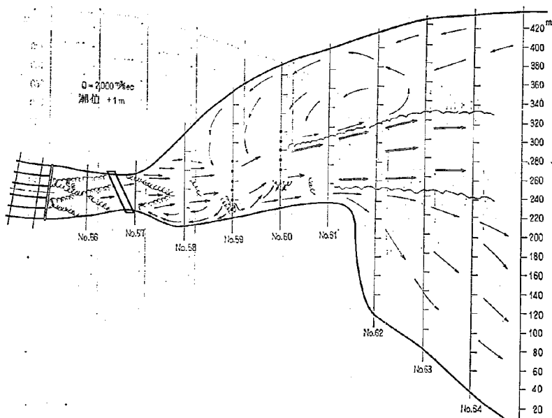
図-37(12) 流線スケッチ 模型形状 2-17 型
