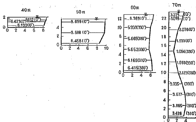
図-8(5) 2-12 型における流速図
