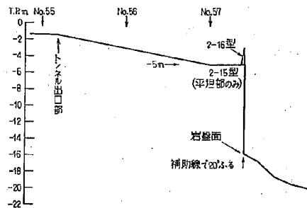
図-2.7 2-15型、2-16型 縦断面
