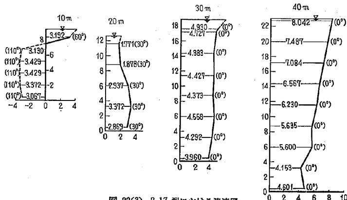
図-22(3) 2-17 型における流速図
