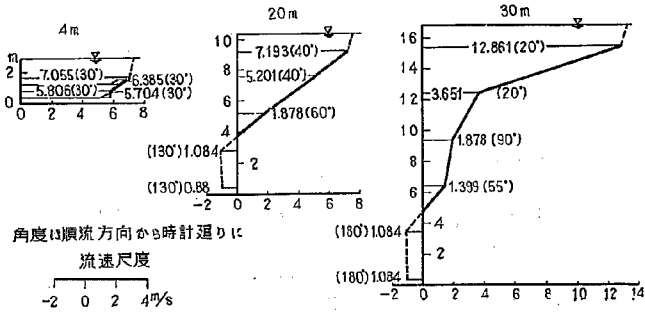
図-10(1) 2-13型における流速図
