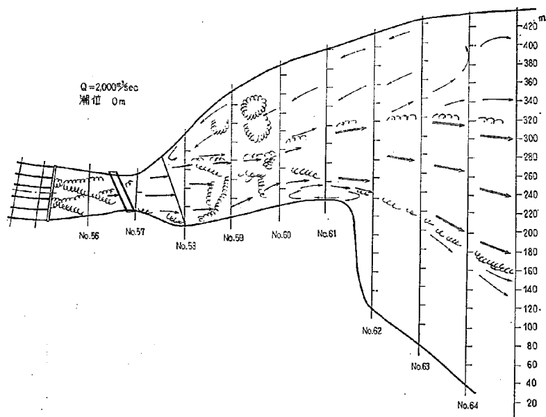
図-37(21) 流線スケッチ 模型形状 2-21 型 (右岸岩礁掘削 T.P. -4.0 m)
