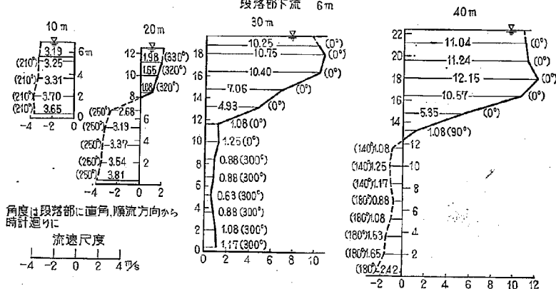
図-25(1) 2-19 型における流速図
