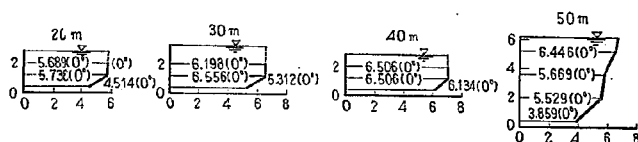
図-31(6) 2-21 型における流速図
