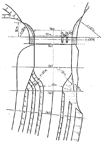
図-16 分流せき上・下流取付形状(Ⅲ型)
