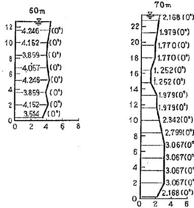
図-31(7) 2-21 型における流速図
