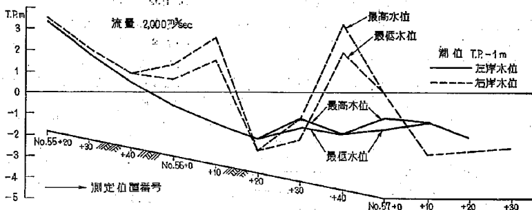
図-7.2 放水路内両壁沿い水位縦断
