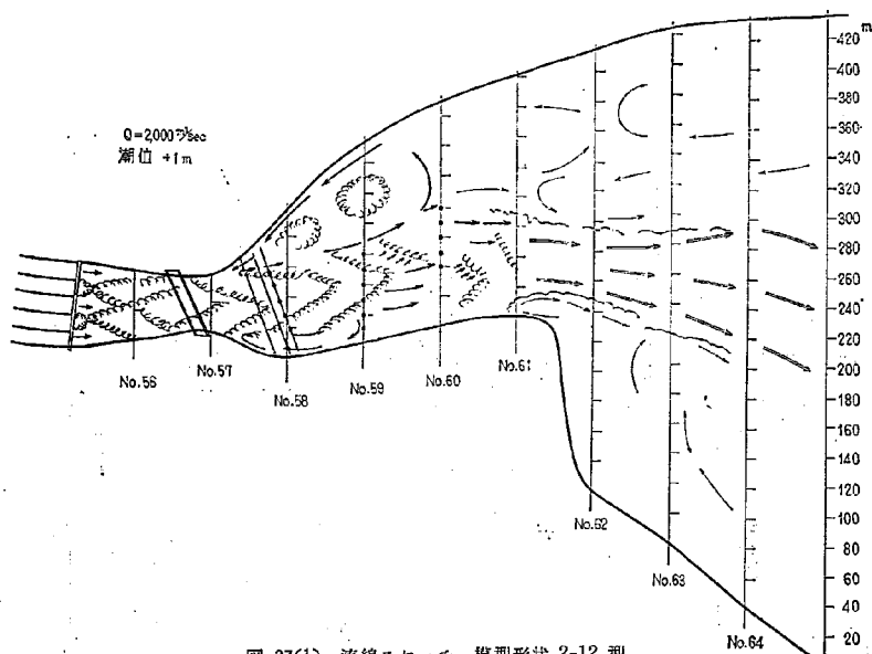
図-37(1) 流線スケッチ 模型形状 2-12 型
