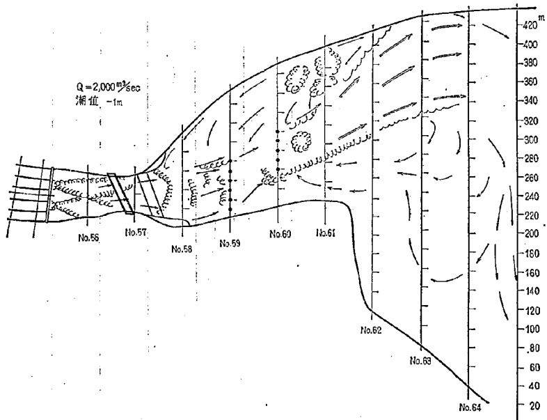
図-37(15) 流線スケッチ 模型形状 2-18 型
