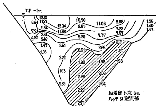
図-5.6 2-14 型 流量 2,000 m³/sec, 潮位 T.P. -1m
