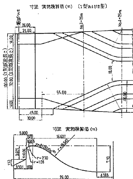
図-13 分流せきおよび下流取付け形状図
