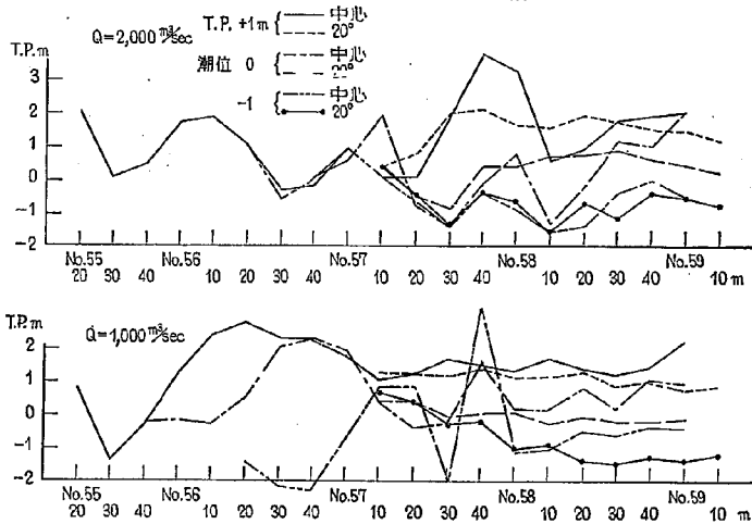
図-3 2-13型模型における水位縦断面図
