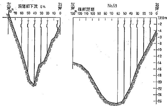
図-6(1) 流速測定位置横断面図
