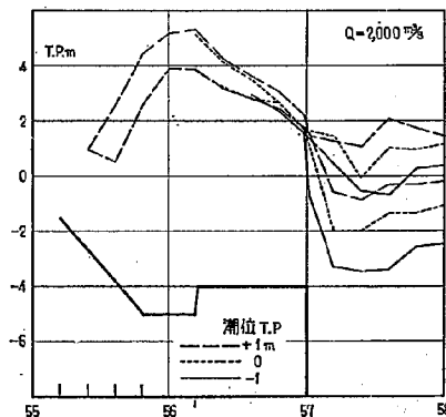
図-3.3 2-4 型 模型の水位縦断
