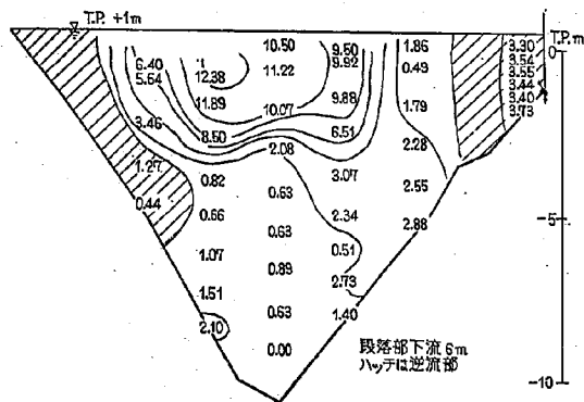
図-5.1 2-12 型 流量 2,000 m³/sec, 潮位 T.P. +1m
