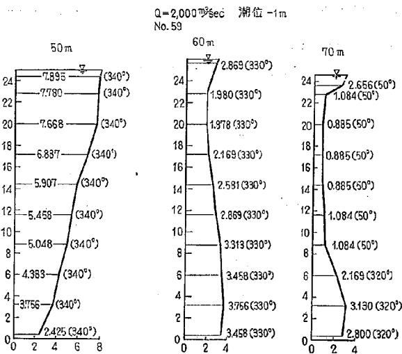
図-24(5) 2-18 型における流速図
