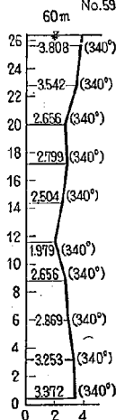
図-16(5) 2-15 型における流速図
