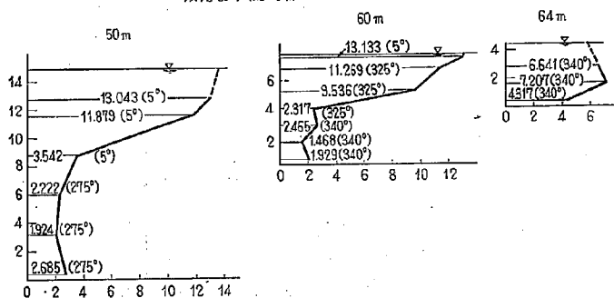
図-12(2) 2-14 型における流速図
