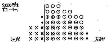
図-10.3 流量 2,000 m³/sec, 潮位 T.P. -1m
