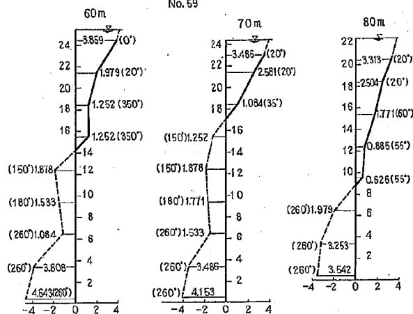
図-10(4) 2-13 型における流速図
