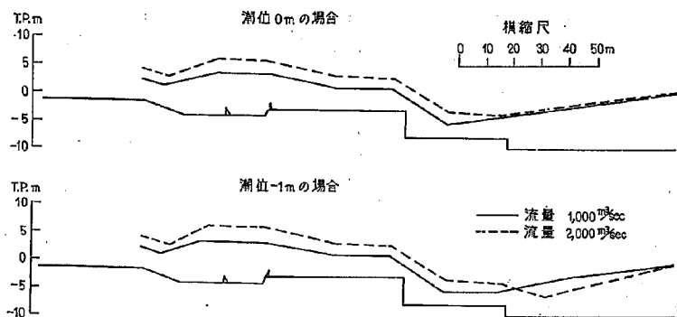
図-1.3.3 シル高 1m の 1-3 型 模型における水位縦断
