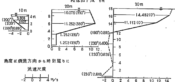
図-22(1) 2-17 型における流速図
