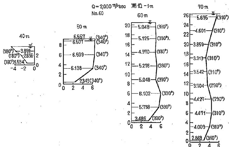
図-22(5) 2-17 型における流速図
