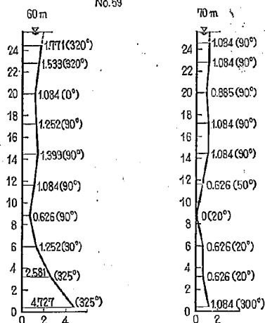
図-15(4) 2-15 型における流速図
