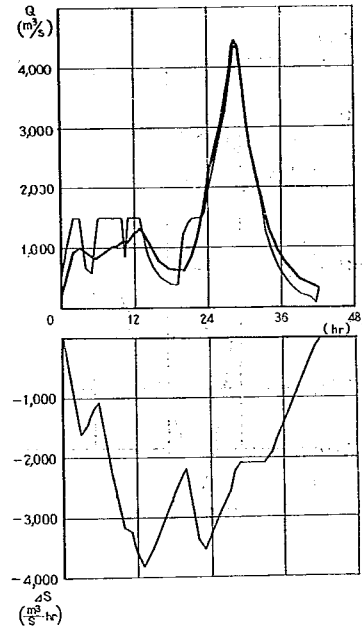
洪水番号 10 風 屋 ( D_2 )
