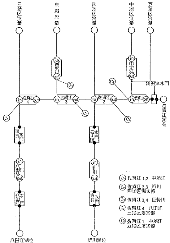
図-28 佐賀江川回路図
