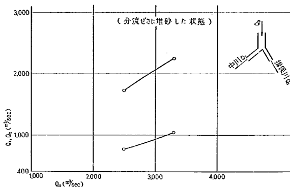
図-25 総流量 ( Q_0 ) と分流量 ( Q_2 ) および残流量 ( Q_1 )
