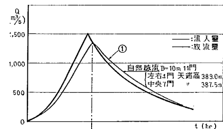
図-8② 小森ダム ( D_i ) の洪水処理方式
