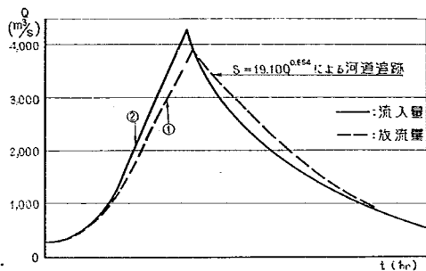
図-8① 二津野ダム ( D_s ) 洪水処理方式
