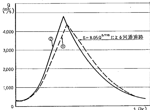
図-8② 小森ダム ( D_i ) の洪水処理方式
