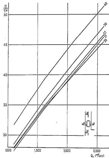
図-13 各断面計算水位—流量曲線
