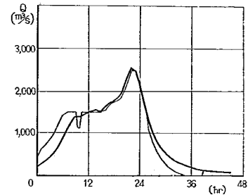
洪水番号 6 風 屋 ( D_2 )
