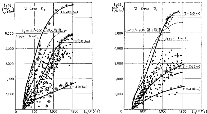
図-15 流入量 I_D ~ 総予備放流量 |\Delta S|
