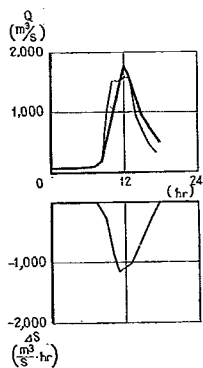
洪水番号 7 池 原 ( D_3 )
