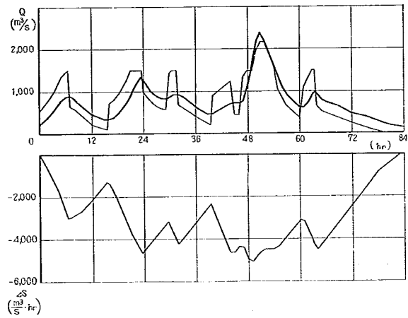
洪水番号 18 池 原 ( D_5 )
