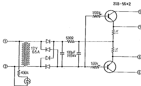
図-20 R 部回路図
