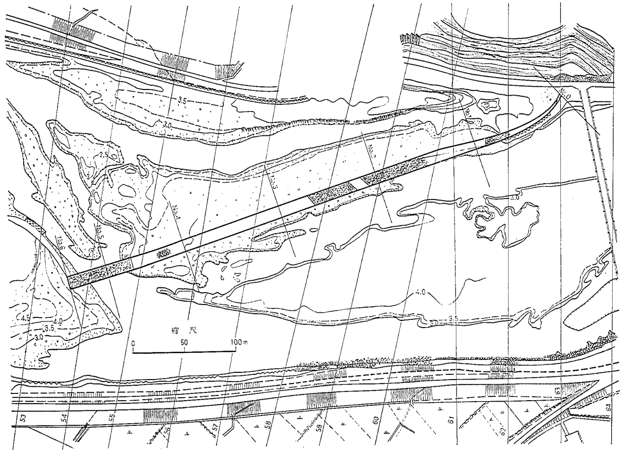
図-21 掛保川分流せき平面図
