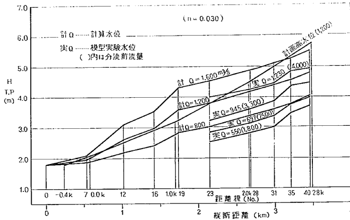
図-5 揖保川水位縦断面図
