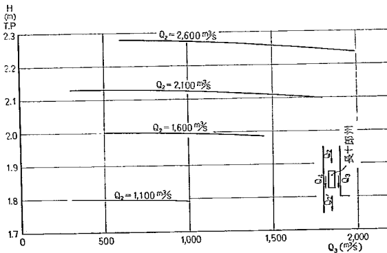
図-9 中川No.8 (元川合流前) 計算水位—流量曲線
