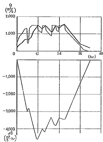
洪水番号 13 風 屋 ( D_2 )
