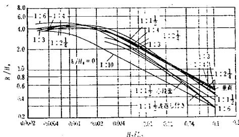
図-3 堤脚水深が0のときのうちあげ高 (Saville)
