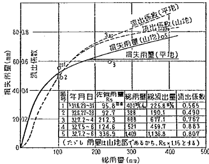
図-23 流出係数曲線図 徳永川(念仏橋)
