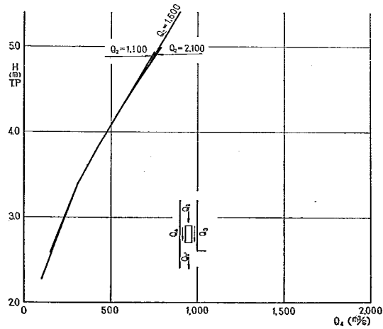
図-16 元川No.21 計算水位—流量曲線
