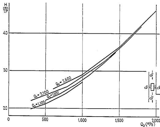
図-11 中川No.18 (元川分流後) 計算水位—流量曲線
