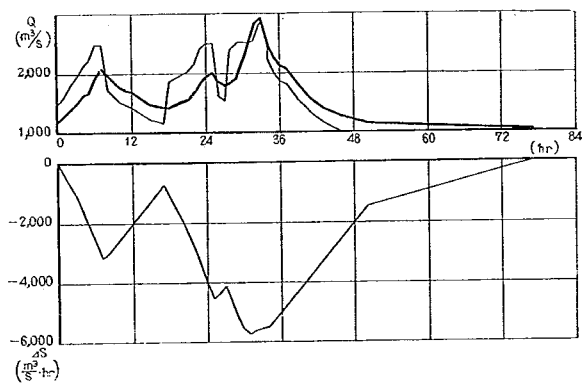
洪水番号 13 池 原 ( D_3 )
