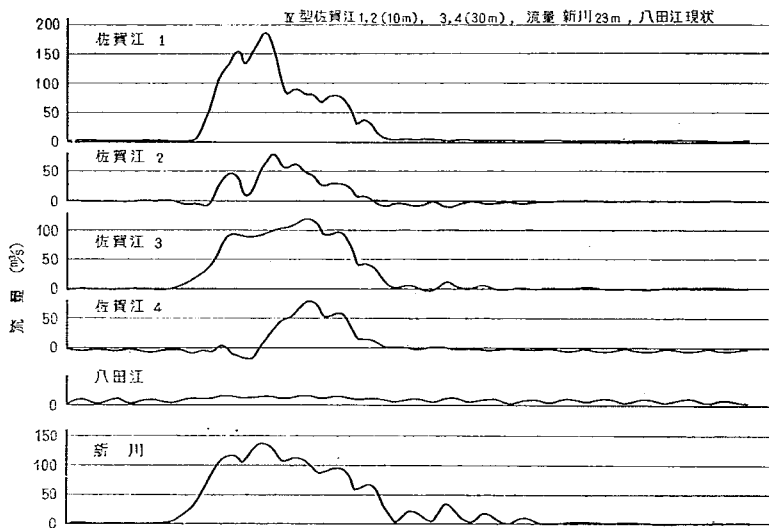
圖-31 IV型洪水流量曲線
