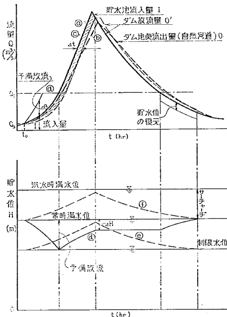
図-4 利水ダム洪水処理基本図(模式図)
