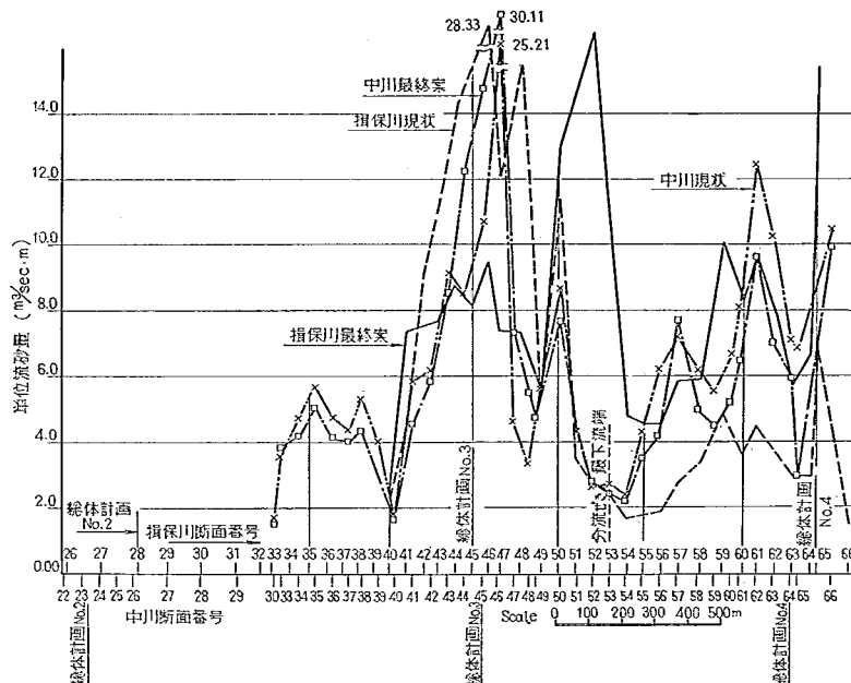
図-40 単 位 幅 流 砂 量
