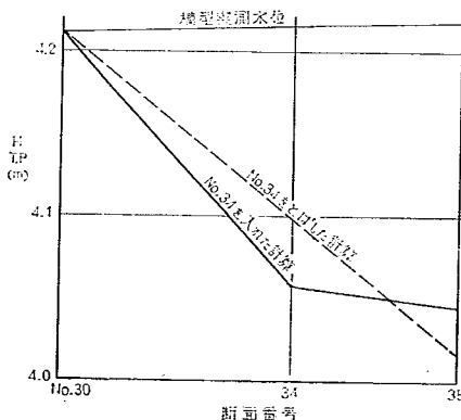
図-20 No.35 断面水位図
