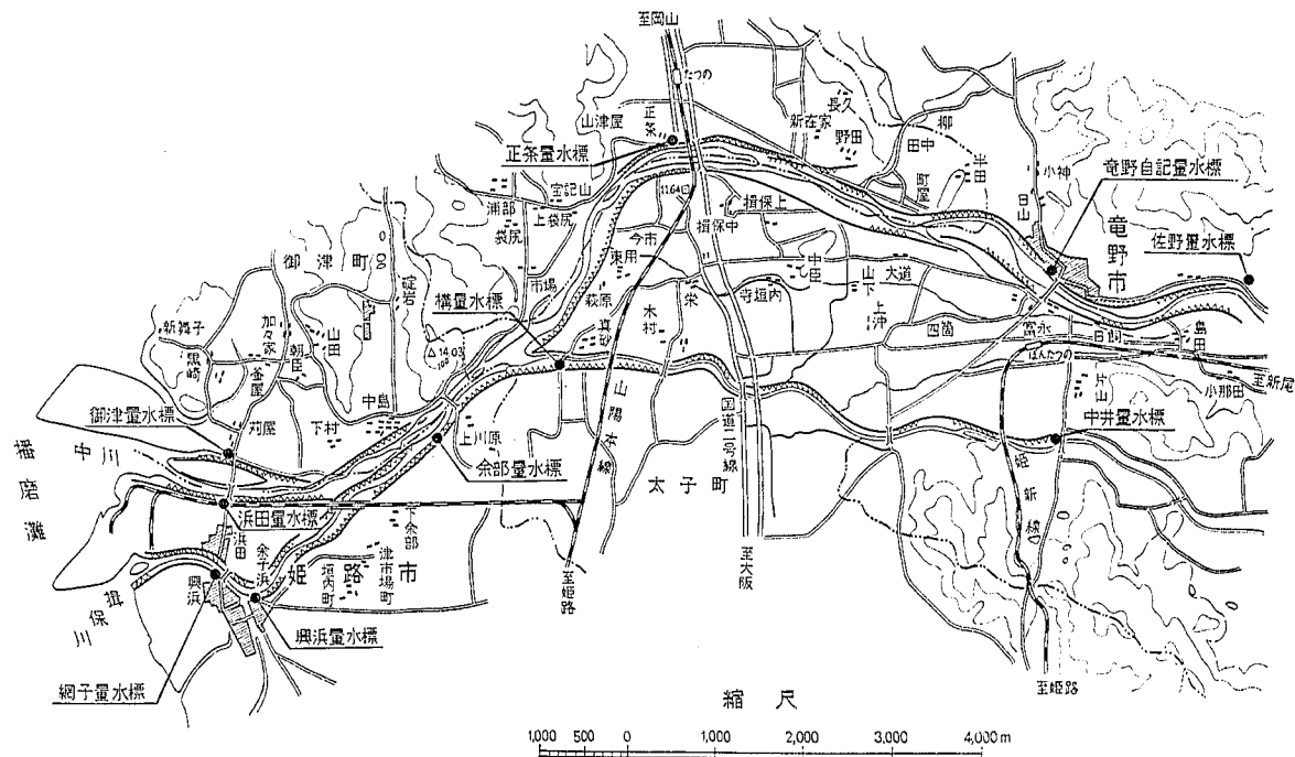
図-2 揖保川下流平面図
