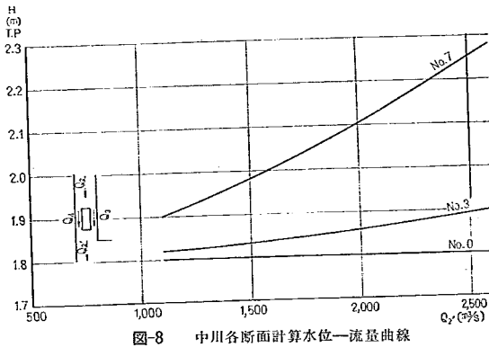
図-8 中川各断面計算水位—流量曲線
