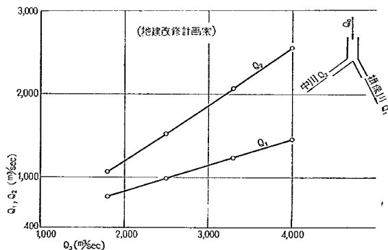
図-34 総流量 ( Q_0 ) と分流量 ( Q_2 ) および残流量 ( Q_1 )
