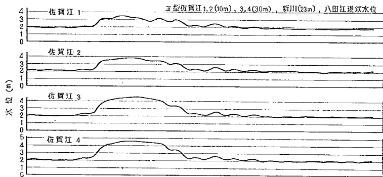
圖-30 IV型洪水水位曲線
