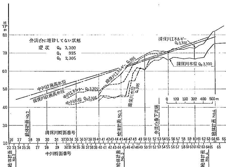
図-28 実験水位縦断面図
