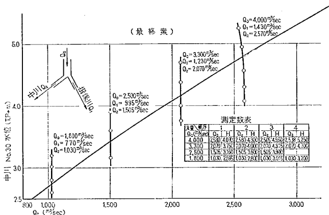
図-35 各流量時の中川No.30水位と分流量 ( Q_2 )
