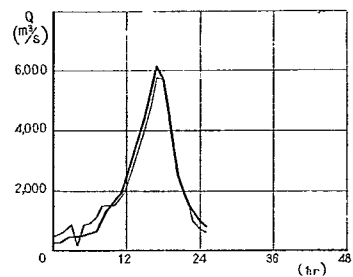
洪水番号 14 伊 屋 ( D_1 )
