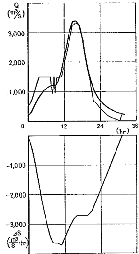
洪水番号 2 風 屋 ( D_2 )
