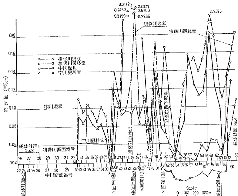
図-39 流砂量縦断面図
