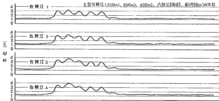
圖-29 III型洪水水位曲線
