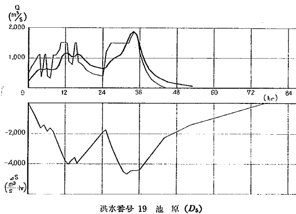
参考図 貯水池流入量・貯水放流量・貯水量の変化図
