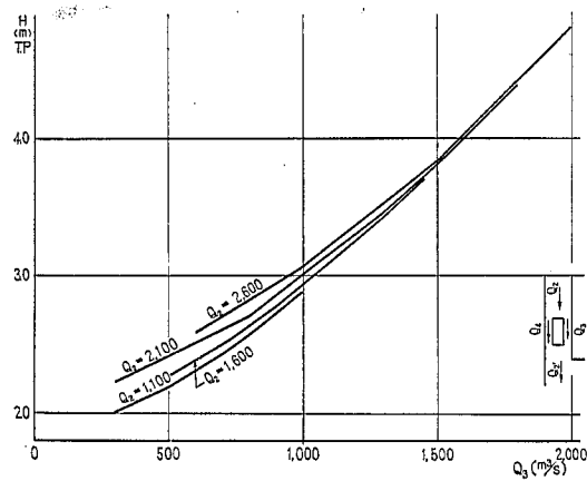
図-12 中川No.21 (元川分流後) 計算水位—流量曲線
