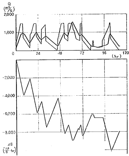
洪水番号 18 風 屋 ( D_2 )
