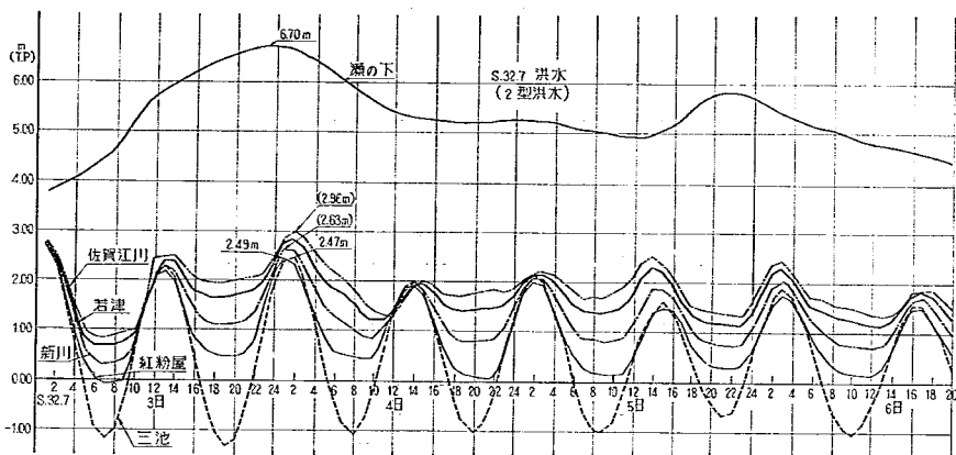
図-27 S.32.7月洪水時の水位曲線
