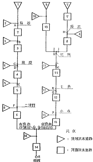
図-2 熊野川洪水解析系統図(自然状態)
