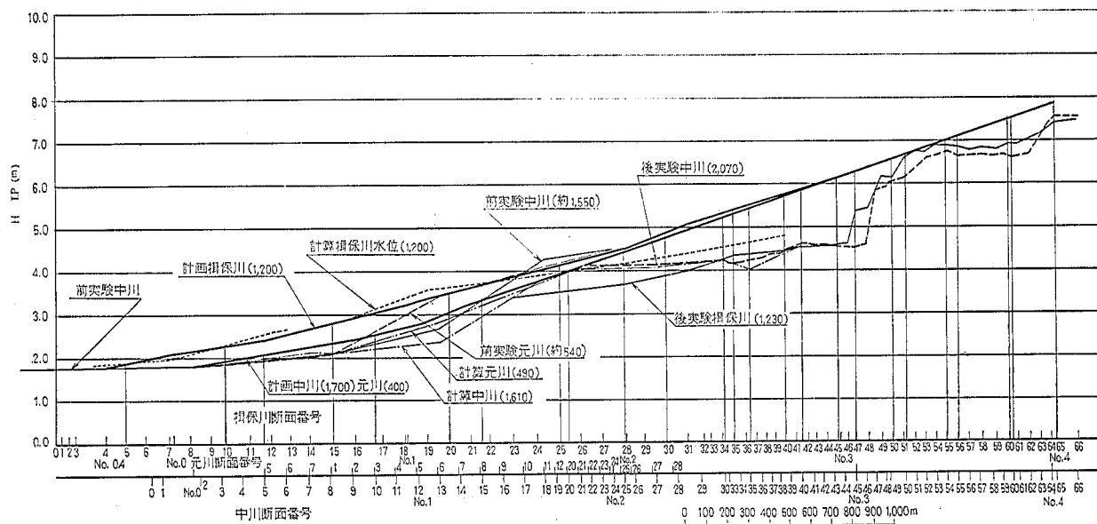
図-17 各水位比較図
