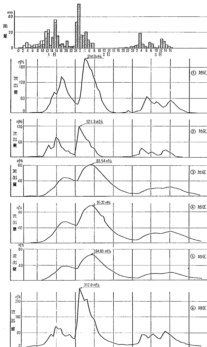
図-24 Ⅱ型降雨に対する各地区よりの流出量
