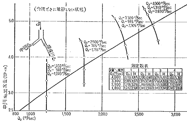
図-22 各流量時の中川 No.30 水位と分流量 ( Q_2 )
