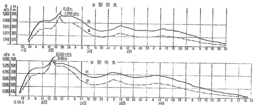
図-26 筑後本川の水位、流量曲線図(瀬ノ下地点)
