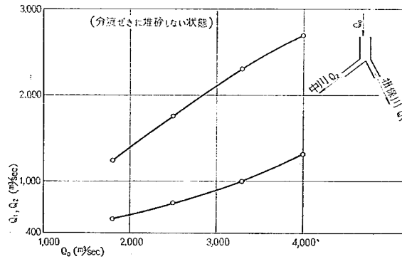
図-23 総流量 ( Q_0 ) と分流量 ( Q_2 ) および残流量 ( Q_1 )
