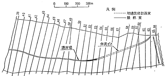
図-31 改修計画改造平面図
