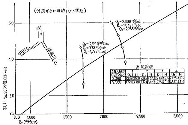
図-24 各流量時の中川 No.30 水位と分流量 ( Q_2 )
