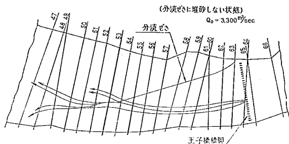
図-30 分 流 点 流 向 図
