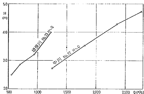
図-29 両派川支配断面 H \sim Q
