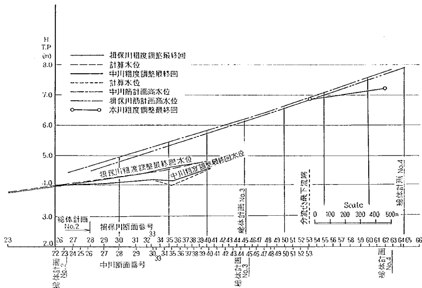
図-19 粗度調整水位縦断面図
