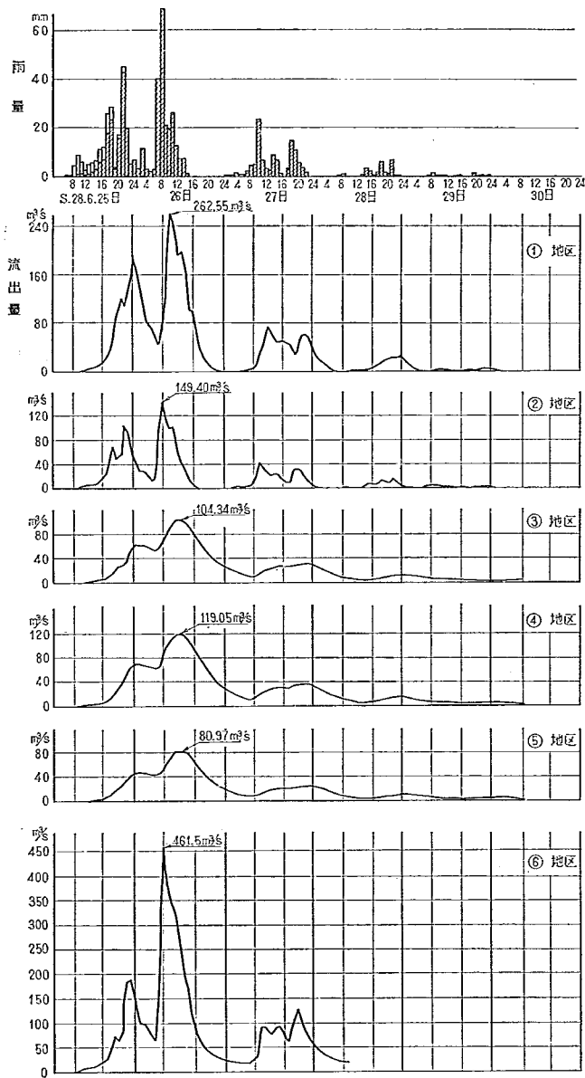
図-25 IV型降雨に対する各地区よりの流出量
