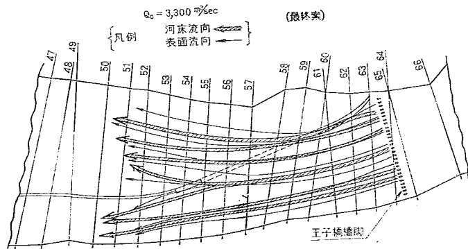
図-38 分流せき付近河床および表面流向図
