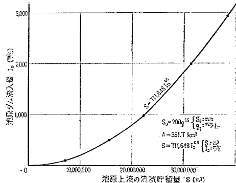
図-12 池原流域貯留量曲線
