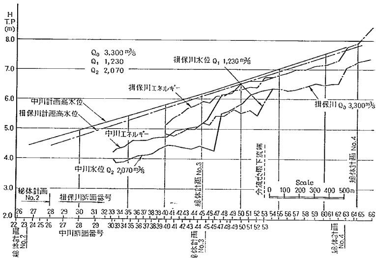
図-37 最終案実験水位縦断面図
