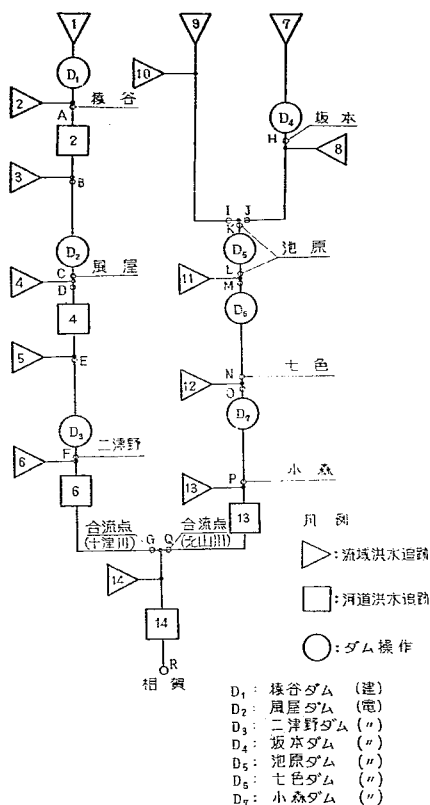
図-3 熊野川洪水解析系統図 (ダムカット)
