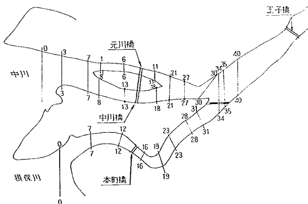
図-4 不等流計算断面位置図
