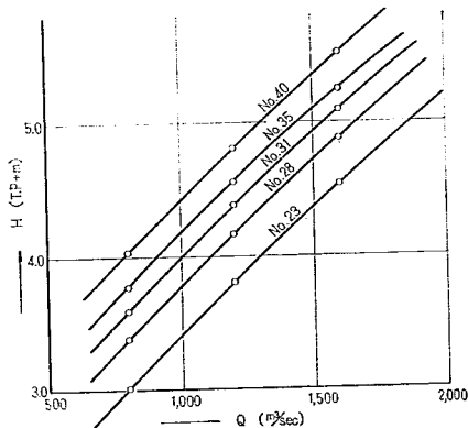
図-6 揖保川各断面計算水位～流量曲線
