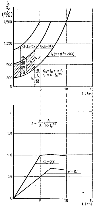
図7 流域貯留を考慮した予備放流
