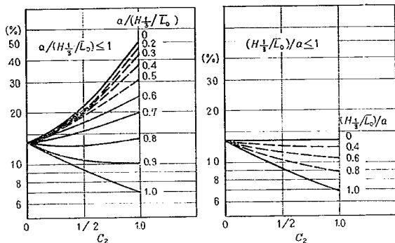
図-8 有義波からきめたうちあげ高をこえる割合
