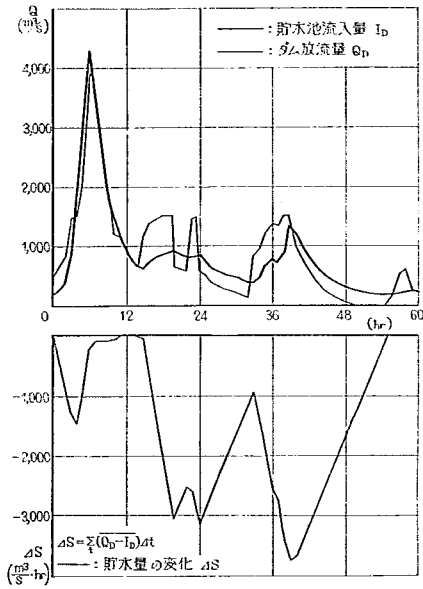
洪水番号 1 風 屋 ( D_2 )
