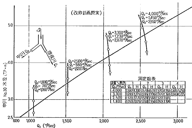
図-33 各流量時の中川No.30水位と分流量 ( Q_2 )
