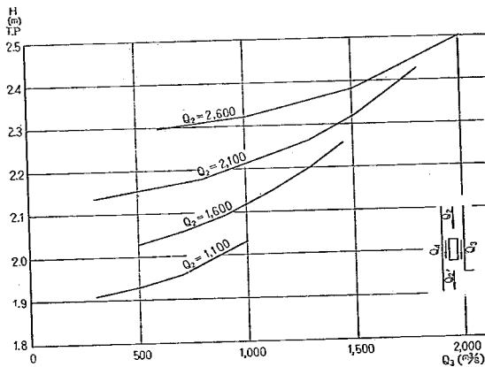
図-10 中川No.13計算水位—流量曲線
