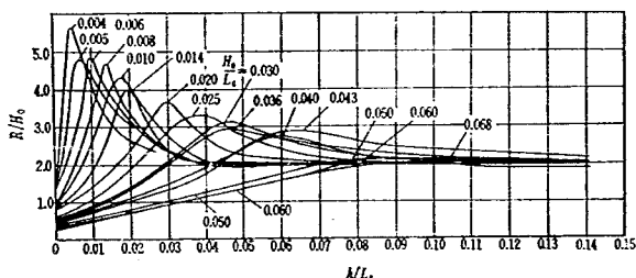
図-4 2割堤防のうちあげ高 (佐藤, 岸)
