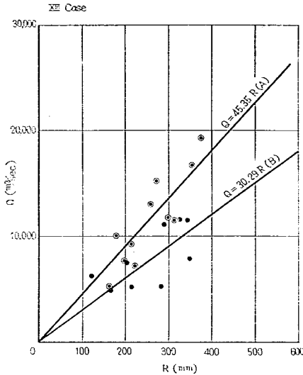
図-13(m) 相賀地点ピーク流量～流域平均2日雨量相関図
