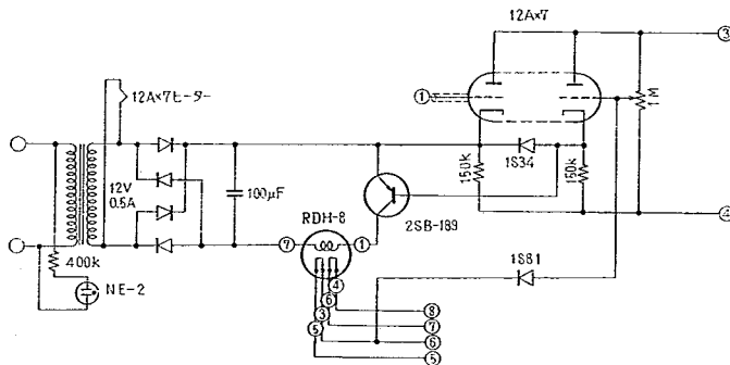
図-21 H.C 部回路図
