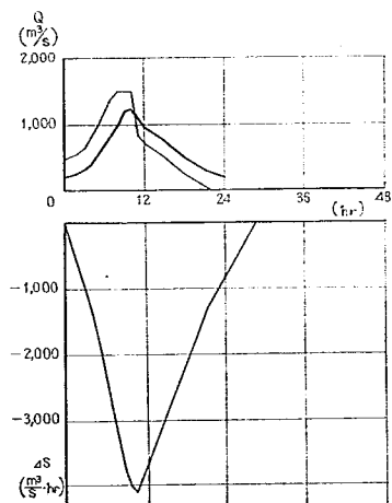
洪水番号 12 池 原 ( D_5 )
