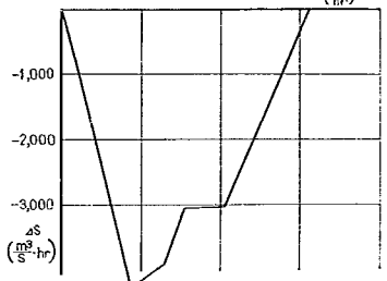
洪水番号 16 風屋 ( D_2 )
