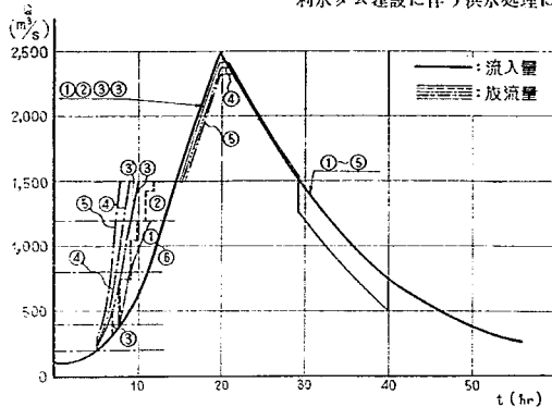
図-11① 池原ダム ( D_5 ) 洪水処理方式 (模式図)
