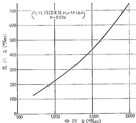
図-18 中川No.21(分流点)分流量曲線
