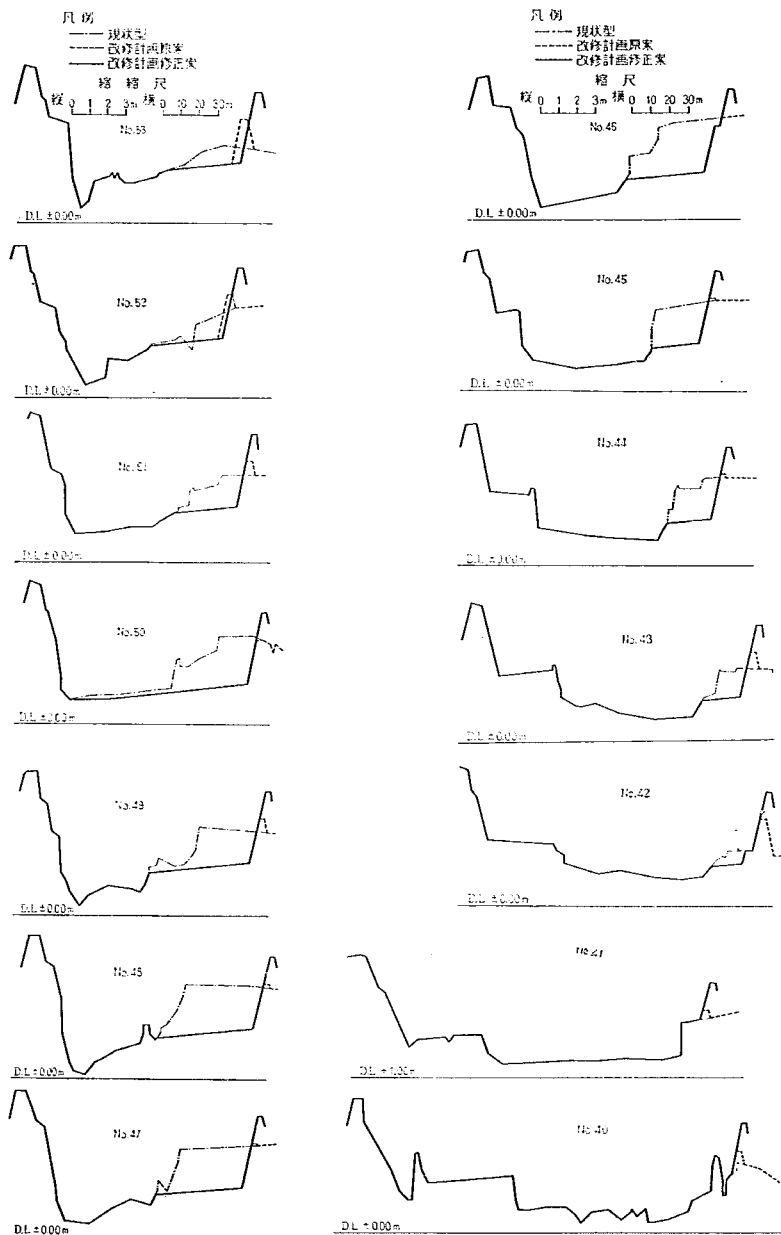
圖-32 改修計画改造横断面圖
