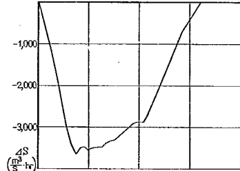
洪水番号 6 池 原 ( D_5 )
