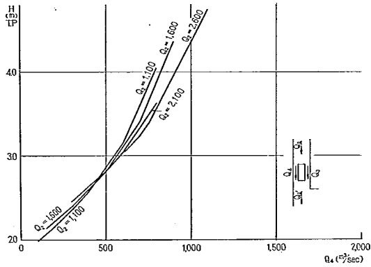
図-15 元川No.6 計算水位—流量曲線
