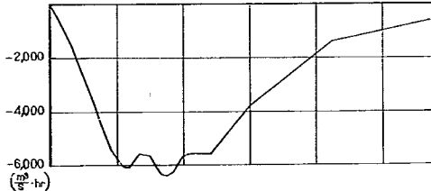
洪水番号 16 池原 ( D_3 )
