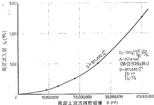
図-6 風屋流域貯留量曲線
