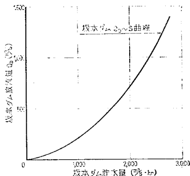
図-10 坂本ダム放流量 Q_D ~ 貯流量曲線
