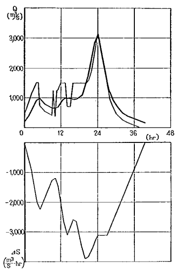
洪水番号 8 風 屋 ( D_2 )
