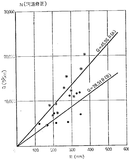
図-13(o) 相賀地点ピーク流量～流域平均2日雨量相関図
