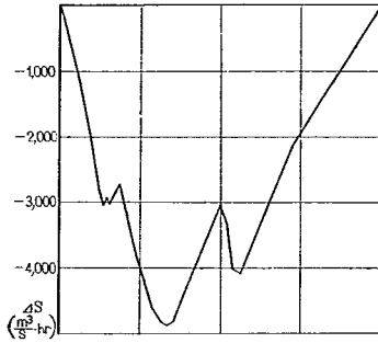
洪水番号 5 風 屋 ( D_2 )
