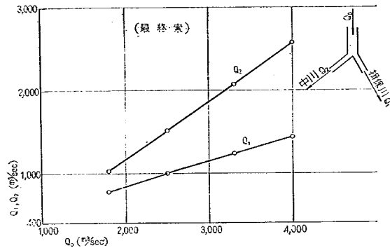
図-36 総流量 ( Q_0 ) と分流量 ( Q_2 ) および残流量 ( Q_1 )
