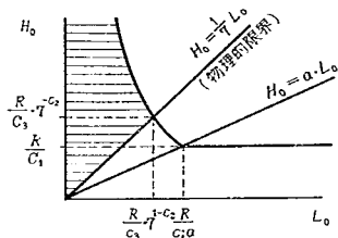
図-7 積分領域の修正量
