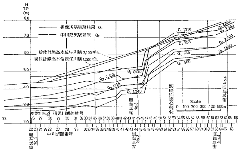
図-27 実験結果水位縦断面図
