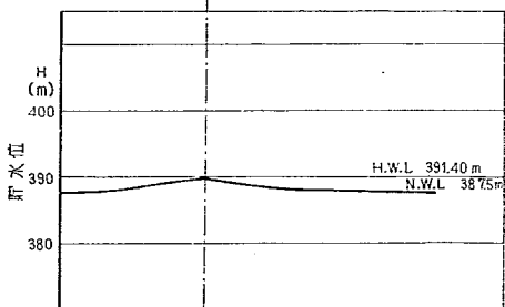
図-9 坂本ダム ( D_i ) 洪水調節図 (模式図)
