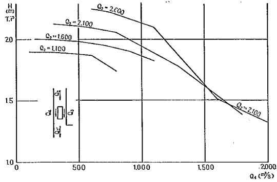
図-14 元川No.1 計算水位—流量曲線
