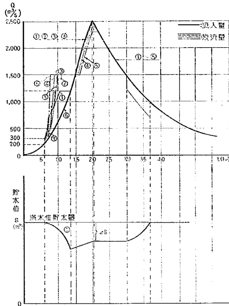
図-5 風屋ダム ( D_2 ) 洪水処理方式 (模式図)
