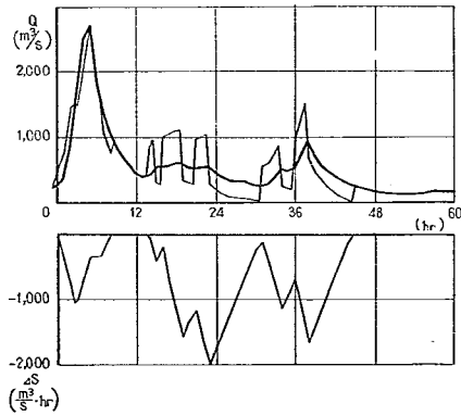
洪水番号 1 池 原 ( D_5 )
