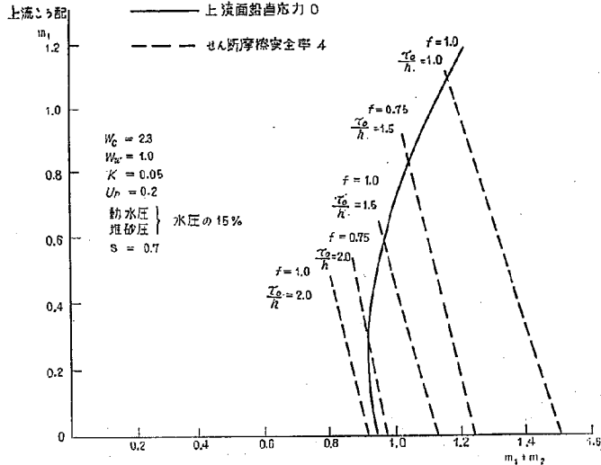
図-5 上流こう配～上下流こう配和(中空重力ダム)
