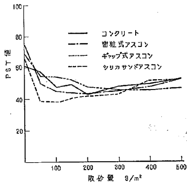
図-5.12 (b) ポータブルテスターによる結果 (湿潤)
