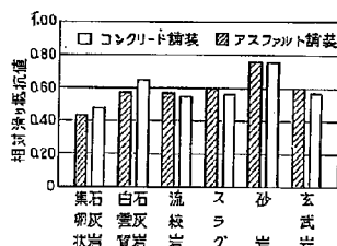
図-5.7 舗装の種類別、岩種別によるすべり抵抗値 (J. W. Shope)
