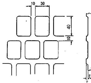
図-5.60 铸鉄覆工板
