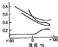
図-2.14 温度と摩擦係数 (King, Tabor)
