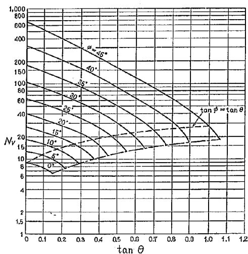
図-8 N_v (q/c=4 \text{ のとき}) を求めるグラフ
