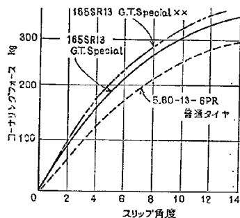
図-5.6 ラジアルタイヤのコーナーリングフォース G. T. Special は横浜ゴムレイヨン90度 カーカスラジアルタイヤ G. T. Special ××は横浜ゴムナイロン 70度カーカスラジアルタイヤ
