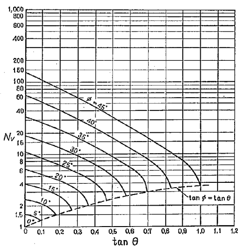
図-9 N_v (=N_{q0}, \text{ただし } c=0 \text{ のとき}) を求めるグラフ
