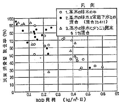
図-5.23 BOD負荷と汚濁負荷除去率との関係
