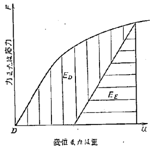
図-4 構造物に入射したエネルギーの逸散と蓄積
