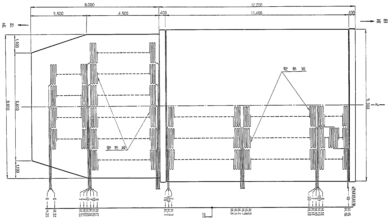
圖-4.6 (a) 電 熱 線 配 置 平 面 圖
