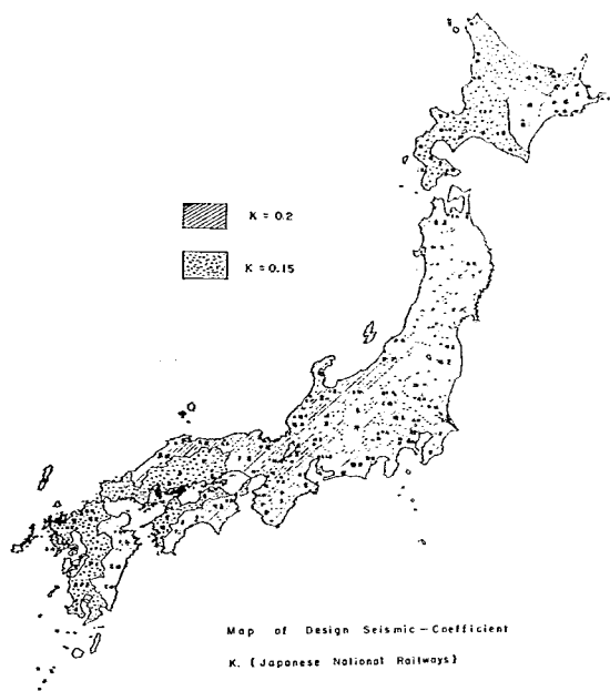
図-10 国鉄で使用されている地域別地震危険度
