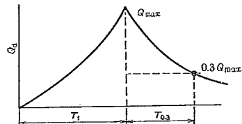
図-3 流量と時間の関係
