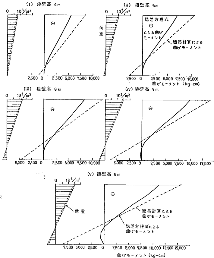
図-3.16 底版の曲げモーメント分布図
