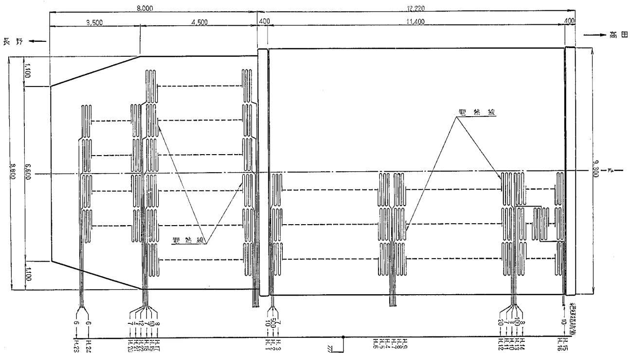
図-4.6 (a) 電線配置平面図
