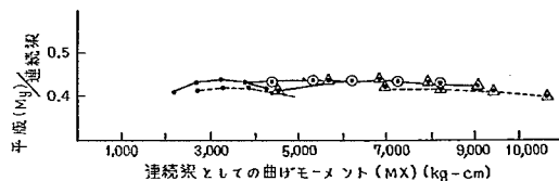
図-3.13 (MY)/(連続梁による曲げモーメント)と連続梁としての曲げモーメント関係図
