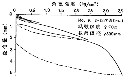
図-3.19 載荷試験における荷重—沈下曲線 (18)
