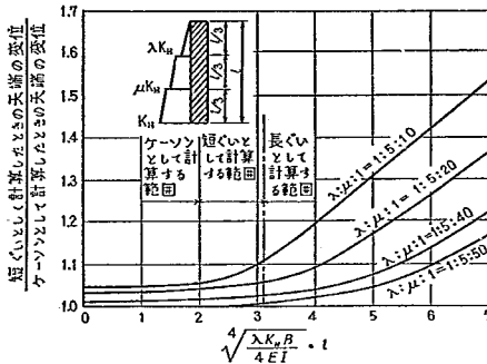
図-5.1 剛体として計算した場合と短くとして計算した場合の変位の比較
