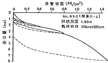
図-3.24 載荷試験における荷重—沈下曲線 (23)
