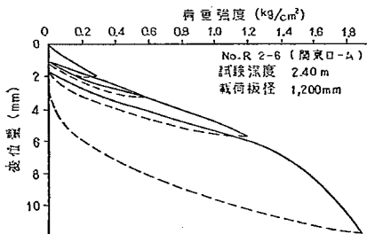
図-3.22 載荷試験における荷重—沈下曲線 (21)
