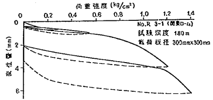
図-3.23 載荷試験における荷重—沈下曲線 (22)
