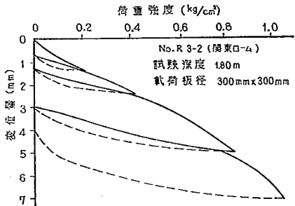
図-3.25 載荷試験による荷重—沈下曲線 (24)
