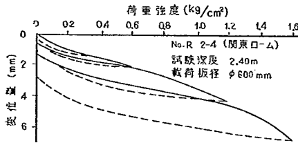
図-3.20 載荷試験における荷重—沈下曲線 (19)
