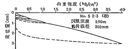
図-3.7 載荷試験における荷重—変位曲線 (6)
