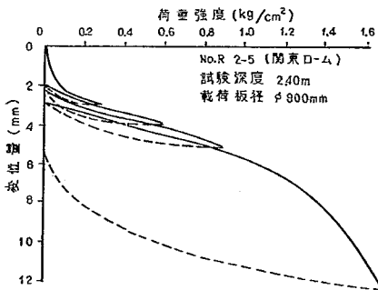
図-3.21 載荷試験における荷重—沈下曲線 (20)
