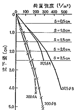
図-4.8 明石層載荷試験の荷重—沈下量曲線
