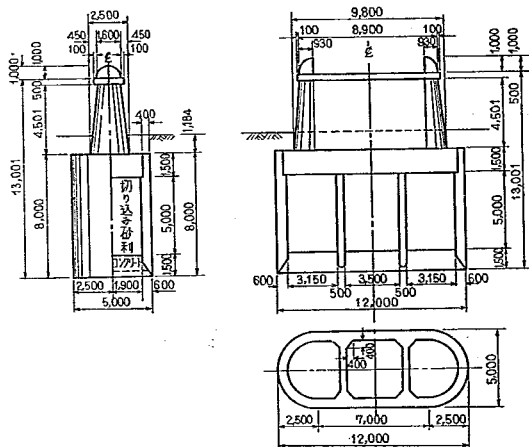
圖-7.3 現橋橋脚一般圖
