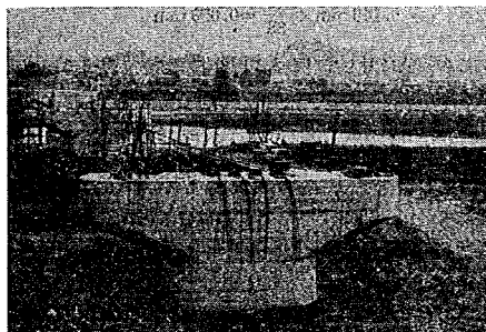
写真-7.1 関戸橋ケーソン載荷試験状況
