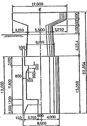
图-7.2 P_3 橋脚一般図
