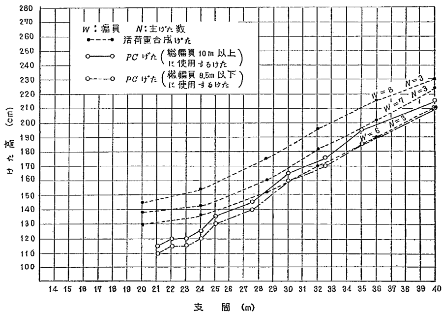
付図-2 活荷重合けたと標準設計における支間とけた高の比較
