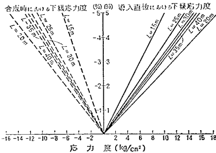
図-18 プレストレスの誤差が導入直後および合成時下縁応力度に及ぼす影響
