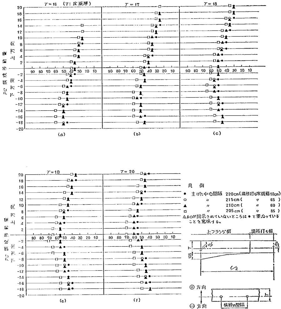
図-22 PC鋼筋の円心移動に対する横筋の間隔
