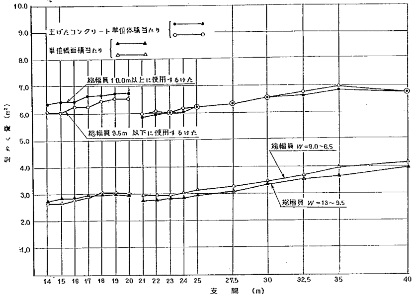
付図-13 主げたコンクリート単位体積当たり・単位橋面積当たり型わく量
