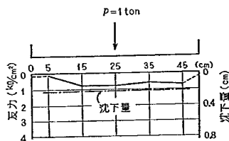
図-4.11 砂地盤上のブロック載荷試験 (底面反力と沈下量の関係)
