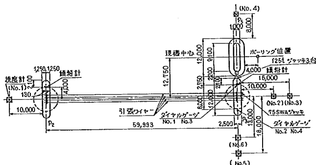
図-7.4 載荷試験方法一般図
