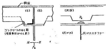
図-5.2 コンクリートのはく離
