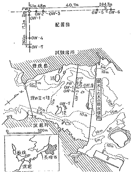
図-5 井戸配置図および試験場所平面図
