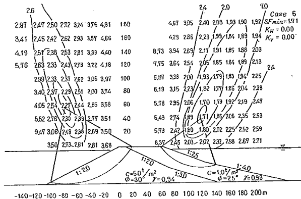
図-5 平時における堤体の安定性
