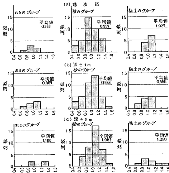
図-13 含水比のばらつき
