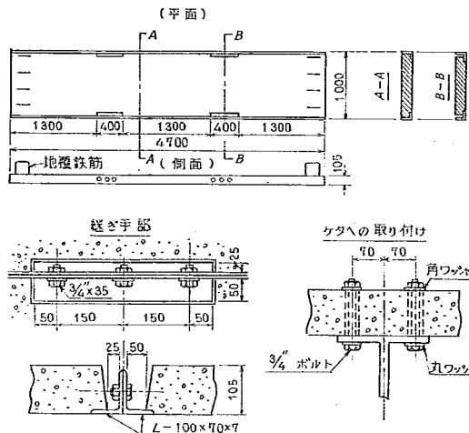
図-1.3 プレストレストコンクリート床版(日本プレストレストコンクリート工業株式会社)
