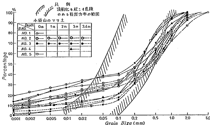
図-14 新潟地方の流動化した砂と小笠山のマサ土の粒度分布
