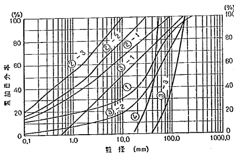
図-1 フィルタイプダム材料の粒度分布
