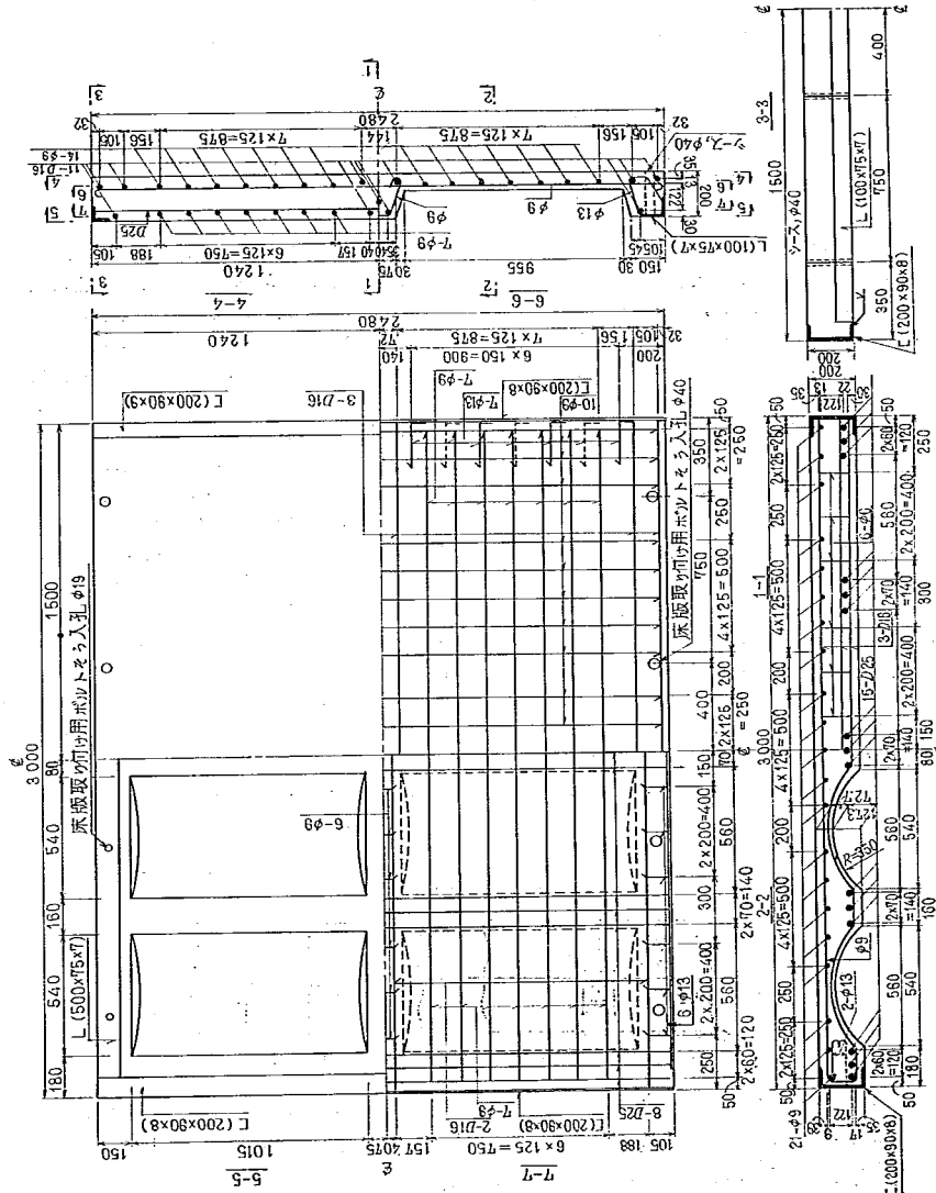
図-3.3 破壊試験供試体
