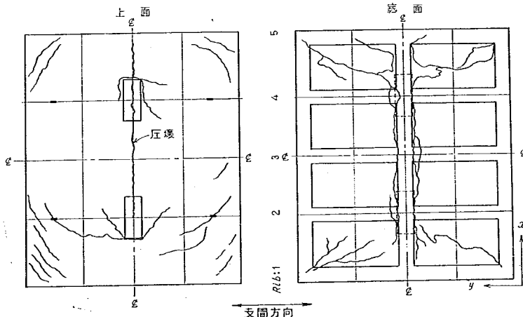
図-3.10 破壊時 ( P=82t ) におけるき裂の状況
