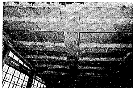
写真-4.8 供 試 体 (底面)
