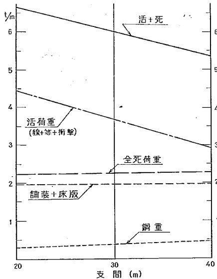
図-1.1 活荷重合成げたにおける荷重強度 (主げた1本当たり) (活荷重合成げた橋標準設計, 昭和38年)
