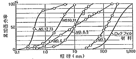
図-2 混合粒径の粒度分布
