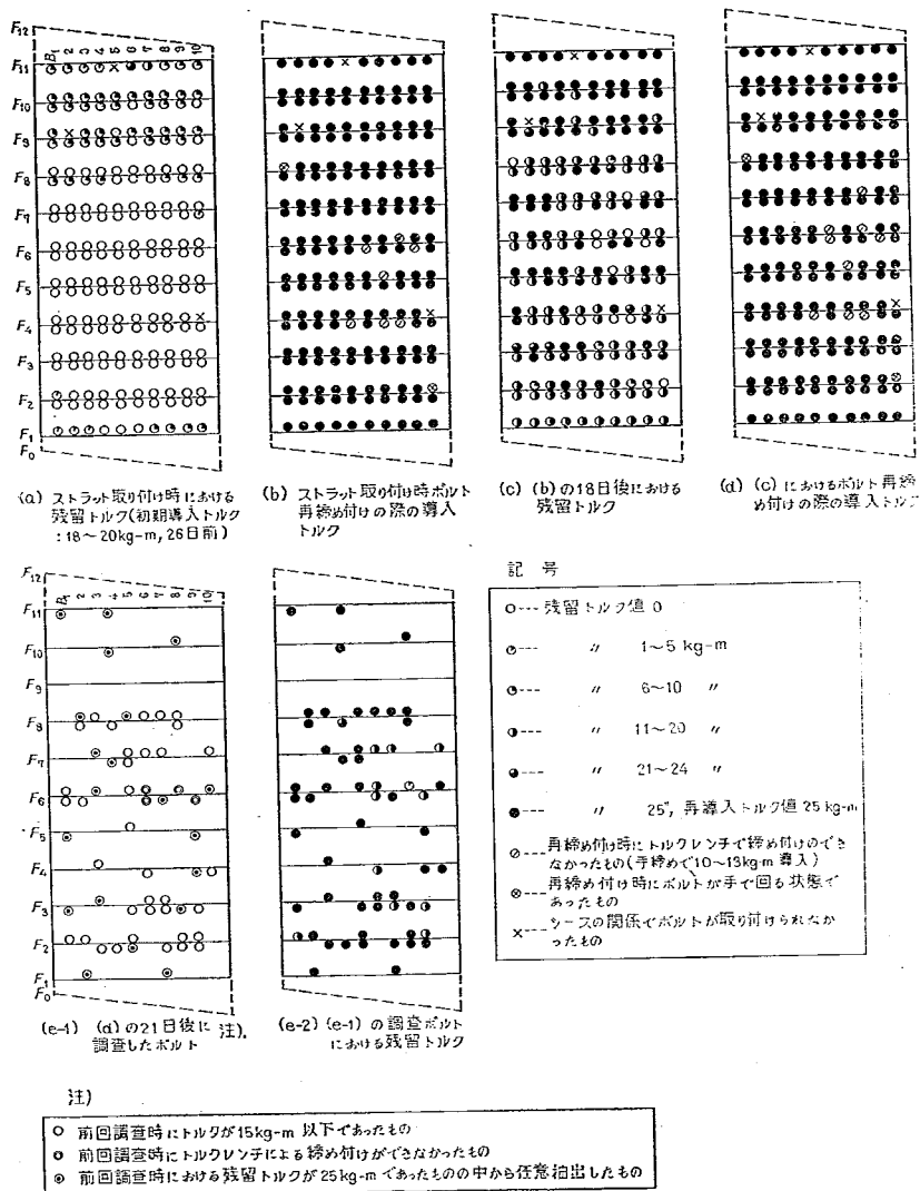
図-5.7 各時点におけるボルトのトルク
