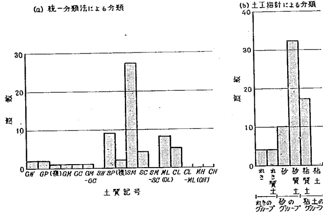
図-2 堤体材料の分類
