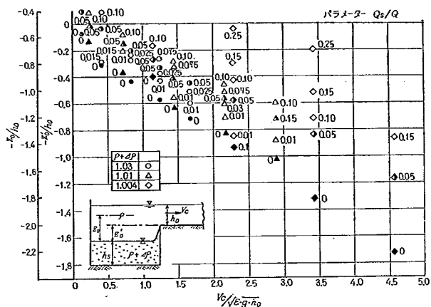
図-5.12 -Z_0/h_0 \sim F_{r,i} 関係図
