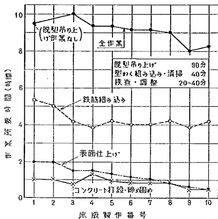
図-4.4 作業所要時間
