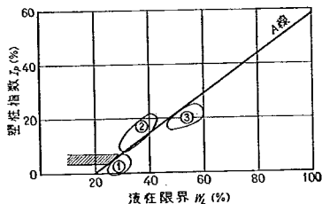
図-4 塑性図による土質分類
