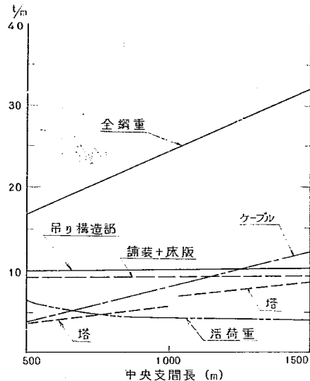
図-1.2 本州四国連絡橋 (吊り橋) 鋼重 (土木学会報告書より)
