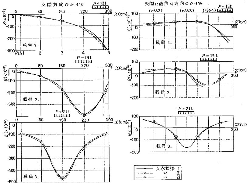
図-3.5 コンクリート圧縮縁のひずみ (支間中央断面)
