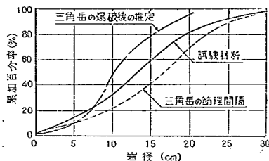
図-3 試験材料の粒度分布
