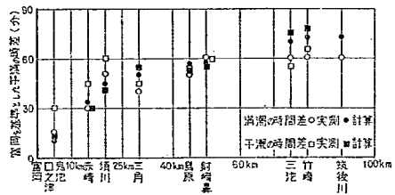
図-6 時差の実測値と計算値の比較
