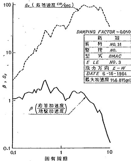
図-12 新潟地震スペクトル曲線(h=0.05)
