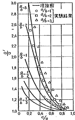
図-18 ポテンシャル理論による理論解と電気模型による実験結果の比較
