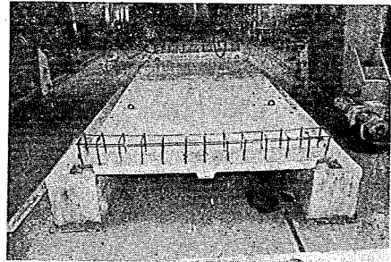
写真-4.7 供 試 体 外 観
