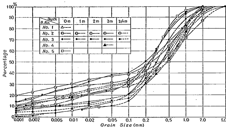
図-11 小袋山のマサ土粒度分布
