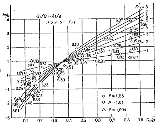
図-3.5 Q_i/Q \sim h_i/a パラメーター F_{ri}
