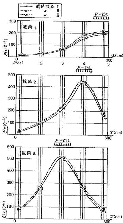
図-3.4 主鉄筋のひずみ(支間中央断面)
