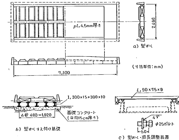
図-4.2 型わく
