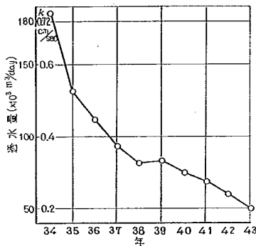
図-14 錦海湾締切堤防の透水係数の経年変化
