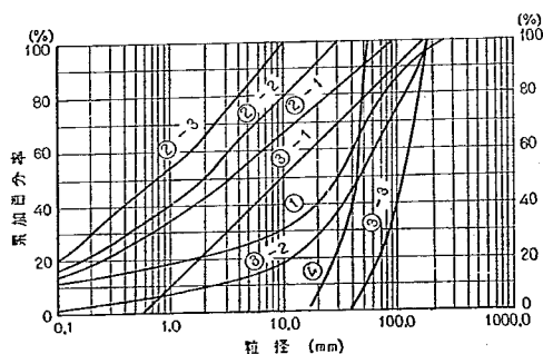
図-1 フィルタイプダム材料の粒度分布
