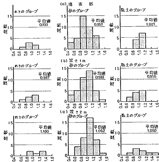
図-13 含水比のばらつき
