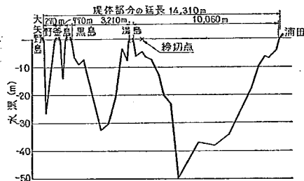
図-3 大矢野線縦断面図
