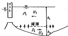
図-2.2 第2次淡水化過程
