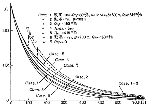
図-4.11 上層密度の時間的変化
