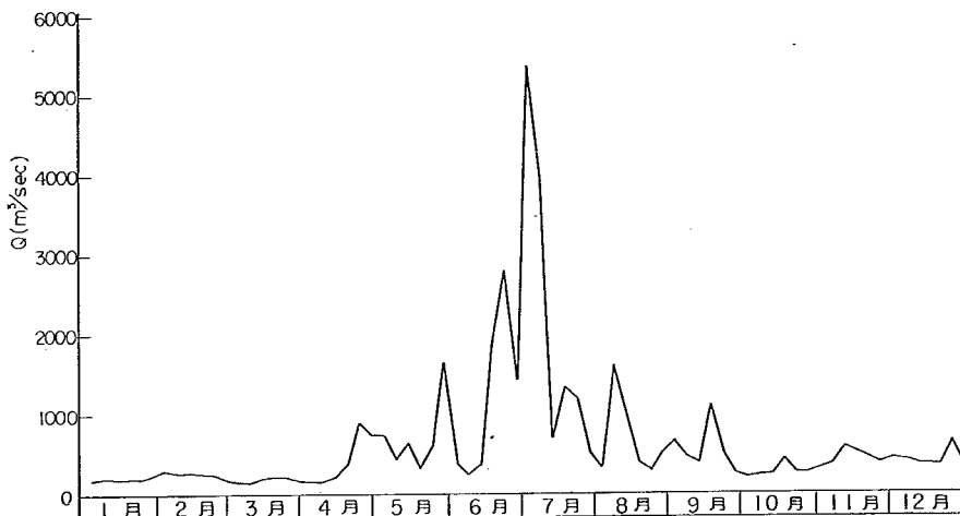
図-10.15 有明海半旬平均合計流入量図 昭和40年
