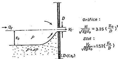
図-5.9 Craya の取水限界に関する実験式
