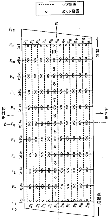
図-5.3 床版, 床げた, ボルトおよび リブの記号, 番号
