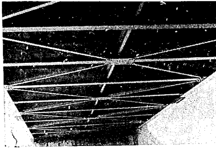
写真-4.11 床組(ストラット取り付け後)
