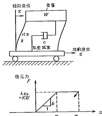
図-8 1自由度モデル
