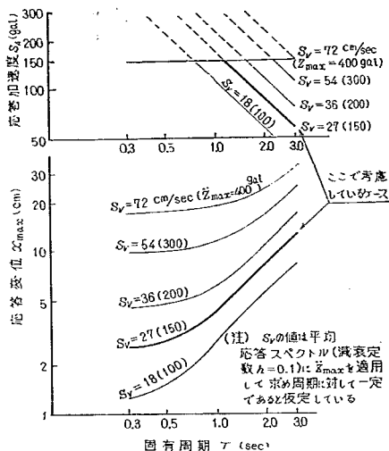
図-11 堤体の固有周期に対する応答位 および応答加速度の関係
