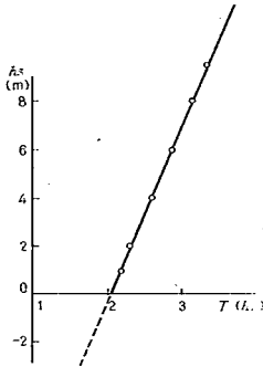
図-4.5 h_s \sim T の関係
