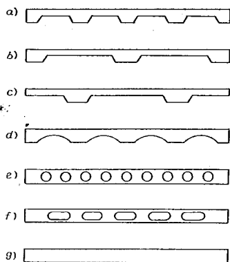
図-2.1 RC (PC) 床版の断面形状
