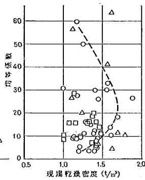
図-6 均等係数と乾燥密度の関係
