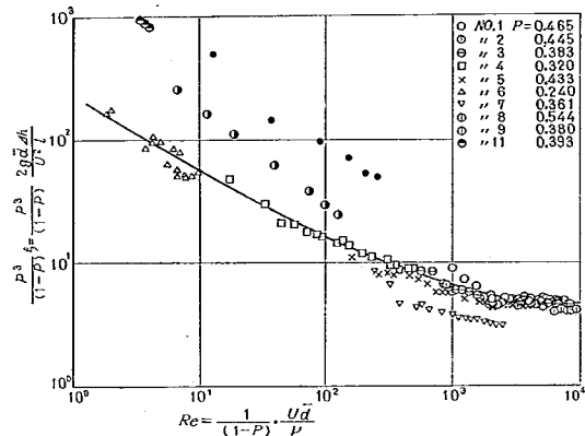
図-4 空けきを考慮した抵抗係数とレイノルズ数の関係
