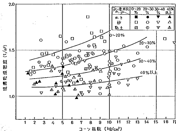
図-11 現場乾燥密度とコーン指数の関係
