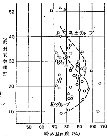
図-9 現場含水比と締め固め度の関係
