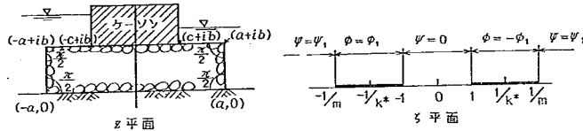
図-16 模型化したケーソン堤断面とその写像
