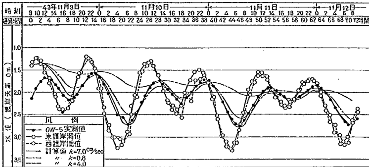
図-7 潮汐による地下水位の変動観測および解析結果
