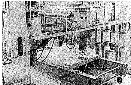
写真-3.1 試験状況
