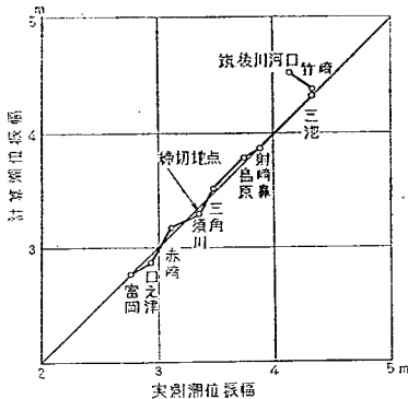
図-5 実測潮位振幅と計算潮位振幅の比較(現状)
