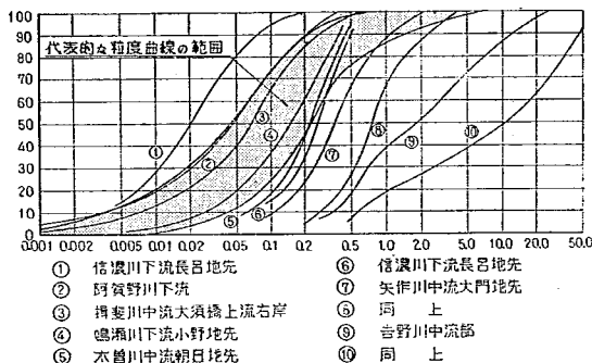
図-3 東北地方の河川堤防材料の代表的な粒度曲線の範囲と各地方の堤防の粒度曲線
