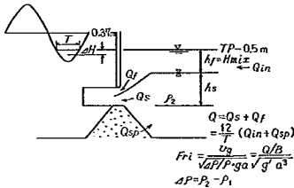
図-2.7 せき付近の模式図
