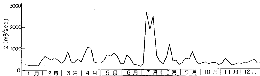
圖-10.9 有明海半旬平均合計流入量圖 昭和34年
