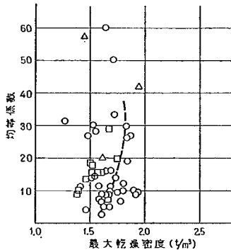
図-7 均等係数と最大乾燥密度
