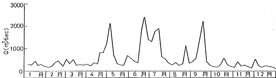
図-10.2 有明海半旬平均合計流入量図 昭和27年
