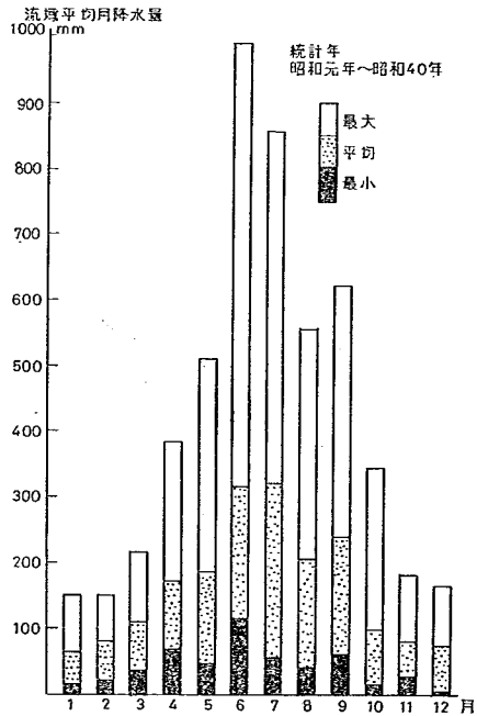
図-6 熊本、佐賀の月雨量図
