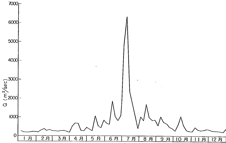
図-10.12 有明海半旬平均合計流入量図 昭和37年
