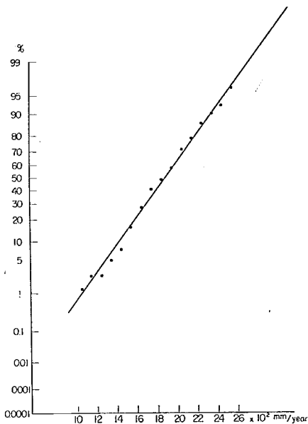
図-16 年降水量度数分布
