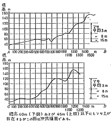
図-3 金山～四反田地区地形断面図およびマサ土平均厚さ(推定)
