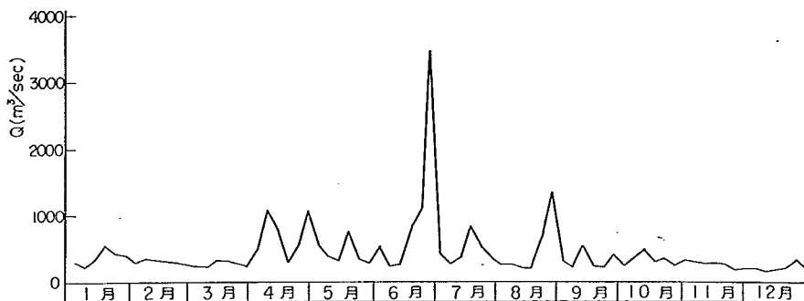
図-10.14 有明海半旬平均合計流入量図 昭和39年
