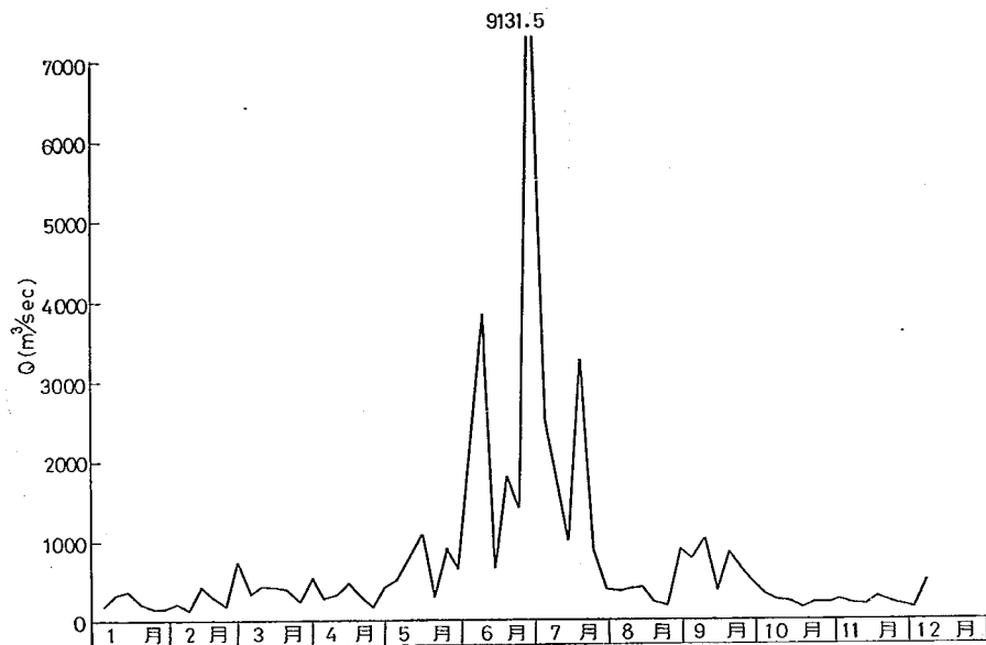
圖-10.3 有明海半旬平均合計流入量圖 昭和28年
