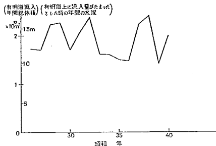
図-12 15年間の有明海流入毎年総量
