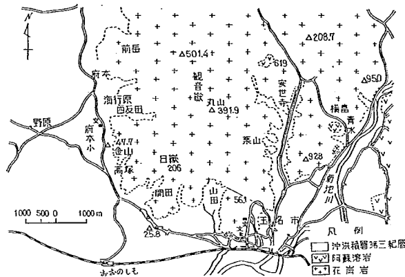
図-2 玉名地区花崗岩分布図
