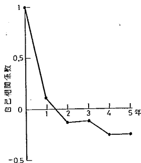
図-14 年降水量コレログラム
