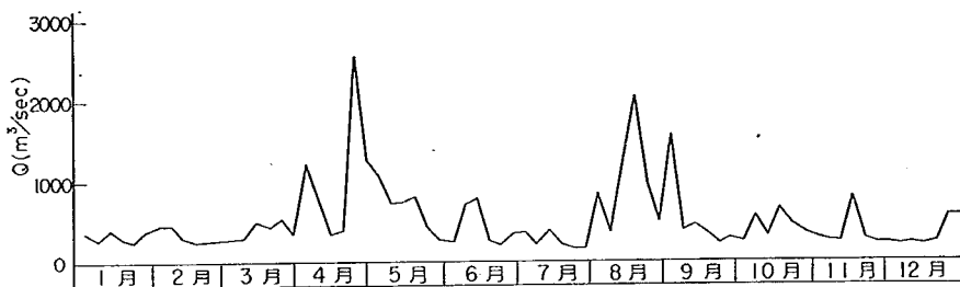
圖-10.8 有明海半旬平均合計流入量圖 昭和33年
