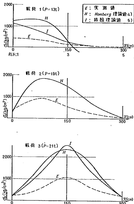
図-3.6 主鉄筋の引張応力度 実測値と理論値との比較一
