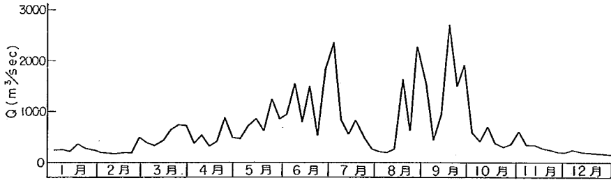
図-10.6 有明海半旬平均合計流入量図 昭和31年
