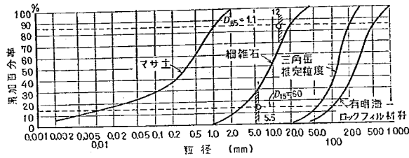
図-1 各材料の粒度分布
