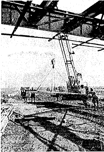
写真-4.6 架 設
