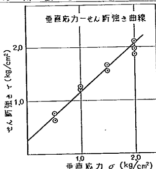
図-4 直接せん断試験結果
