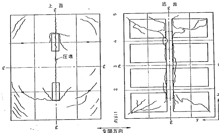
図-3.10 破壊時 ( P=82t ) におけるき裂の状況
