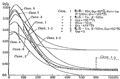
図-4.13 Q_s/Q の時間的変化
