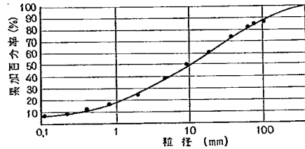
図-6 現場揚水試験地の粒度分布曲線
