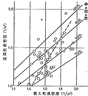
図-8 現場乾燥密度と最大乾燥密度の関係
