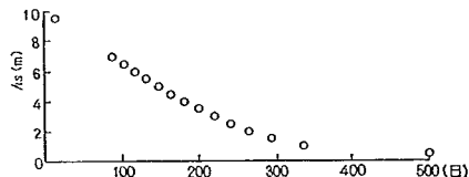
図-4.10 淡水境界面の時間的变化 (Model 1)
