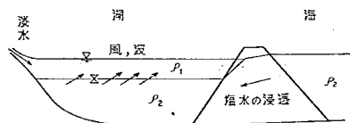
図-2.6 淡水化過程の模式図
