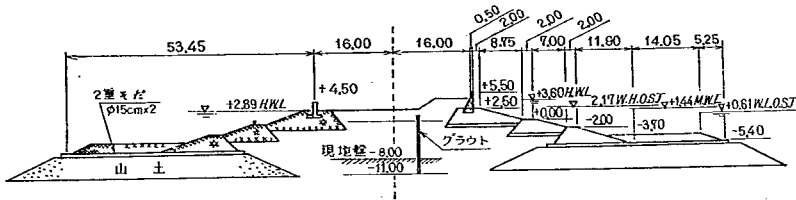
図-15 児島湾締切堤防標準断面図
