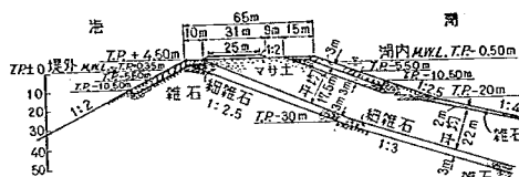
図-1 有明海大崎切堤防標準断面図
