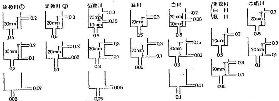
図-8 タンクモデル
