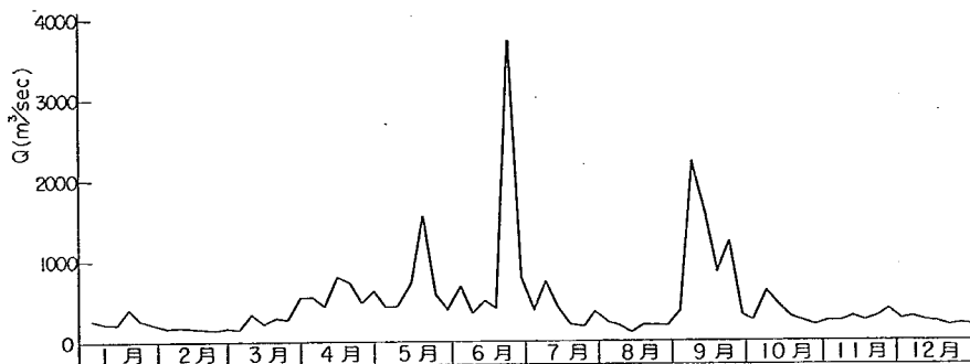
圖-10.10 有明海半旬平均合計流入量圖 昭和35年
