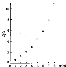
図-4.4 a \sim Cq' \cdot a の関係
