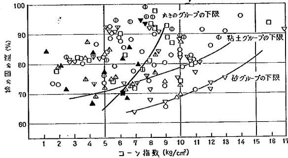
図-12 締め固め度とコーン指数の関係
