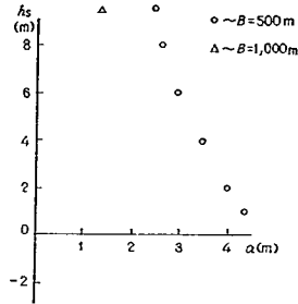
図-4.8 h_s \sim a の関係
