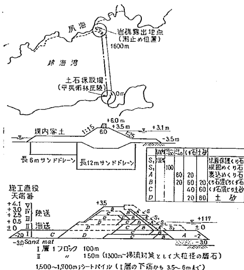
図-13 錦海湾締切堤の概要
