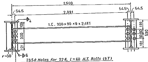
図-5.4 ストラット
