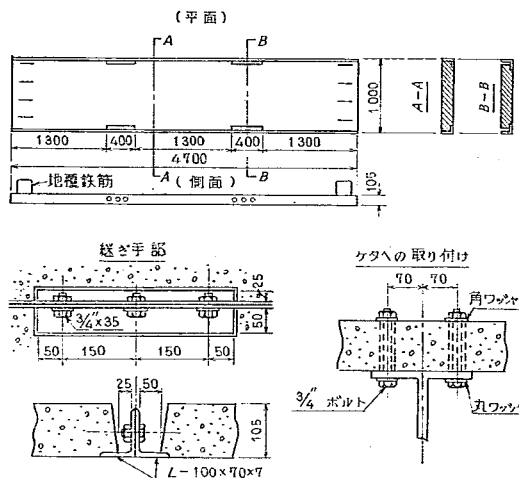
図-1.3 プレキャストコンクリート床版(日本プレストレストコンクリート工業株式会社)
