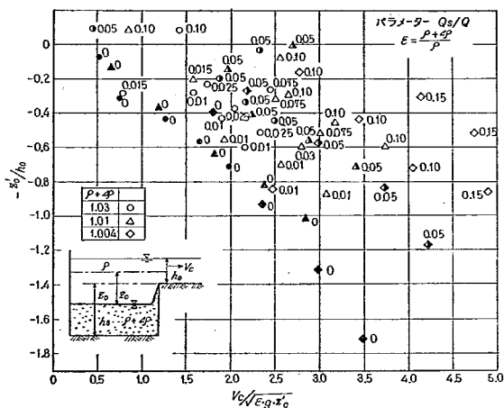
図-5.11 -Z_0/h_0 \sim V_c/\sqrt{\epsilon g s_0} 関係図
