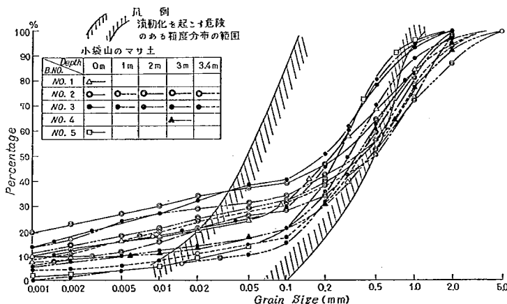
図-14 新潟地方の流動化した砂と小袋山のマサ土の粒度分布
