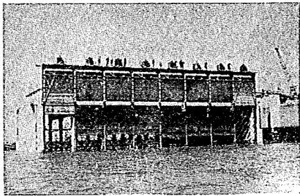
写真-1 オランダのデルタプランの締切に使用されたゲート付きケーソン
