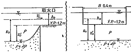
図-5.7 取水口断面図
