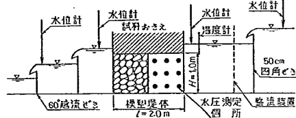
図-1 透水実験装置概要図 (水路幅 B=1.5 m)
