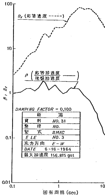
図-13 新潟地震スペクトル曲線 (h=0.1)
