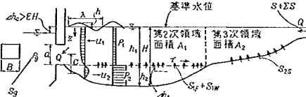
図-2.4 淡水湖の一般モデル
