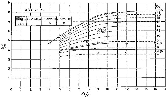
図-5.5 Q_2/Q=0.5 h_1/a \sim H_2/a
