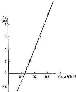
図-4.6 h_s \sim \Delta H の関係
