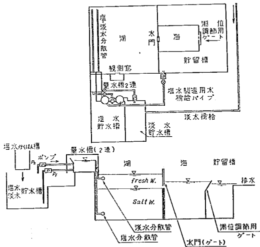
図-3.2 実験施設図
