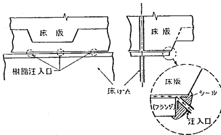
図-5.8 樹脂注入位置
