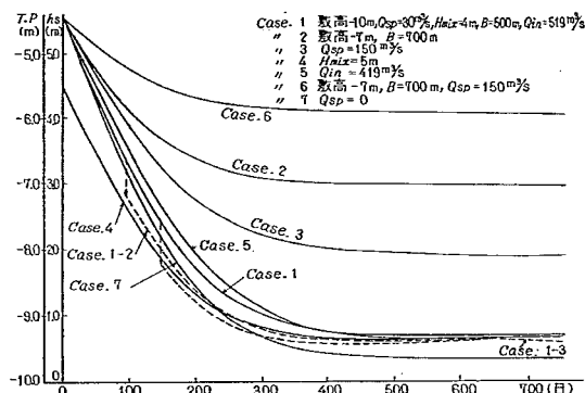
図-4.12 淡水境界面の時間的変化
