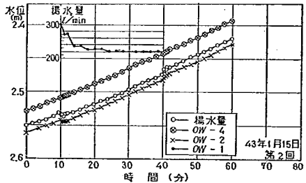
図-9 揚水による地下水位の変動
