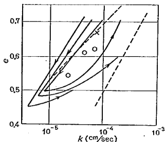
図-12 マサ土の透水係数
