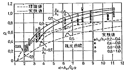
図-4.3 もぐり流出の関係曲線(トッホによる)
