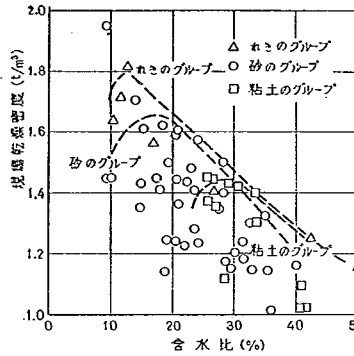
図-5 乾燥密度と含水比の関係
