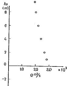
図-4.7 h_s \sim Q の関係
