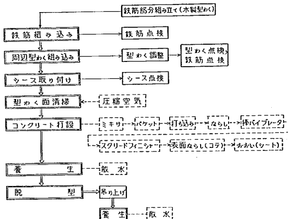
図-4.3 床版製作作業工程
