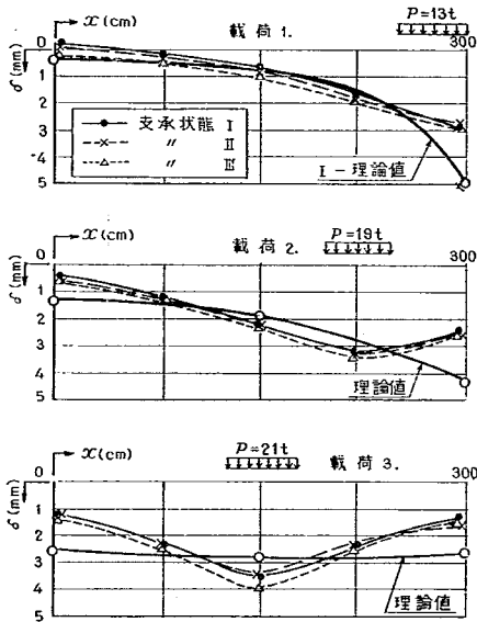
図-3.8 版のたわみ (支間中央断面)
