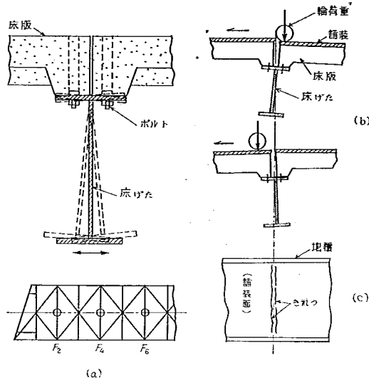
図-5.1 床版と床げたの挙動(ストラット取り付け前)
