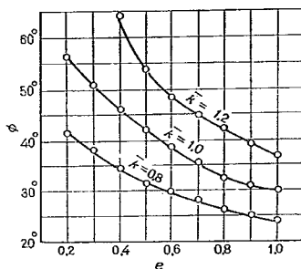
図-2 最上の理論による e と \phi の関係
