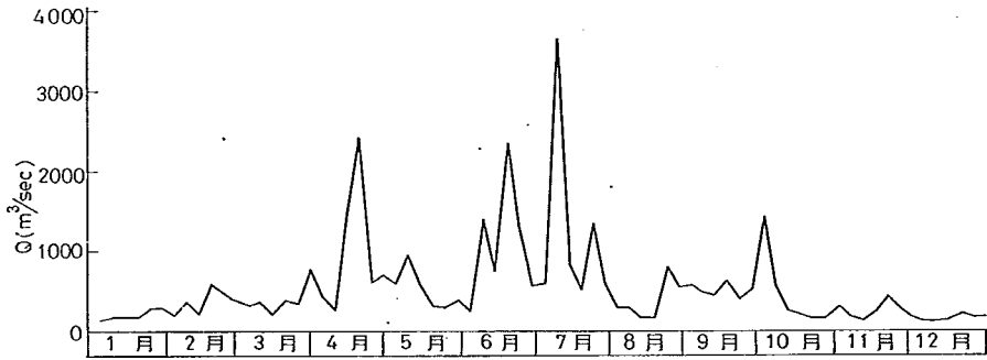
図-10.5 有明海半旬平均合計流入量図 昭和30年
