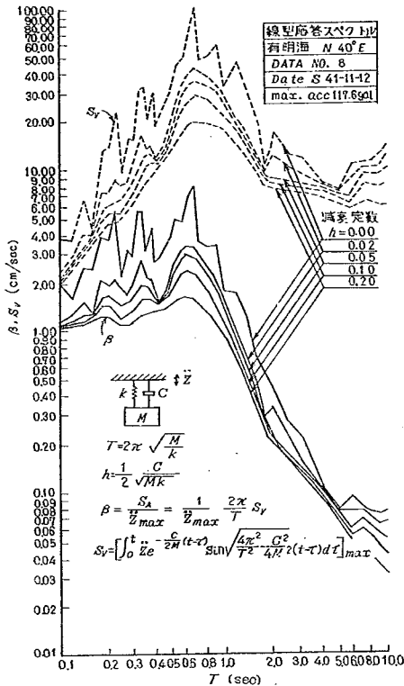
図-3 地震応答スペクトル曲線
