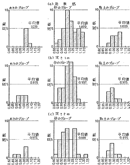
図-14 乾燥密度のばらつき
