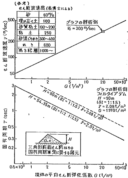
図-10 堤体のせん断弾性係数に対する固有周期およびせん断波速度の関係
