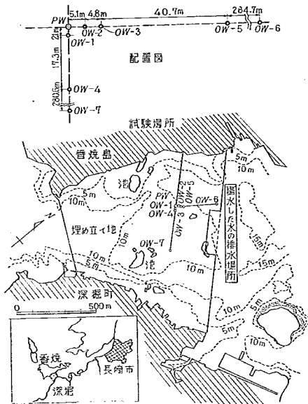
図-5 井戸配置図および試験場所平面図
