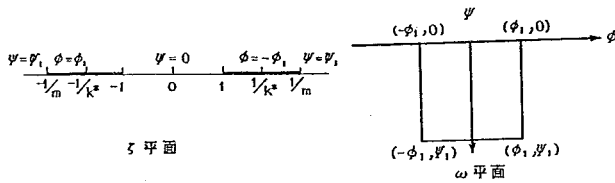
図-17 ξ平面からw平面への写像
