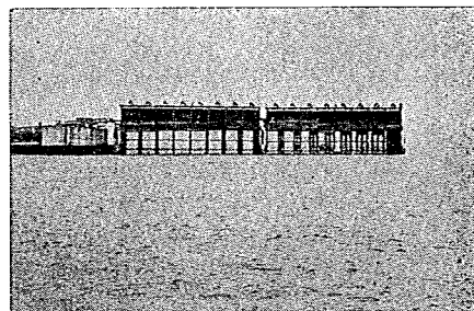
写真-2 オランダのデルタプランの締切に使用されたゲート付きケーソン
