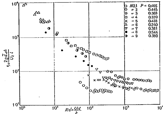
図-3 抵抗係数とレイノルズ数の関係
