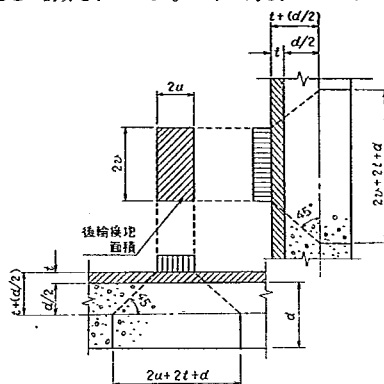
図-3.1 輪荷重分布の仮定
