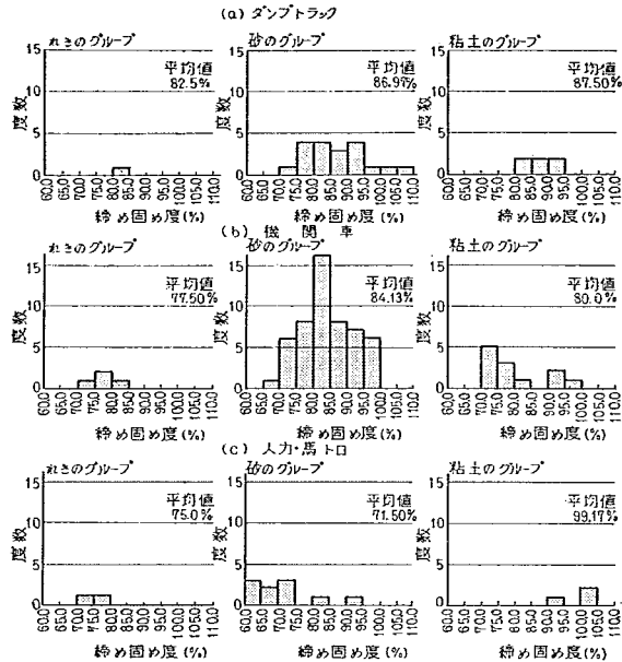
図-15 施工法による締め固め度のばらつき
