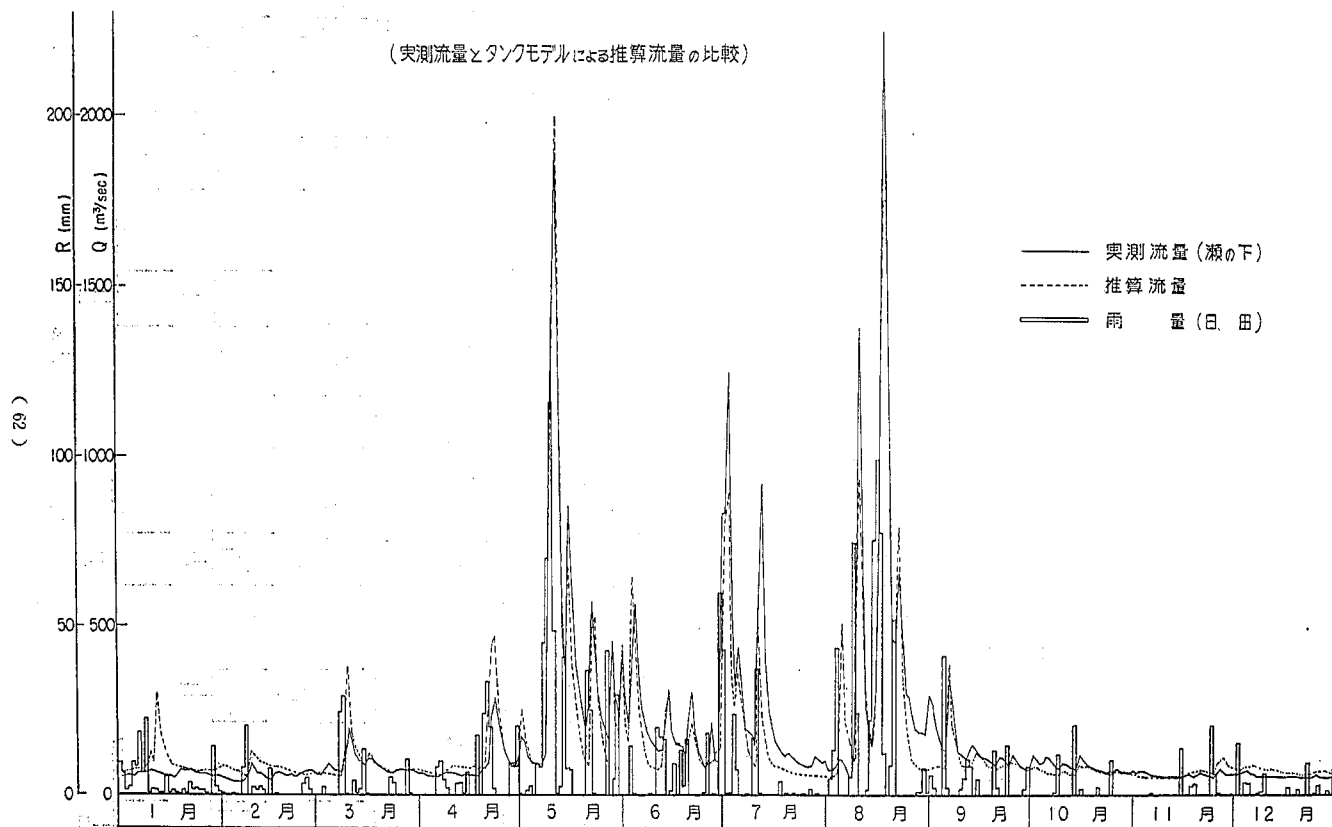
図-9.1 筑後川 日流量, 日雨量図 昭和38年
