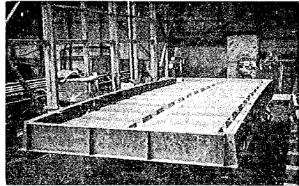
写真-4.2 型わく
