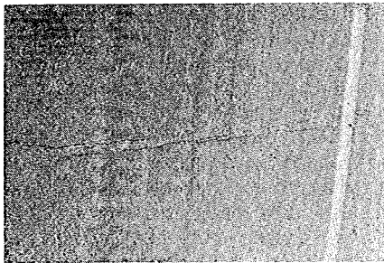
写真-4.10 舗装面のひびわれ
