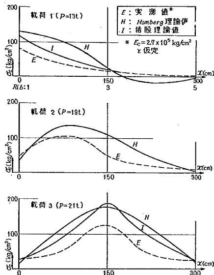
図-3.7 コンクリートの圧縮応力度 一実測値と理論値との比較一
