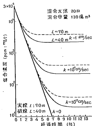
図-2.5 締切に伴う塩分濃度変化曲線
