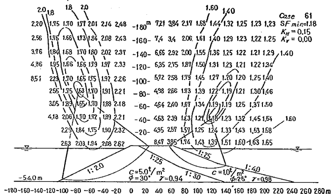
図-6 地震時における堤体の安定性
