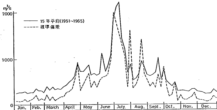
図-11 有明海流入半月流量 (15年平均と標準偏差)
