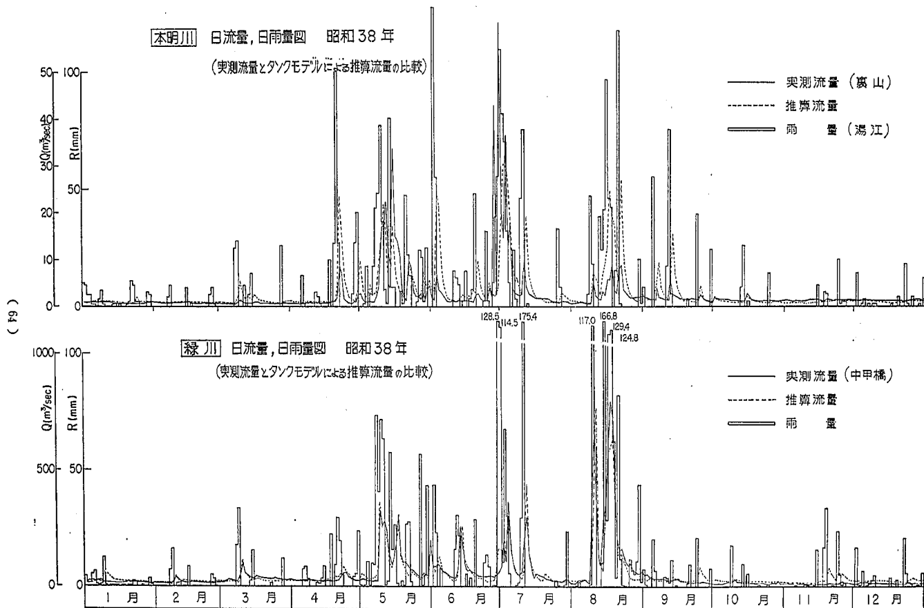
図-9.3 本明川、緑川 日流量、日雨量図 昭和38年
