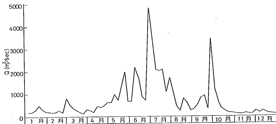
圖-10.4 有明海半旬平均合計流入量圖 昭和29年
