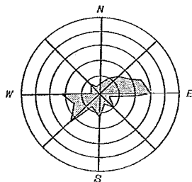
図-9 湯島の風配図
