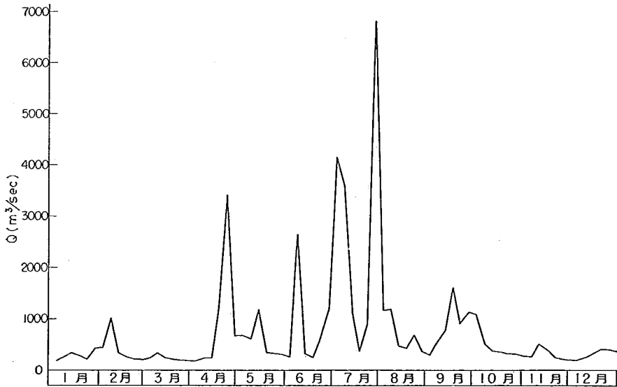
図-10.7 有明海半旬平均合計流入量図 昭和32年
