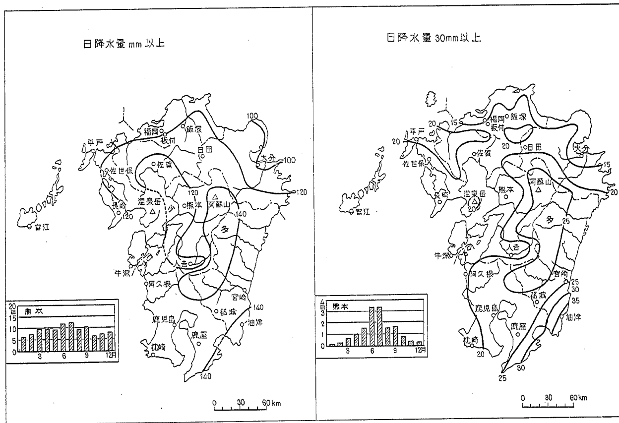
図-5 年間降水日数分布図と熊本の月間降水日数の年変化図（日本の気候 和達清夫より）
