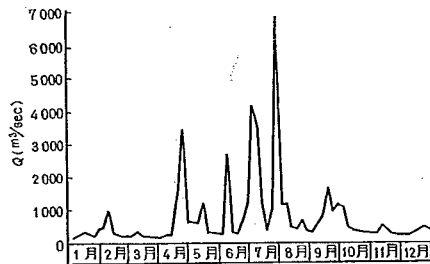
図-2.9 有明海半旬平均合計流入量図
