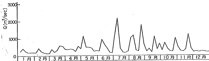
圖-10.11 有明海半旬平均合計流入量圖 昭和36年
