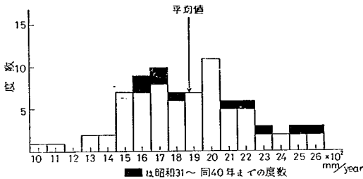
図-15 年降水量度数分布
