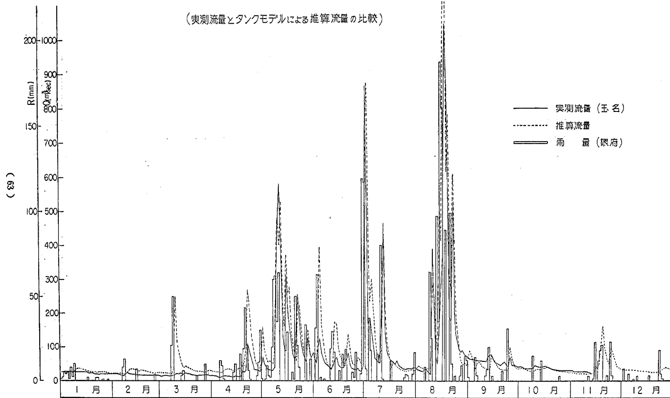
図-9.2 菊池川 日流量, 日雨量図 昭和38年
