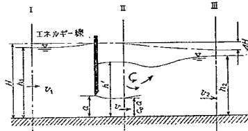
水門からのもぐり流出
