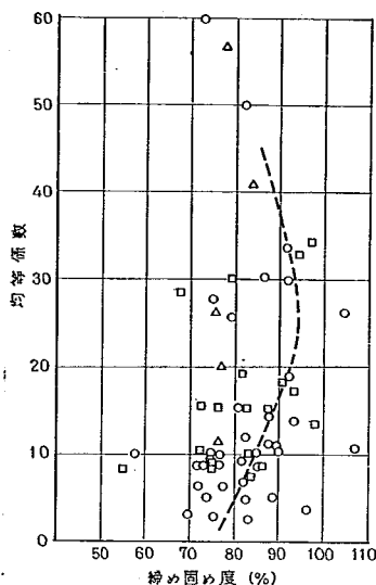
図-10 均等係数と締め固め度の関係
