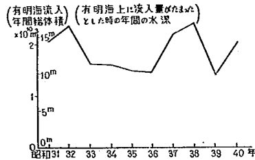
図-2.8 10年間の有明海流入量年間総量
