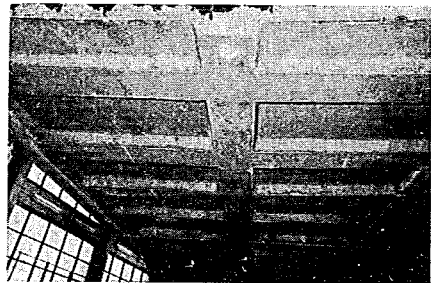
写真-4.8 供 試 体 (底面)
