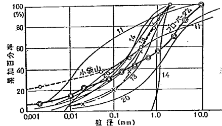
図-10 マサ土の粒度分布
