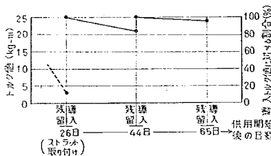
図-5.5 ボルト全体としてのトルク減少度
