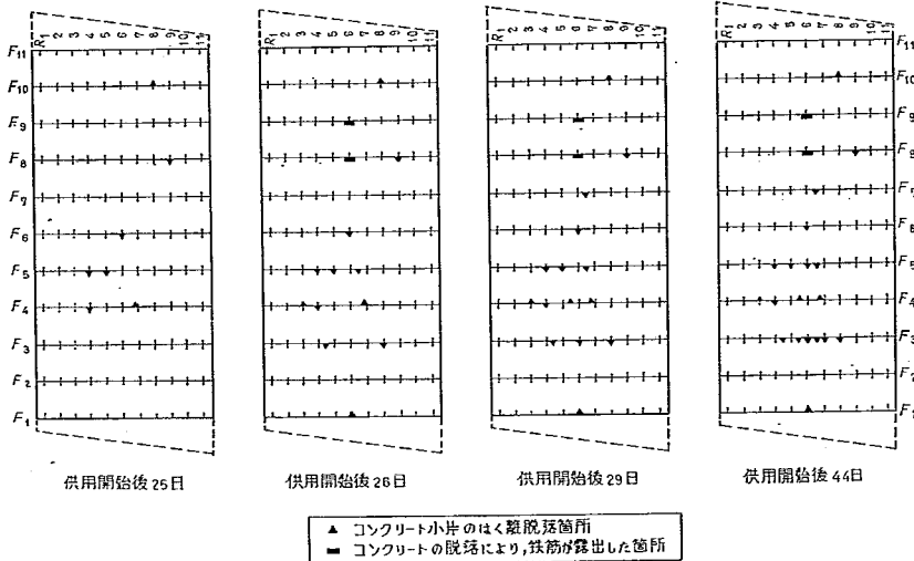
図-5.6 床版コンクリートの破損箇所
