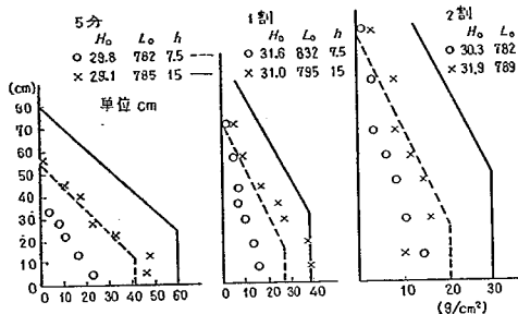
図-34 傾斜堤における砕波圧分布の実験値と計算値との比較
