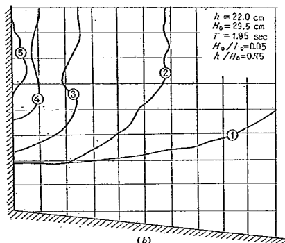
図-15 砕波衝撃圧発生時の波の衝突状況
