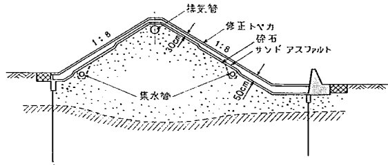
図-5 越流堤の構造
