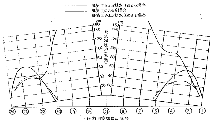
図-20 空気抜きおよび排水工の効果の比較
