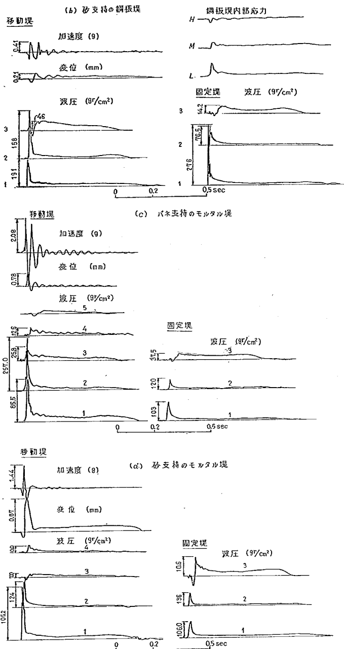
図-21 (b), (c), (d), 堤防に作用する波圧, および変位, 加速度, 応力の時間変化 (24)
