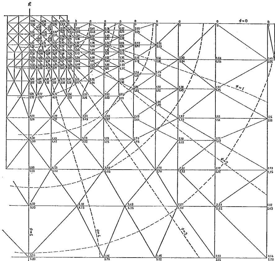
図-5 理論値と計算値との比較
