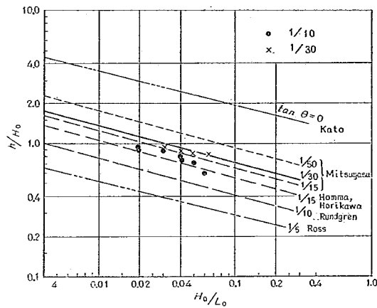
図-14 最大衝撃圧が発生する設置水深
