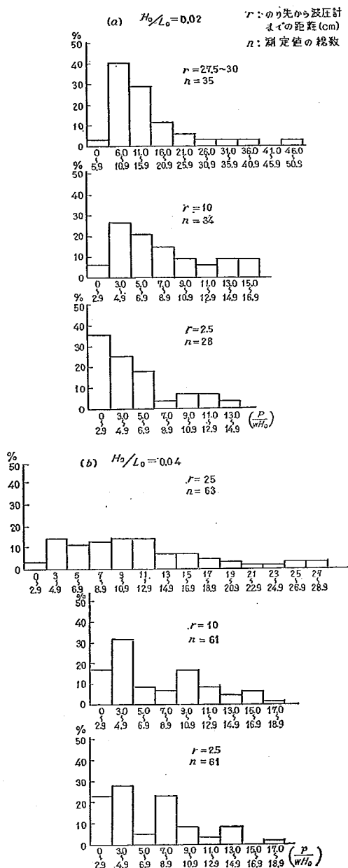
図-18 最大衝撃圧のひん度分布
