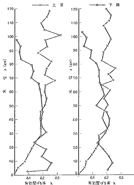
図-9 有効間引き率の測定結果
