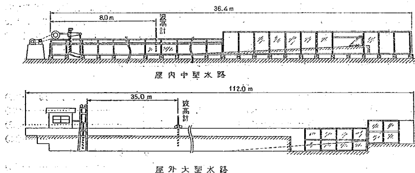
図-1 造波水路
