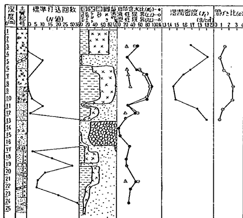
図-3 渡良瀬越流堤築造地点の代表的ボーリング調査結果
