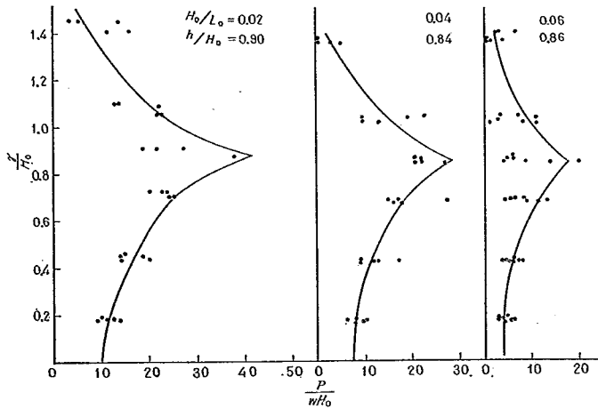
図-17 碎波衝撃圧の鉛直分布
