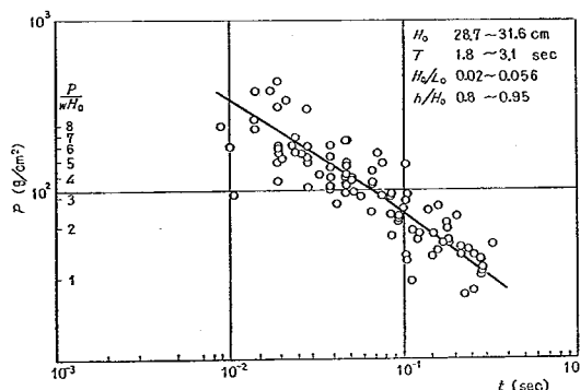
図-43 波圧強度と作用時間 (5 分堤)
