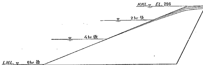
図-10 k=1 \times 10^{-2} cm/sec の場合の浸潤面
