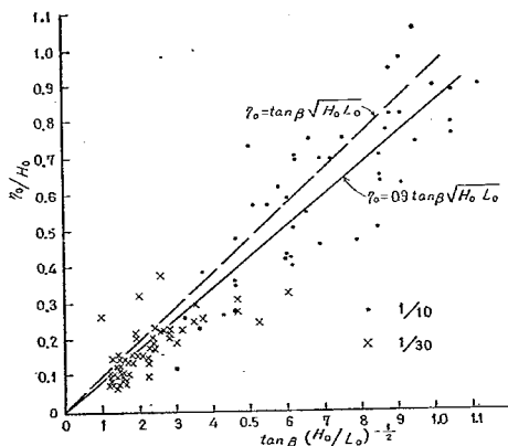
図-26 汀線における波頂高と波形こう配および海底こう配との関係
