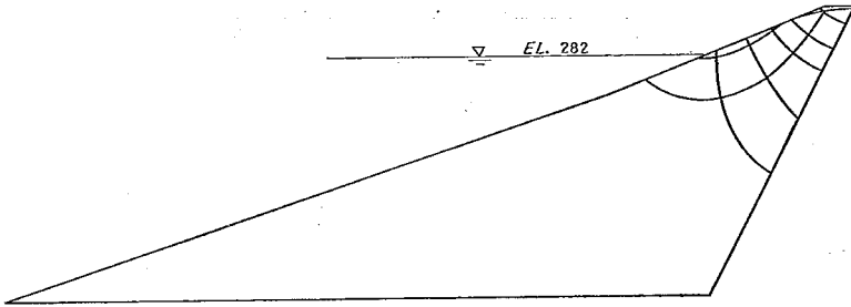
(b) k=10^{-2} cm/sec, 4時間 経過後
