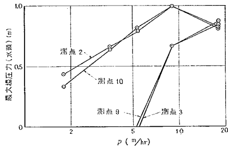
図-15 P と最大揚圧力の関係
