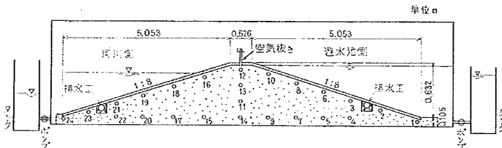
図-12 砂模型実験装置（単位m）
