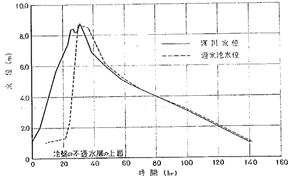
図-10 計画洪水の水位曲線
