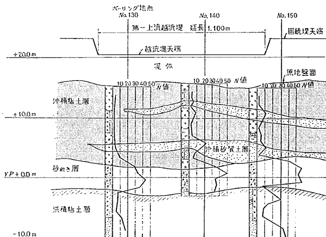
図-2 越流堤築造箇所の地層断面
