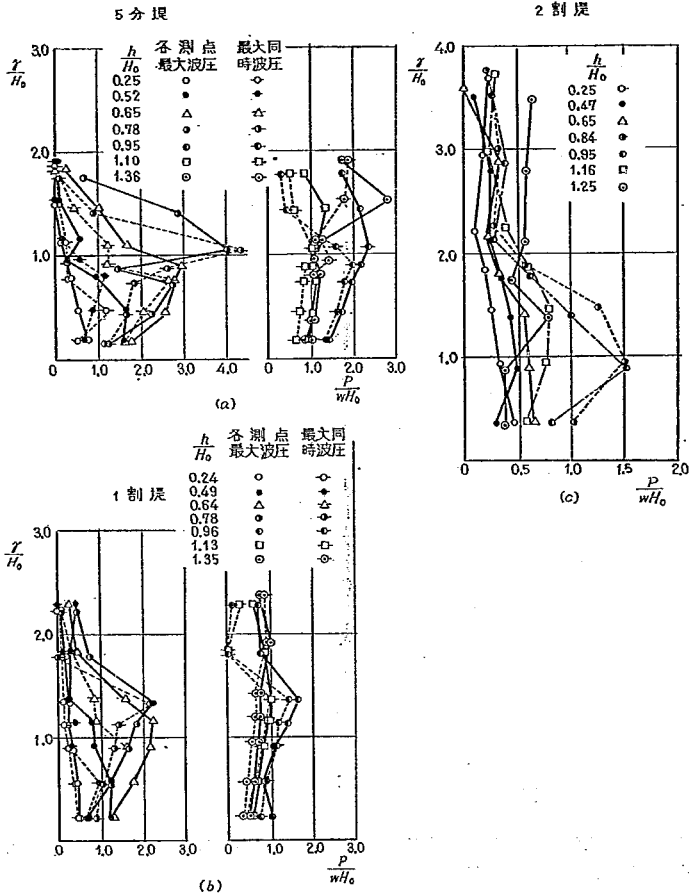
図-10 傾斜堤の波圧分布 (波形こう配0.04)
