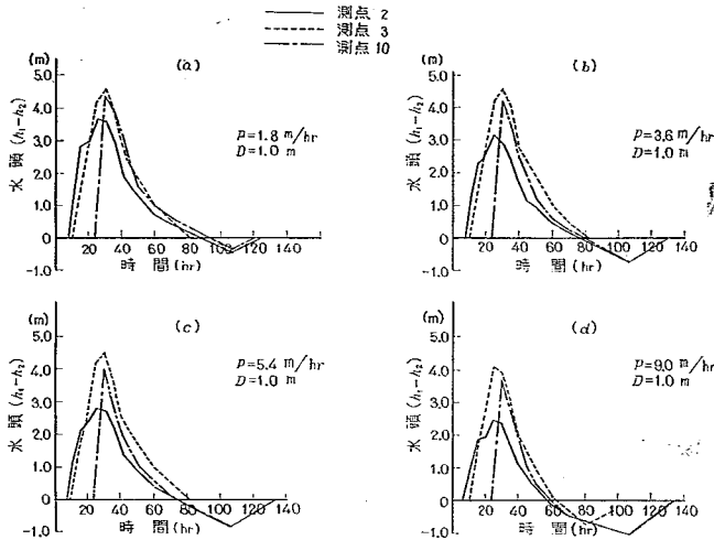
図-14 フェイシングに作用する水頭
