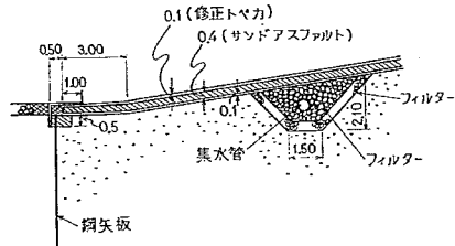
図-22 のり尻の排水施設の構造
