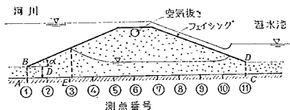
図-7 越流堤体内への浸透状態
