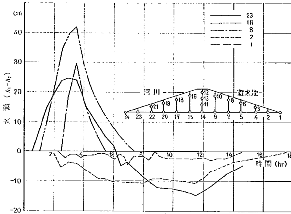
図-17 フェイシングに作用する水頭 (砂模型の実験結果の1例)
