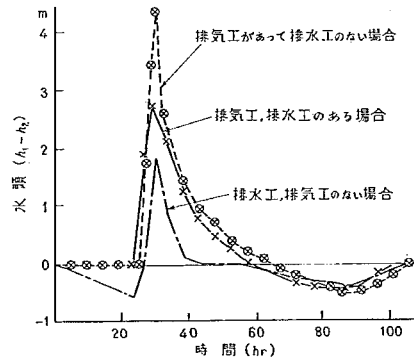
図-19 のり尻付近のフェイシングに作用する水頭
