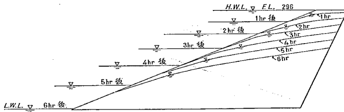
図-9 k=1 \times 10^{-1} cm/sec の場合の浸潤面
