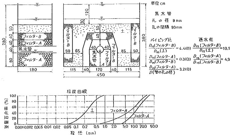
図-24 集水管の実験
