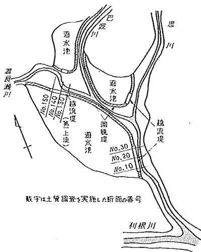
図-1 渡良瀬川越流堤築造箇所平面図
