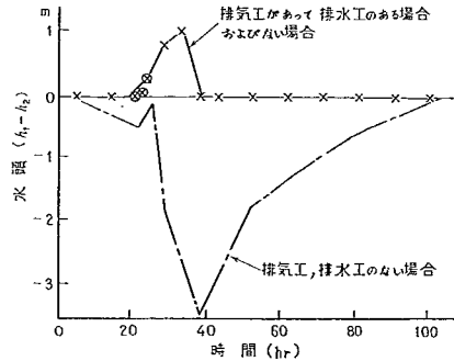
図-18 天端のフェイシングに作用する水頭
