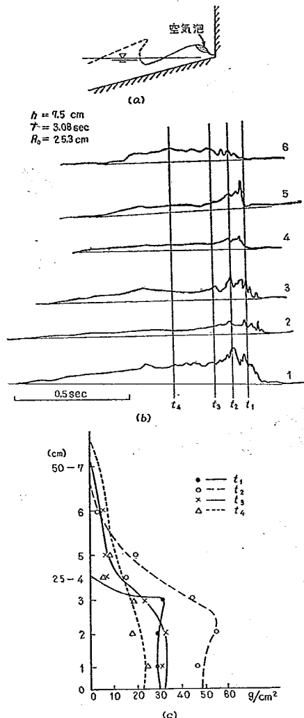
図-4 砕波圧領域における波の衝突状況と波圧の時間変化
