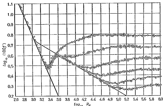
図-1 Nikuradse の実験
