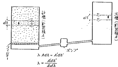
図-8 有効間げき率の測定装置の原理
