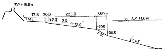
図-35 浦原海岸の海底こう配および堤断面
