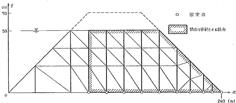
図-6 アースダム の定常浸透流計算例 (均質材料の堤体の要素分割)
