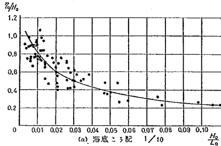
(a) 海底こう配 1/10
