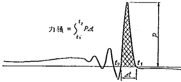
図-19 力積の計算説明
