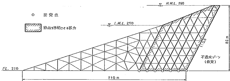
図-8 非定常浸透流計算例 (喜撰山ロックフィルダム堤体の要素分割)
