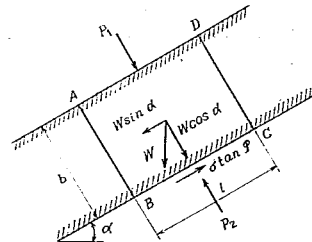
図-6 フェイシングの微小部分のつり合い
