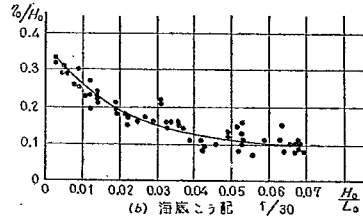
図-24 汀線における波頂高
