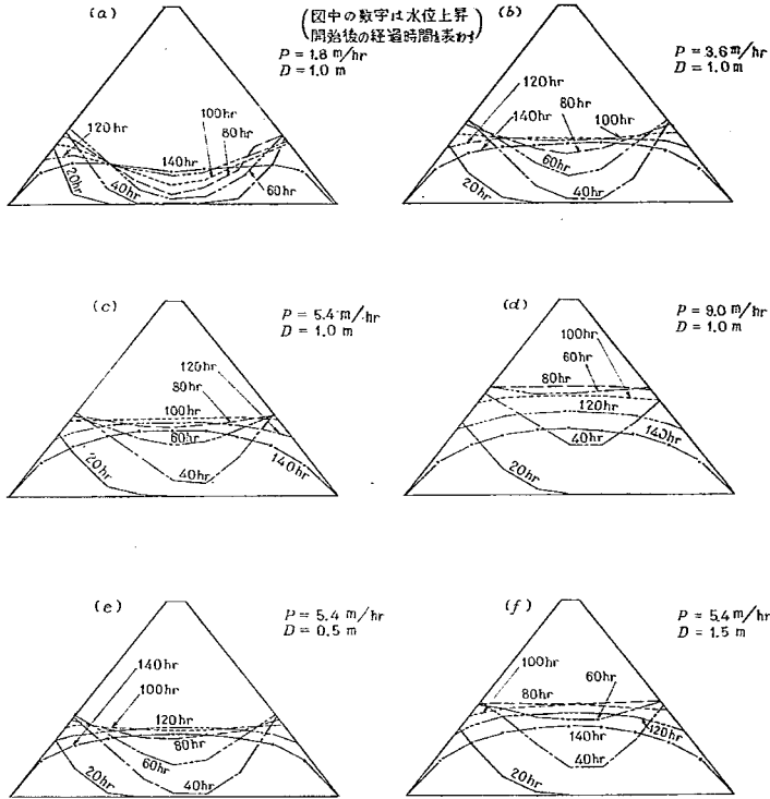
図-13 計算より求めた堤体内の自由水面の変化
