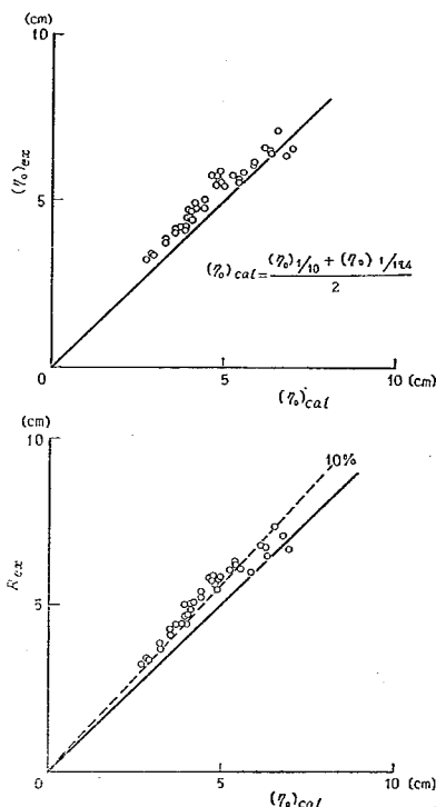
図-29 汀線においてこう配が変わる場合 の波頂高とそ上高
