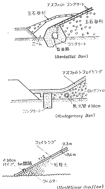
図-21 排水工の例
