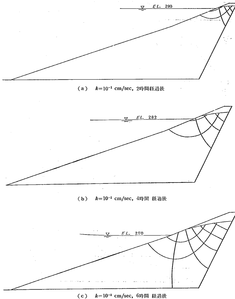
図-11 k=1 \times 10^{-1} cm/sec の場合のフローネット
