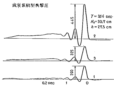
図-16 砕波衝撃圧の波形
