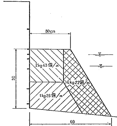
図-22 消波工の形状
