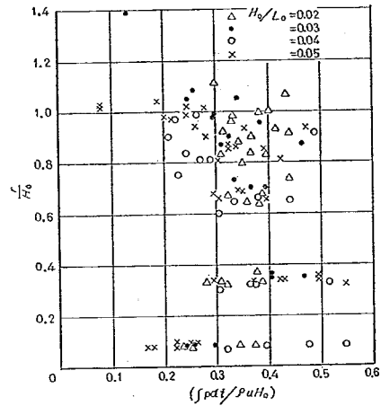
図-20 砕波衝撃圧の力積
