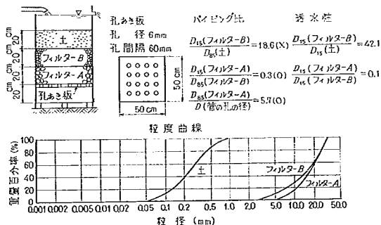
図-23 孔あき板を用いたフィルターの実験の1例
