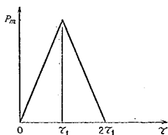
図-39 波圧の時間変化モデル
