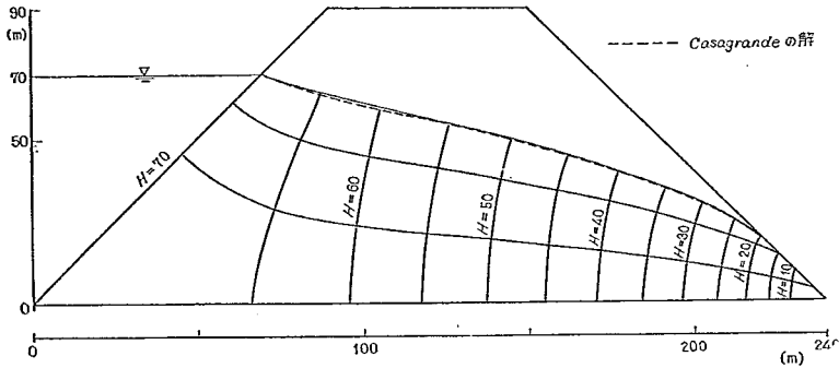
図-7 堤体定常浸透流 ( k=1.0 \times 10^{-3} cm/sec, Q=1.35 \times 10^{-4} m 3 /sec/m)
