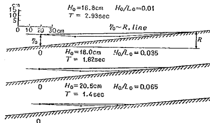
図-25 汀線より陸側におけるそ上水面形
