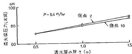
図-16 透水層の厚さと最大揚圧力の関係
