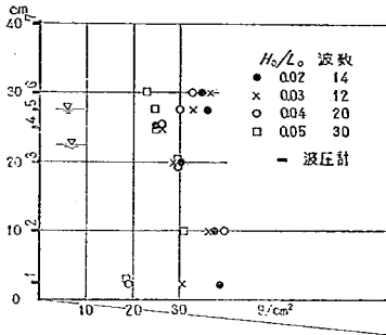
図-23 消波工の波圧減殺効果
