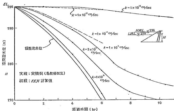
図-13 実験値と計算値の比較 (喜撰山ダム)
