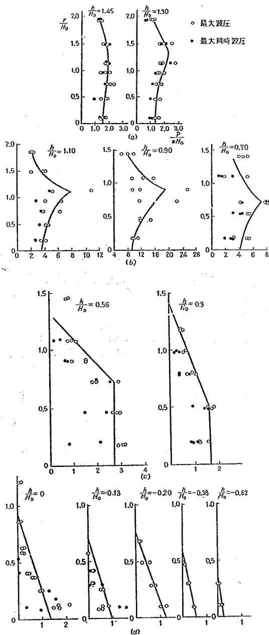
図-8 波 圧 の 鉛 直 分 布
