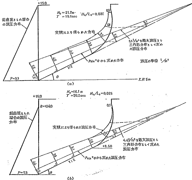
図-36 浦原海岸の波圧実験値と計算値との比較例
