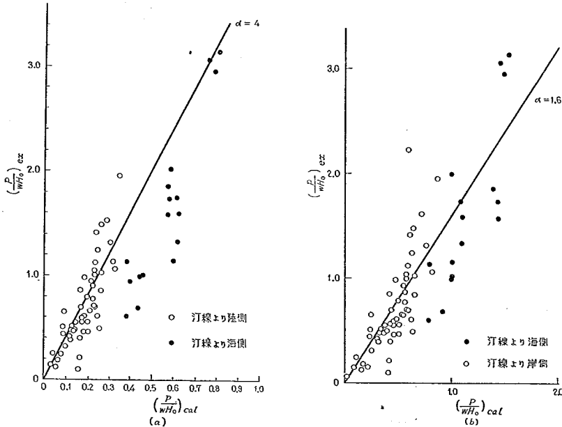
図-28 碎波圧の実験値と計算値との比較
