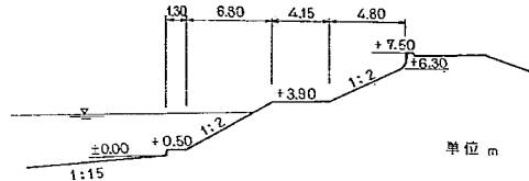
図-15 城南海岸堤防の形状
