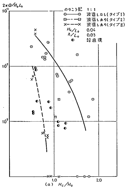
図-19 (a) 1 割堤における波返の効果
