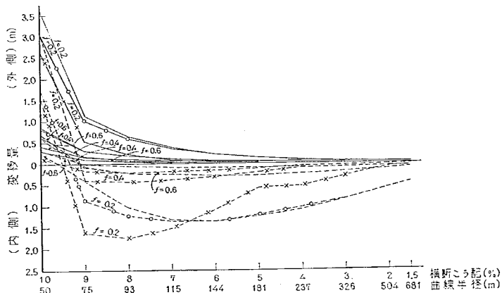
図-3-7(d) 特殊断面での最大変移量 (設計速度 V=40 \text{ km/h} )
