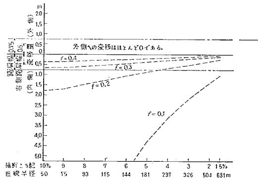
図-3-6(c) 最大変移量 (設計速度 20km/h、 V=40-20=20 )
