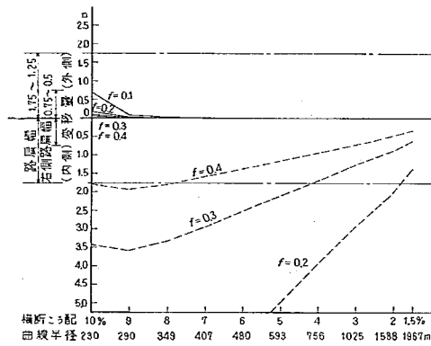
図-3-6(b) 最大変移量 (設計速度 20km/h、 V=80-20=60 )
