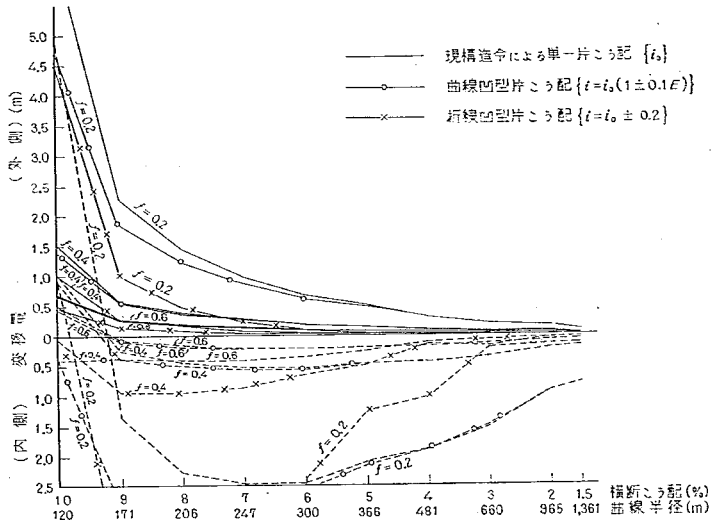
図-3-7(c) 特殊断面での最大変移量 (設計速度 V=60 \text{ km/h} )
