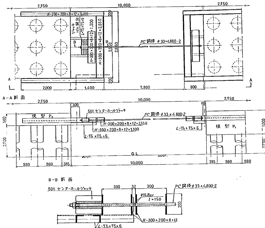
図-6.4 フーチング部载荷試験装置
