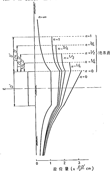
図-3.28 载荷面の変位分布
