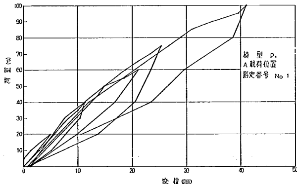
図-6.9 荷重-変位曲線 (校型 P_1 、A載荷位置、測定番号No. 1)
