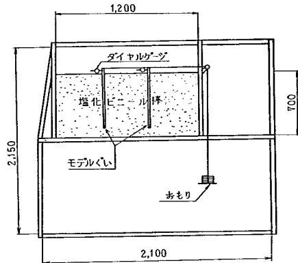
図-4.4 二次元枠モデル試験装置一般図
