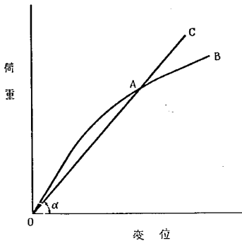
図-3.1 荷重と変位の関係
