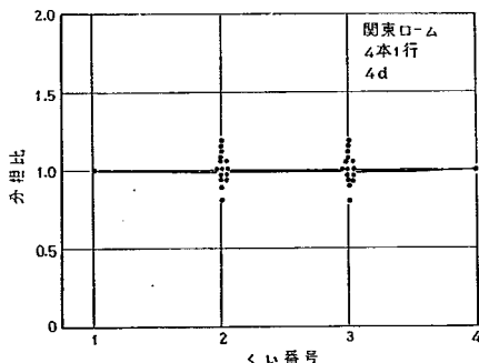
図-4.49 行構成ぐいの荷重分担割合 (関東ローム, 4本1行, 4d)
