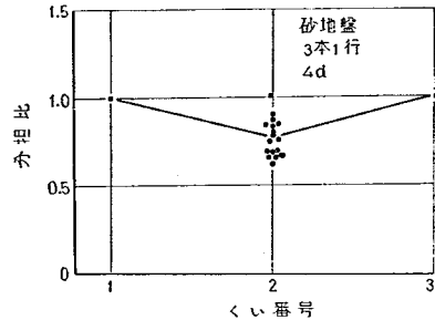
図-4.40 行構成ぐいの荷重分担割合 (砂地盤, 3本1行, 4d)
