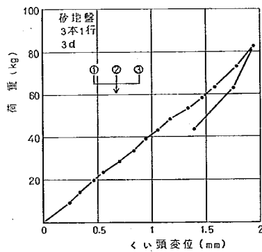
図-4.17 载荷試験結果 (3本1行, 3d, 砂地盤)
