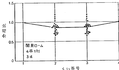
図-4.48 行構成ぐいの荷重分担割合 (関東ローム, 4本1行, 3d)
