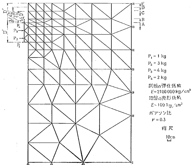
図-3.27 要素の分割と計算条件
