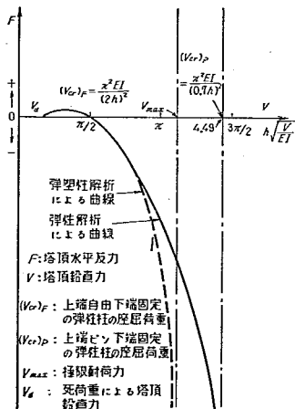
図-5.8 主塔の極限耐荷力のもつ意味
