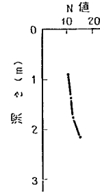
図-3.4 標準貫入試験結果
