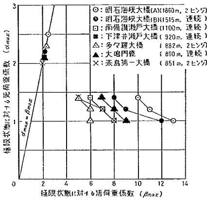
図-6.5 \alpha_{max} と \beta_{max} の関係
