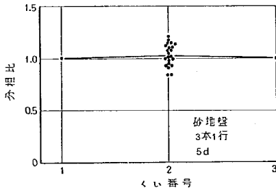
図-4.41 行構成ぐいの荷重分担割合 (砂地盤, 3本1行, 5d)
