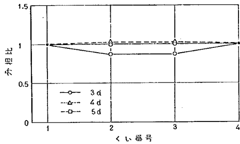
図-4.57 行構成の荷重分担割合 (関東ローム, 4本1行)
