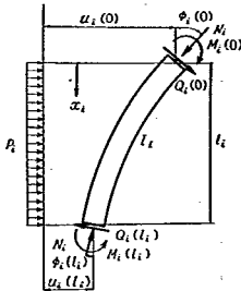
図-4.2 格間 i に作用する力
