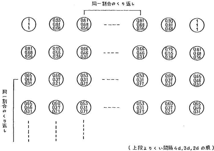
図-7.2 群ぐいの水平方向地盤反力係数の割合
