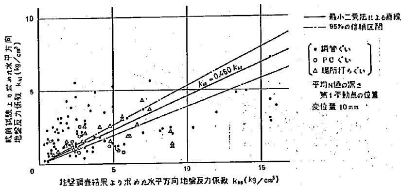
図-3.44 水平方向地盤反力係数の関係(7)
