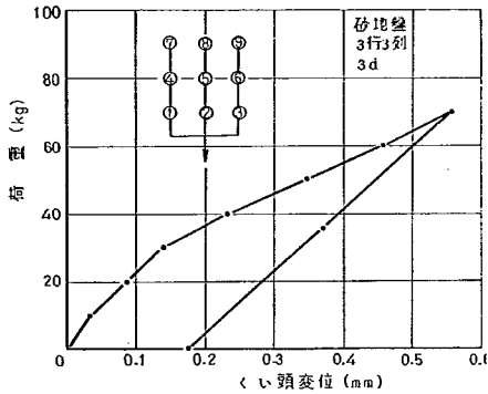
図-4.20 載荷試験結果 (3行3列, 3d, 砂地盤)
