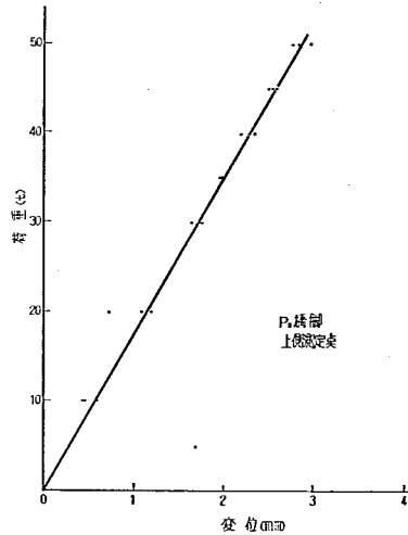
図-6.50 直線関係の推定 (4)
