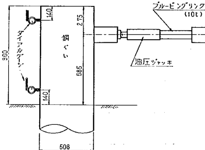
図-6.8 単ぐいの試験状況
