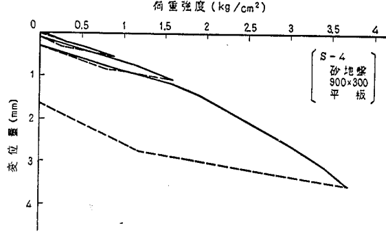
図-3.11 荷重一変位曲線(4)
