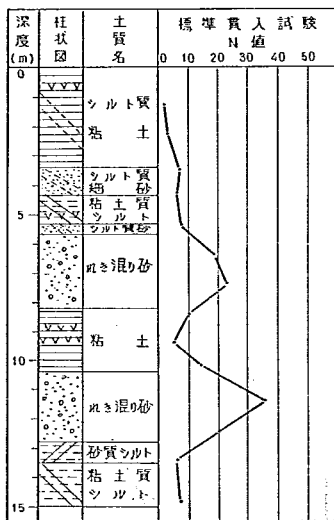
図-6.51 土質柱状図 (No. 323+9.0m)
