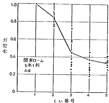
図-4.34 列構成の荷重分担割合 (関東ローム, 5本1列, 4d)
