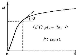
図-5.1 M-\phi-P 曲線を用いた曲げ剛性の求め方
