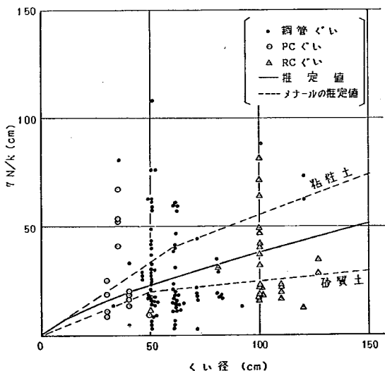
図-3.57 くい径との相関
