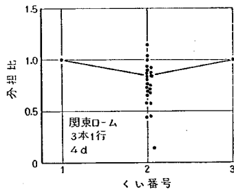
図-4.46 行構成ぐいの荷重分担割合 (関東ローム, 3本1行, 4d)
