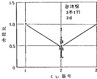
図-4.39 行構成ぐいの荷重分担割合 (砂地盤, 3本1行, 3d)
