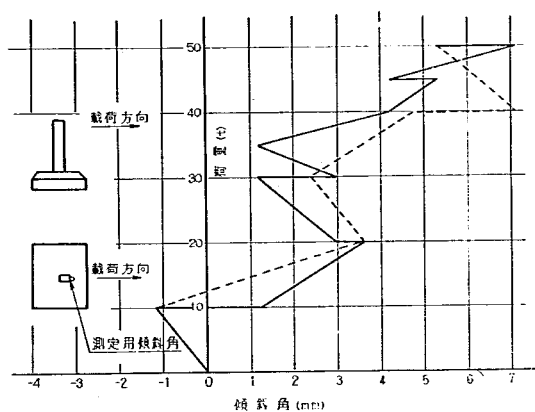
図-6.45 荷重-傾斜角曲線 (P 2 橋脚)
