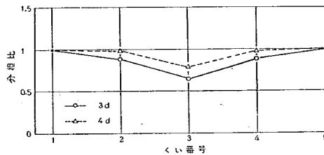
図-4.58 行構成の荷重分担割合 (関東ローム, 5本1行)
