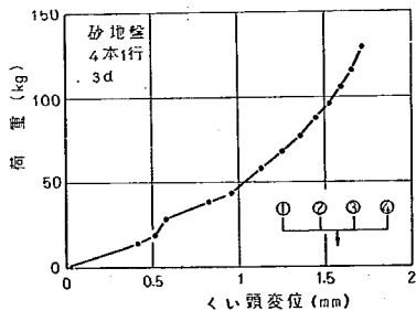
図-4.18 载荷試験結果 (4本1行, 3d, 砂地盤)
