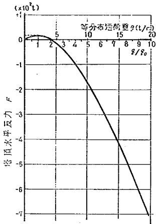
図-4.6 塔頂水平反力 F と等分布活荷重 q の関係
