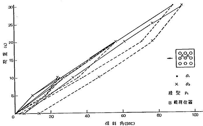
圖-6.23 荷重—傾斜角曲線 (模型P 1 , B載荷位置)
