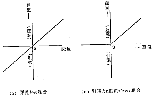
図-5.1 地盤の荷重-変位関係
