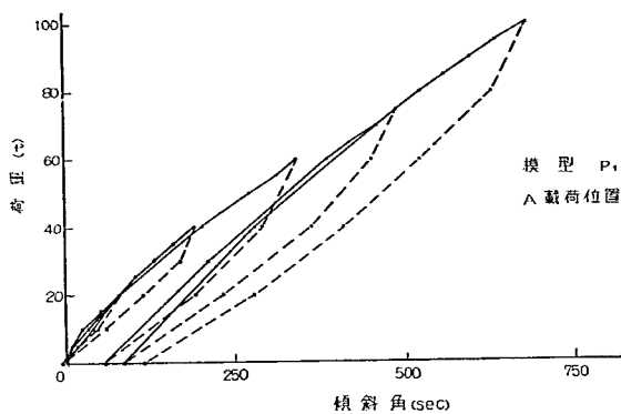
圖6.21 荷重—傾斜角曲線 (模型P 1 , A載荷位置)
