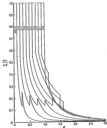
図-5.5 dm/d\phi - \phi - p 曲線
