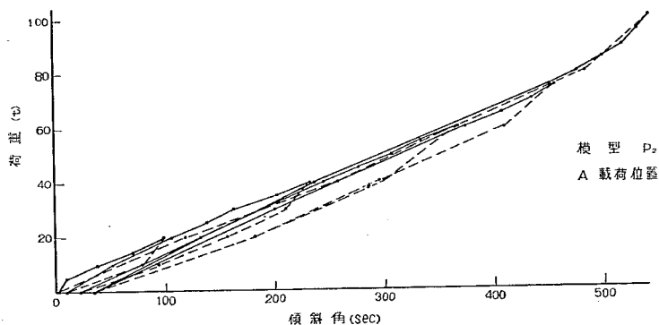
圖-6.22 荷重—傾斜角曲線 (模型P 2 , A載荷位置)
