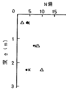
図-4.13 N値の結果
