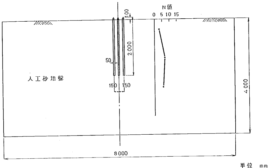
図-5.7 対象とする計算モデル
