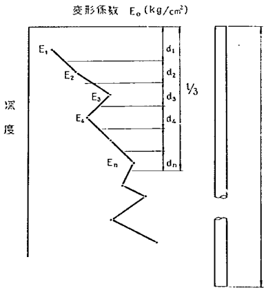
図-3.55 地盤のモデル化
