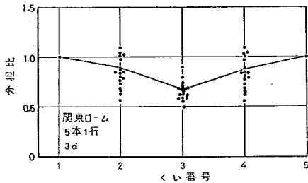
図-4.51 行構成の荷重分担割合 (関東ローム, 5本1行, 3d)
