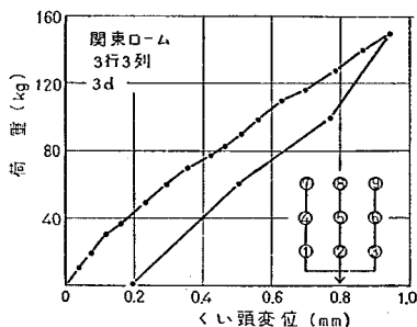
図-4.26 载荷試験結果 (3行3列, 3d, 関東ローム)
