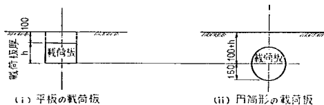
(a) 載荷板設置状況 ( h = 150 または 200 mm)
