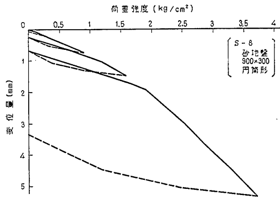
図-3.15 荷重—変位曲線(8)
