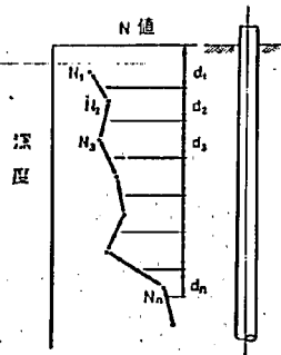
図-3.37 N 値の取扱い
