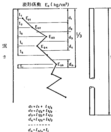
図-7.1 地盤のモデル化
