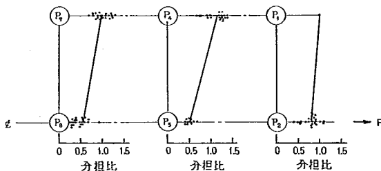
図-4.70 行列構成ぐいの荷重分担割合 (関東ローム, 3行3列, 5 d)
