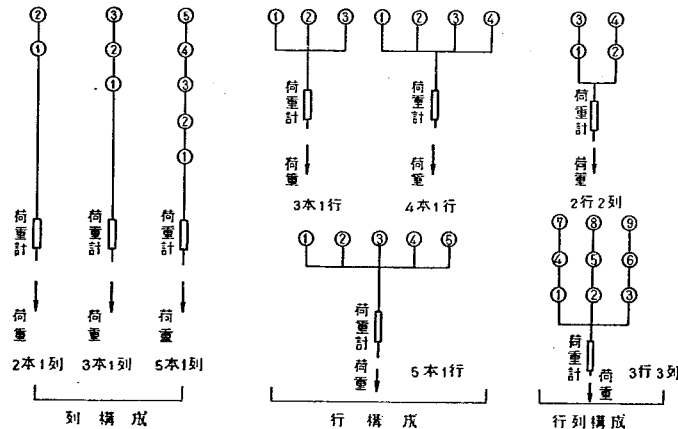
図-4.14 試験のくい構成
