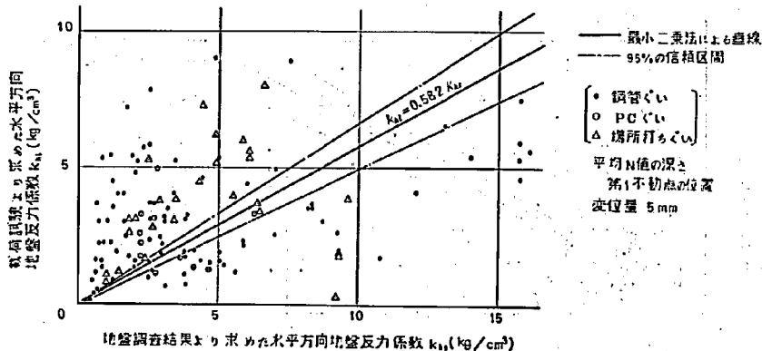
図-3.39 水平方向地盤反力係数の関係(2)
