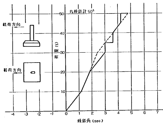
図-6.46 荷重-傾斜角曲線 (P 3 橋脚)
