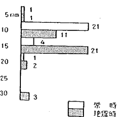
図-3.36 許容変位量の調査結果
