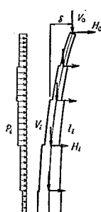
図-1.4 主塔に作用する外力と変位
