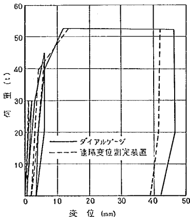
図-8.6 鉛直変位測定による比較
