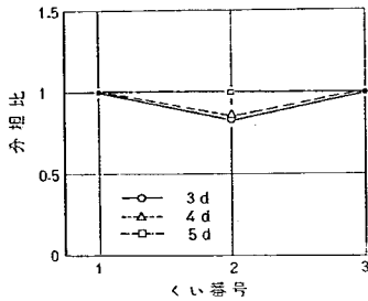
図-4.56 行構成の荷重分担割合 (関東ローム, 3本1行)
