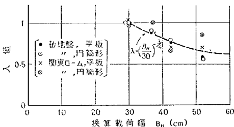
図-3.24 載荷幅に対する関係
