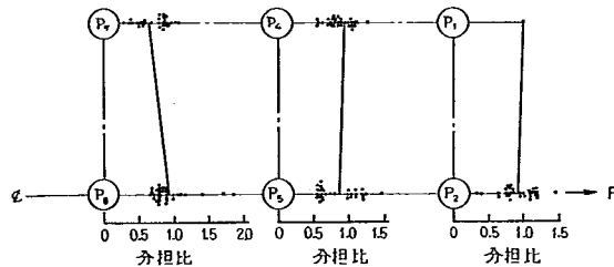
図-4.68 行列構成くいの荷重分担割合 (関東ローム, 3行3列, 3d)
