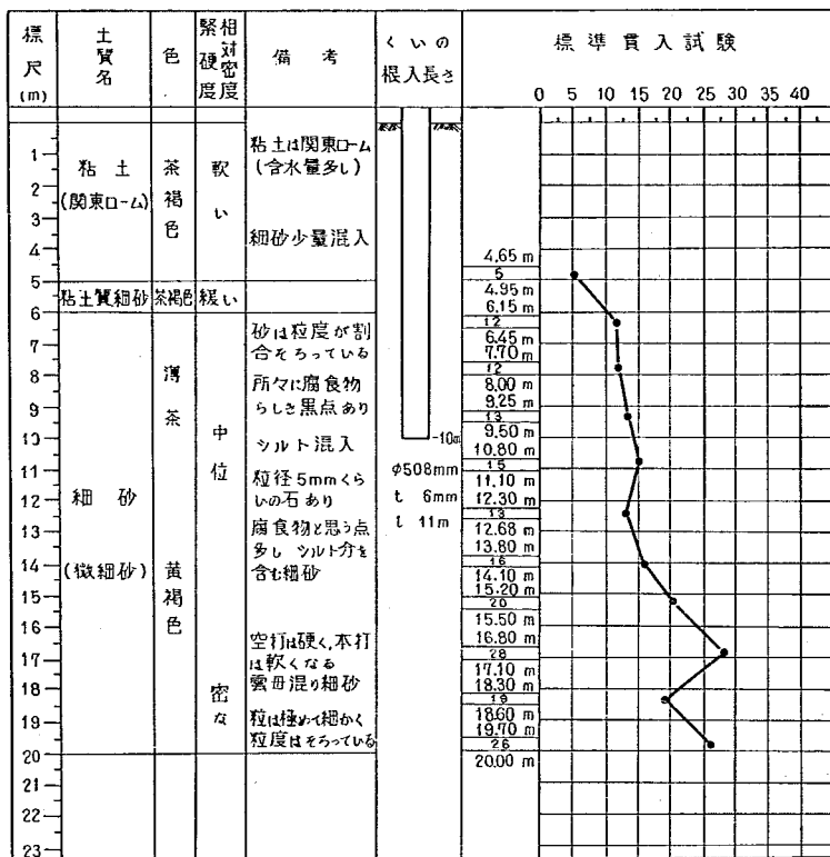
図-3.53 土質柱状図
