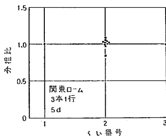
図-4.47 行構成ぐいの荷重分担割合 (関東ローム, 3本1行, 5d)
