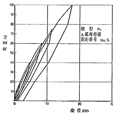
図-6.11 荷重—変位曲線 (模型 P_1 , A 載荷位置, 測定番号No. 5)
