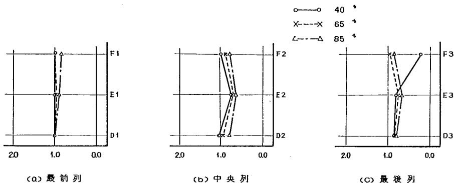
図-6.29 水平力の分担割合 (模型P 2 )
