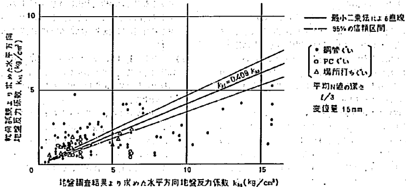
図-3.51 水平方向地盤反力係数の関係(14)
