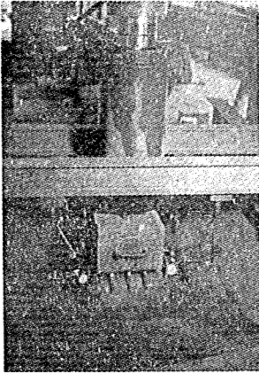
写真-3.1 砂地盤における試験状況
