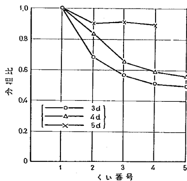
図-4.35 列ぐいの荷重分担割合 (砂地盤)
