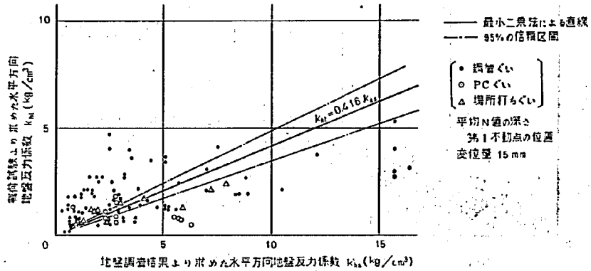
図-3.49 水平方向地盤反力係数の関係(12)
