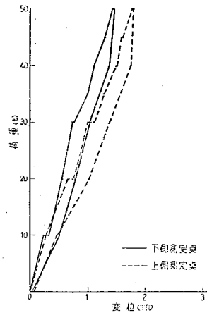
図-6.41 荷重-変位曲線 (P 2 橋脚)
