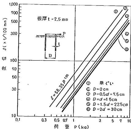
図-4.7 2列ぐいの荷重-変位曲線 (2)
