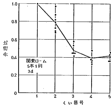
図-4.33 列構成の荷重分担割合 (関東ローム, 5本1列, 3d)
