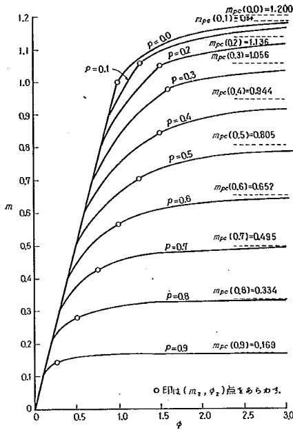
図-5.4 m - \phi - p 曲線
