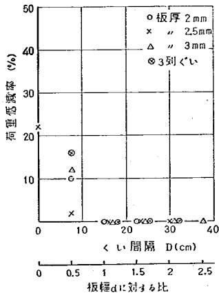
図-4.9 2列ぐいの荷重分担割合
