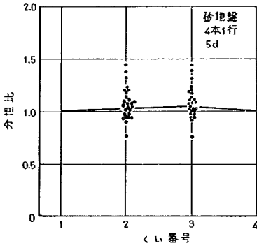
図-4.43 行構成ぐいの荷重分担割合 (砂地盤, 4本1行, 5d)
