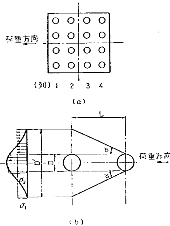
図-2.1 荷重分布状態(くい基礎の設計編による)
