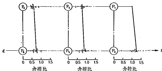
図-4.69 行列構成ぐいの荷重分担割合 (関東ローム, 3行3列, 4 d)
