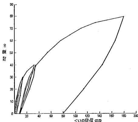
図-6.56 荷重-変位曲線 (No.1, No.3の平均値)
