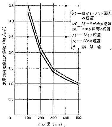
図-3.54 水平方向地盤反力係数の計算結果
