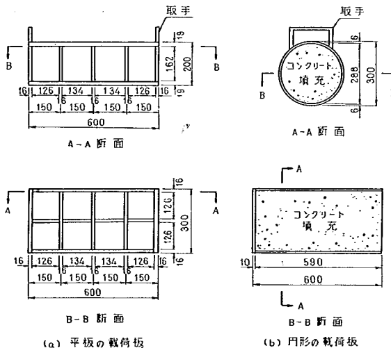
図-3.2 載荷板の形状 (600×300mm)
