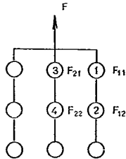
図-4.71 行列構成ぐいの重ね合わせ
