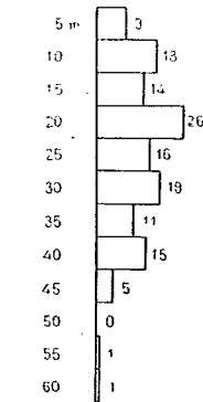
図-3.31 ぐいの根入れ長さによる分類
