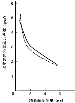
図-6.26 地表面変位量との関係
