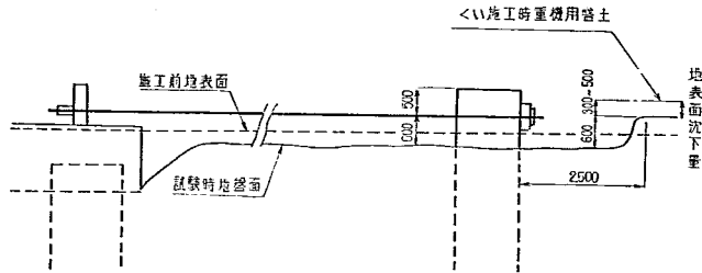
図-6.53 試験状況
