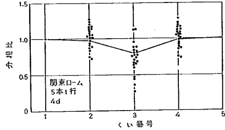
図-4.52 行構成の荷重分担割合 (関東ローム, 5本1行, 4d)
