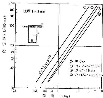
図-4.6 2列ぐいの荷重-変位曲線 (1)
