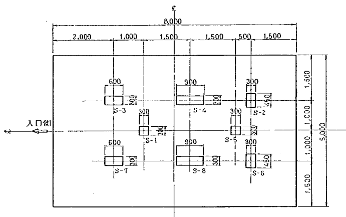
図-3.5 砂地盤における載荷板の配置
