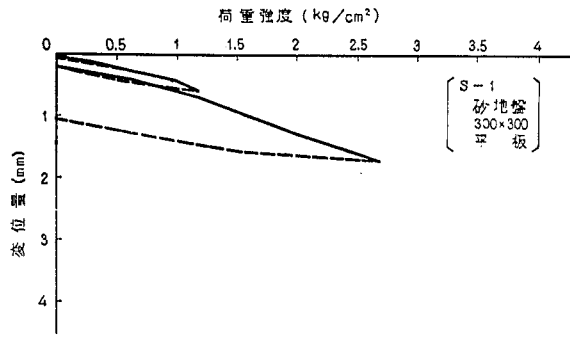
図-3.8 荷重一変位曲線(1)
