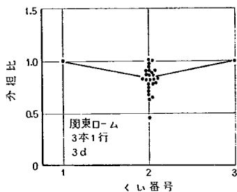
図-4.45 行構成ぐいの荷重分担割合 (関東ローム, 3本1行, 3d)
