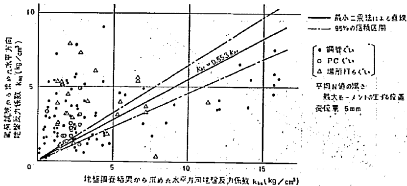
図-3.38 水平方向地盤反力係数の関係(1)
