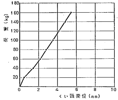
図-4.21 載荷試験結果 (単ぐい, 閉端ローム)
