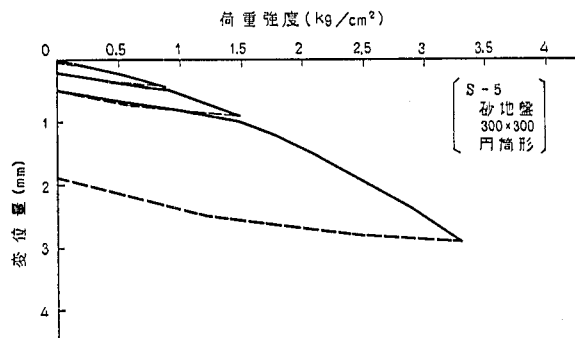
図-3.12 荷重—変位曲線(5)
