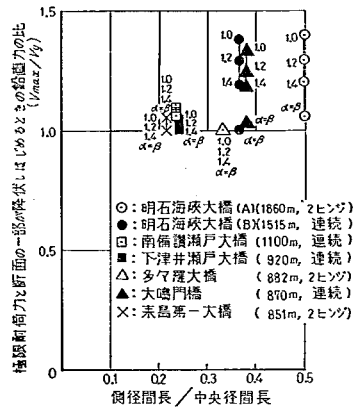
図-6.6 V_{max}/V_y と側径間長/中央径間長の関係
