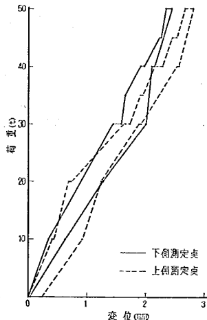
図-6.44 荷重-変位曲線 (P 3 橋脚)
