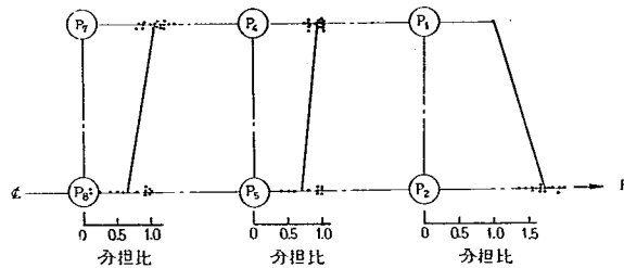
図-4.66 行列構成くいの荷重分担割合 (砂地盤, 3行3列, 4d)
