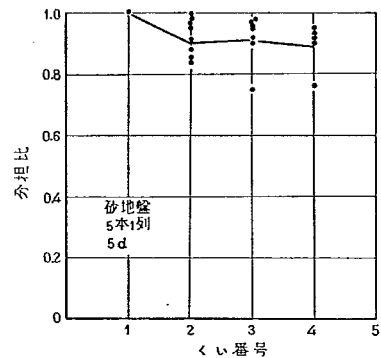
図-4.32 列構成の荷重分担割合 (砂地盤, 5本1列, 5d)
