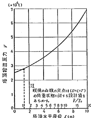
図-2.3 塔頂鉛直反力 V と塔頂水平変位 \delta の関係
