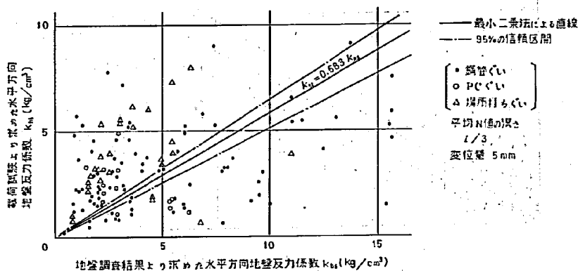
図-3.41 水平方向地盤反力係数の関係(4)
