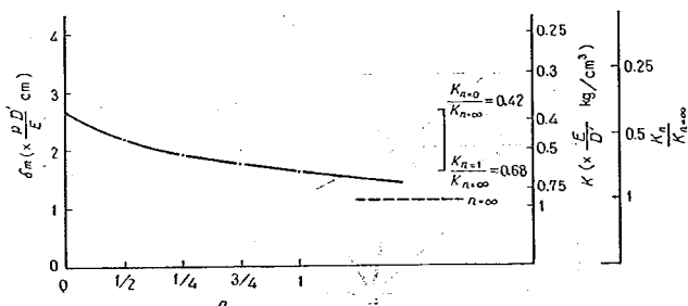
図-3.29 n と K_n/K_{n=\infty} との関係
