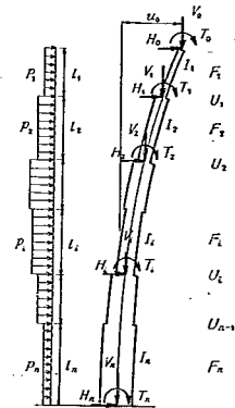
図-4.1 変断面主塔に作用する外力と変位
