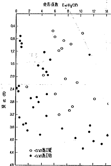
図-6.52 くい施工前後の土質性状の変化
