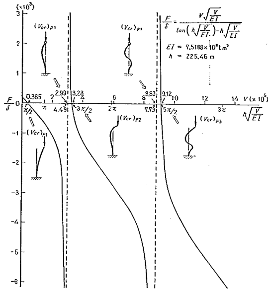
図-3.2 等断面弾性柱に作用する垂直力 V と水平反力 F の関係
