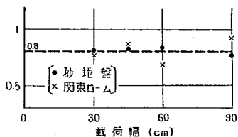
図-3.25 載荷板の相異による割合
