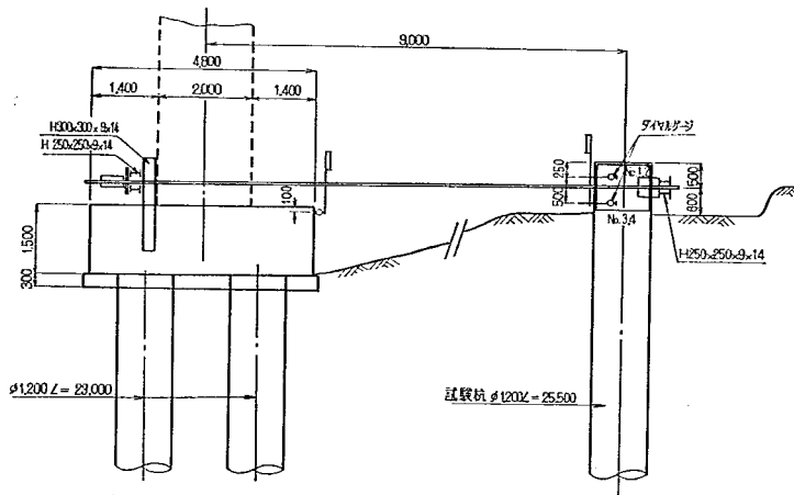
図-6.54 荷重装置側面図
