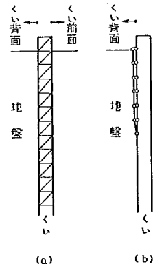
図-5.2 節点の取扱い
