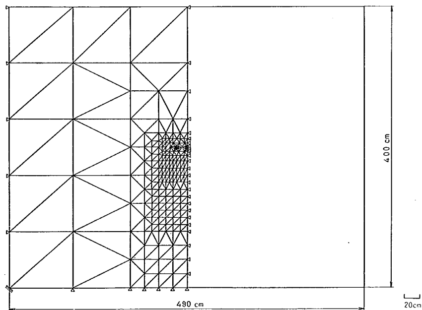
図-5.9 3本1行構成の要素分割
