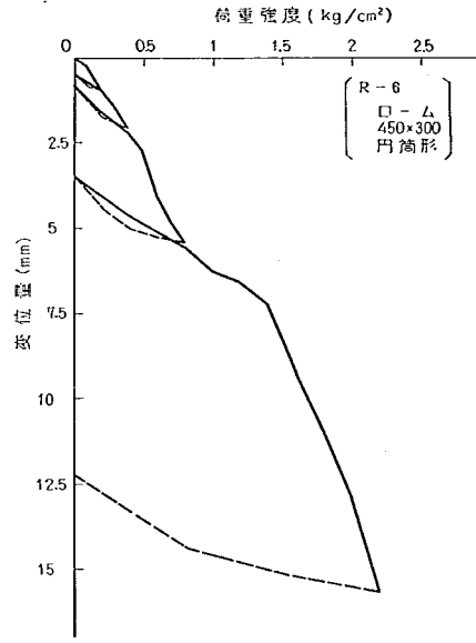
図-3.21 荷重一変位曲線 (14)
