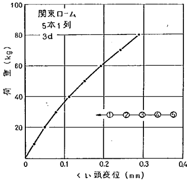
図-4.22 載荷試験結果 (5本1列, 3d, 閉端ローム)
