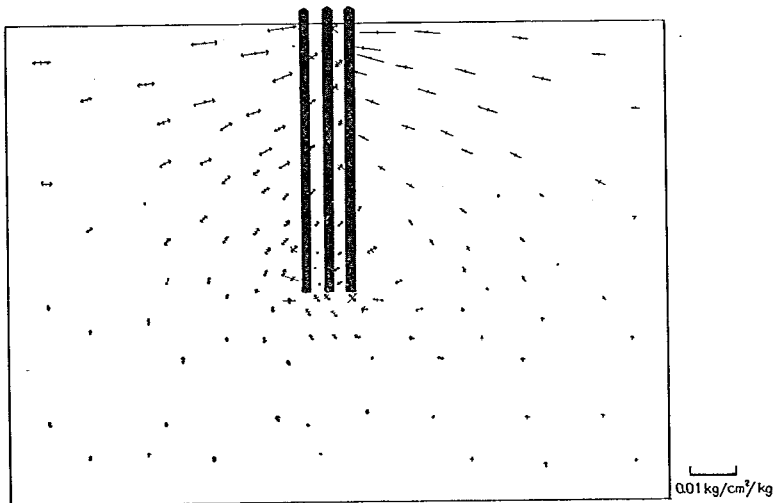
(a) STEP 1 (弾性地盤の場合)
