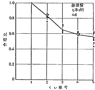
図-4.31 列構成の荷重分担割合 (砂地盤, 5本1列, 4d)
