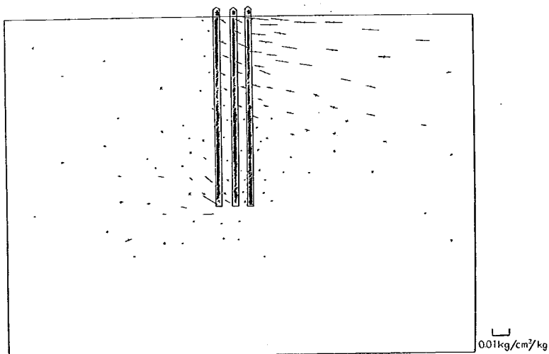
(g) STEP 10 (引張抵抗を無視した場合)
