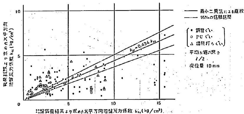
図-3.47 水平方向地盤反力係数の関係 (10)
