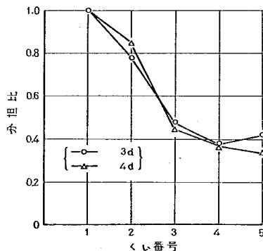
図-4.38 列構成の荷重分担割合 (関東ローム)
