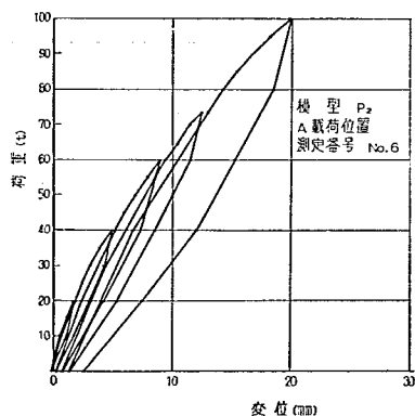
図-6.14 荷重—変位曲線 (模型 P_2 , A 載荷位置, 測定番号No. 6)
