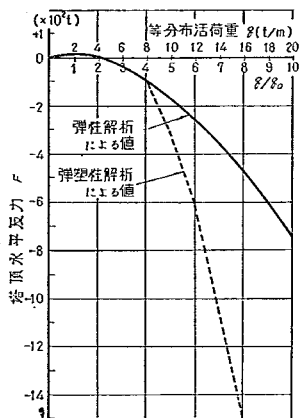
図-5.10 塔頂水平反力 F と等分布活荷重 q の関係
