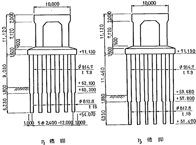
図-6.32 橋脚一般図
