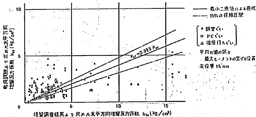
図-3.48 水平方向地盤反力係数の関係 (11)
