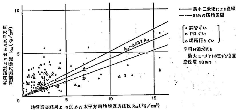
図-3.43 水平方向地盤反力係数の関係(6)
