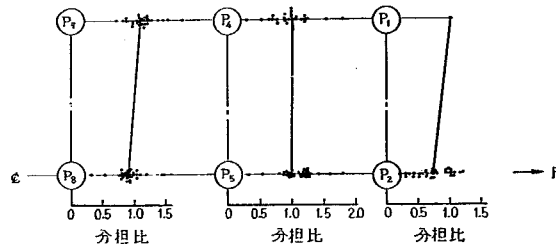
図-4.67 行列構成くいの荷重分担割合 (砂地盤, 3行3列, 5d)
