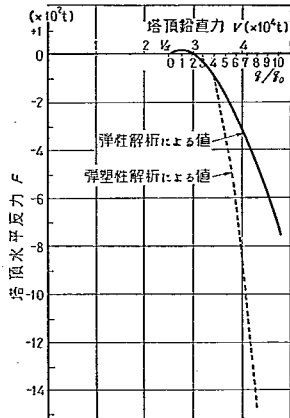
図-5.12 塔頂水平反力 F と塔頂鉛直力 V の関係
