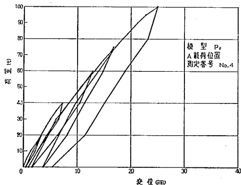
図-6.13 荷重—変位曲線 (模型 P_2 , A 載荷位置, 測定番号No. 4)
