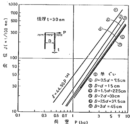
図-4.8 2列ぐいの荷重-変位曲線 (3)
