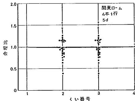
図-4.50 行構成ぐいの荷重分担割合 (関東ローム, 4本1行, 5d)
