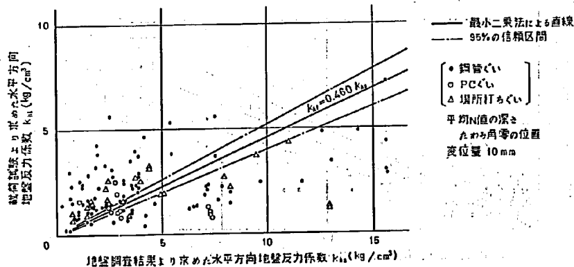
図-3.45 水平方向地盤反力係数の関係(8)
