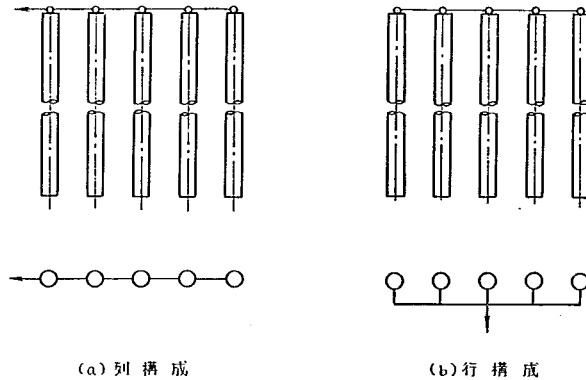
図-4.2 くい群の分解
