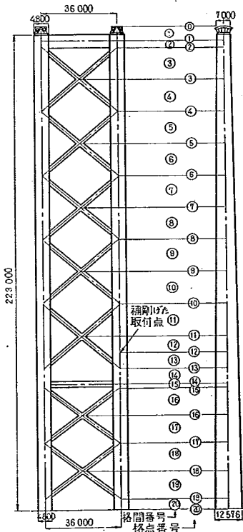
図-4.5 本四1,500m吊橋主塔の一般図
