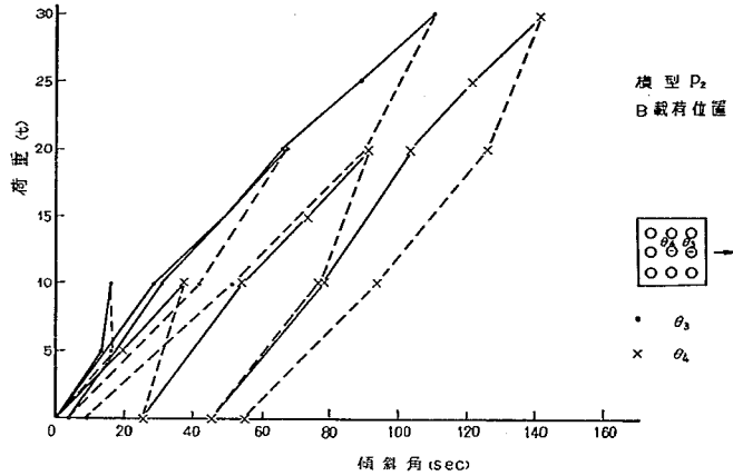
図-6.24 荷重—傾斜角曲線 (模型P2, B載荷位置)
