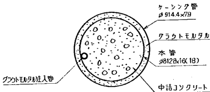
図-6.33 基礎くい断面図
