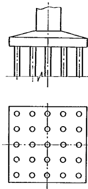
図-4.1 くい基礎
