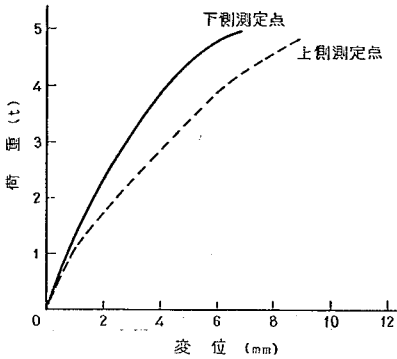
図-6.7 単ぐいの荷重-変位曲線
