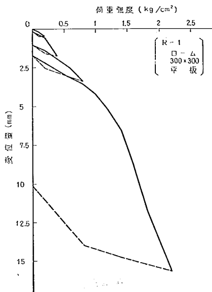
圖-3.16 荷重—変位曲線(9)
