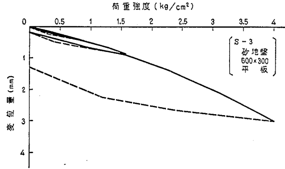
図-3.10 荷重一変位曲線(3)
