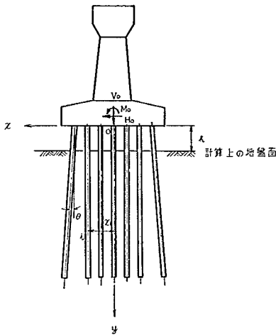
図-6.27 群ぐいの計算
