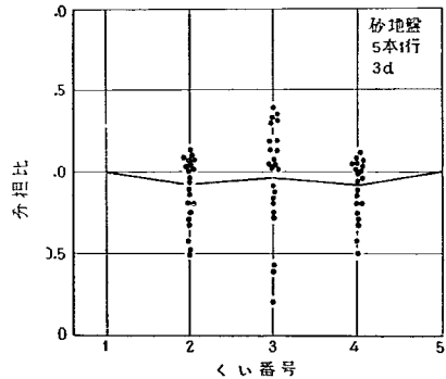
図-4.44 行構成ぐいの荷重分担割合 (砂地盤, 5本1行, 3d)
