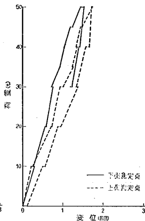
図-6.40 荷重-変位曲線 (P 2 橋脚)
