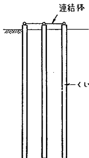
図-5.4 連結棒による結合
