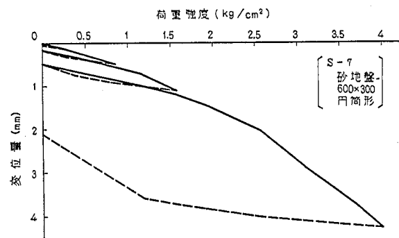
図-3.14 荷重—変位曲線(7)
