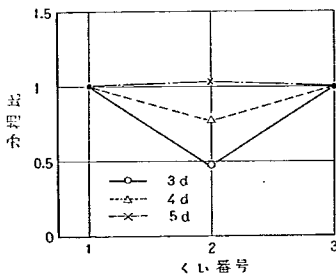
図-4.53 行構成の荷重分担割合 (砂地盤, 3本1行)
