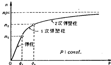
図-5.2 m - \phi 曲線
