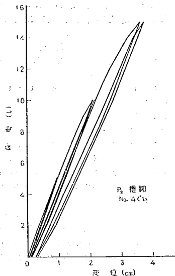
図-6.37 単くいの水平載荷試験 ( P_2 橋脚)
