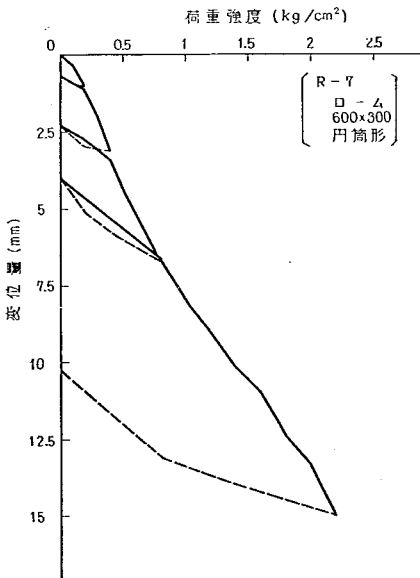
図-3.22 荷重一変位曲線 (15)
