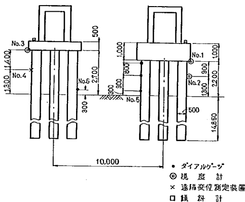
図-6.6 変位の測定位置
