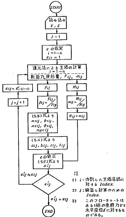
図-5.6 主塔の弾塑性解析のフローチャート
