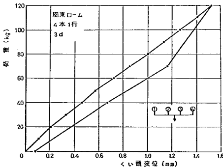
図-4.24 載荷試験結果 (4本1行, 3d, 閉端ローム)
