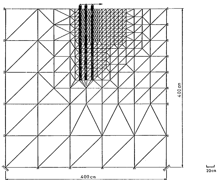
図-5.8 3本1列構成の要素分割
