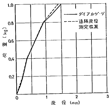
図-8.2 室内における検定結果
