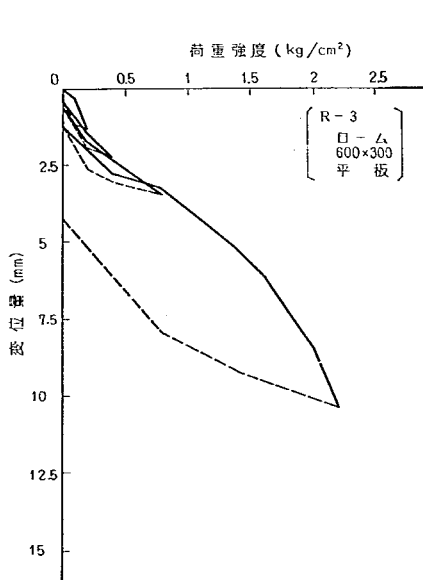
圖-3.18 荷重—変位曲線(11)
