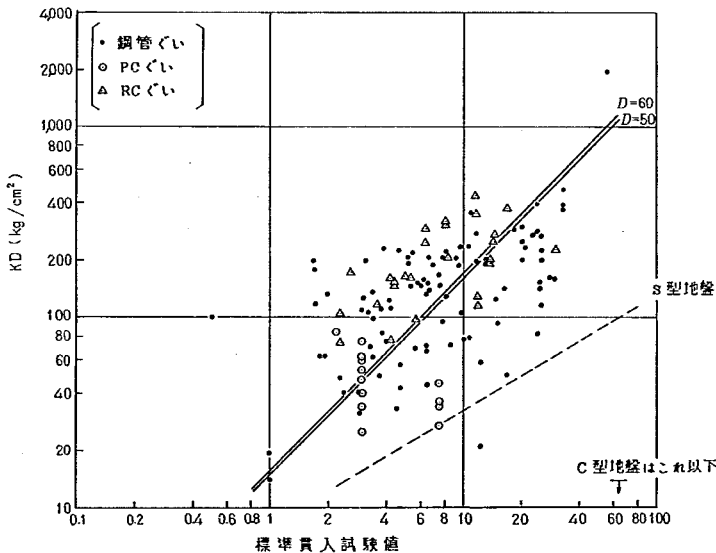
図-3.58 非線型性理論との比較
