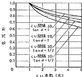
図-2.2 水平荷重の方向に1列に並んだ群ぐいの低減率 (玉野、大内による)
