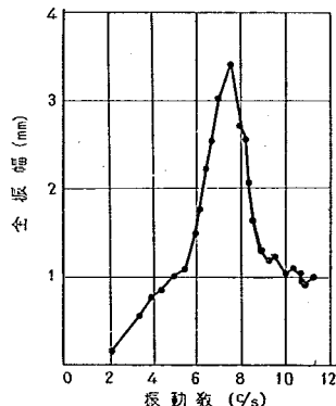
図-8.7 振動測定例
