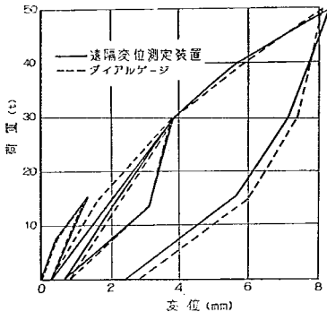
図-8.5 プレキャストウエルの試験での対比
