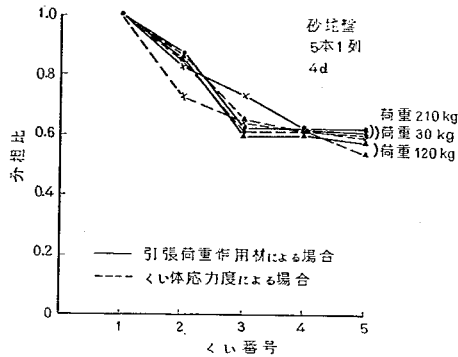
(b) 4 d の場合
