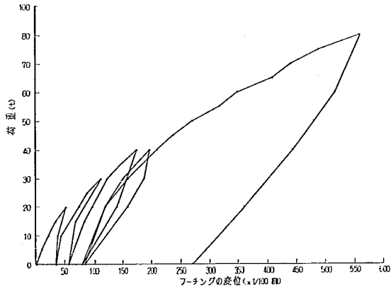
図-6.58 群ぐいの荷重-変位曲線
