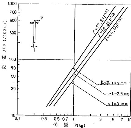
図-4.5 単ぐいの水平载荷試験結果
