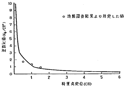
図-6.59 単ぐいの水平方向地盤反力係数の換算
