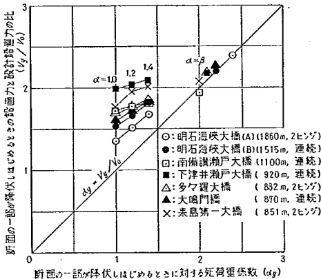
図-6.3 \alpha_\gamma と V_y/V_0 の関係
