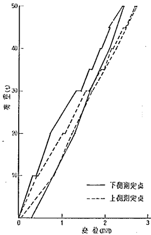
図-6.42 荷重-変位曲線 (P 3 橋脚)
