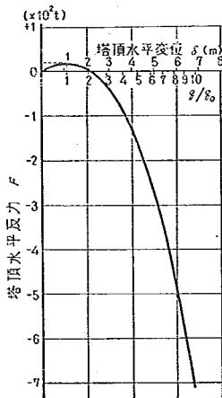
図-4.7 塔頂水平反力 F と塔頂水平変位 \delta の関係
