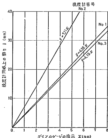
図-6.5 換度計較正結果
