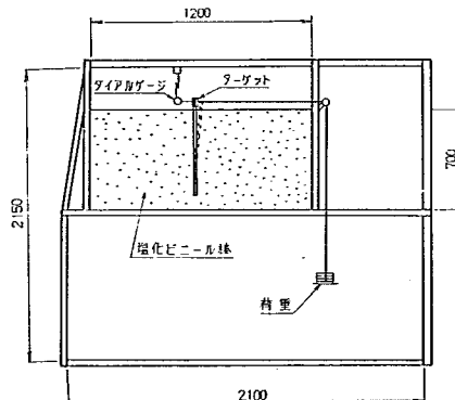
図-8.1 遠隔変位測定装置の検定方法
