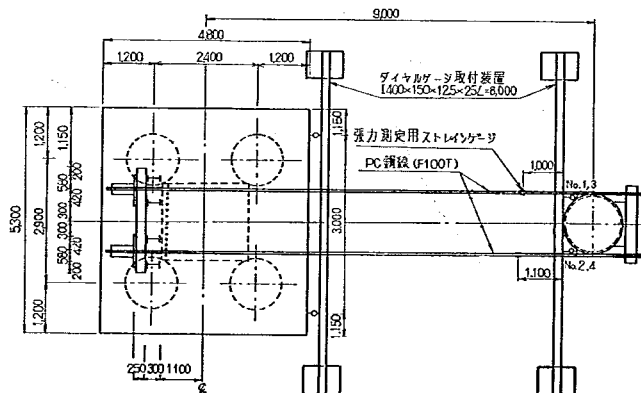
図-6.55 荷重装置平面図
