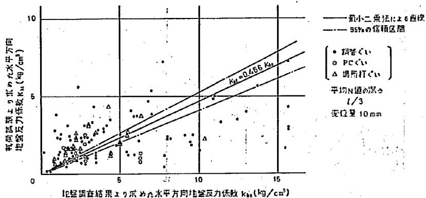
図-3.46 水平方向地盤反力係数の関係 (9)
