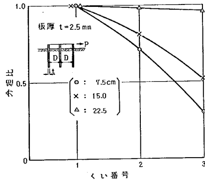
図-4.11 各くいの分担荷重
