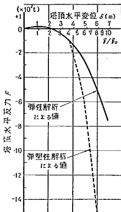
図-5.11 塔頂水平反力 F と塔頂水平変位 \delta の関係
