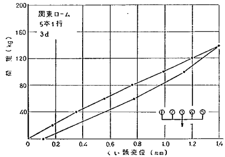
図-4.25 載荷試験結果 (5本1行, 3d, 閉端ローム)
