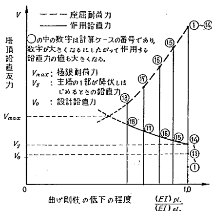
図-5.7 主塔の極限耐荷力の求め方
