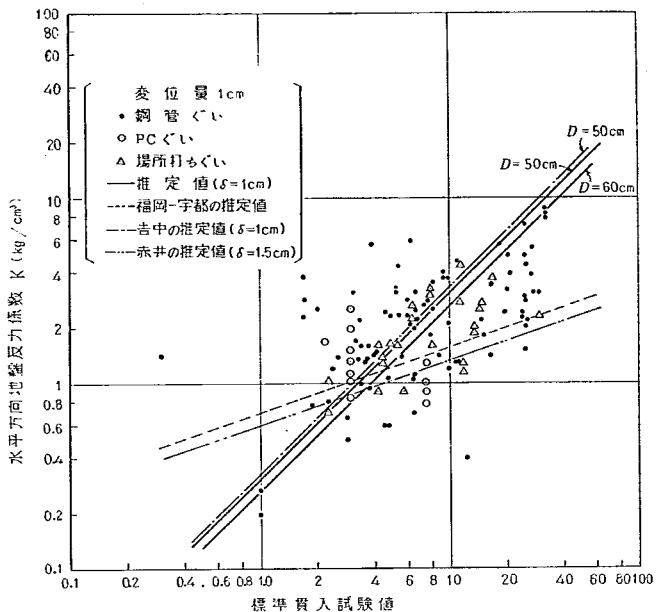
図-3.56 標準貫入試験値との比較
