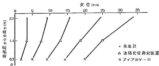
図-8.4 変形状況での比較
