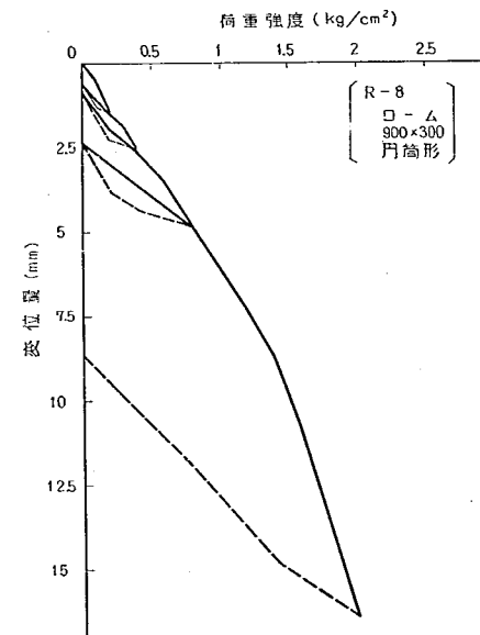
図-3.23 荷重一変位曲線 (16)
