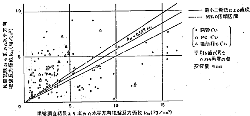
図-3.40 水平方向地盤反力係数の関係(3)
