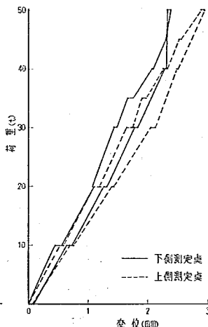
図-6.43 荷重-変位曲線 (P 3 橋脚)
