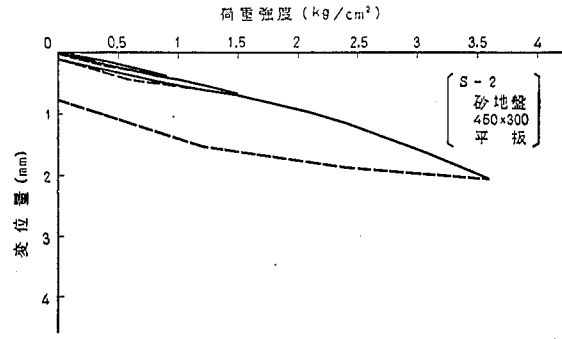
図-3.9 荷重一変位曲線(2)
