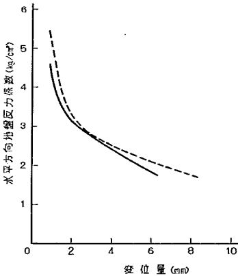
図-6.25 単いりの水平方向地盤反力係数
