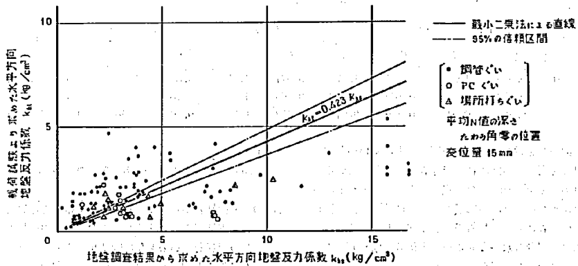
図-3.50 水平方向地盤反力係数の関係(13)
