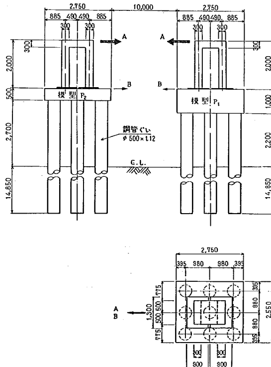
図-6.2 試験模型の形状寸法
