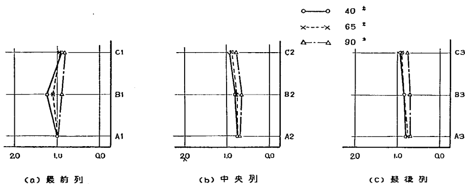
図-6.28 水平力の分担割合 (模型P 1 )
