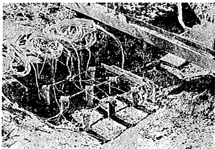
写真-4.2 試験状況(関東ローム)
