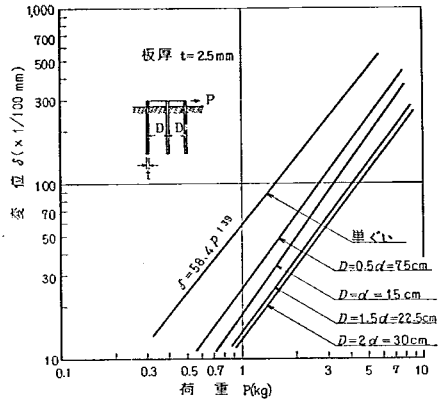
図-4.10 3列ぐいの荷重-変位曲線
