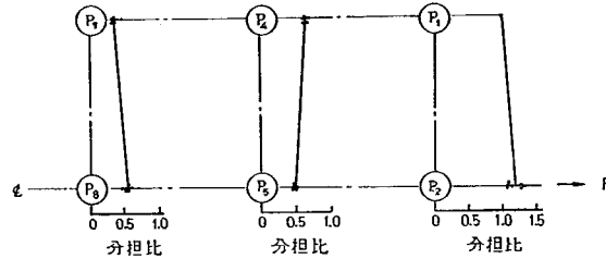
図-4.65 行列構成くいの荷重分担割合 (砂地盤, 3行3列, 3d)
