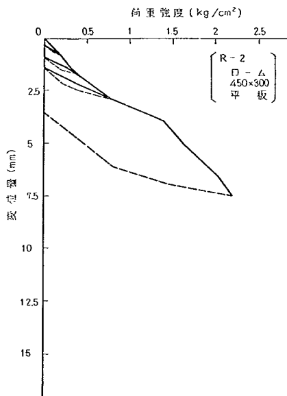
圖-3.17 荷重—変位曲線(10)
