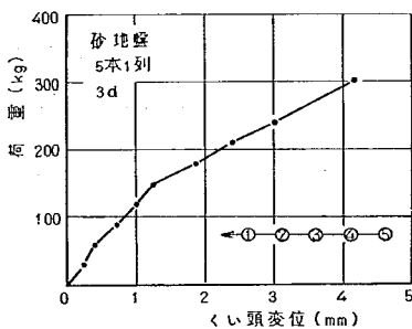
図-4.16 载荷試験結果 (5本1列, 3d, 砂地盤)
