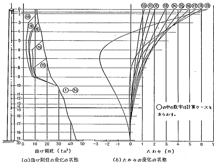
図-5.9 主塔の弾塑性変形形状
