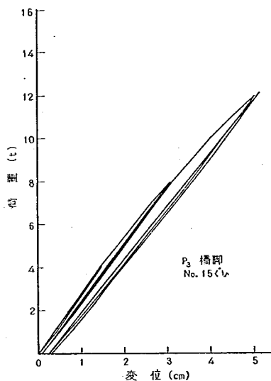
図-6.38 単くいの水平載荷試験 ( P_3 橋脚)
