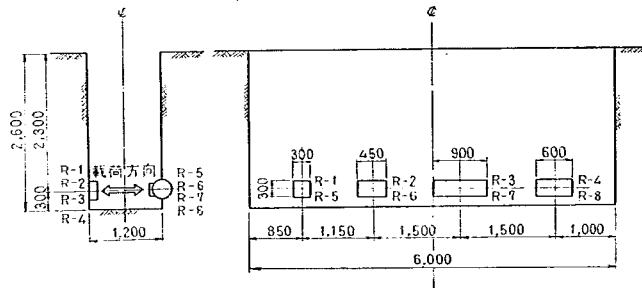
図-3.7 関東ロームにおける載荷板の配置
