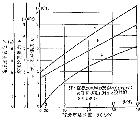
図-2.2 塔頂水平変位 \delta , 塔頂鉛直反力 V , ケーブル水平張力 H と等分布活荷重 q の関係
