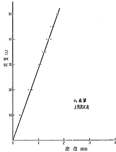
図-6.48 直線関係の推定 (2)
