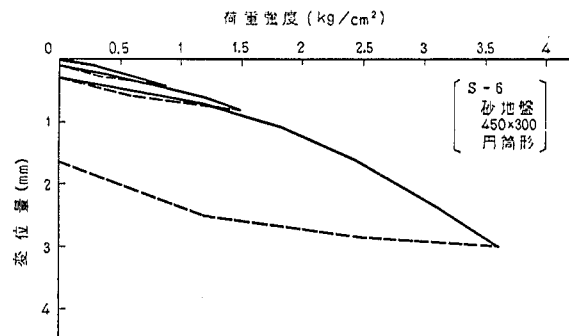
図-3.13 荷重—変位曲線(6)
