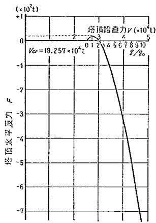
図-4.8 塔頂水平反力 F と塔頂鉛直力 V の関係
