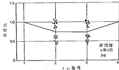
図-4.42 行構成ぐいの荷重分担割合 (砂地盤, 4本1行, 3d)
