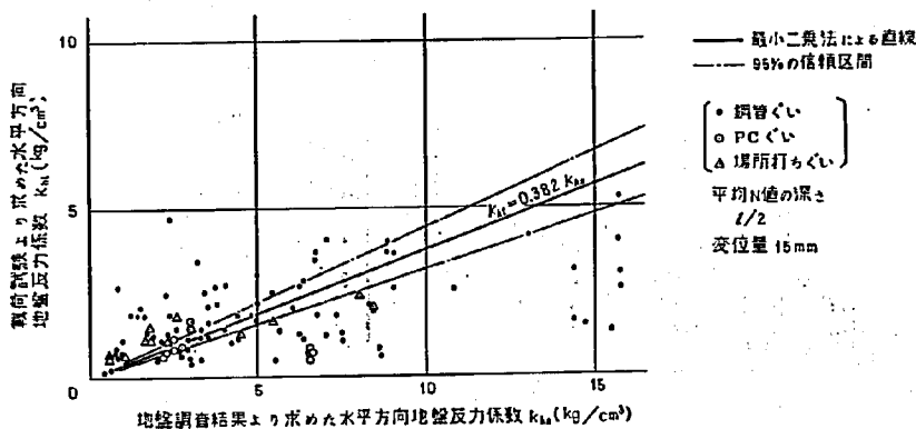
図-3.52 水平方向地盤反力係数の関係 (15)
