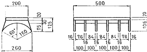
図-3.3 当て板 (600×300, 900×300用)
