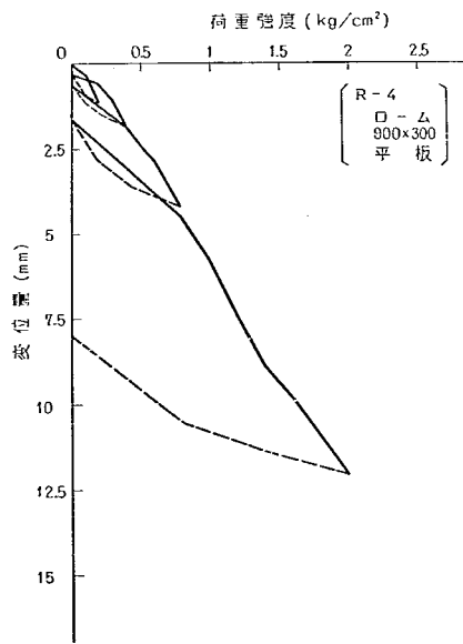
圖-3.19 荷重—変位曲線(12)
