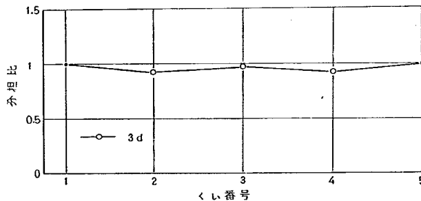
図-4.55 行構成の荷重分担割合 (砂地盤, 5本1行)
