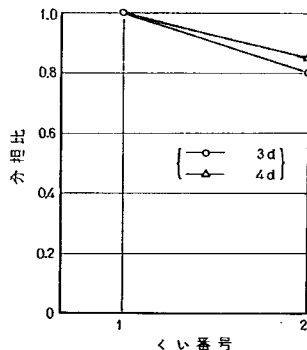
図-4.36 列ぐいの荷重分担割合 (関東ローム)
