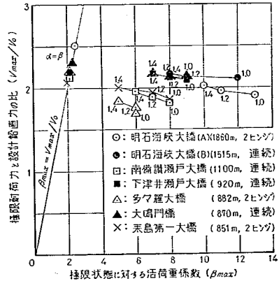
図-6.2 \beta_{max} と V_{max}/V_0 の関係
