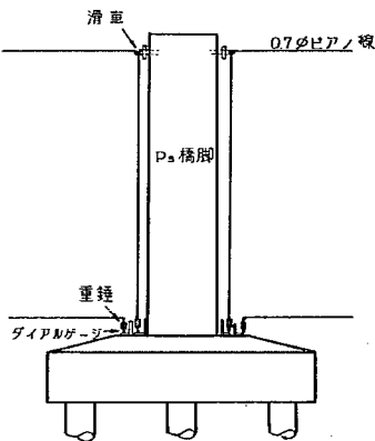
図-6.36 測定装置
