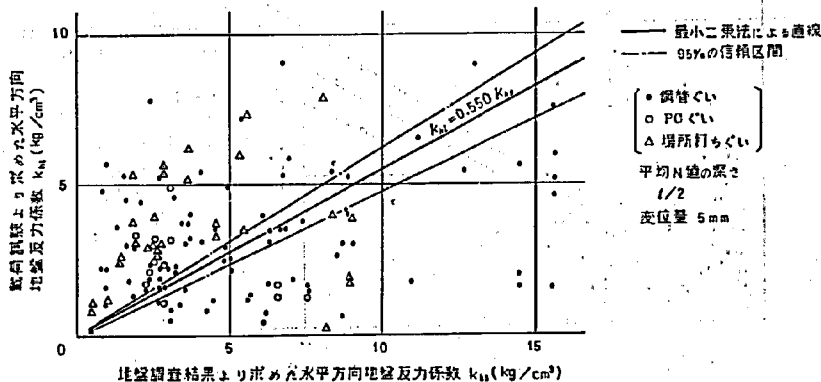
図-3.42 水平方向地盤反力係数の関係(5)
