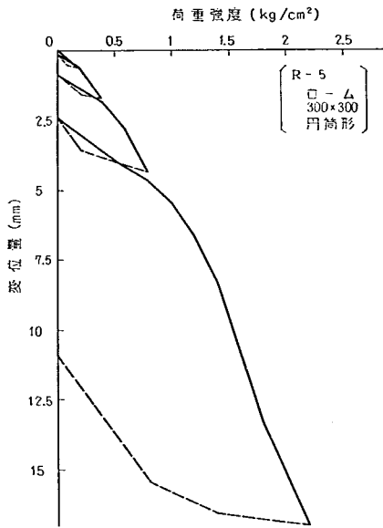
図-3.20 荷重一変位曲線 (13)
