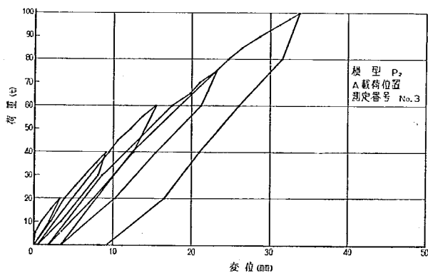
図-6.12 荷重—変位曲線 (模型 P_2 , A 載荷位置, 測定番号No. 3)
