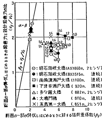
図-6.4 \beta_\gamma と V_y/V_0 の関係
