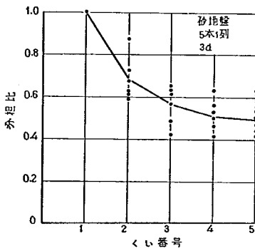
図-4.30 列構成の荷重分担割合 (砂地盤, 5本1列, 3d)
