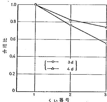
図-4.37 列ぐいの荷重分担割合 (関東ローム)
