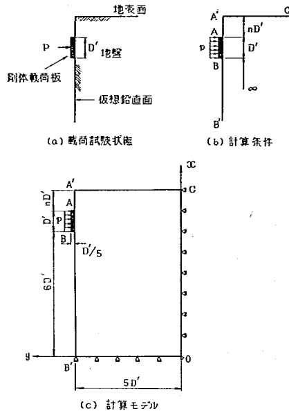
図-3.26 計算のモデル化
