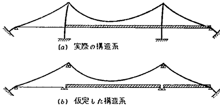
図-1.2 主塔の塔頂に作用する垂直力と水平変位を計算するときの吊橋造系の仮定
