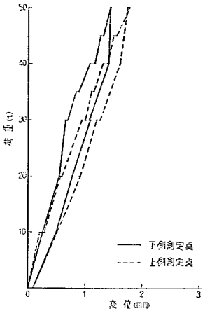
図-6.39 荷重-変位曲線 (P 2 橋脚)
