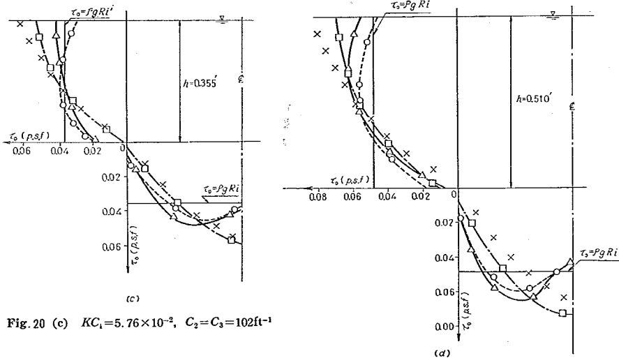
Fig. 20 (d) KC_1 = 6.18 \times 10^{-2}, C_2 = C_3 = 102 \text{ ft}^{-1}
