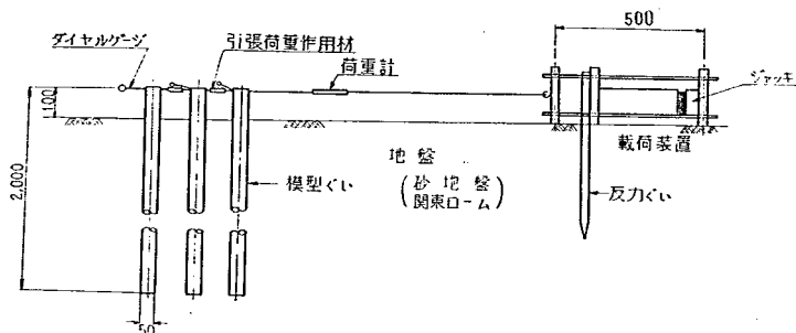
図-4.12 試験装置
