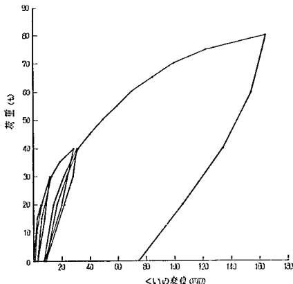
図-6.57 荷重-変位曲線 (No.2, No.4の平均値)
