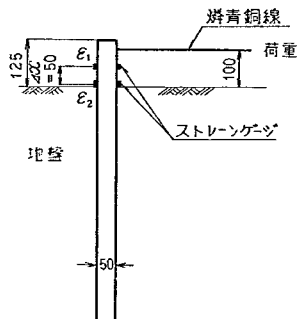
図-4.28 くい体の応力度の測定
