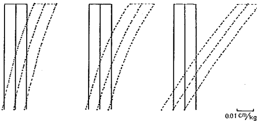
(a) 弾性地盤の場合 (b) 背面付着力一部無視の場合 (c) 引張無視の場合
