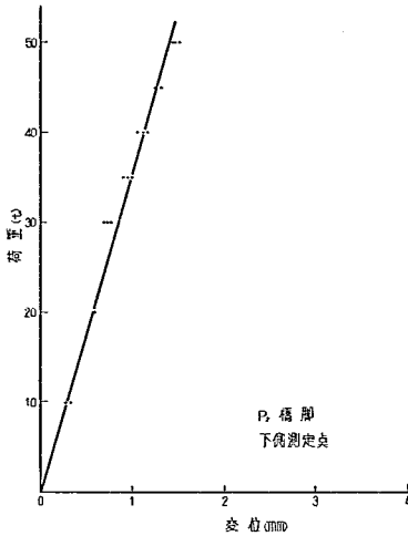
図-6.47 直線関係の推定 (1)
