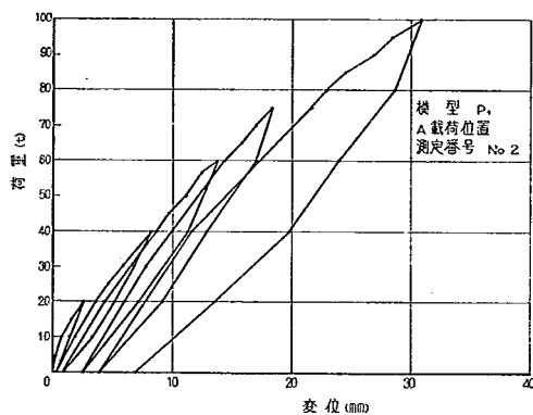
図-6.10 荷重—変位曲線 (模型 P_1 , A 載荷位置, 測定番号No. 2)
