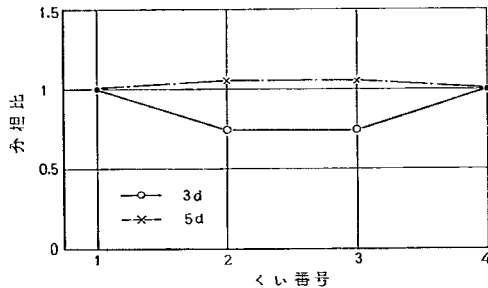
図-4.54 行構成の荷重分担割合 (砂地盤, 4本1行)
